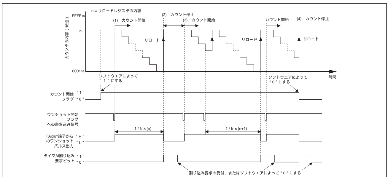
図1 ワンショットタイマモード動作タイミング
