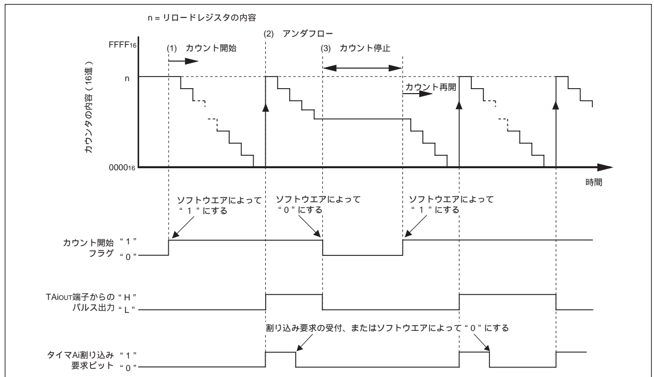
図1 タイマモード、ゲート機能選択時の動作タイミング
