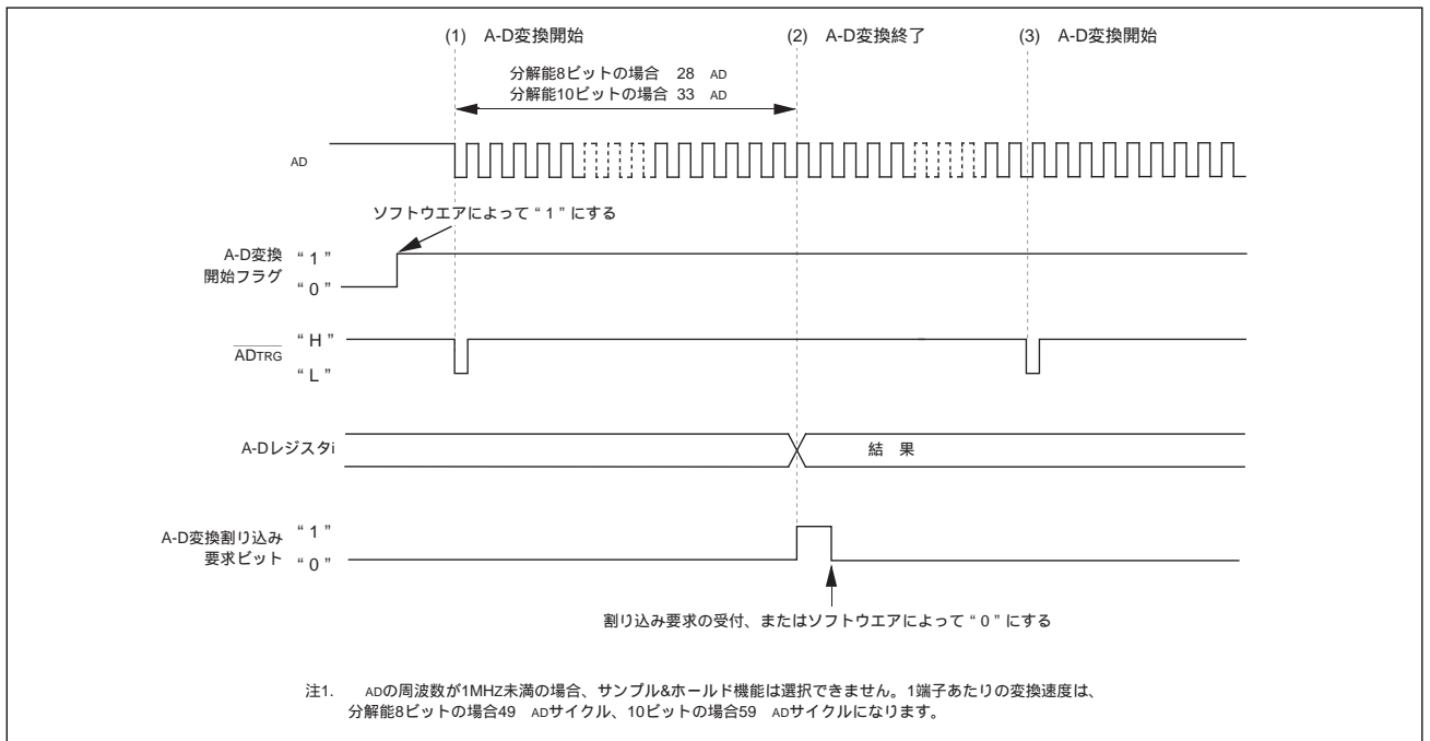
図1 単発モード、外部トリガ選択時の動作タイミング
