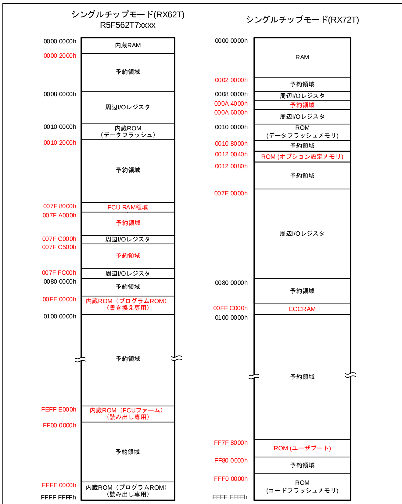
図 2.2 シングルチップモードのメモリマップ比較(RX62T : R5F562T7xxxx)
