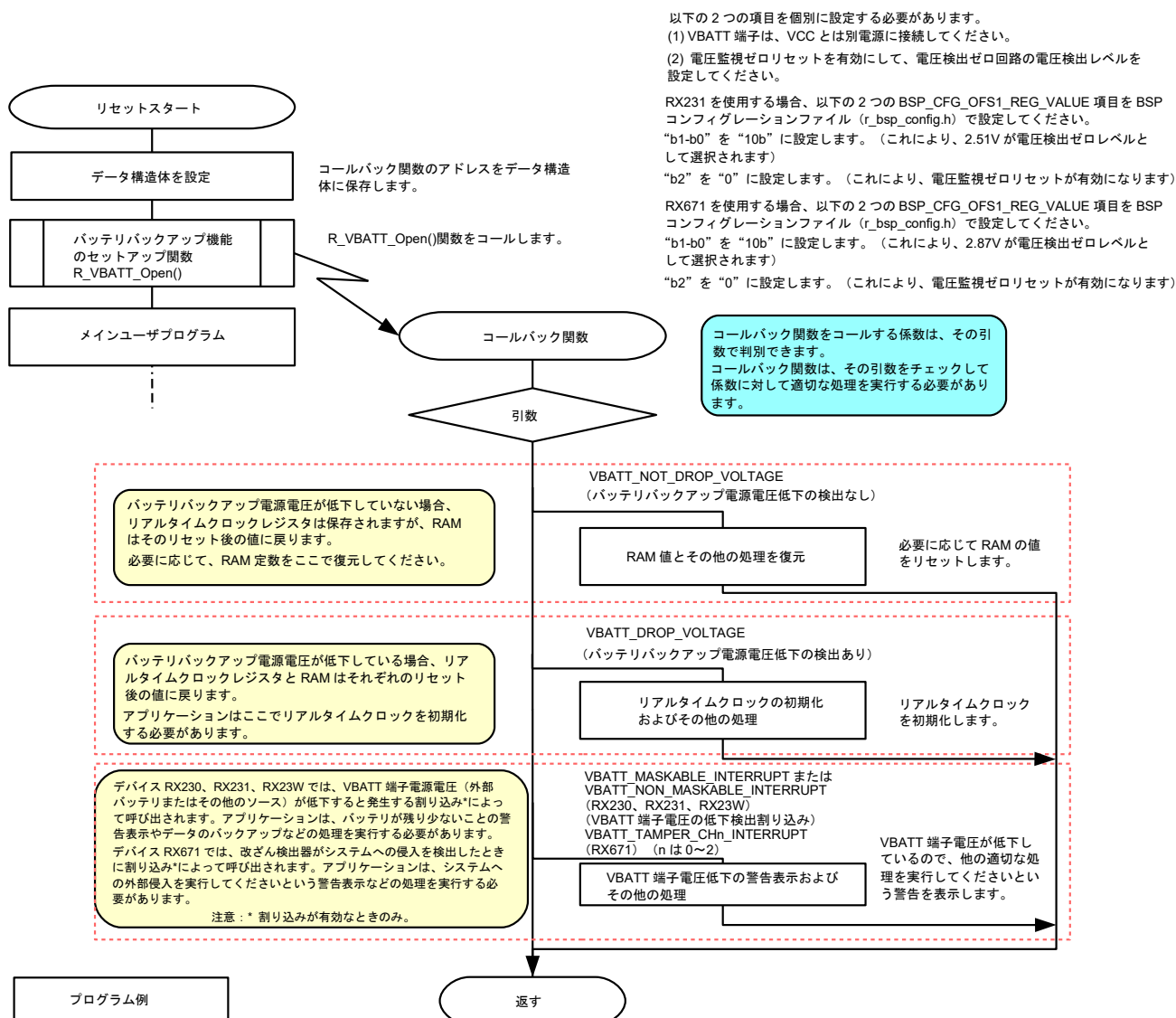
図1.6 バッテリーバックアップ機能 FIT モジュールの使用例
