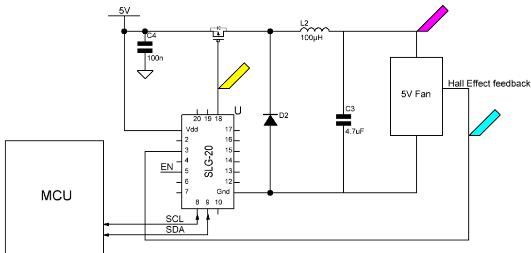
Figure 12. PWM Fan circuit
