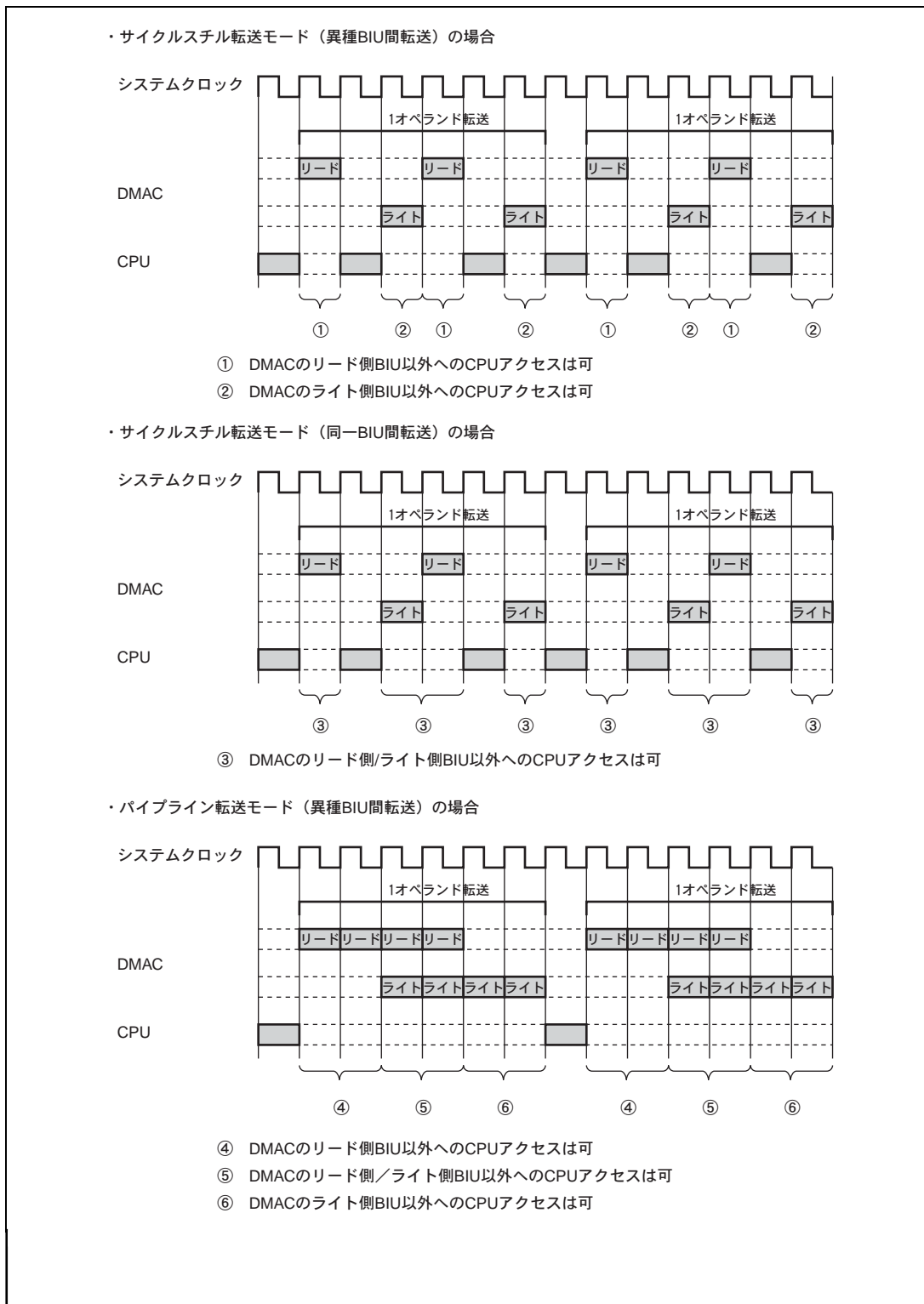
図 11.2 DMA 転送モードと DMAC/CPU のバス権の状態例
