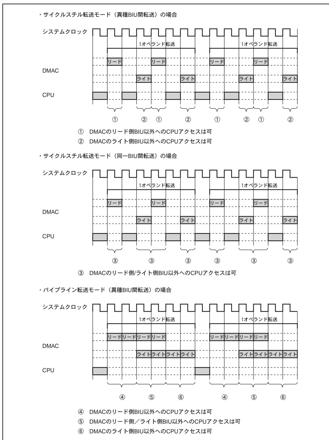
図 11.2 DMA 転送モードと DMAC/CPU のバス権の状態例
