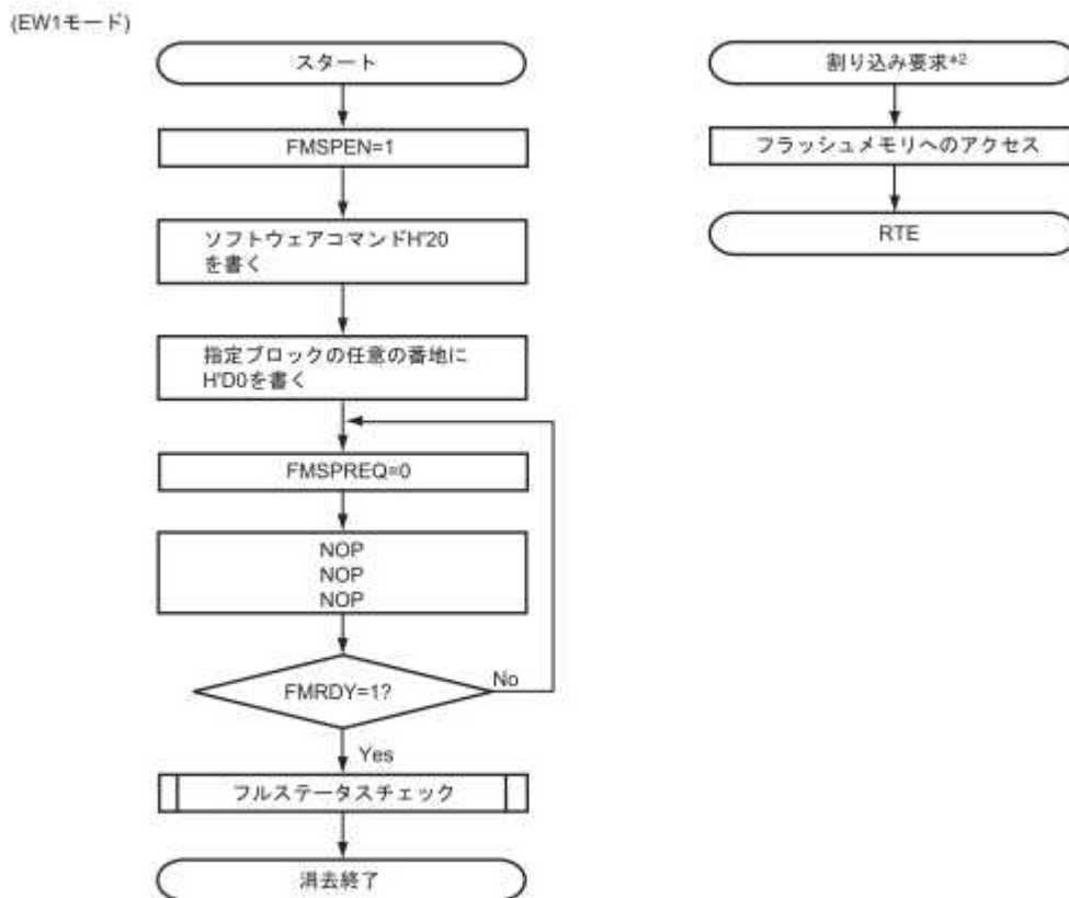
図 7.15 イレースサスペンド機能使用時のフロー EW1モード
