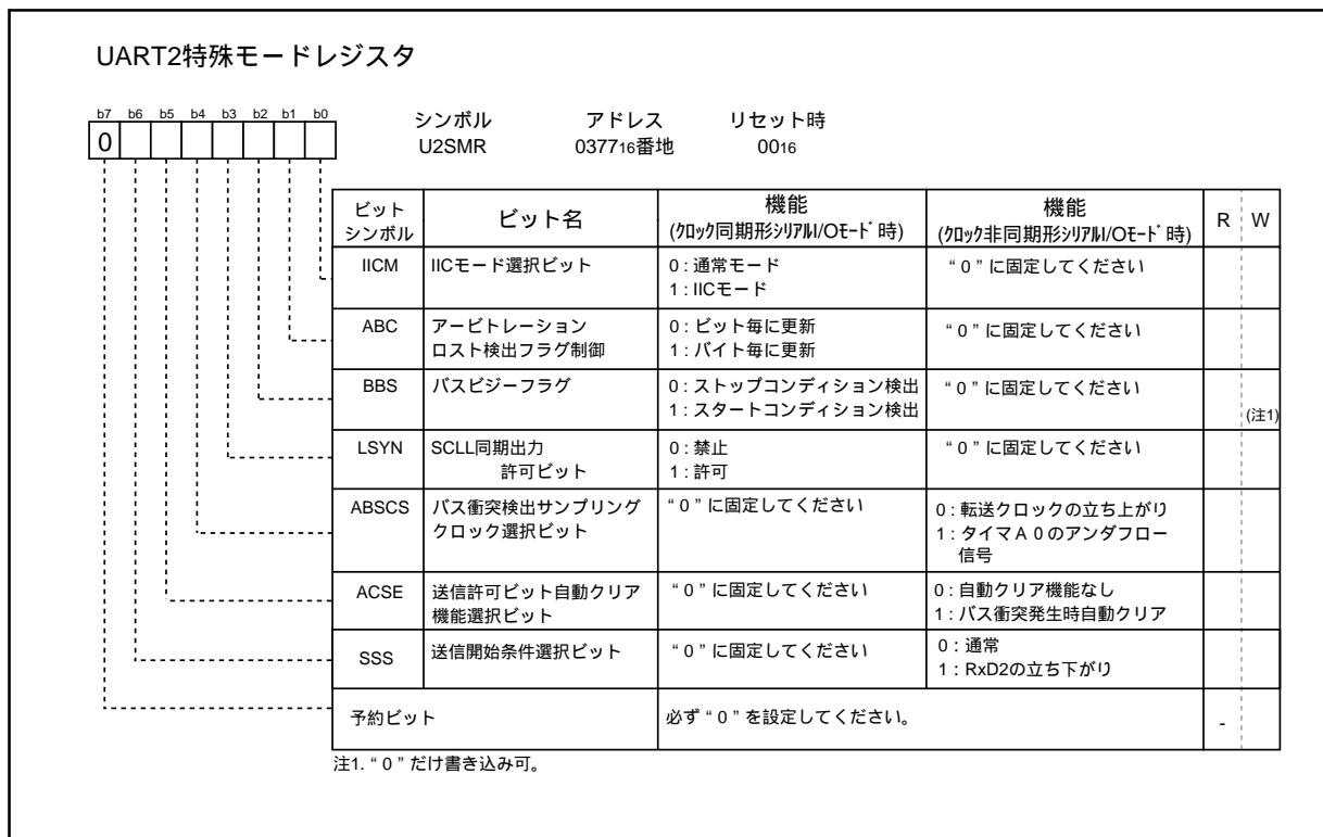
図 1. UART2 特殊モードレジスタの構成
