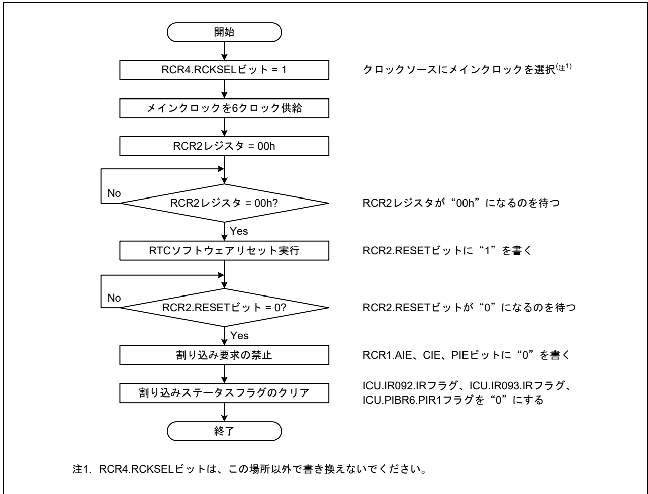
図 31.14 初期化手順 (メインクロック使用時)
