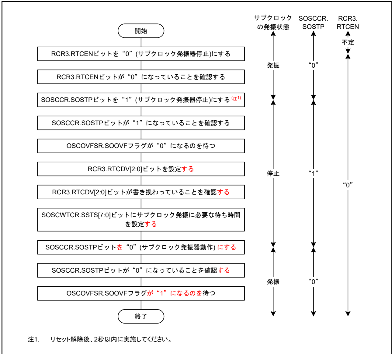
図 9.14 サブクロックを RTC のクロックソースに使用しない場合の初期化フローチャート例
