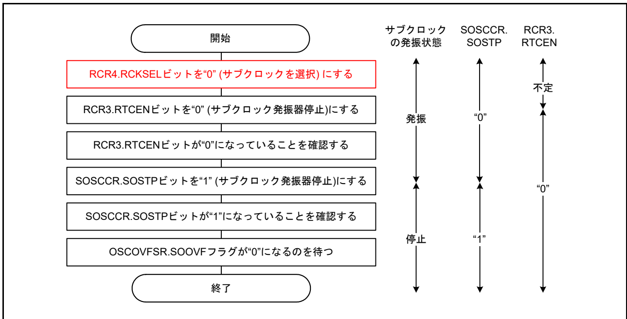
図 9.15 サブクロックを使用しない場合のフローチャート例
