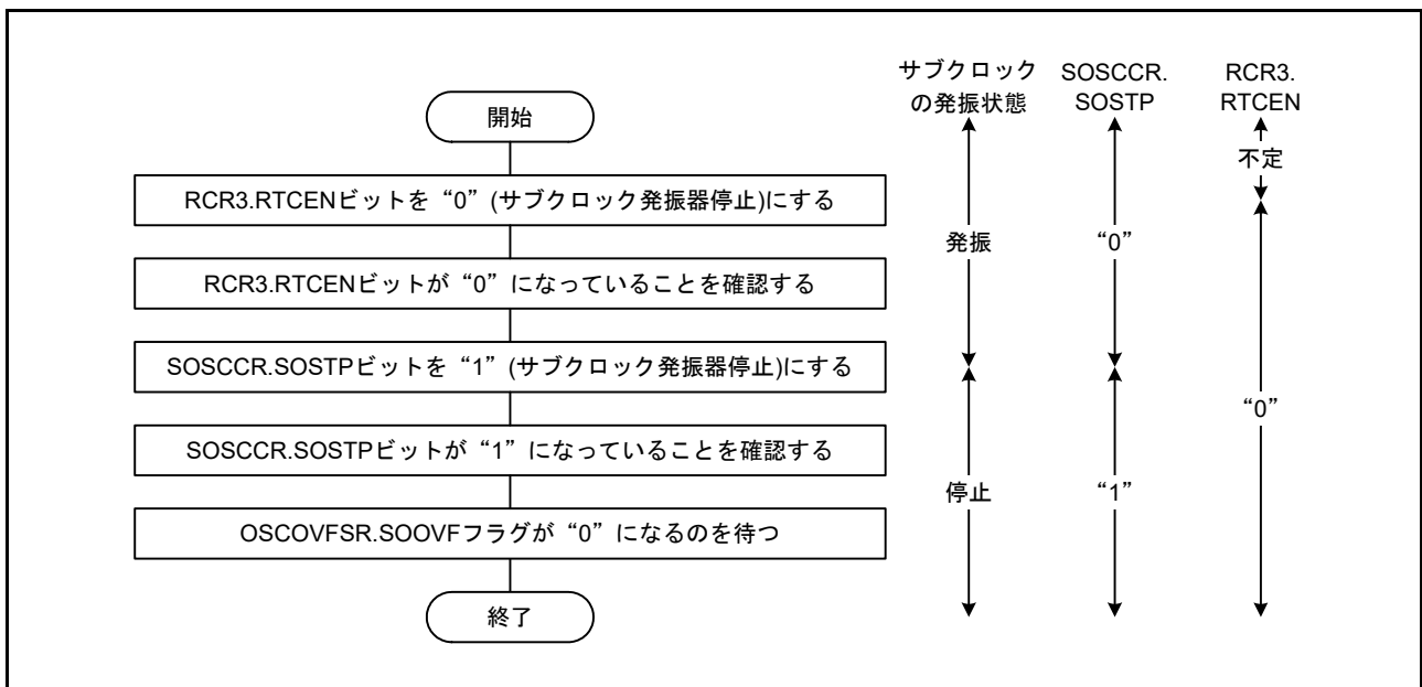
図 9.15 サブクロックを使用しない場合のフローチャート例
