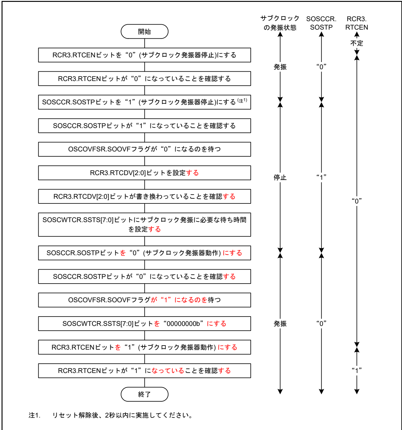
図 9.13 サブクロックを RTC のクロックソースに使用する場合の初期化フローチャート例
