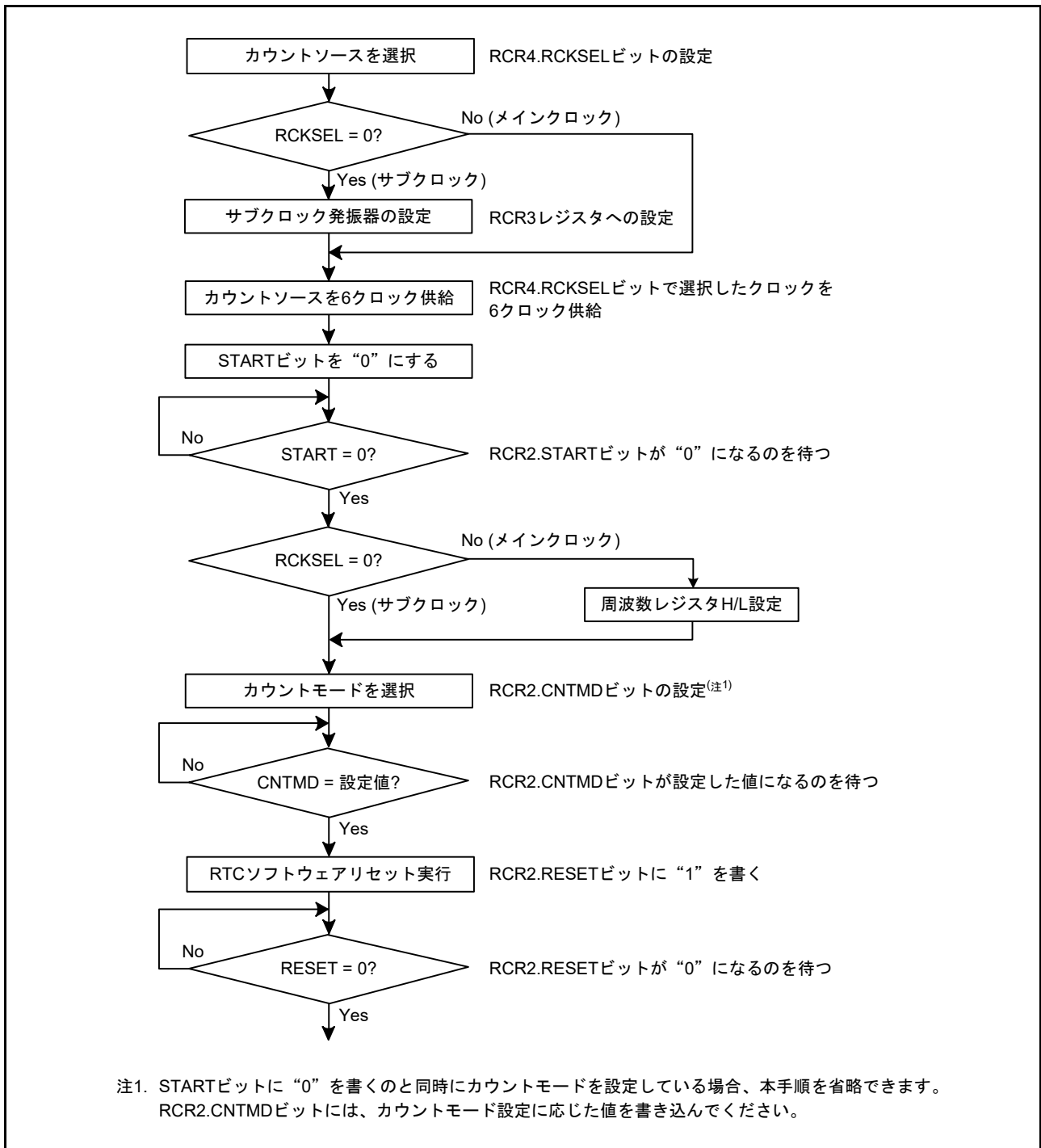
図 31.3 クロック設定手順
