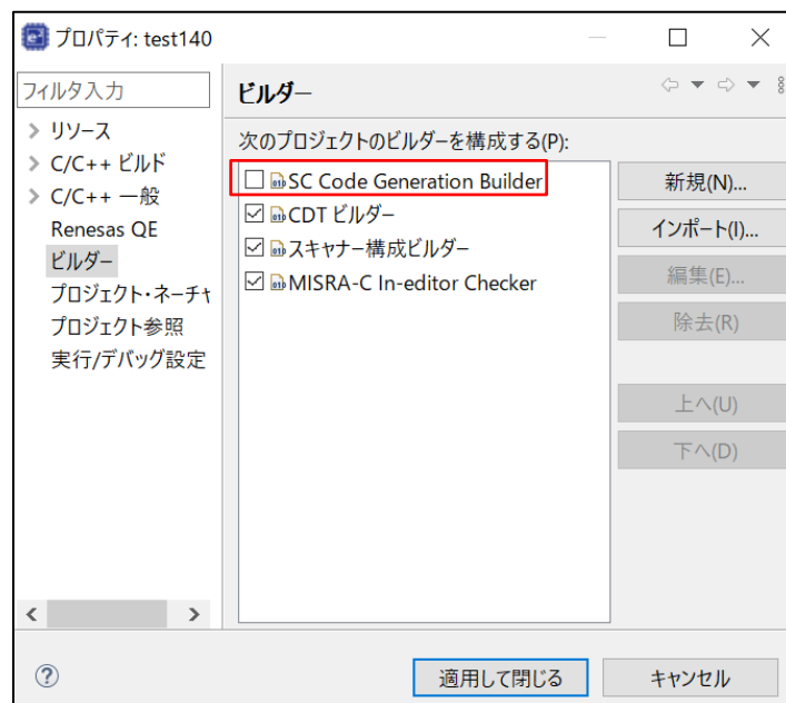
図 2-2 プロジェクトのプロパティの「SC Code Generation Builder」設定
