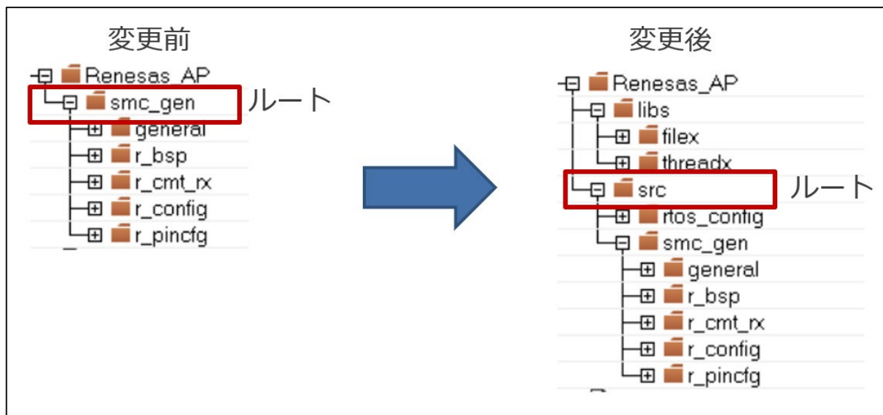
図 3-2 IAR IPCF ファイル構造の変更
