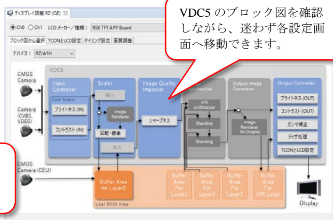
図 3 : ブロック図表示画面
