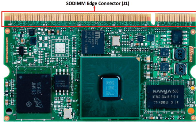
Top View of RZ/G1E SODIMM SOM
