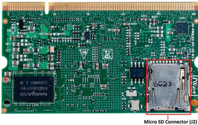
Bottom View of RZ/G1E SODIMM SOM
