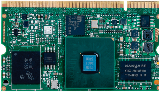
RZ/G1E SODIMM SOM
