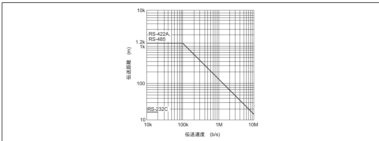
図 1 伝送距離と伝送速度の関係
