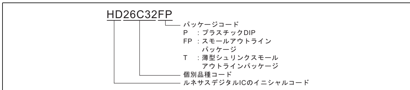
図1 パッケージ呼称
