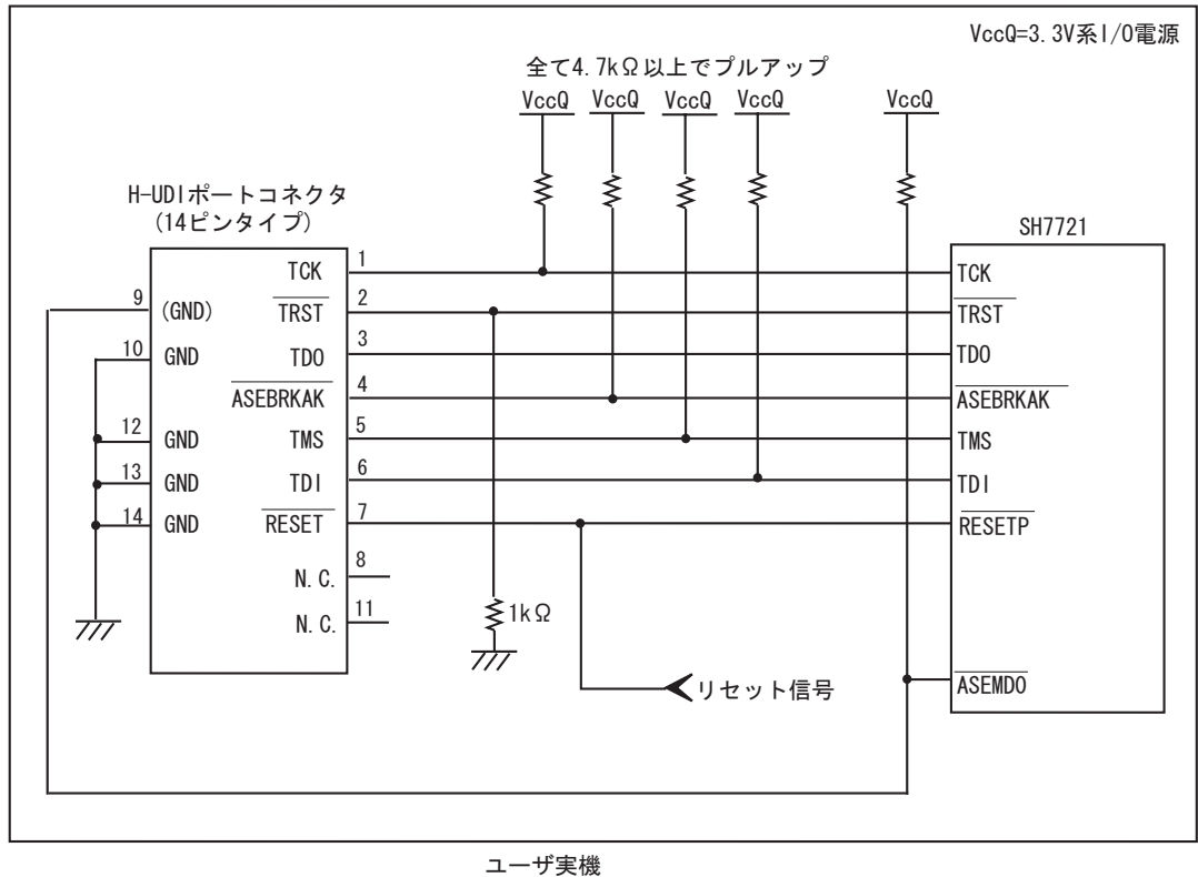
図 1.6 E10A-USB 使用時の H-UDI ポートコネクタ - チップ間の接続例 (14 ピンタイプ UVCC 未接続時 [注1] )
