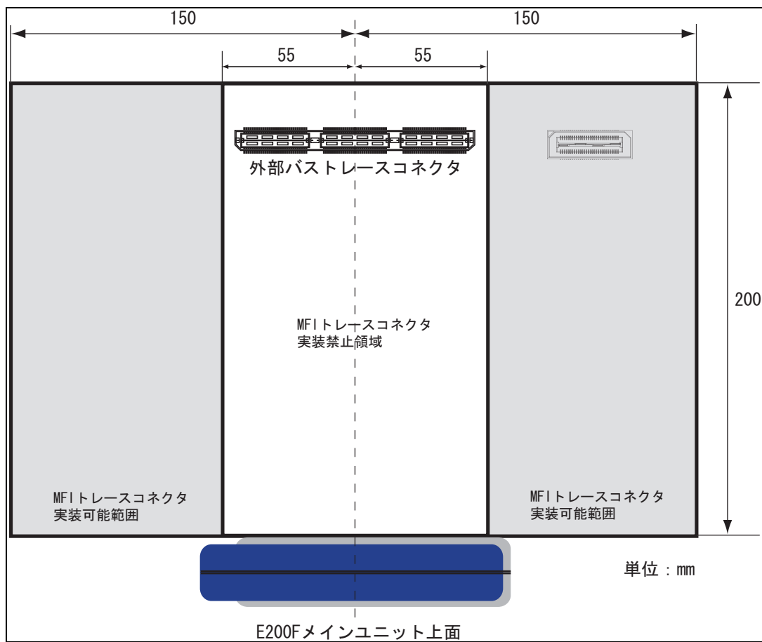
図 3.7 MFI トレースコネクタの実装位置 (トレースユニットを使用する場合)
