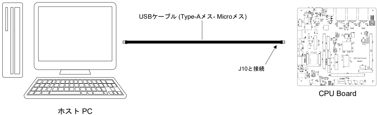
図 4-3: デバッグ環境の接続関係(J-Link® OB)
