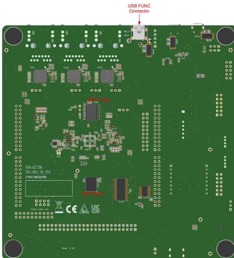
図 3-2: ボードレイアウト(ハンダ面)
