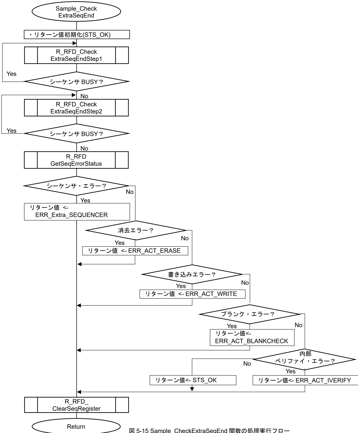
図 5-15 Sample_CheckExtraSeqEnd 関数の処理実行フロー
