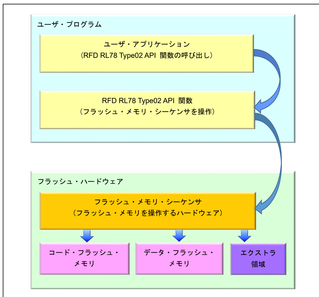
図 1-1 RFD RL78 Type02 の API 関数を使ったフラッシュ・メモリの操作イメージ
