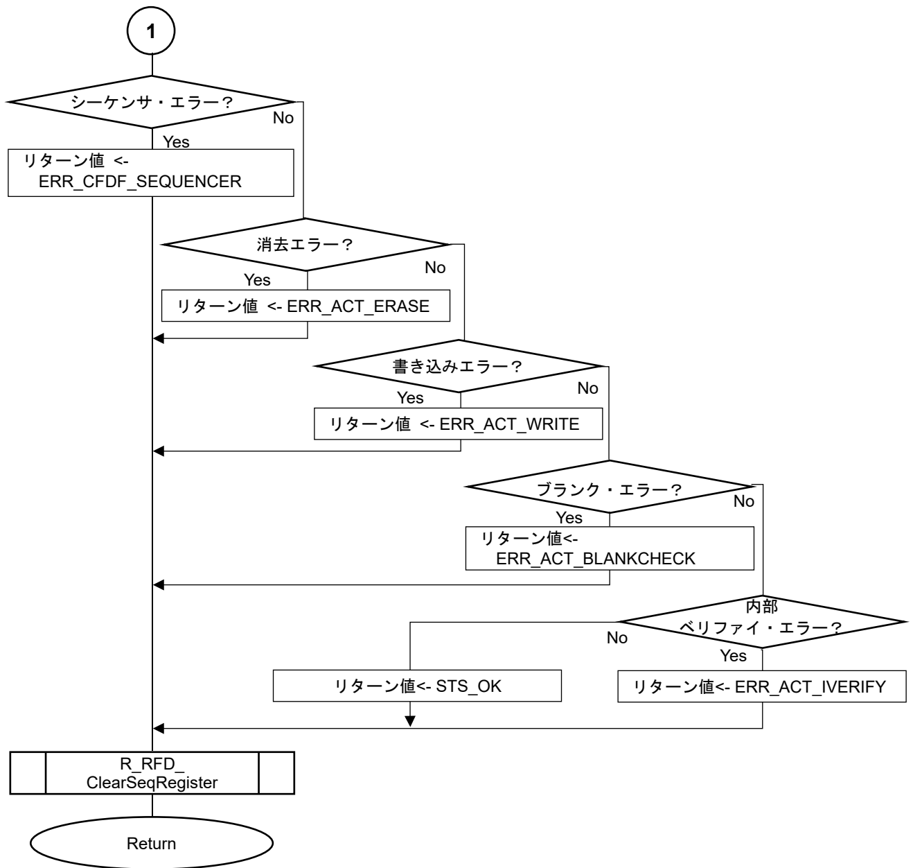
図 5-14 Sample_CheckCFDFSeqEnd 関数の処理実行フロー(2/2)
