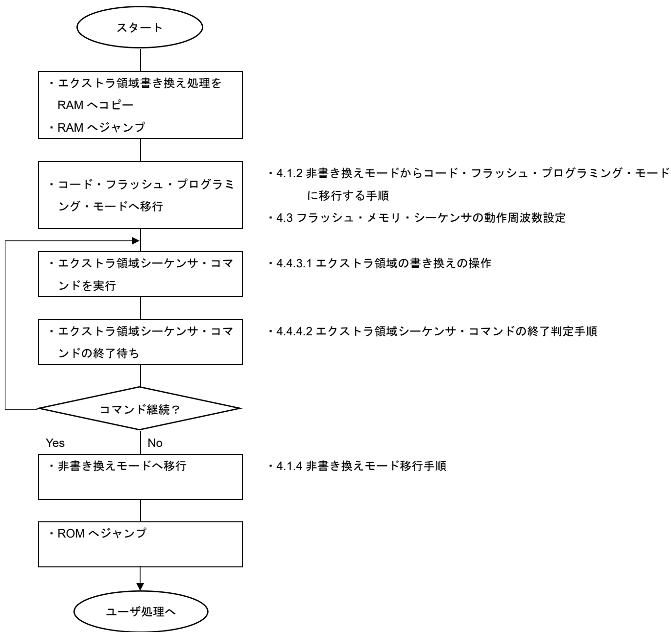
図 4-4 エクストラ領域書き換え時のコマンド実行フロー
