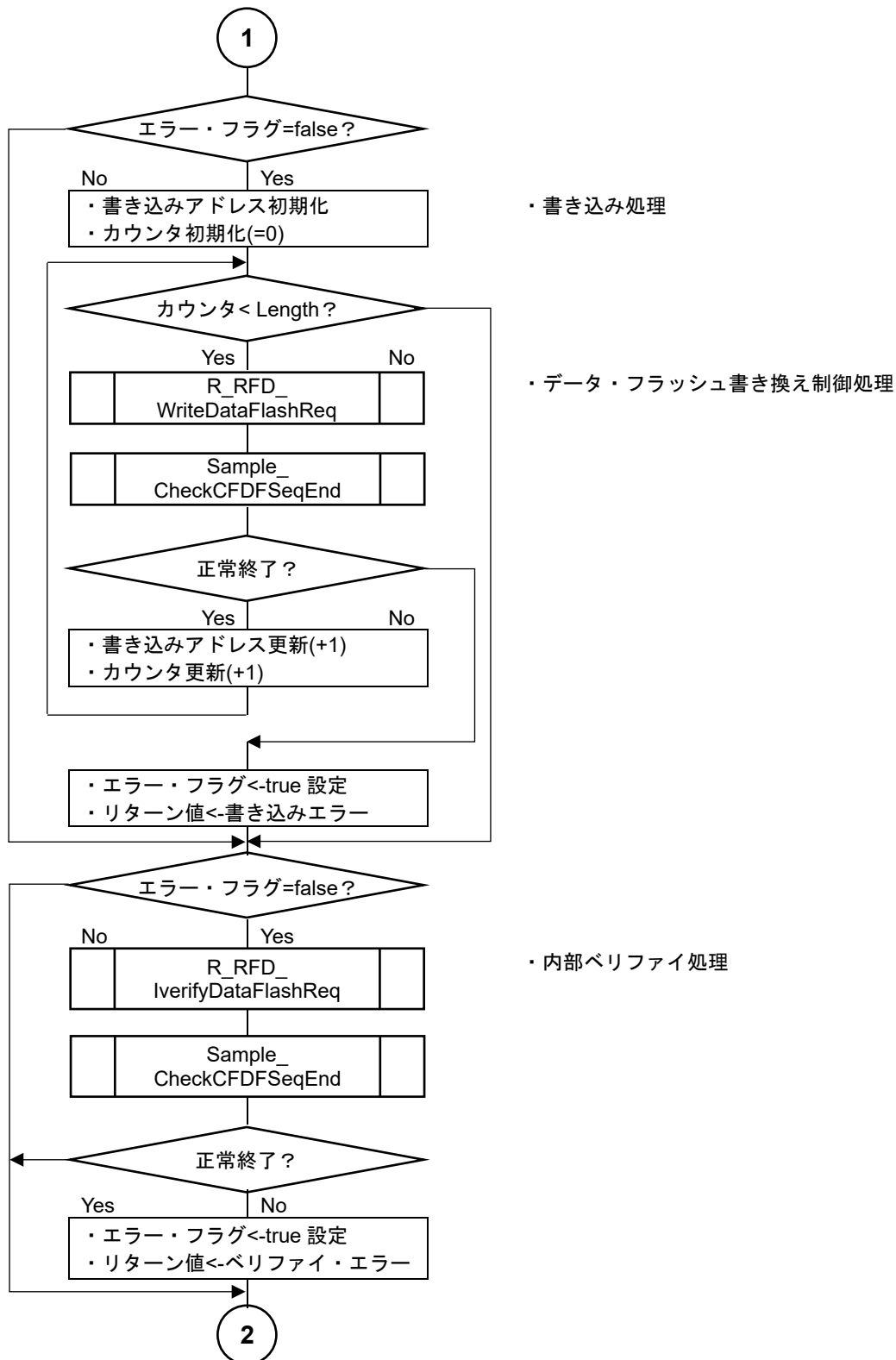
図 5-8 データ・フラッシュ書き換え制御サンプルの処理実行フロー(2/3)
