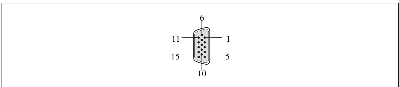
図10.11 ターゲットケーブル（14 ピンタイプ）D-sub 15 ピン（オス）のピン配置
