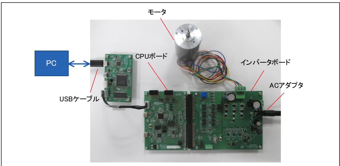
図 4-6 ハードウェア接続例(通信ボード使用)
