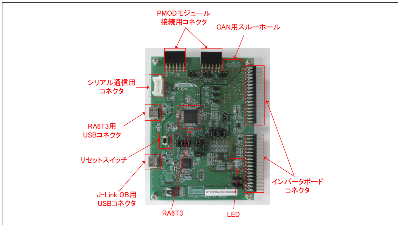
図 4-2 CPU ボードのレイアウト
