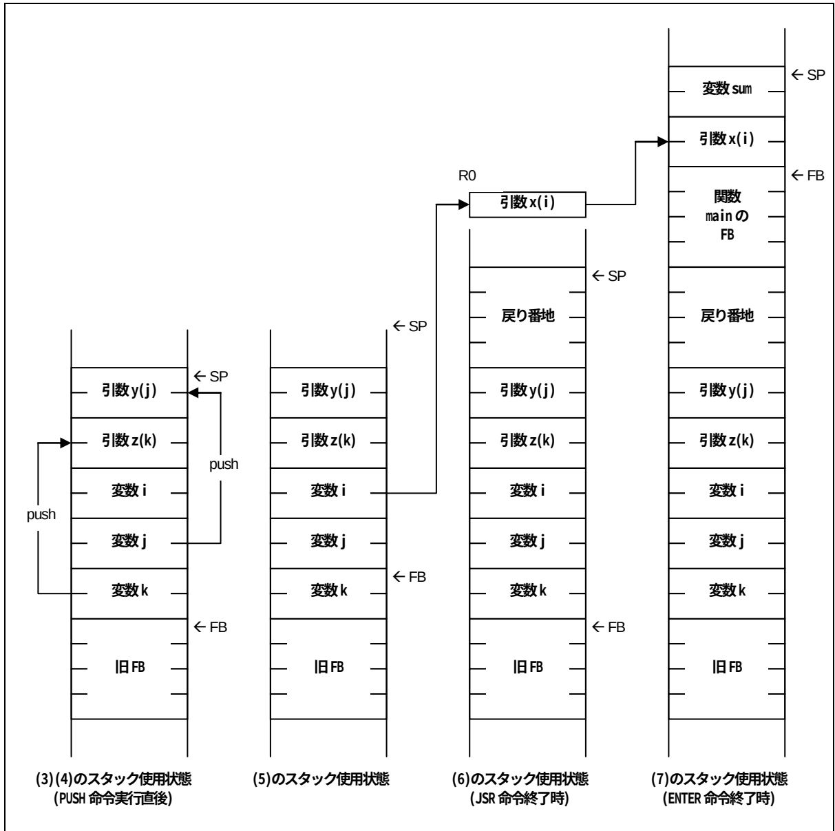
図D.18 関数 func の呼び出し及び、入入口処理
