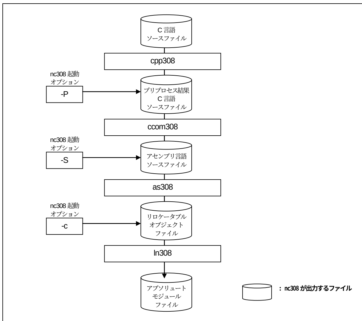
図1.6 nc308 起動オプションと出力ファイルの相互関係図
