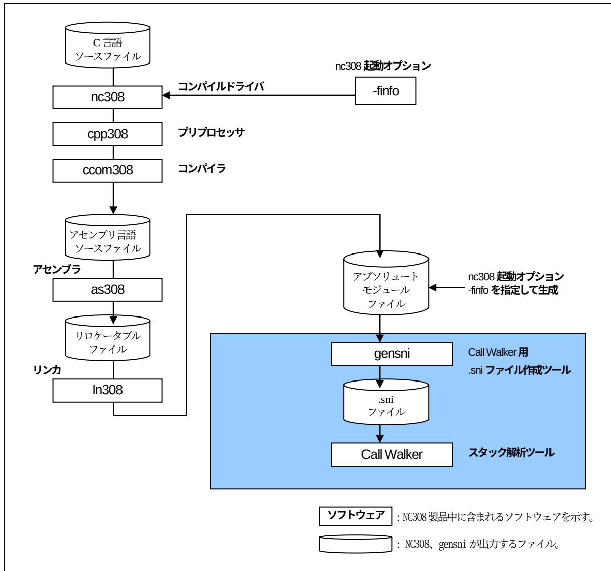
図H.1 NC308 の処理フロー
