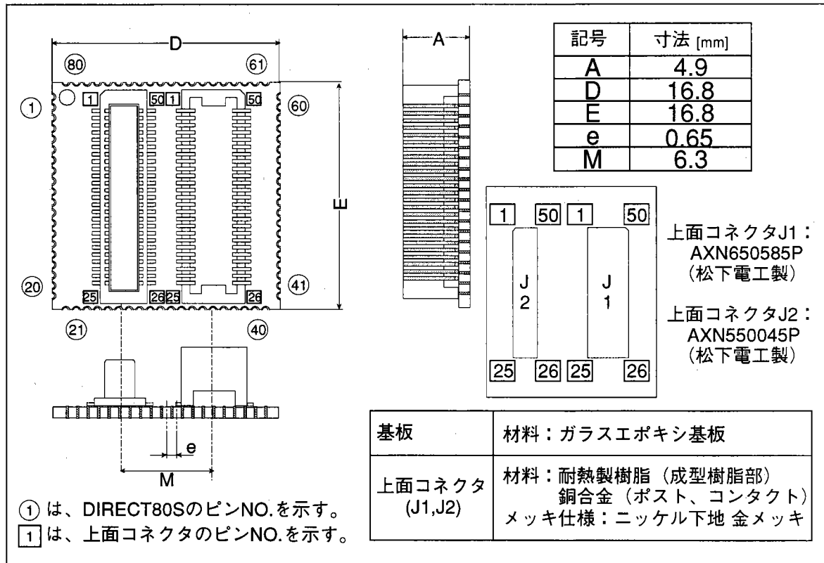
図4 DIRECT80Sの寸法
