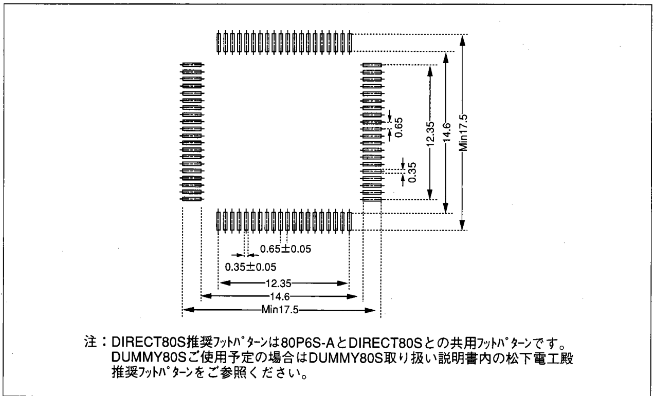
図3 DIRECT80S推奨フットパターン寸法
