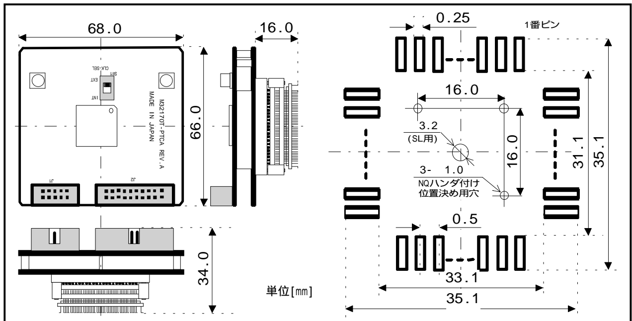
図4 M32170T-PTC の寸法図及び参考フットパターン
