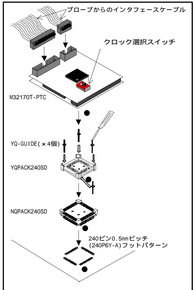
図3 M32170T-PTC 装着手順
