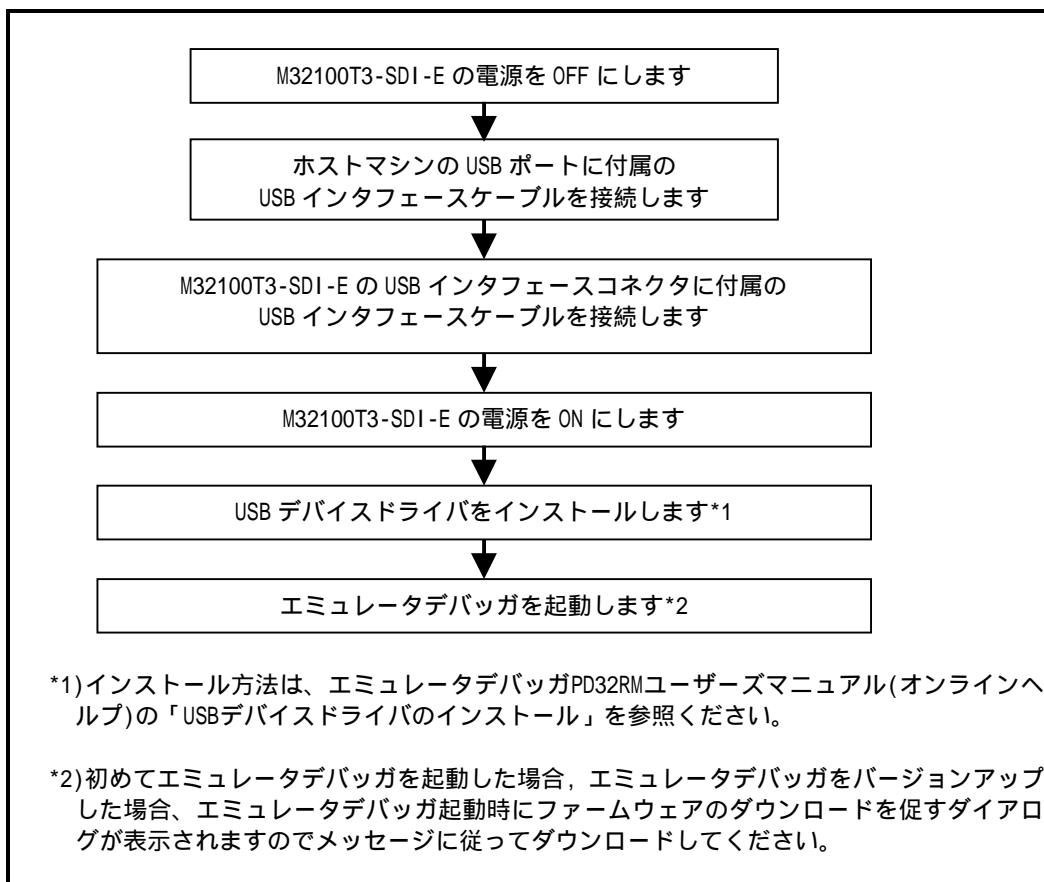
図 3.3 USB インターフェースの接続手順
