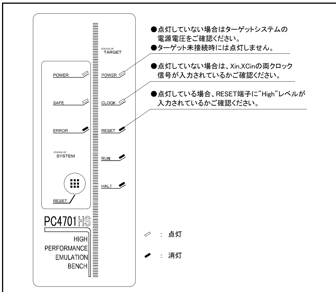
図 4.1 電源投入時の PC4701 の LED 表示
