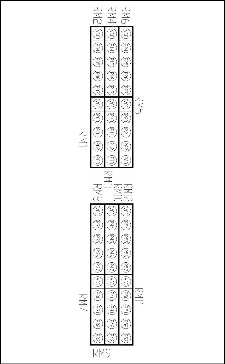
図 3.3 プルアップ抵抗取り付け位置
