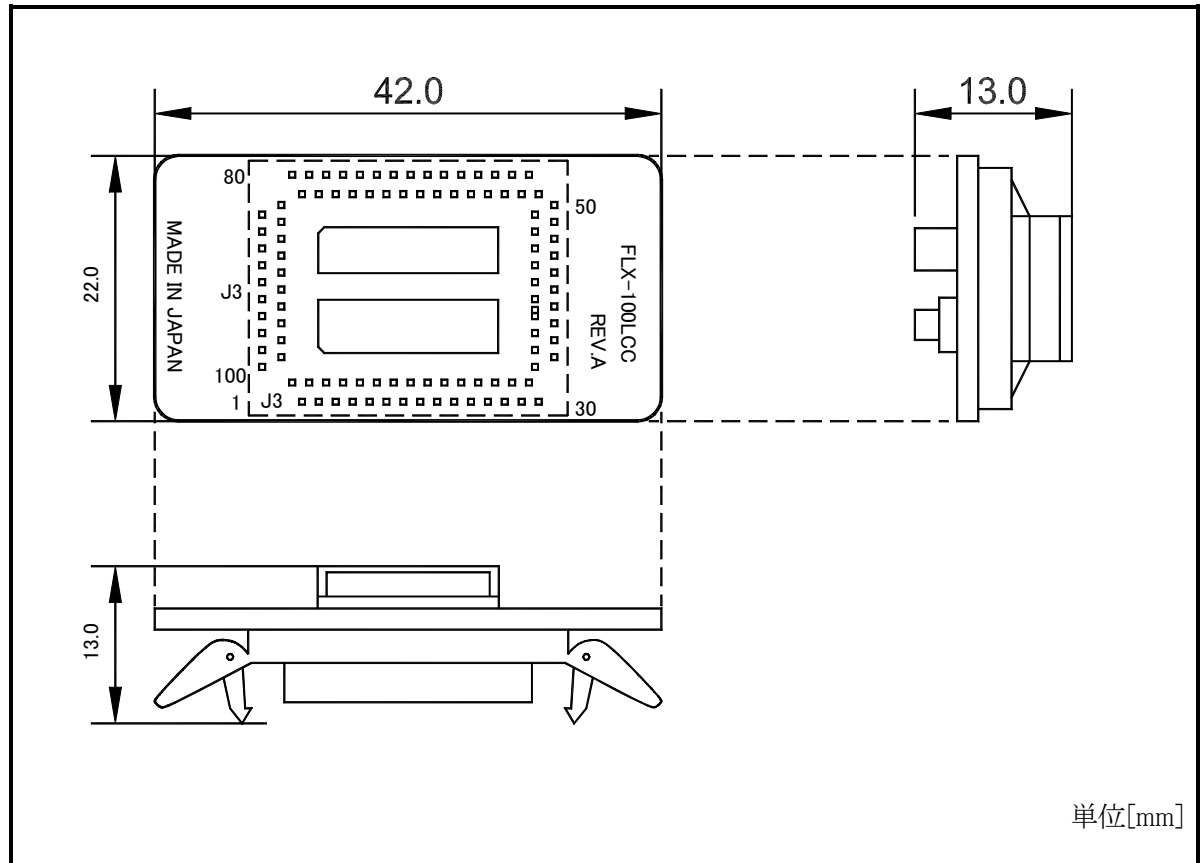
図 5.8 変換基板(FLX-100LCC)寸法図
