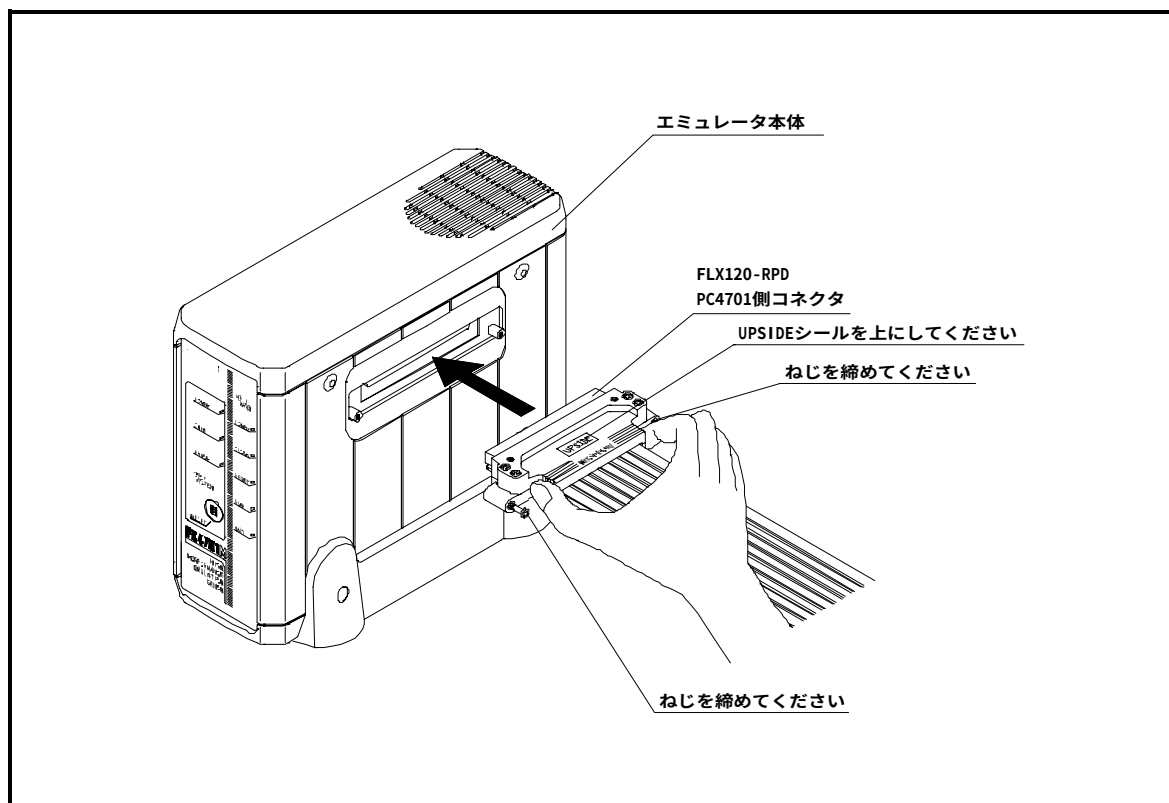
図 3.9 PC4701 とケーブル接続
