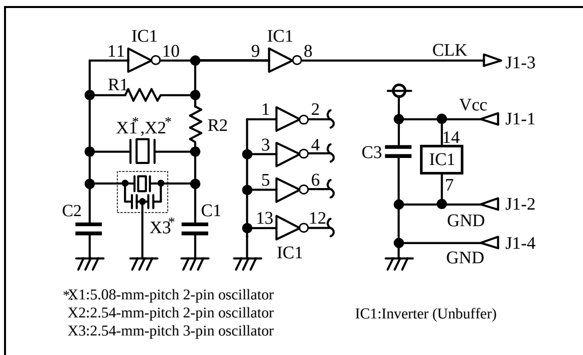
図 3.7 発振回路基板(OSC-2)回路
