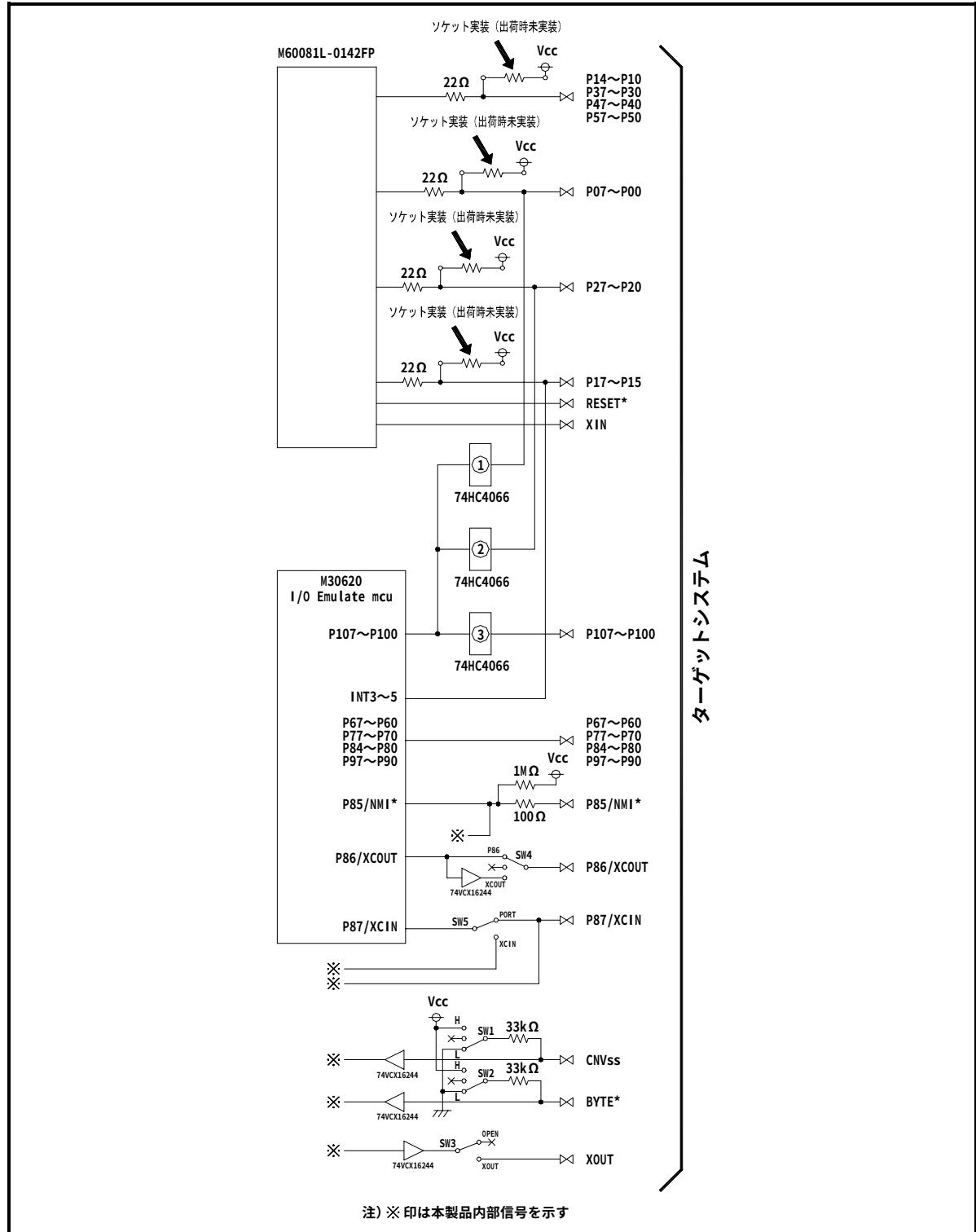
図 5.6 接続図
