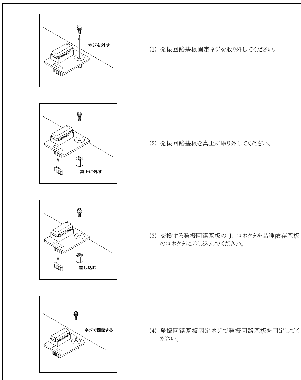
図 3.8 発振回路基板の交換方法
