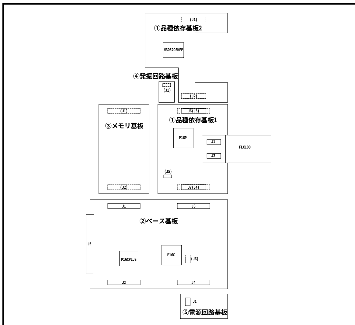
図 2.2 エミュレーションポッド内部基板構成
