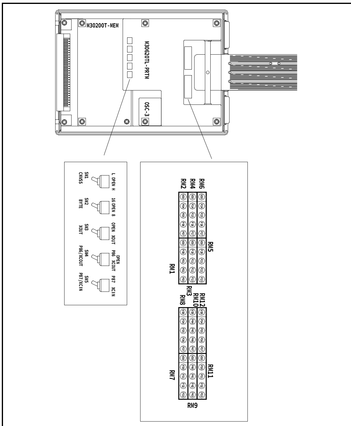
図 3.2 スイッチの位置と出荷時の設定
