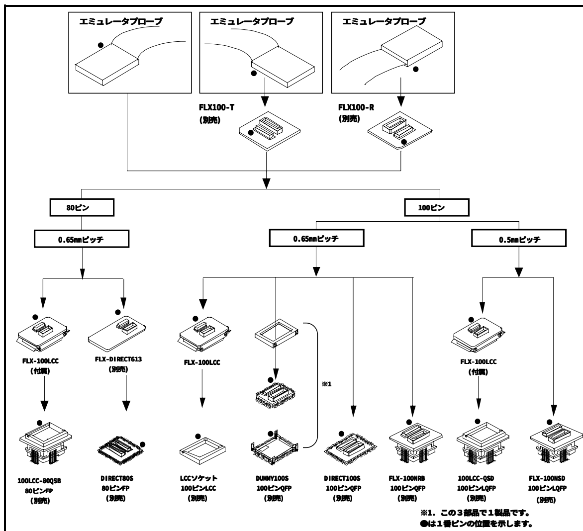
図 3.11 ターゲットシステムとの接続
