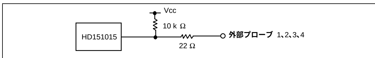
図 2-8 外部プローブ 1 インタフェース回路
