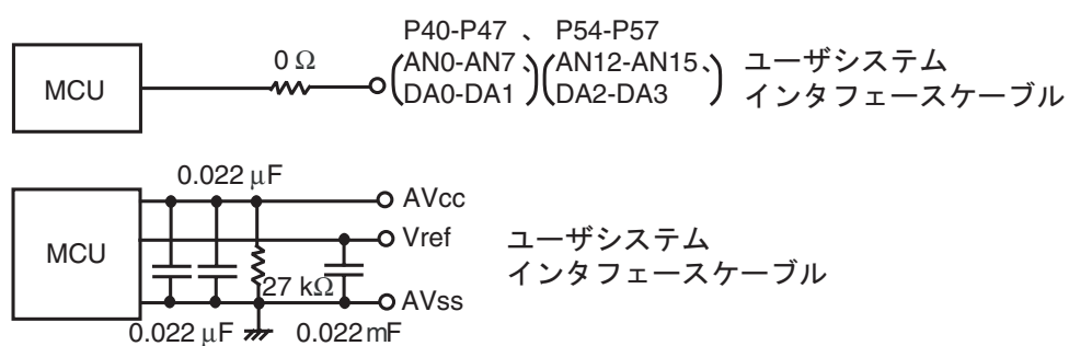
図 7-4 P40-P47、P54-P57、Vcc、AVcc、AVss、Vref 信号回路
