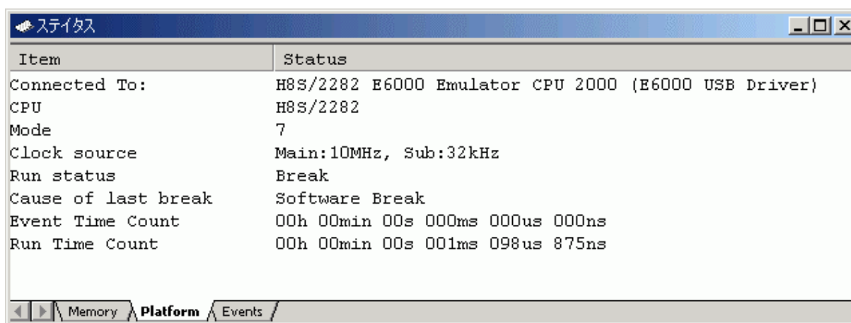
図 6-34 [ステイタス]ウィンドウの表示内容 (ソフトウェアブレーク)
