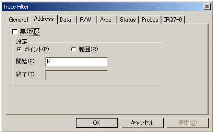
図 5-47 Trace Filter ダイアログボックス(Address ページ)
