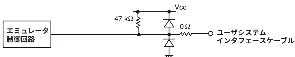
図 7-3 RESET 信号回路
