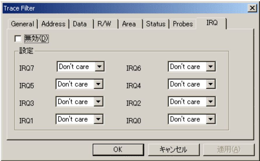
図 8-4 Trace Filter ダイアログボックス(IRQ ページ)
