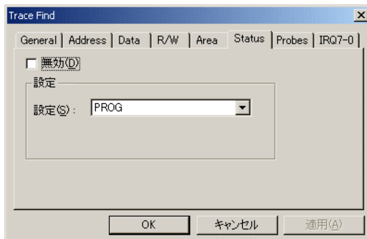
図 5-42 Trace Find ダイアログボックス(Status ページ)
