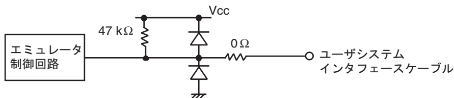
図 7-2 モード端子, NMI, WAIT 信号回路
