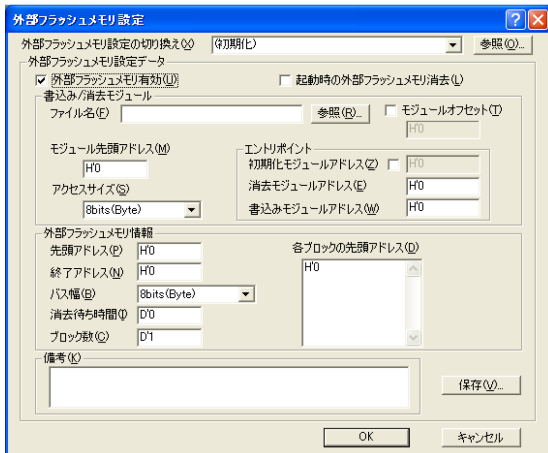
図 2.3 [外部フラッシュメモリ設定]ダイアログボックス
