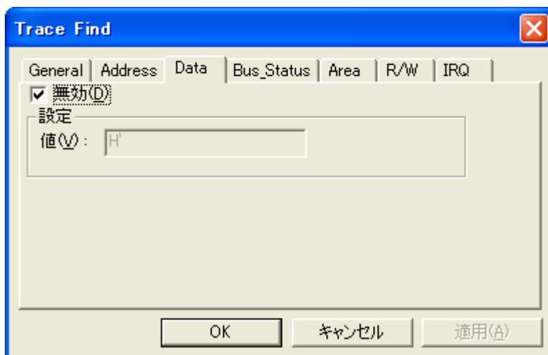
図 2.13 [Data]ページ
