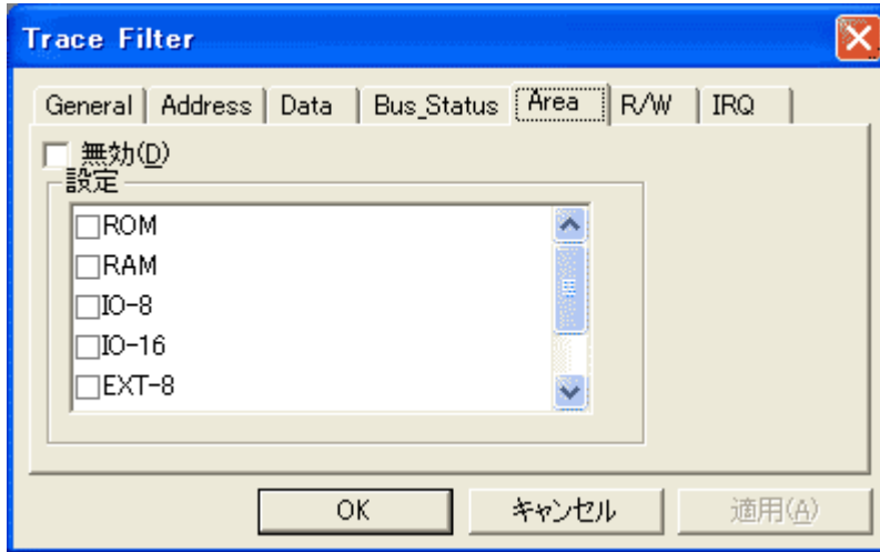
図 2.8 [Area]ページ
