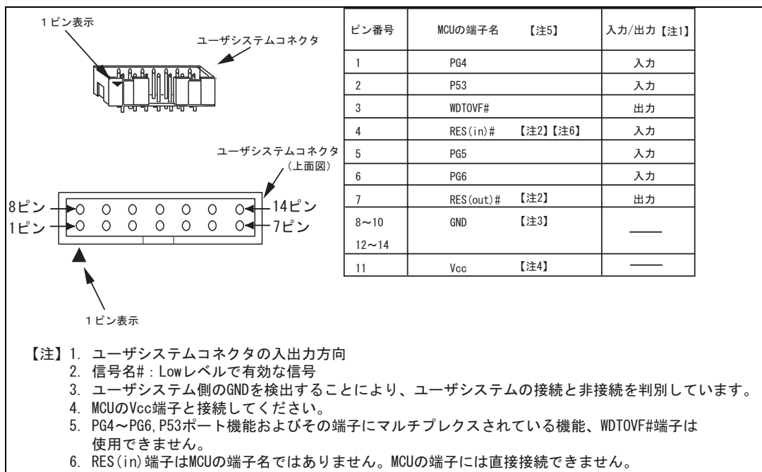
図 1.2 ユーザシステムコネクタのピン配置
