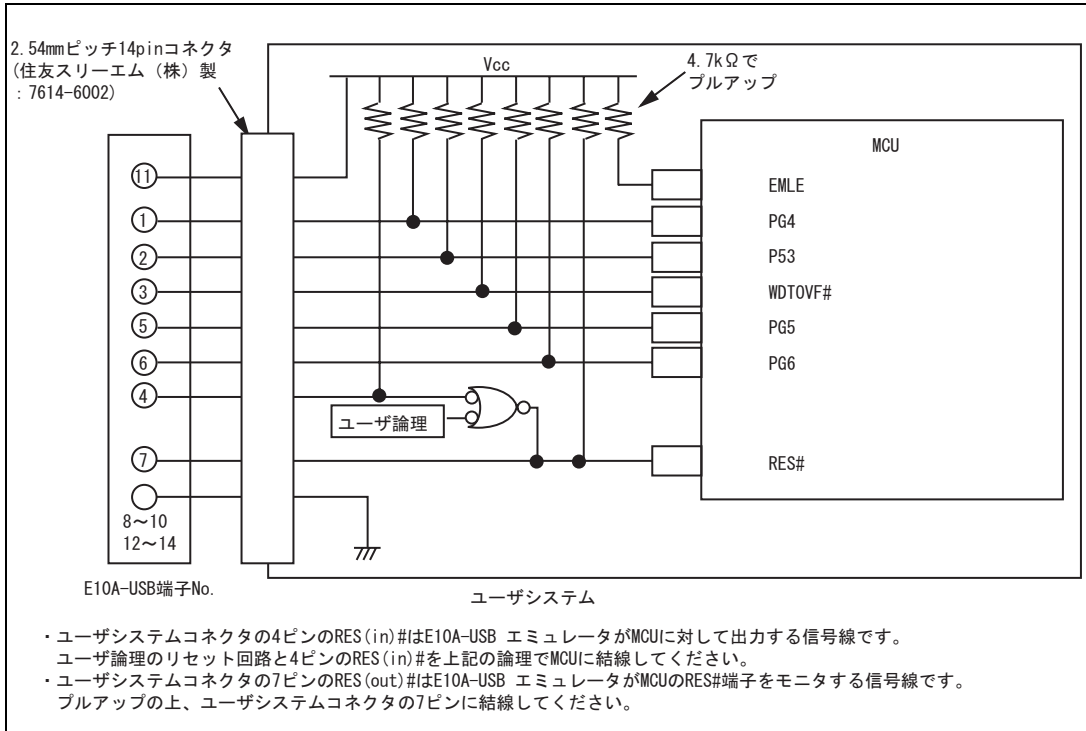
図 1.3 E10A-USB の接続例
