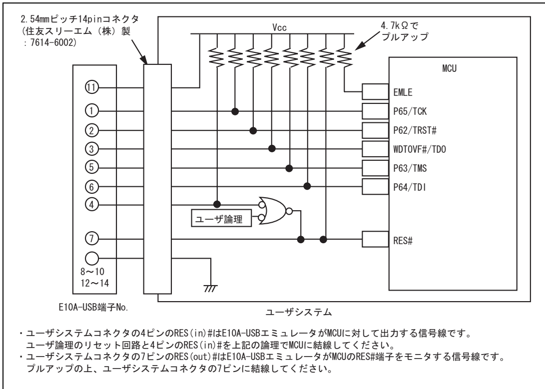
図 1.3 E10A-USB の接続例
