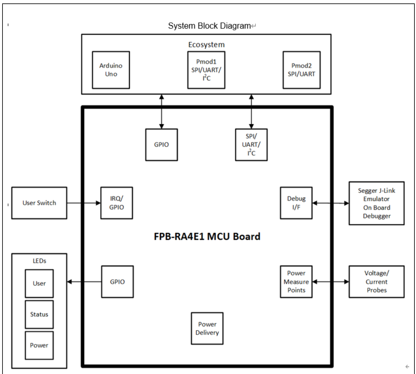
図 4 FPB-RA4E1 ボードブロック図
