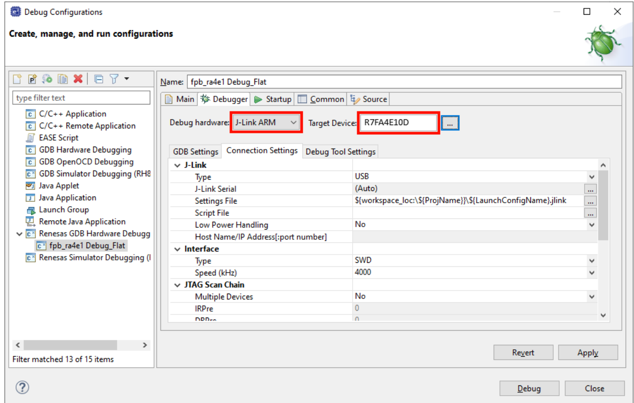
図 8 e 2 studio デバッグ設定
