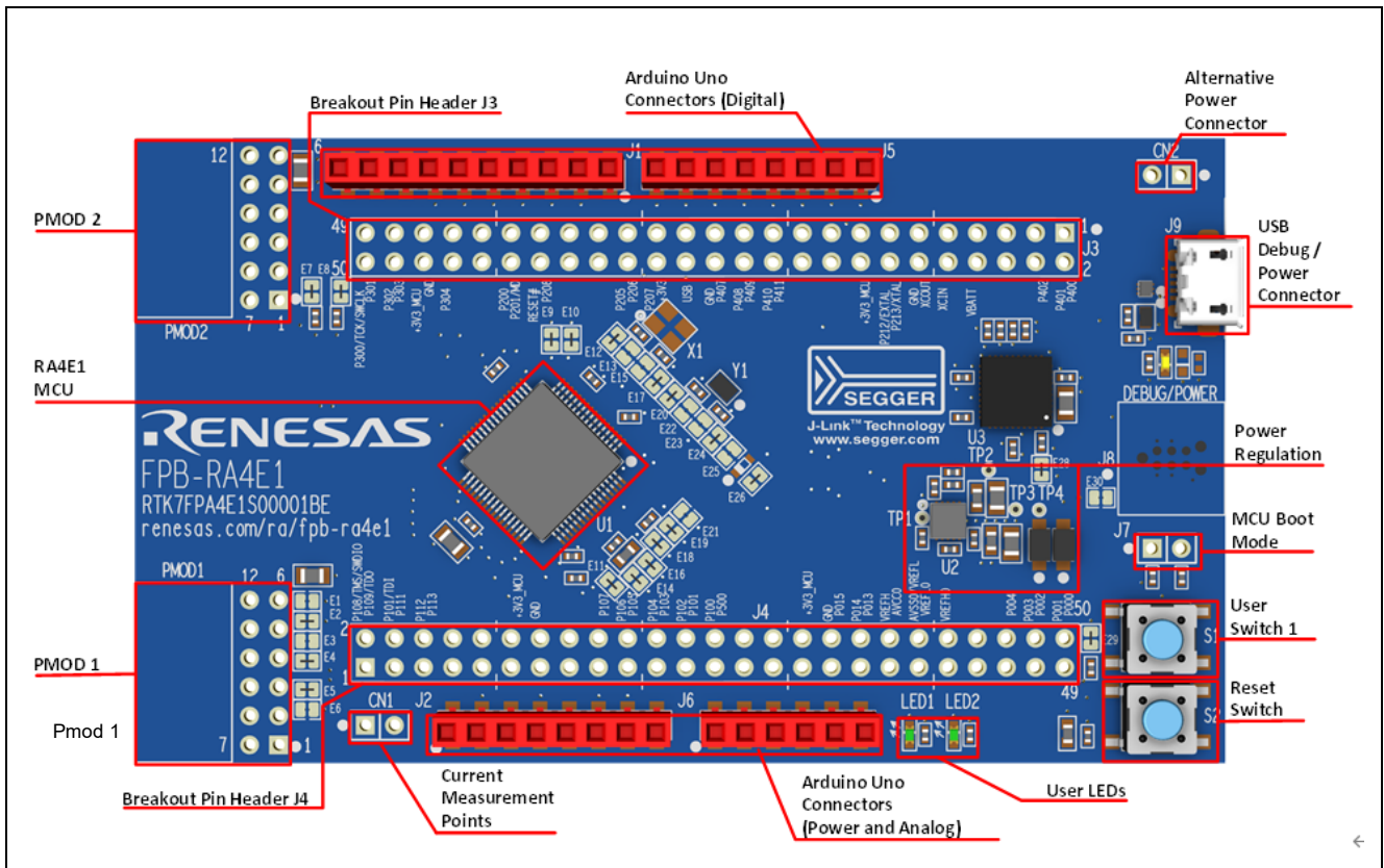
図 1 FPB-RA4E1 ボード (上面)
