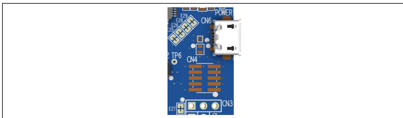
図 7 FPB-RA4E1 デバッグインタフェース
