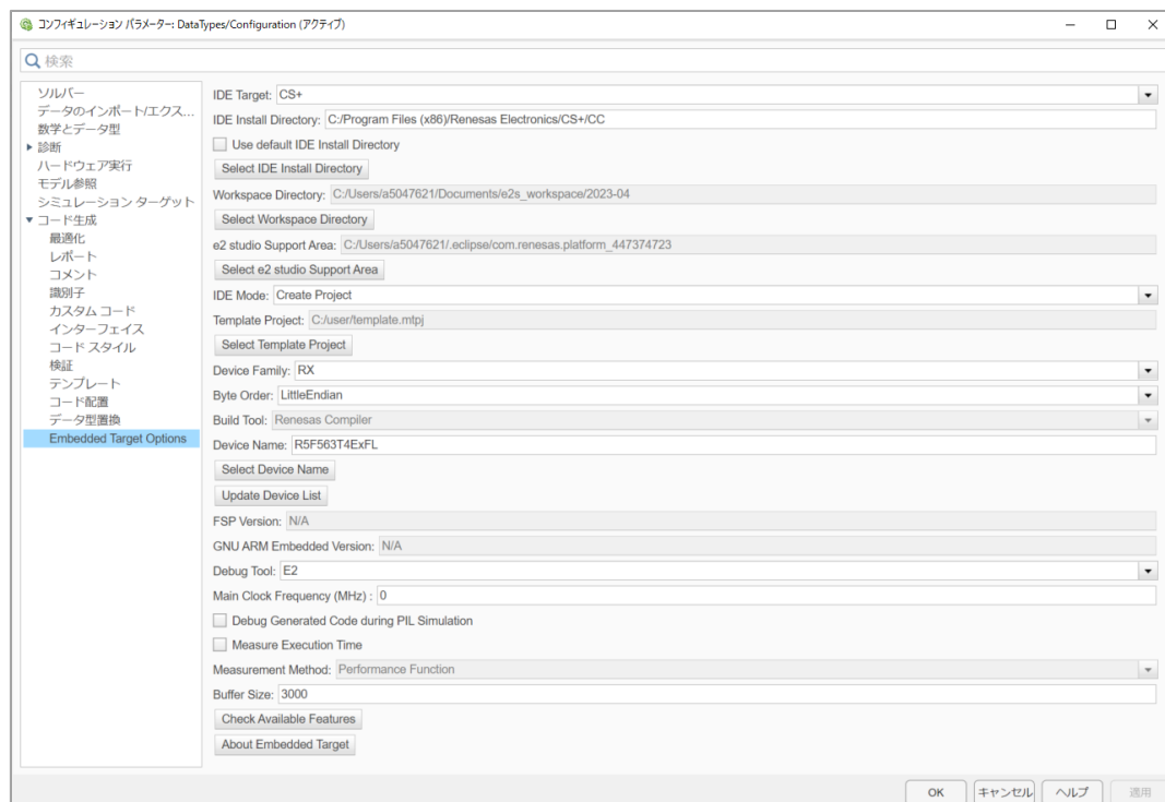
図 3-6 [Embedded Target Options]設定
