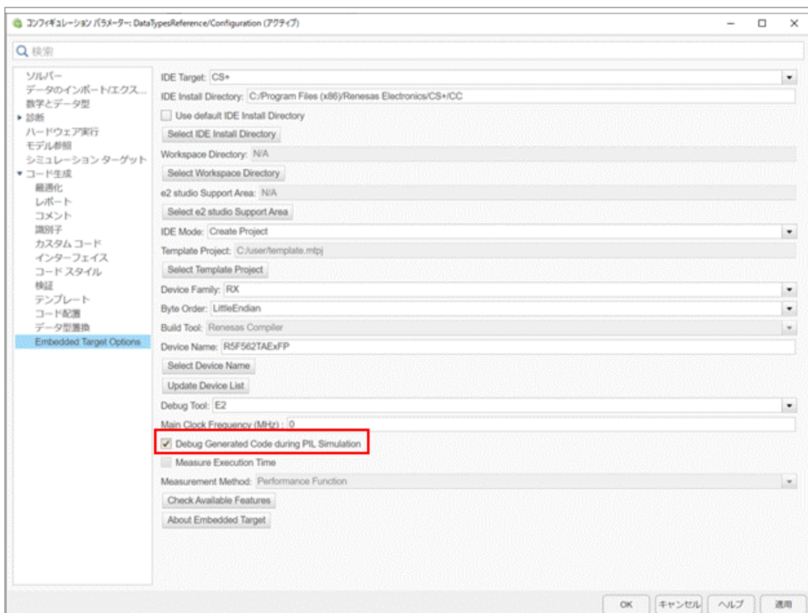
図 3-25 PILシミュレーション中の生成コードデバッグの有効化
