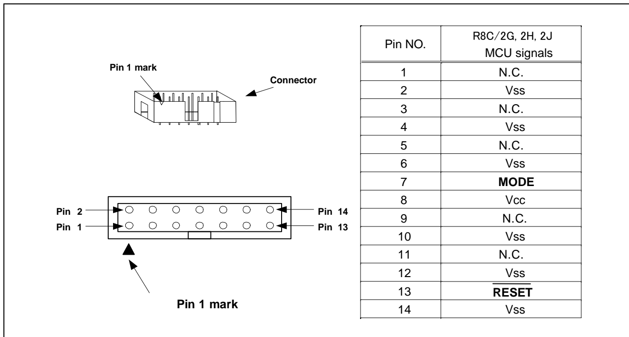
図 4.1 E8 接続コネクタのピン配置
