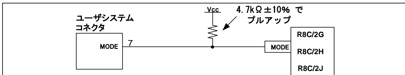
図 5.2 E8 エミュレータと MODE 端子の接続
