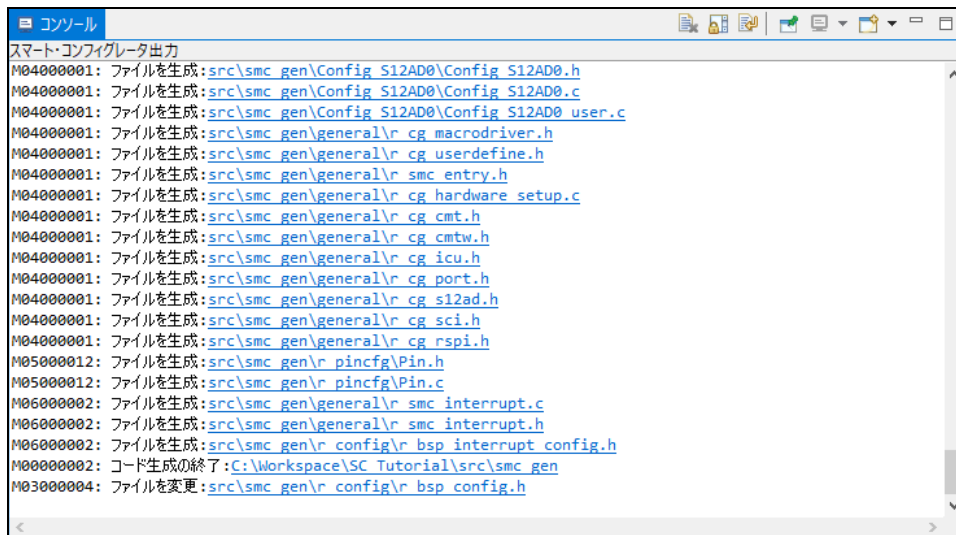
図 4-52 コード生成
