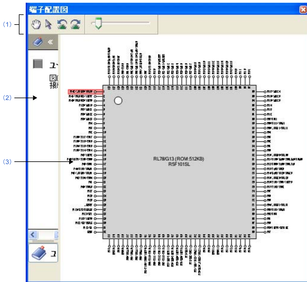
図 A—15 端子配置図 パネル
