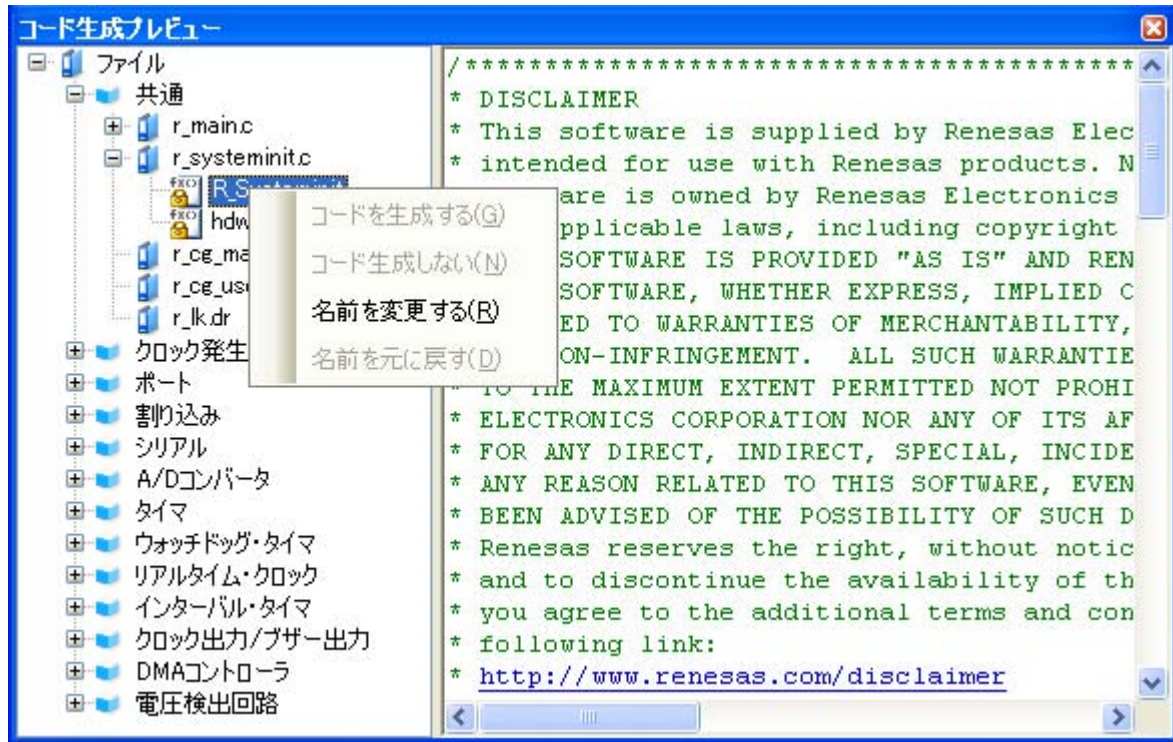
図 3—10 API 関数名の変更
