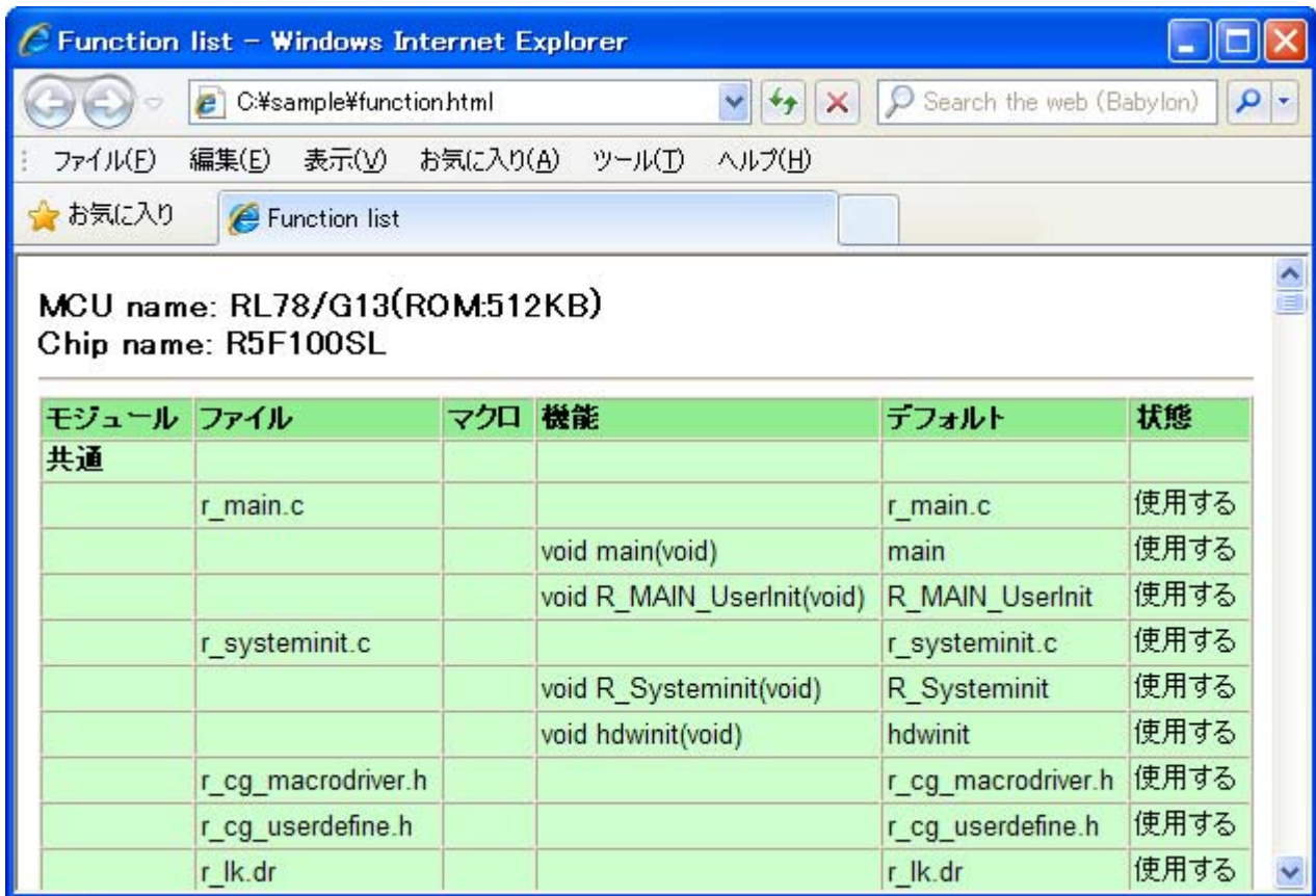
図 3—14 レポート・ファイル function の出力例
