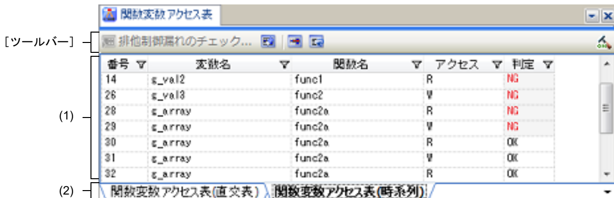
図 A.55 関数変数アクセス表 パネル : [関数変数アクセス表 (時系列)] タブ
