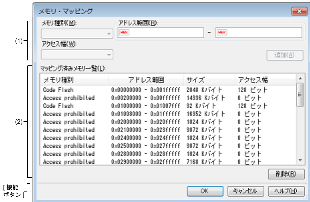
図 A.25 メモリ・マッピング ダイアログ 【Full-spec emulator】【E1】【E20】
