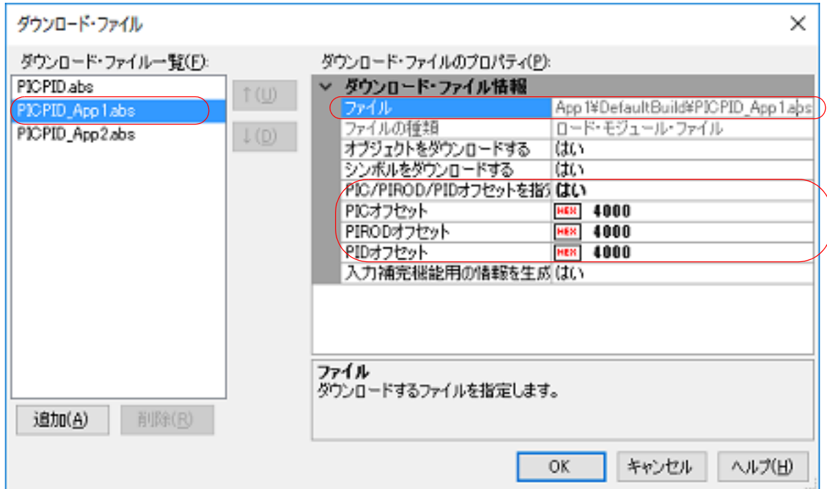
図 2.26 ダウンロード・ファイルの追加とダウンロード条件の変更 (ダウンロード・ファイル ダイアログ)
