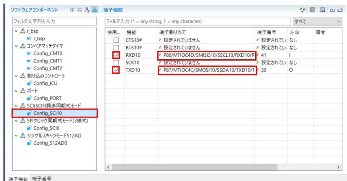
図 4-49: 端子設定 – Config_SCI10
