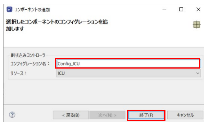
図 4-21: リソース選択 - ICU
