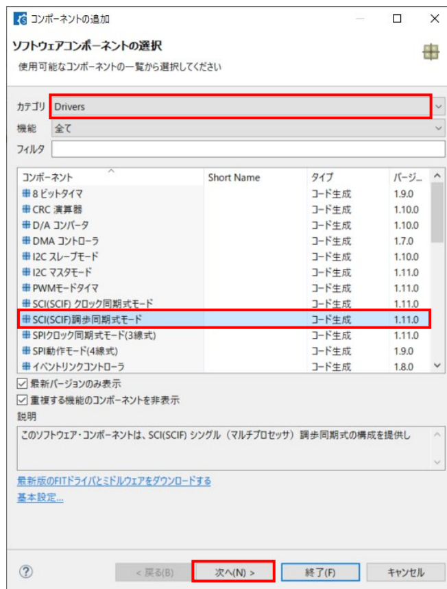
図 4-32: SCI(SCIF)調歩同期式モード選択
