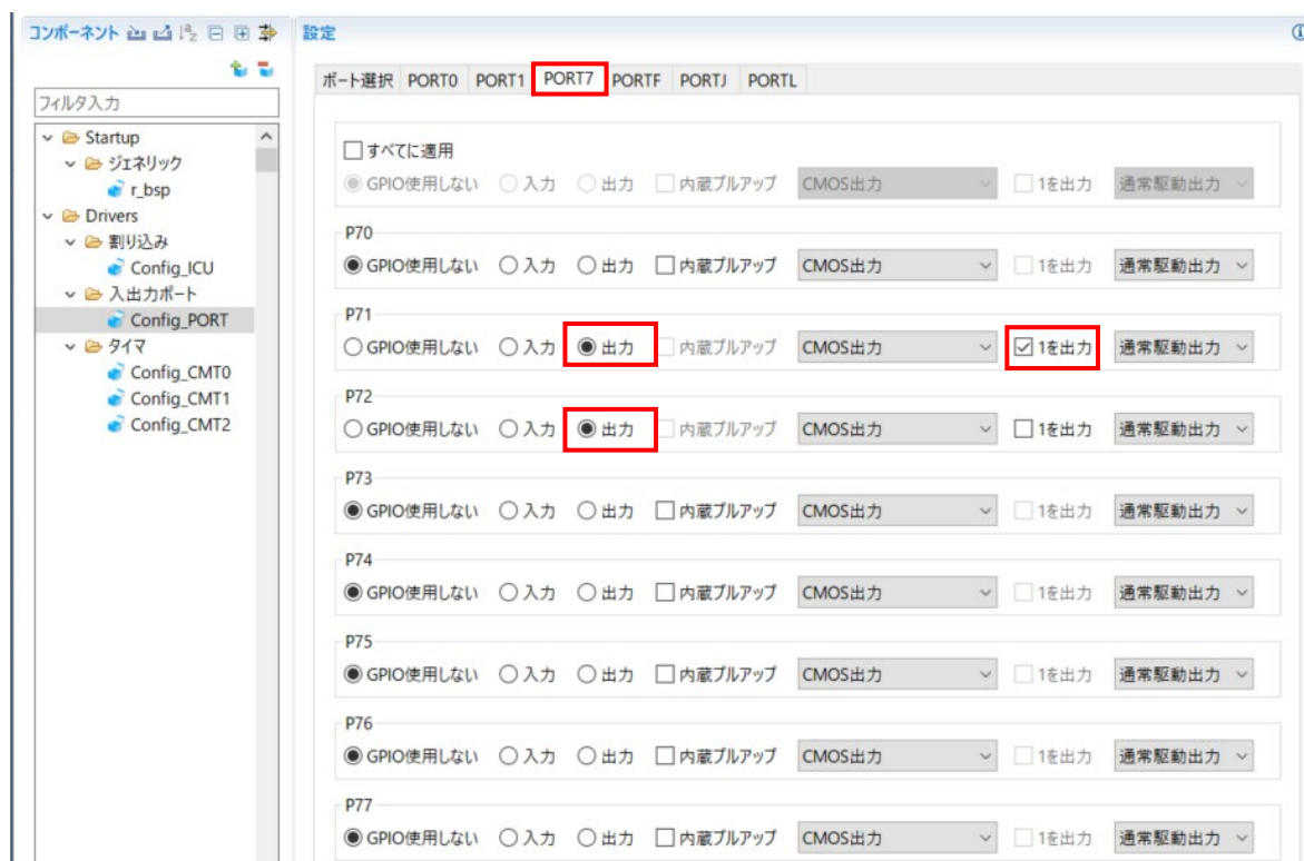
図 4-28: PORT7 タブ選択
