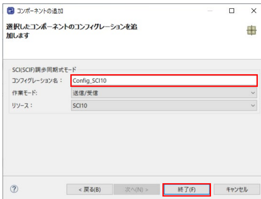
図 4-34: コンフィグレーション名 – Config_SCI10
