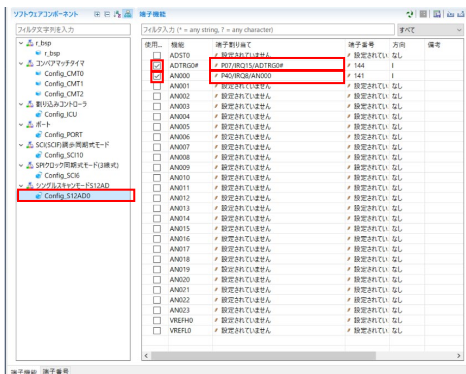
図 4-51: 端子設定 – Config_S12AD0
