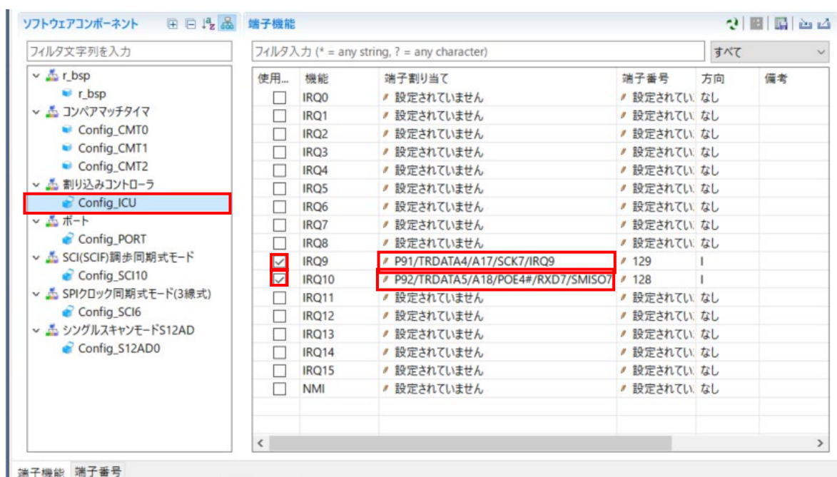
図 4-48: 端子設定 – Config_ICU
