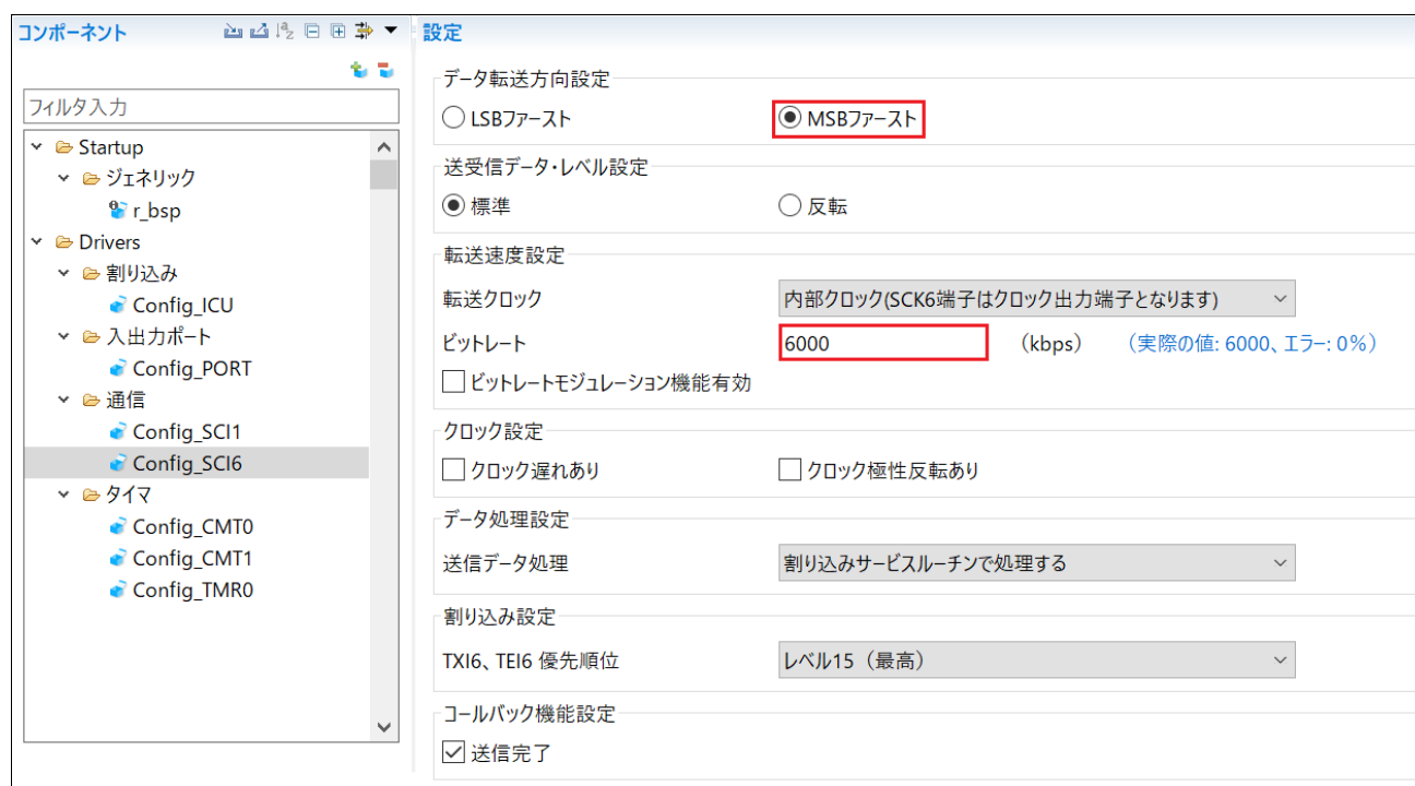
図 4-39: Config_SCI6 設定
