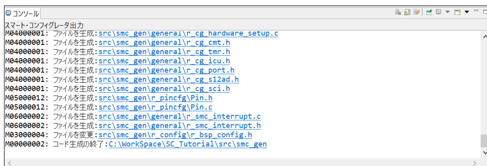
図 4-52: コード生成
