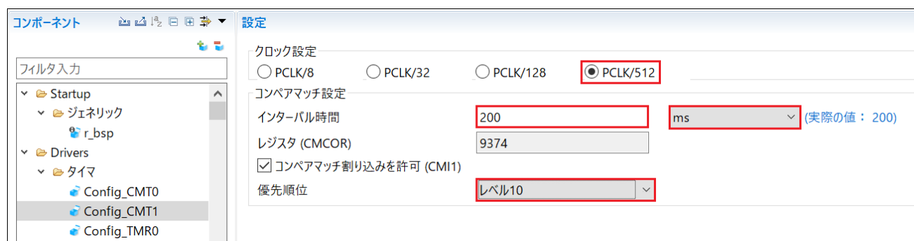
図 4-19: Config_CMT1 設定
