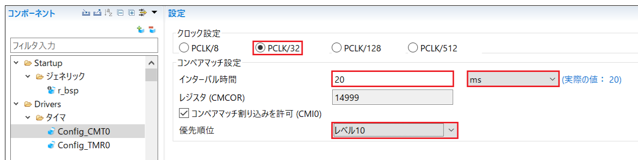
図 4-16: Config_CMT0 設定
