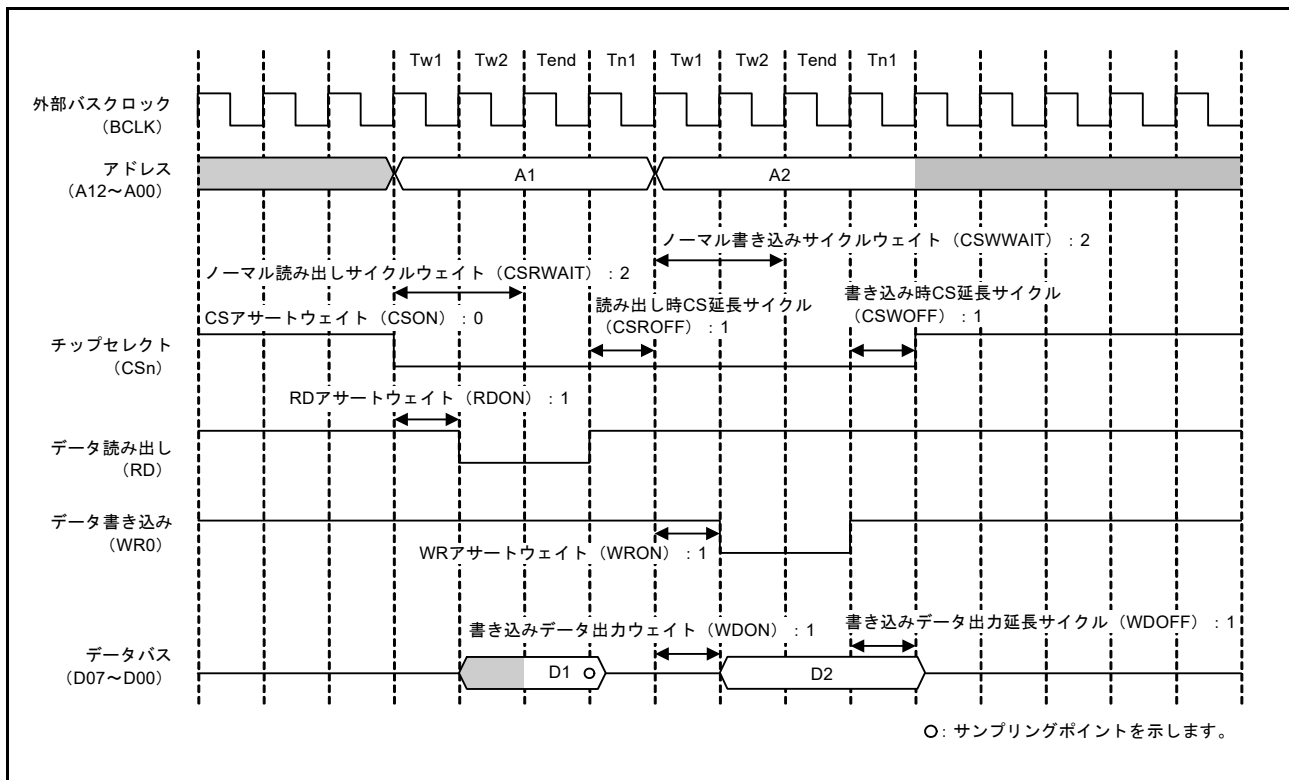
図 15.7 ノーマルアクセスの動作例 (読み出し/書き込み) (n = 0, 1, 4 ~ 7)
