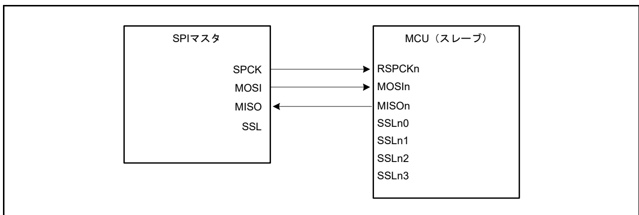
図 34.12 クロック同期式動作のマスタ/スレーブの構成例 (MCU はスレーブ、CPHA = 1)
