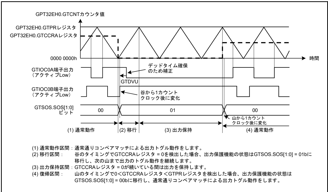
図 23.99 谷でのバッファ転送中に GTCCRA レジスタが 0 になった場合の出力保護機能の動作例 (山でのバッファ転送中に 0 < \text{GTCCRA レジスタ} < \text{GTPR レジスタ} を回復、アクティブ Low の場合)
