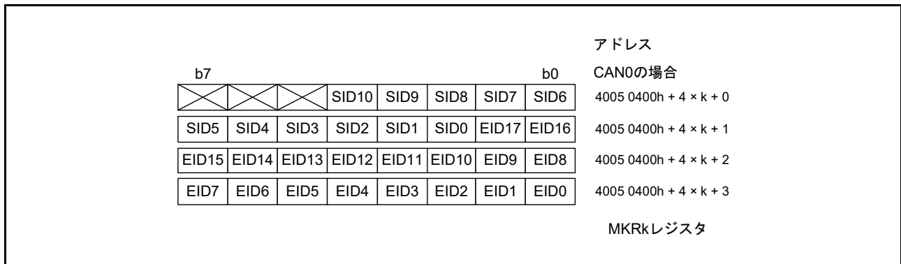
図 33.14 MKR k レジスタの構成 (k = 0 ~ 7)
