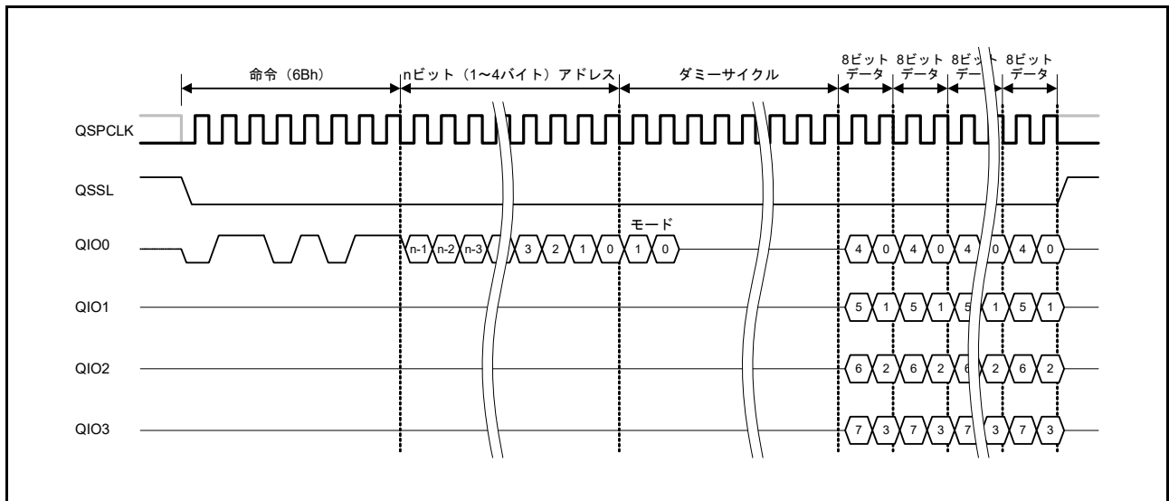
図 35.23 ファストリード Quad 出力バスサイクル
