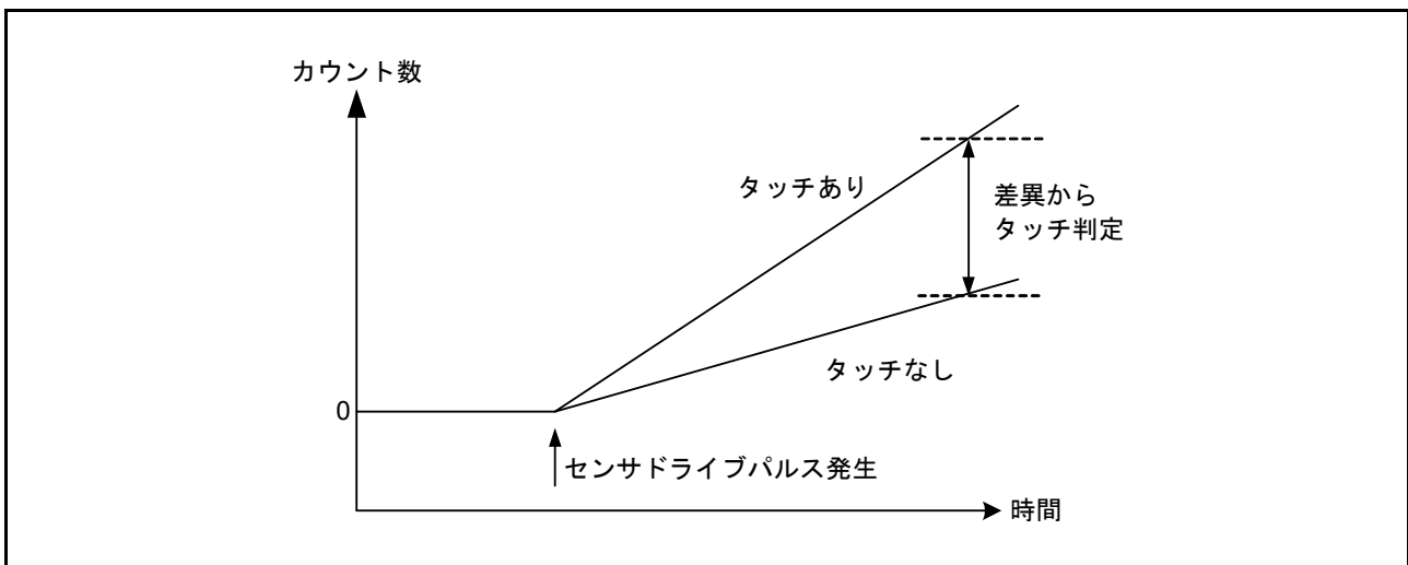
図 46.7 接触／非接触による計測値の変化
