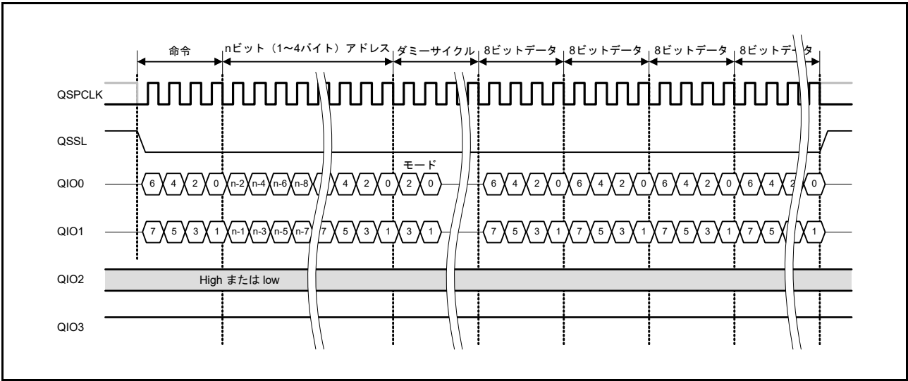
図 35.6 Dual-SPI プロトコル例 (ファストリード)
