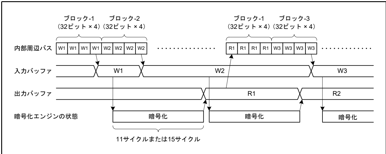
図 41.3 暗号化と復号タイミング (AES)
