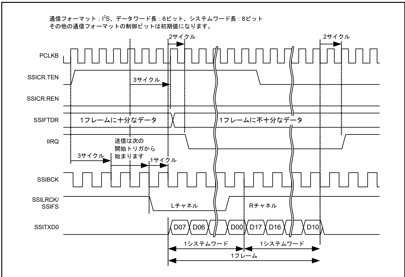
図 37.13 IIRQ 設定タイミング (送信)
