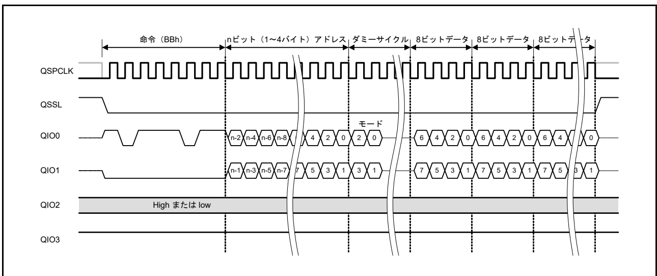
図 35.21 ファストリード Dual I/O バスサイクル
