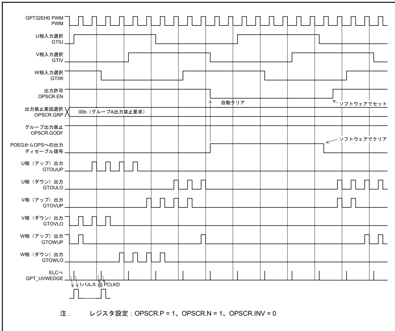
図 23.84 グループ出力禁止制御動作例
