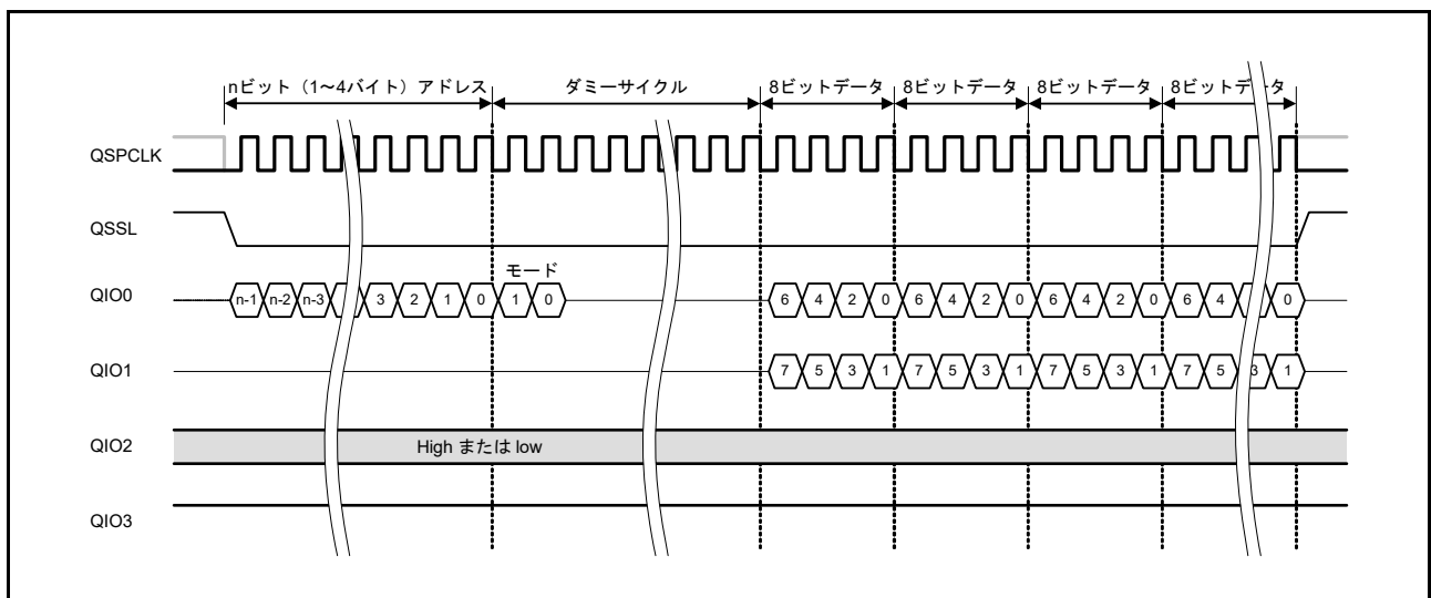
図 35.20 XIP モード時のファストリード Dual 出力バスサイクル
