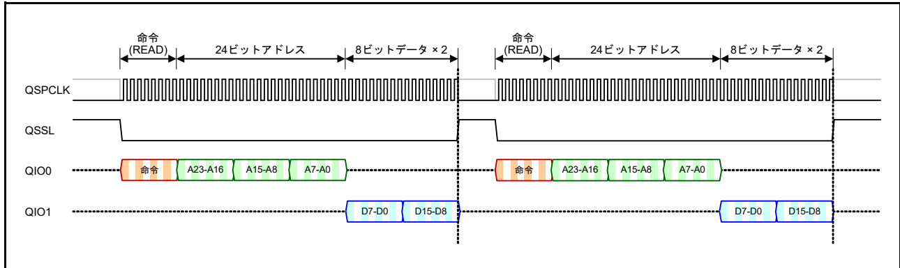
図 35.30 個々の変換に基づく連続データリード動作
