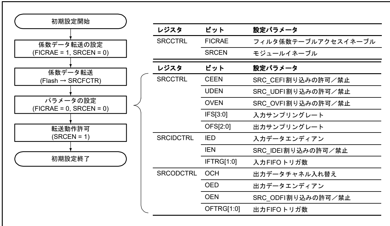
図 38.2 初期設定のフロー例
