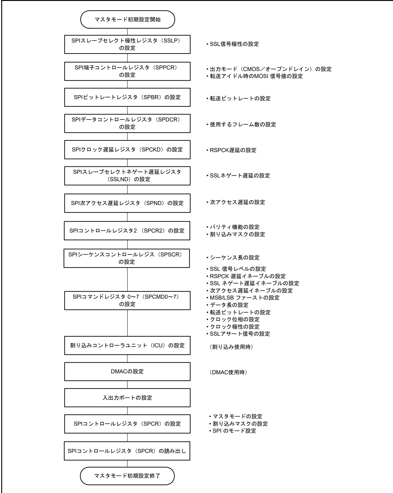
図 34.36 マスタモード時の SPI 動作の初期化フロー例
