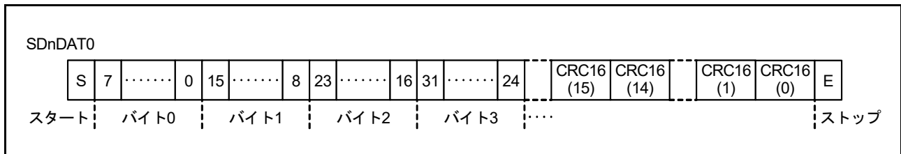
図 39.2 1 ビット幅モードの SDnDAT
