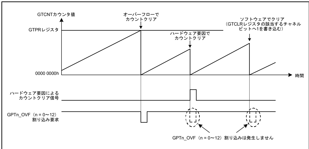
図 23.60 ハードウェア要因によるカウンタクリアと GPTn_OVF (n=0~12) 割り込みの関係
