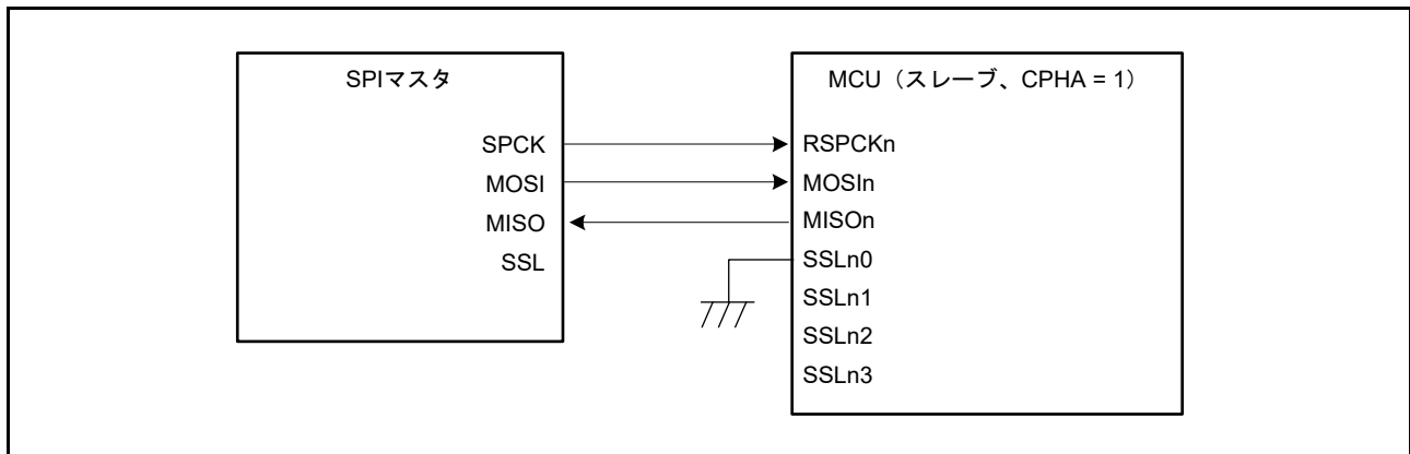
図 34.7 シングルマスタ/シングルスレーブの構成例 (MCU はスレーブ、CPHA = 1)
