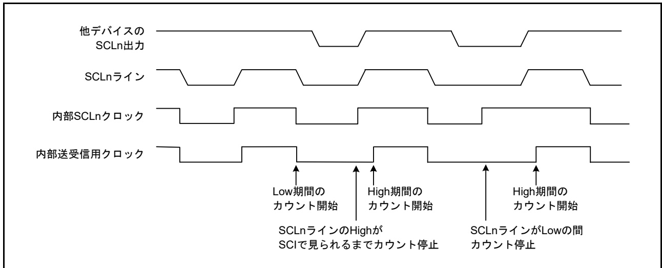
図 30.61 クロック同期化の動作例
