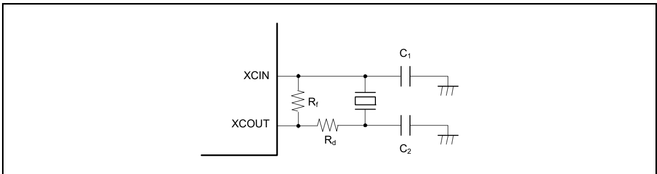
図 9.9 32.768kHz 水晶振動子の接続例
