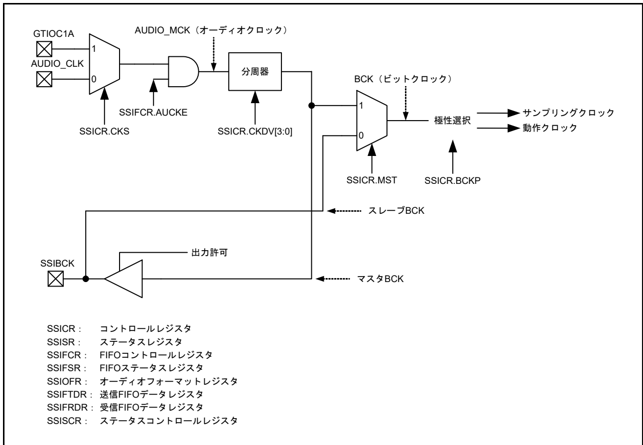
図 37.3 SSIE クロック構成
