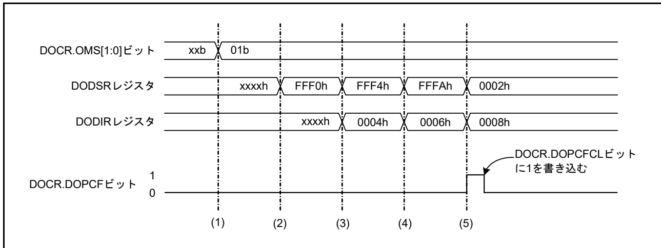
図 47.3 データ加算モードの動作例
