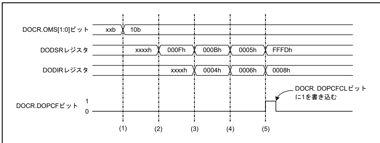
図 47.4 データ減算モードの動作例
