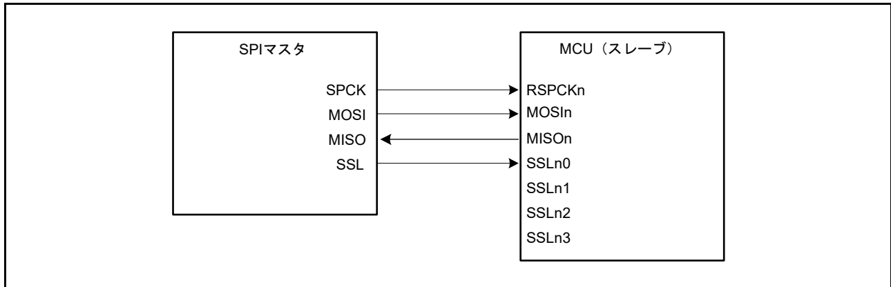
図 34.6 シングルマスタ/シングルスレーブの構成例 (MCU はスレーブ、CPHA = 0)
