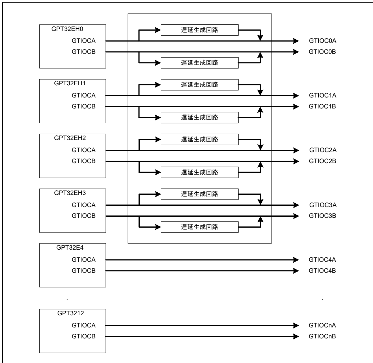
図 24.1 PWM 遅延生成回路のブロック図
