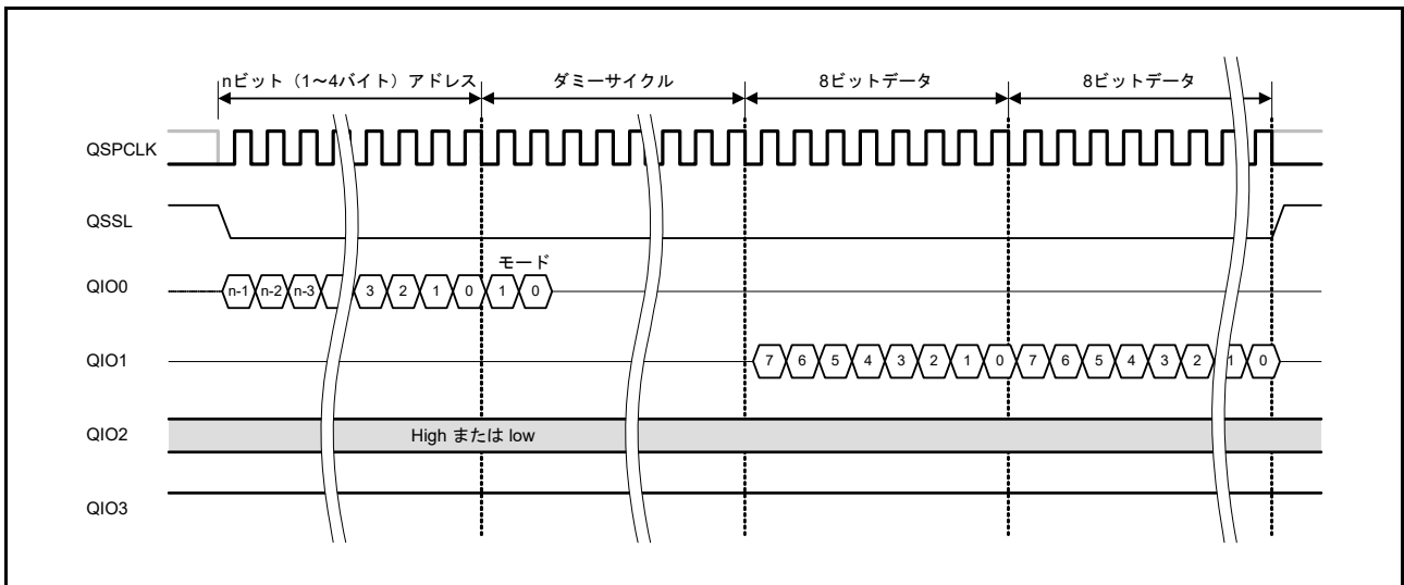
図 35.18 XIP モード時のファストリードバスサイクル
