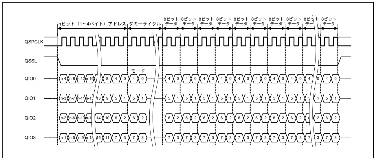
図 35.26 XIP モード時のファストリード Quad I/O バスサイクル
