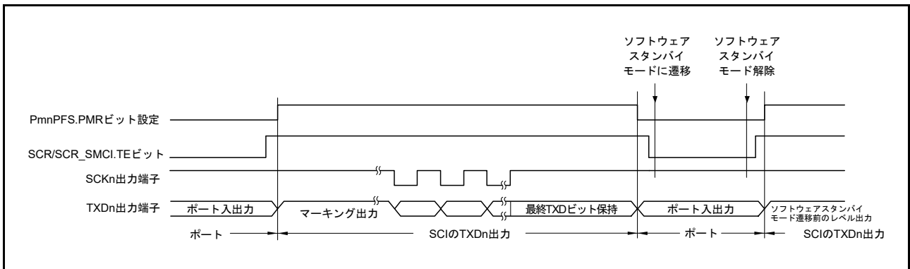
図 30.75 ソフトウェアスタンバイモード移行中のポートの端子状態 (内部クロック、クロック同期送信)
