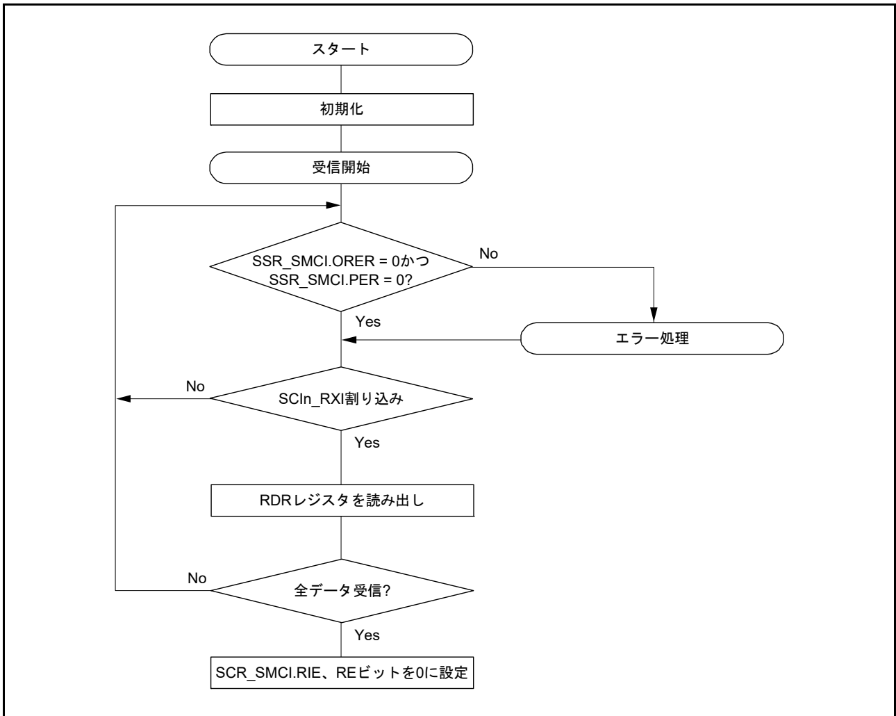
図 30.56 スマートカードインタフェース受信のフローチャート例
