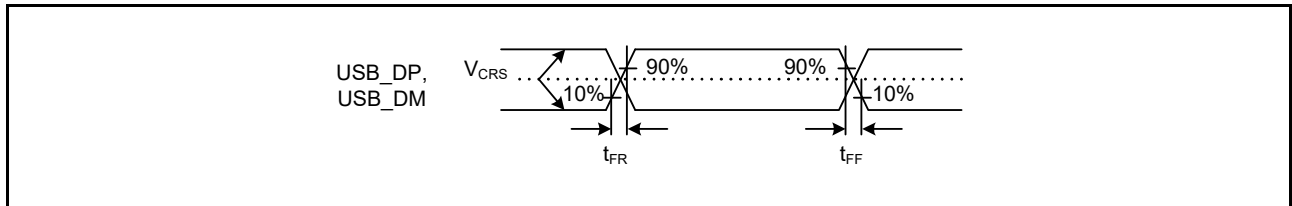
図 52.62 フルスピードモードにおける USB_DP、USB_DM の出力タイミング
