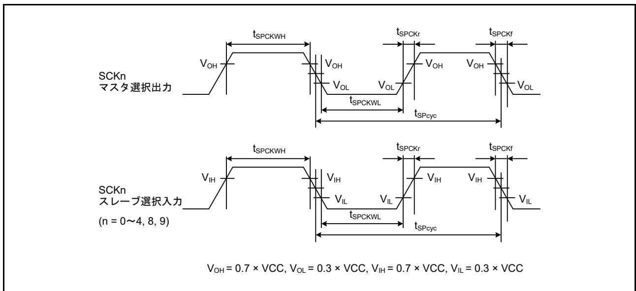
図 52.38 SCI 簡易 SPI モードクロックタイミング
