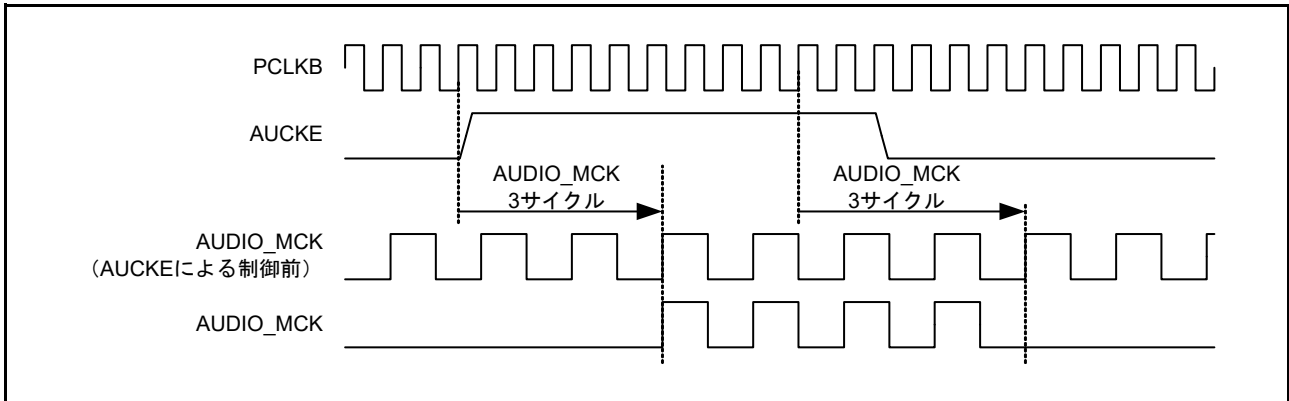
図 37.24 AUDIO_MCK の停止/再開
