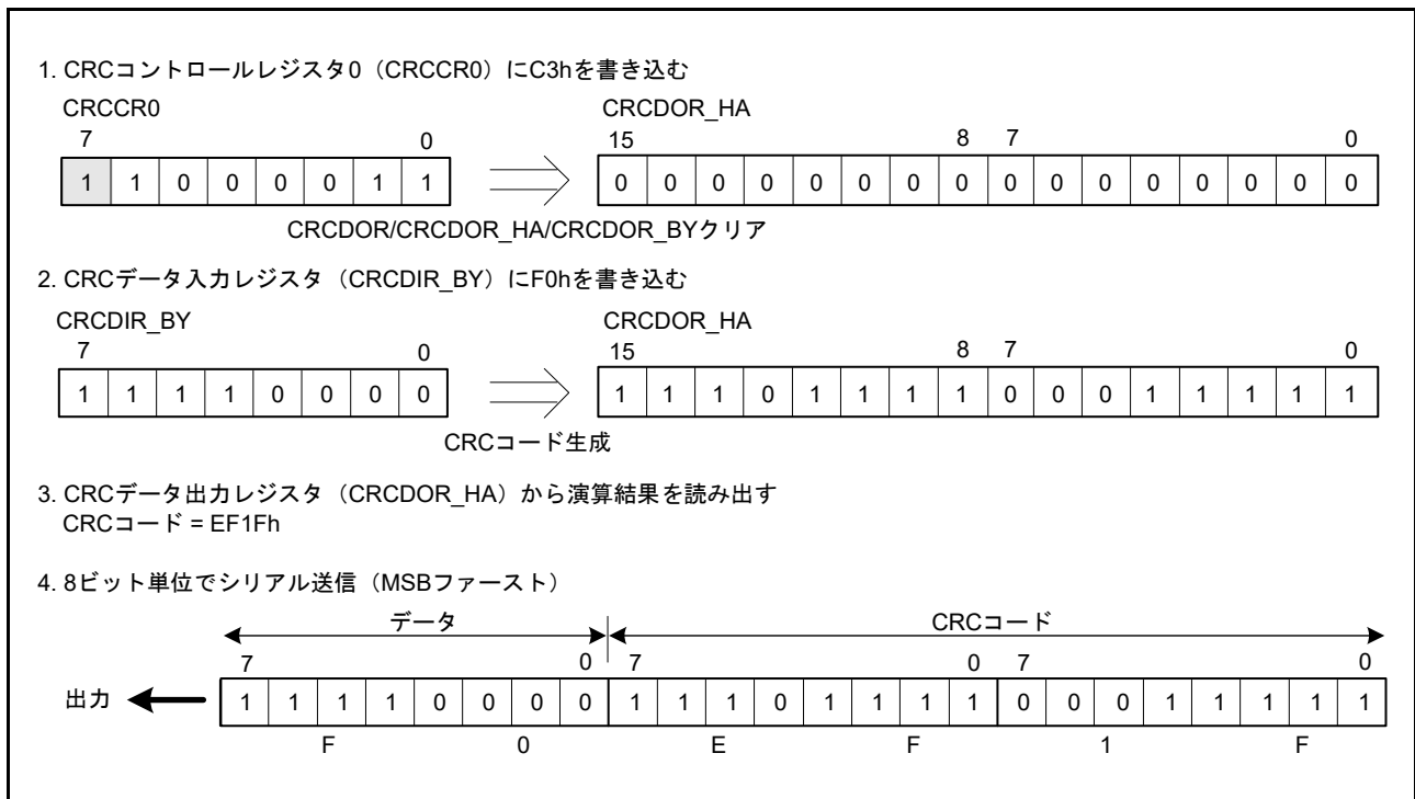
図 36.3 MSB ファーストのデータ送信
