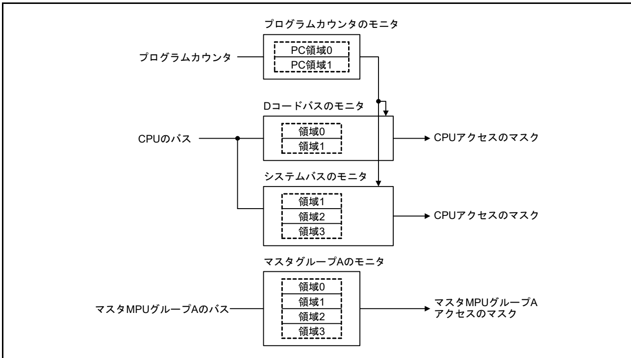
図 16.10 セキュリティ MPU のブロック図
