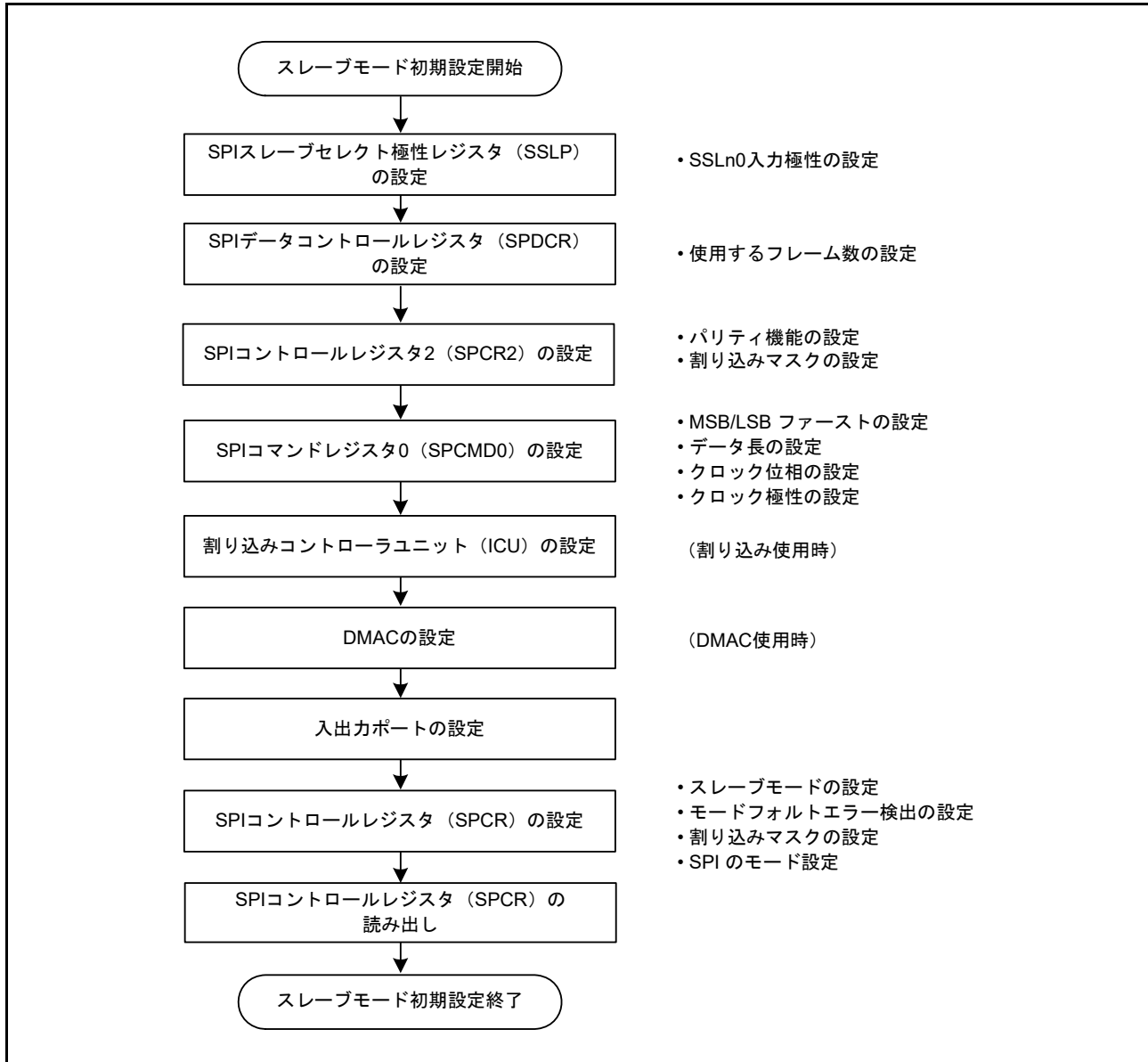
図 34.40 スレーブモード時の SPI 動作の初期化フロー例
