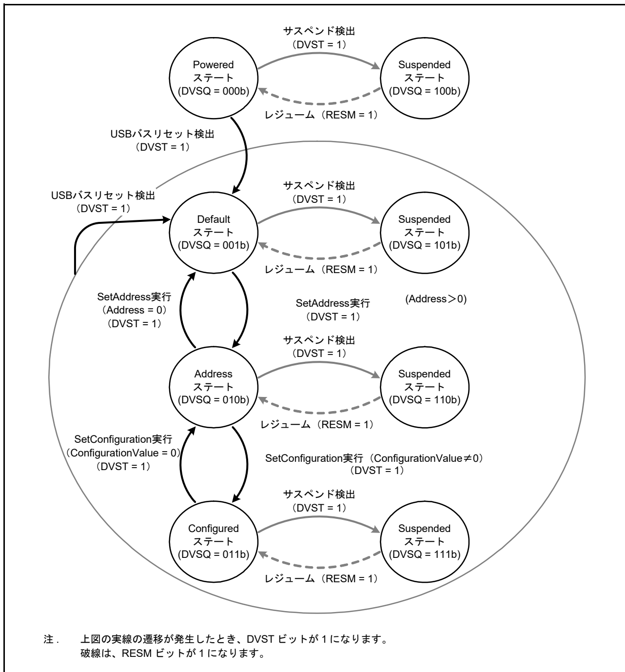
図 29.14 デバイスステートの遷移
