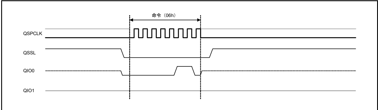
図 35.29 ライトイネーブルバスサイクル
