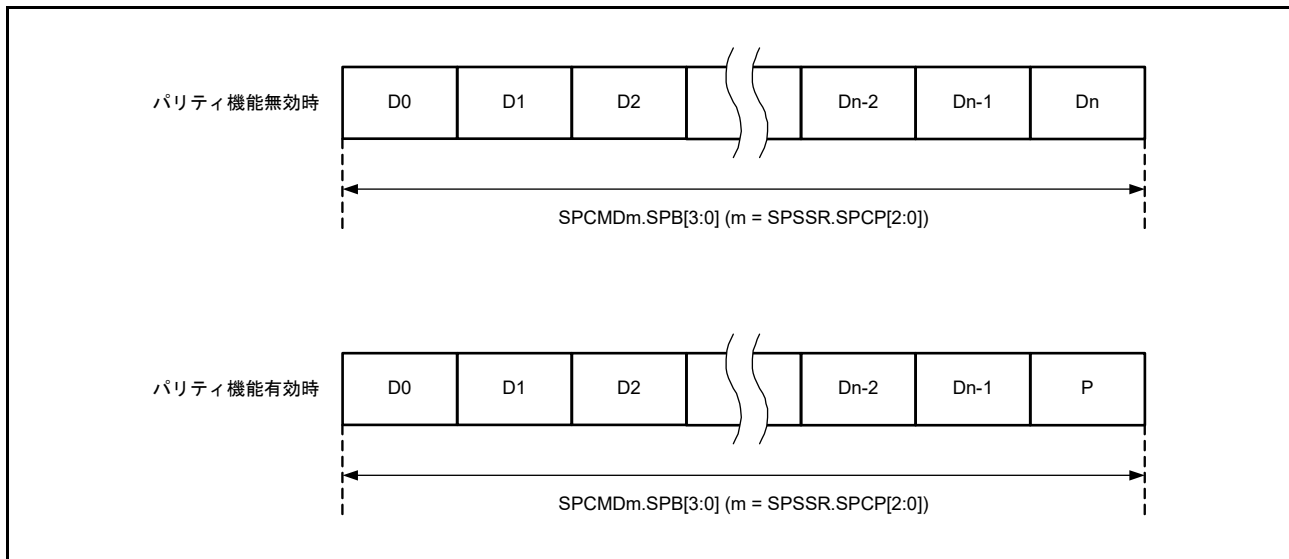
図 34.13 パリティ機能無効時と有効時のデータフォーマット
