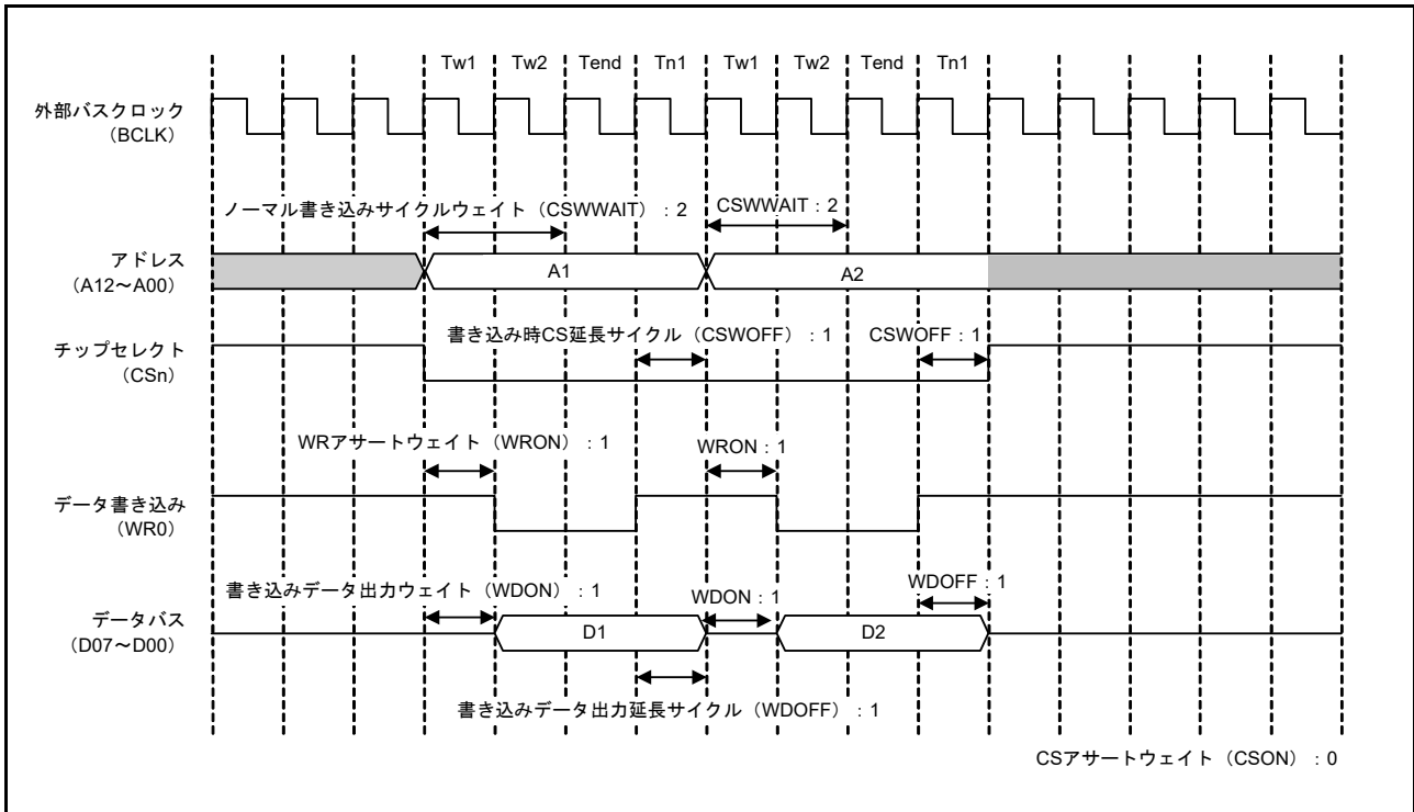
図 15.9 ノーマルライトアクセスの動作例 (1 転送要求に対して 2 回バスアクセスが発生する場合 : 1 ライトストローブモード時) (n = 0, 1, 4 ~ 7)
