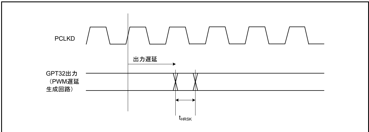
図 52.32 GPT32 (PWM 遅延生成回路) 出力遅延スキュー
