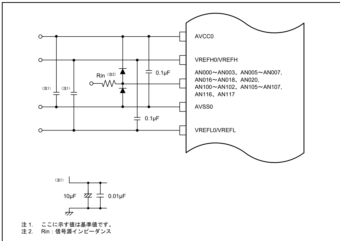
図 42.42 アナログ入力用保護回路例
