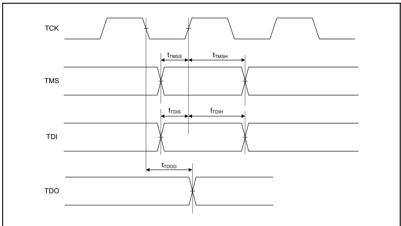
図 52.76 JTAG 入出力タイミング
