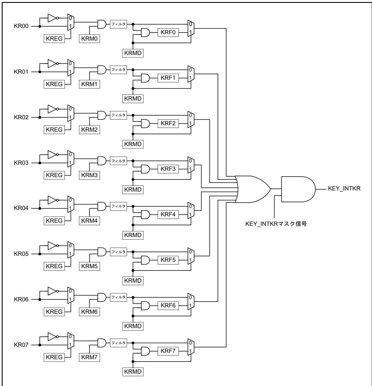
図 21.1 キー割り込み機能のブロック図
