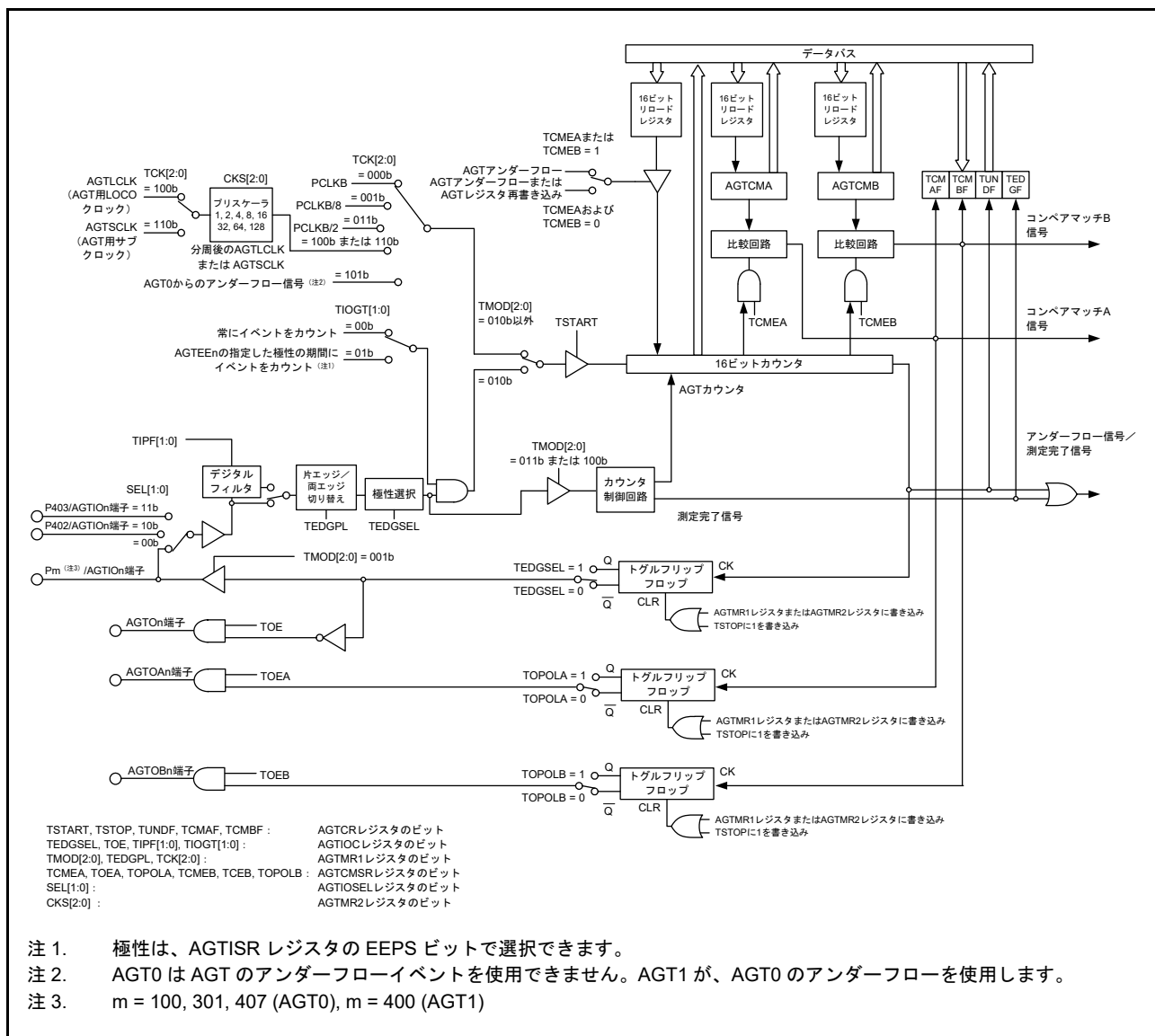
図 25.1 AGT のブロック図
