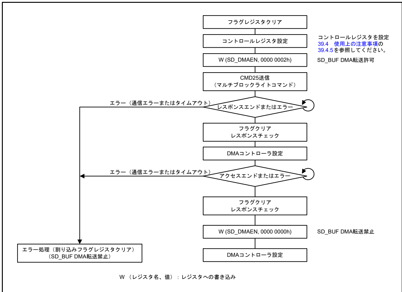
図 39.23 SD_BUF_DMA ライト動作の例
