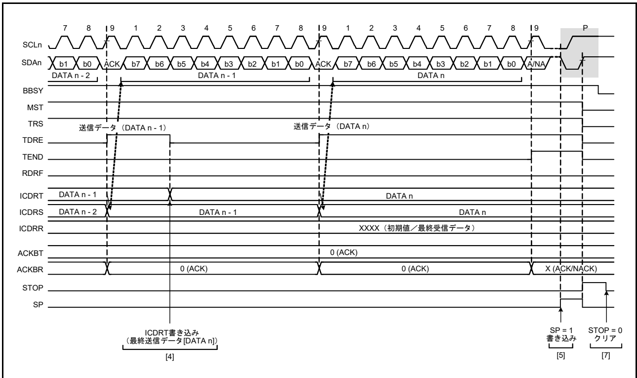
図 32.9 マスタ送信の動作タイミング (3)
