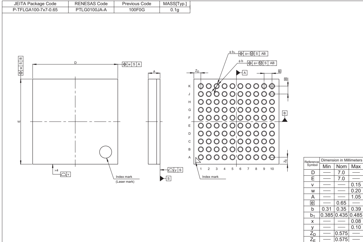
図 2.1 100 ピン LGA
