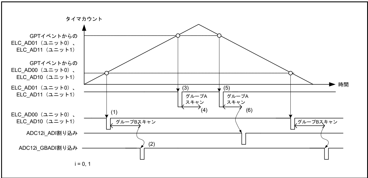
図 42.24 グループスキャンモードでダブルトリガモードを使用する場合の基本動作例 (ELC からの同期トリガ使用時)
