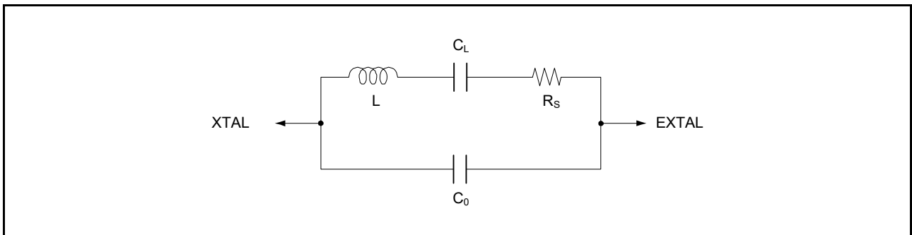
図 9.7 水晶振動子の等価回路
