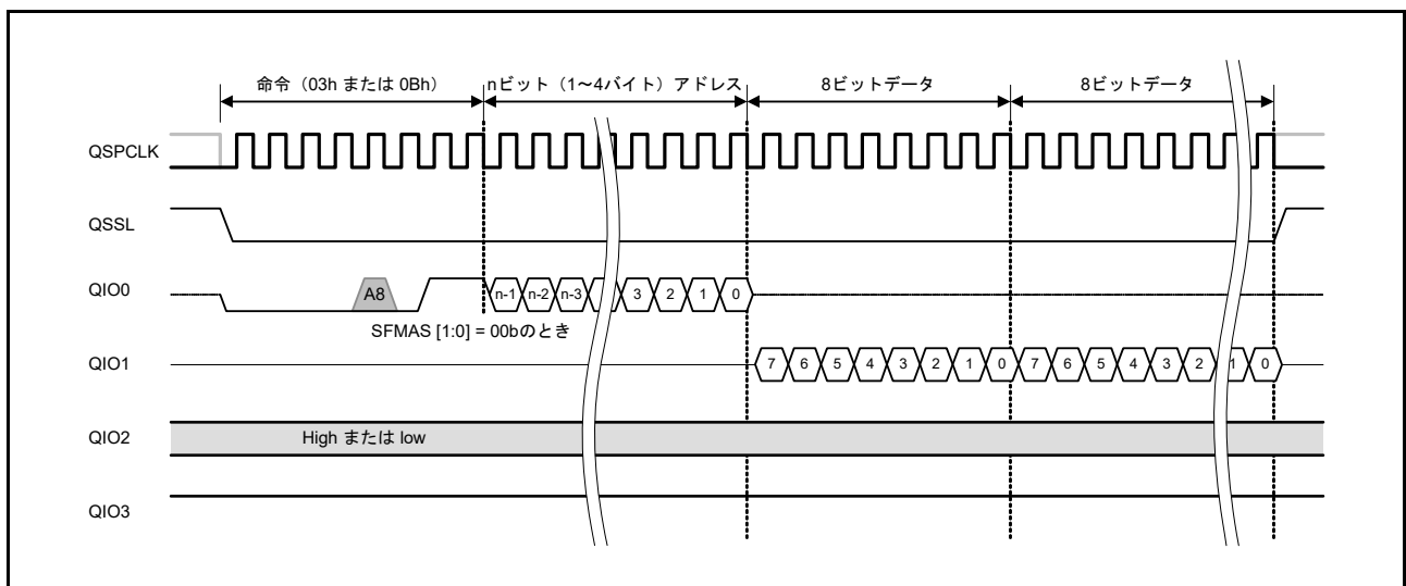
図 35.16 標準リードバスサイクル
