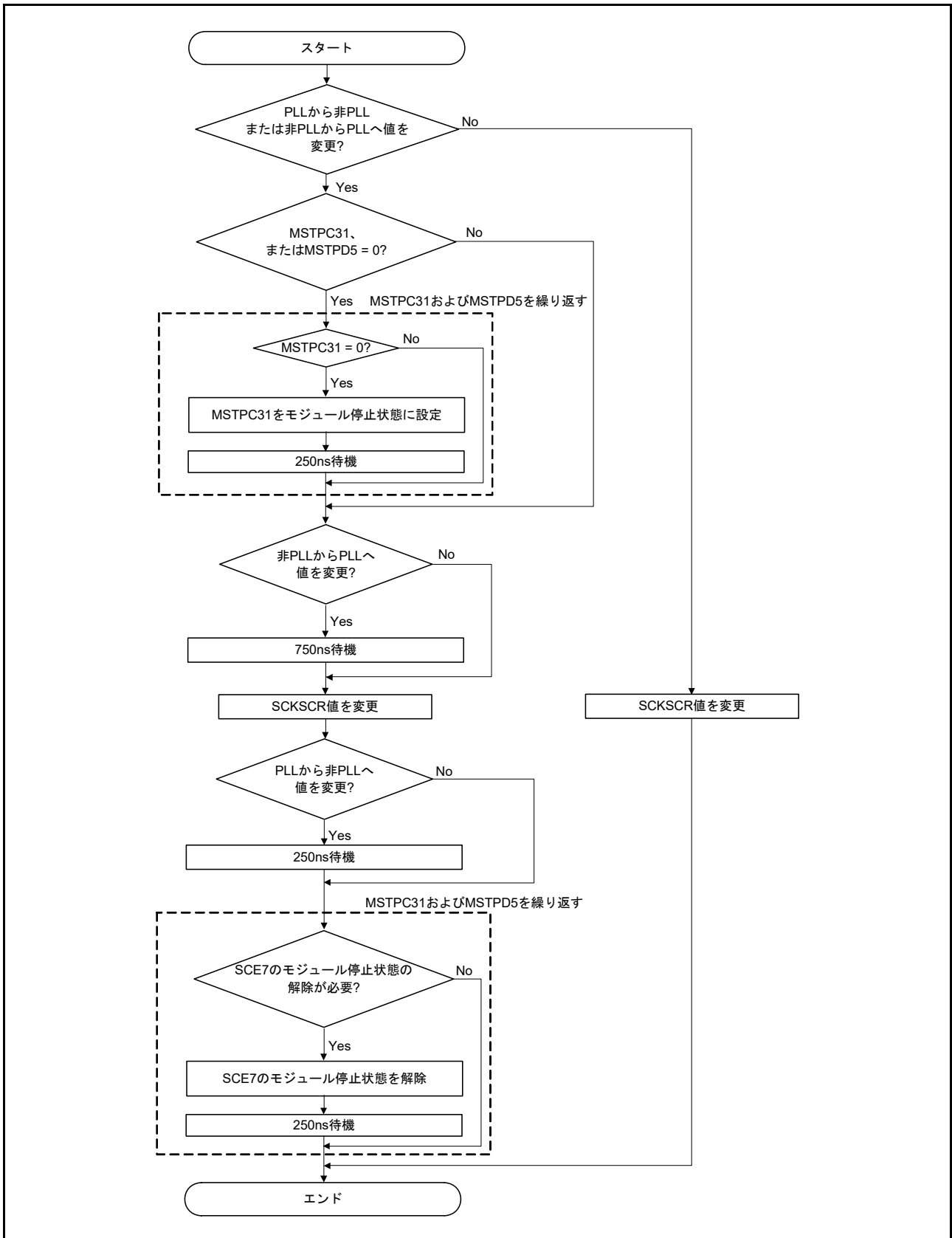
図 9.3 SCKSCR 値変更のフロー例
