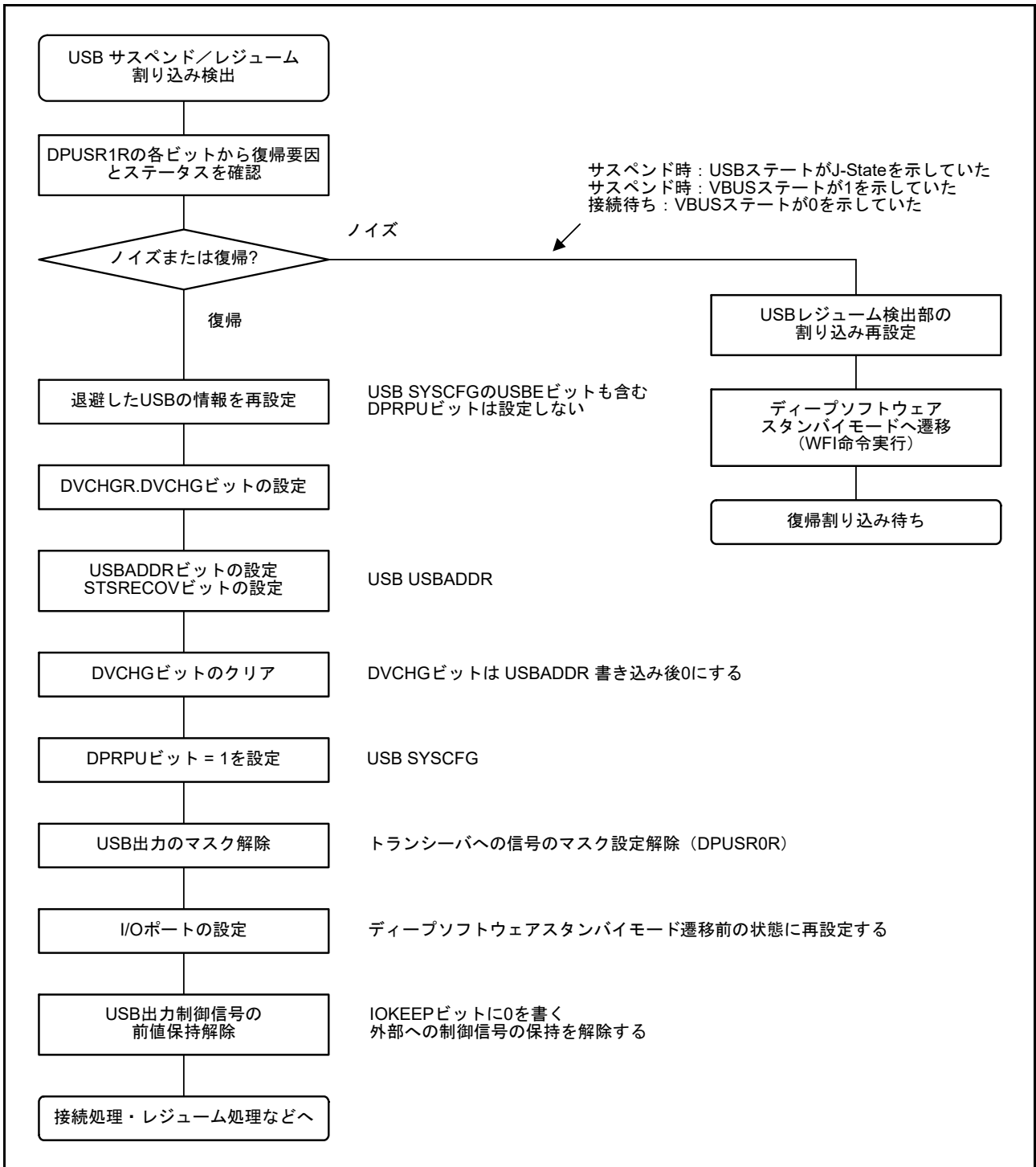
図 29.9 デバイスコントローラ機能選択時におけるディープソフトウェアスタンバイモード解除時の USBFS 設定フロー
