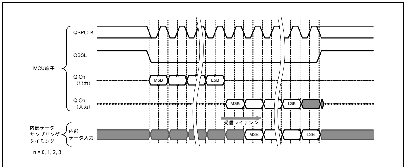
図 35.15 受信レイテンシ
