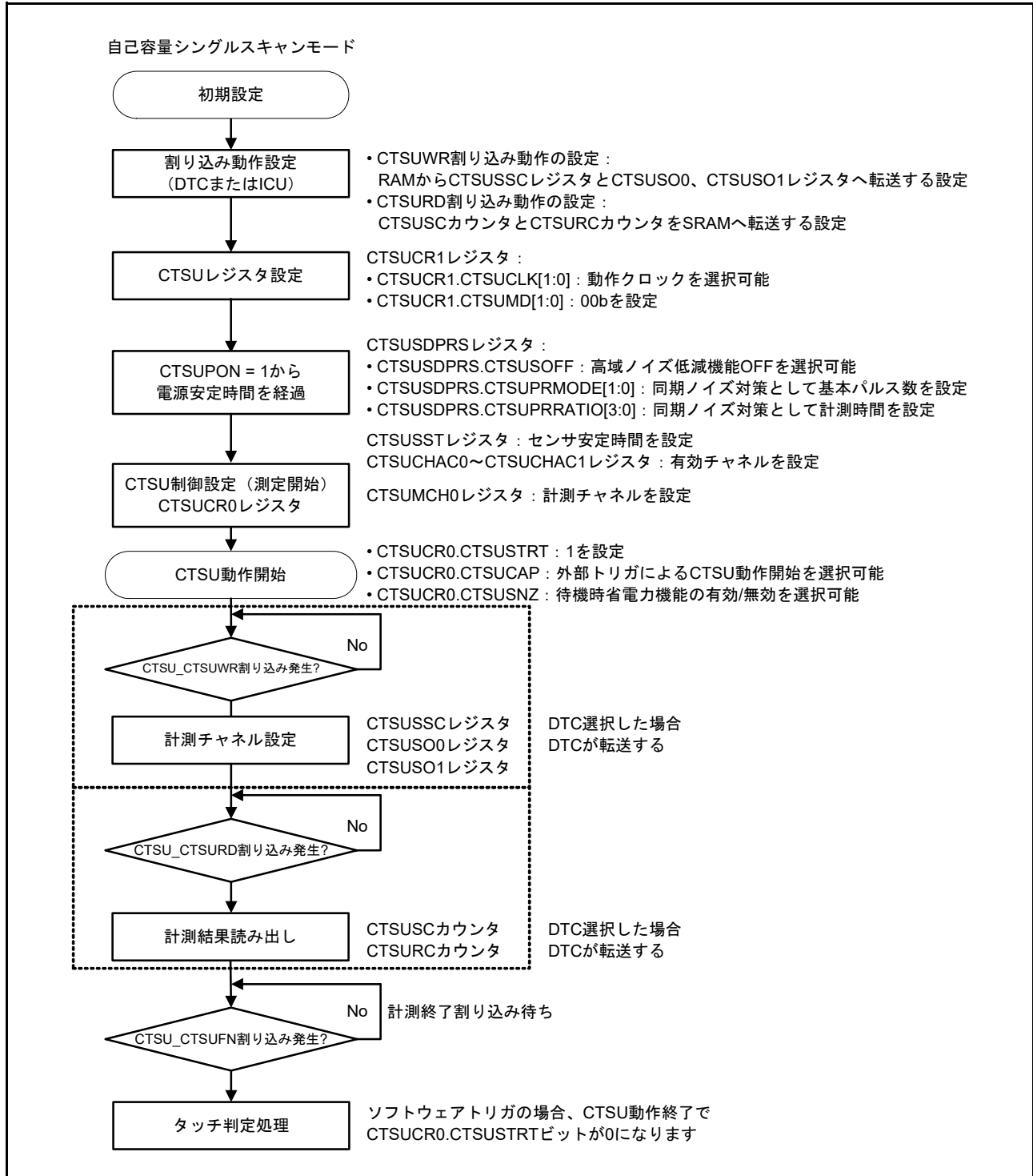
図 46.12 自己容量シングルスキャンモードのソフトウェアフローと動作例
