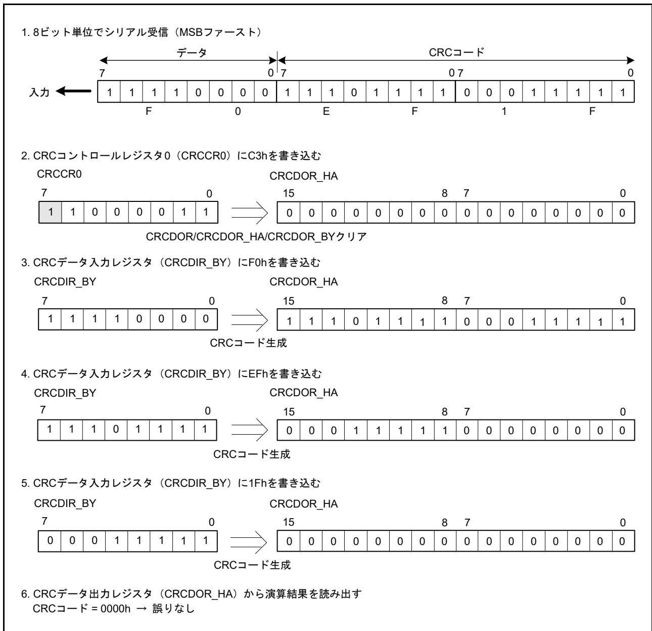
図 36.5 MSB ファーストのデータ受信
