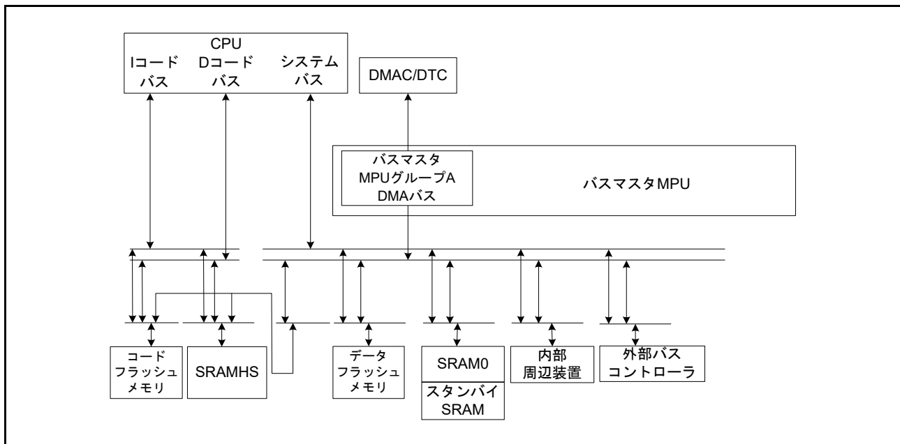
図 16.3 バスマスタ MPU ブロック図
