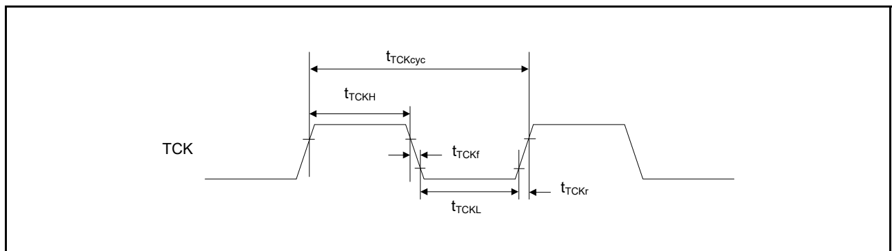
図 52.75 JTAG TCK タイミング
