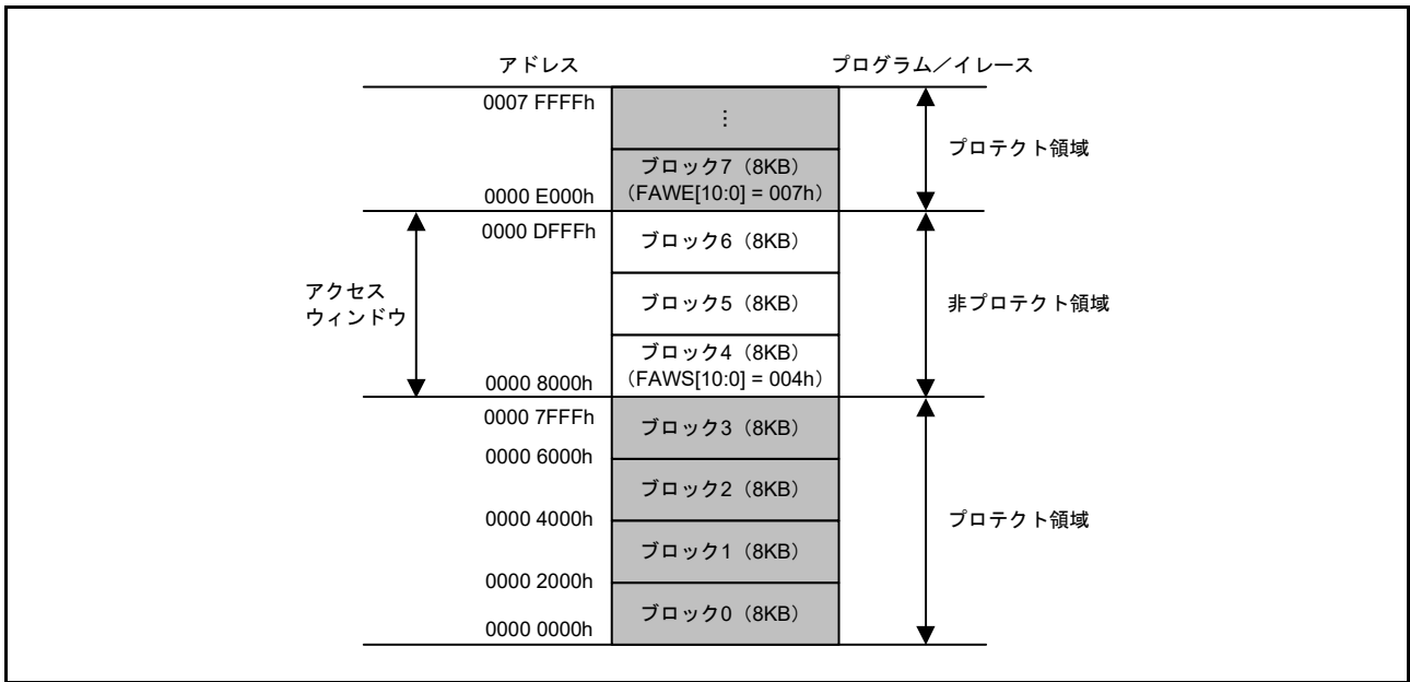
図 50.8 アクセスウィンドウに 8KB のブロックのみ含まれる場合のアクセスウィンドウの開始ブロックアドレス (FAWS) と終了ブロックアドレス (FAWE)
