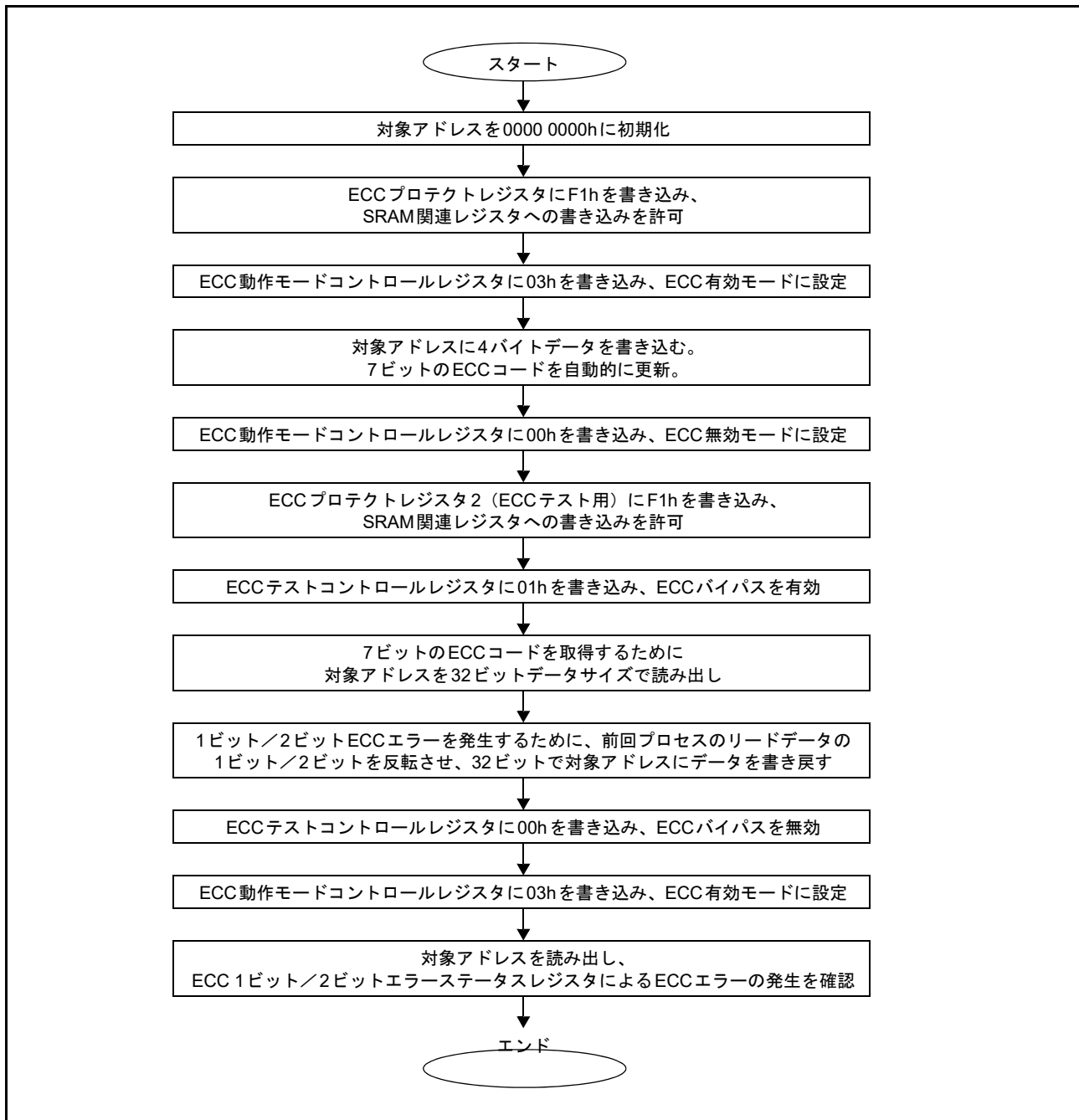
図 48.1 ECC デコーダのテスト方法
