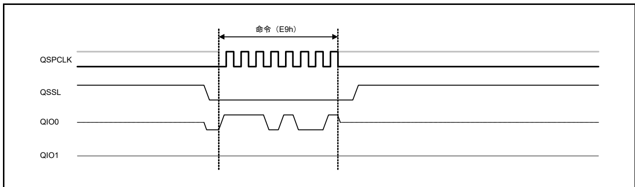
図 35.28 4 バイトモード解除バスサイクル
