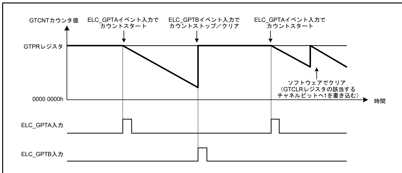
図 23.58 ハードウェア要因によるカウンタクリア動作例 (のこぎり波ダウンカウント、ELC_GPTA イベント入力スタート、ELC_GPTB イベント入力でストップ/クリアの場合)
