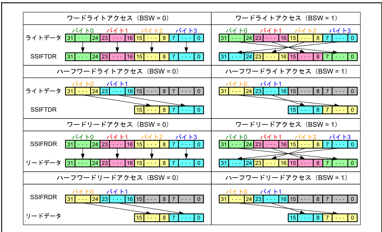
図 37.23 バイトスワップの動作例
