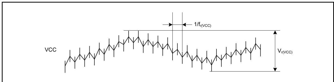
図 52.6 リップル波形
