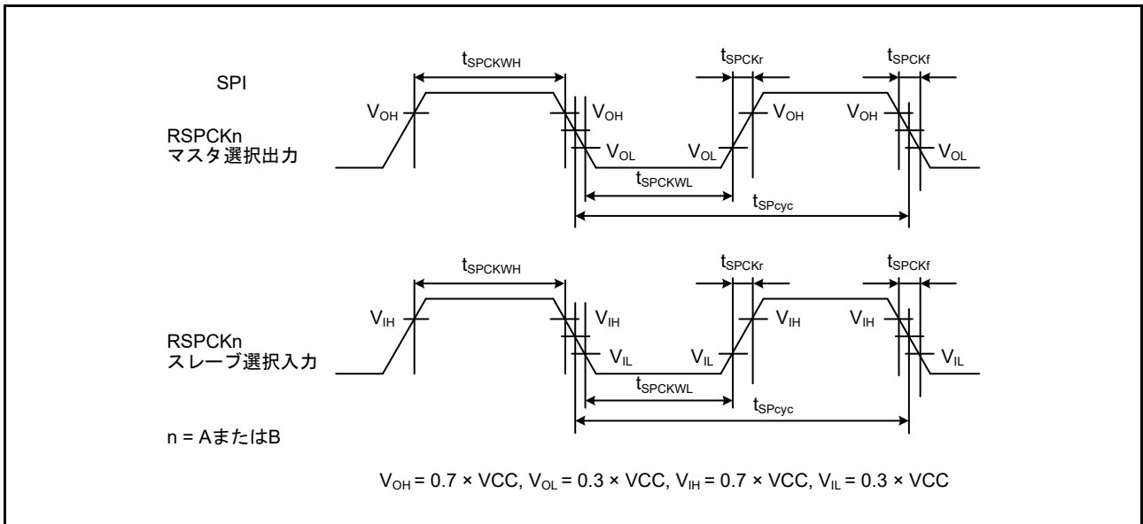
図 52.44 SPI クロックタイミング
