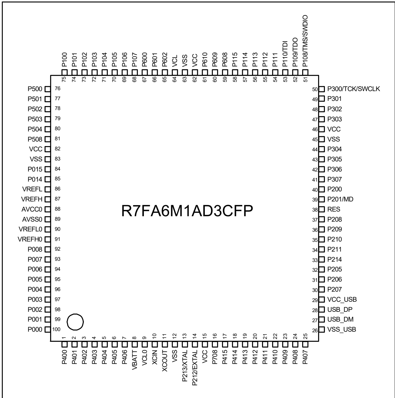
図 1.4 100-pin LQFP のピン配置図 (上面図)
