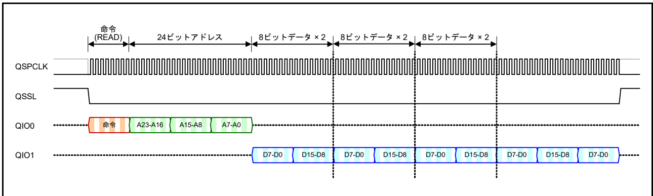
図 35.31 プリフェッチ機能を使用した連続データのリード動作
