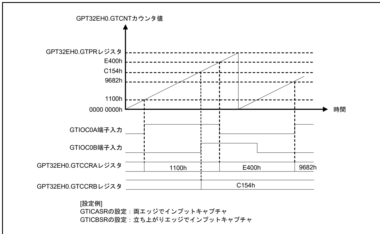
図 23.16 インพุットキャプチャ動作例
