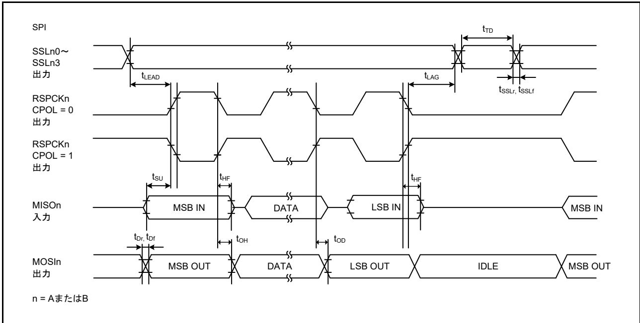
図 52.46 CPHA = 0 で、PCLKA/2 にピットレートが設定されている場合におけるマスタの SPI タイミング
