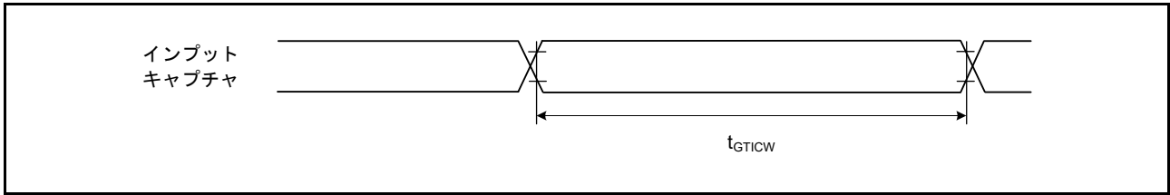
図 52.29 GPT32 インプットキャプチャタイミング
