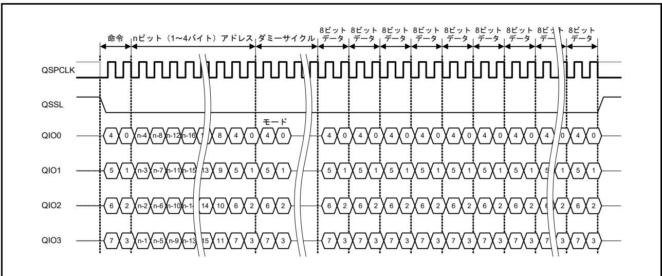
図 35.7 Quad-SPI プロトコル例 (ファストリード)
