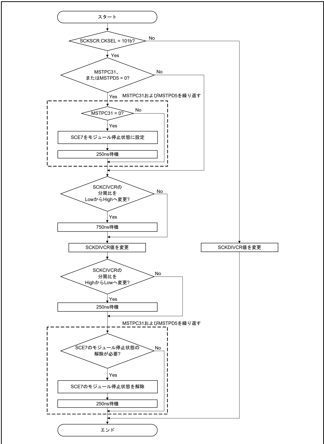
図 9.2 SCKDIVCR 値の変更フロー例
