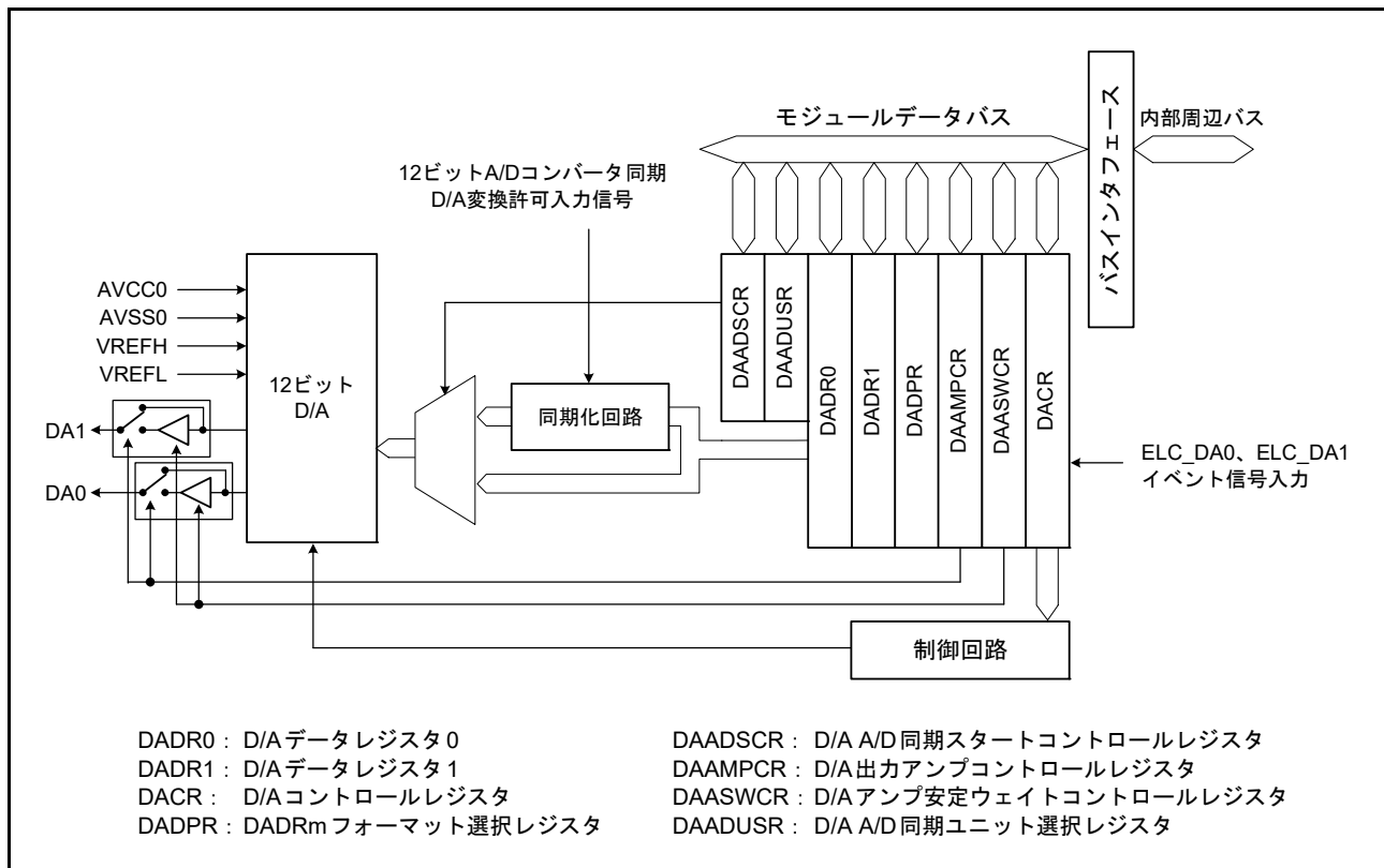
図 43.1 DAC12のブロック図
