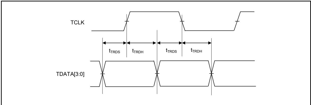
図 52.80 ETM 出力タイミング
