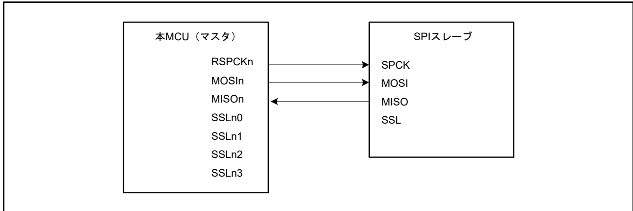
図 34.11 クロック同期式動作のマスタ/スレーブの構成例 (MCU はマスタ)
