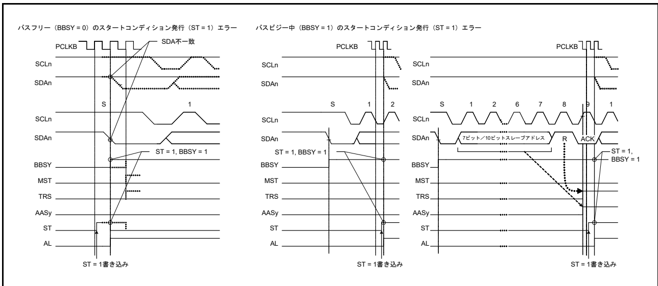
図 32.42 スタートコンディション発行時のアービトレーションロスト (MALE = 1 の場合)
