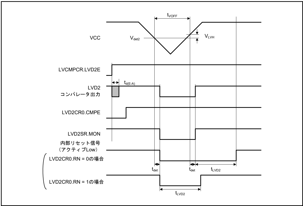
図 52.69 電圧検出回路タイミング ( V_{det2} )
