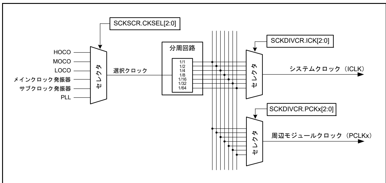
図 9.13 クロックソース選択ブロック図
