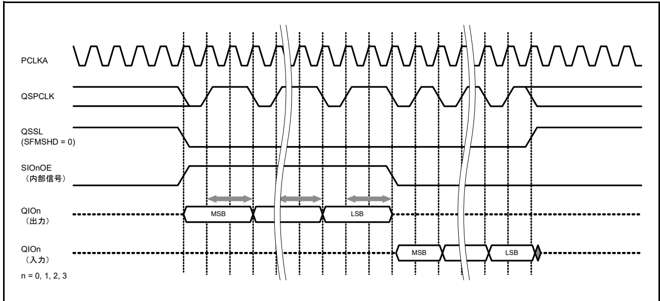
図 35.14 SFMOHW ビットを使用したシリアルデータ出力のホールド時間調整
