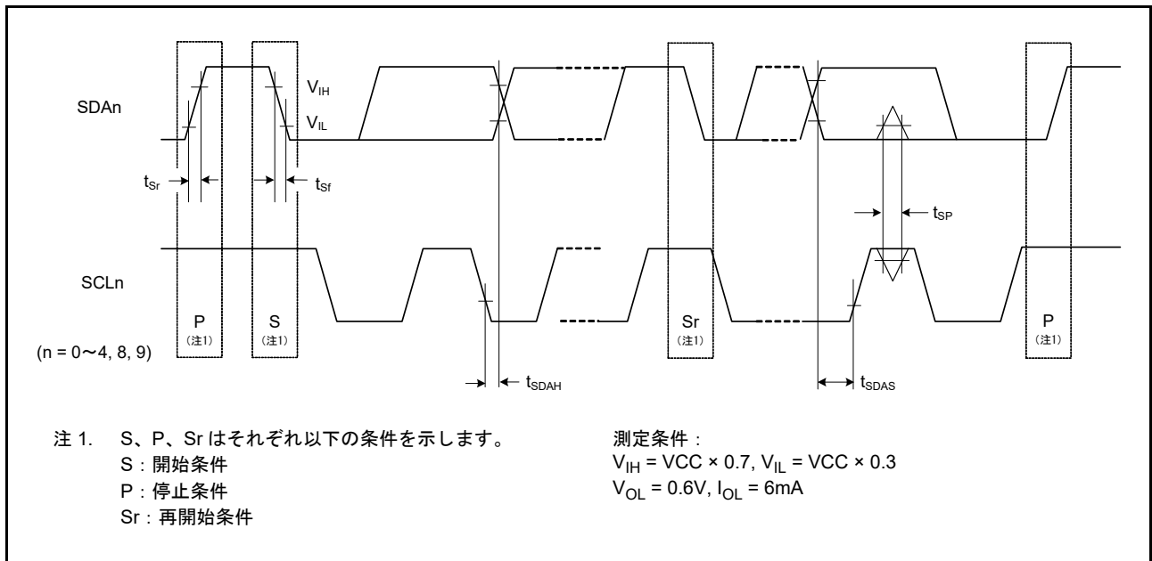
図 52.43 SCI 簡易 IIC モード タイミング
