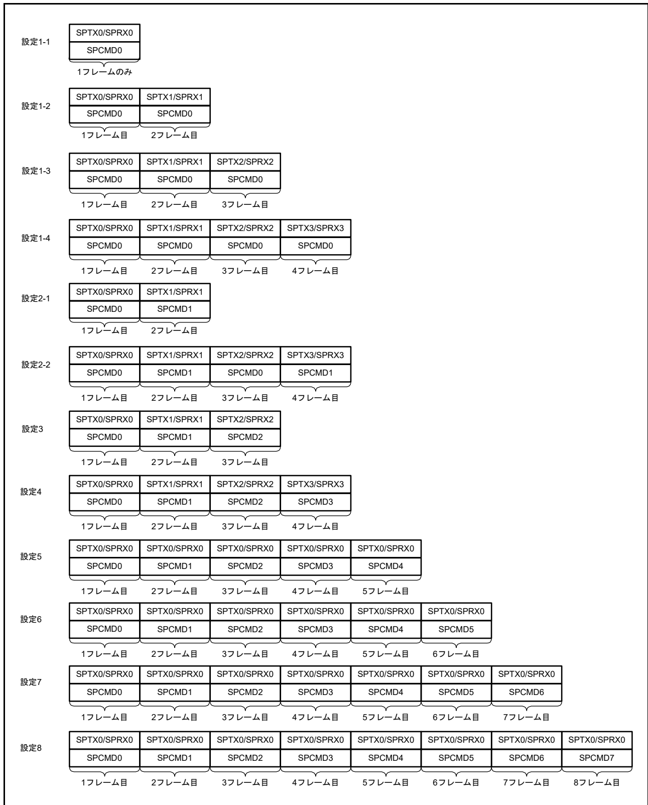
図 34.46 シーケンス動作時の SPI コマンドレジスタと送受信バッファの対応関係
