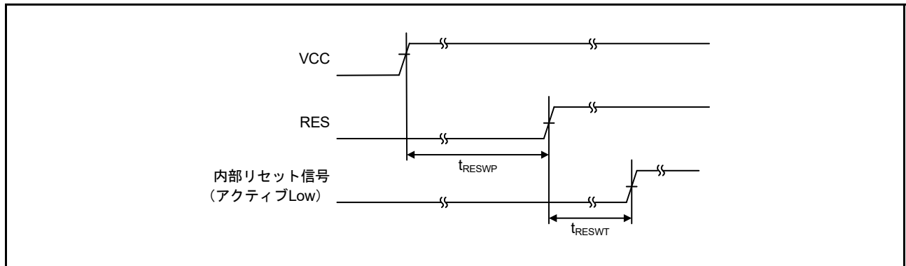
図 52.13 パワーオンリセットタイミング
