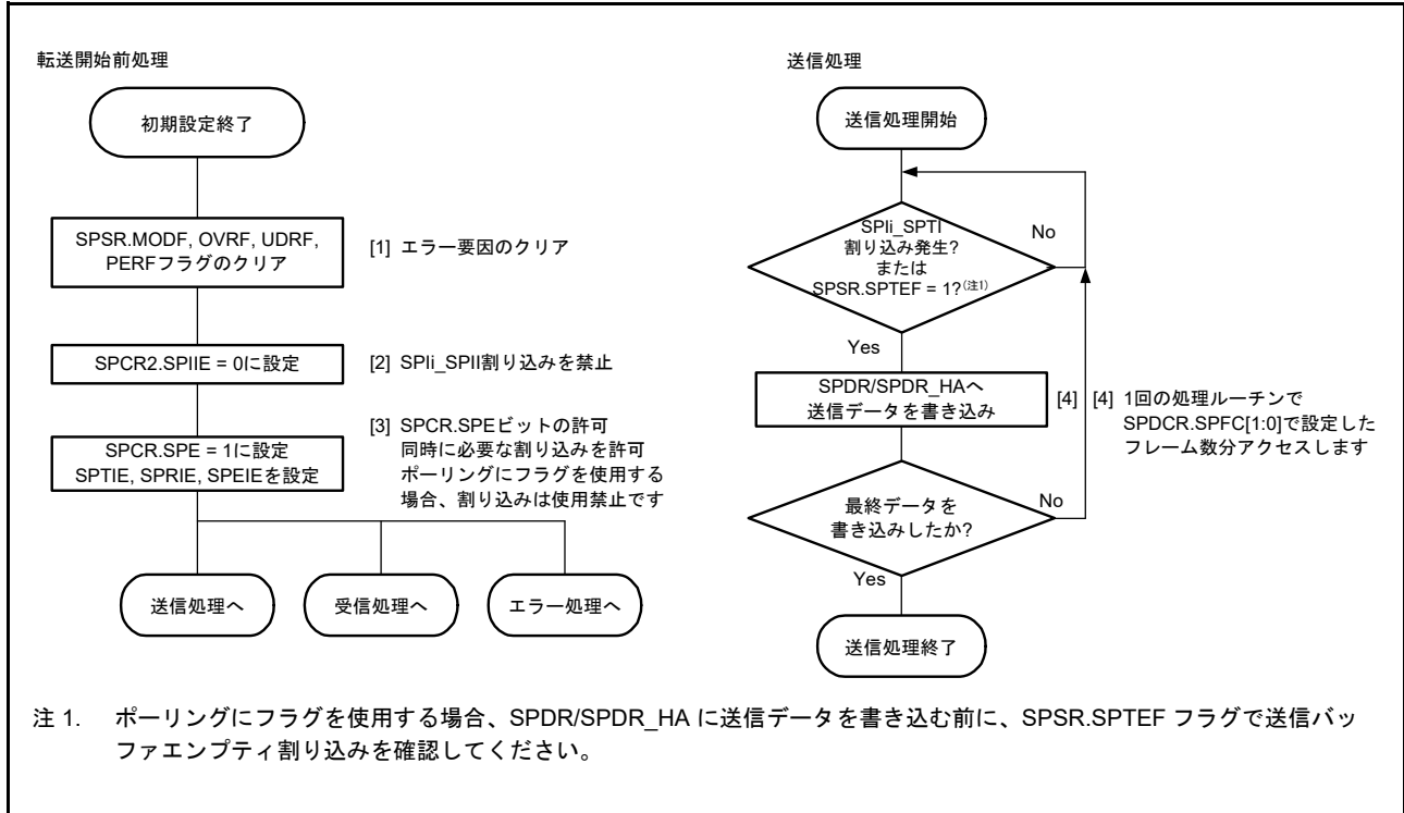
図 34.41 スレーブモードでの送信フロー
