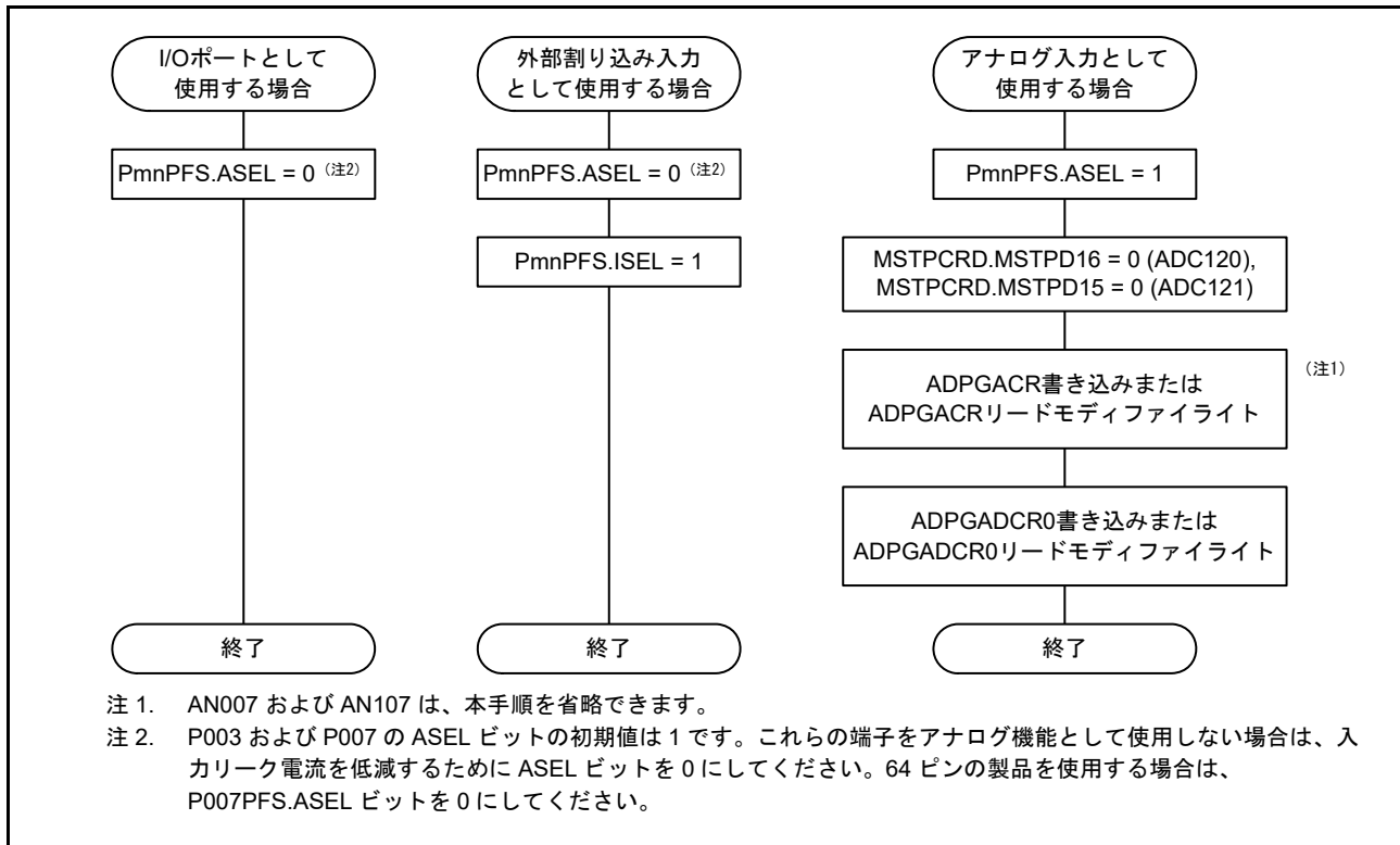
図 42.41 レジスタの設定手順
