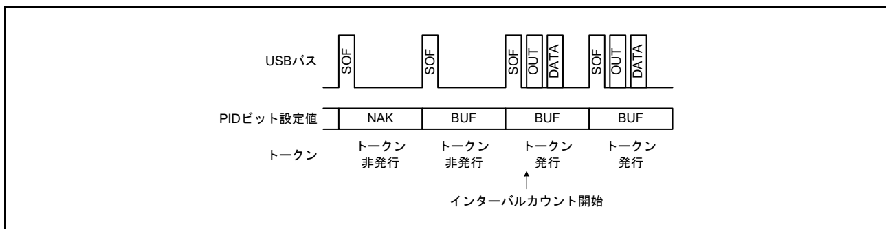
図 29.16 IITV = 0 の場合のトークン発行の有無
