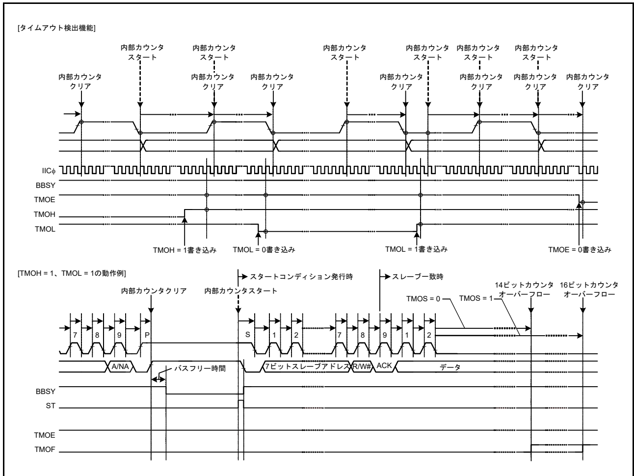
図 32.48 タイムアウト検出機能 (TMOE、TMOS、TMOH および TMOL ビットの使用)
