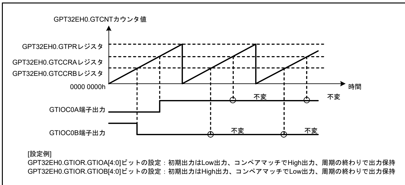
図 23.11 Low 出力 / High 出力動作例
