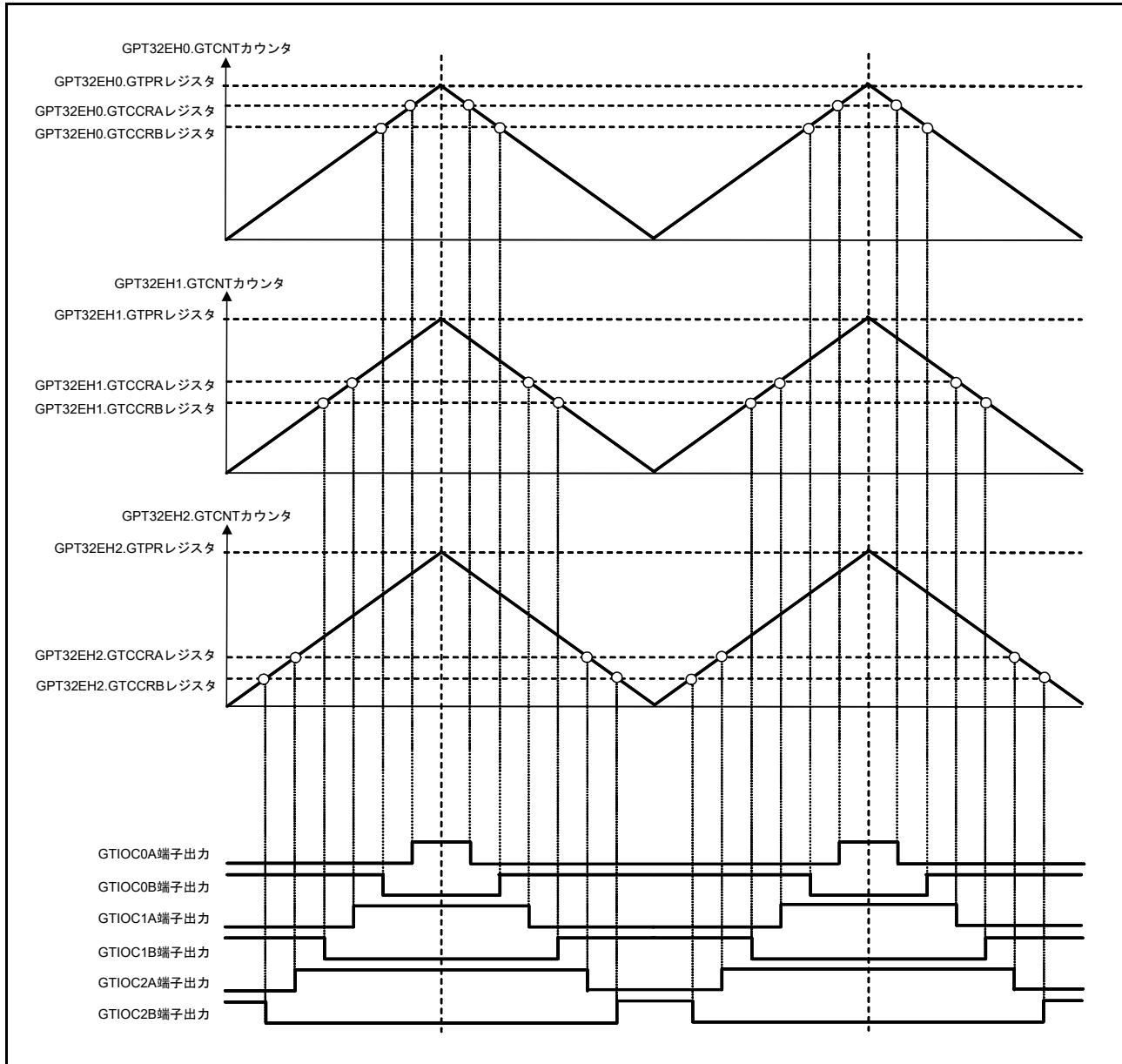
図 23.68 三角波 3 相相補 PWM 出力例
