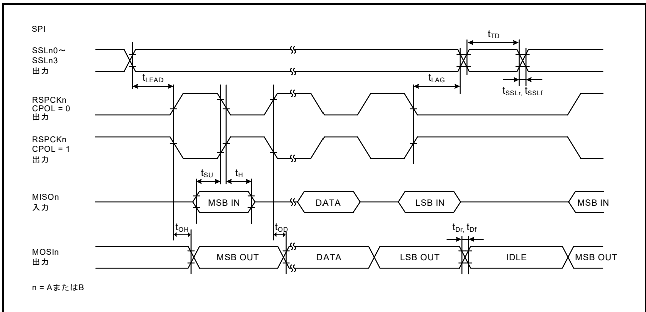
図 52.47 CPHA = 1 の場合におけるマスタの SPI タイミング
