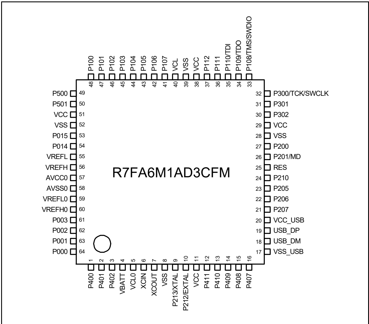
図 1.5 64-pin LQFP のピン配置図 (上面図)
