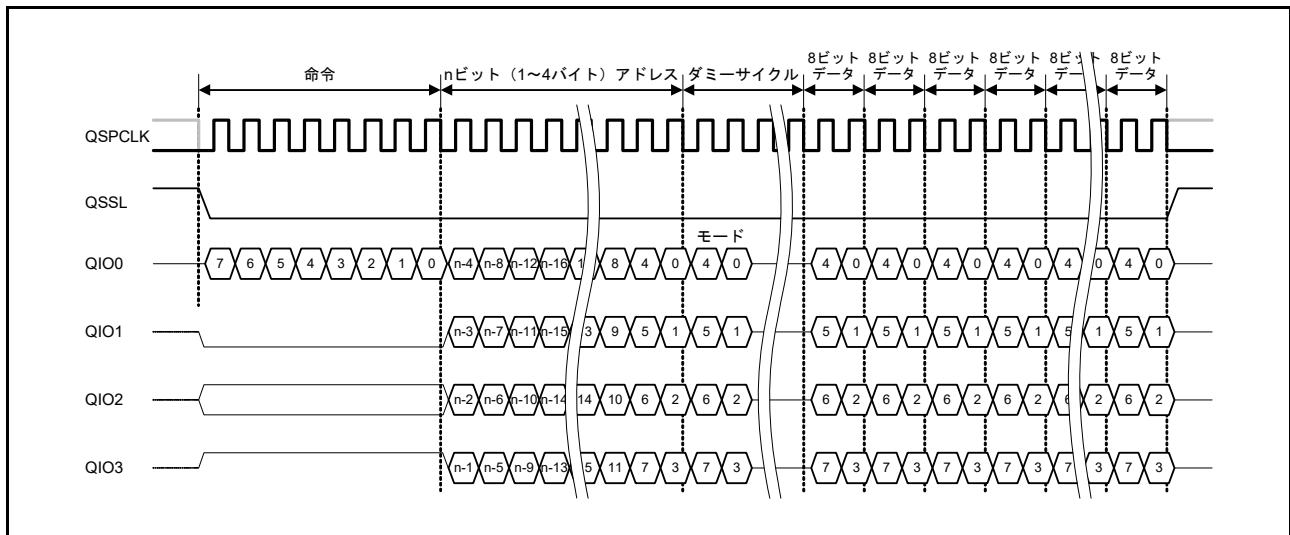
図 35.5 拡張 SPI プロトコル例 2 (ファストリード Quad I/O)
