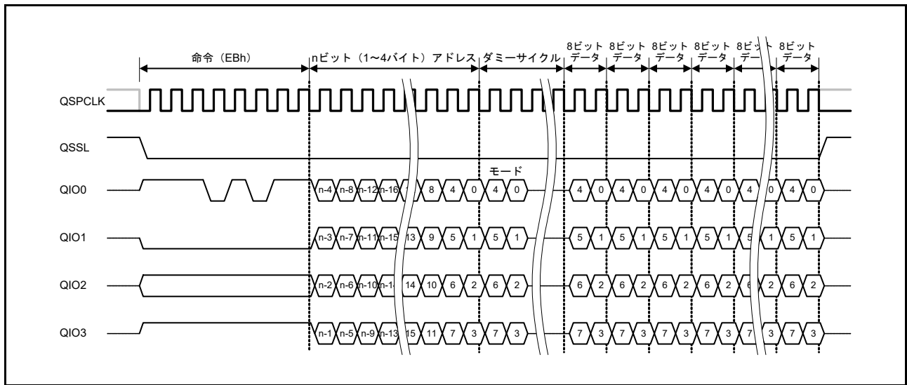
図 35.25 ファストリード Quad I/O バスサイクル
