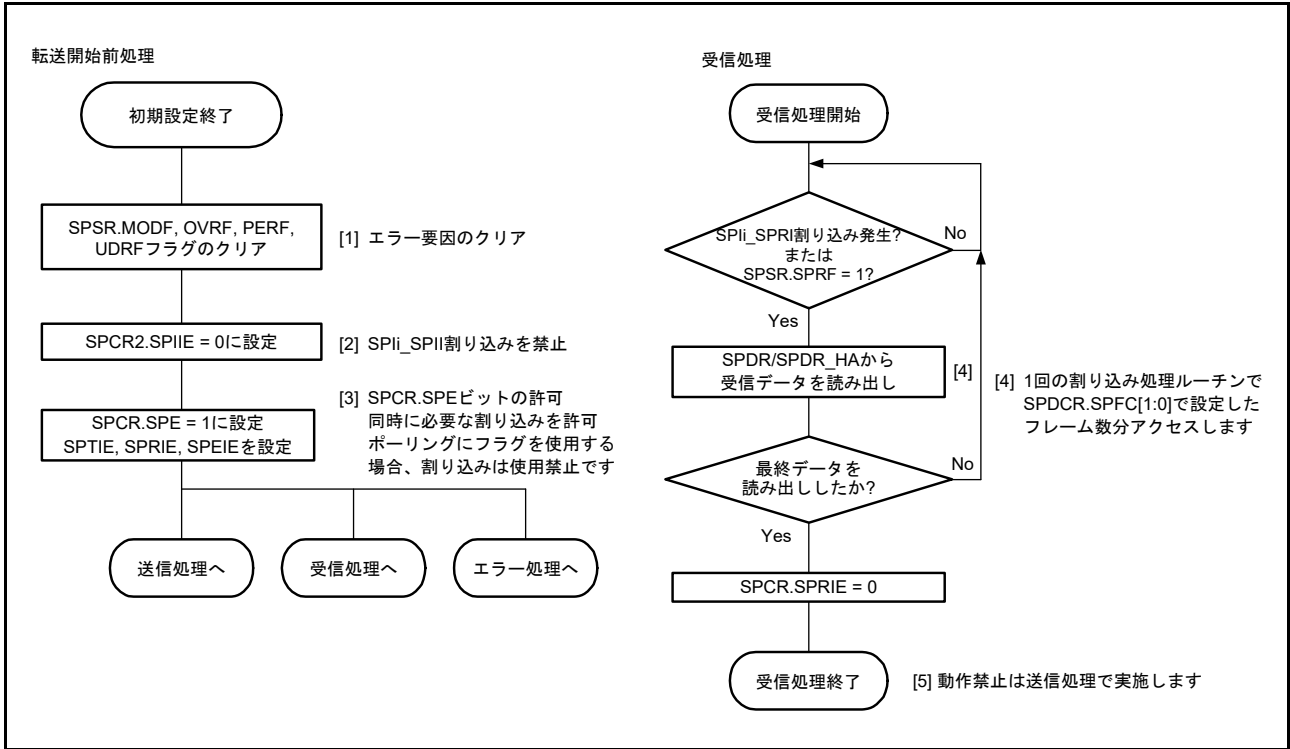
図 34.38 マスタモードでの受信フロー
