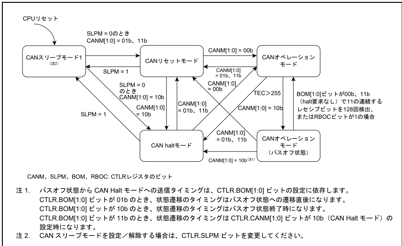
図 33.9 各動作モード間の遷移
