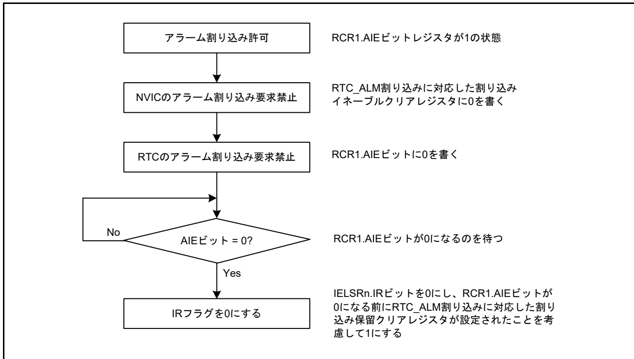
図 26.8 アラーム割り込み要求の禁止手順
