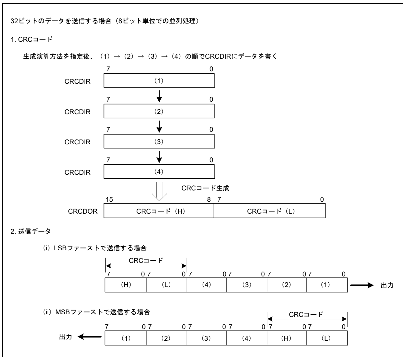
図 36.6 LSB ファーストと MSB ファーストのデータ送信
