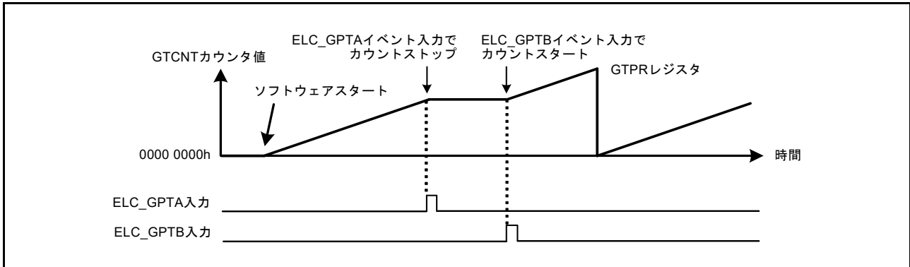
図 23.53 ハードウェア要因によるカウントストップ動作例 (ソフトウェアによるスタート、ELC_GPTA 入力でのストップ、ELC_GPTB 入力での再スタートの場合)
