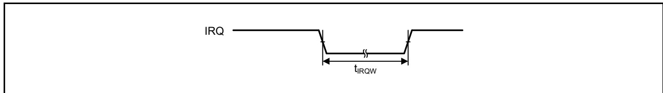
図 52.19 IRQ 割り込み入力タイミング
