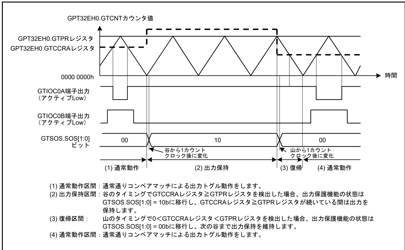
図 23.103 谷でのバッファ転送中に GTCCRA レジスタ \geq GTPR レジスタとなった場合の出力保護機能の動作例 (山でのバッファ転送中に 0 < GTCCRA レジスタ < GTPR レジスタを回復、アクティブ Low の場合)
