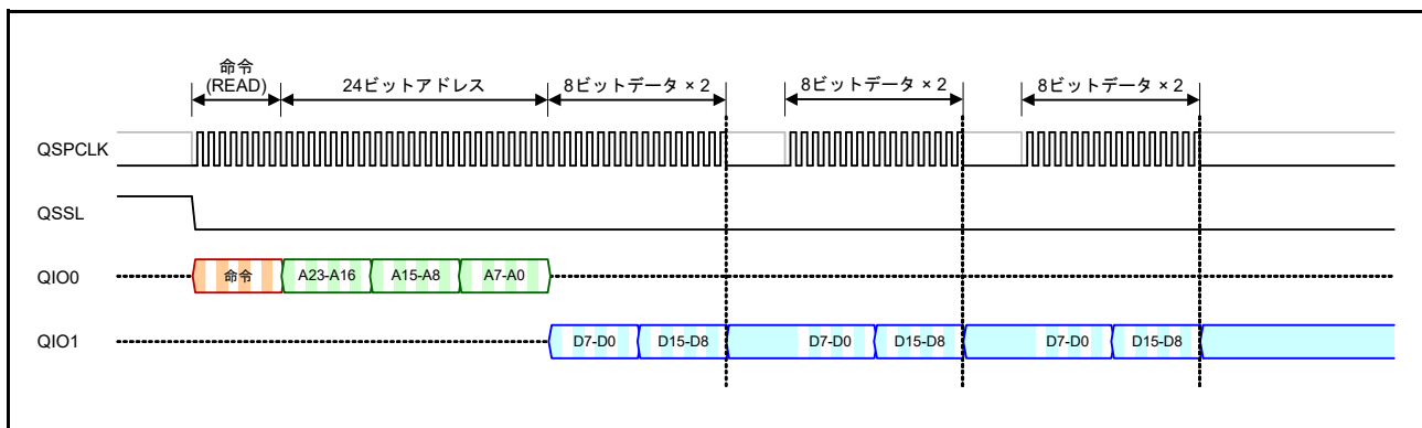
図 35.32 SPI バスサイクル拡張を使用した連続データのリード動作
