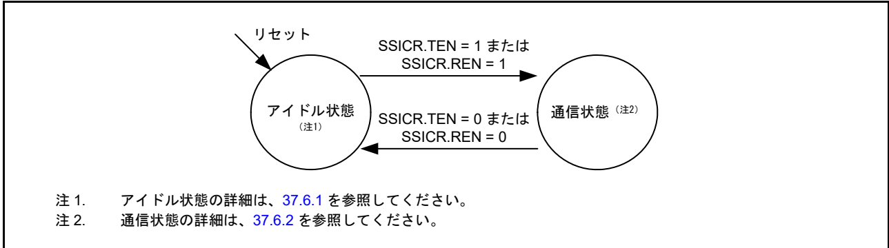
図 37.42 SSIE の状態遷移
