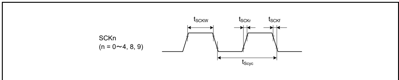
図 52.36 SCK クロック入出力タイミング
