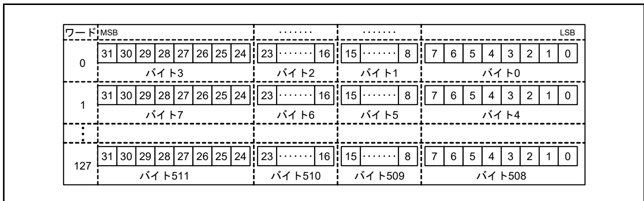
図 39.4 SD_BUF 格納データ
