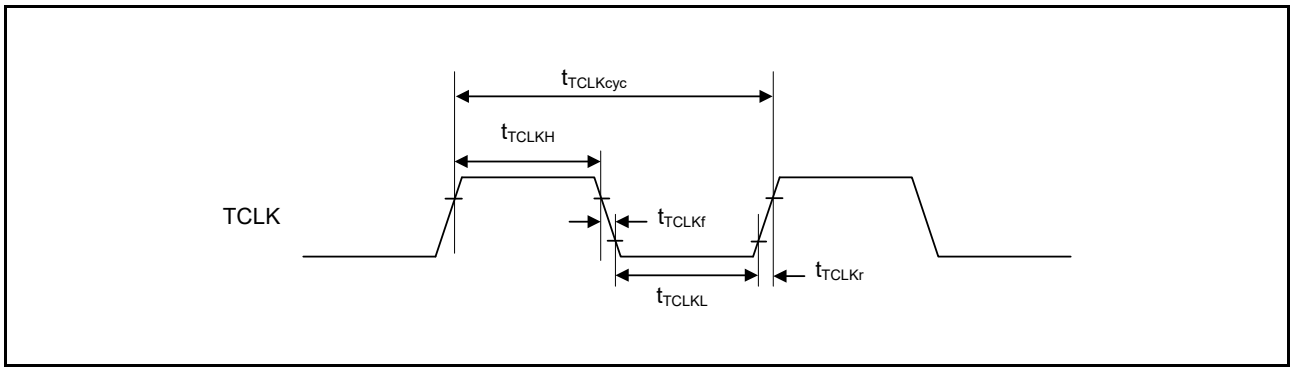
図 52.79 ETM TCLK タイミング
