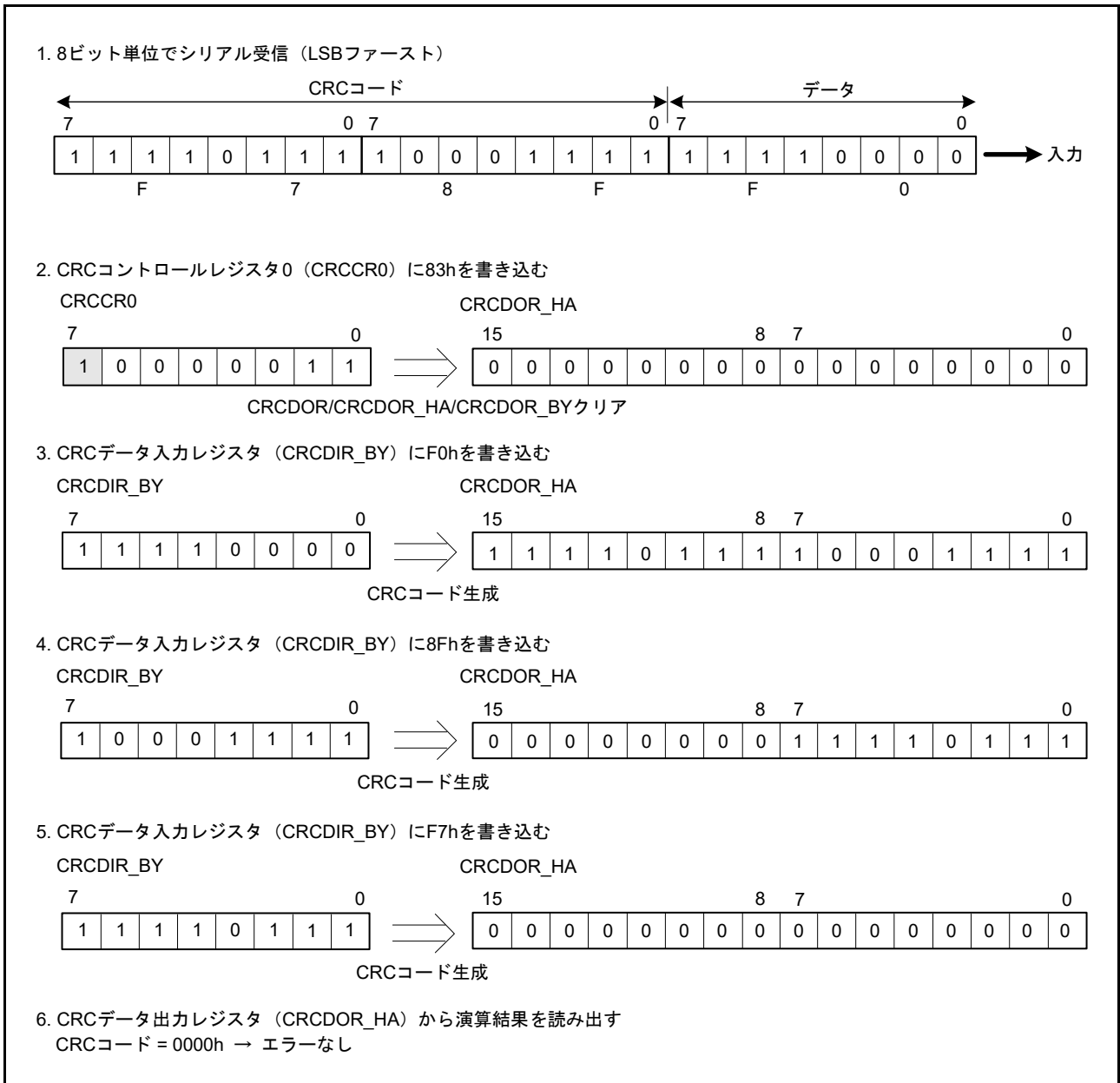
図 36.4 LSB ファーストのデータ受信
