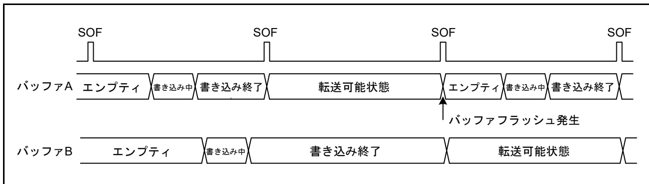
図 29.21 バッファフラッシュ動作例
