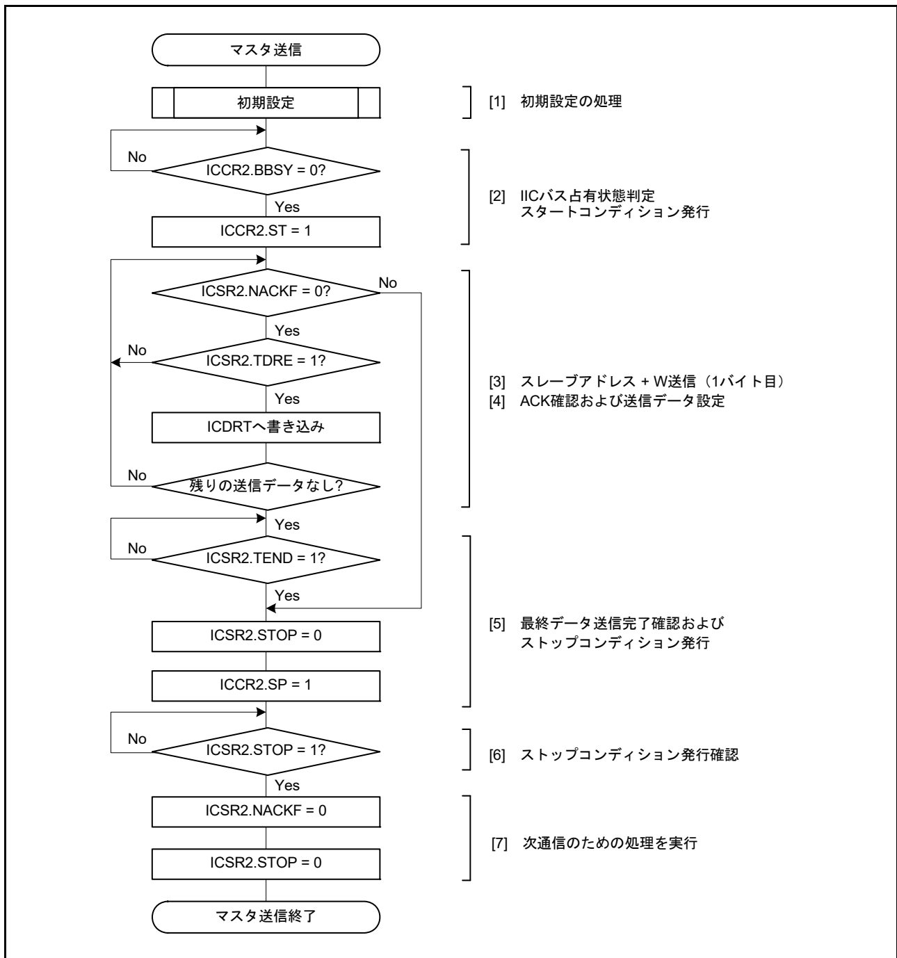
図 32.6 マスタ送信のフロー例
