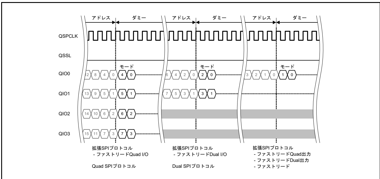
図 35.33 XIP モード制御データ
