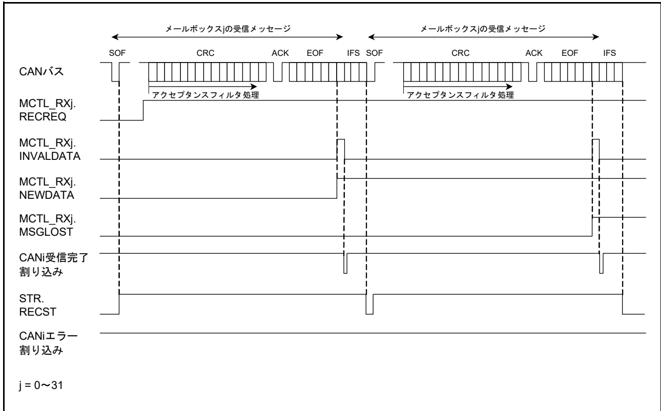
図 33.18 データフレーム受信時の動作例（オーバーライトモードの場合）
