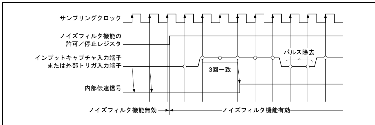
図 23.94 ノイズフィルタのタイミング
