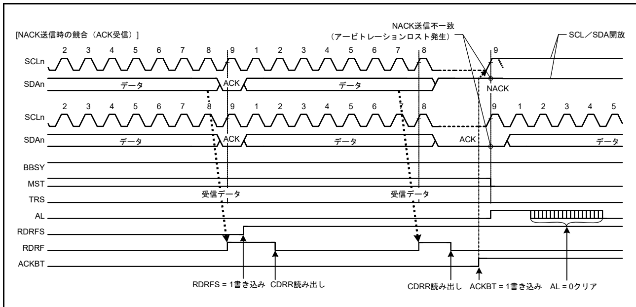
図 32.43 NACK 送信中のアービトレーションロスト検出の動作例 (NALE = 1 の場合)
