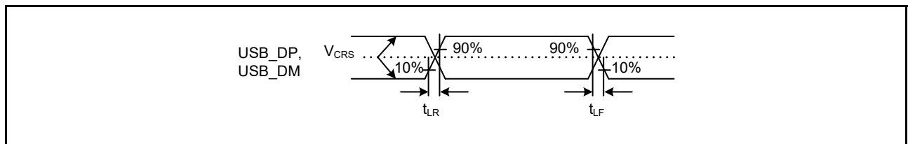
図 52.60 Low-speed モードにおける USB_DP、USB_DM の出力タイミング
