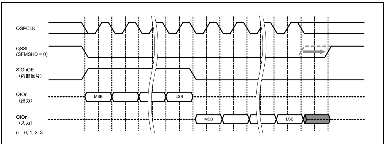
図 35.11 SFMSHD ビットを使用した QSSL 信号のホールド時間調整
