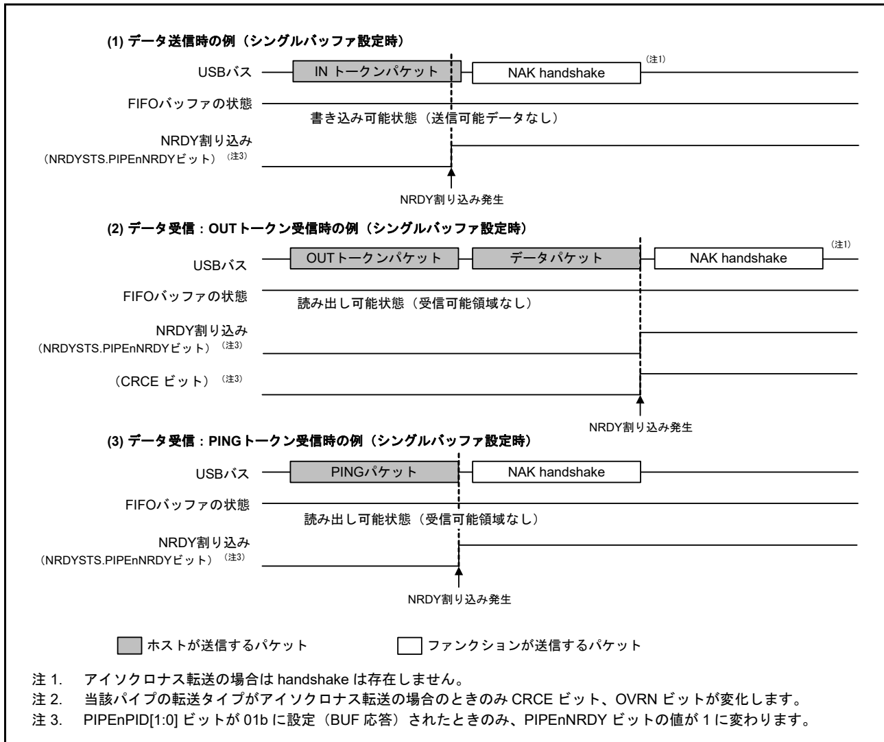
図 29.12 デバイスコントローラモード時の NRDY 割り込み発生タイミング
