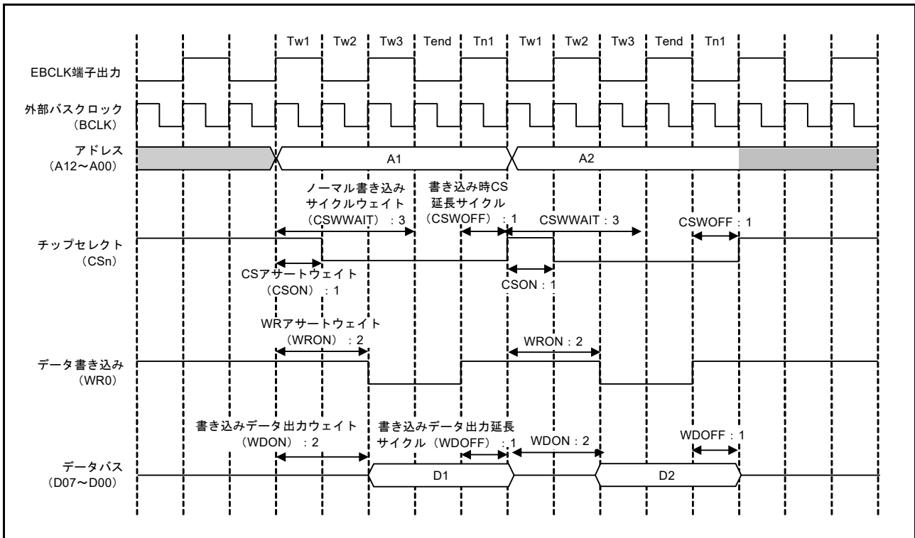
図 15.14 ノーマルライトアクセスの動作例 (EBCLK 端子出力選択ビットで BCLK の 2 分周を設定した場合、および 1 転送要求に対して 2 回バスアクセスが発生する場合) (n = 0, 1, 4 ~ 7)
