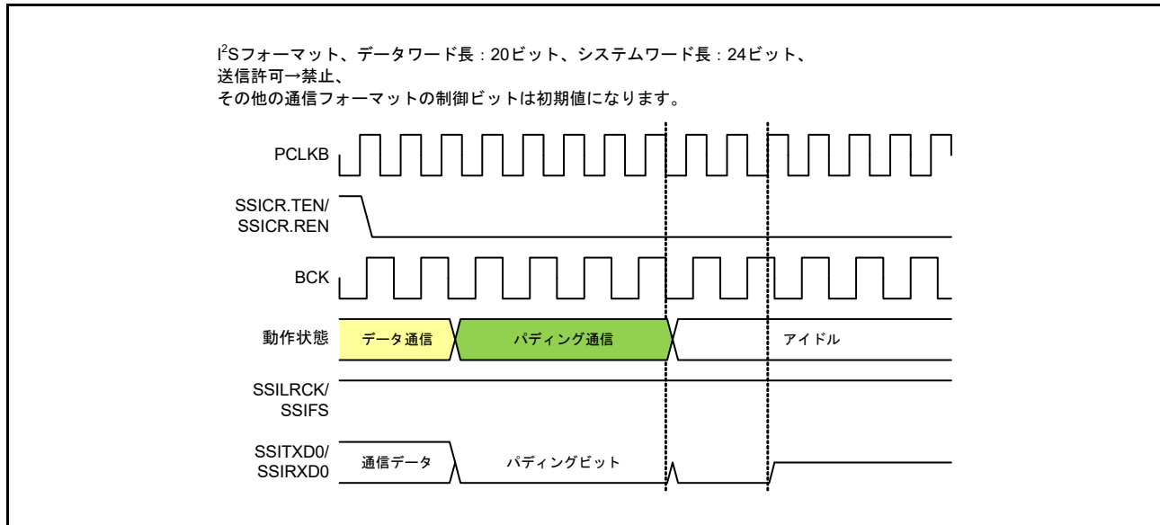
図 37.50 パディング通信からの停止
