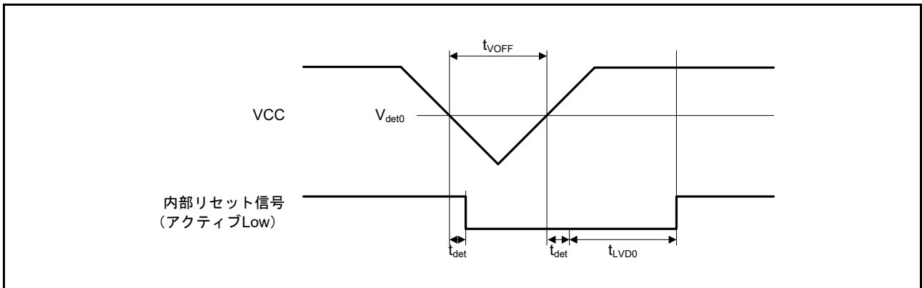
図 52.67 電圧検出回路タイミング ( V_{det0} )
