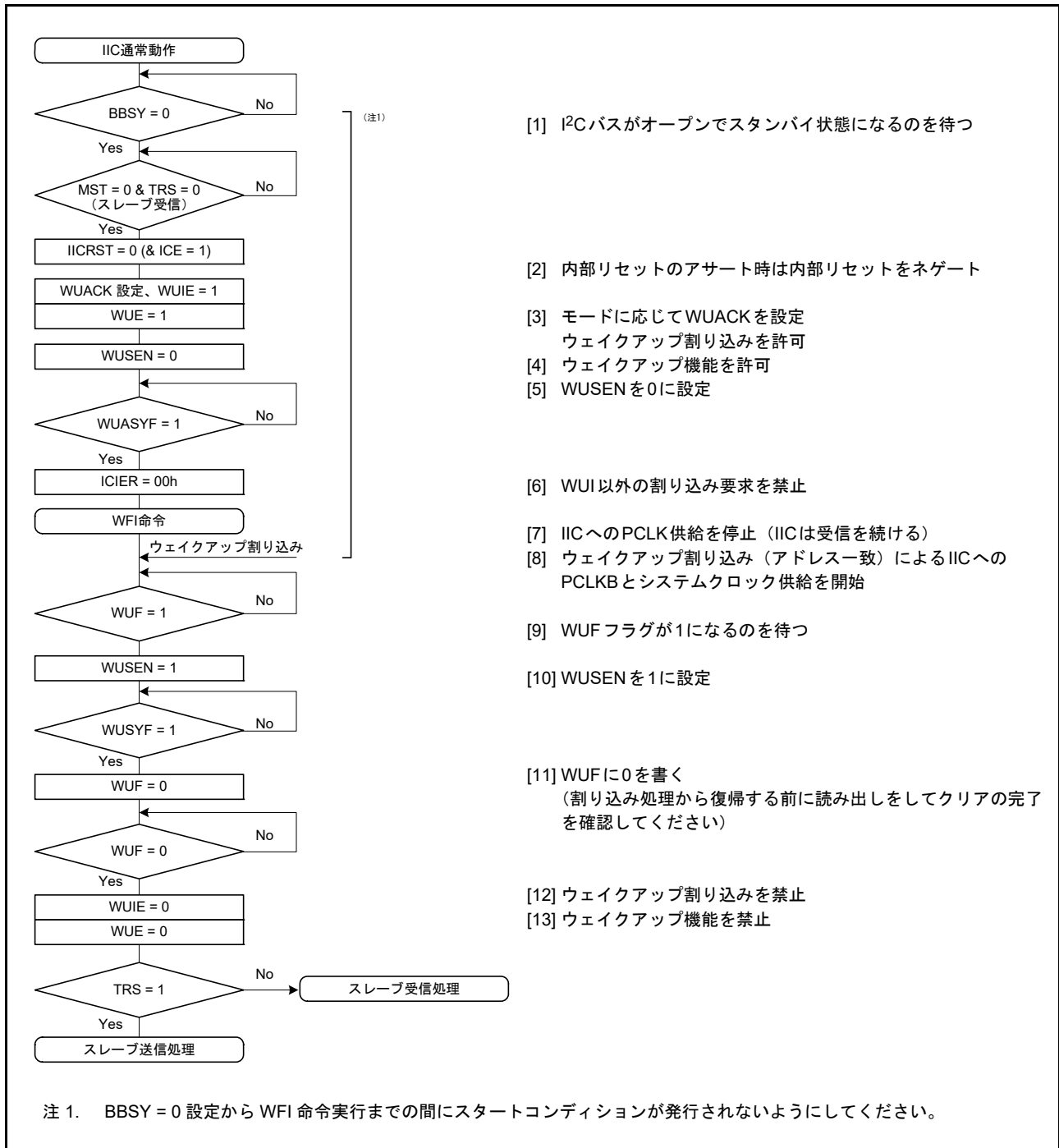
図 32.30 ノーマルウェイクアップモード1の動作例 (スレーブアドレス一致時のウェイクアップ割り込みによるウェイクアップの場合)
