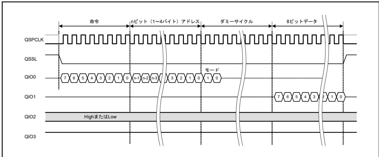
図 35.4 拡張 SPI プロトコル例 1 (ファストリード)
