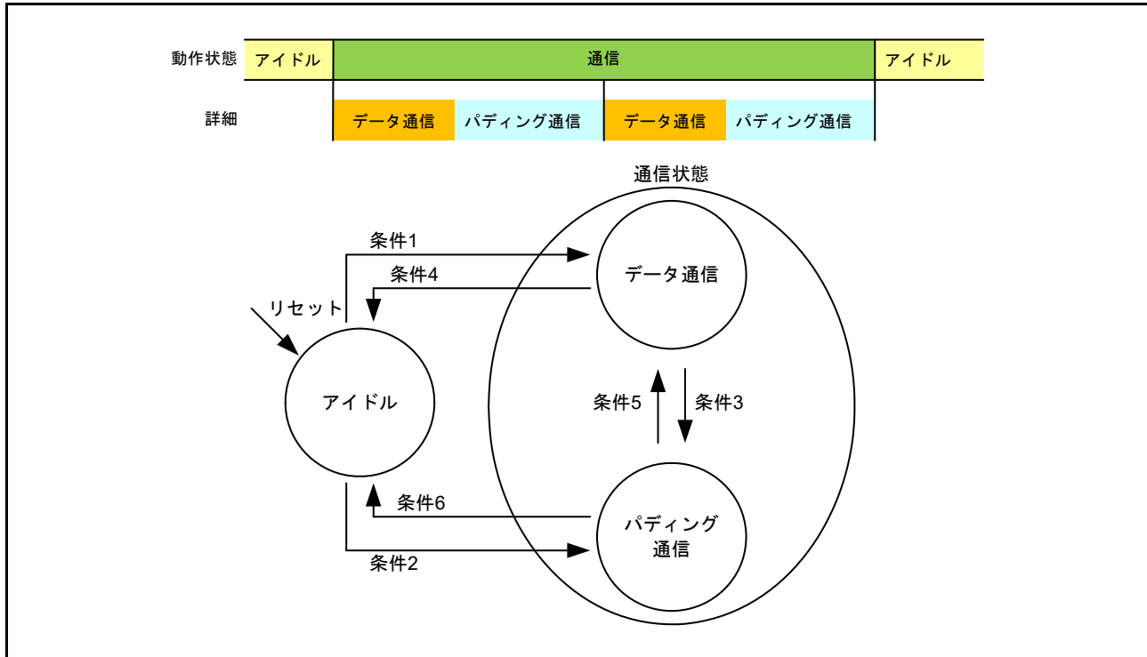
図 37.45 通信の状態遷移
