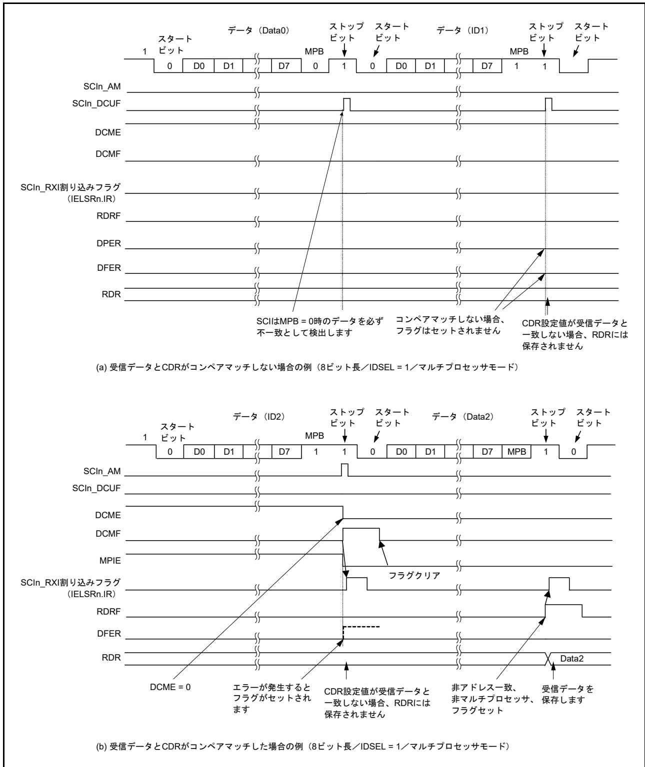
図 30.6 アドレス一致検出の例 (2) (マルチプロセッサモード)
