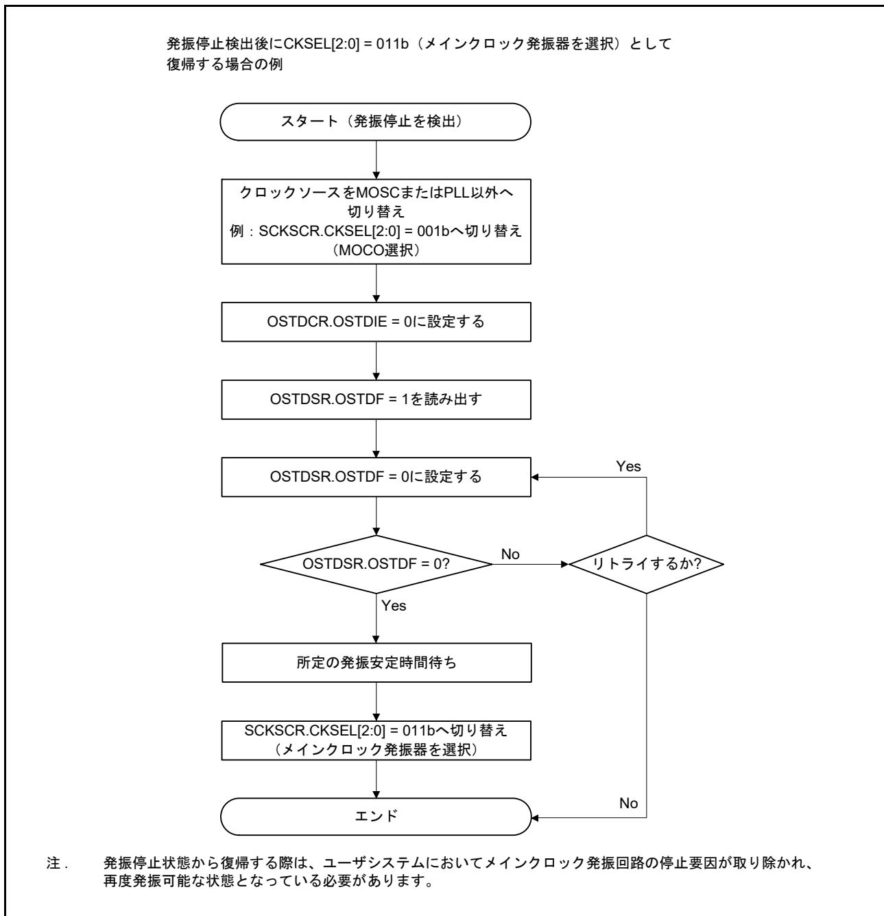
図 9.12 発振停止検出時の復帰フロー
