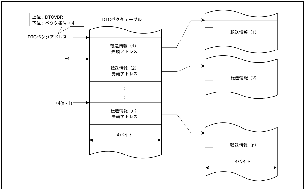
図 18.2 DTC ベクタテーブルと転送情報の対応関係
