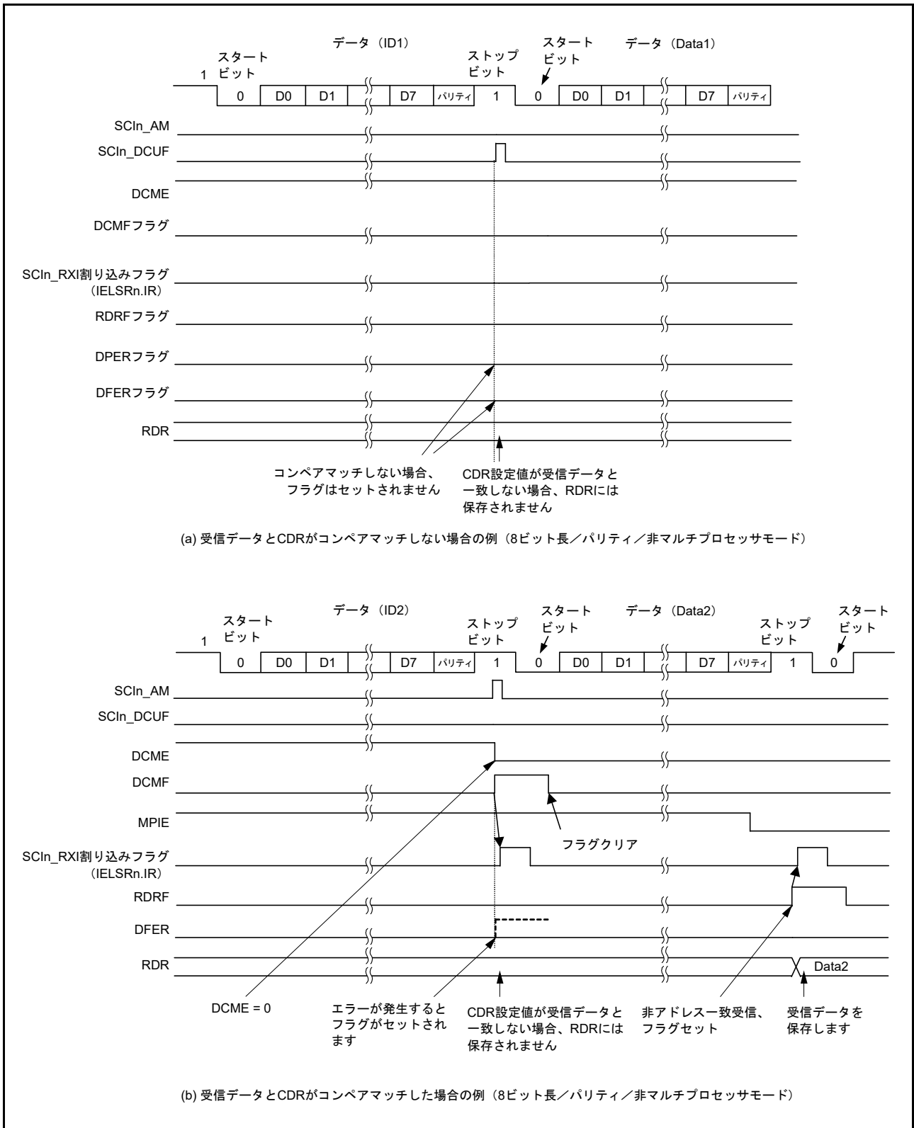
図 30.5 アドレス一致検出の例 (1) (非マルチプロセッサモード)
