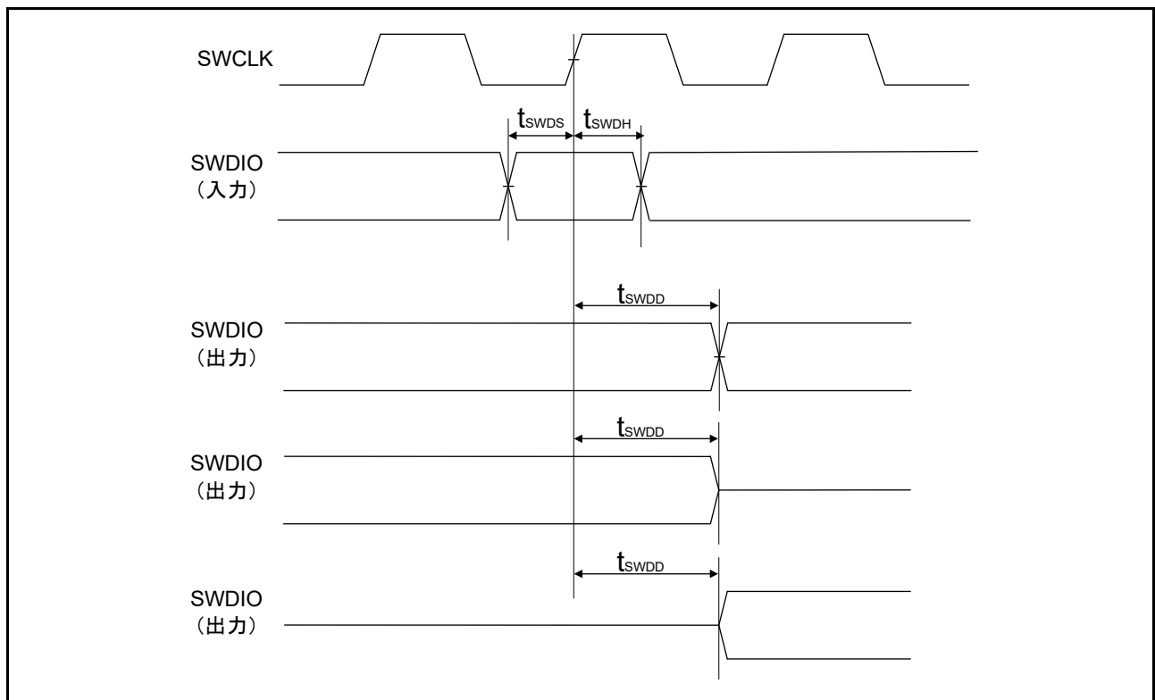
図 52.78 SWD 入出力タイミング
