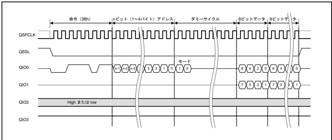
図 35.19 ファストリード Dual 出力バスサイクル
