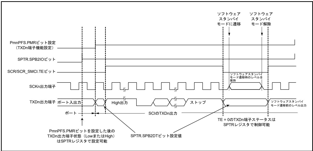
図 30.74 ソフトウェアスタンバイモード移行中のポートの端子状態 (内部クロック、調歩同期送信)
