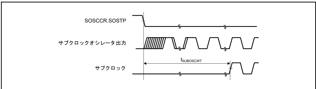
図 52.12 サブクロック発振開始タイミング
