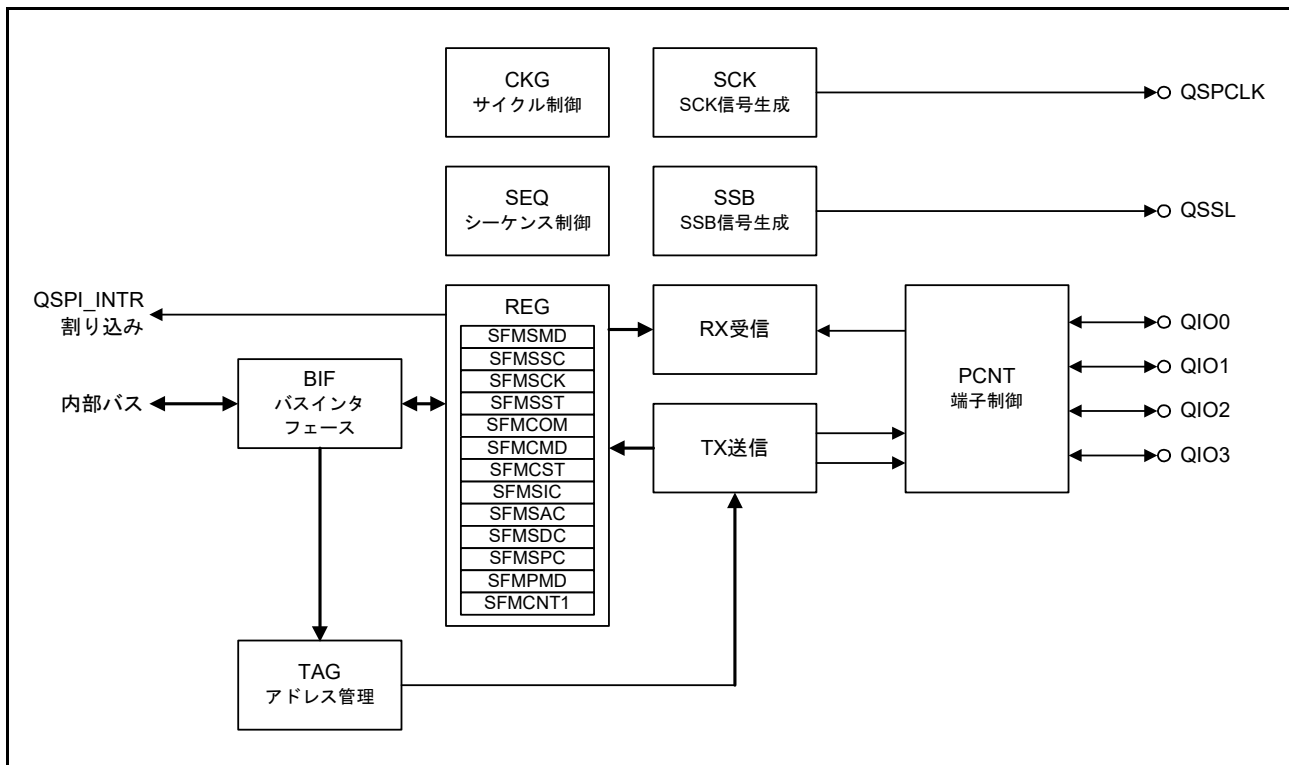
図 35.1 QSPIのブロック図
