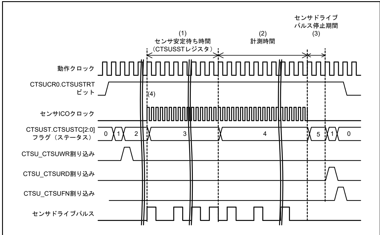
図 46.18 センサ安定待ちと計測のタイミング
