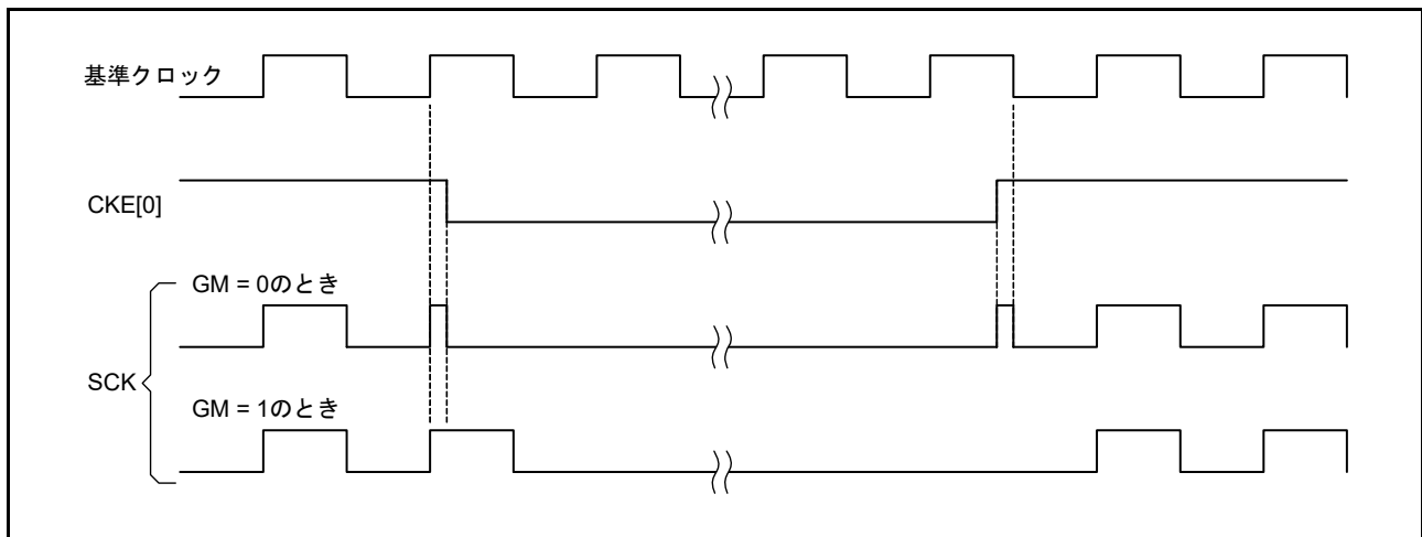
図 30.57 クロック出力制御
