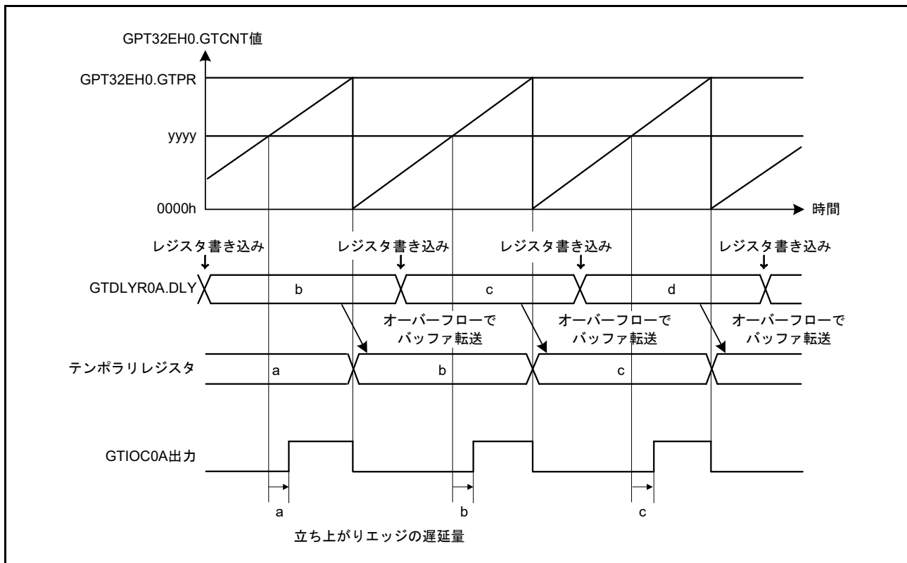
図 24.3 GTDLYR0A レジスタの動作例（PWMのこぎり波生成時）
