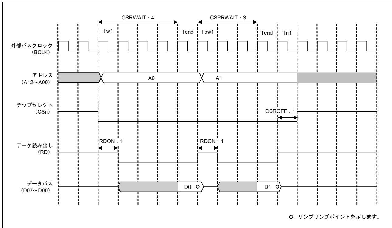
図 15.17 ページリードアクセスの動作例 (8 ビットバス空間に対する 16 ビットアクセスの場合) (n = 0, 1, 4 ~ 7)
