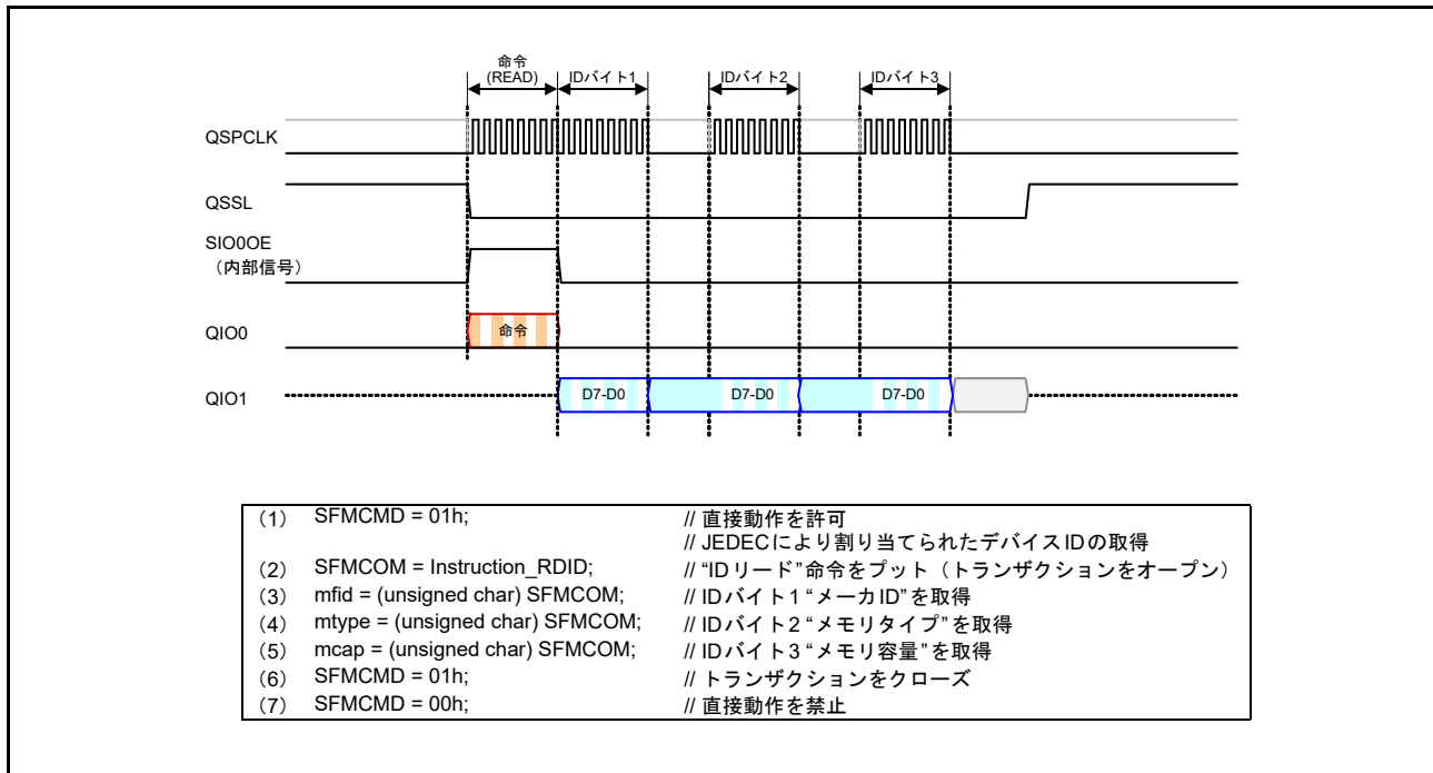
図 35.34 ID リードの直接通信タイミング例
