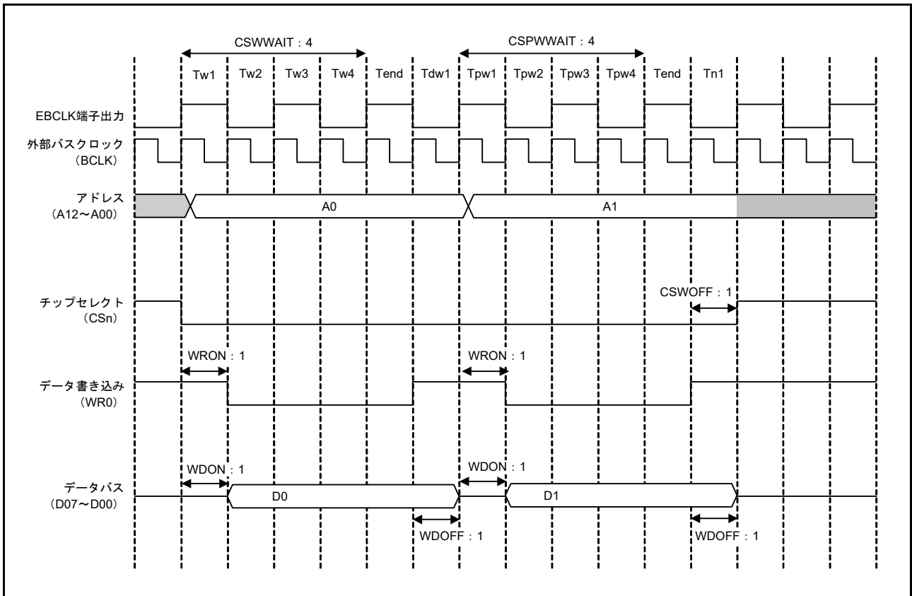
図 15.20 ページライトアクセスの動作例 (EBCLK 端子出力選択ビットで BCLK の 2 分周を設定した場合、および 1 転送要求に対して 2 回バスアクセスが発生する場合、バイトストローブモード時) (n = 0, 1, 4 ~ 7)
