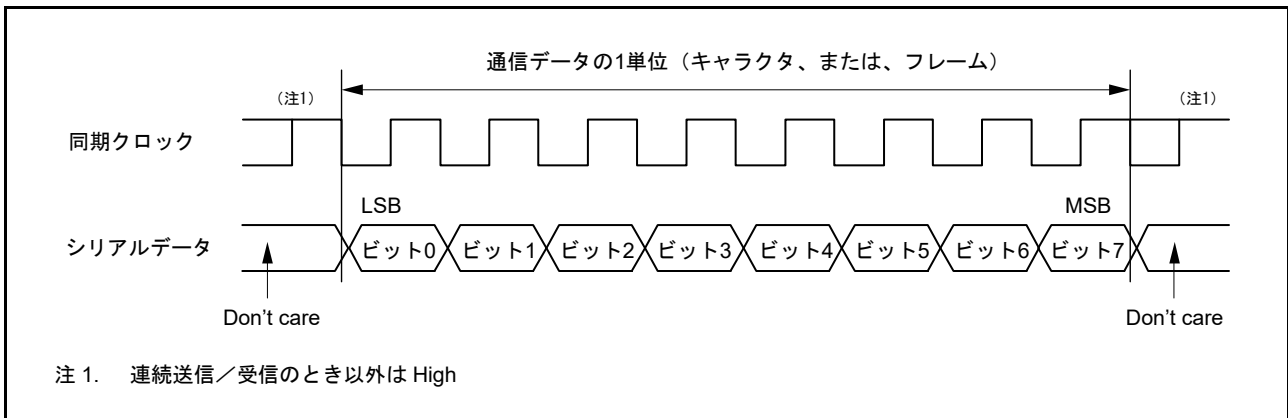
図 30.31 クロック同期式シリアル通信のデータフォーマット (LSB ファーストの場合)
