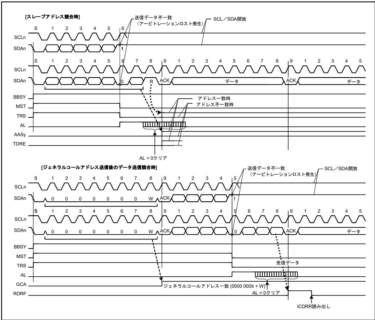
図 32.41 マスタアービトレーションロスト検出の動作例 (MALE = 1 の場合)
