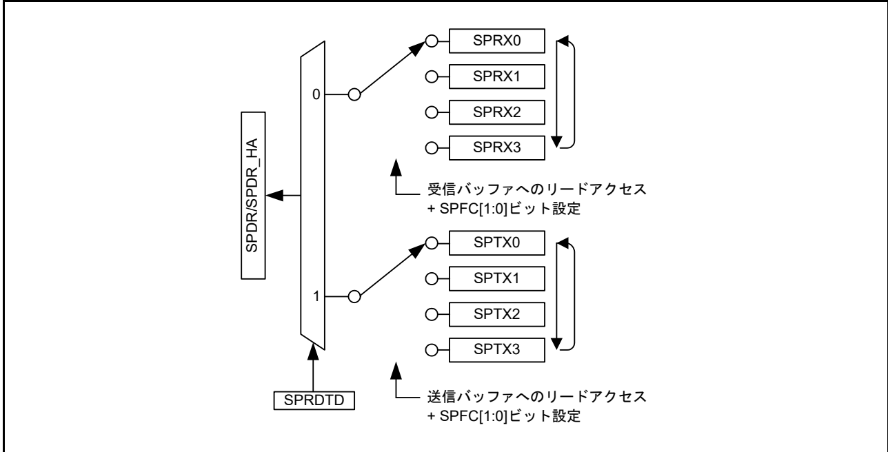
図 34.4 読み出し時の SPDR/SPDR_HA レジスタの構成図
