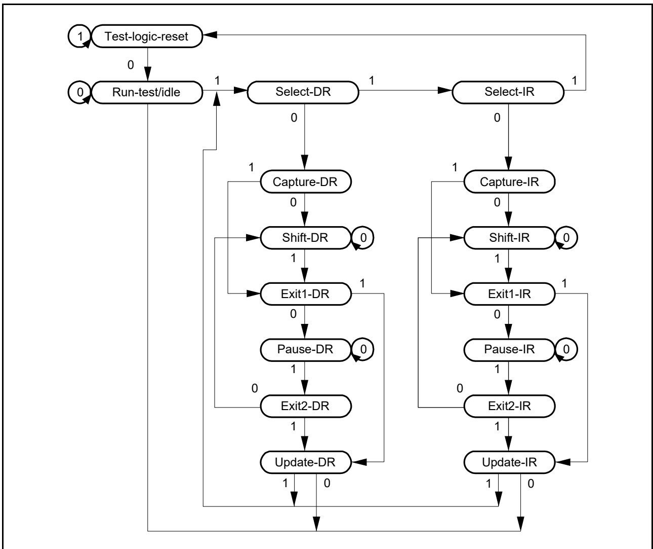
図 40.2 TAP コントローラの状態遷移図
