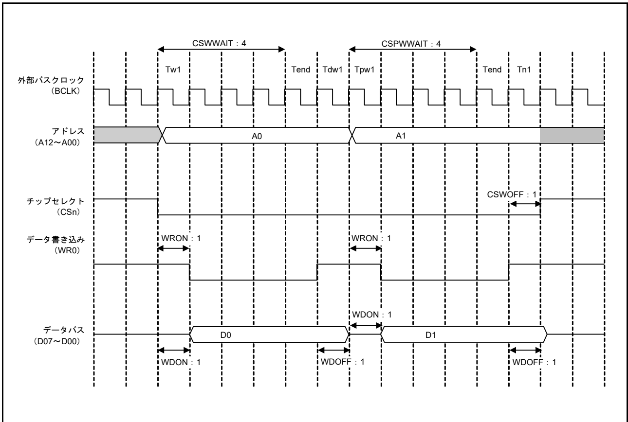
図 15.18 ページライトアクセスの動作例 (8 ビットバス空間に対する 16 ビットアクセスの場合、1 ライトストロブモード時) (n = 0, 1, 4 ~ 7)
