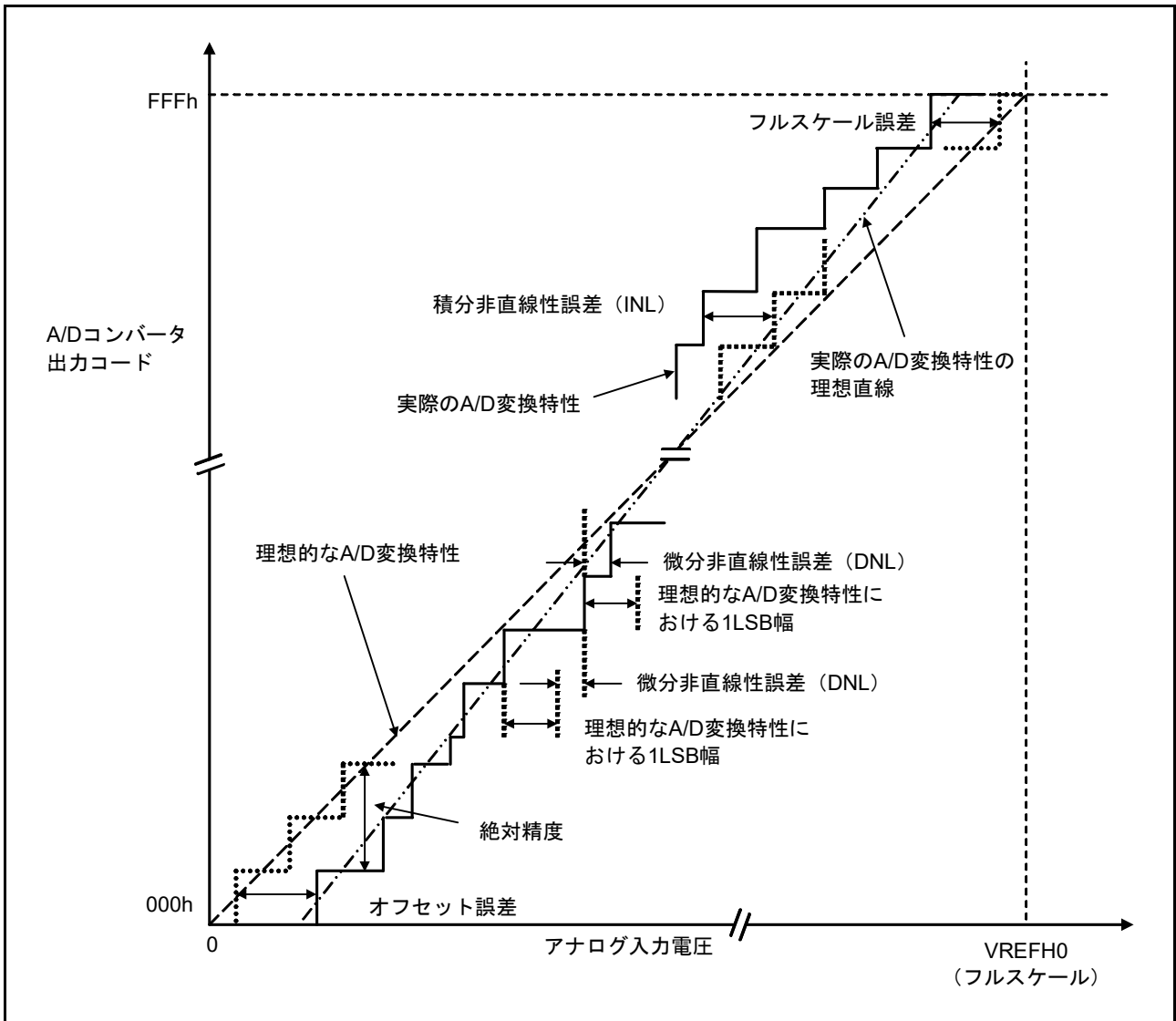
図 52.64 ADC12 特性用語の解説図
