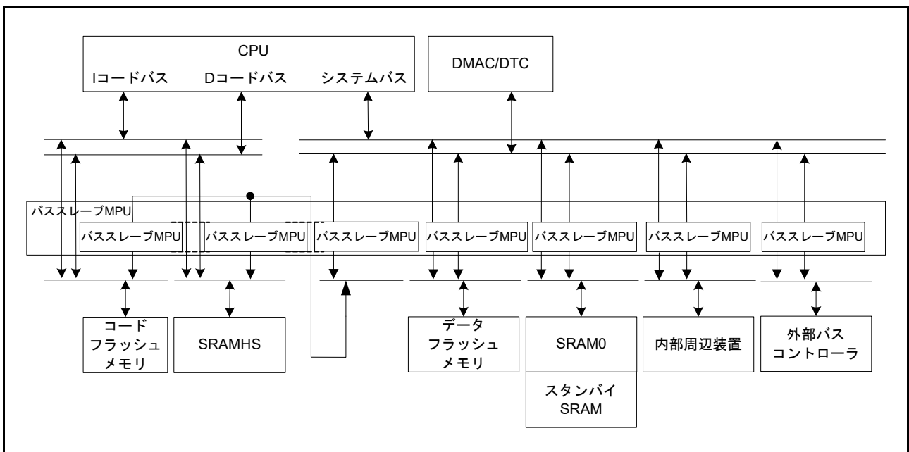
図 16.9 バススレーブ MPU ブロック図
