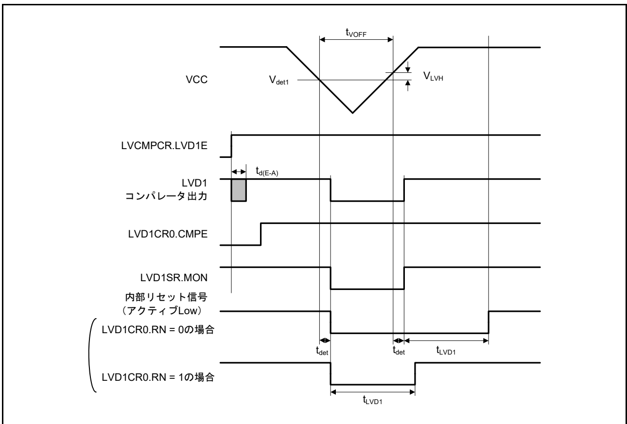
図 52.68 電圧検出回路タイミング ( V_{det1} )
