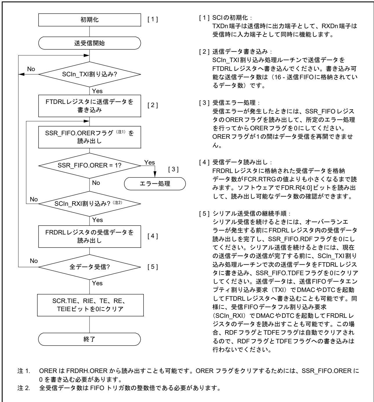
図 30.44 クロック同期式モードにおけるシリアル同時送受信動作のフローチャート例 (FIFO 選択時)
