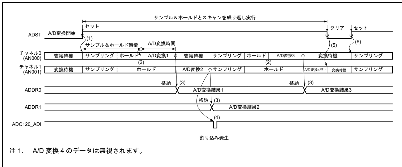
図 42.17 連続スキャンモードの動作例 (チャンネル専用サンプル&ホールド回路使用、AN000 および AN001 選択)
