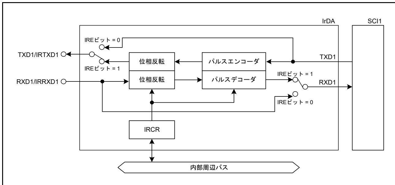
図 31.1 IrDA インタフェースと SCI1 の連携
