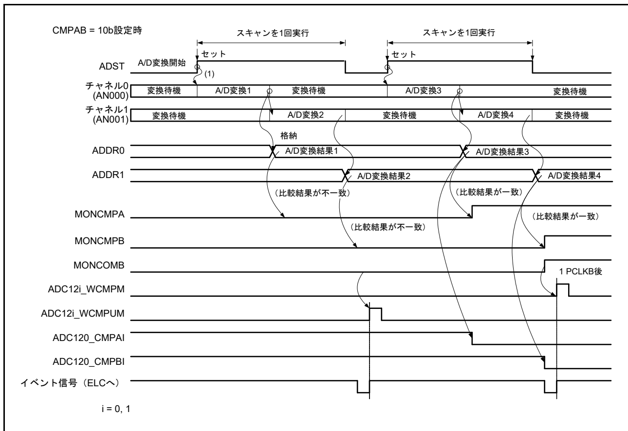
図 42.33 コンペア機能のイベント出力動作例 (AN000 ~ AN001 を比較)
