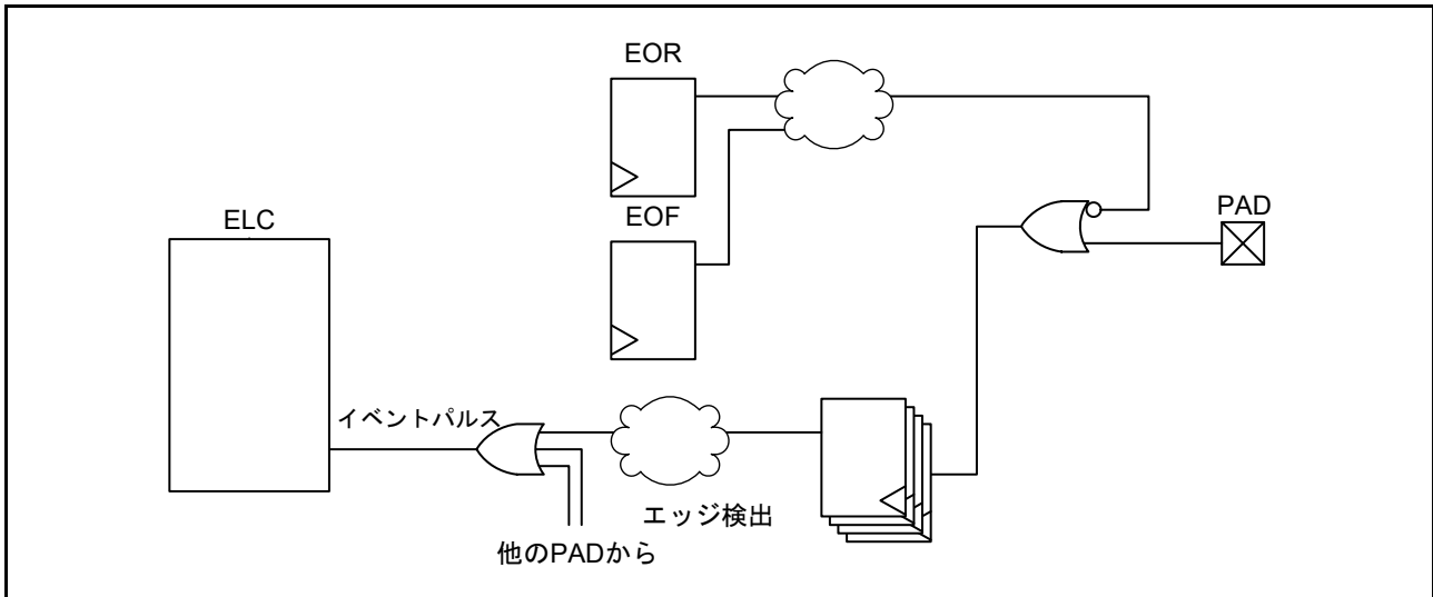
図 20.4 イベントパルスの発生
