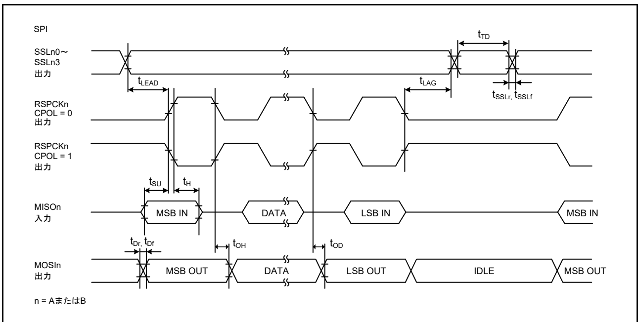
図 52.45 CPHA = 0 の場合におけるマスタの SPI タイミング
