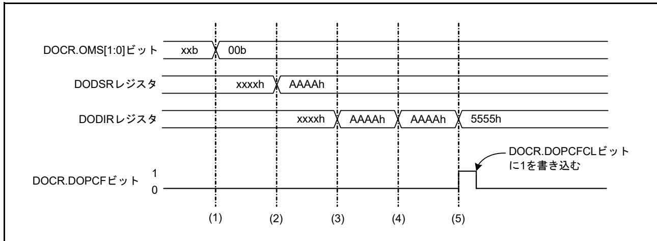
図 47.2 データ比較モードの動作例
