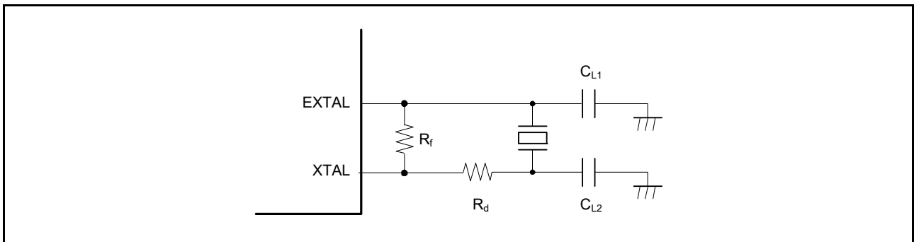
図 9.6 水晶振動子の接続例
