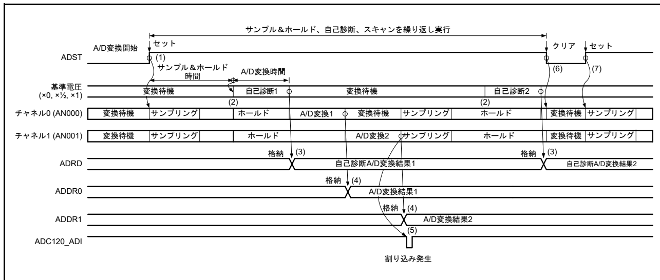
図 42.20 連続スキャンモードの動作例 (チャンネル専用サンプル&ホールド回路使用、AN000 および AN001 選択 + 自己診断)
