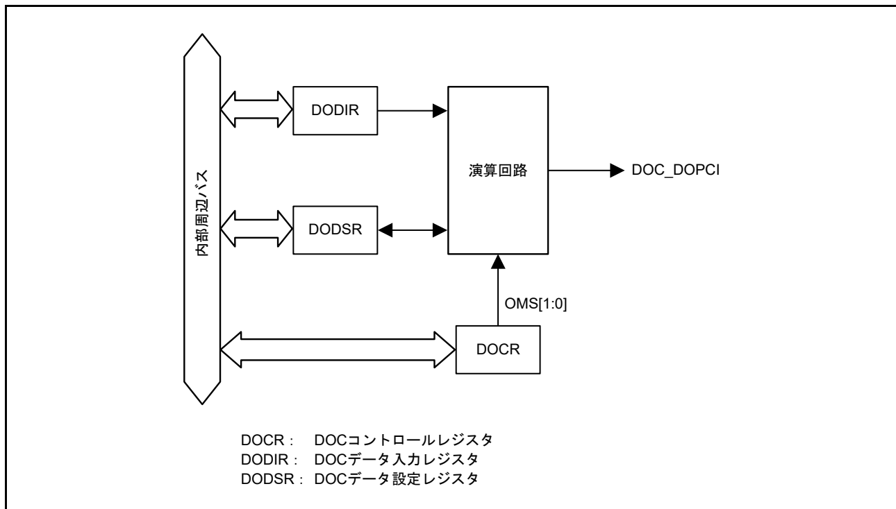
図 47.1 DOC ブロック図
