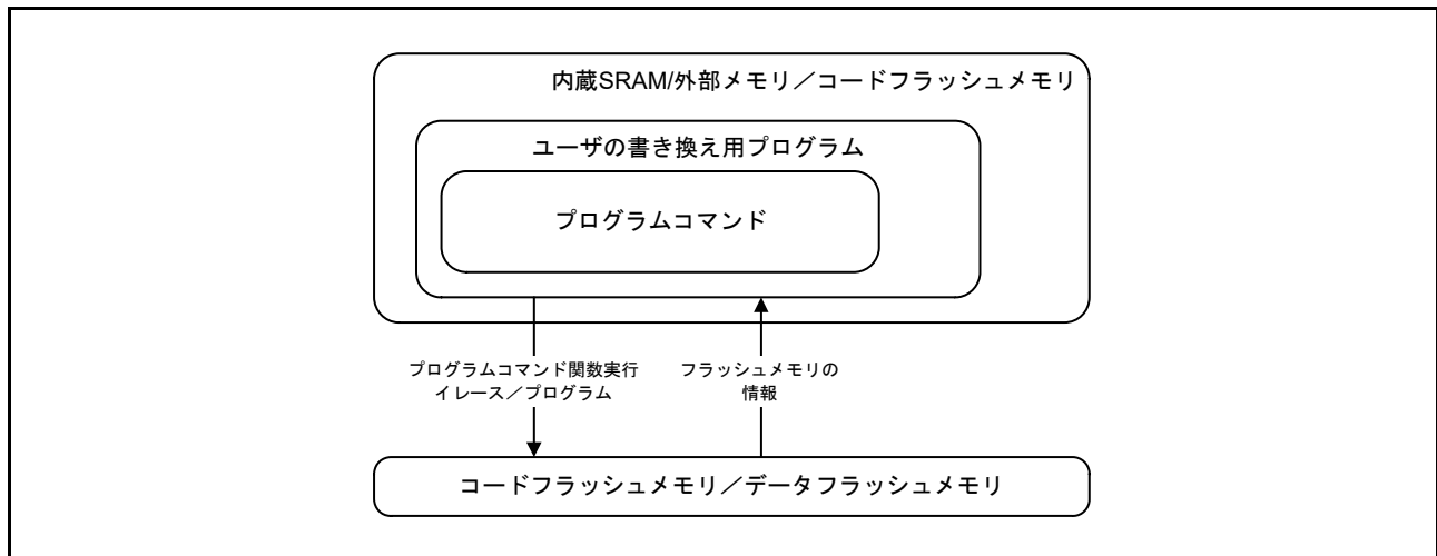
図 50.15 セルフプログラミングの概念
