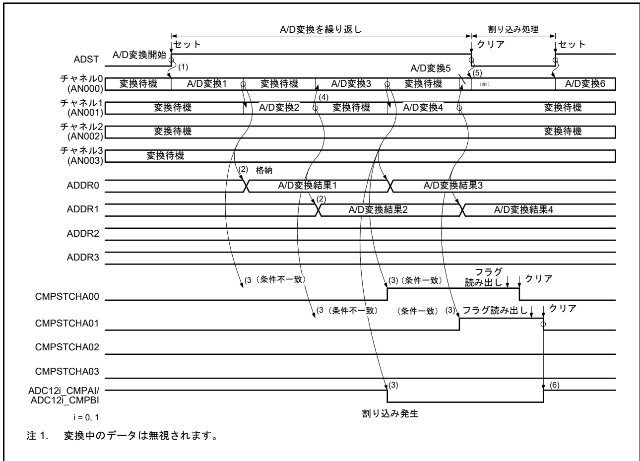
図 42.31 コンペア機能の動作例 (AN000 ~ AN003 を比較)
