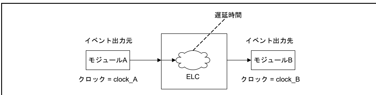
図 19.2 ELC 遅延時間
