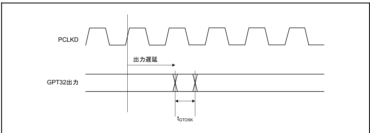
図 52.31 OPS の GPT32 出力遅延スキュー
