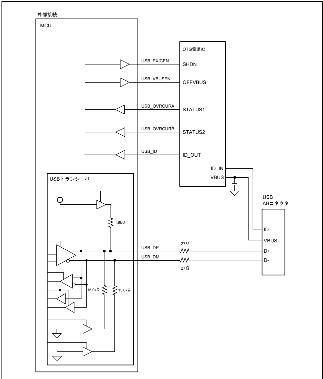
図 29.2 セルフパワー状態での OTG 接続例
