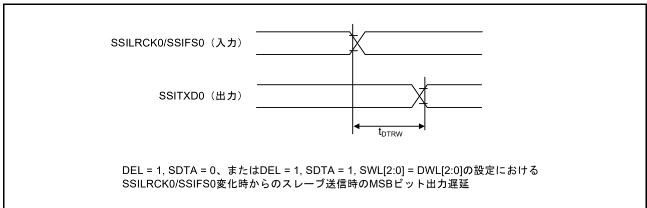
図 52.58 SSILRCK0/SSIFS0 変化時からの SSIE データ出力遅延
