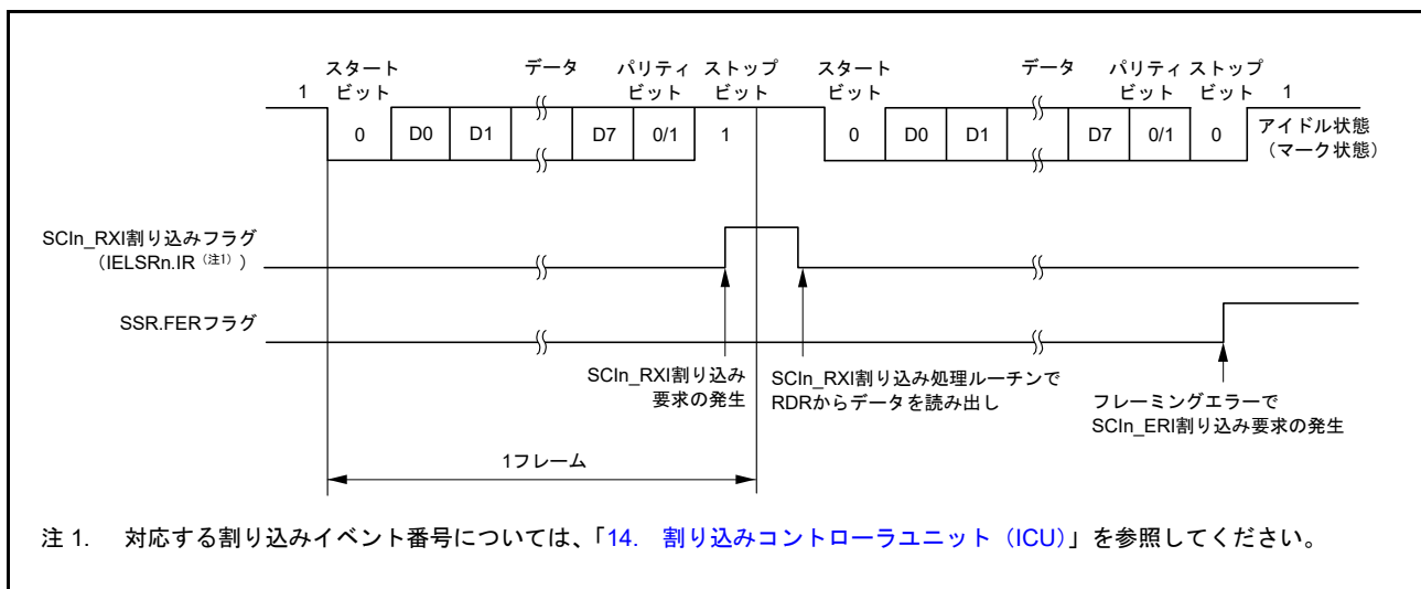
図 30.15 調歩同期式モードにおけるシリアル受信の動作例 (1) (RTS 機能を使用しない場合) (8 ビットデータ / パリティあり / 1 ストップビットの場合)
