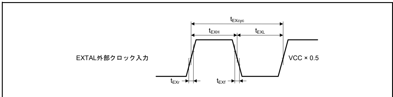
図 52.8 EXTERNAL 外部クロック入カタイミング
