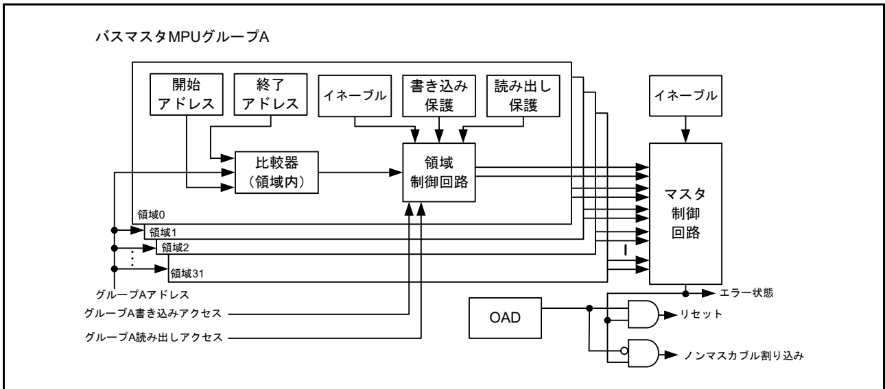
図 16.4 バスマスタ MPU グループ A
