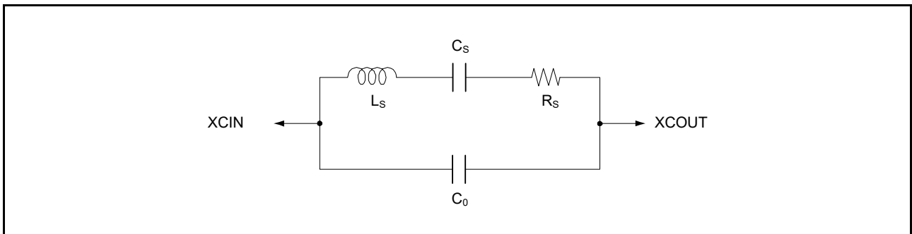
図 9.10 32.768kHz 水晶振動子の等価回路
