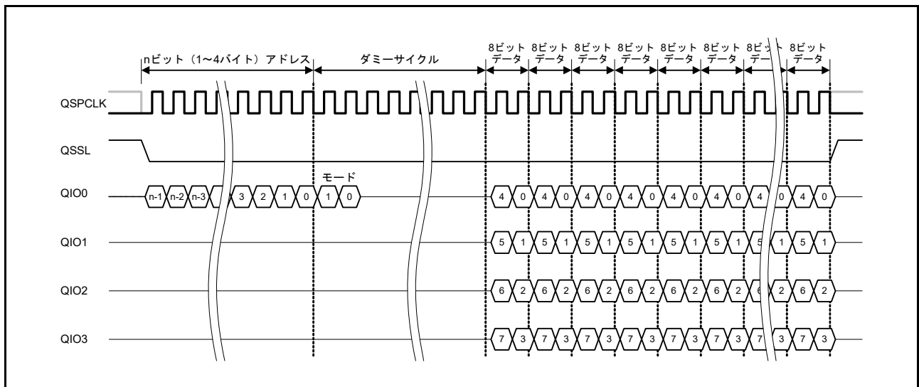
図 35.24 XIP モード時のファストリード Quad 出力バスサイクル
