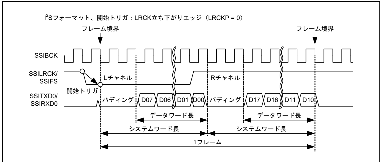
図 37.1 SSIE 通信フォーマット
