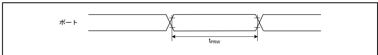
図 52.27 I/O ポート入力タイミング
