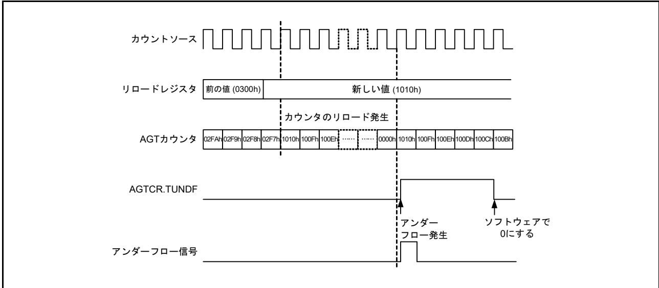
図 25.5 タイマモードでの動作例
