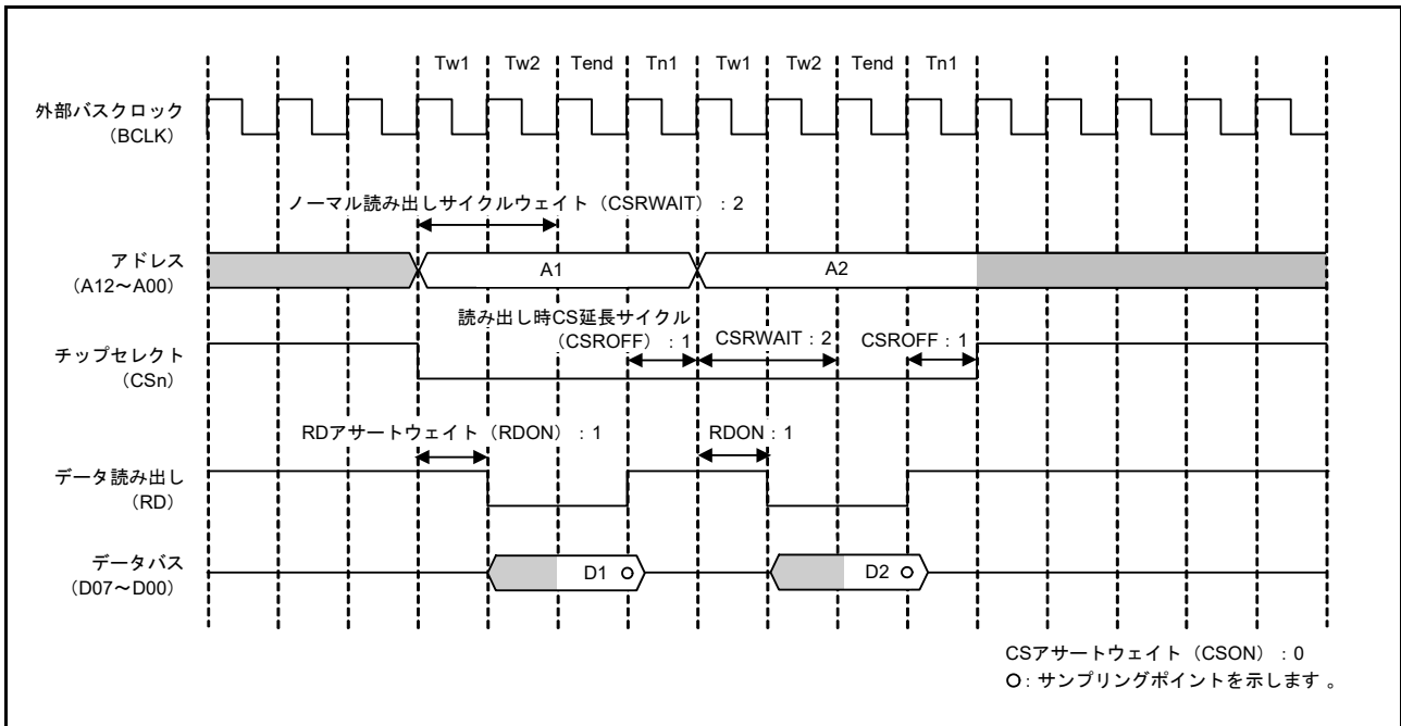
図 15.8 ノーマルリードアクセスの動作例 (1 転送要求に対して 2 回バスアクセスが発生する場合) (n = 0, 1, 4 ~ 7)
