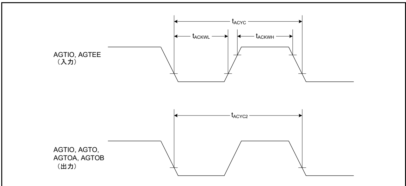
図 52.33 AGT 入出力タイミング
