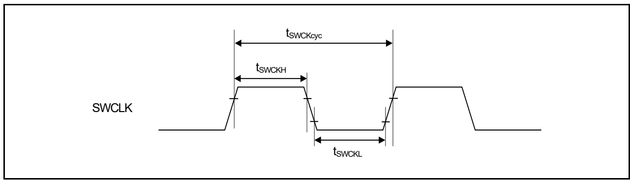
図 52.77 SWD SWCLK タイミング
