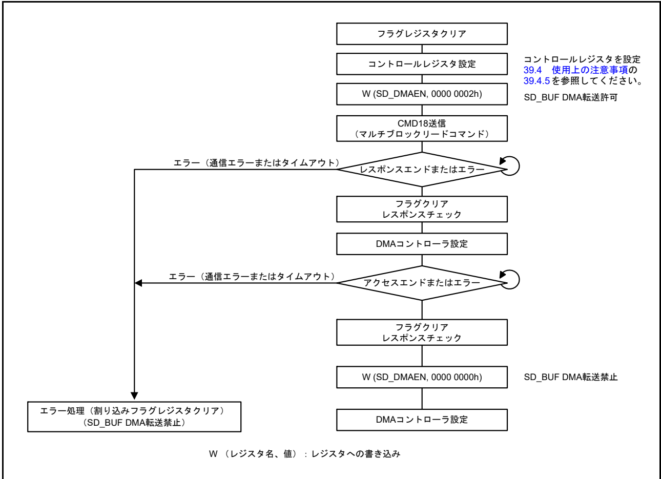
図 39.22 SD_BUF_DMA リード動作の例
