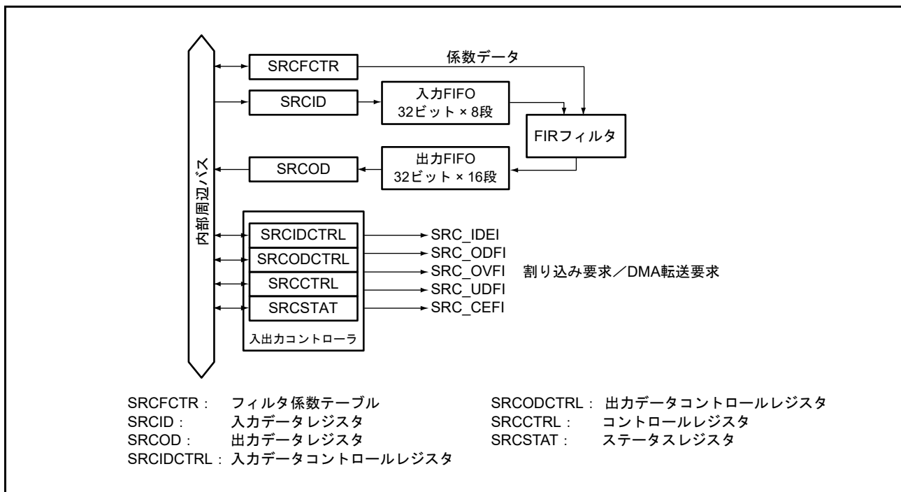
図 38.1 SRC のブロック図
