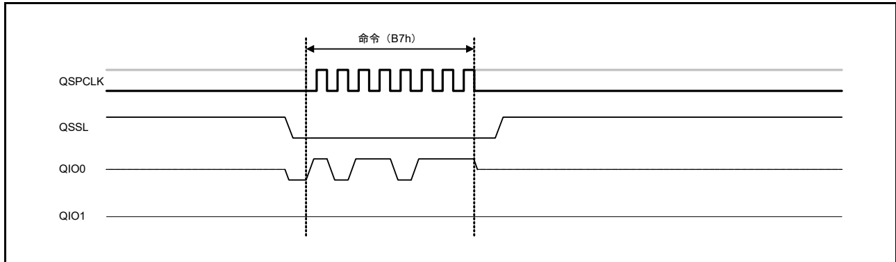
図 35.27 4 バイトモード遷移バスサイクル
