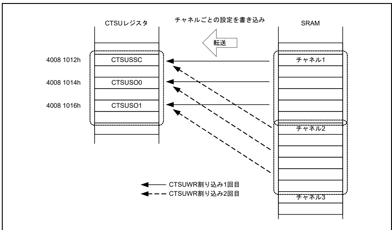
図 46.19 CTSU_CTSUWR 割り込みを用いた DTC 転送動作例
