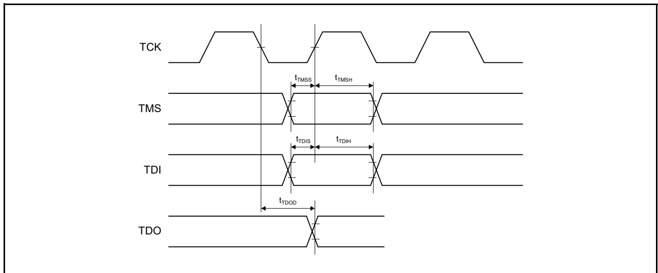
図 52.73 バウンダリスキャン入出力タイミング
