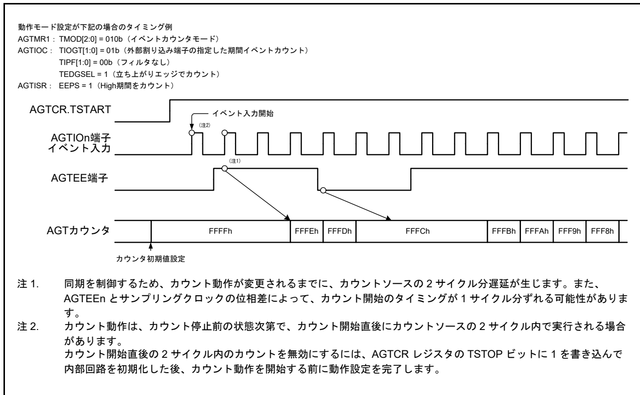
図 25.8 イベントカウンタモードでの動作例 2
