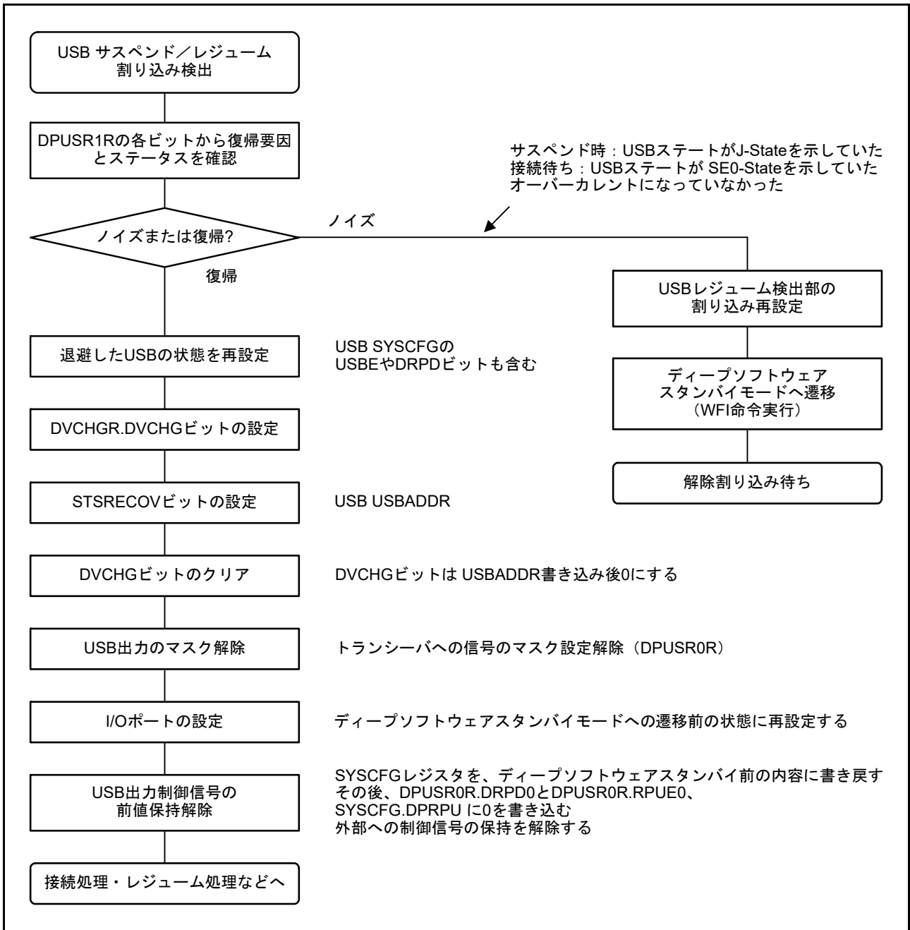
図 29.8 ホストコントローラ機能選択時におけるディープソフトウェアスタンバイモード解除時の USBFS 設定フロー
