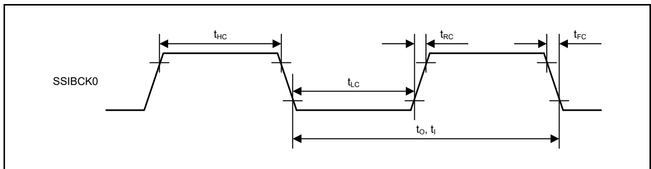
図 52.54 SSIE クロック入出力タイミング
