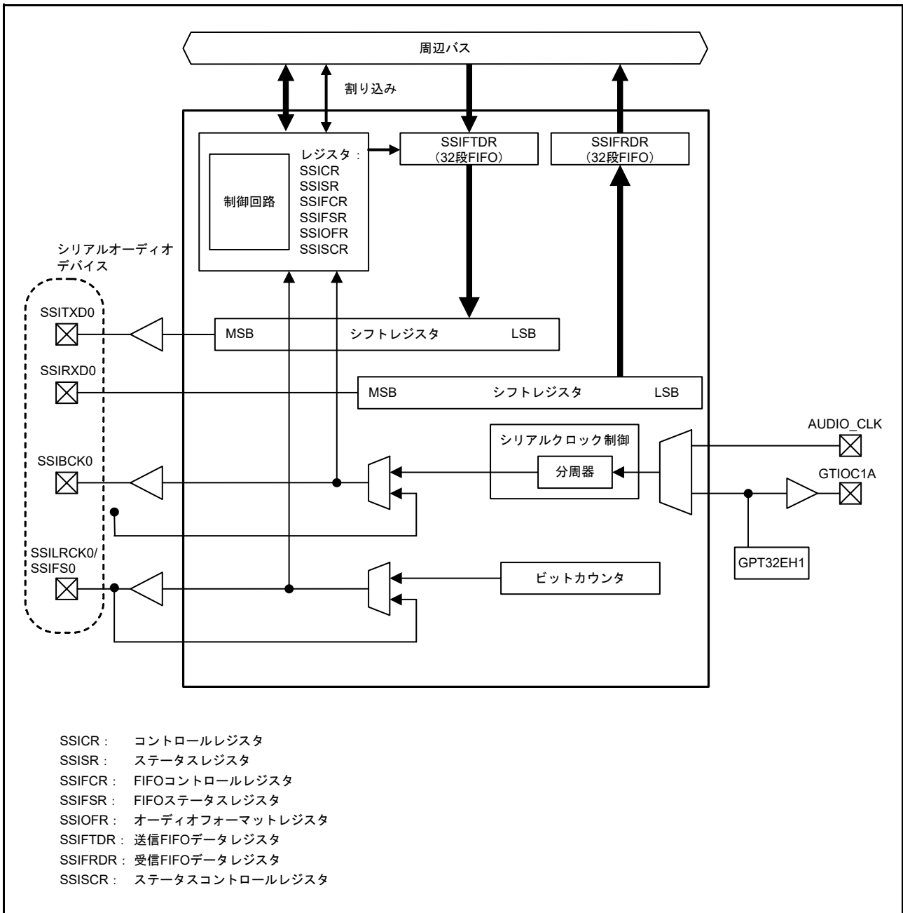
図 37.2 全二重通信の SSIE ブロック図 (SSIE0)
