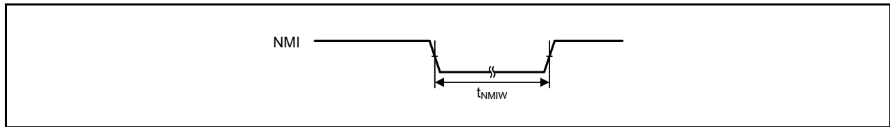
図 52.18 NMI 割り込み入力タイミング
