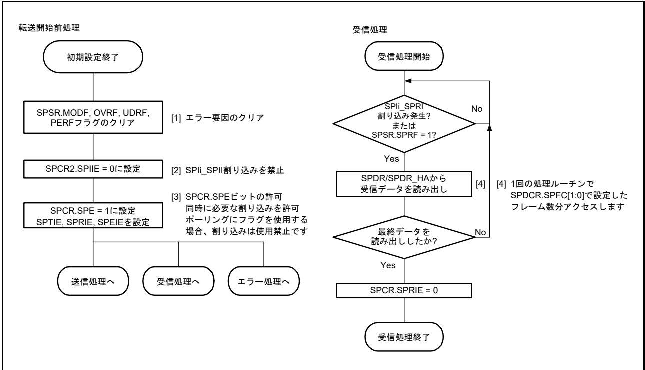
図 34.42 スレーブモードでの受信フロー
