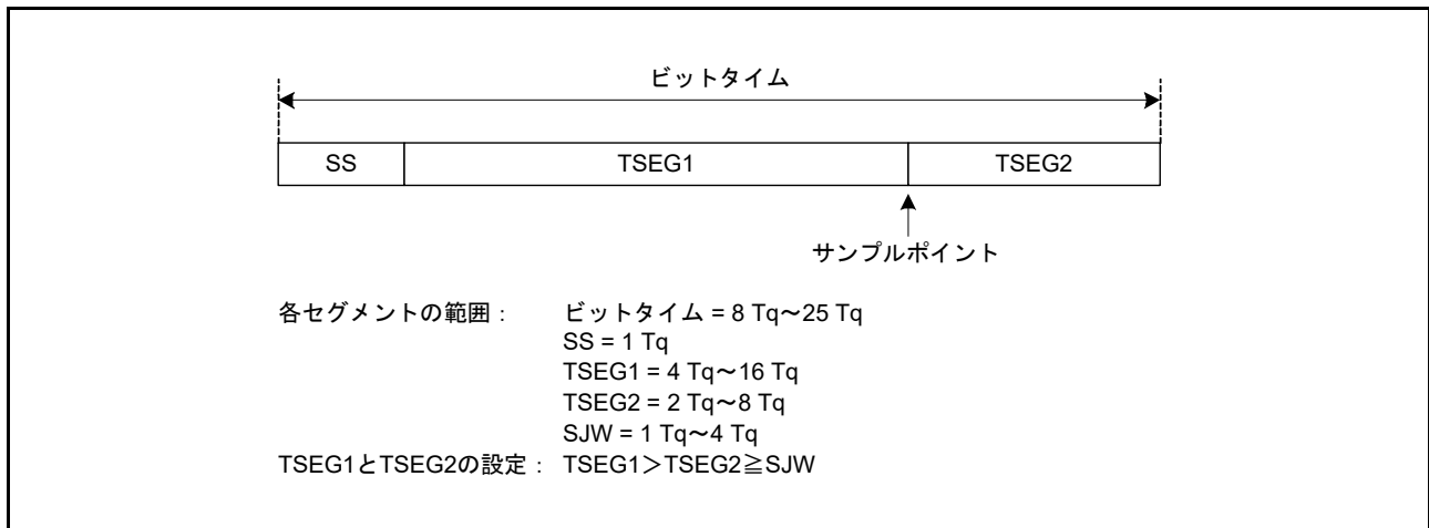
図 33.12 ビットタイミング
