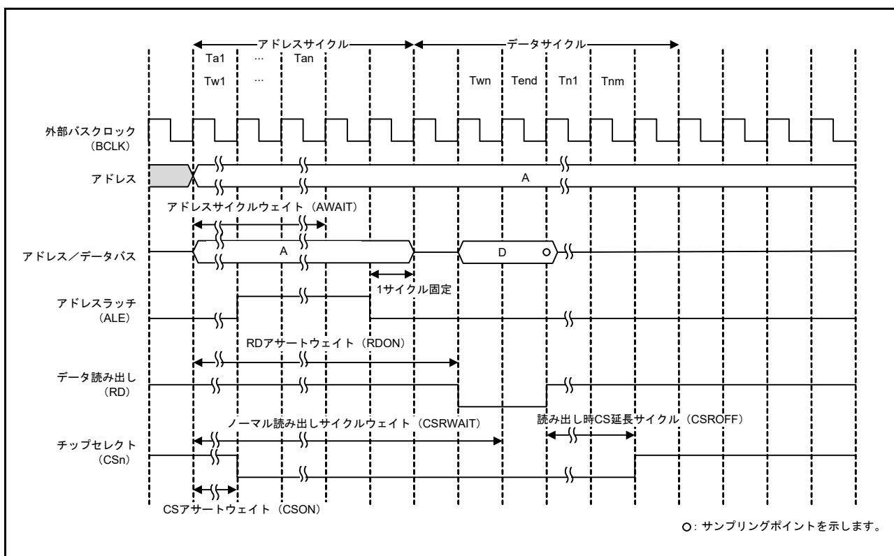
図 15.21 アドレス/データマルチプレクス I/O インタフェース時のリードアクセスの動作例 (n = 0, 1, 4 ~ 7)
