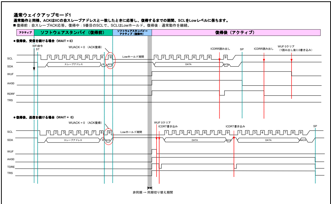
図 32.32 ノーマルウェイクアップモード1のタイミング
