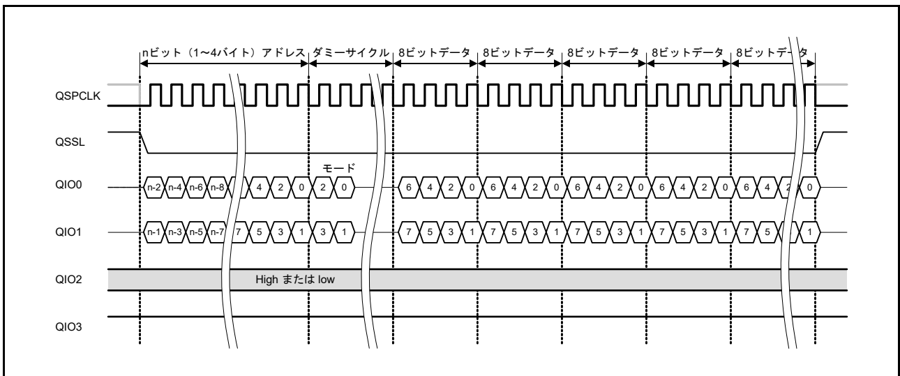
図 35.22 XIP モード時のファストリード Dual I/O バスサイクル
