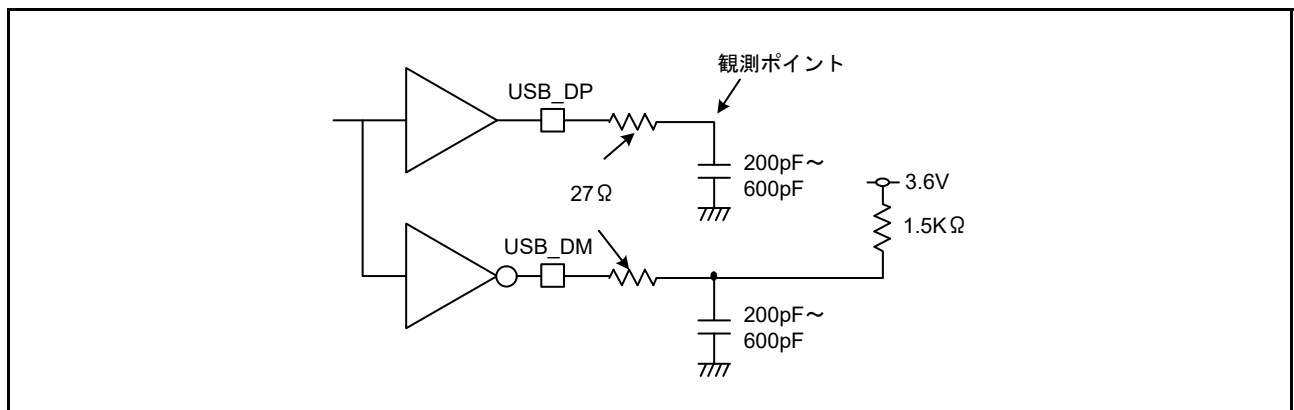
図 52.61 Low-speed モードにおける測定回路
