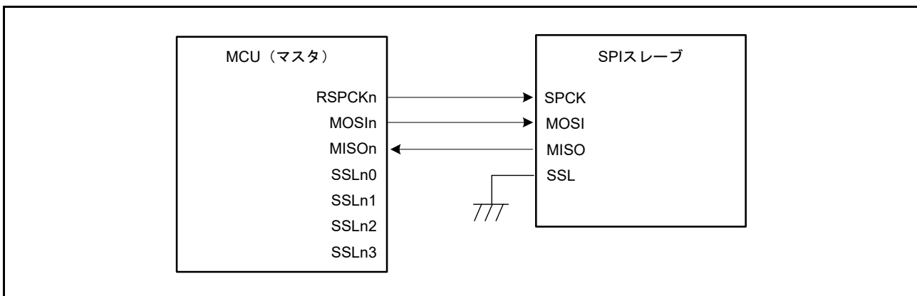
図 34.5 シングルマスタ/シングルスレーブの構成例 (MCU はマスタ)
