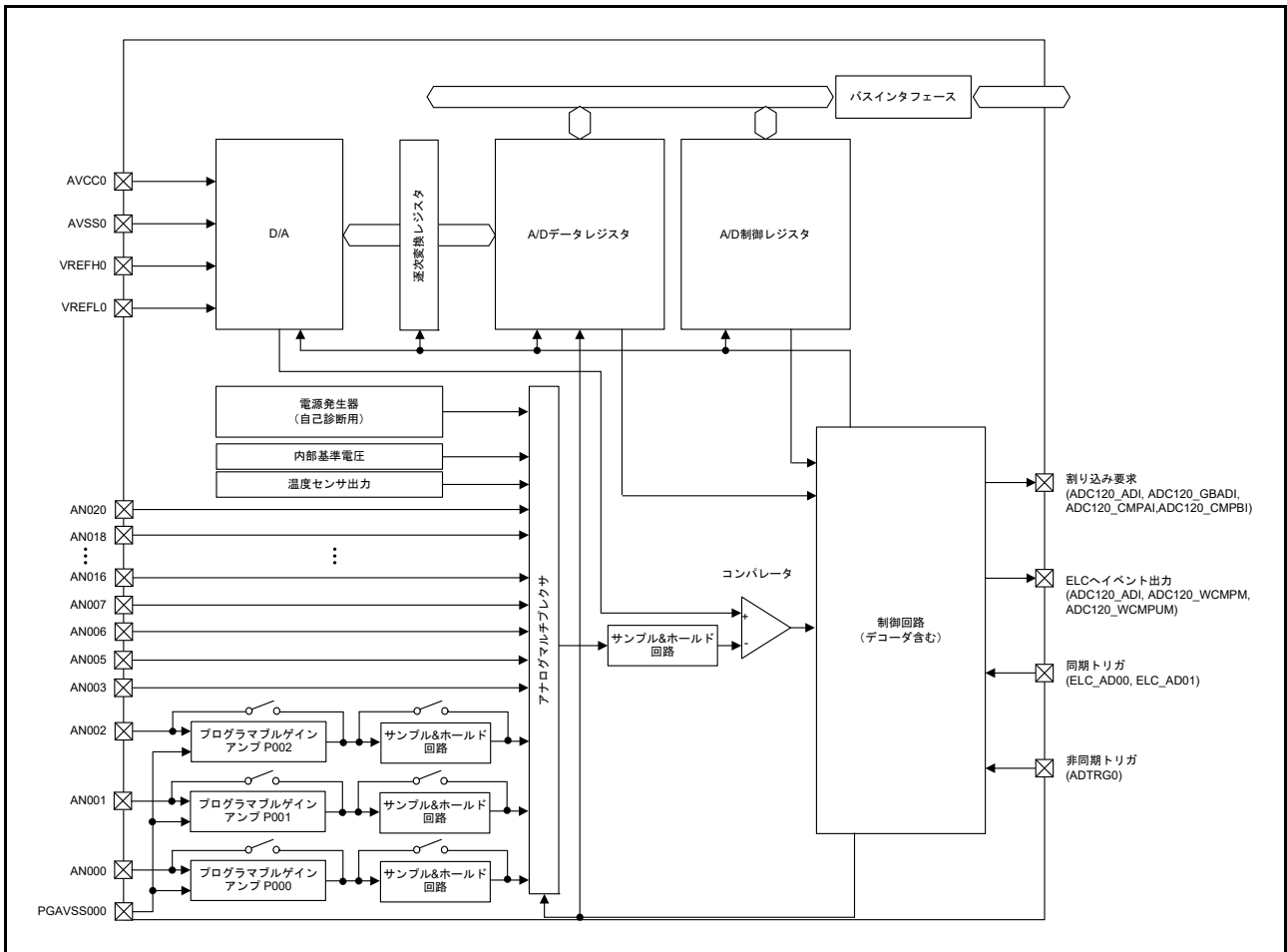
図 42.1 ADC12 (ユニット 0) のブロック図
