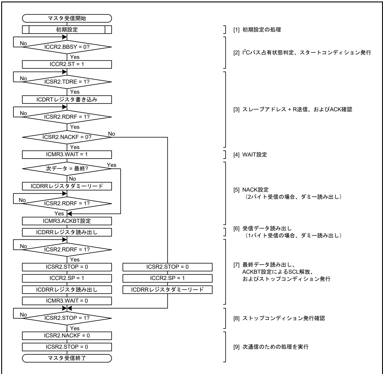
図 32.10 マスタ受信のフローチャート例 (7ビットアドレスフォーマットで1または2バイト受信の場合)
