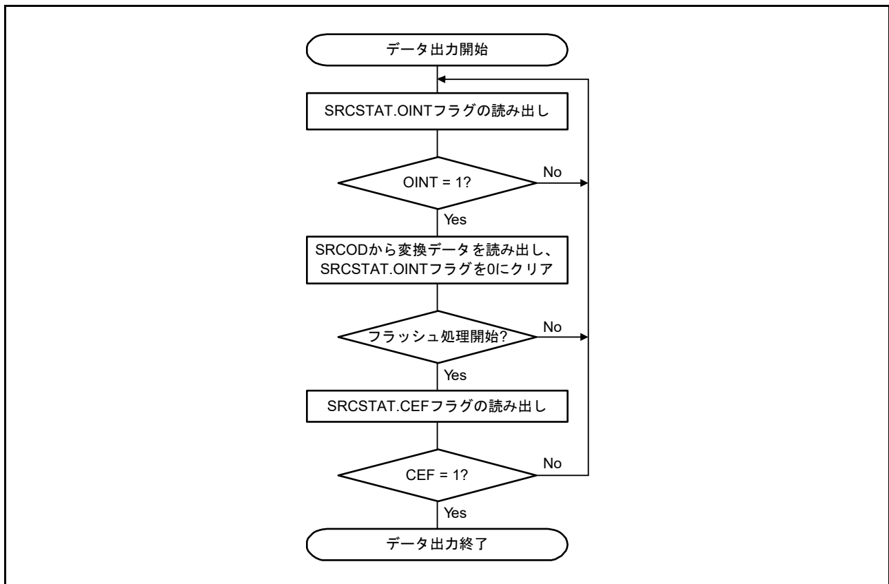
図 38.4 データ出力フロー
