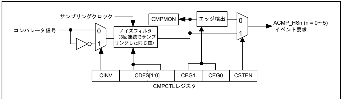
図 45.3 ノイズフィルタおよびエッジ検出の構成
