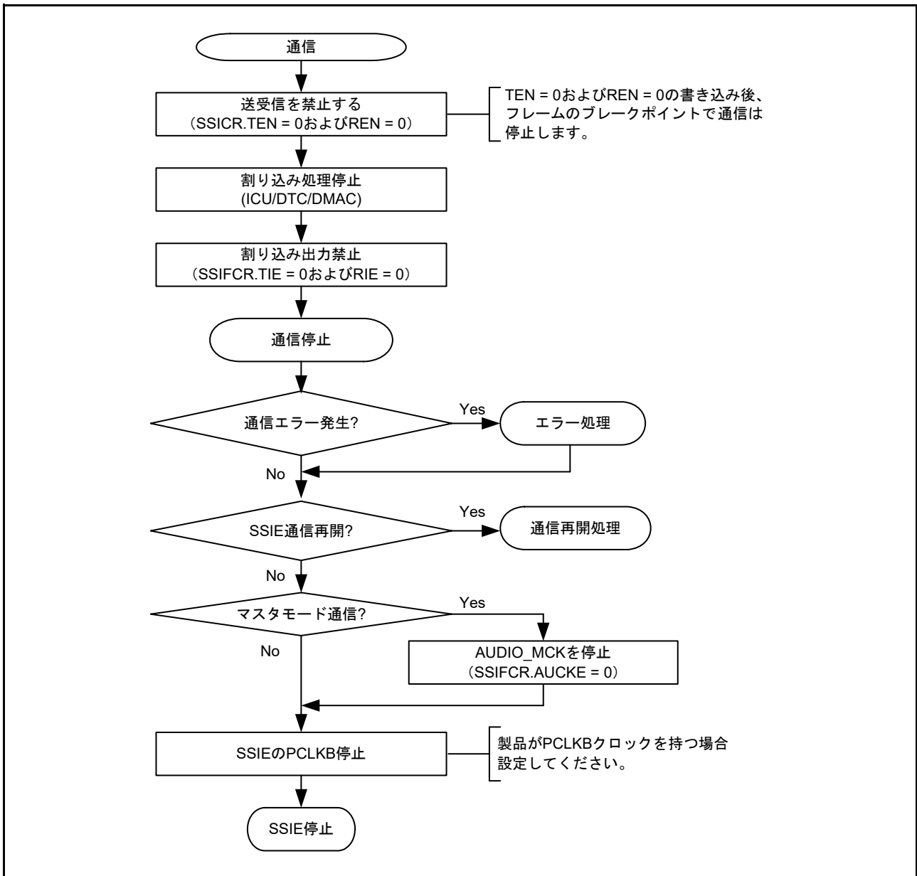
図 37.55 通信停止手順 (CPU 動作手順)
