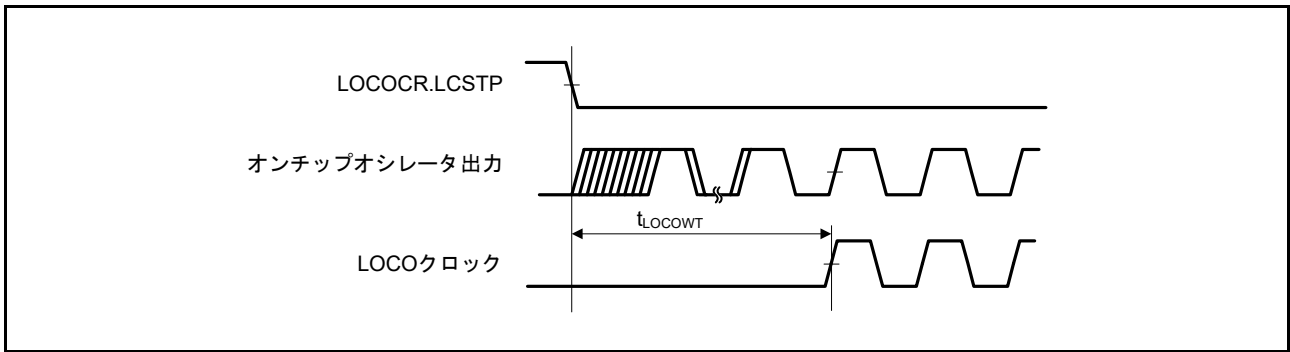
図 52.10 LOCO クロック発振開始タイミング
