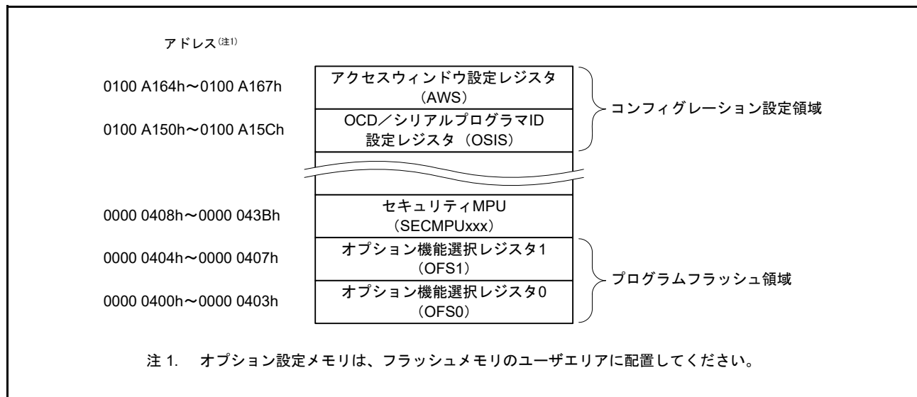
図 7.1 オプション設定メモリの領域
