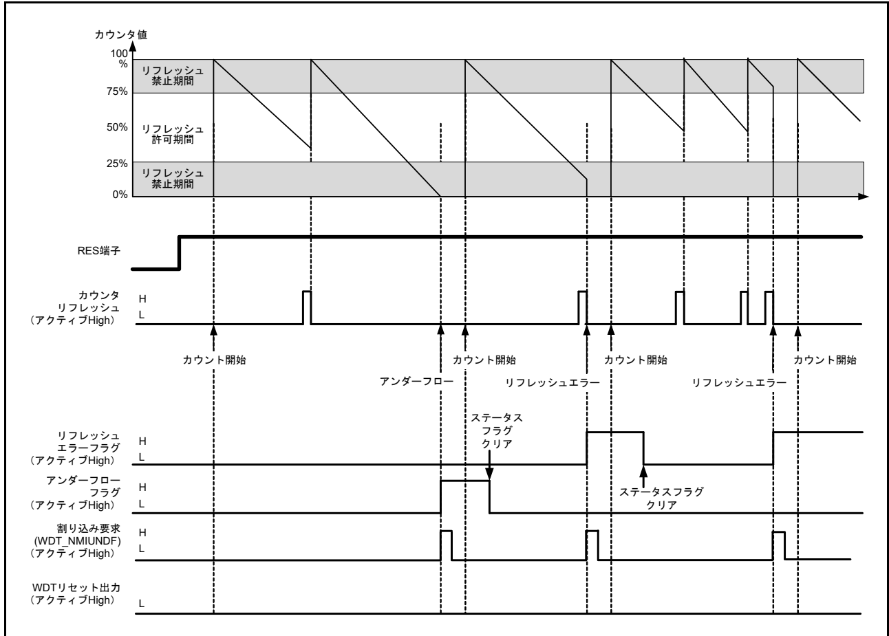
図 27.4 オートスタートモードでの動作例
