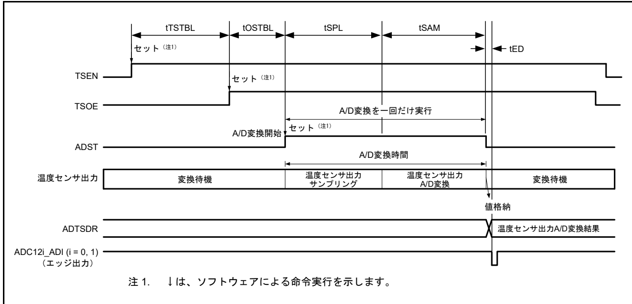
図 44.3 温度センサの動作開始から A/D 変換完了までのタイミング
