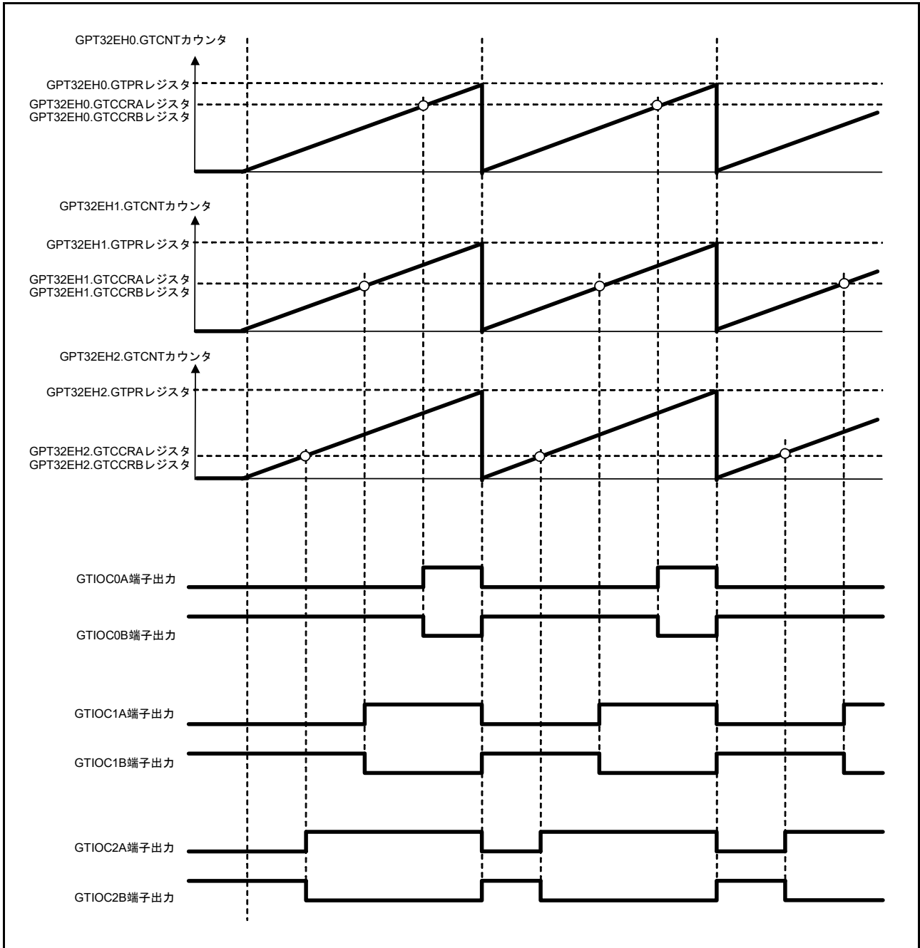
図 23.66 のこぎり波 3 相相補 PWM 出力例
