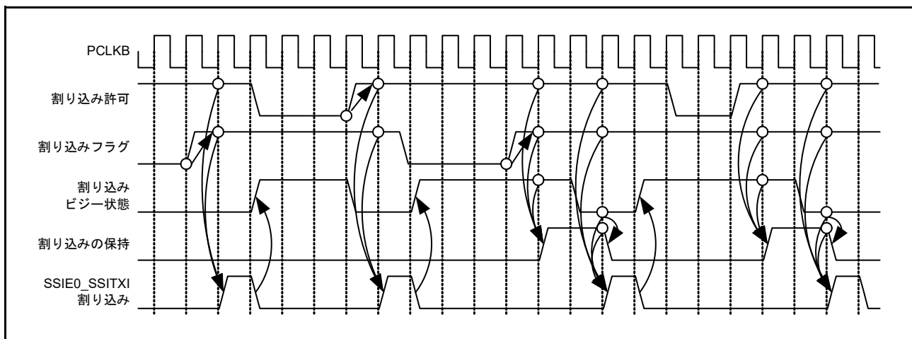
図 37.59 SSIE0_SSITXI 割り込みのタイミング図
