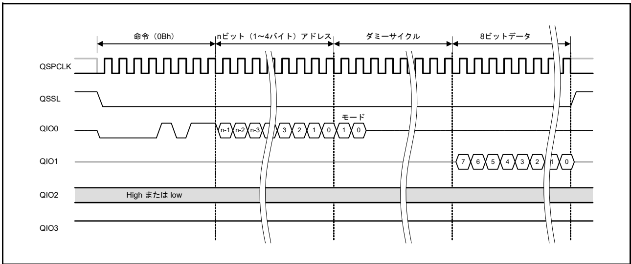
図 35.17 ファストリードバスサイクル
