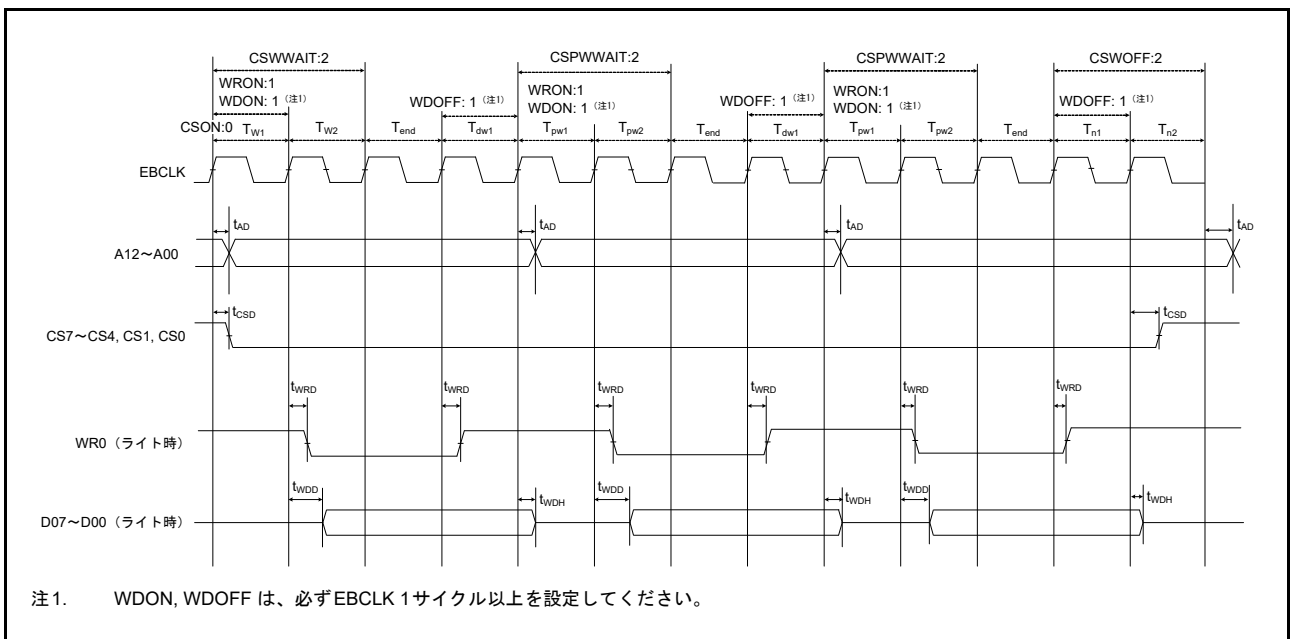
図 52.25 バスクロック同期を使用したページライトサイクルの外部バスタイミング
