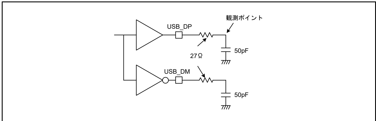
図 52.63 フルスピードモードにおける測定回路
