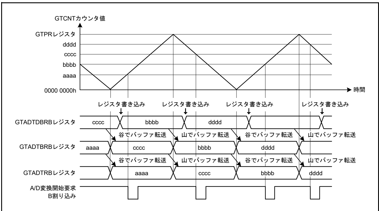
図 23.31 GTADTRA、GTADTRB レジスタのダブルバッファ動作例 (三角波、谷と山の両方でバッファ転送、アップカウントとダウンカウント両方で A/D 変換開始要求割り込み発生の場合)
