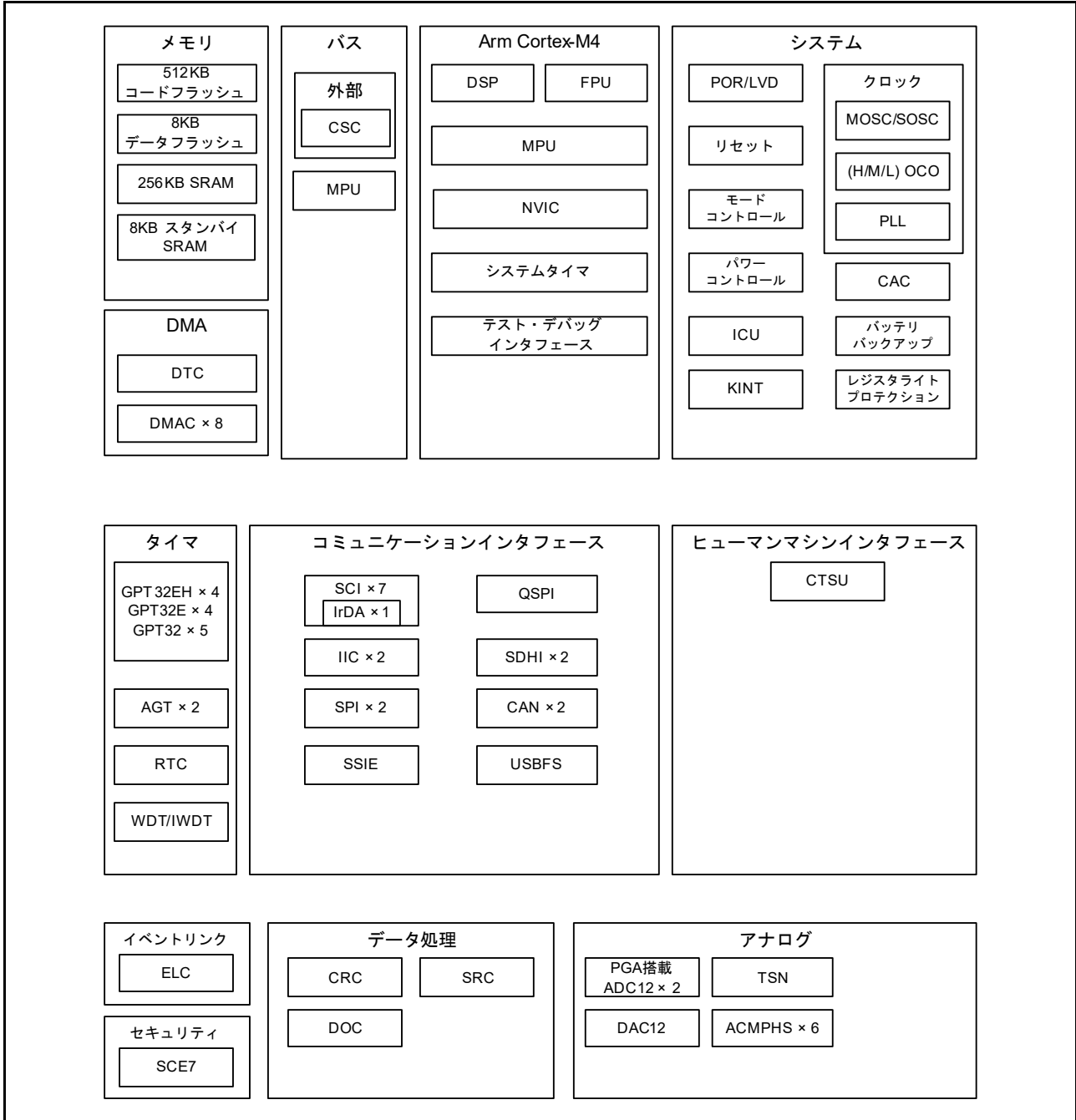
図 1.1 ブロック図
