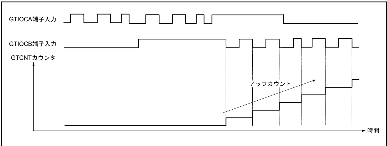
図 23.80 位相計数モード5の動作例 (B)
