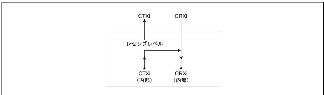
図 33.6 リッスンオンリモード選択時の接続 (i = 0, 1)
