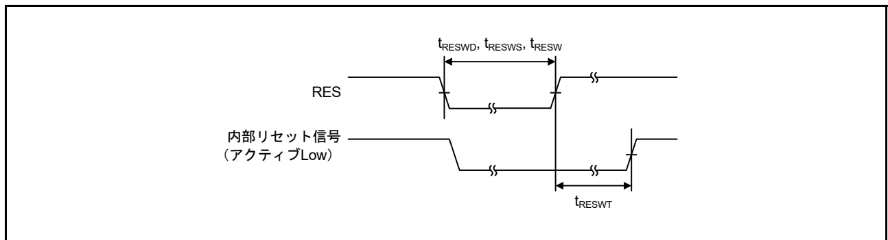
図 52.14 リセット入力タイミング
