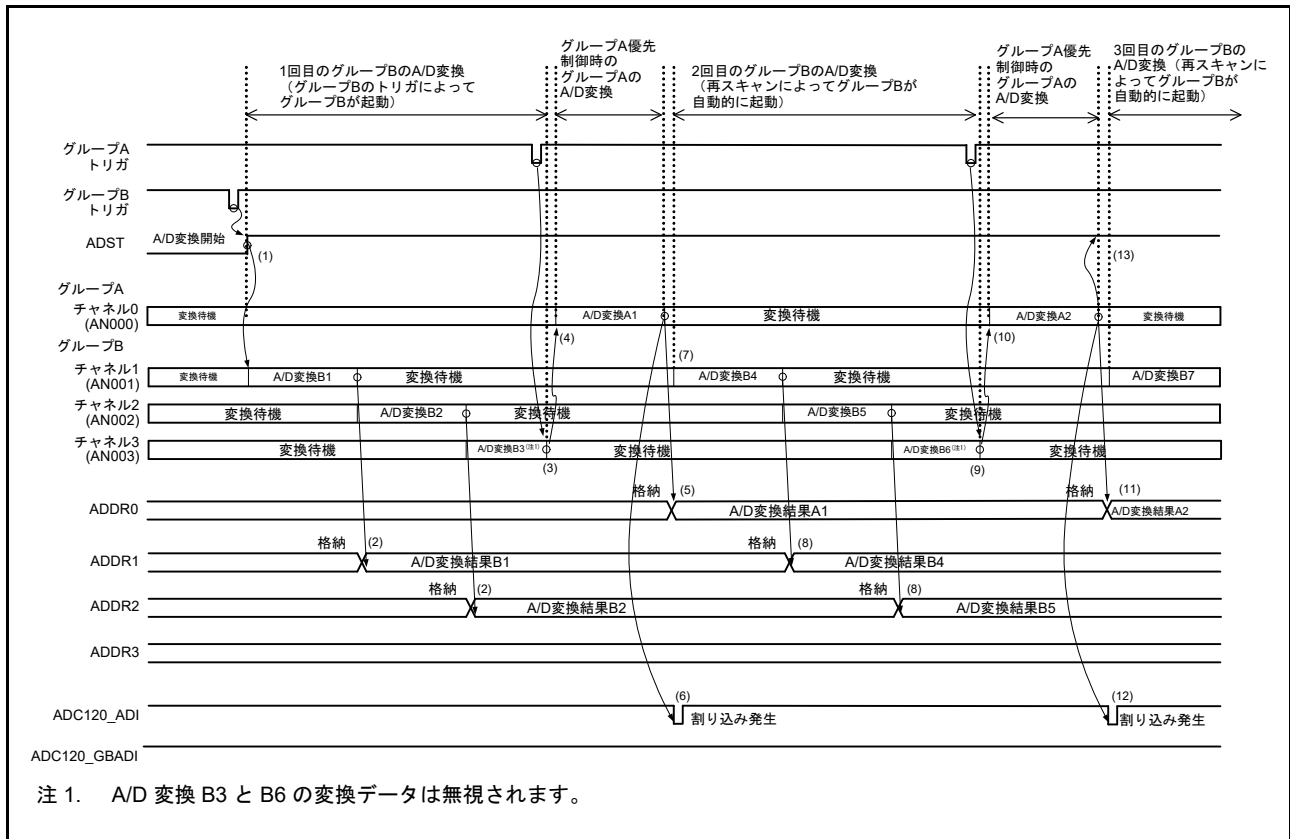
図 42.27 グループ A 優先制御の動作例 (2) (ADGSPCR.GBRSCN = 1、ADGSPCR.GBRP = 0 の場合)
