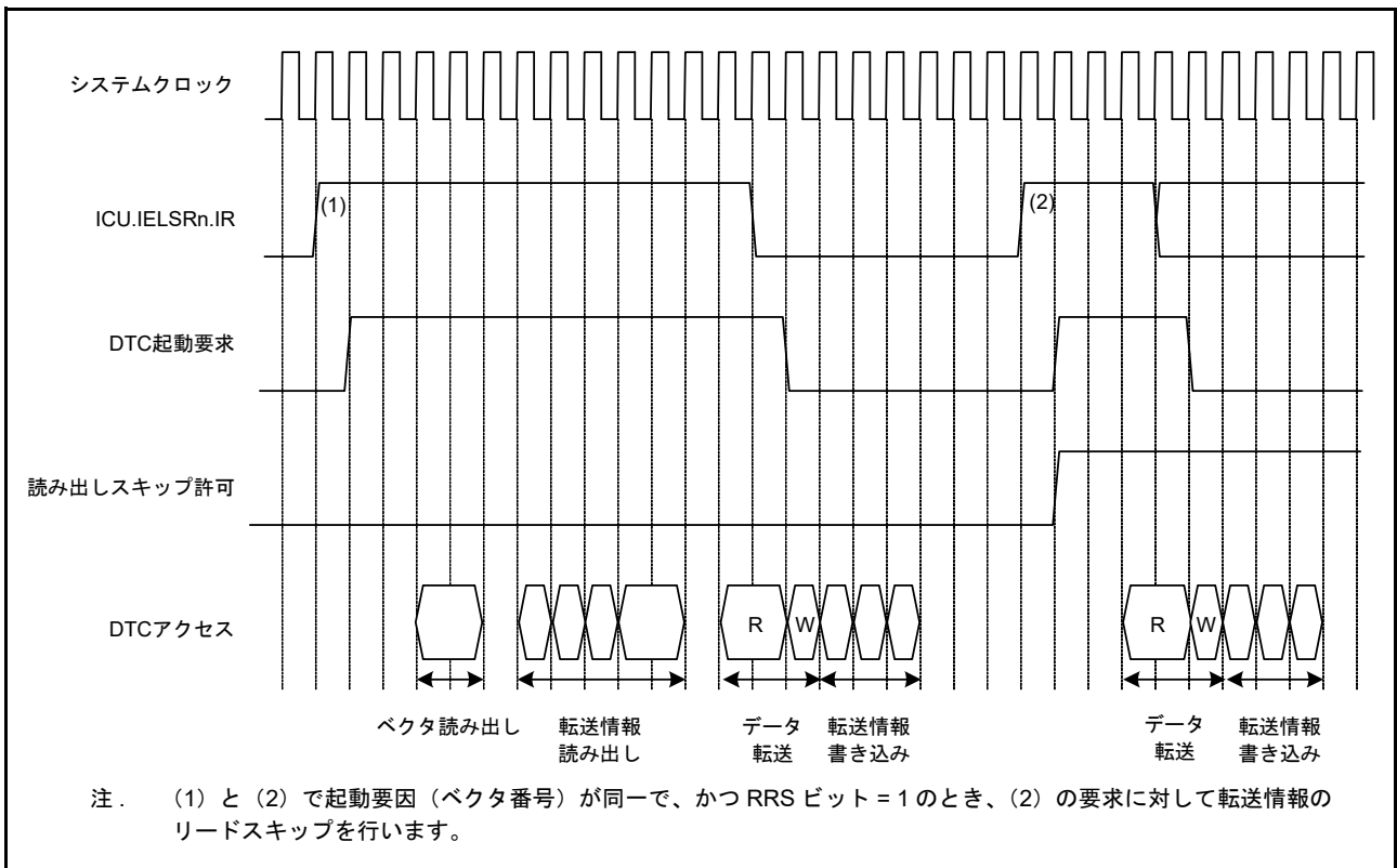
図 18.12 転送情報リードスキップ時の動作例 (ベクタ、転送情報、転送先データが SRAM にあり、転送元データが周辺モジュールにある場合)
