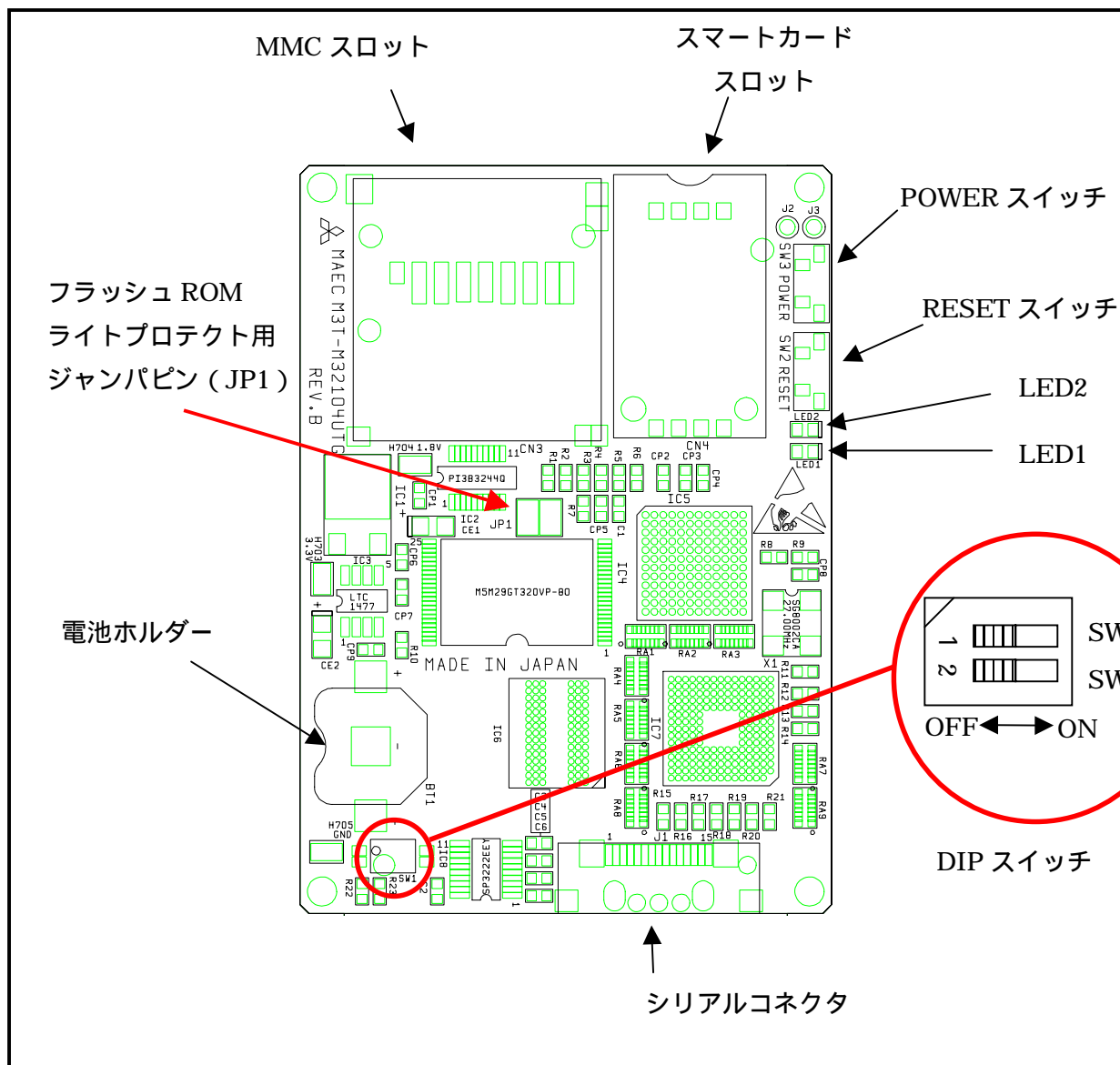
図 5.1.1 表面部品図
