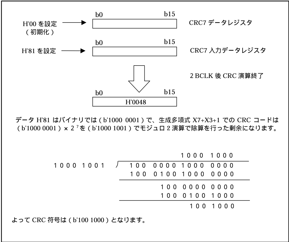
図 4.8.2 CRC 演算回路動作例
