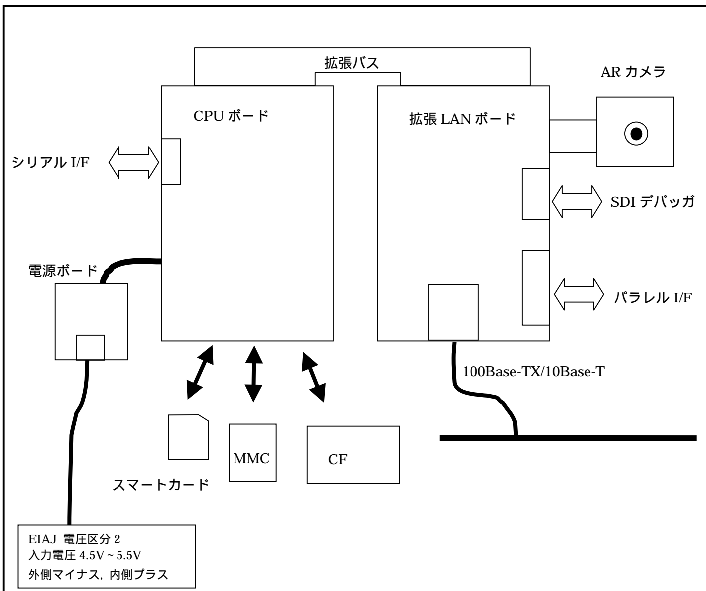
図 2.2.1 製品の構成図
