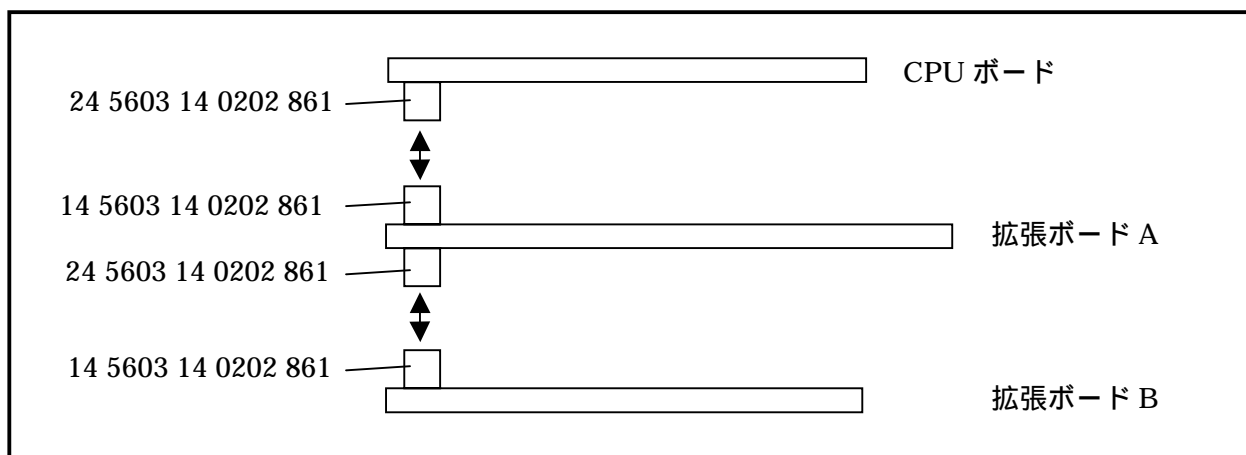
図 3.11.1 拡張ボードコネクタ
