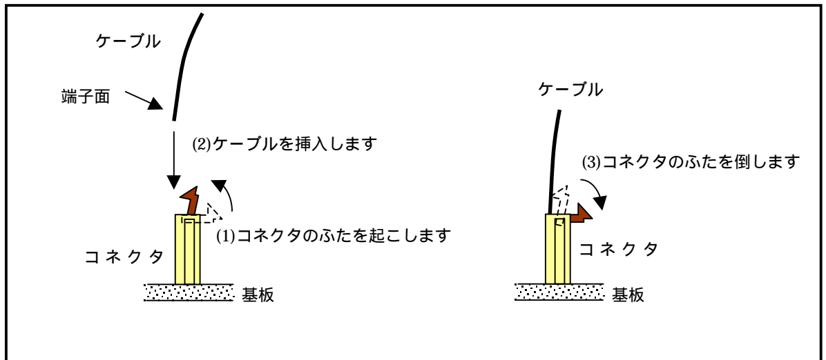
図 5.3.4 AR ボード用ケーブルの接続方法
