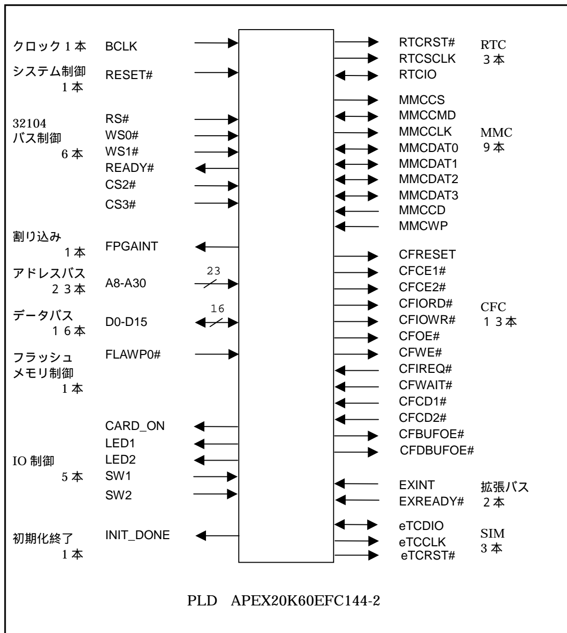
図 4.2.1 PLD 端子機能図
