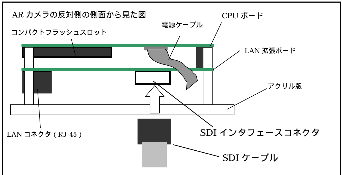
図 5.3.5 SDI エミュレータ接続方法
