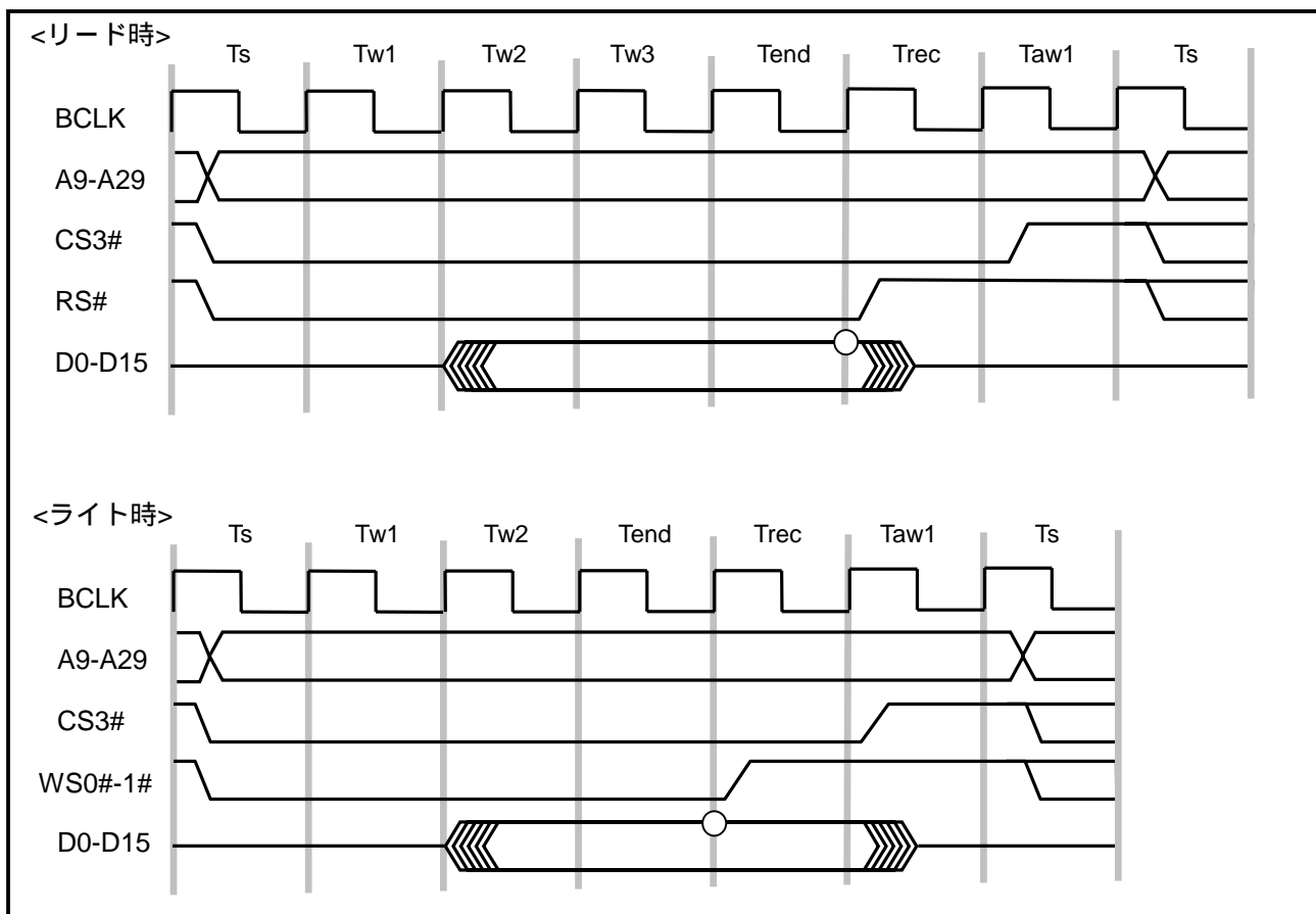
図 4.1.1 PLD リード・ライトレジスタアクセスタイミング
