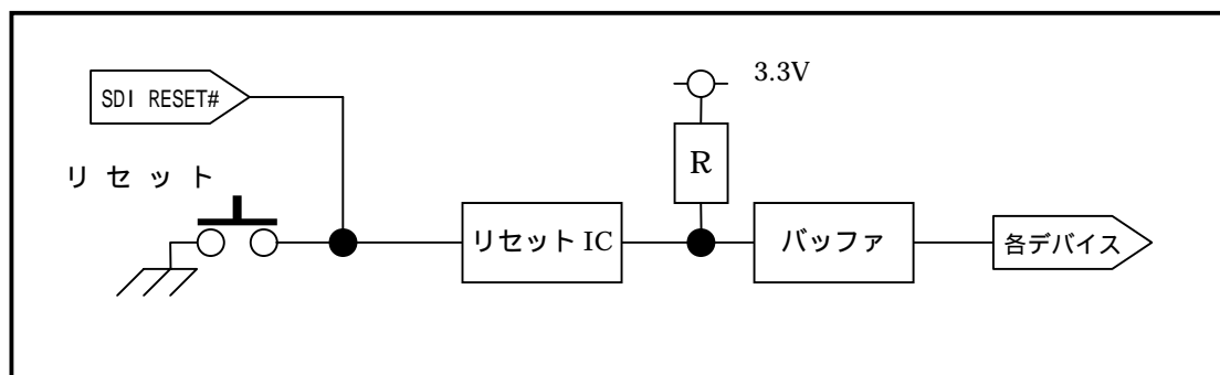
図 3.10.1 リセット系統図
