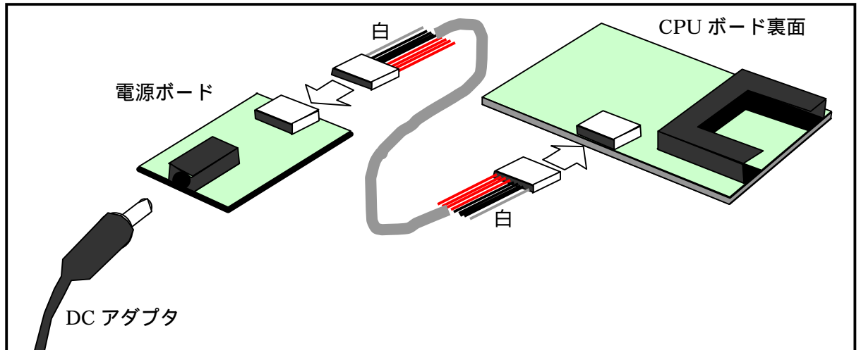
図 5.3.3 電源接続方法
