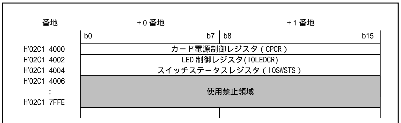
図 4.7.1 IOC レジスタマッピング
