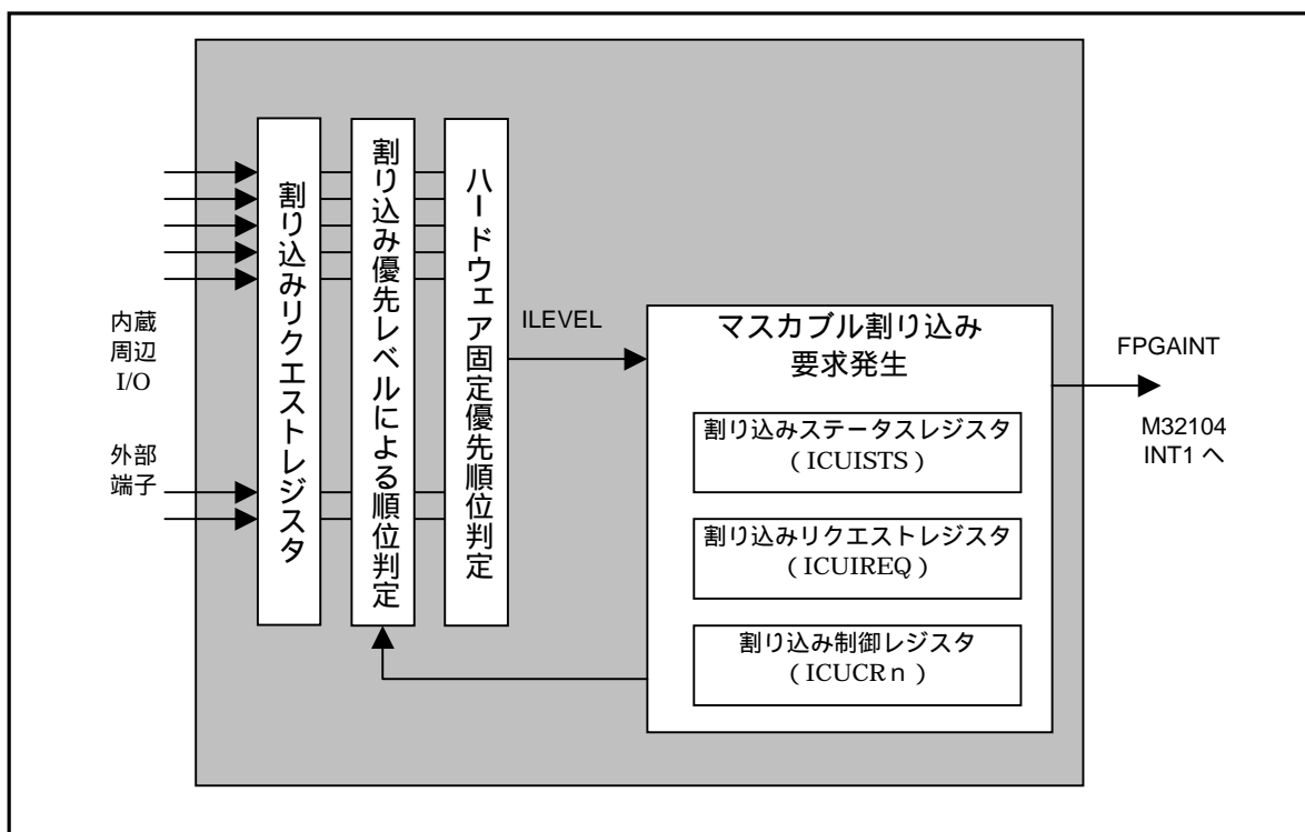
図 4.6.1 ICU ブロック図
