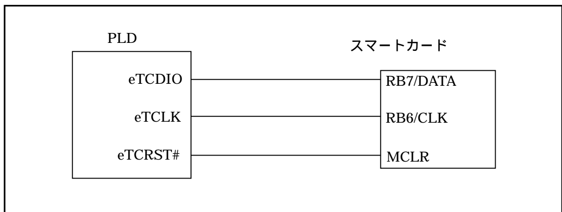
図 4.10.1 スマートカード接続図
