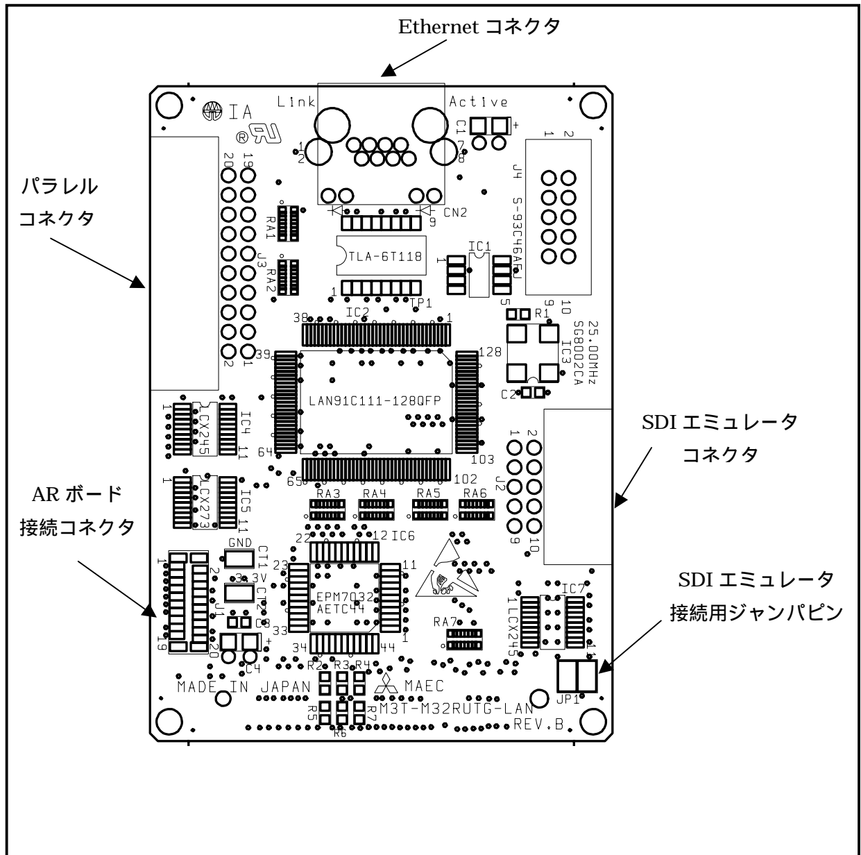
図 5.1.3 拡張 LAN ボード表面
