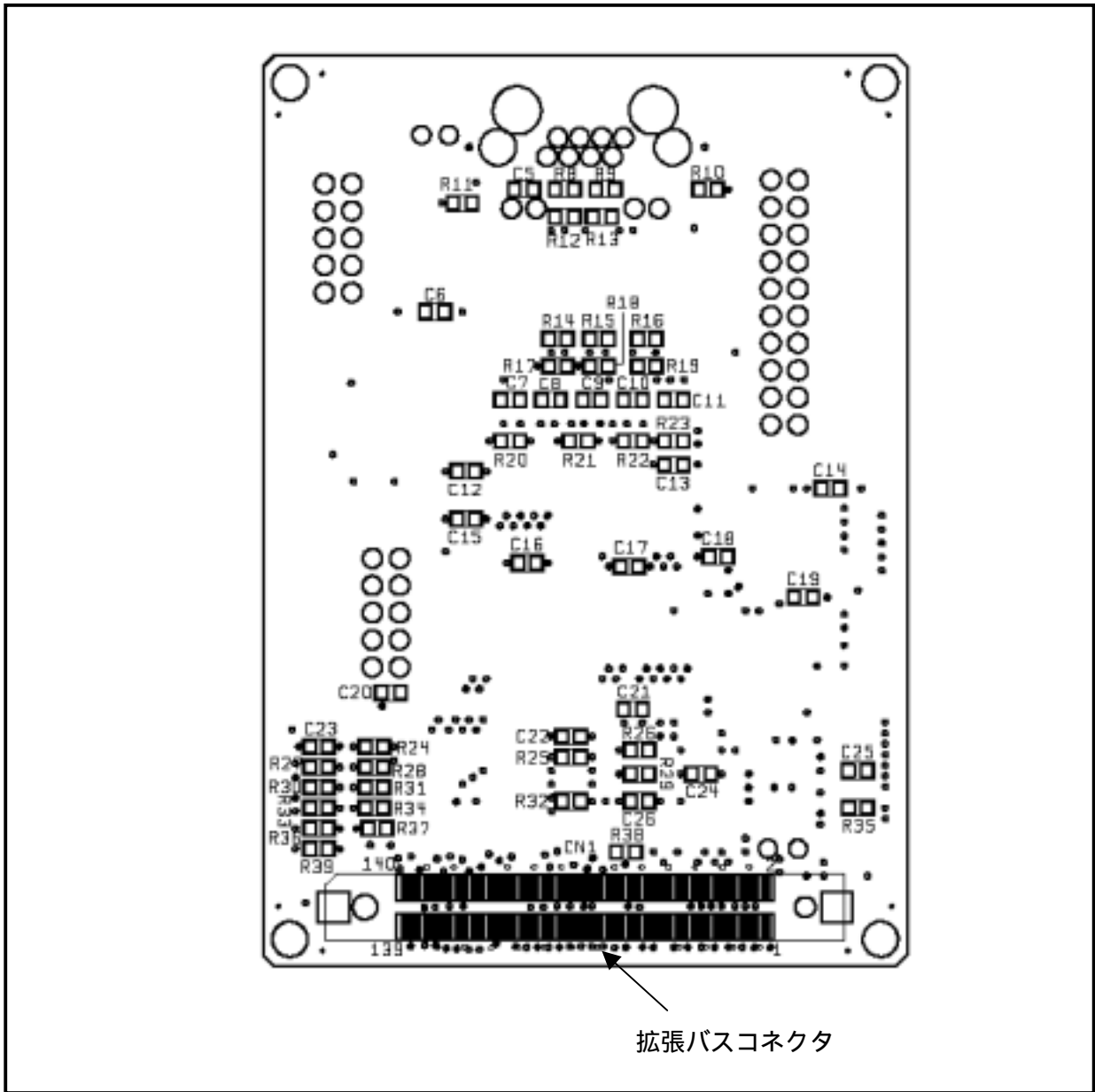
図 5.1.4 拡張 LAN ボード裏面
