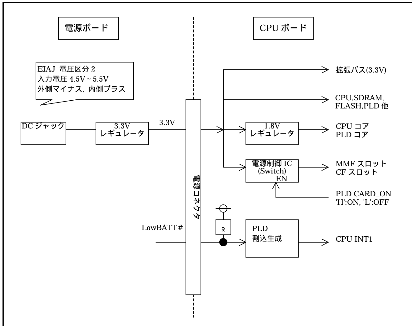
図 3.8.1 電源系統説明図
