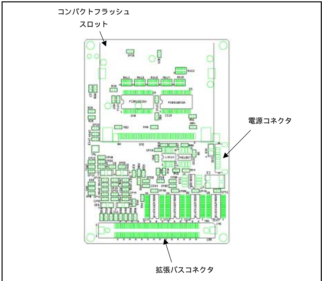
図 5.1.2 裏面部品図
