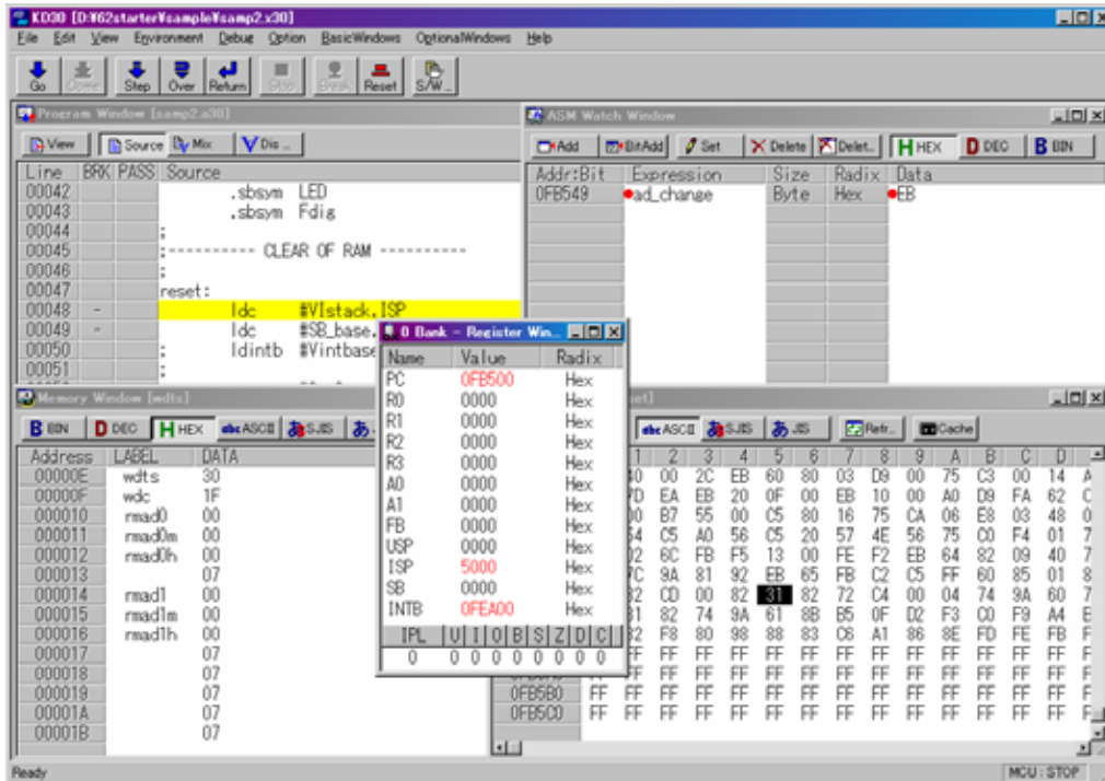
図 4.2 KD3083起動ウィンドウ
