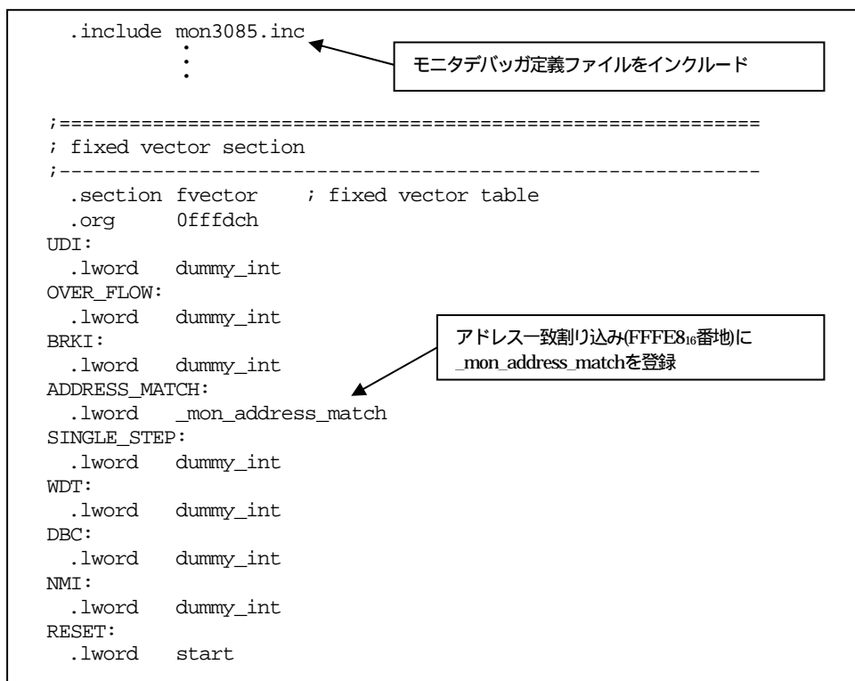
図 5.3 モニタデバッグ用割り込み処理の登録例
