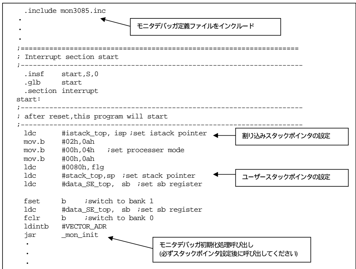
図 5.4 モニタデバッグ初期化処理呼び出し例
