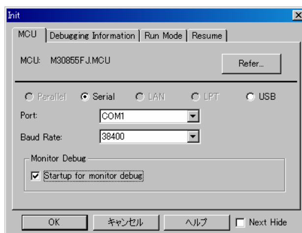
図 4.1 Init ウィンドウ
