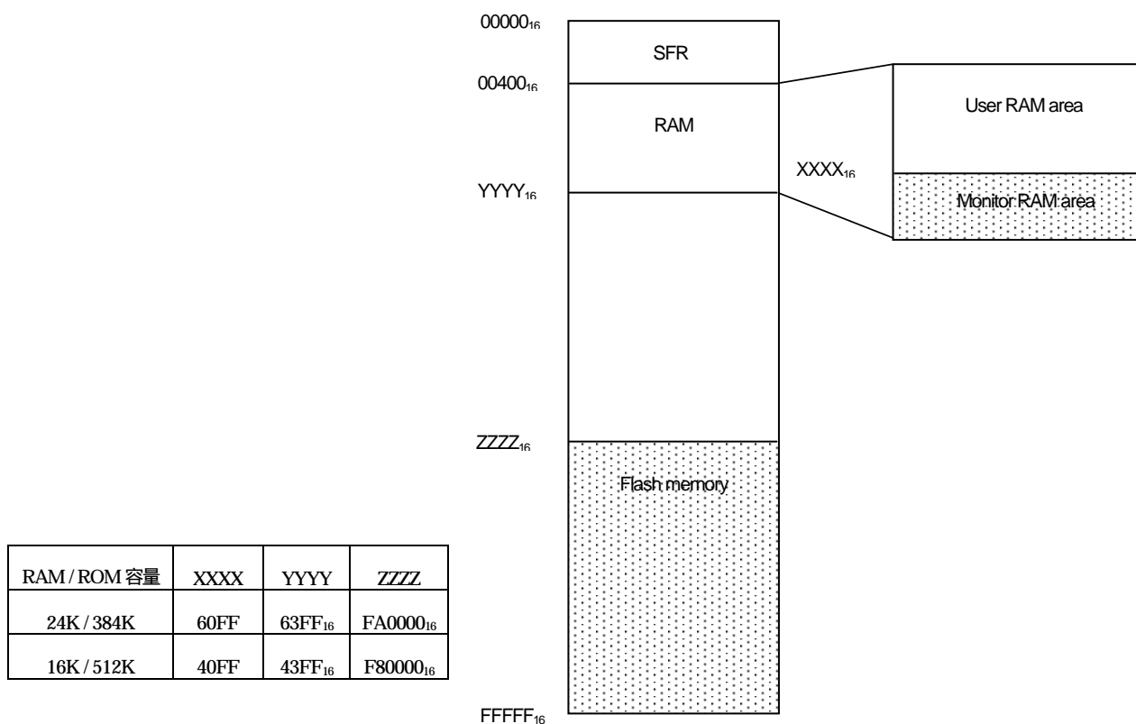
図 6.1 M32C/85 モニタデバッグメモリマップ
