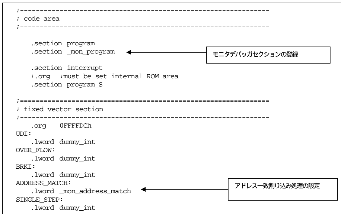
図 6.3 sect308.inc の修正例
