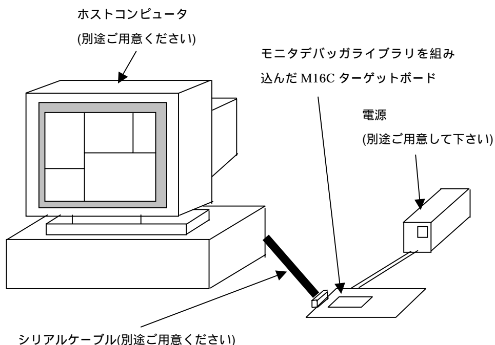
図 3.1 M16C モニタデバッガのシステム構成図
