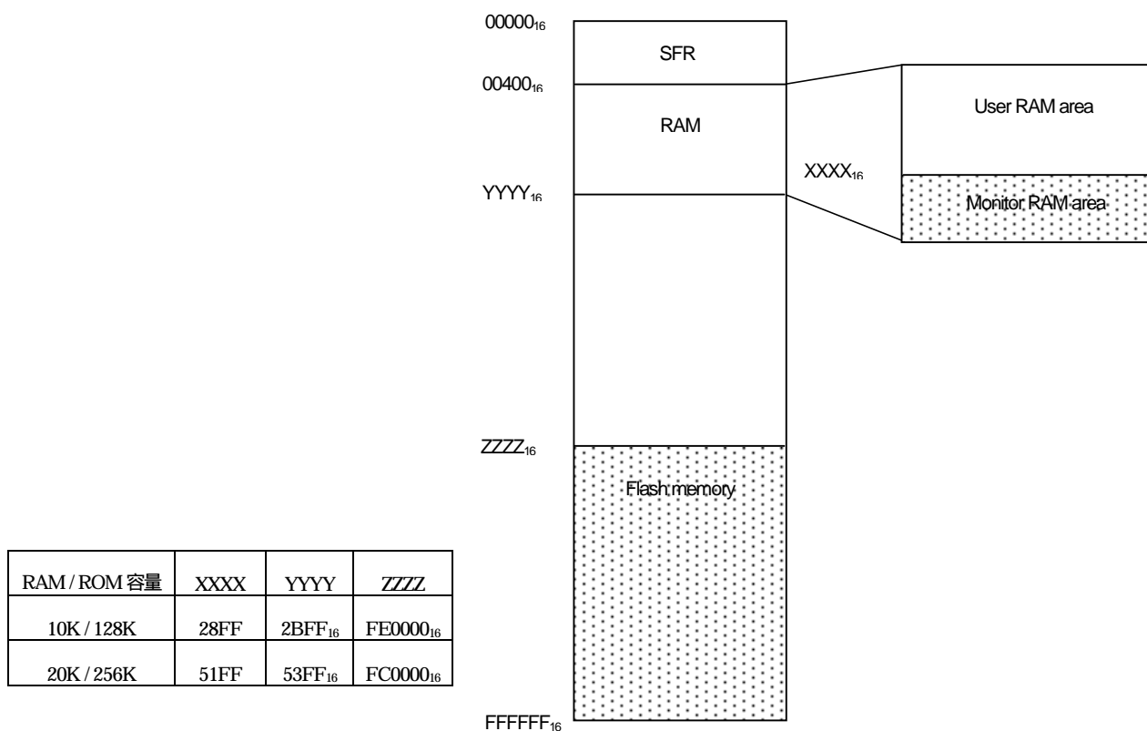
図 6.1 M16C/80 モニタデバッグメモリマップ
