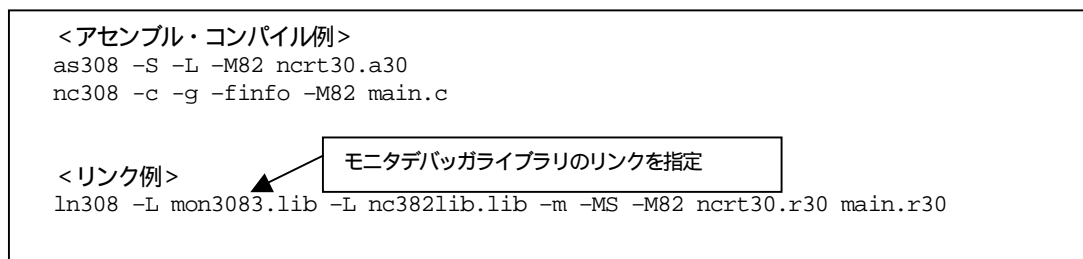
図 5.5 モニタデバッグライブラリのリンク例
