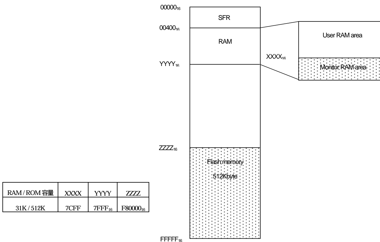
図 6.1 M32C/83 モニタデバッガメモリマップ
