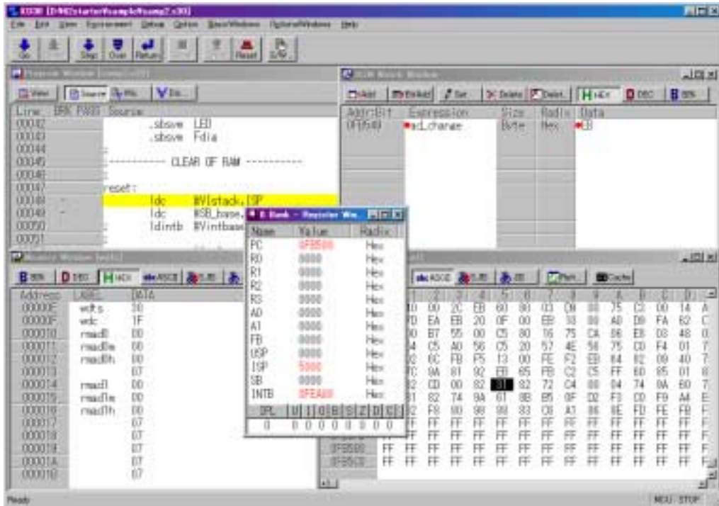
図 4.2 KD3083起動ウィンドウ
