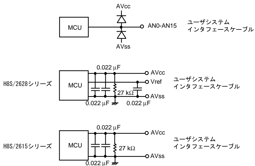
図 2-5 AN0-AN15、AVcc、AVss、Vref信号回路
