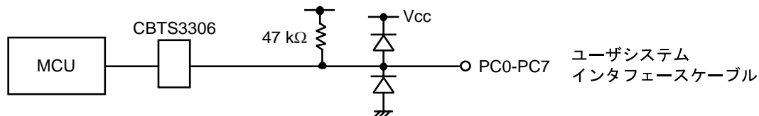
図 2-4 PC0-PC7信号回路
