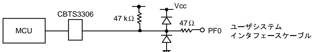
図 2-3 PF0信号回路
