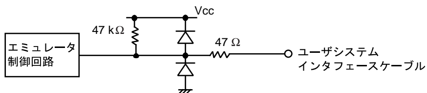
図 2-2 モード端子、NMI、STBY、RESET信号回路
