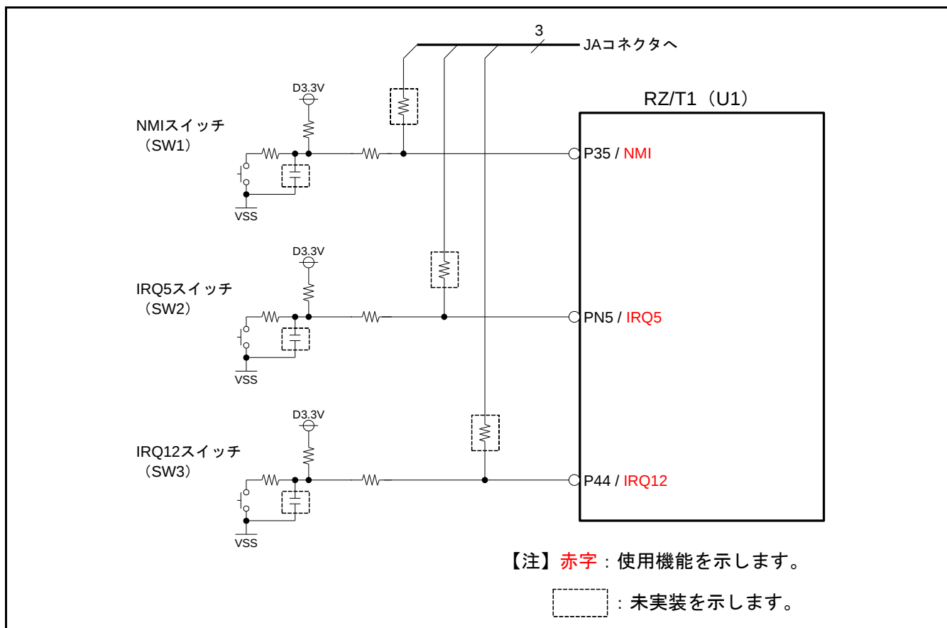
図 2.7.1 割り込みスイッチブロック図
