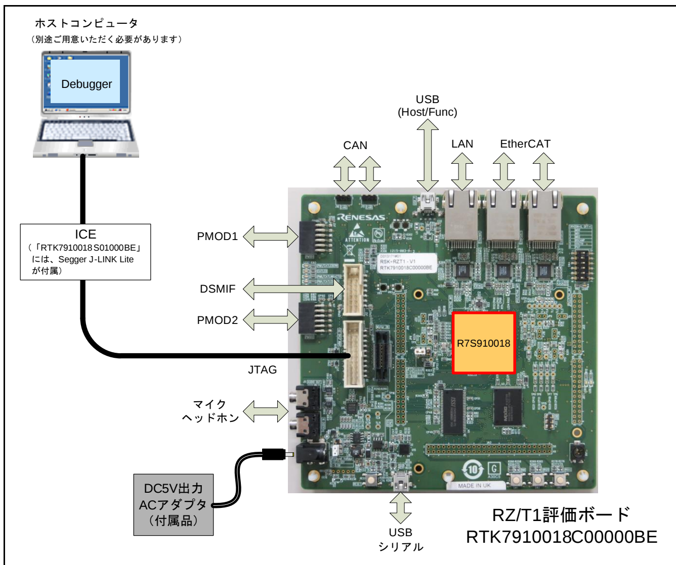
図 1.1 RTK7910018C00000BE を用いたシステム構成例
