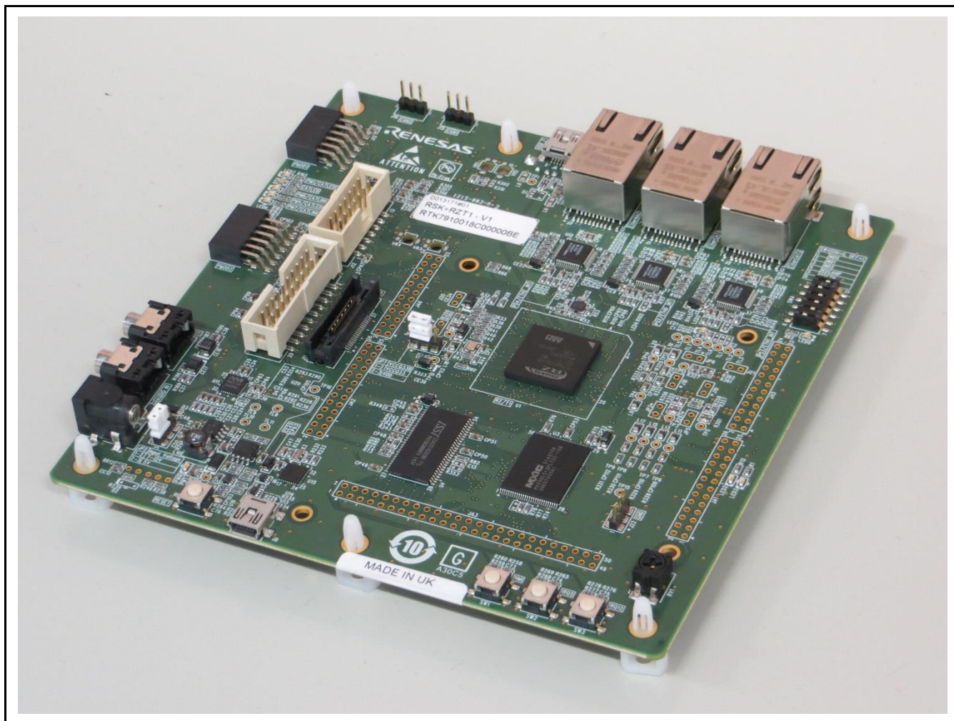
図 1.2 RTK7910018C00000BE 外観図
