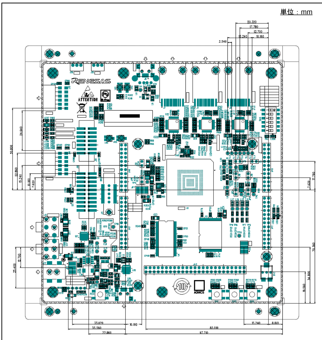
図 3.3.2 RTK7910018C00000BE 外形寸法図 (C 面上面図) (2/2)
