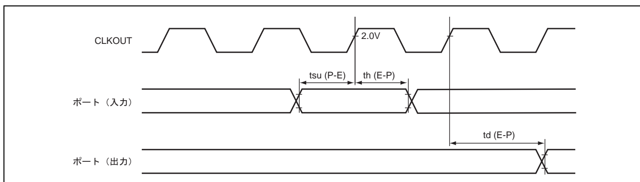
図 38.23 I/O ポート入出力タイミング
