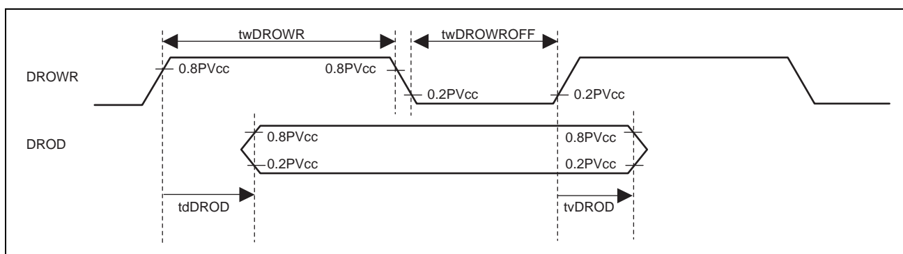
図 38.38 "H"アクティブ選択時のストロブ極性
