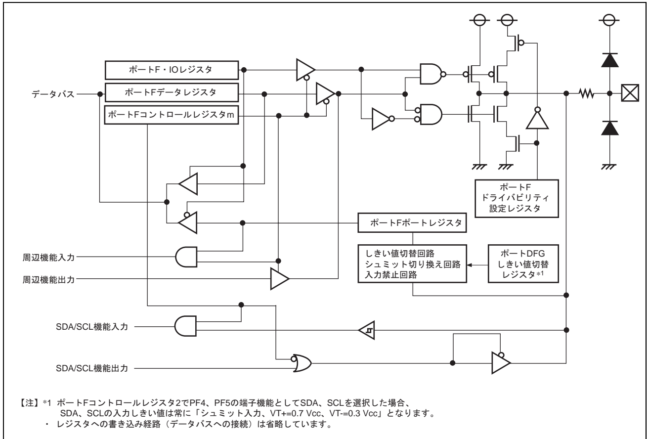
図 18.3 ポート周辺回路図（入力/出力ポート 3）
