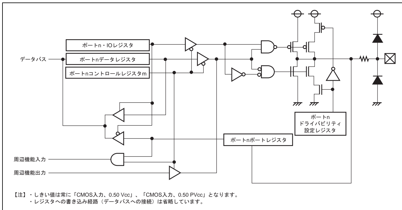
図 18.2 ポート周辺回路図（入力/出力ポート 2）
