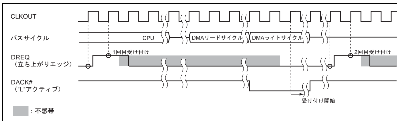
図 20.11 DREQ 入力検出タイミング例 (サイクルスチールモード 1・DACK ライトサイクル出力)
