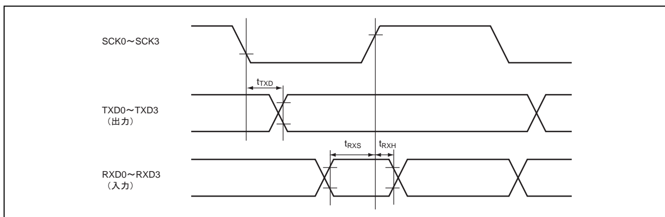
図 38.26 SCI 入出力タイミング
