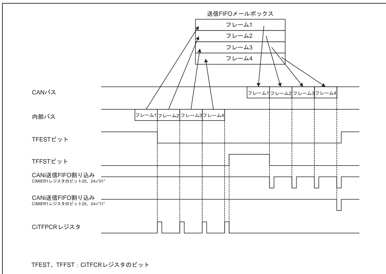
図 26.3 送信 FIFO メールボックスの動作 (CiMIER1 レジスタのビット 25、24 が"01"または"11") (i=0~4)
