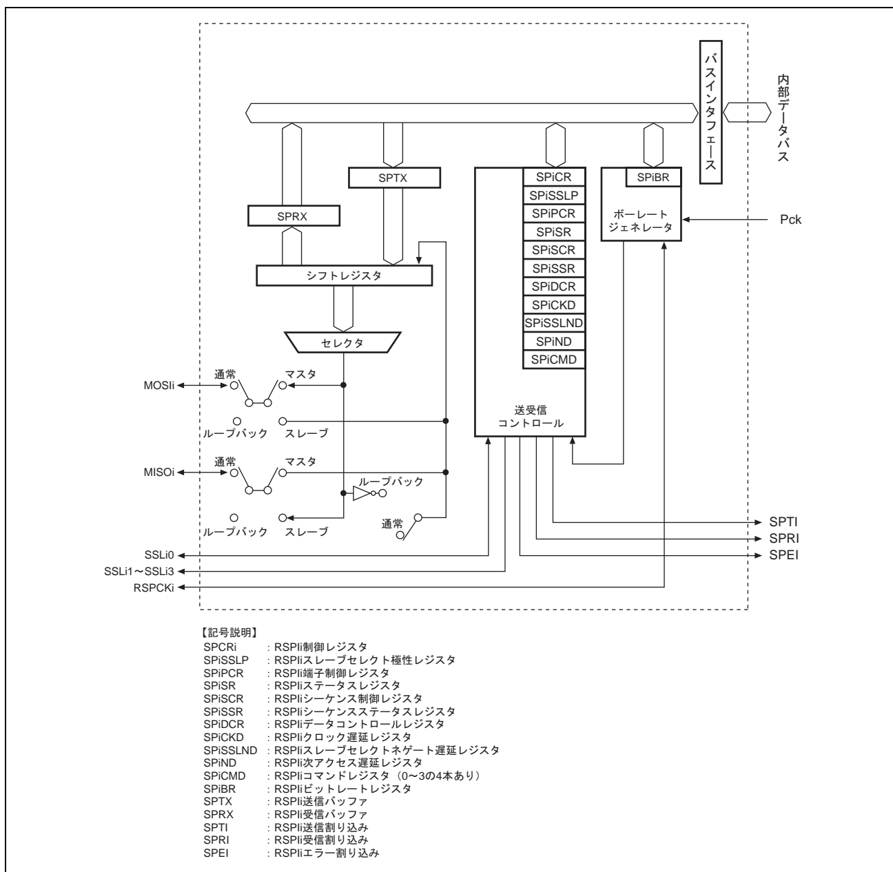
図 24.1 RSPIのブロック図
