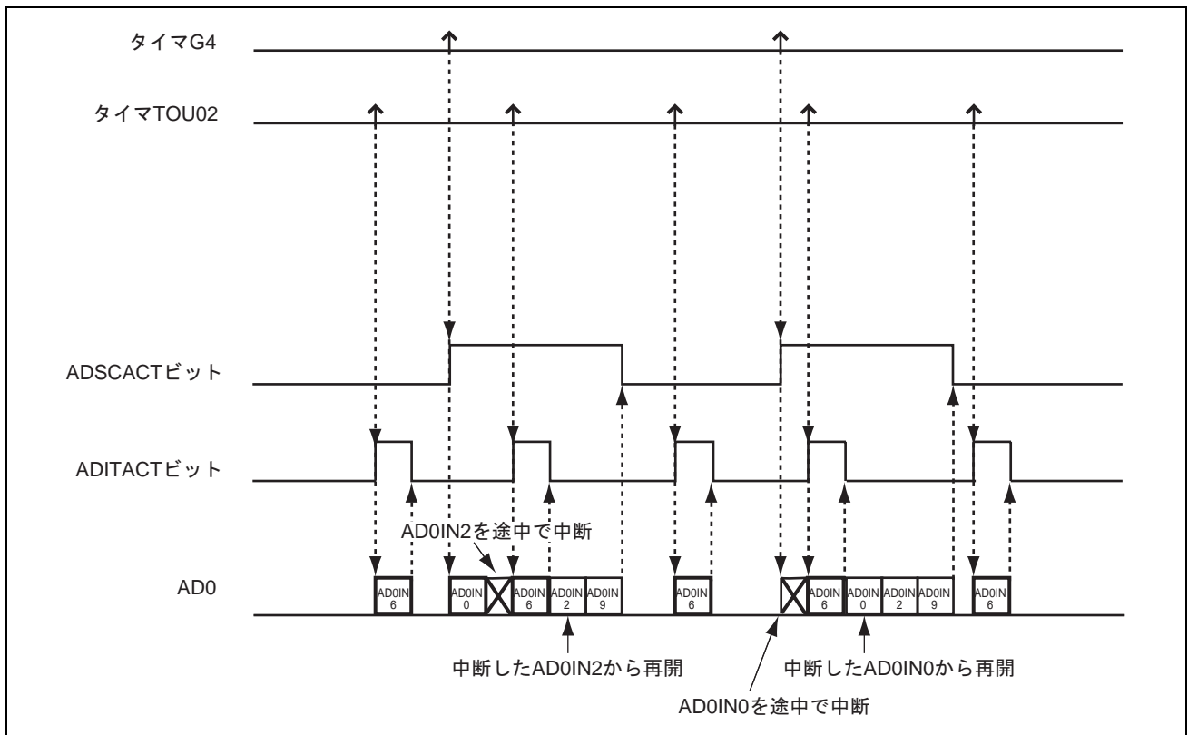
図 27.7 スキャン変換中の割り込み変換の動作例
