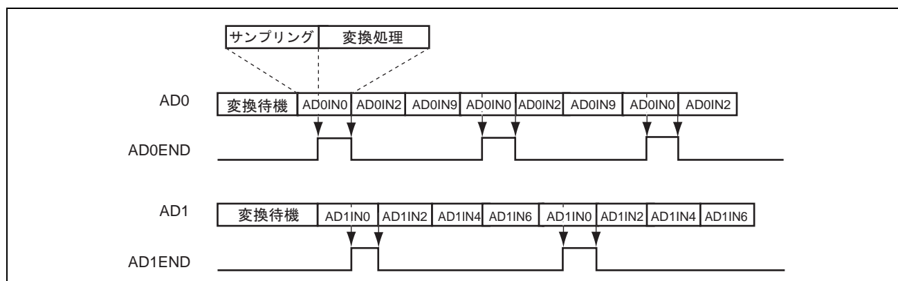
図 27.10 AD0END、AD1END 端子の出力例
