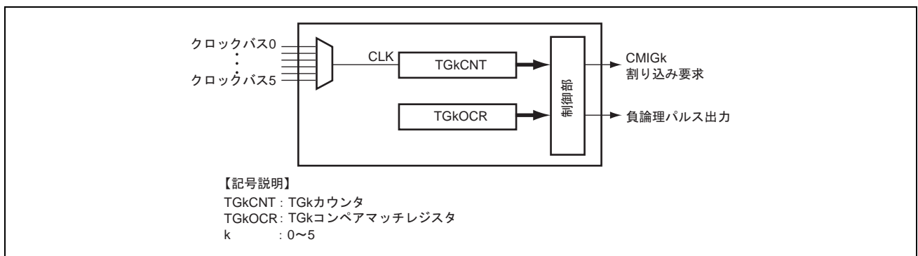
図 21.23 タイマ G のブロック図
