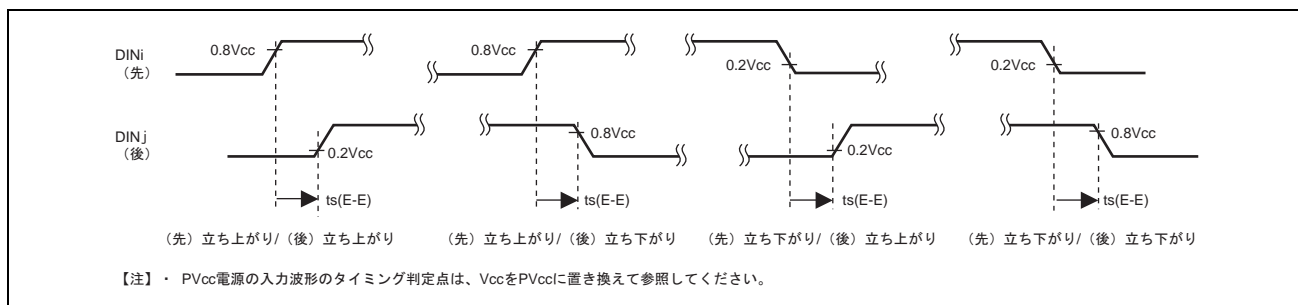
図 38.34 エッジ検出タイミング (DRI 内部でエッジ検出タイミングが同時とならないためのエッジ間隔)
