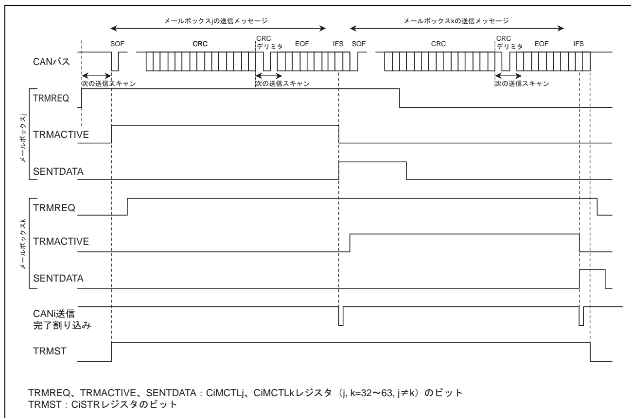
図 26.20 データフレーム送信時の動作例 (i=0~4)
