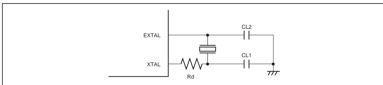
図 14.2 水晶発振子の接続例
