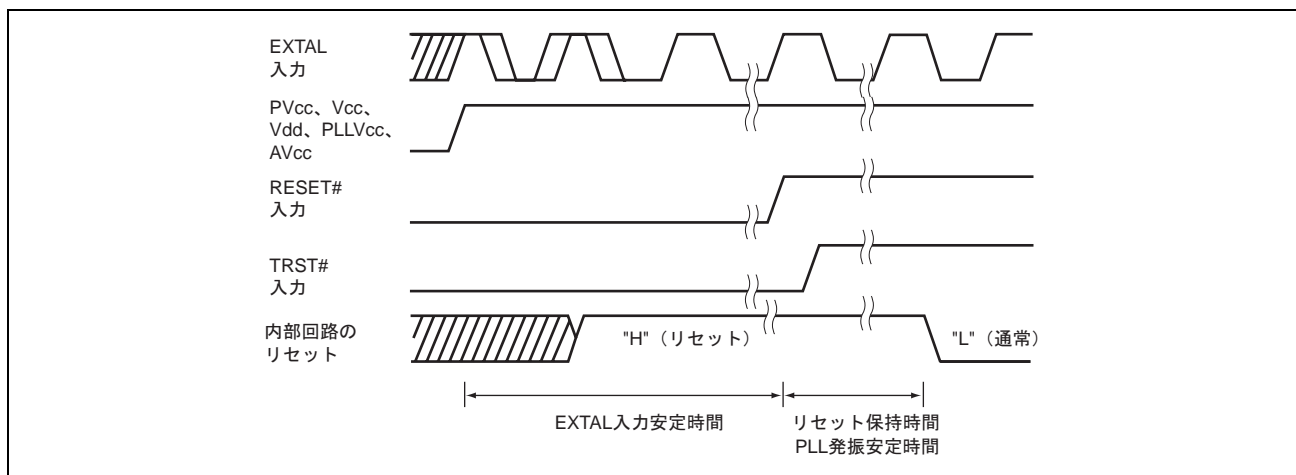
図 16.2 電源投入時のリセット
