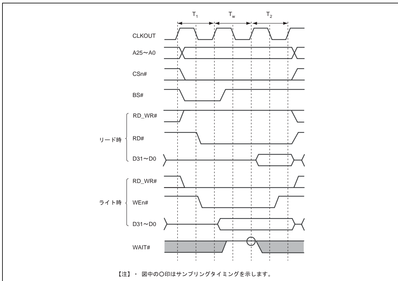
図 19.7 SRAM インタフェース ウェイトタイミング (ソフトウェアウェイトのみ)
