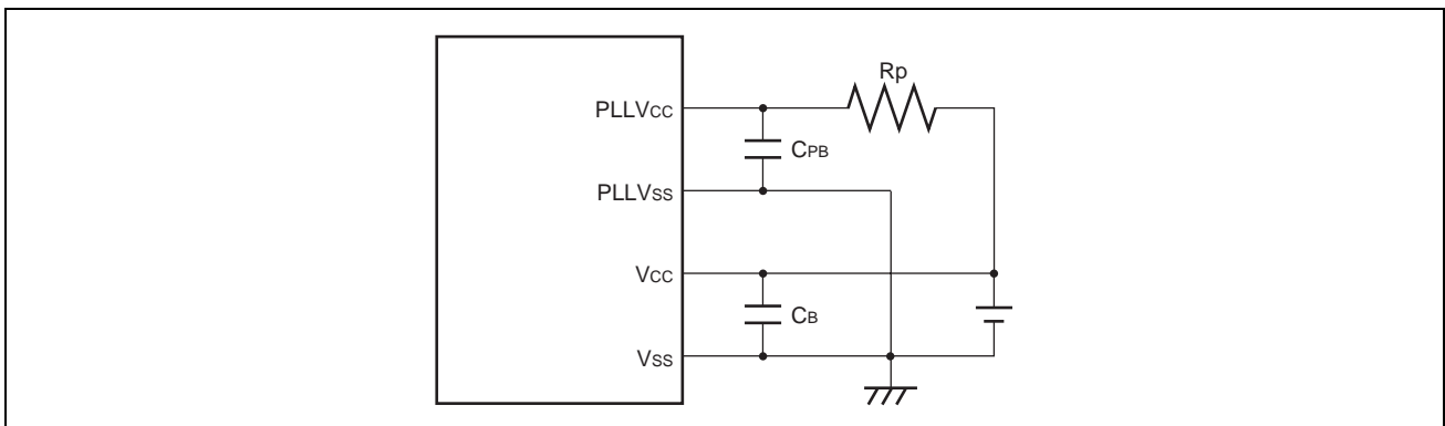
図 14.6 PLL 逡倍回路用電源接続時の注意事項
