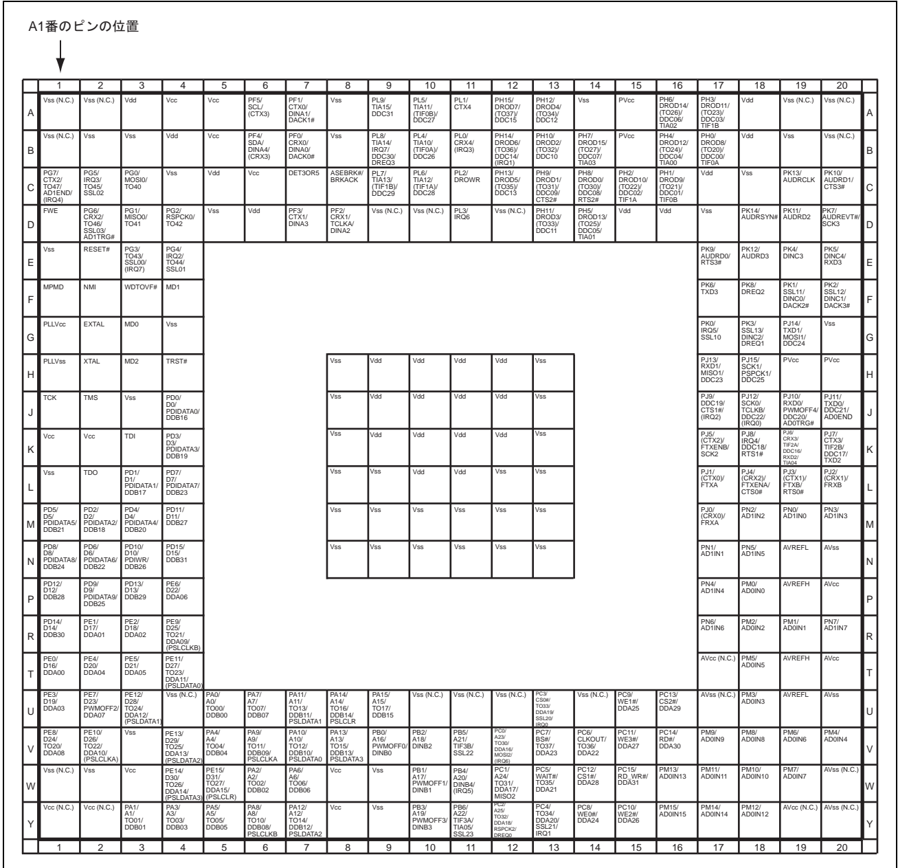
図 1.2 ピン配置図 (上面透視図)
