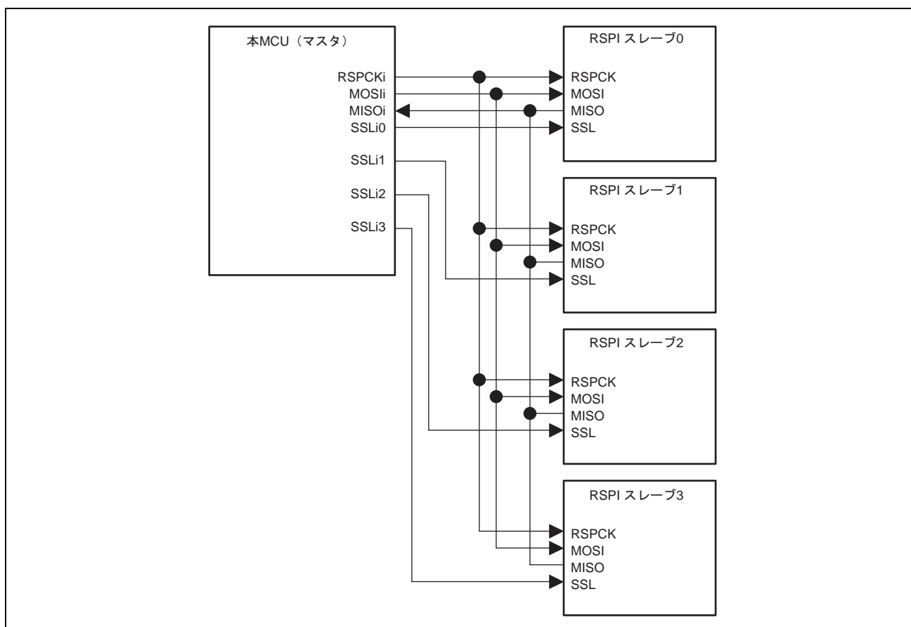
図 24.6 シングルマスタ/マルチスレーブの構成例 (本 MCU=マスタ)
