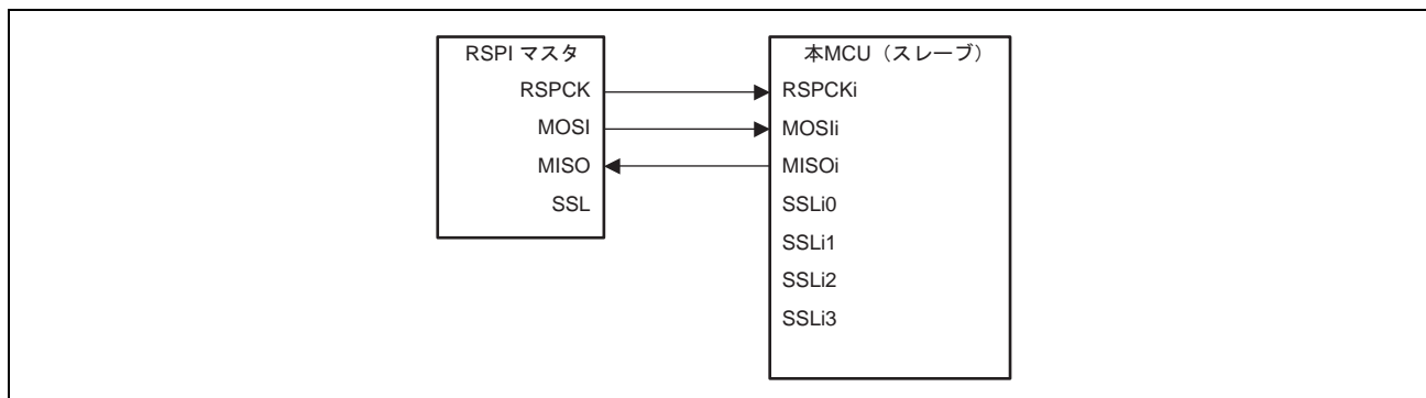
図 24.10 マスタ (クロック同期式動作) /スレーブ (クロック同期式動作) の構成例 (本 MCU = スレーブ、CPHA = "1")
