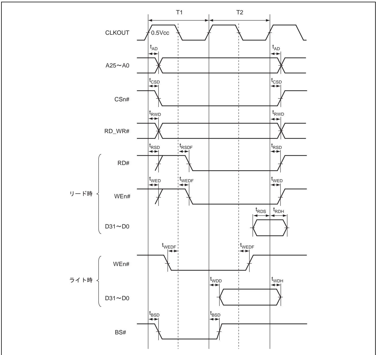
図 38.16 バイト制御 SRAM バスサイクル (ノーウェイト)
