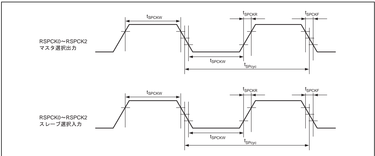
図 38.27 RSPCK クロックタイミング
