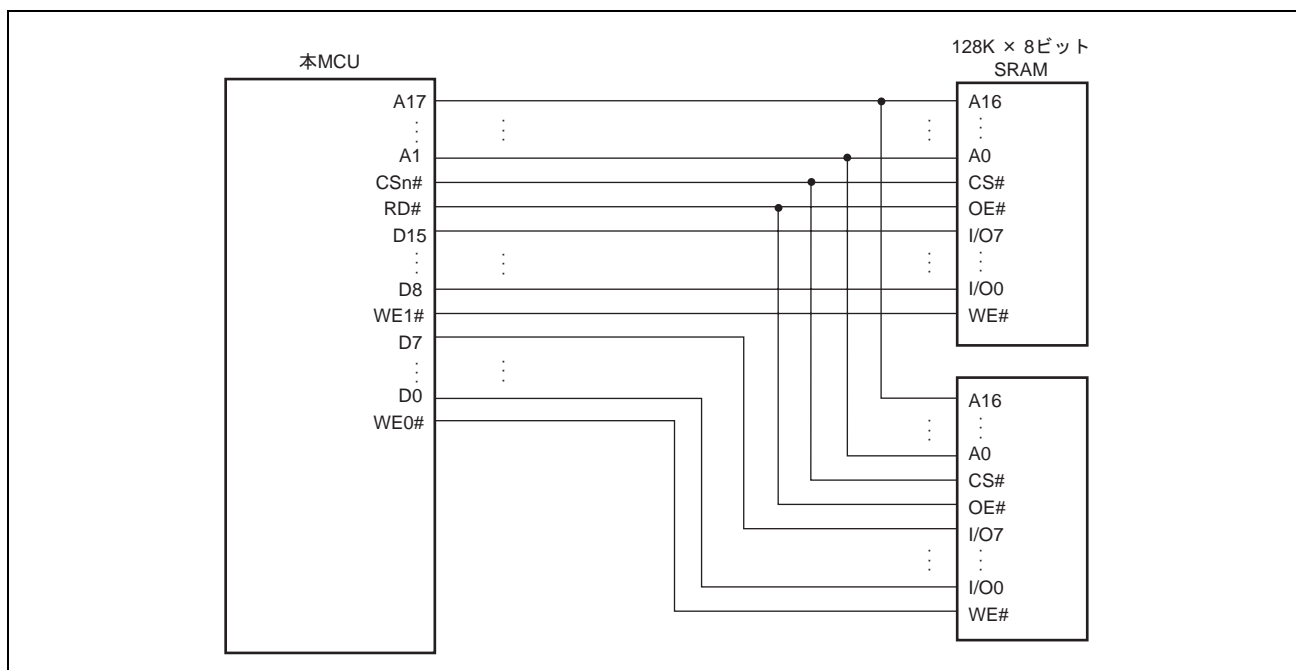
図 19.5 16ビットデータ幅 SRAM 接続例
