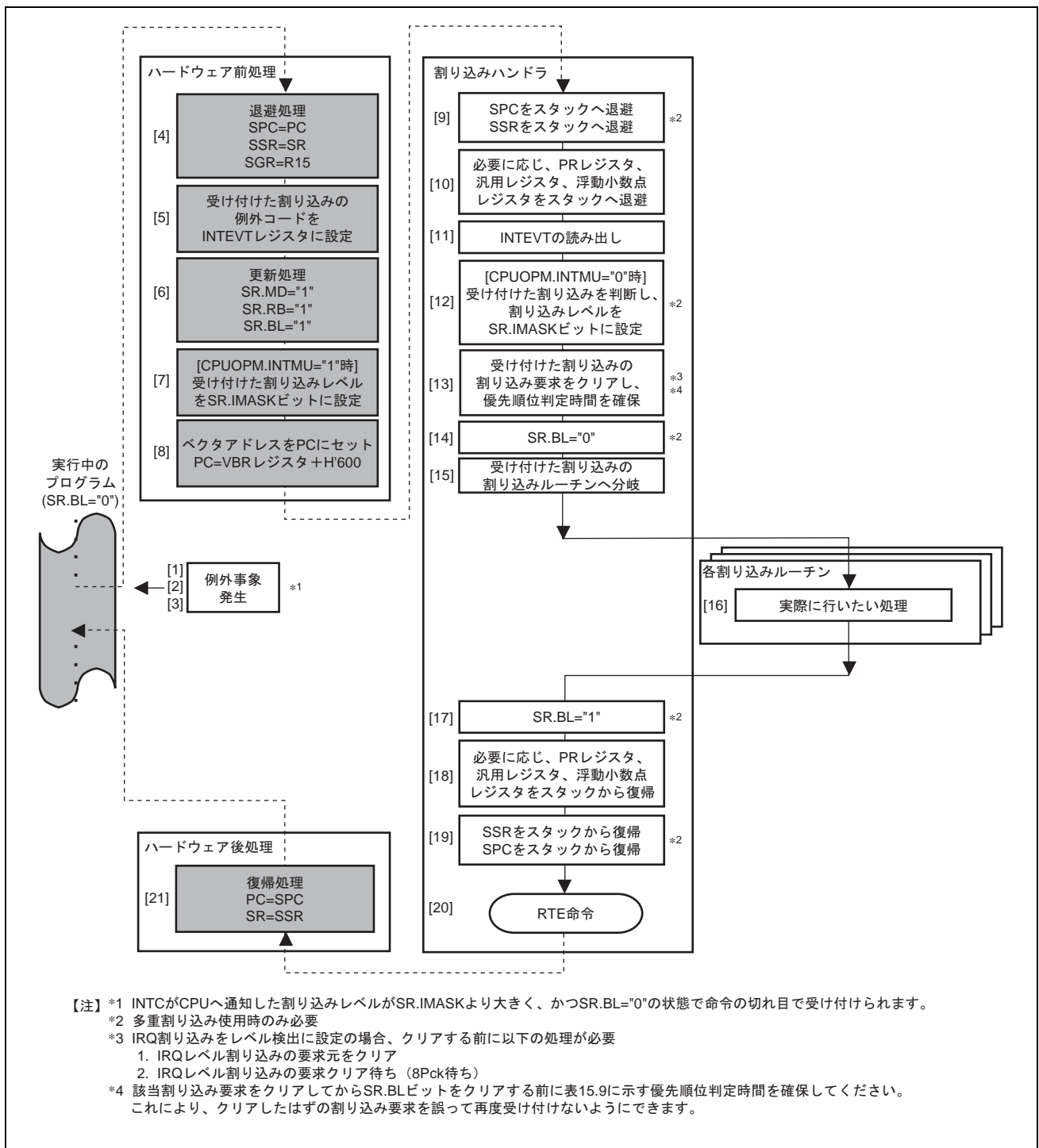
図 15.4 一般割り込みの動作例 1
