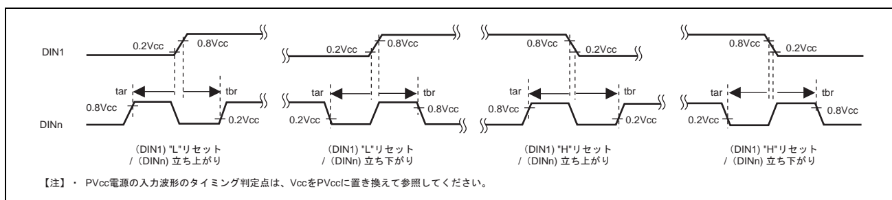
図 38.35 特殊モード時の DIN1/DIN2~DIN4 に関わるタイミング (DIN1 によるリセット解除エッジとその前後のサンプリングエッジ間隔)
