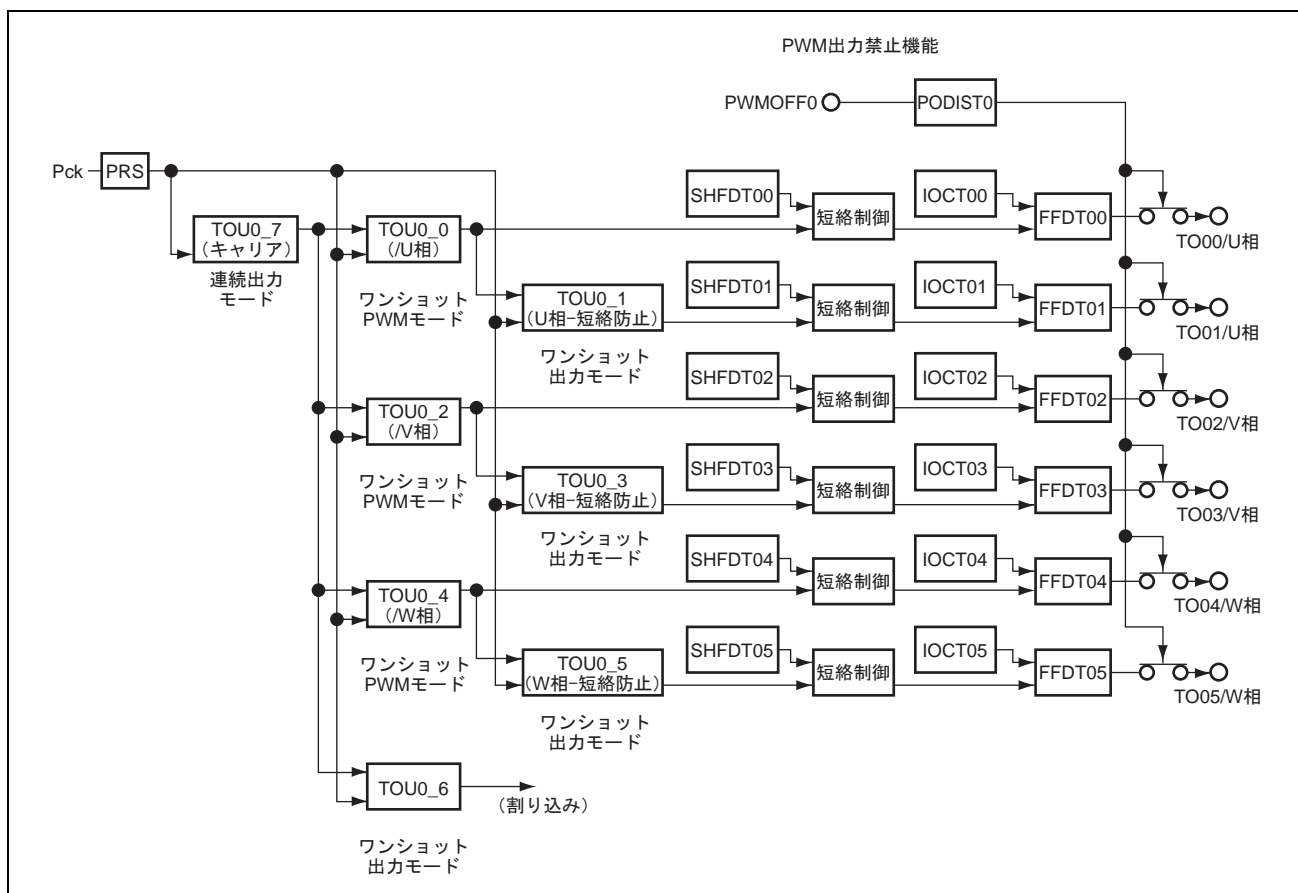
図 21.49 タイマ構成図
