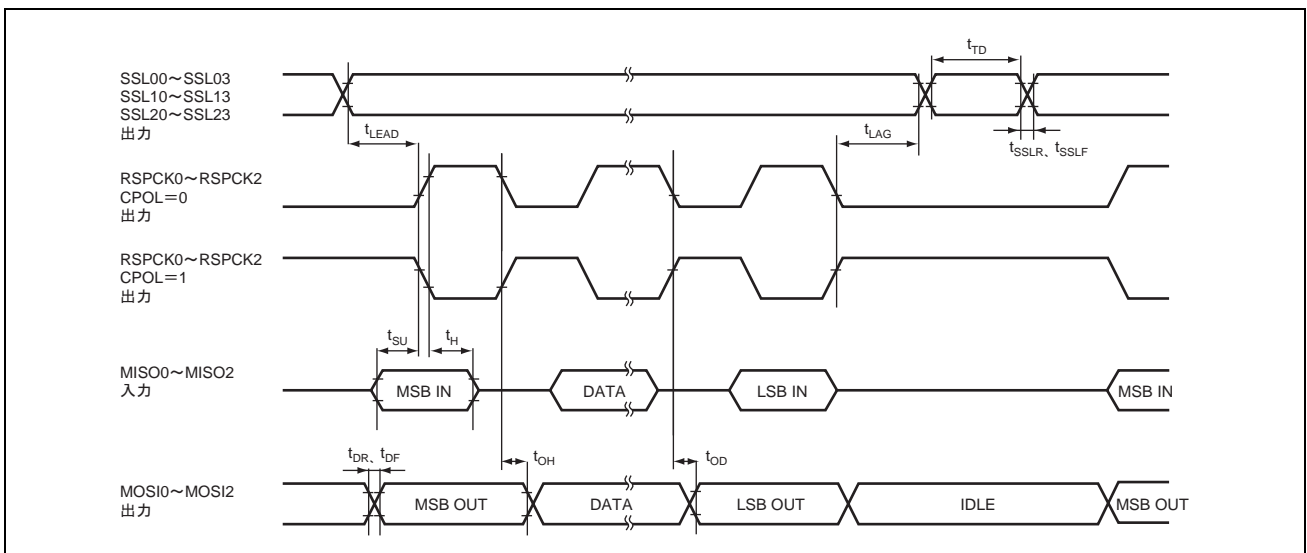
図 38.28 RSPCK タイミング (マスタ、CPHA="0")
