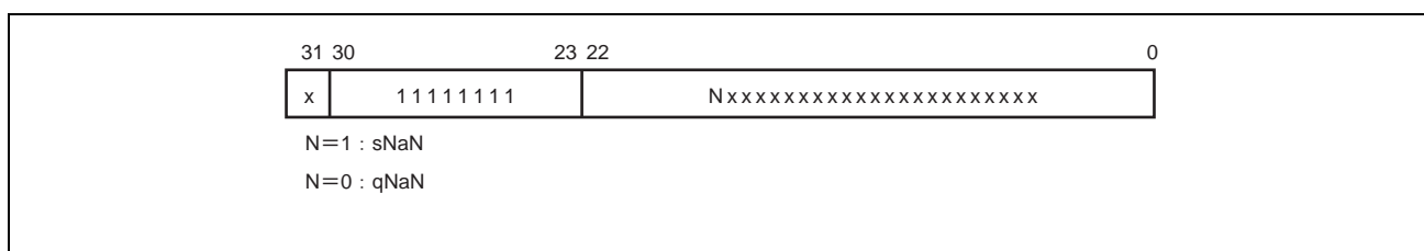
図 6.3 単精度の NaN ビットパターン
