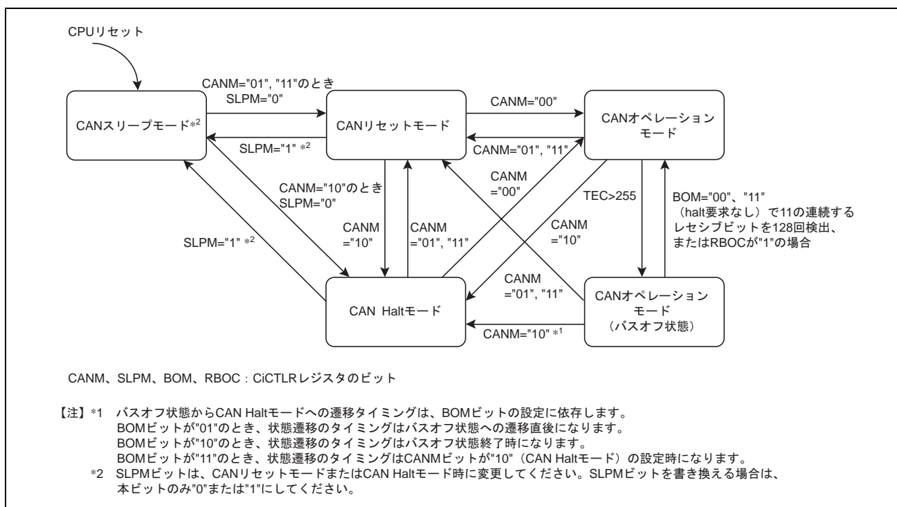
図 26.9 CAN 動作モード間の遷移 (i=0~4)
