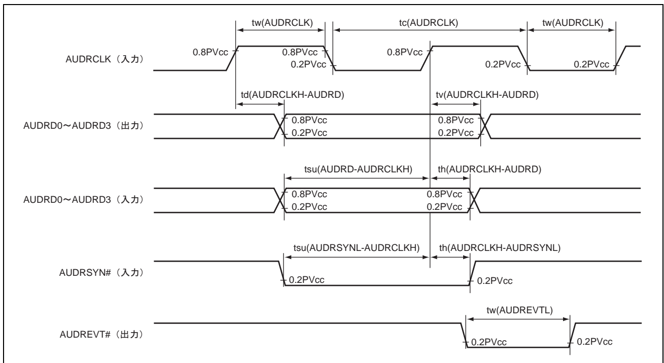
図 38.46 AUDR モジュールタイミング
