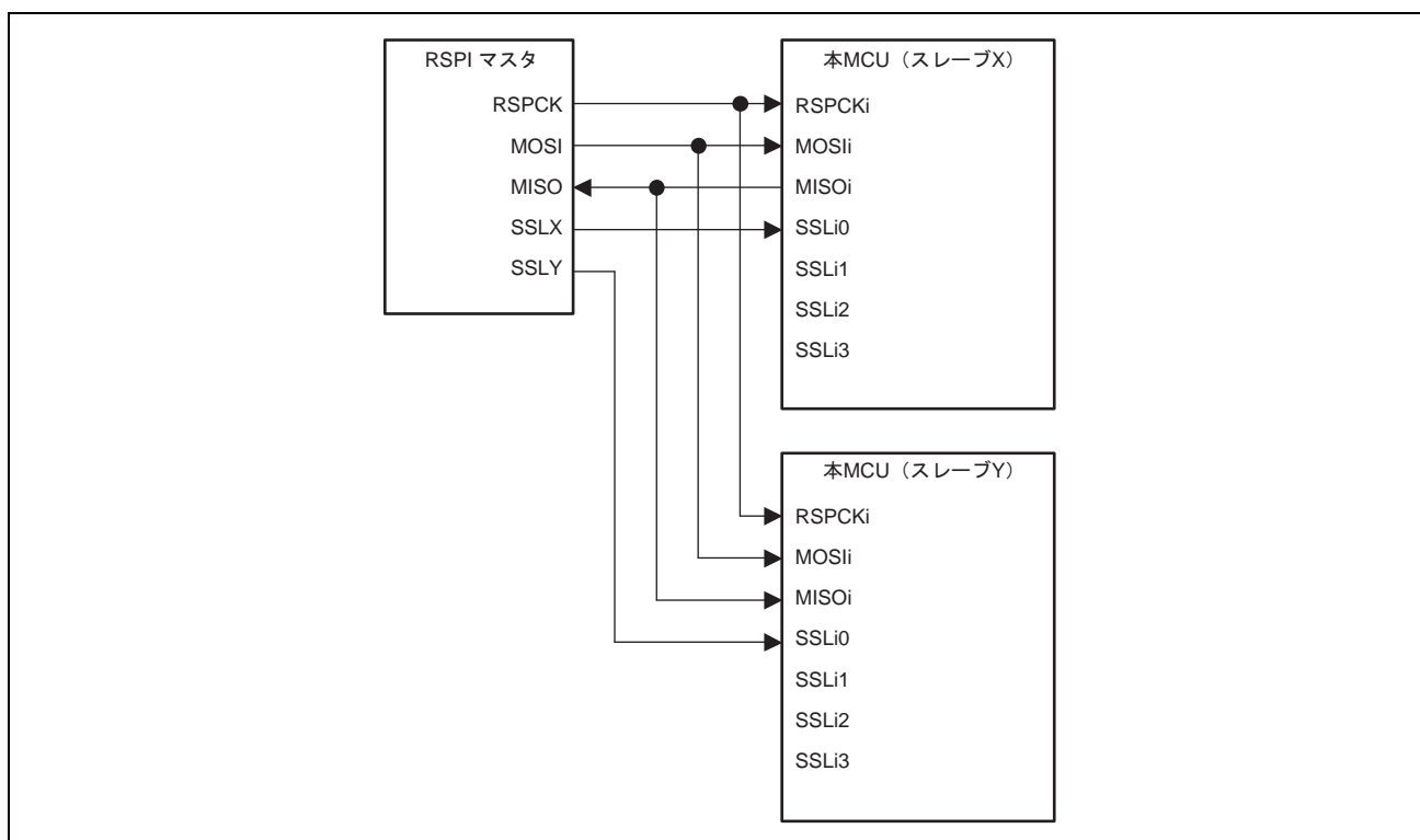
図 24.7 シングルマスタ/マルチスレーブの構成例 (本 MCU=スレーブ)
