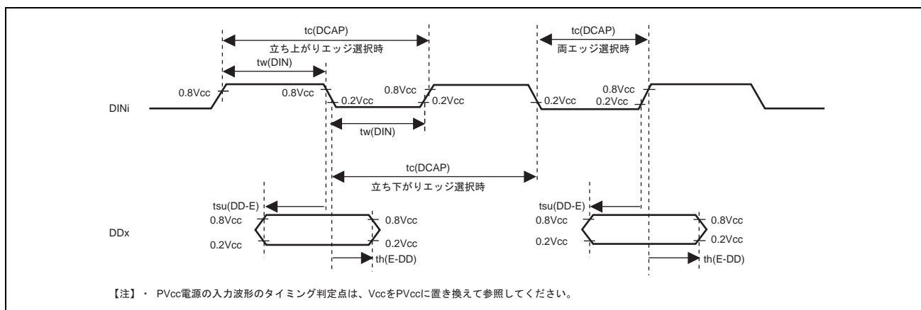
図 38.33 データ取り込み関連タイミング
