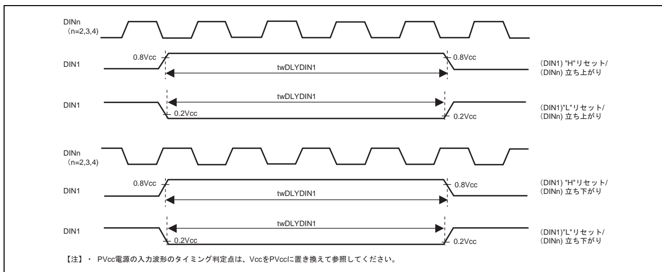
図 38.36 ディレイリセットモード時の DIN1 による初期化レベルの最低 DIN エッジ数 (初期化レベル最低幅)
