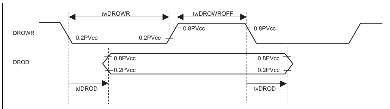
図 38.37 "L"アクティブ選択時のストロブ極性
