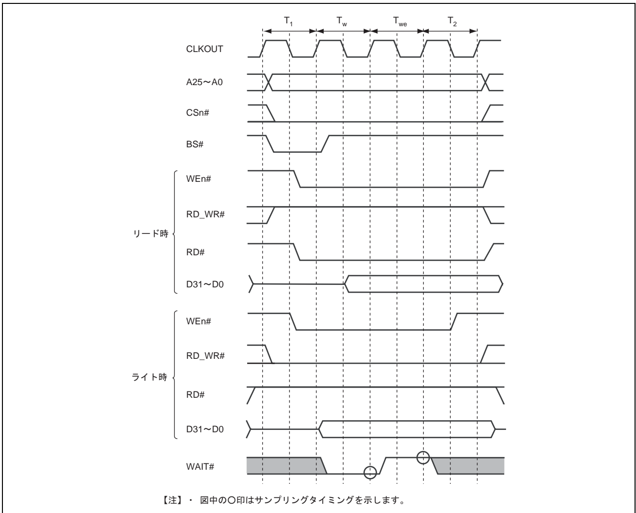
図 19.14 バイト制御 SRAM 基本アクセスタイミング (内部ウェイト 1 サイクル+外部 1 ウェイト)
