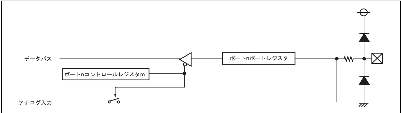
図 18.5 ポート周辺回路図（入力ポート 1）
