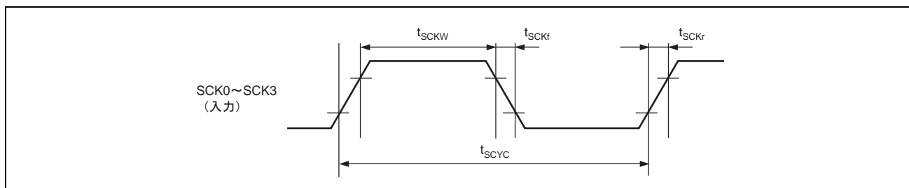
図 38.25 SCK 入力タイミング
