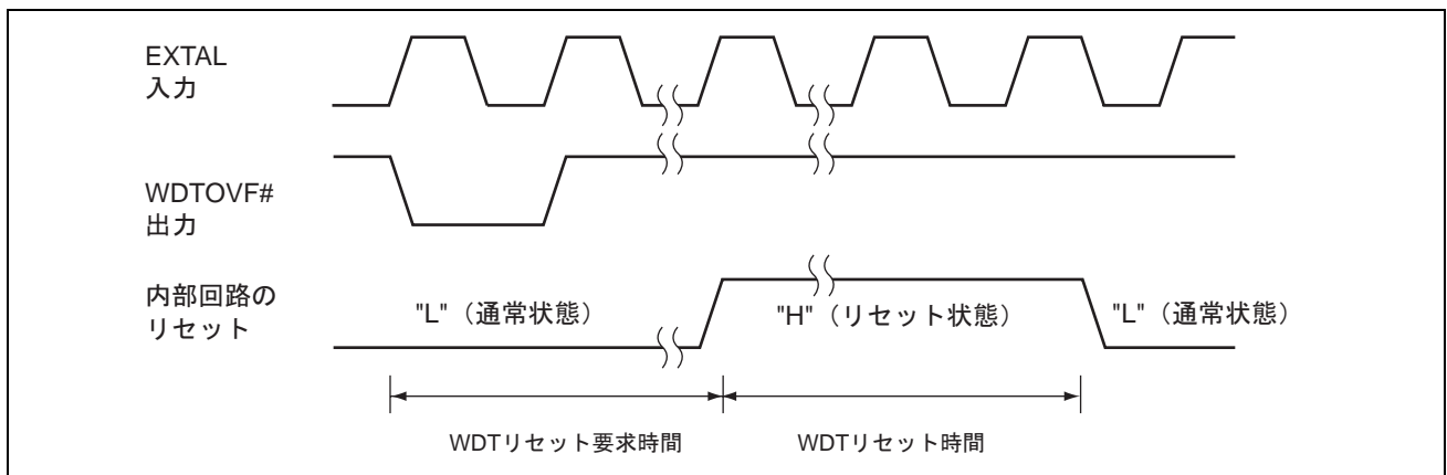
図 17.3 通常動作中の WDT オーバフローによるリセット
