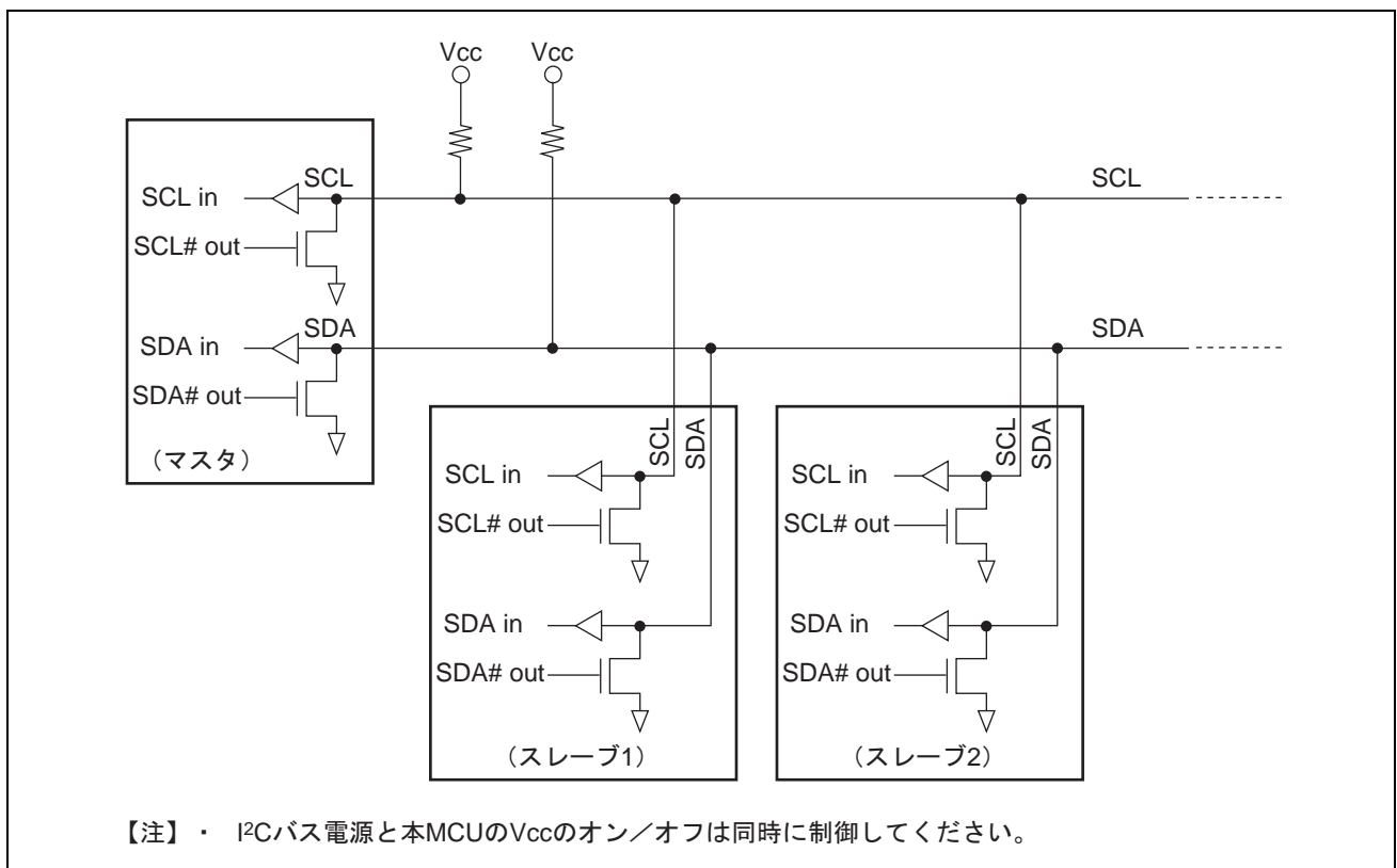
図 25.2 入出力端子の外部回路接続例
