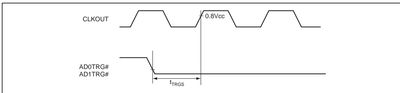
図 38.41 外部トリガ入力タイミング
