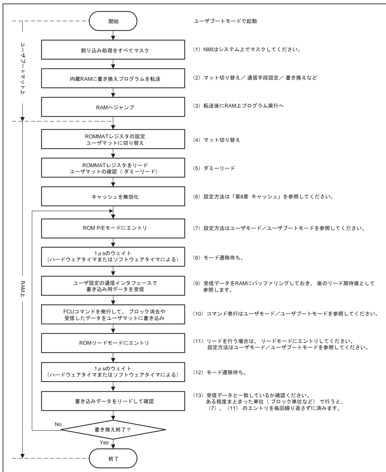
図 12.16 ユーザマットのプログラミング例
