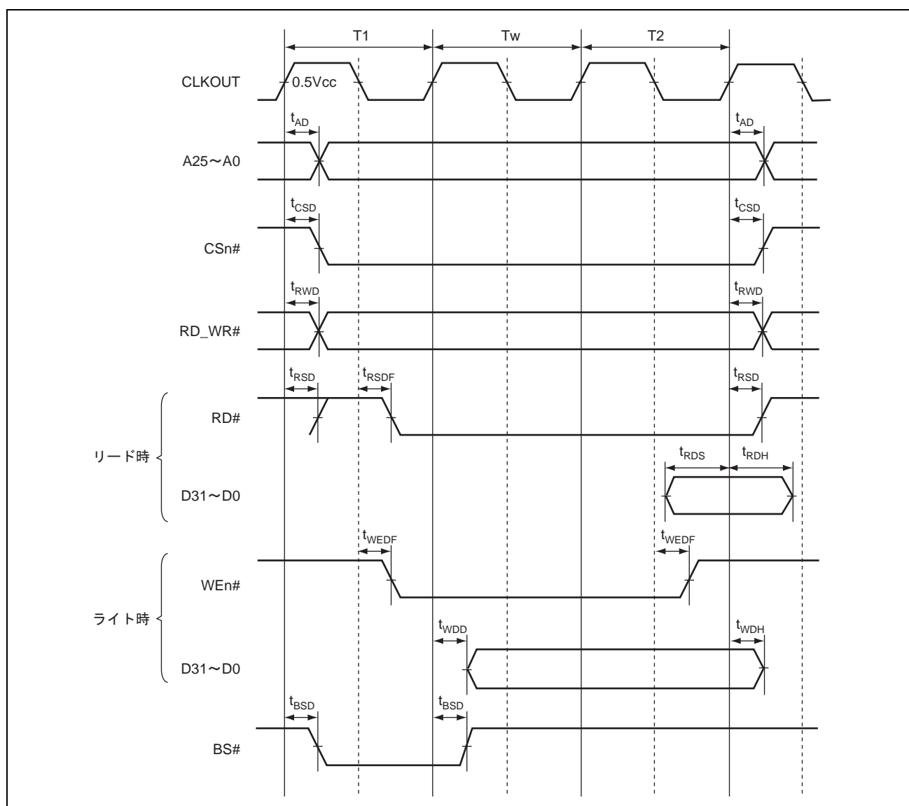
図 38.13 SRAM バスサイクル (ソフトウェアウェイト 1 サイクル)
