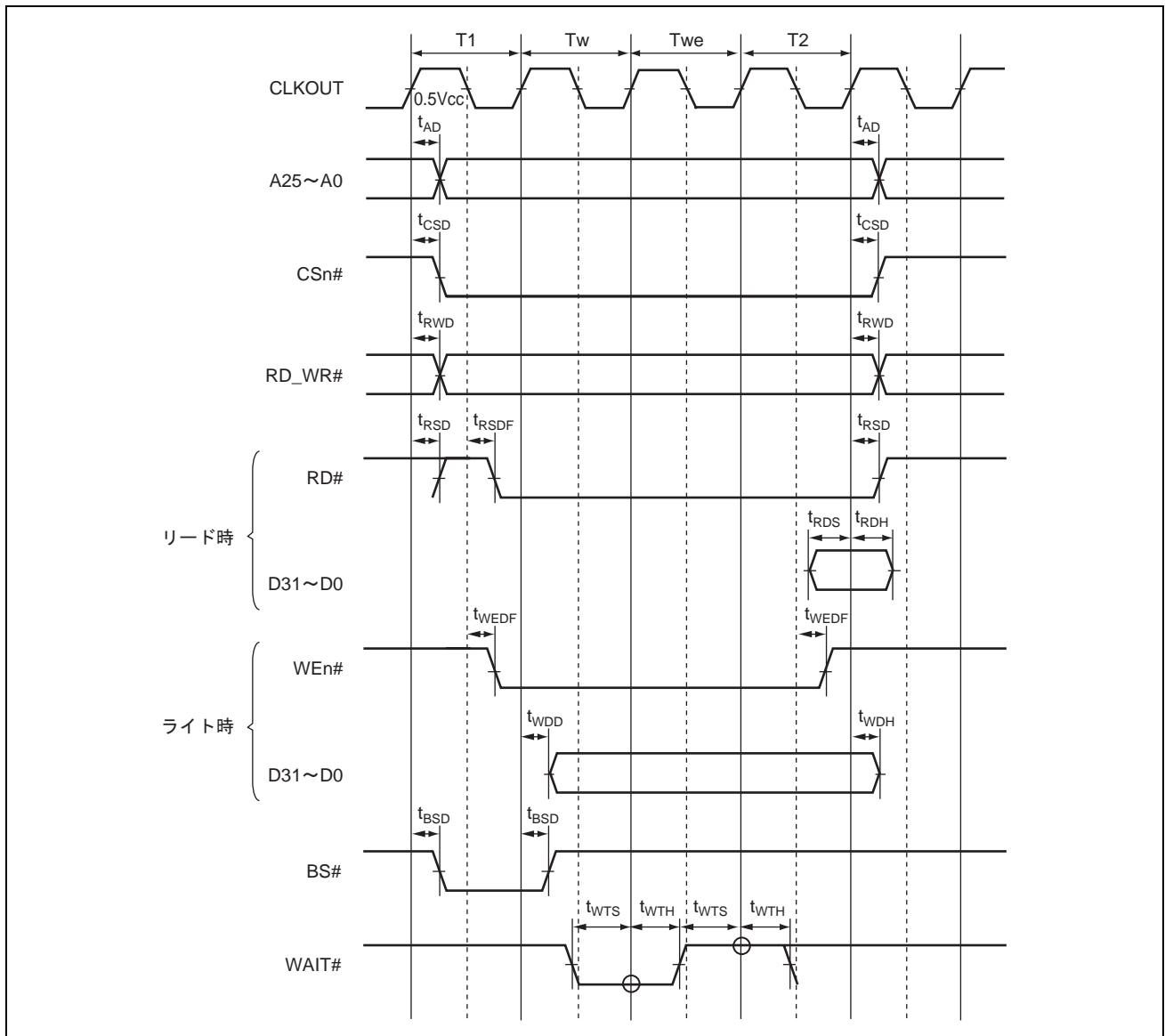
図 38.14 SRAM バスサイクル (ソフトウェアウエイト 1 サイクル+外部ウエイト 1 サイクル)
