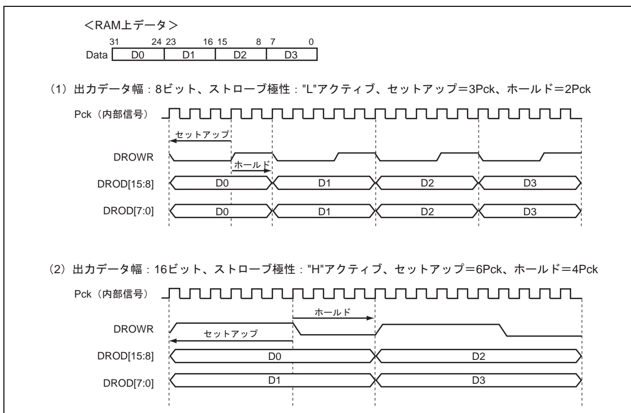
図 29.4 定周期出力のデータフォーマット例
