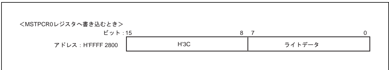
図 33.1 MSTPCR0 レジスタへの書き込み
