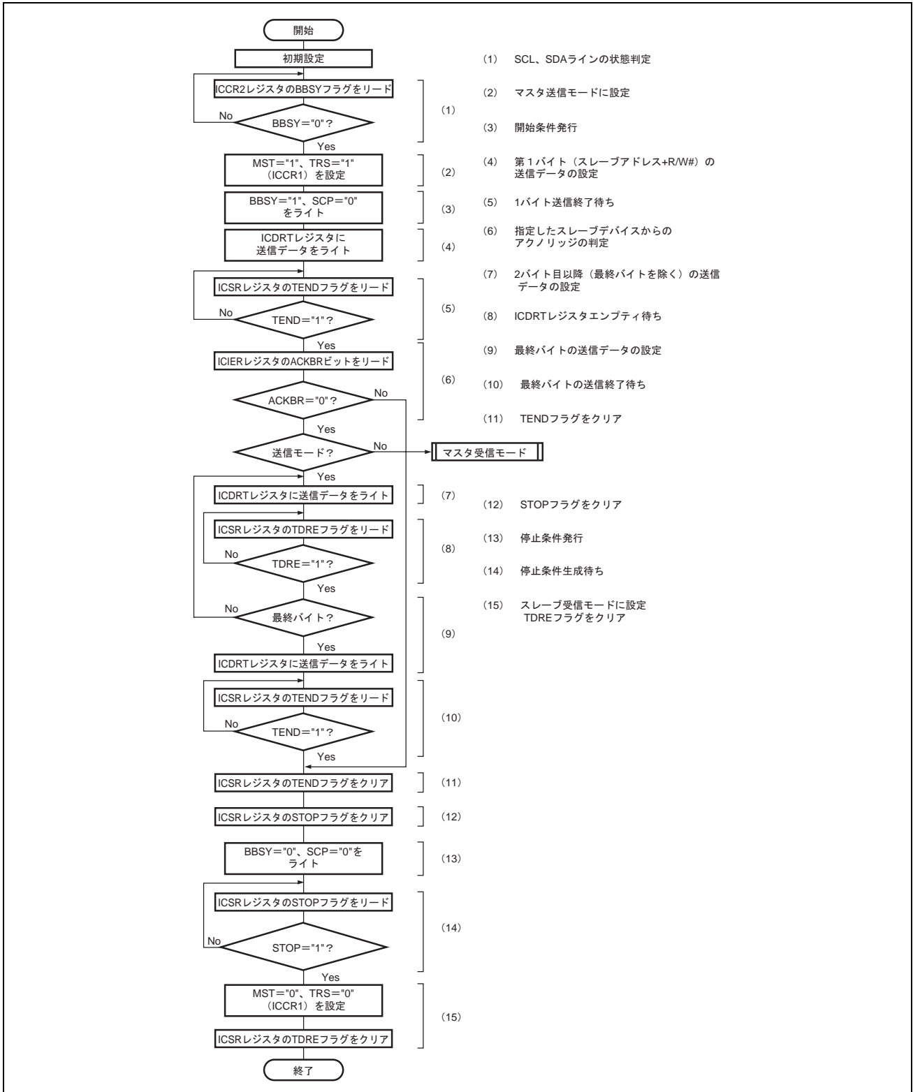
図 25.19 マスタ送信モードのフローチャート例
