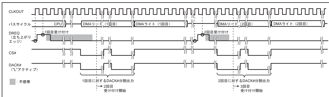
図 20.17 DACK#信号出力分割時のタイミング例 (サイクルスチールモード1または2・DACKリードサイクル出力)
