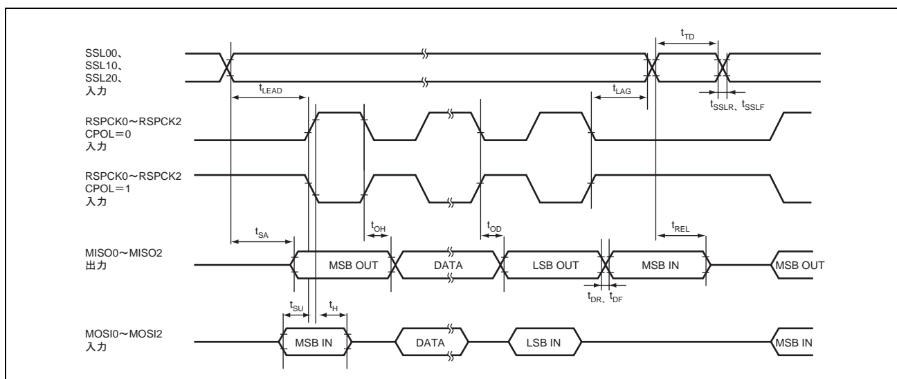
図 38.30 RSPI タイミング (スレーブ、CPHA="0")
