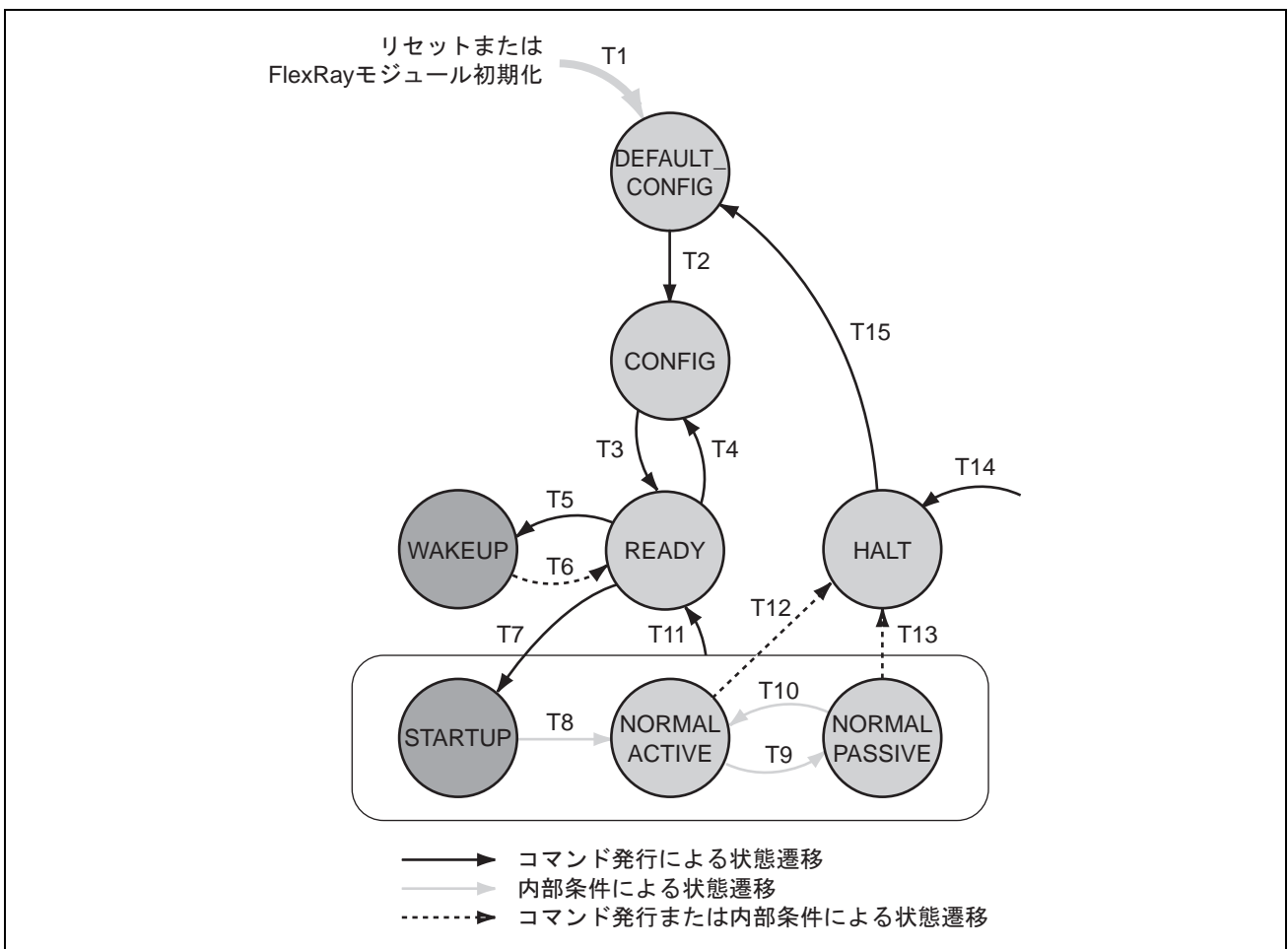
図 32.6 FlexRay モジュールの状態遷移図
