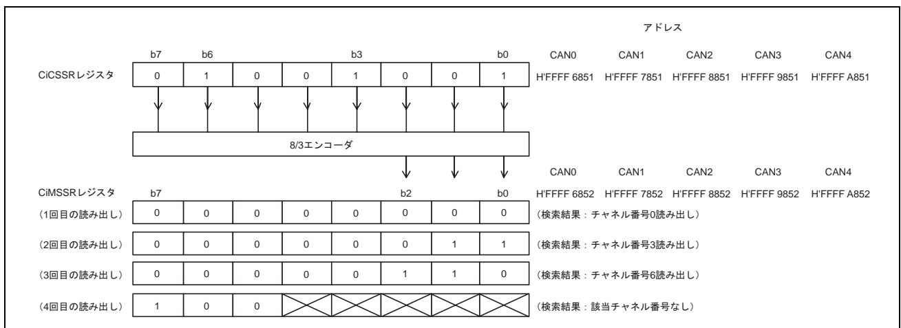
図 26.4 CiCSSR、CiMSSR レジスタの書き込みと読み出し (i=0~4)
