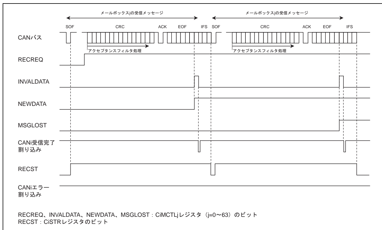
図 26.18 データフレーム受信時の動作例（オーバーライトモードの場合） (i=0~4)
