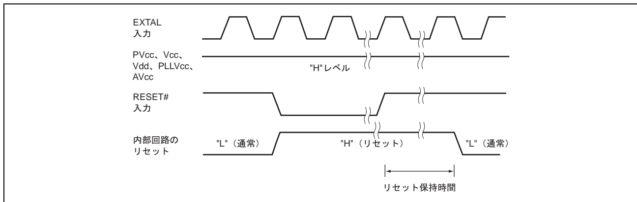
図 16.3 動作中のリセット
