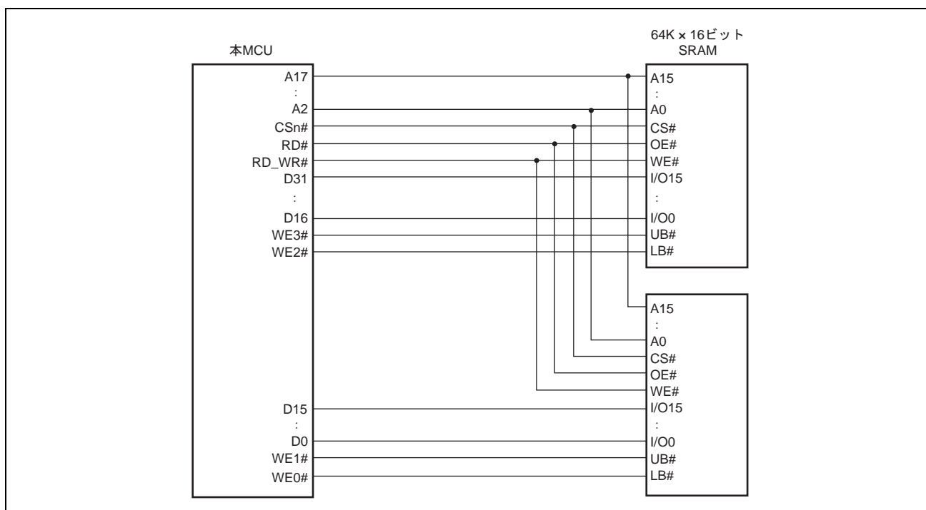
図 19.10 32 ビットデータ幅バイト制御 SRAM 接続例
