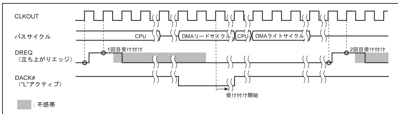
図 20.12 DREQ 入力検出タイミング例 (サイクルスチールモード 2・DACK リードサイクル出力)
