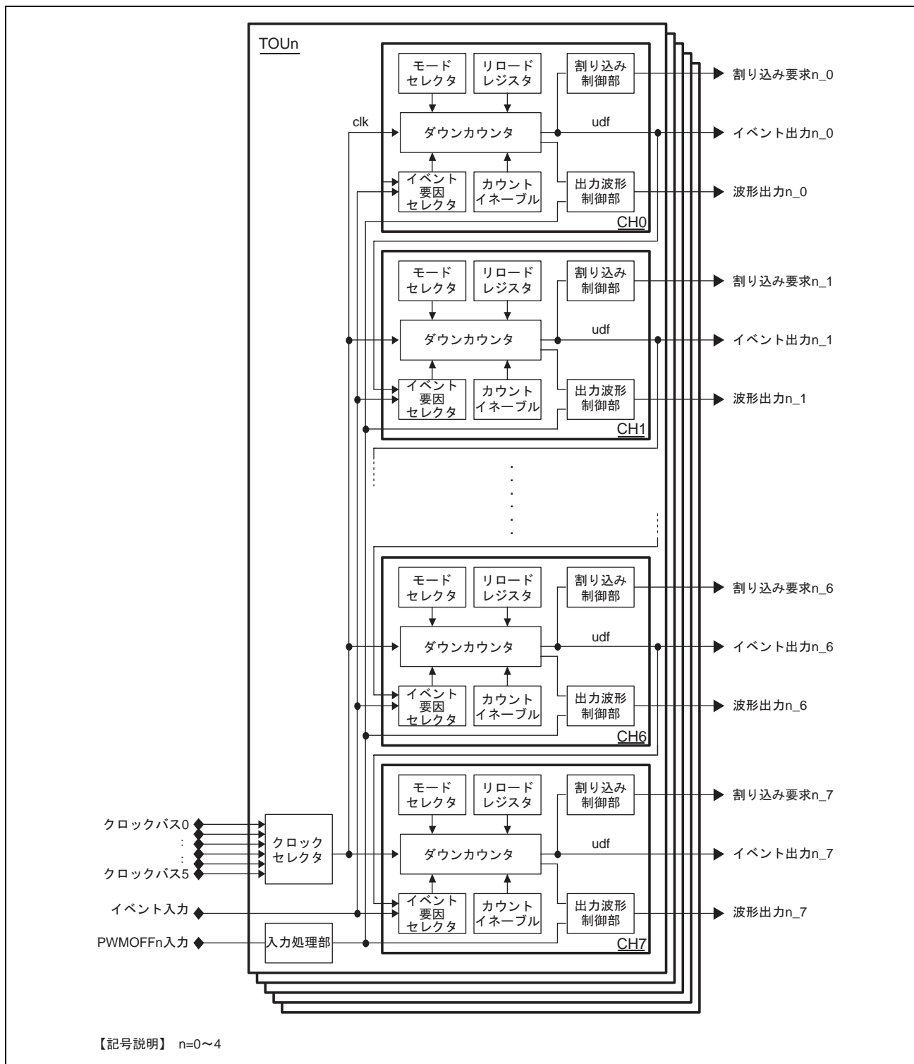
図 21.25 タイマ TOU (出力系 24 ビットタイマ) のブロック図
