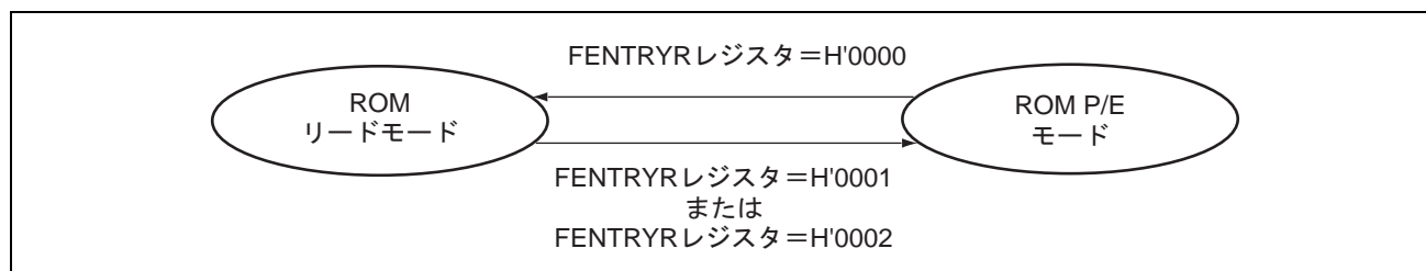
図 12.7 FCU のモード遷移図 (ROM 関連)
