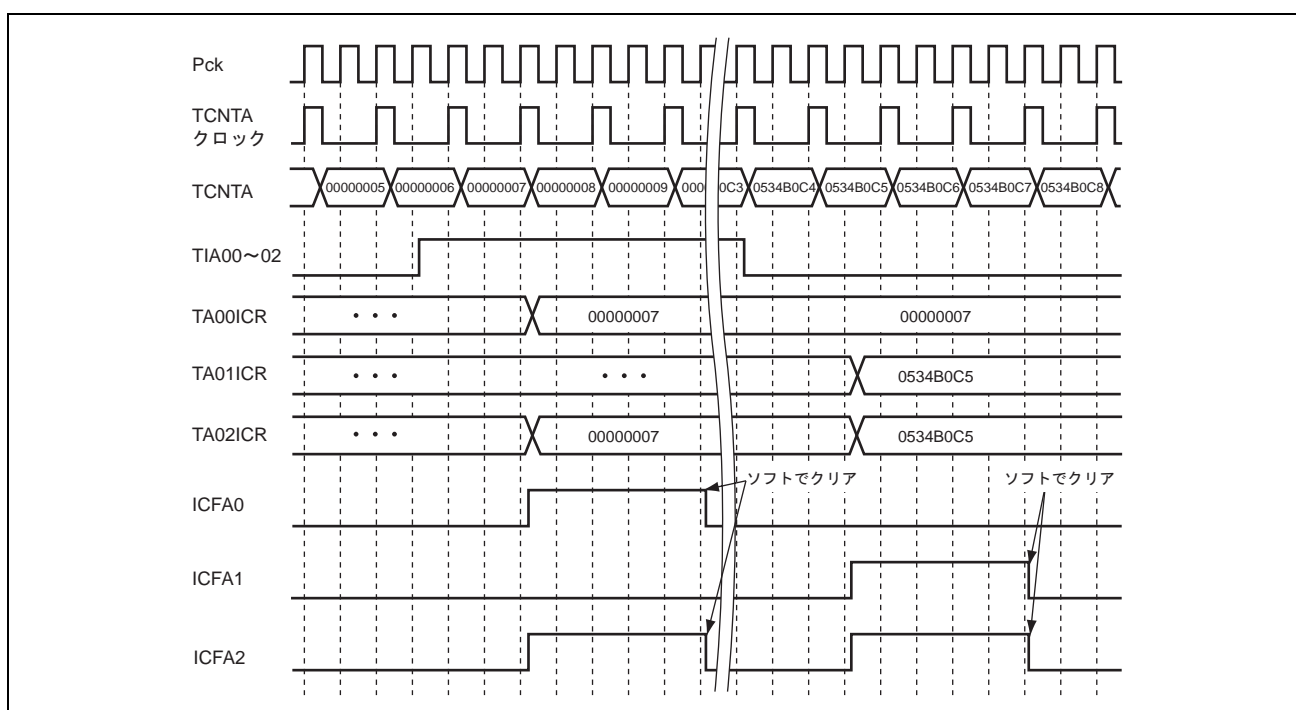
図 21.12 タイマ A のインพุットキャプチャ動作
