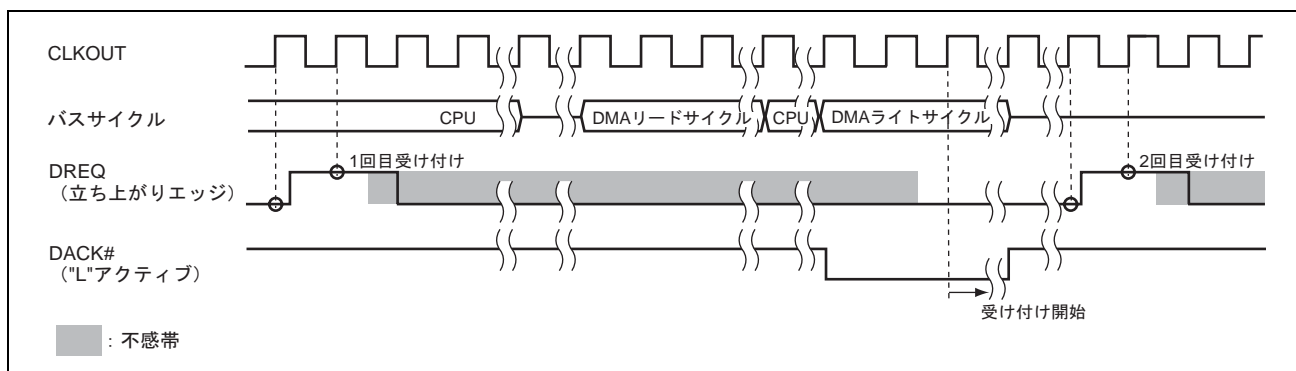
図 20.13 DREQ 入力検出タイミング例 (サイクルスチールモード 2・DACK ライトサイクル出力)
