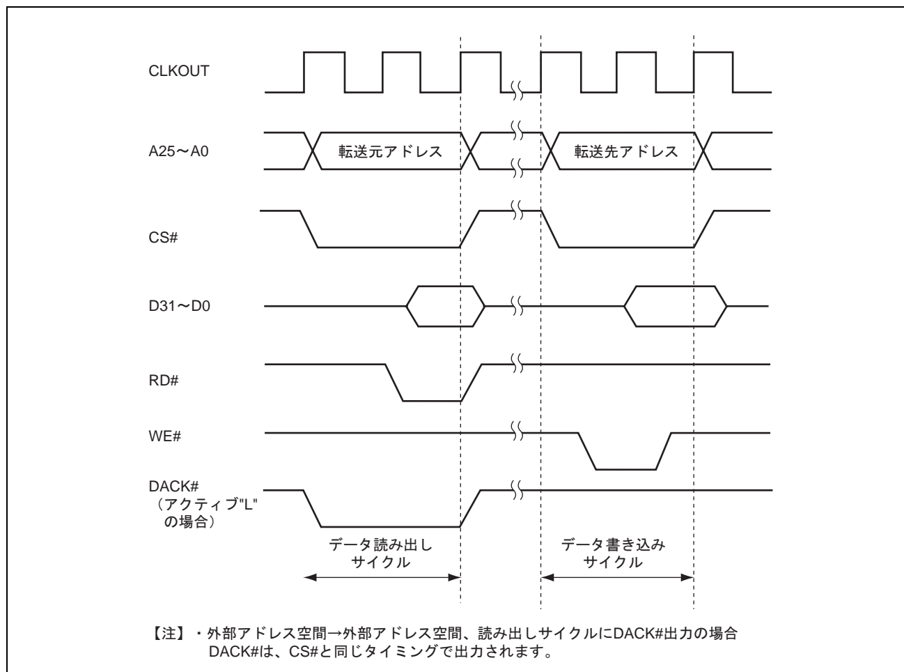
図 20.16 DACK#信号の出力タイミング例（転送元：外部アドレス空間、転送先：外部アドレス空間）
