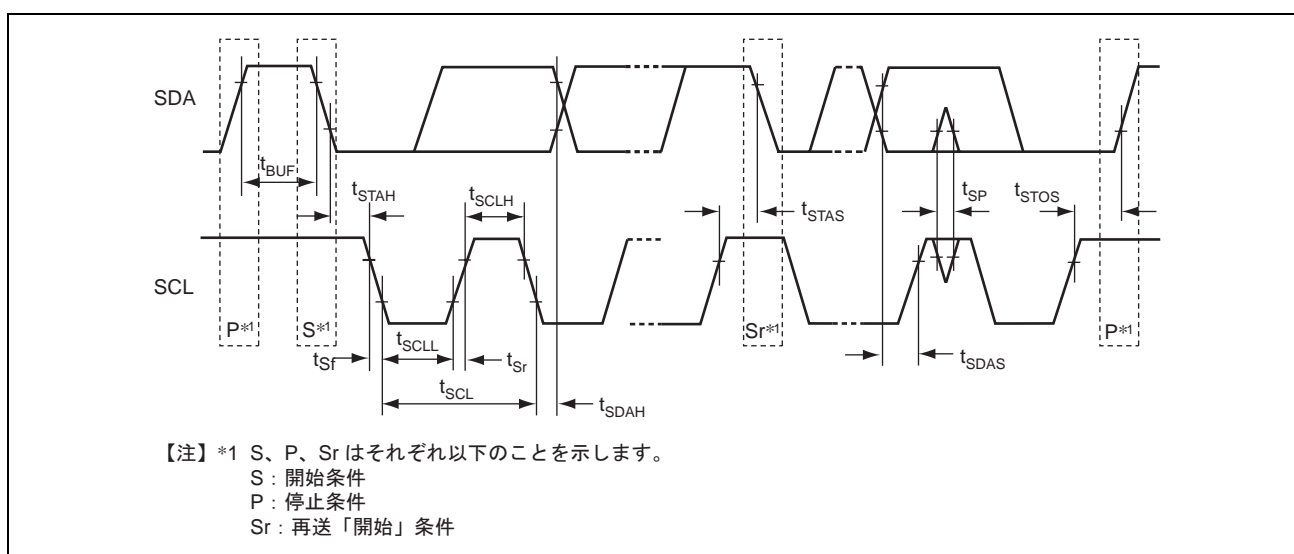
図 38.32 IIC3 モジュール入出力タイミング
