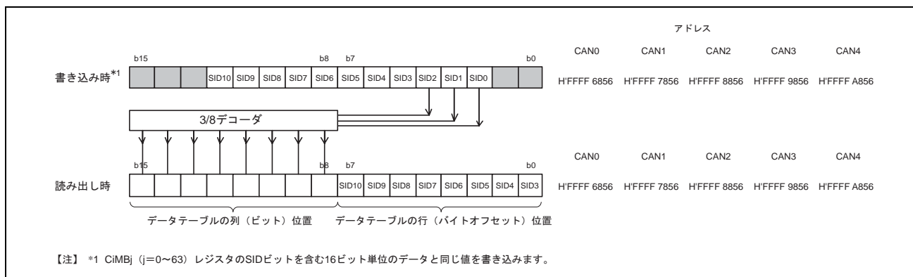
図 26.5 CiAFSR レジスタの書き込み、読み出し (i=0~4)
