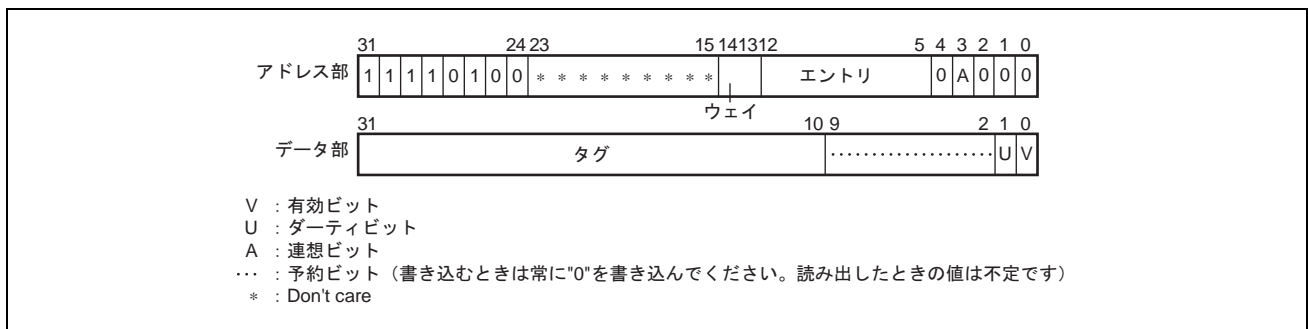
図 8.7 メモリ割り付け OC アドレスアレイ
