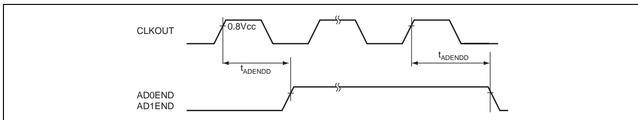
図 38.42 アナログ変換タイミング
