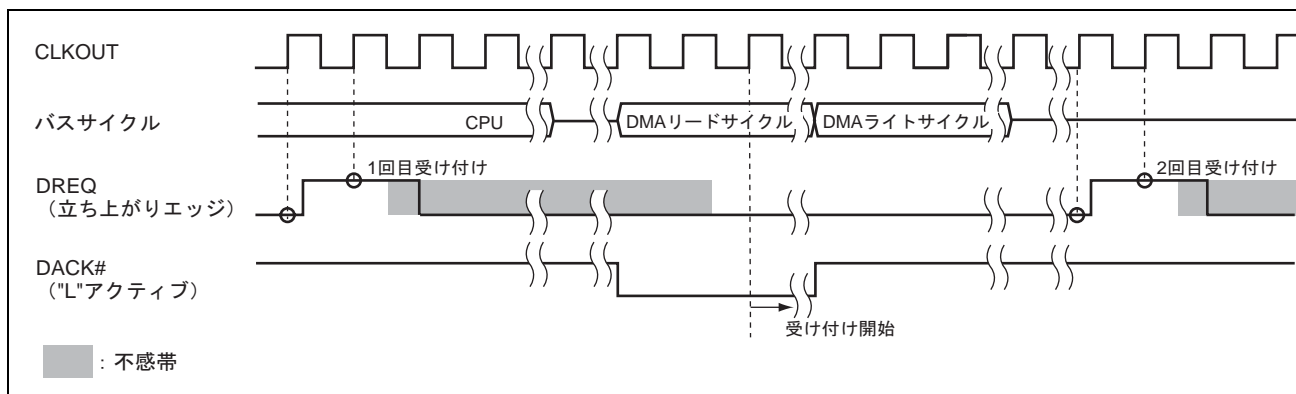
図 20.10 DREQ 入力検出タイミング例 (サイクルスチールモード 1・DACK リードサイクル出力)
