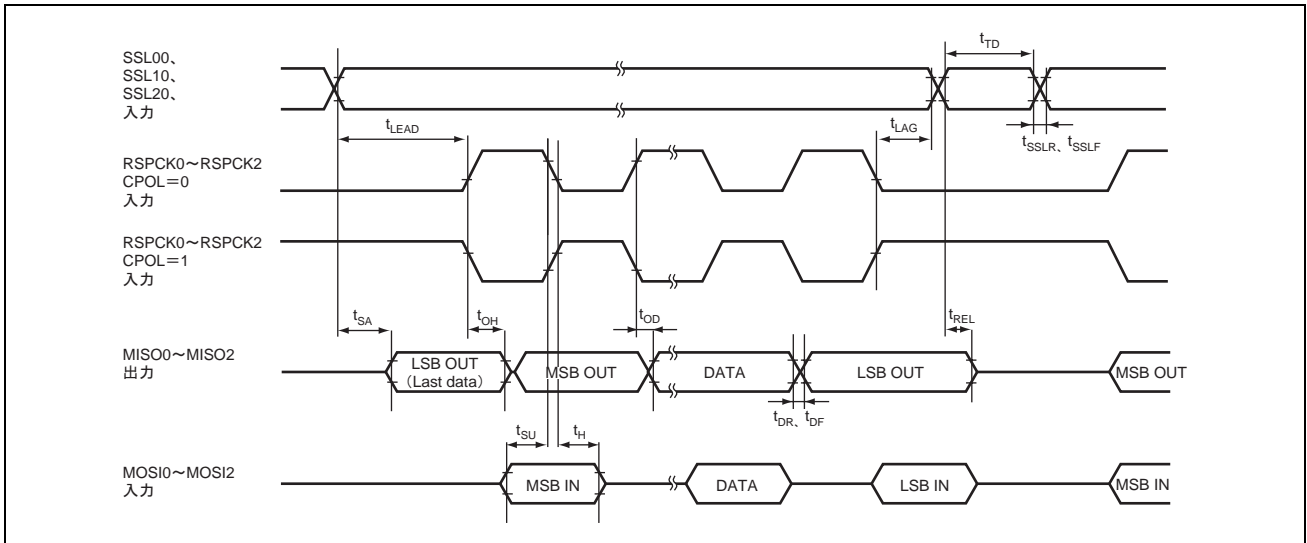
図 38.31 RSPI タイミング (スレーブ、CPHA="1")
