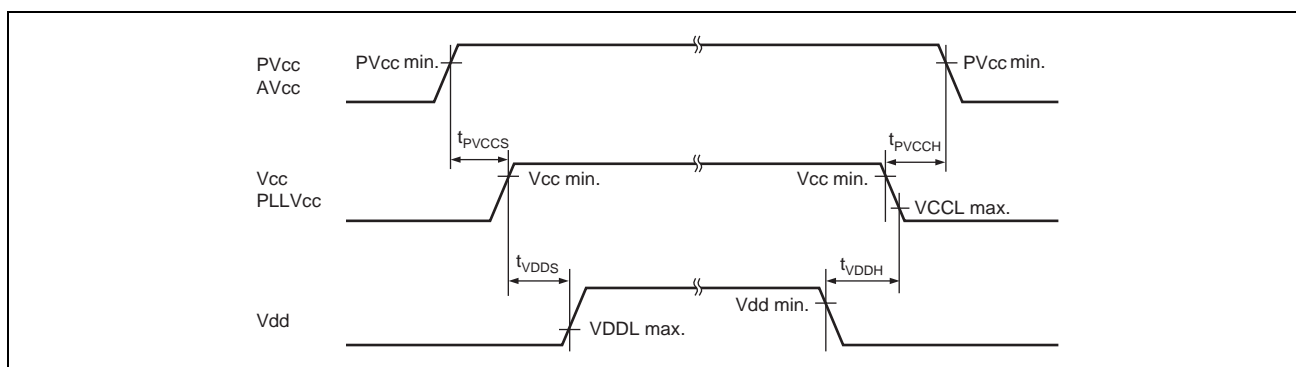
図 38.4 電源投入・切断タイミング
