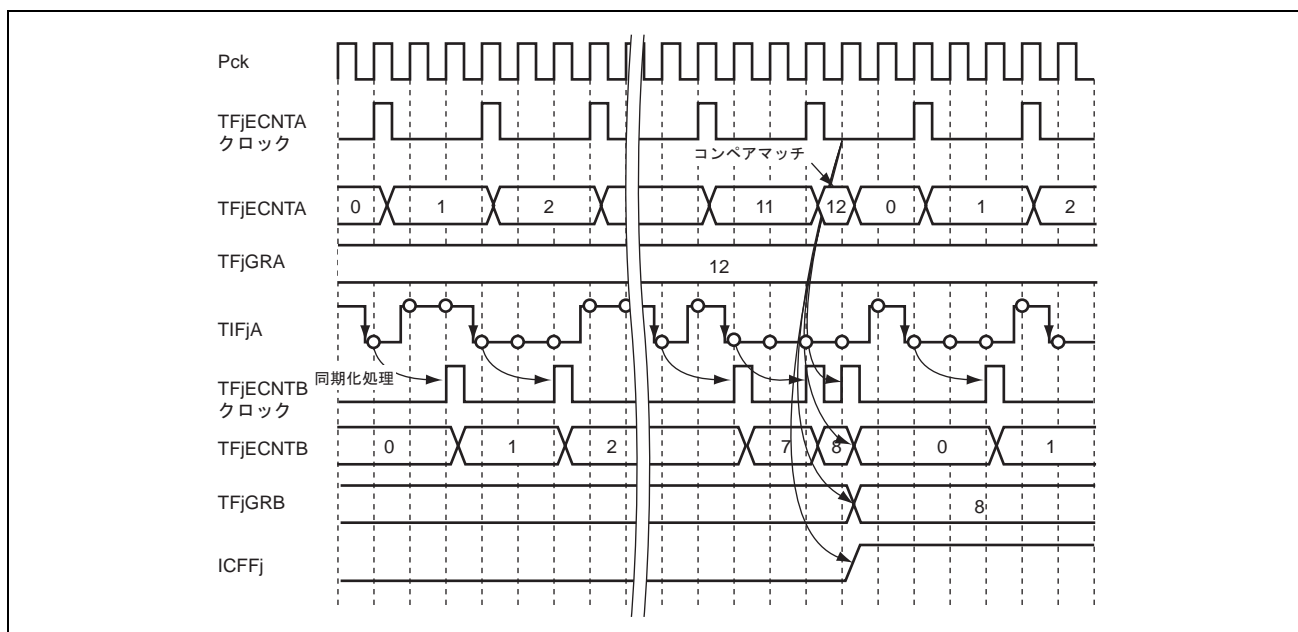
図 21.14 一定時間内エッジカウントの動作例
