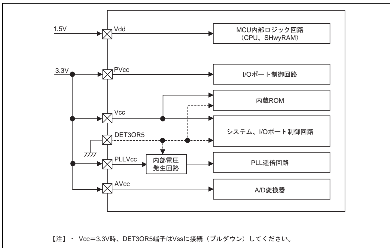
図 34.3 電源回路構成図 (PVcc=Vcc=3.3V 時)
