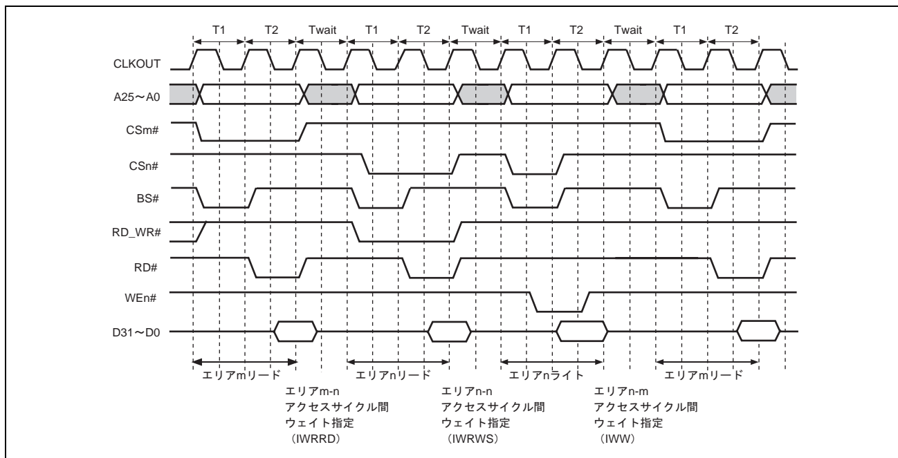
図 19.15 アクセスサイクル間ウェイト
