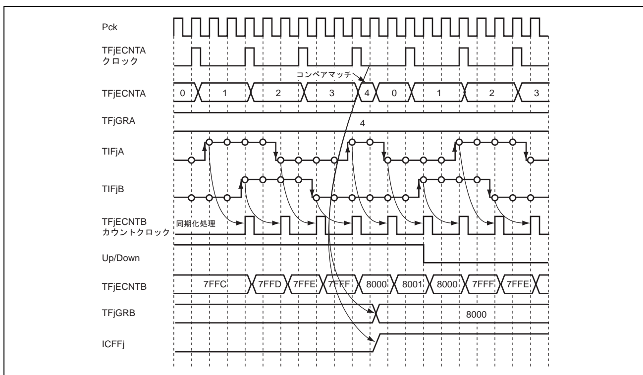
図 21.22 4 通倍イベントカウントの動作例
