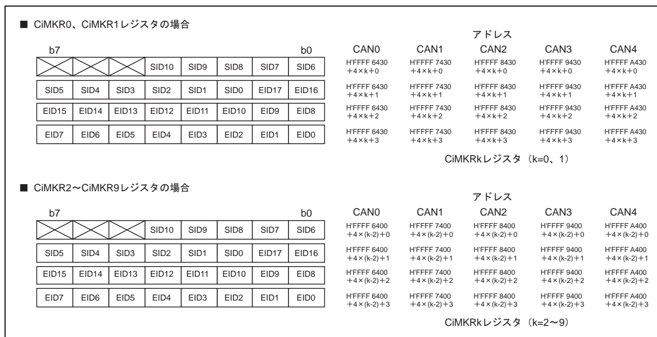
図 26.14 CiMKRk レジスタの構成 (i=0~4、k=0~9)
