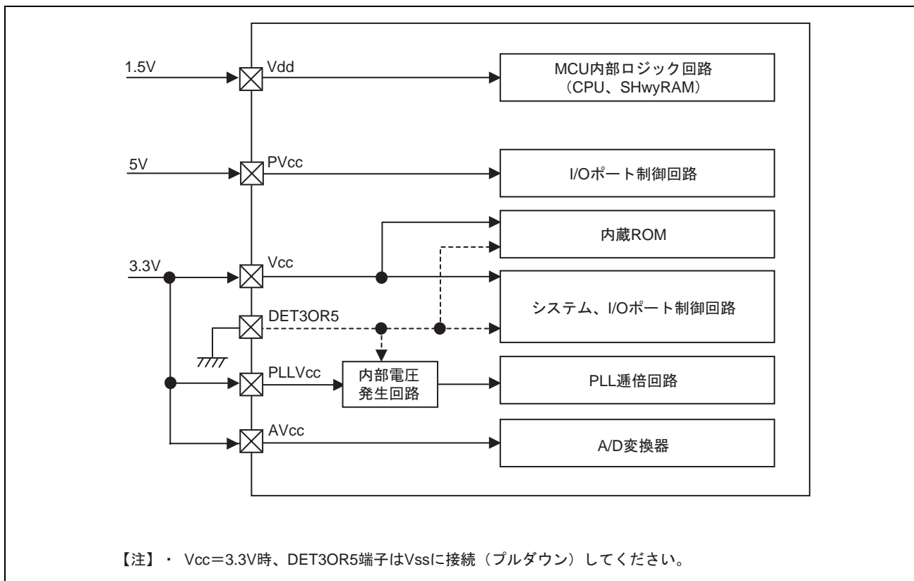
図 34.2 電源回路構成図 (PVcc=5V、Vcc=3.3V 時)
