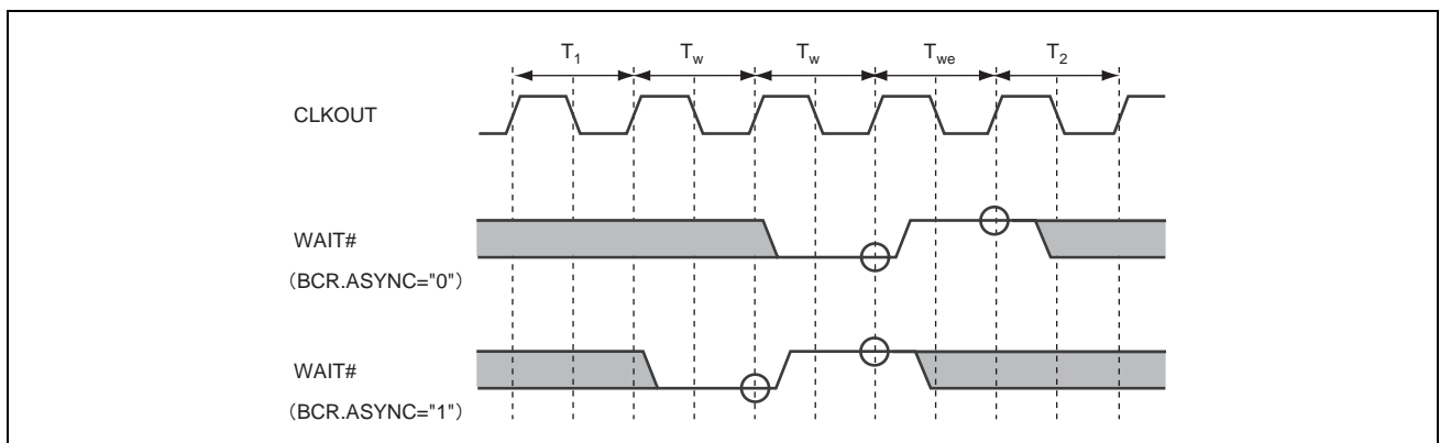
図 19.2 BCR.ASYNC の設定による WAIT#サンプリングタイミング例 (CSnWCR レジスタにより 2 サイクルウェイトが挿入されています。)
