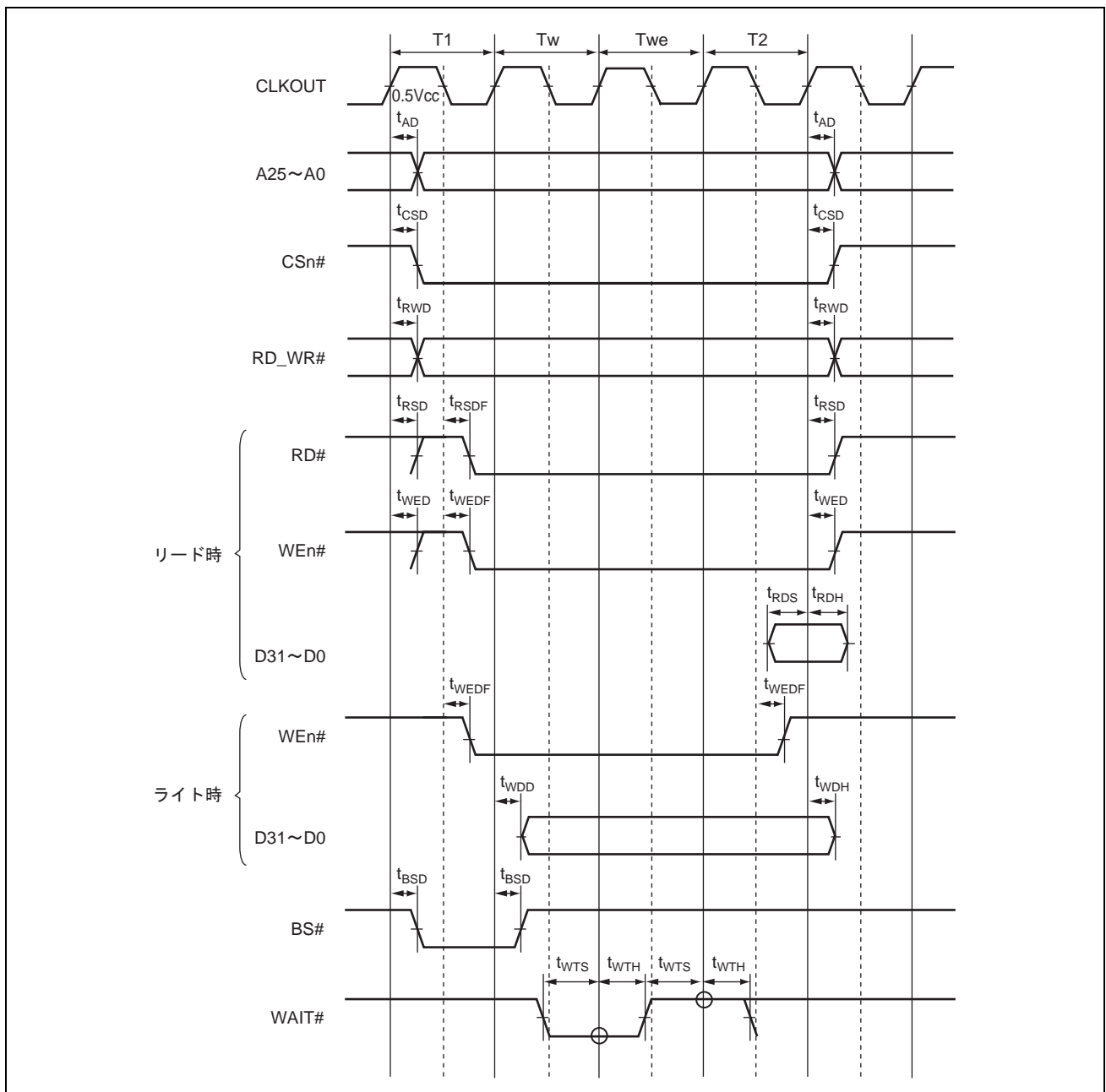
図 38.18 バイト制御 SRAM バスサイクル (ソフトウェアウェイト 1 サイクル+外部ウェイト 1 サイクル)
