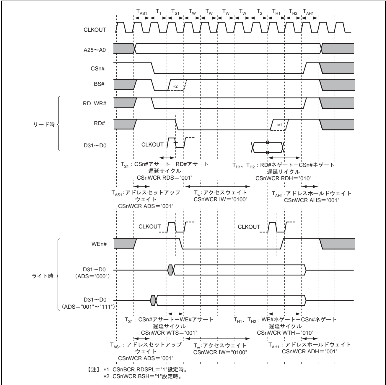
図 19.9 SRAM インタフェースのウェイトステートタイミング (リードストロブネゲートタイミングの設定)
