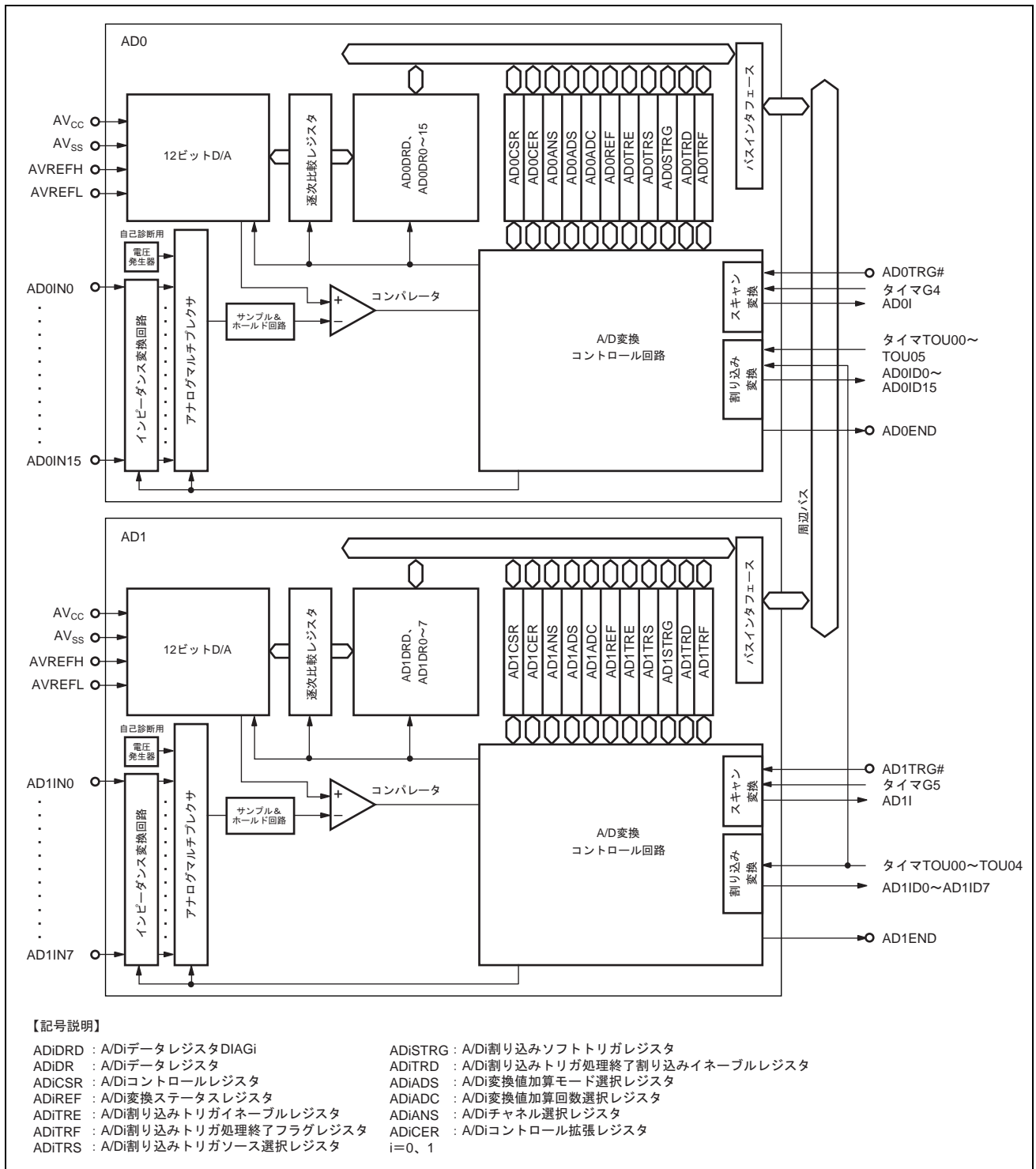
図 27.1 A/D 変換器のブロック図
