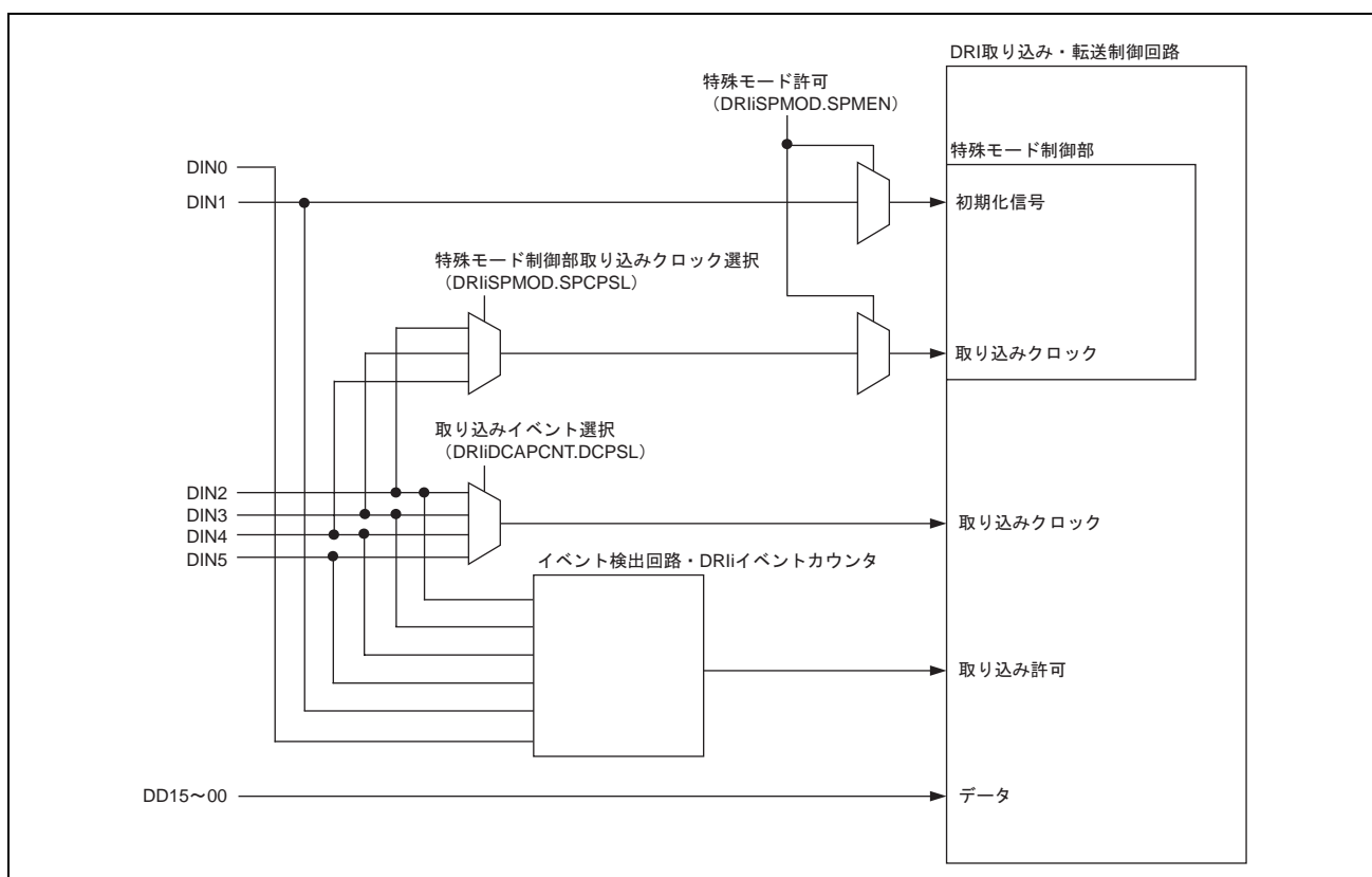
図 28.13 特殊モード ON/OFF 時の接続イメージ
