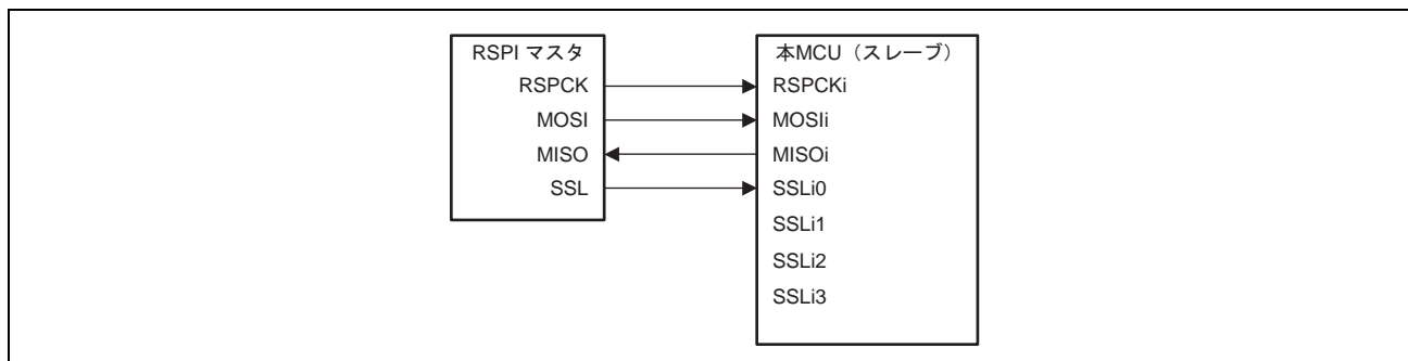
図 24.4 シングルマスタ/シングルスレーブの構成例 (本 MCU=スレーブ)
