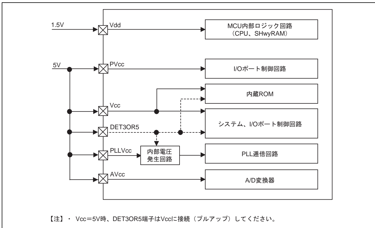
図 34.1 電源回路構成図 (PVcc=Vcc=5V 時)
