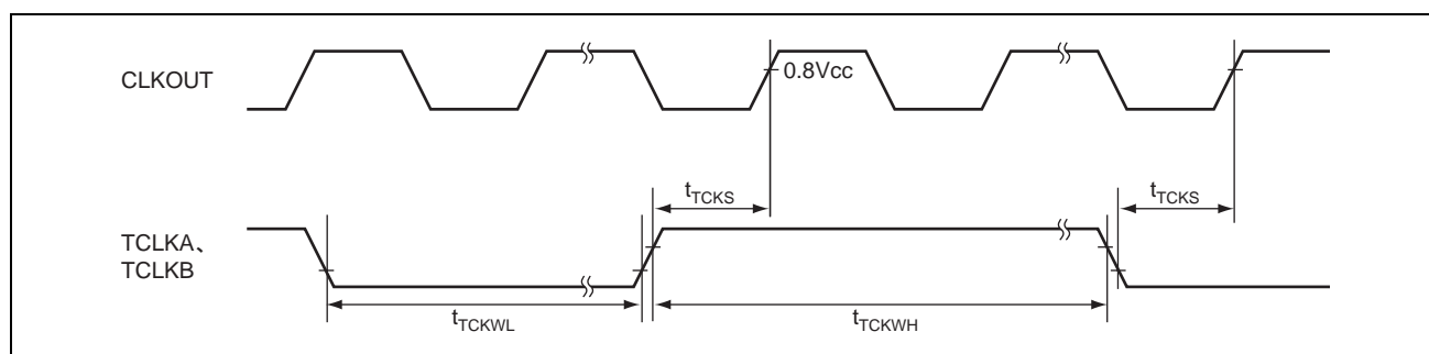
図 38.22 ATU-IIIS クロック入力タイミング
