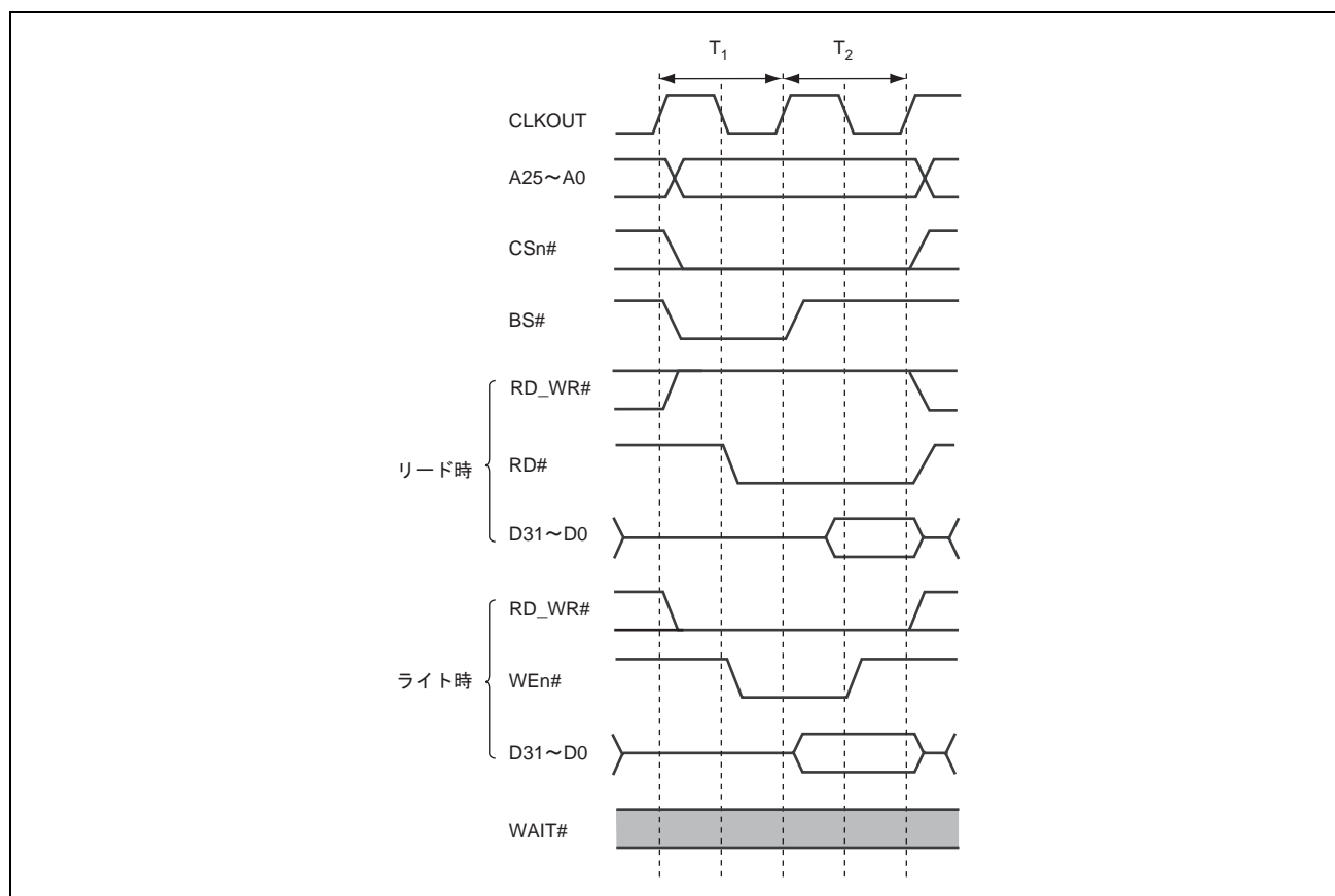
図 19.3 SRAM インタフェース基本タイミング (ウェイトなし)
