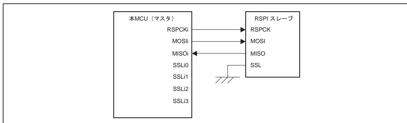
図 24.3 シングルマスタ/シングルスレーブの構成例 (本 MCU=マスタ)
