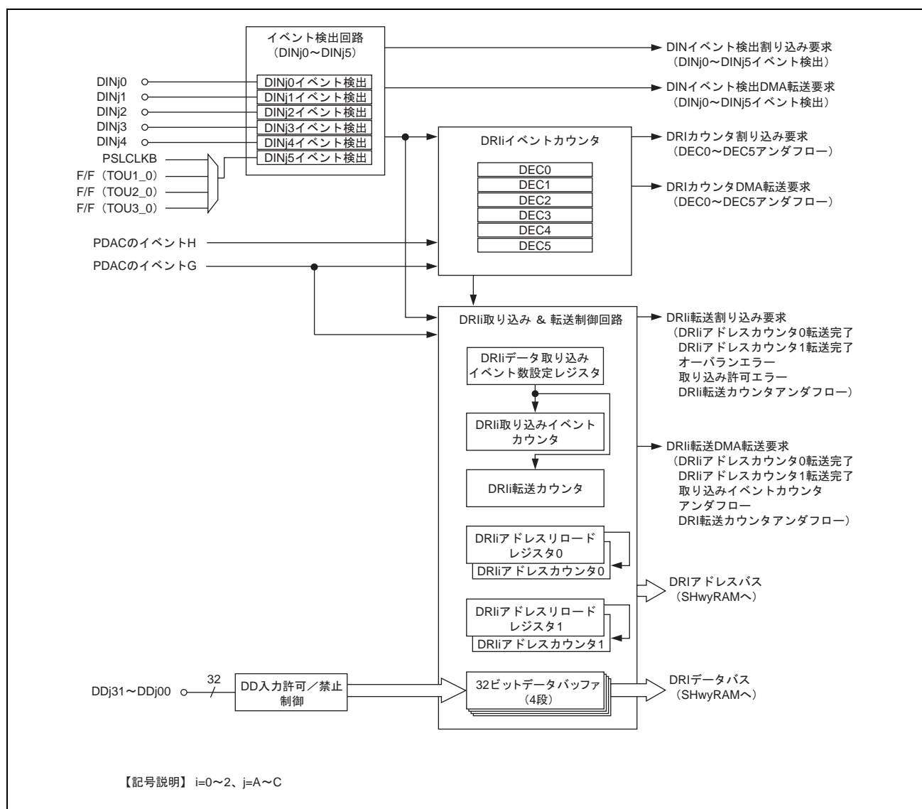
図 28.1 DRli のブロック図
