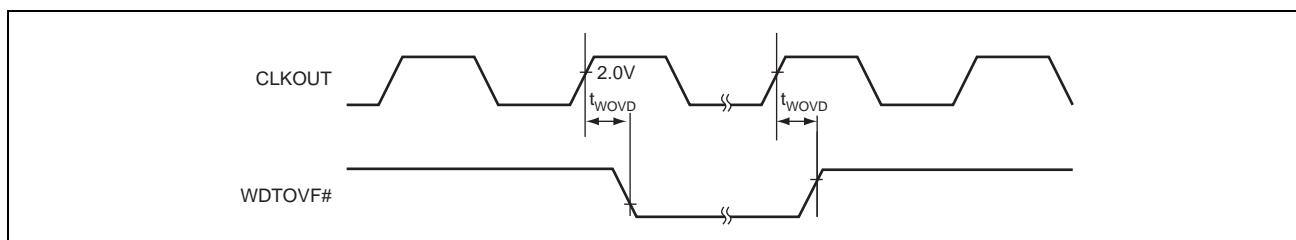
図 38.24 WDT タイミング
