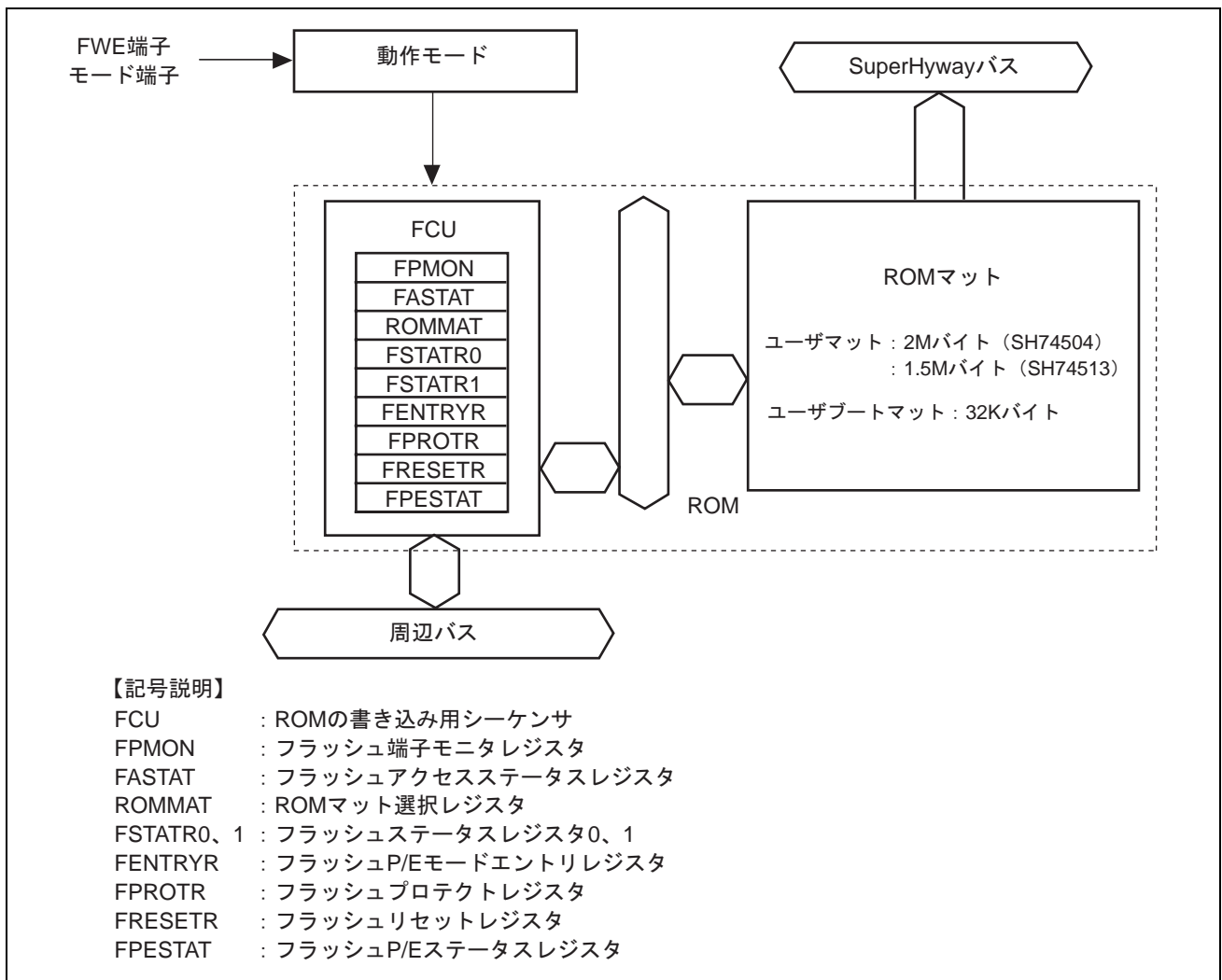
図 12.2 ROM のブロック図
