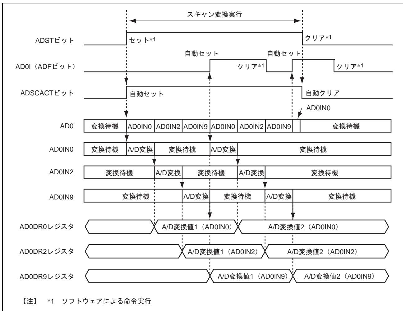
図 27.5 連続スキャンモードの動作例
