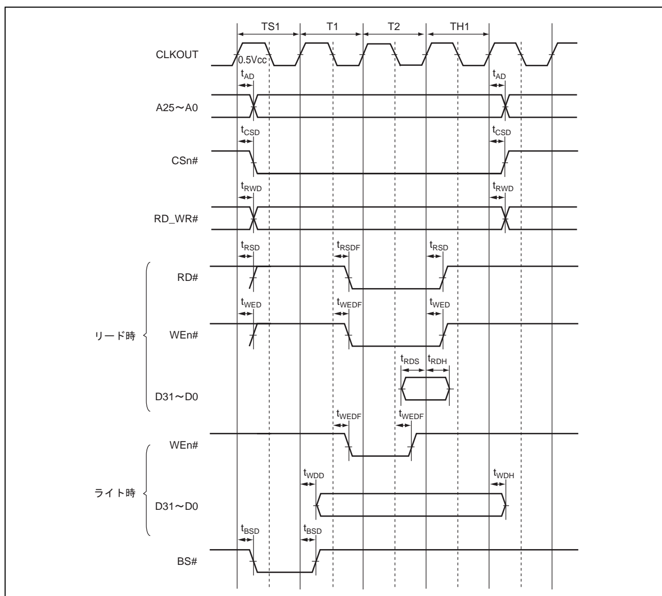
図 38.19 バイト制御 SRAM バスサイクル(ノーウェイト、アドレスセットアップ/ホールド挿入なし、RDS=1、RDH=1、WTS=1、WTH=1)
