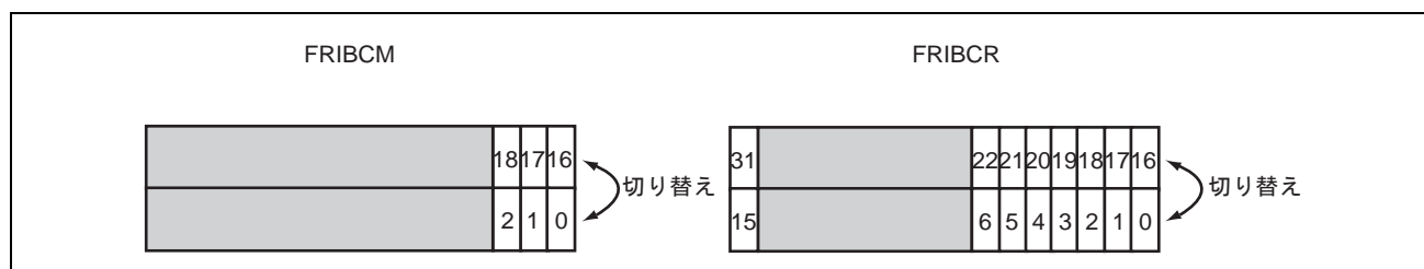
図 32.13 FRIBCM レジスタと FRIBCR レジスタのビットの切り替え
