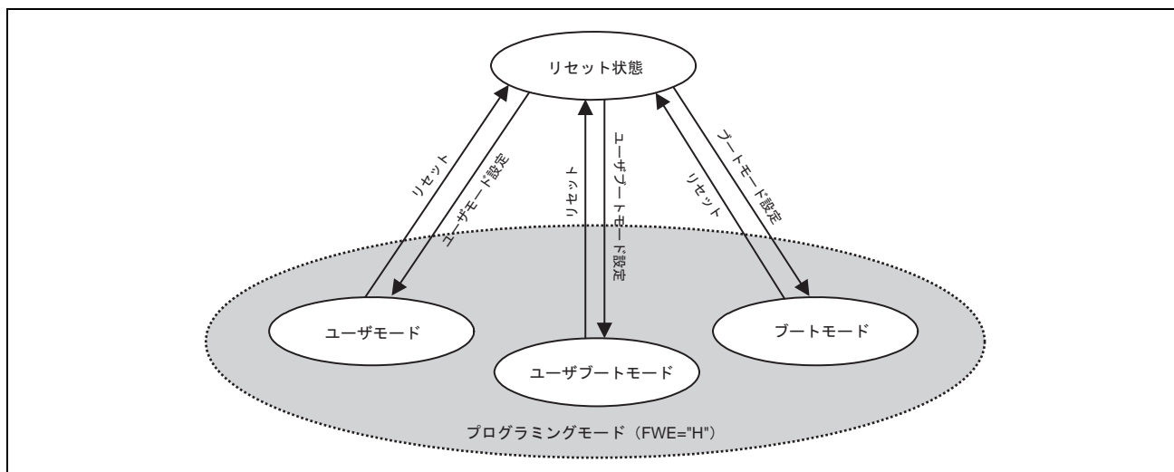
図 12.5 ROM に関するモード遷移図
