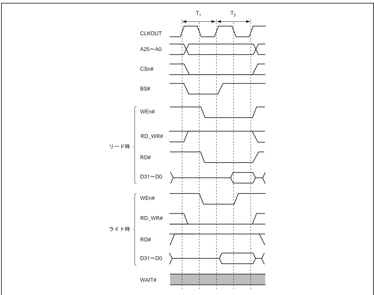
図 19.12 バイト制御 SRAM 基本アクセスタイミング (ウェイトなし)
