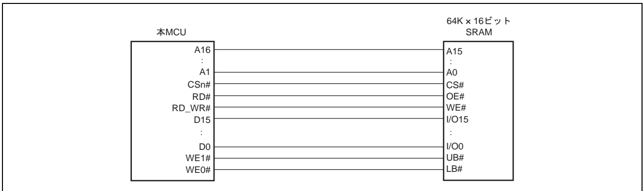
図 19.11 16 ビットデータ幅バイト制御 SRAM 接続例
