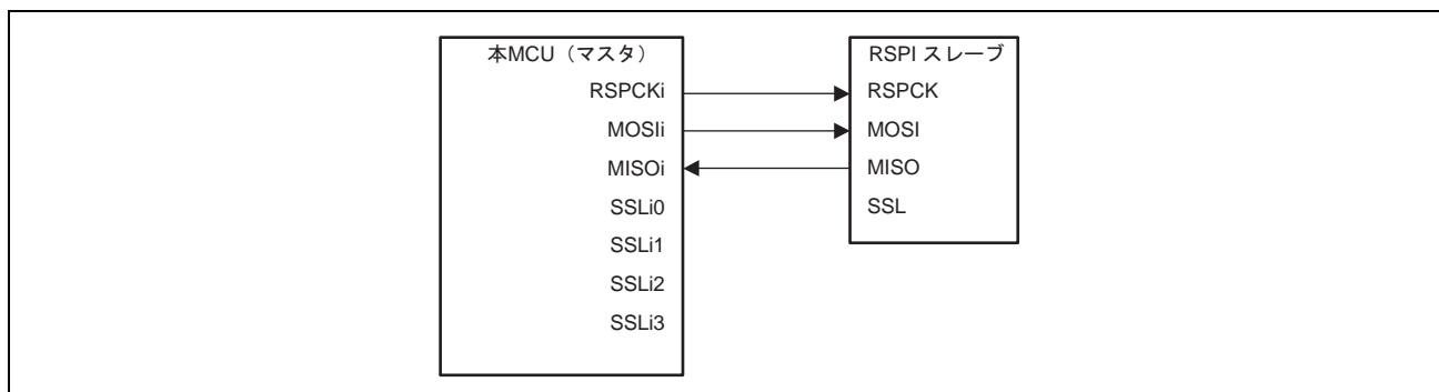
図 24.9 マスタ (クロック同期式動作) /スレーブ (クロック同期式動作) の構成例 (本 MCU = マスタ)
