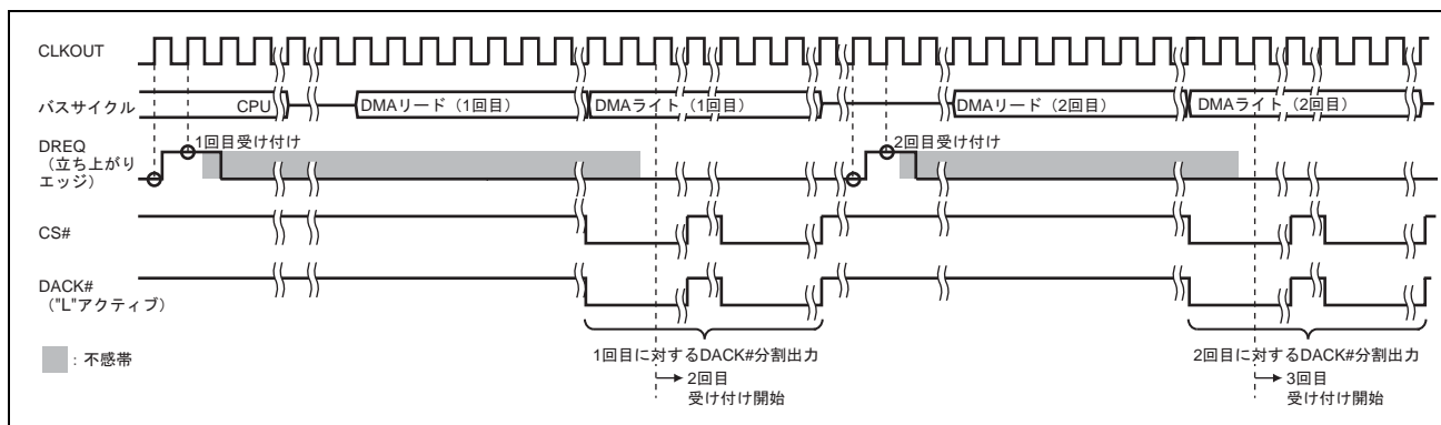
図 20.18 DACK#信号出力分割時のタイミング例 (サイクルスチールモード1または2・DACKライトサイクル出力)
