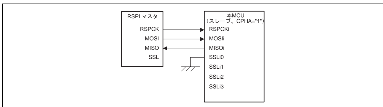
図 24.5 シングルマスタ/シングルスレーブの構成例 (本 MCU=スレーブ、CPHA="1")
