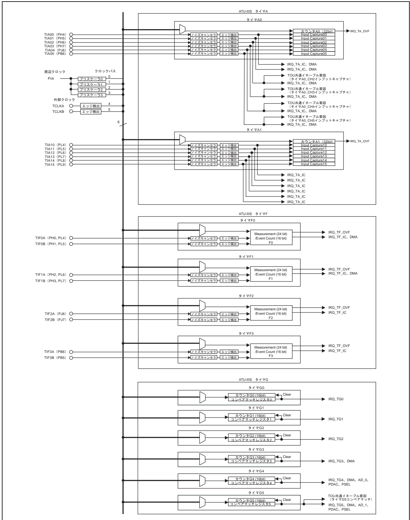
図 21.1 ATU-IIIS のブロック図 (1)
