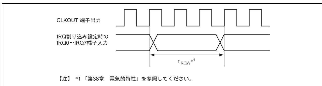
図 15.10 IRQ 端子から入力する割り込み要求の検出に必要な時間
