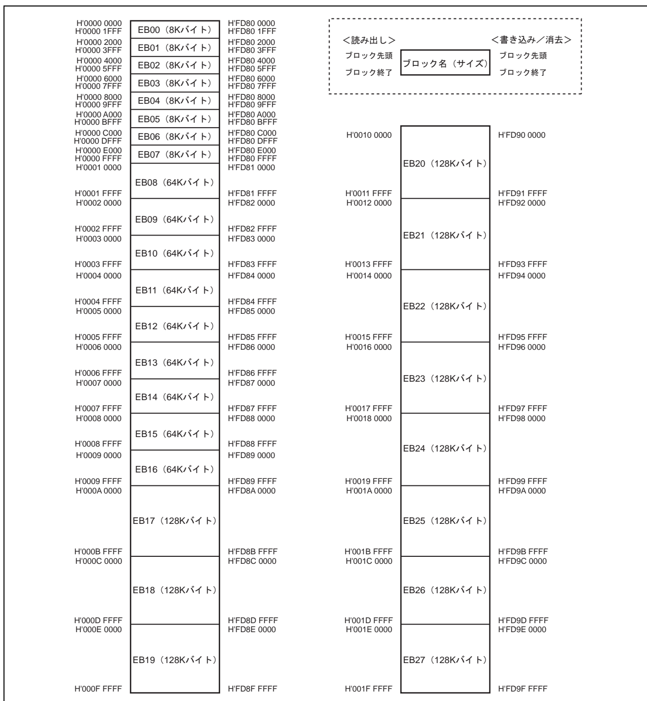
図 12.3 SH74504 のユーザマットのブロック分割
