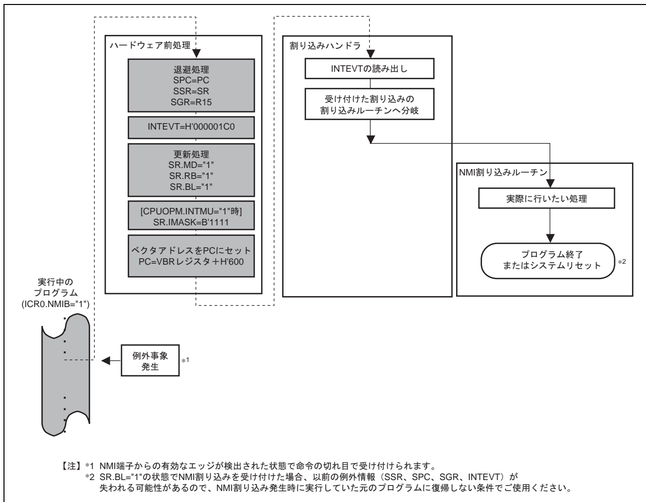
図 15.7 NMI 割り込みの動作例 (ICR0.NMIB="1"の場合)
