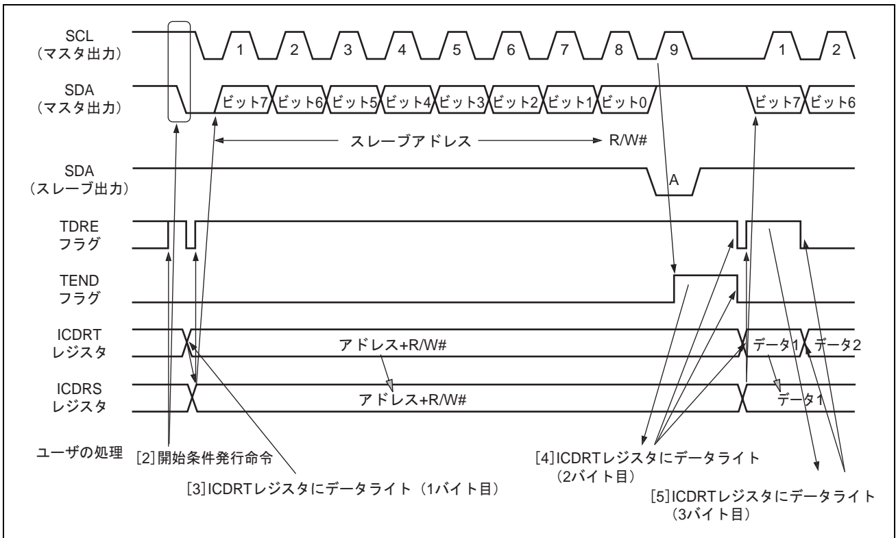
図 25.5 マスタ送信モード動作タイミング (1)
