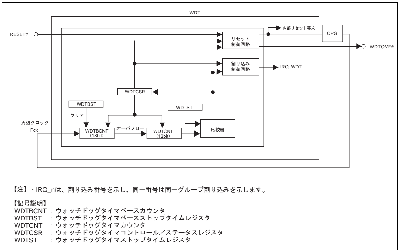
図 17.1 WDT のブロック図
