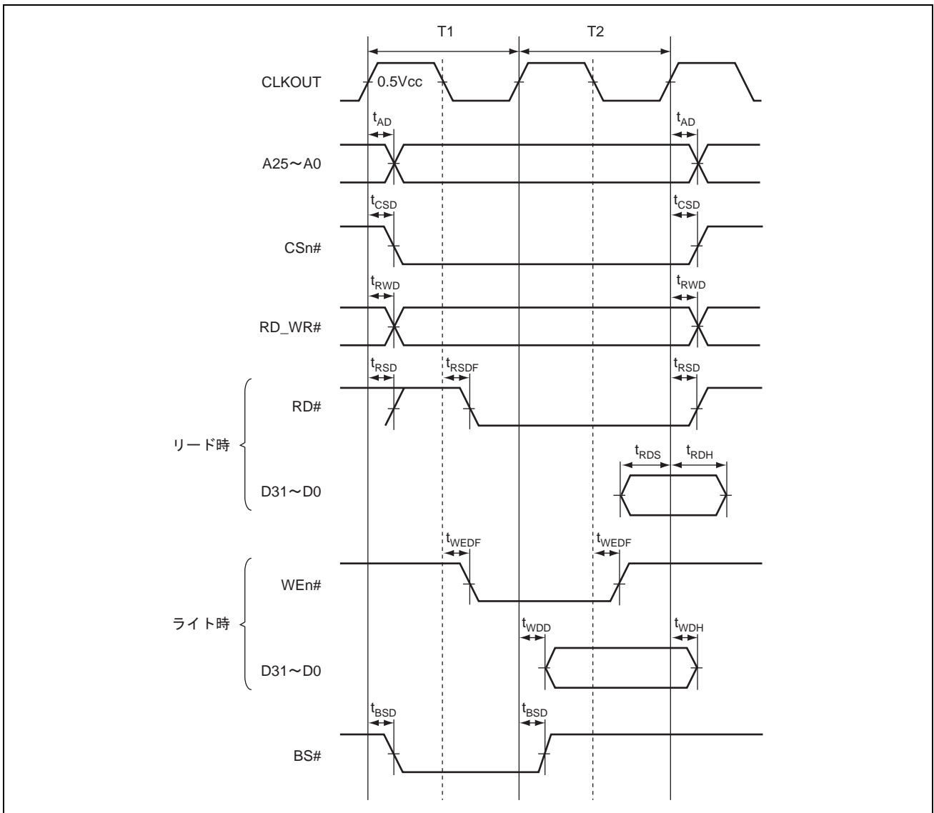
図 38.12 SRAM バスサイクル (ノーウェイト)
