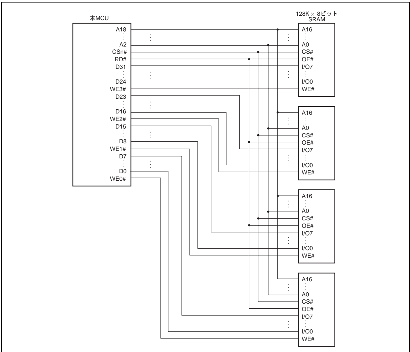
図 19.4 32 ビットデータ幅 SRAM 接続例
