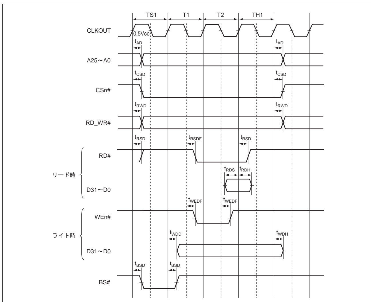
図 38.15 SRAM バスサイクル (ノーウェイト、アドレスセットアップ/ホールド挿入なし、RDS=1、RDH=1、WTS=1、WTH=1)
