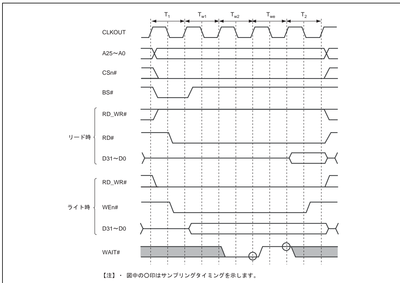
図 19.8 外部空間アクセス ウェイトタイミング (WAIT#信号ウェイト挿入)
