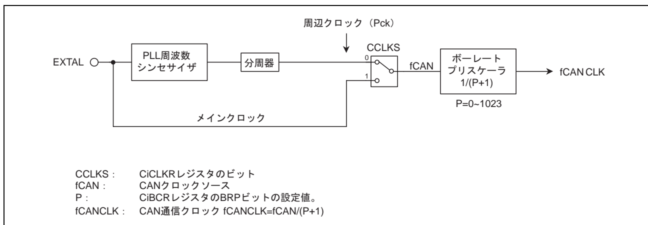
図 26.11 CAN クロック発生回路ブロック図 (i=0~4)
