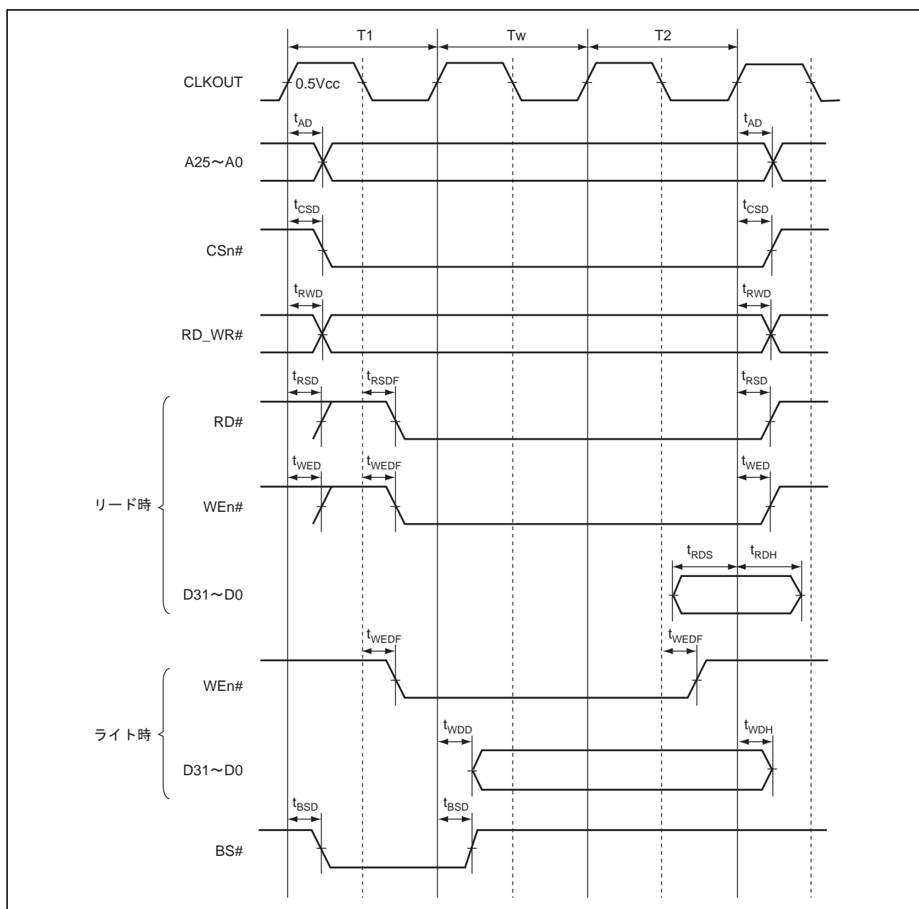
図 38.17 バイト制御 SRAM バスサイクル (ソフトウェアウエイト 1 サイクル)
