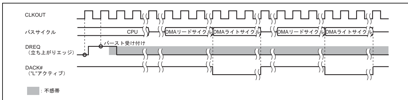
図 20.15 DREQ 入力検出タイミング例 (バーストモード・DACK ライトサイクル出力)
