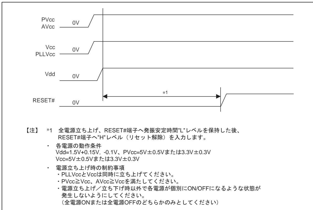
図 34.4 電源立ち上げシーケンス
