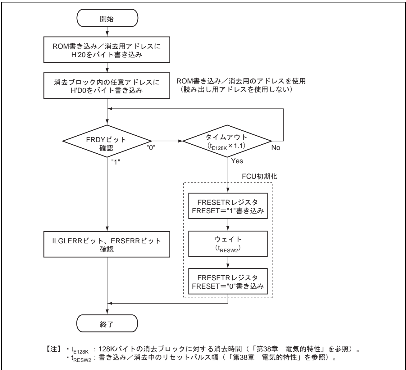
図 12.12 ROM 消去方法
