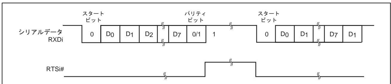
図 23.10 モデムコントロール使用時の動作例 (RTSi#)
