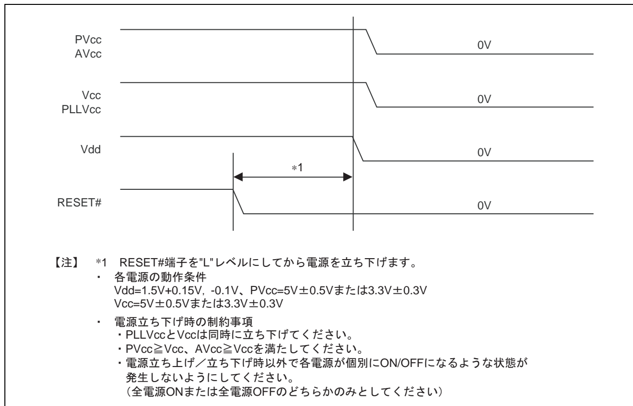
図 34.5 電源立ち下げシーケンス
