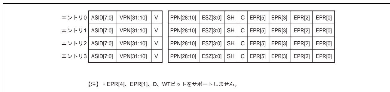
図 7.13 ITLB の構成 (TLB 拡張モード)
