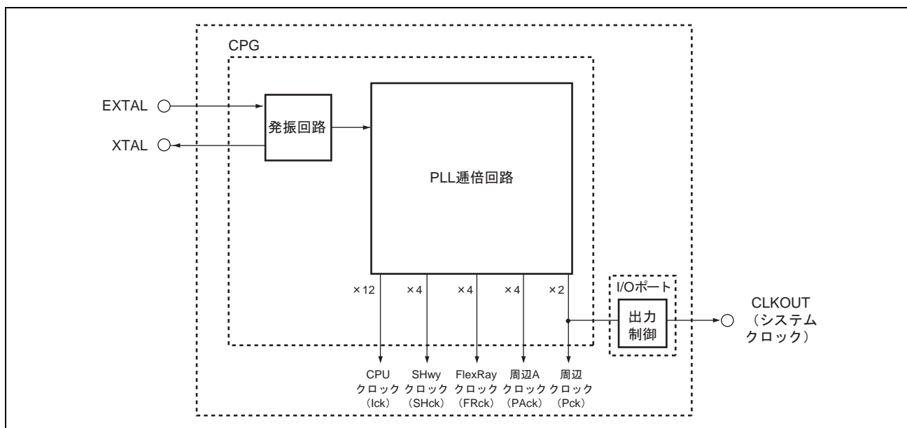
図 14.1 CPG のブロック図
