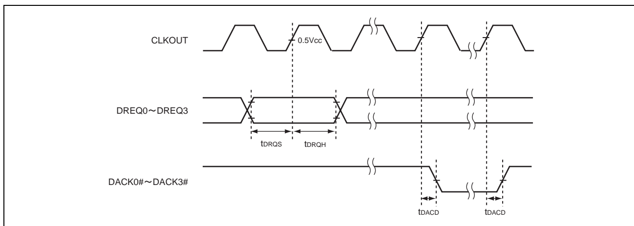
図 38.20 DMAC タイミング
