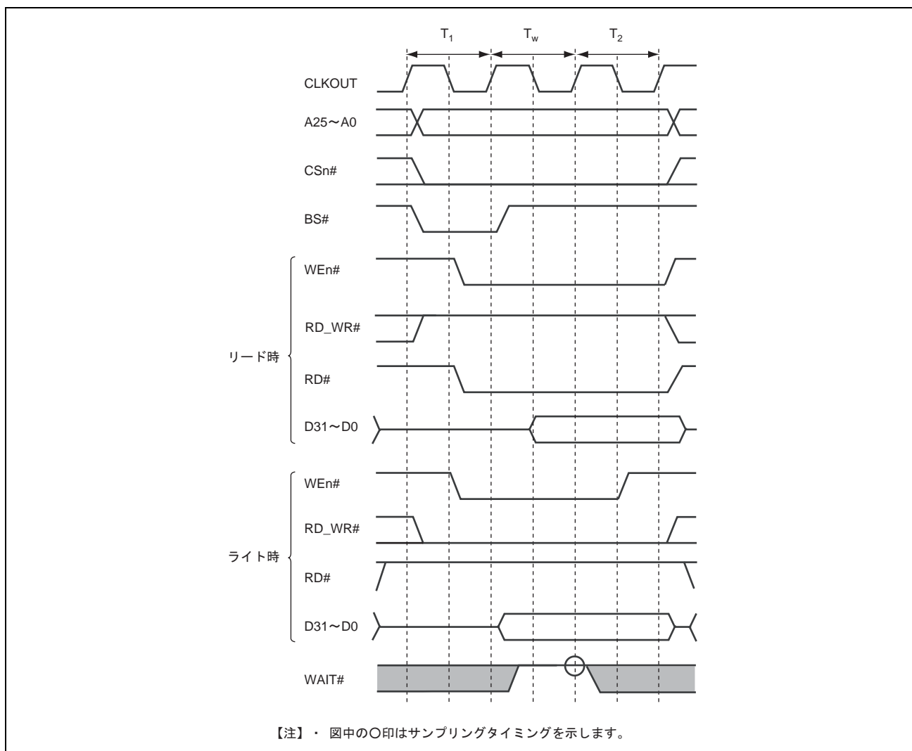
図 19.13 バイト制御 SRAM 基本アクセスタイミング (内部ウェイト1サイクル)
