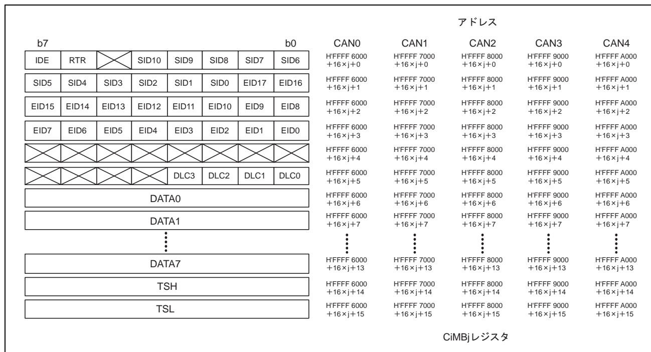
図 26.13 CiMBj レジスタの構成 (i=0~4、j=0~63)
