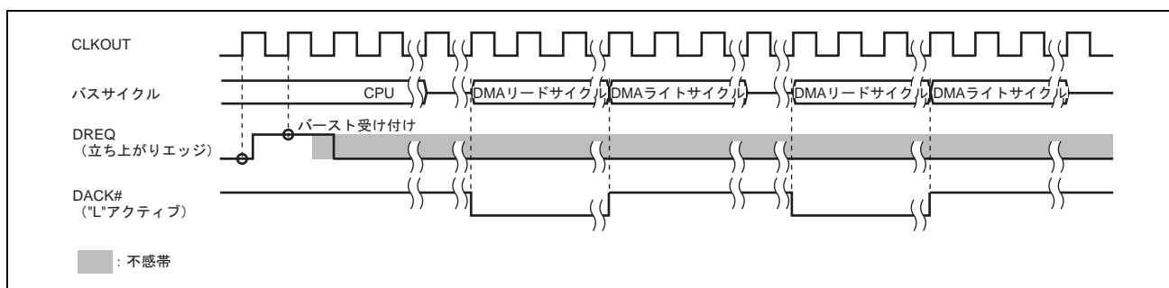
図 20.14 DREQ 入力検出タイミング例 (バーストモード・DACK リードサイクル出力)
