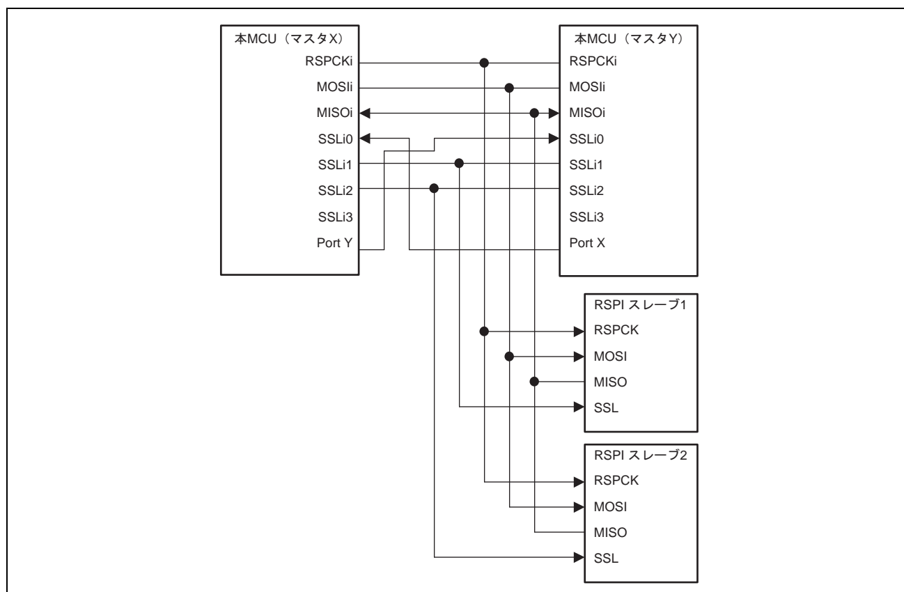
図 24.8 マルチマスタ/マルチスレーブの構成例 (本 MCU=マスタ)
