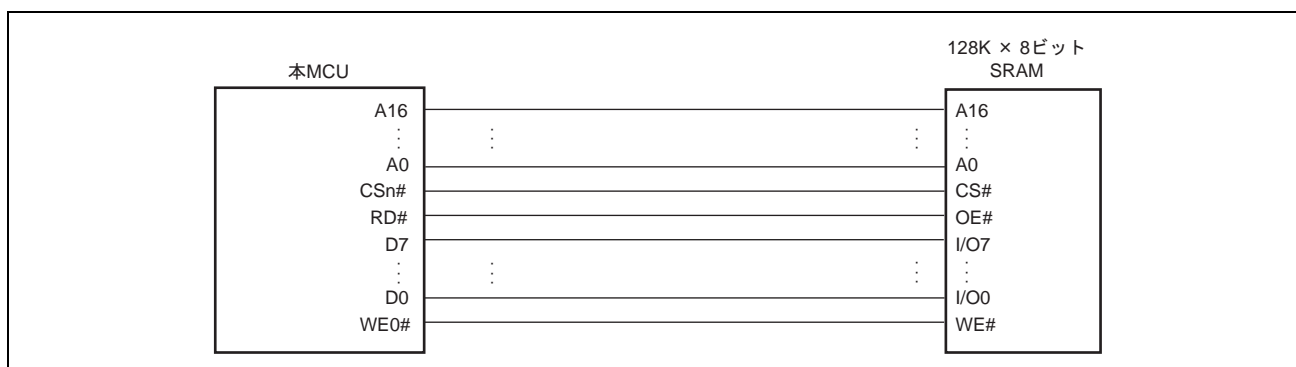
図 19.6 8ビットデータ幅 SRAM 接続例
