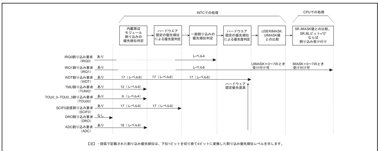
図 15.2 割り込み要求受け付け時の優先順位判定例
