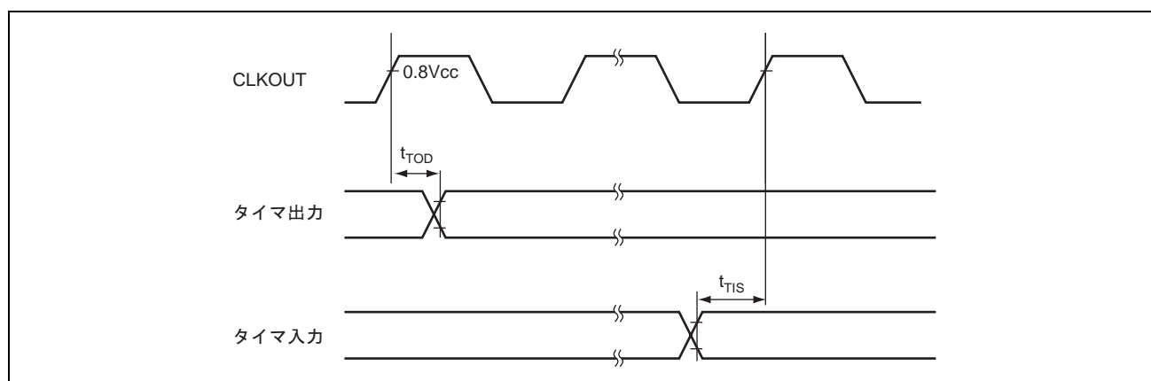
図 38.21 ATU-IIIS 入出力タイミング
