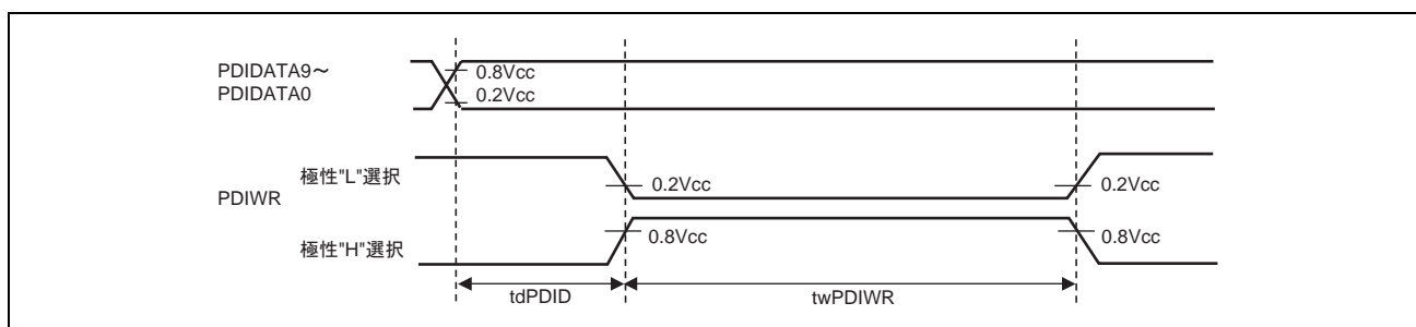
図 38.39 PDAC 出力タイミング
