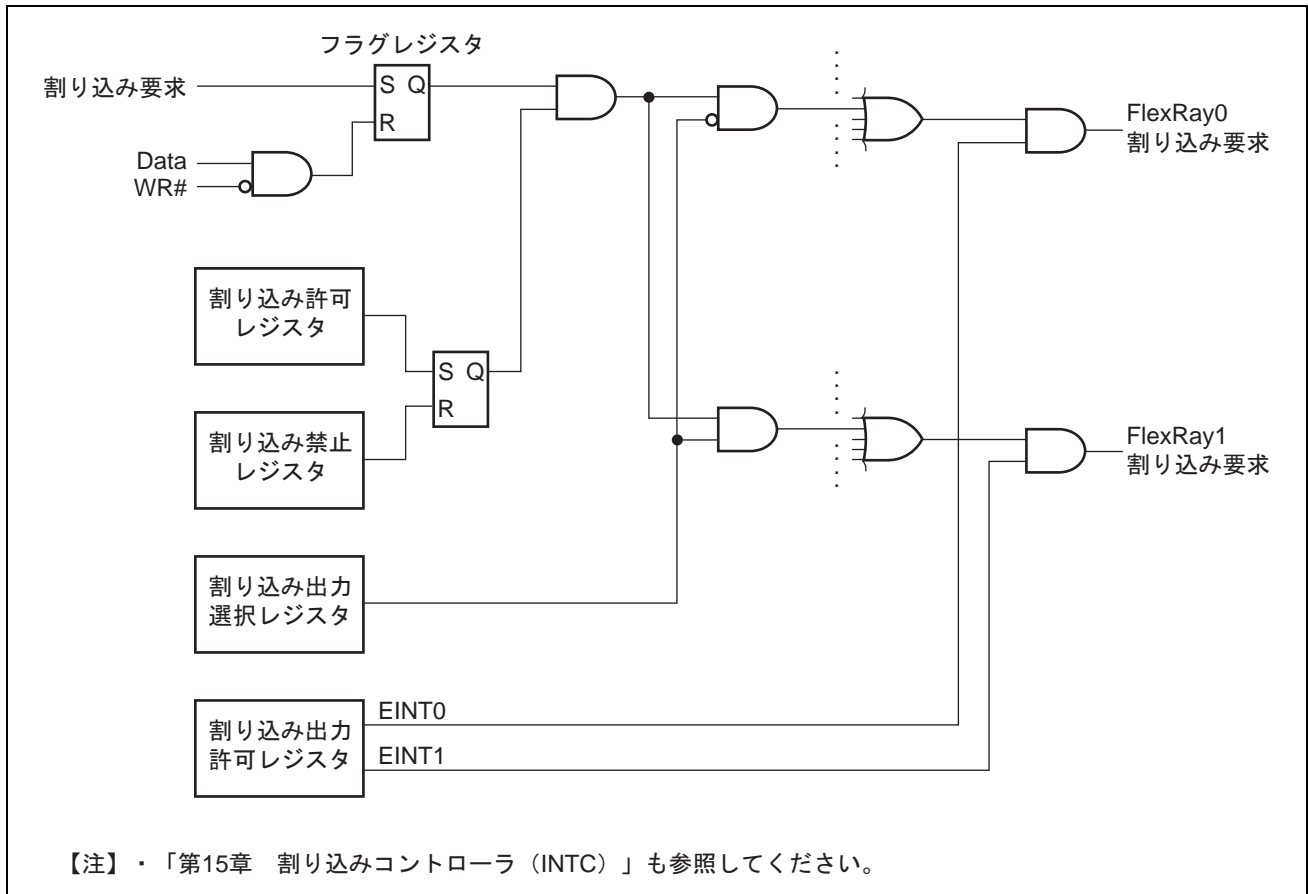
図 32.2 FlexRay0/1 割り込み概略ブロック図
