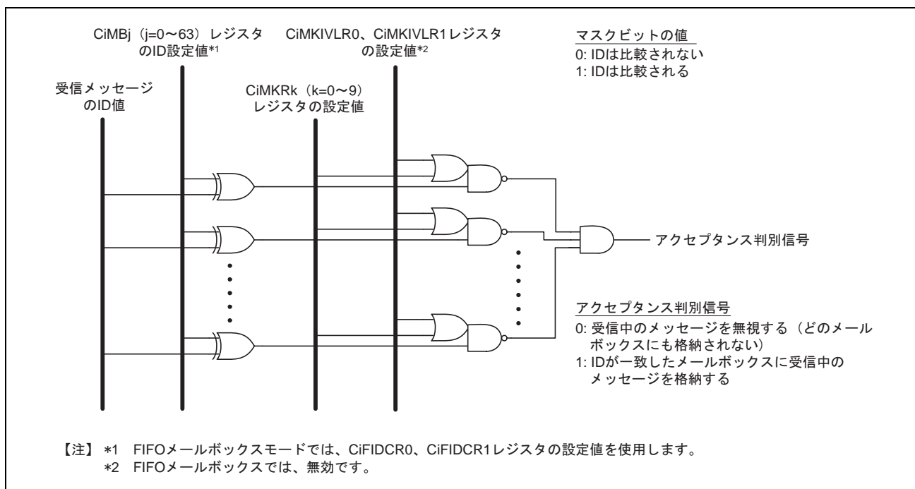
図 26.17 アクセプタンスフィルタ処理 (i=0~4)
