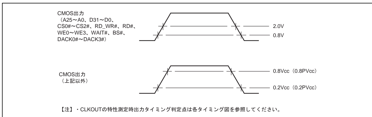
図 38.3 特性測定時出力タイミング判定点
