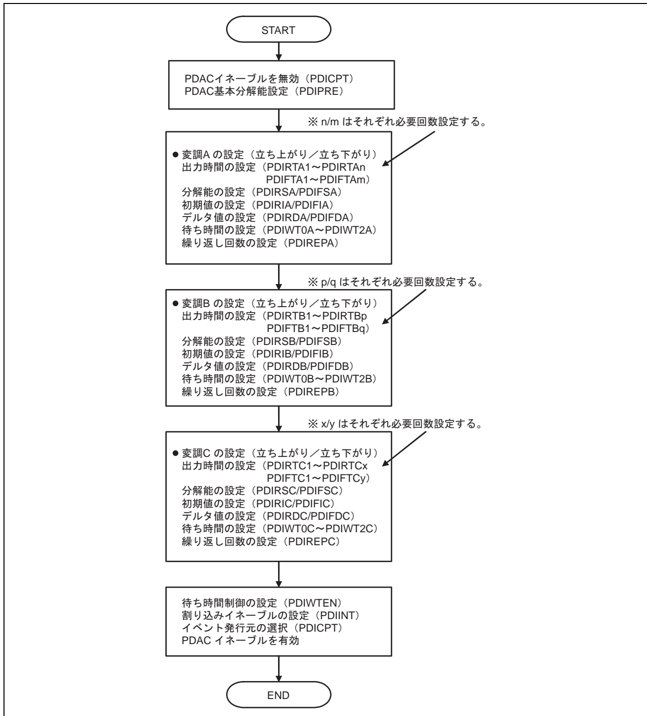
図 30.13 初期設定手順例 (初回起動時)
