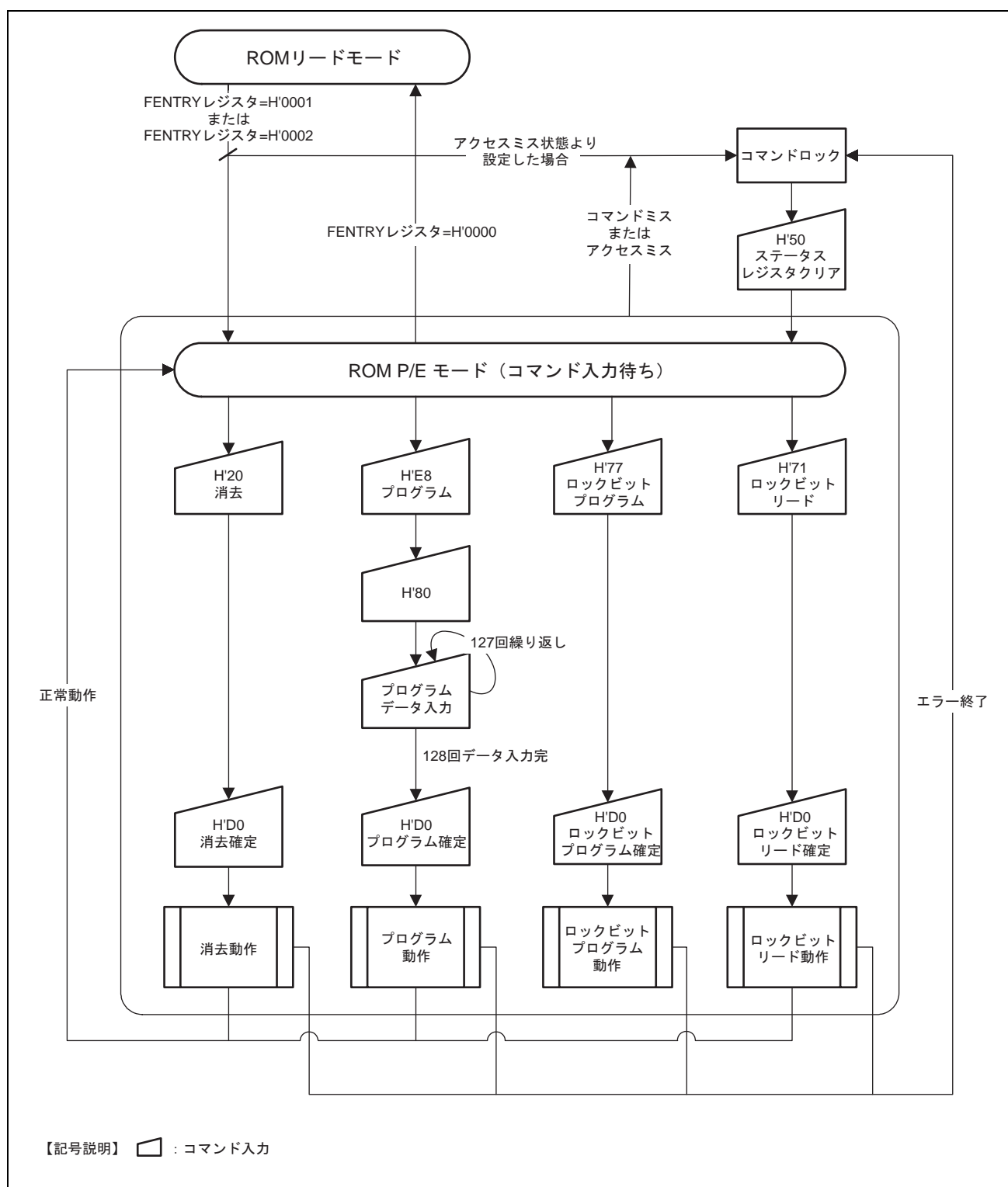
図 12.8 ROM リードモードと P/E モード中のコマンド遷移図
