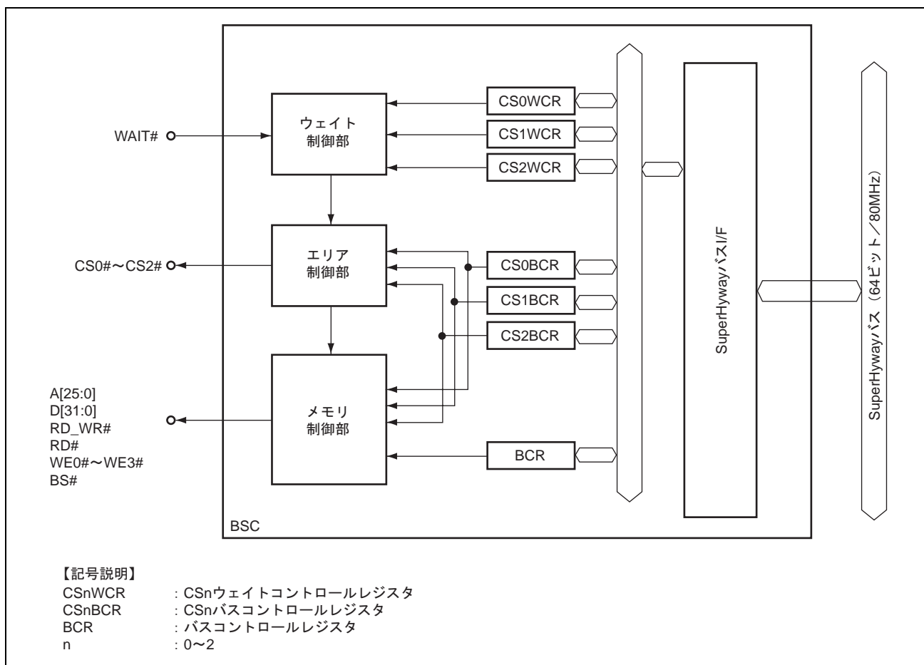
図 19.1 BSC のブロック図
