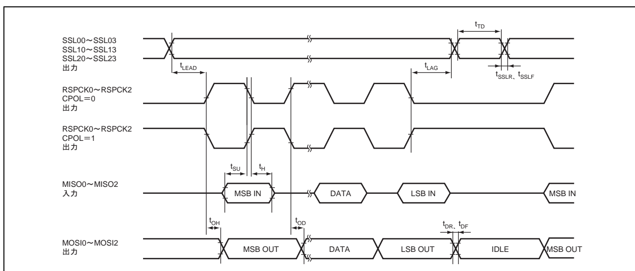
図 38.29 RSPI タイミング (マスター、CPHA="1")
