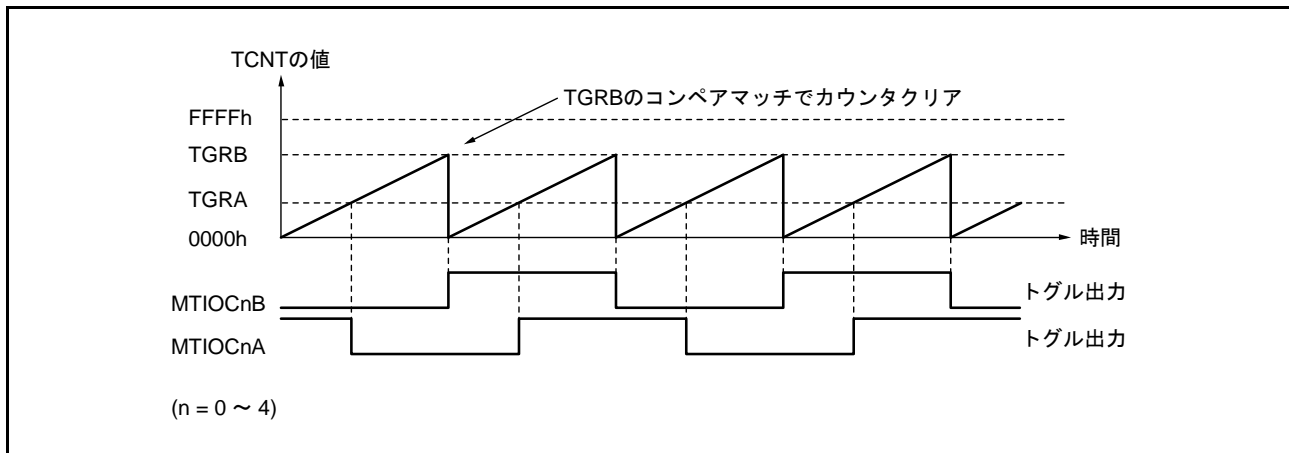
図 23.9 トグル出力の動作例
