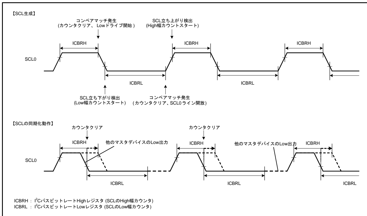
図 35.21 RIIC の SCL 生成および SCL 同期化動作
