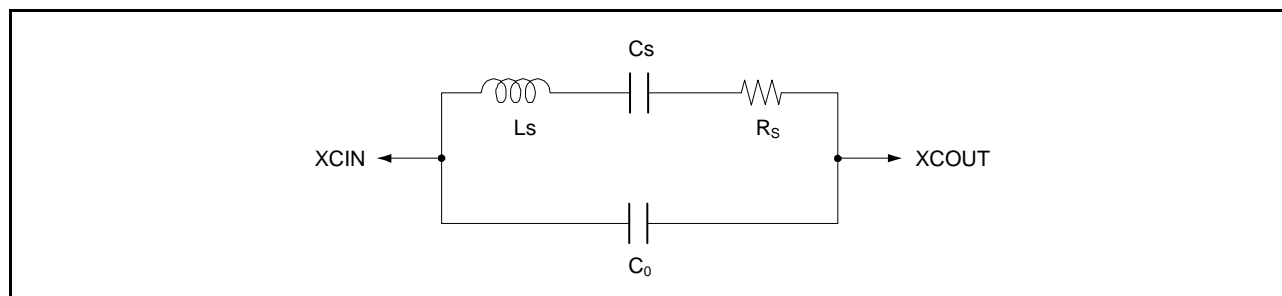
図 9.9 水晶振動子の等価回路
