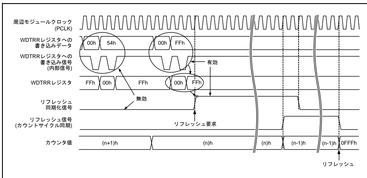
図 30.6 WDT リフレッシュ動作波形 (WDTCR.CKS[3:0] = 0100b、WDTCR.TOPS[1:0] = 01b)
