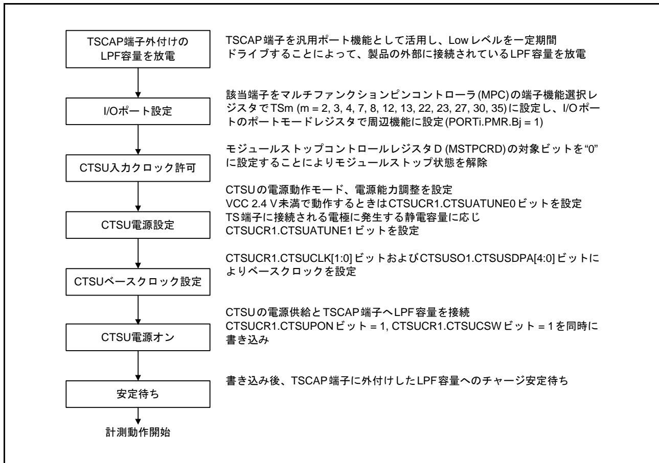
図 43.9 CTSUS 初期設定フロー
