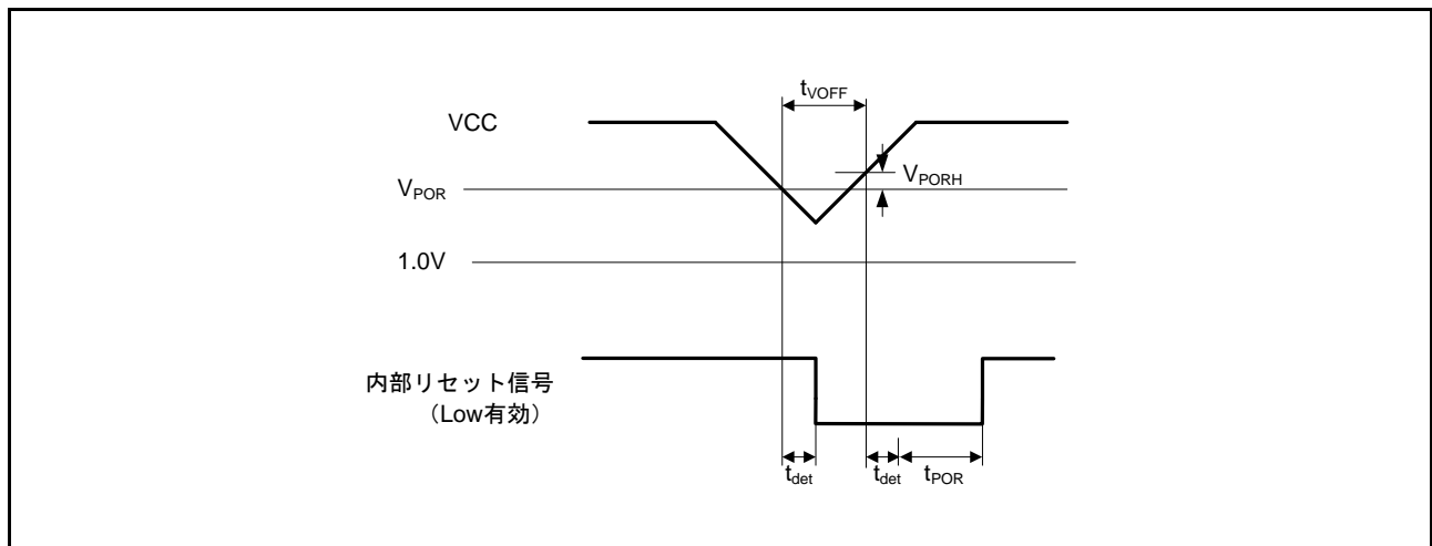
図 51.69 電圧検出リセットタイミング
