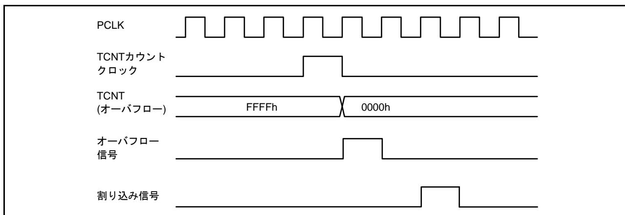
図 23.94 TCIV 割り込みタイミング
