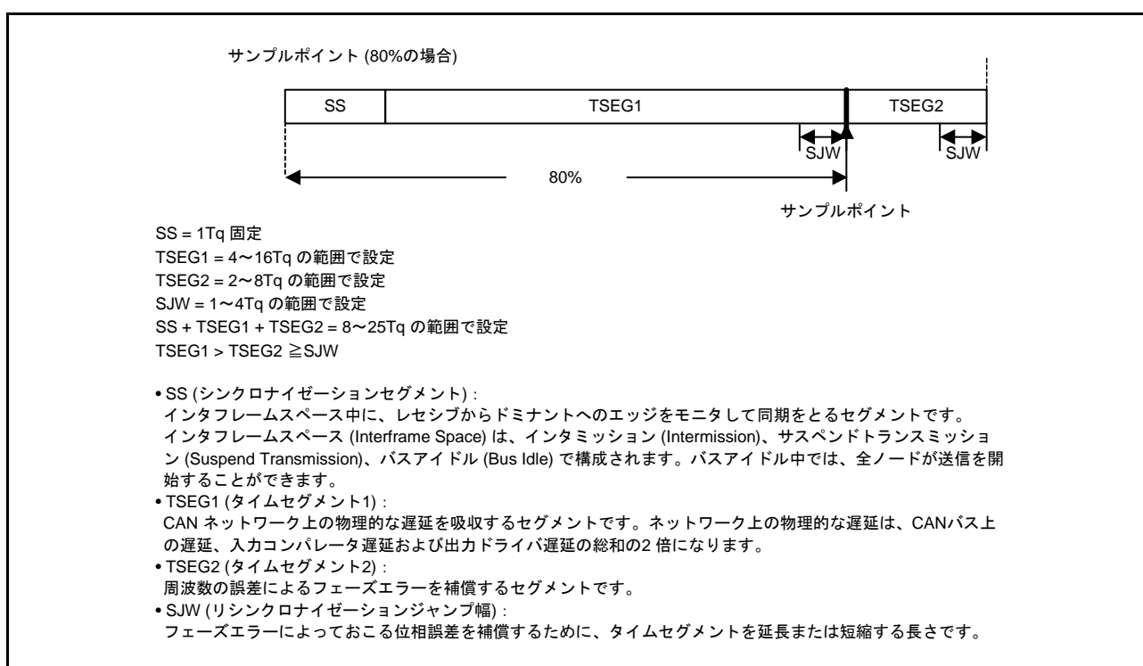
図 36.17 ビットタイミング図
