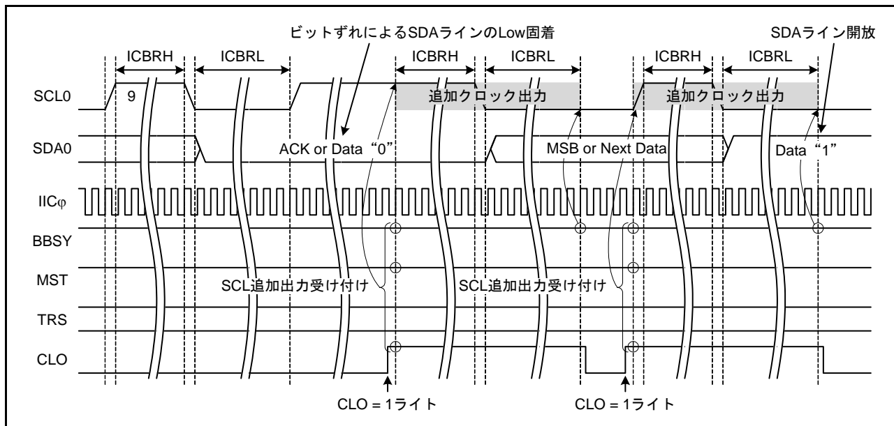
図 35.40 SCL 追加出力機能 (CLO ビット)
