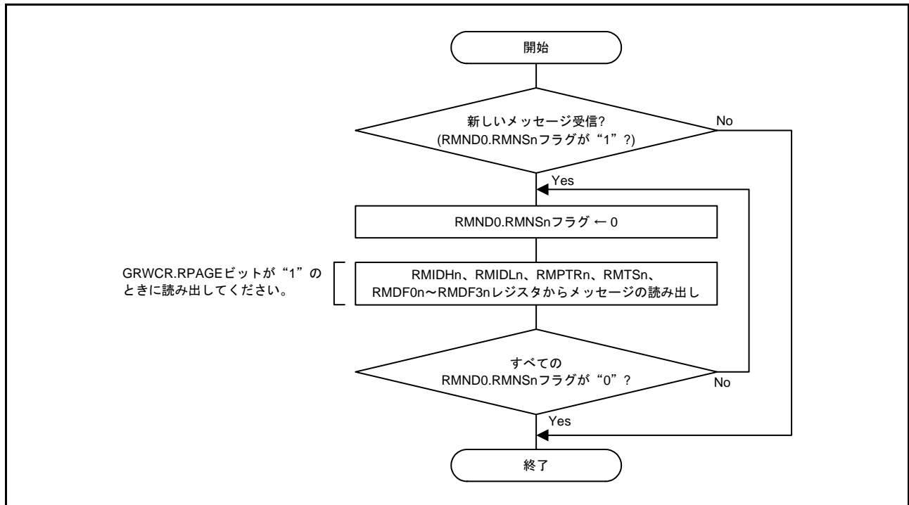
図 36.22 受信バッファの読み出し手順
