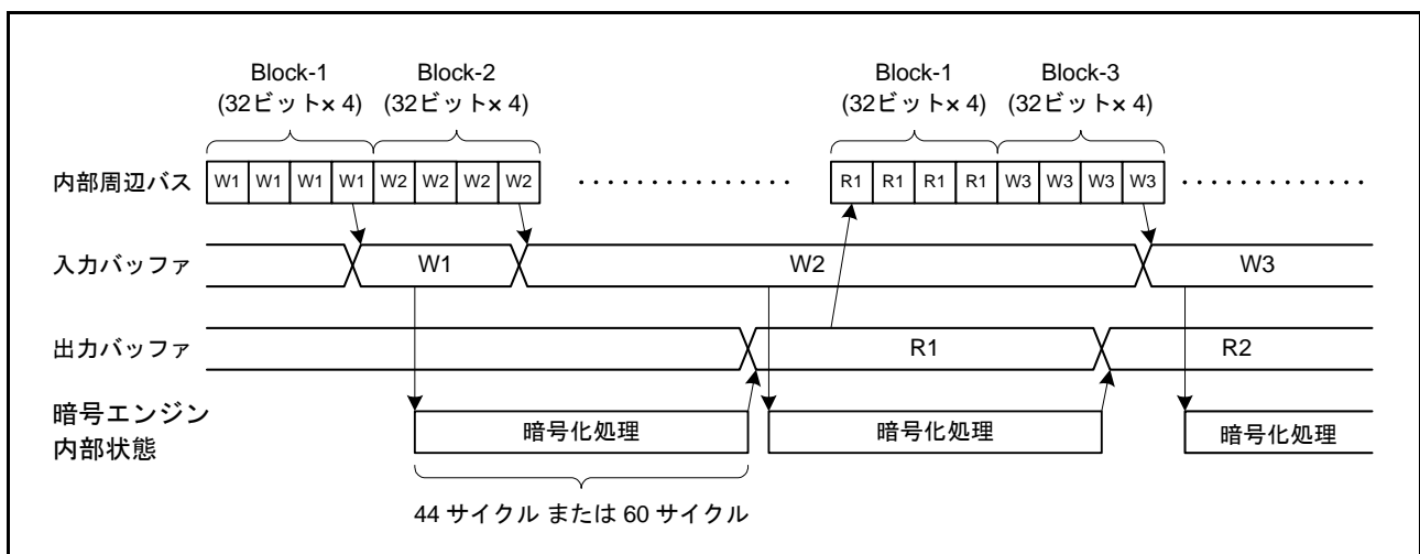
図 42.6 暗号 / 復号処理タイミング図
