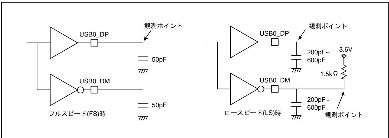
図 51.62 測定回路
