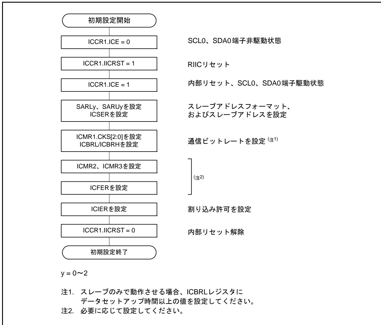
図 35.5 RIIC の初期化フローチャート例
