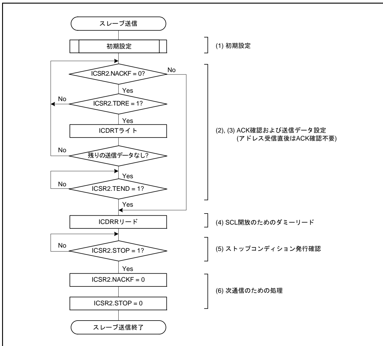
図 35.15 スレーブ送信のフローチャート例
