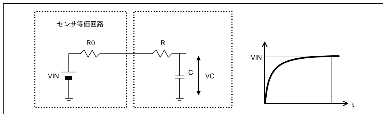
図 44.28 アナログ入力端子と外部センサの等価回路
