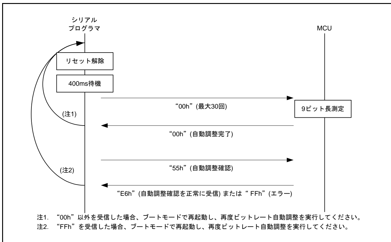
図 50.32 ビットレート自動調整の手順
