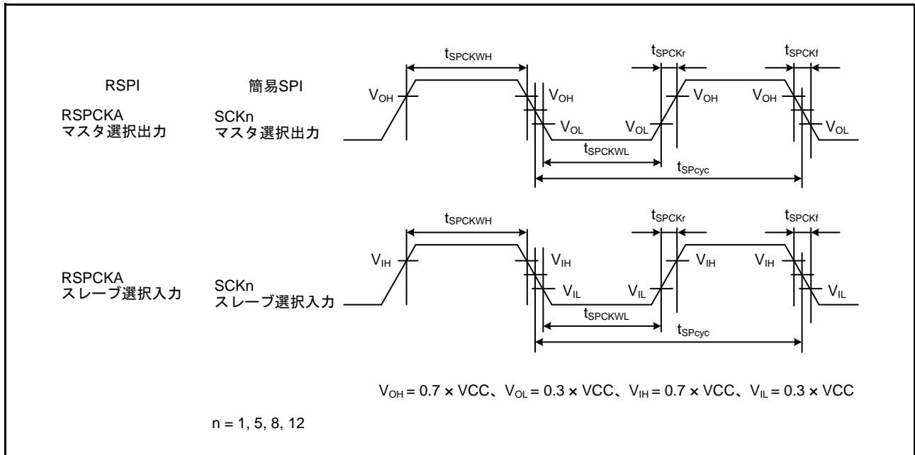
図 51.48 RSPI クロックタイミング / 簡易 SPI クロックタイミング
