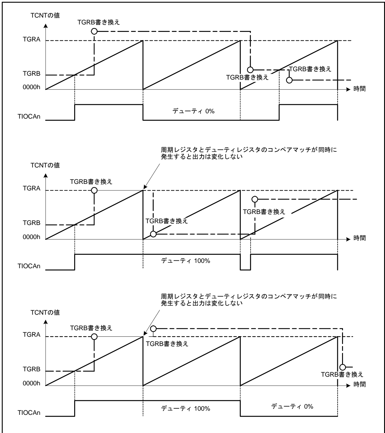
図 25.23 PWMモード動作例(3) (n = 3, 4)
