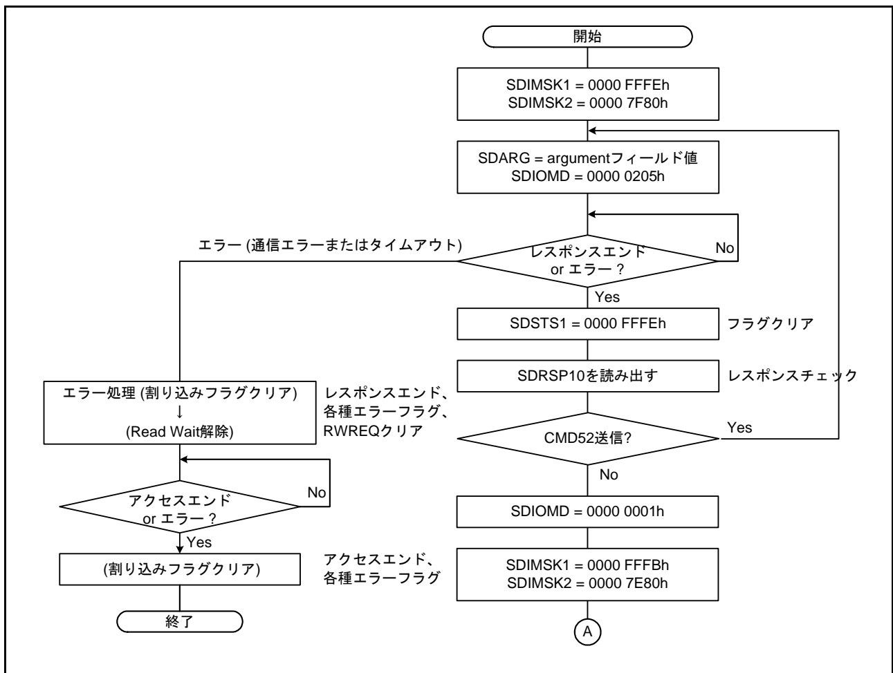
図 40.17 IO_RW_EXTENDED コマンド (CMD53/ マルチブロックリード) のシーケンス中に Read Wait 状態にした後、SDIO none abort コマンド (CMD52) を送信する例
