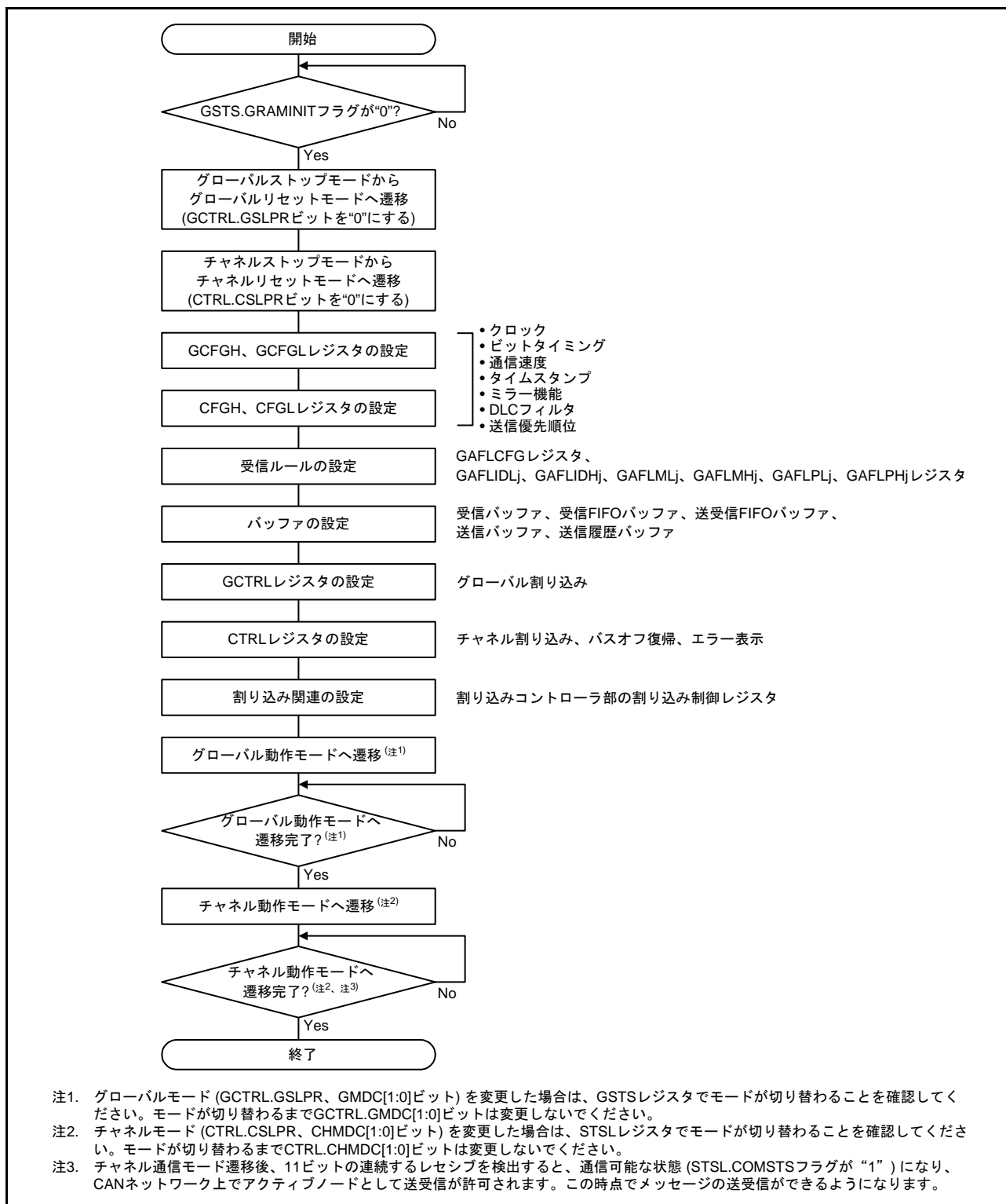
図 36.16 CAN モジュールイネーブル後の設定手順
