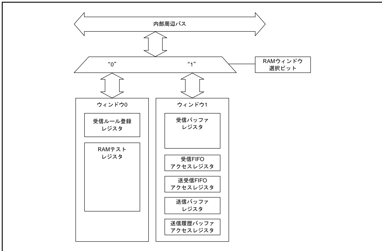
図 36.15 RAM ウィンドウ
