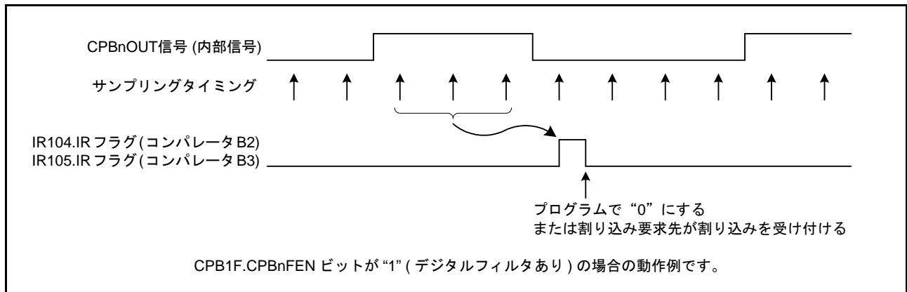
図 47.6 コンパレータ Bn デジタルフィルタの動作例 (n = 2, 3)
