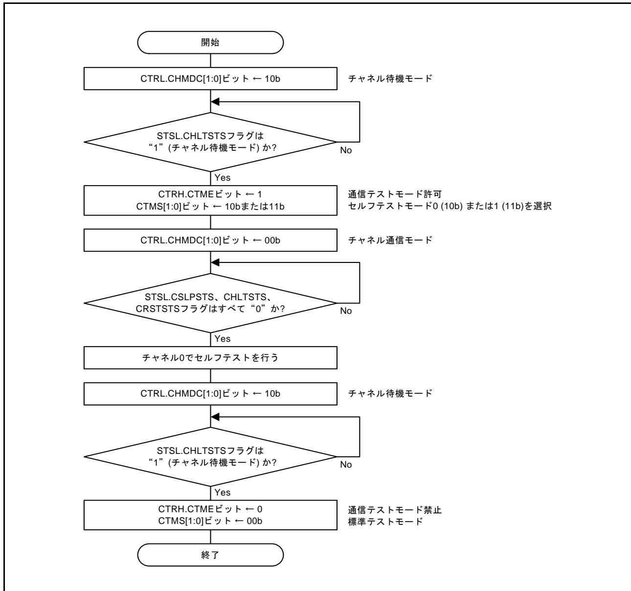
図 36.33 セルフテストモードの設定手順
