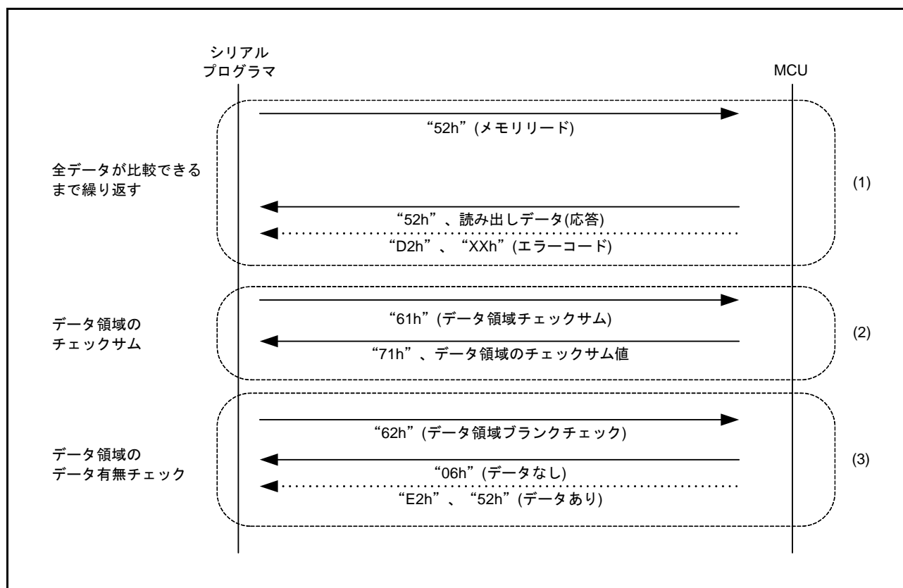
図 50.40 データ領域のデータ確認手順
