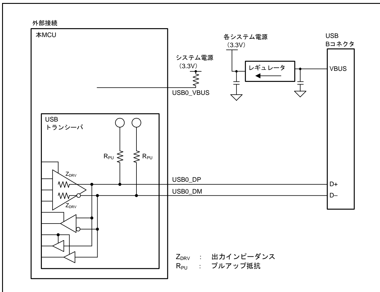
図 32.6 バスパワー時の USB コネクタのファンクション接続例
