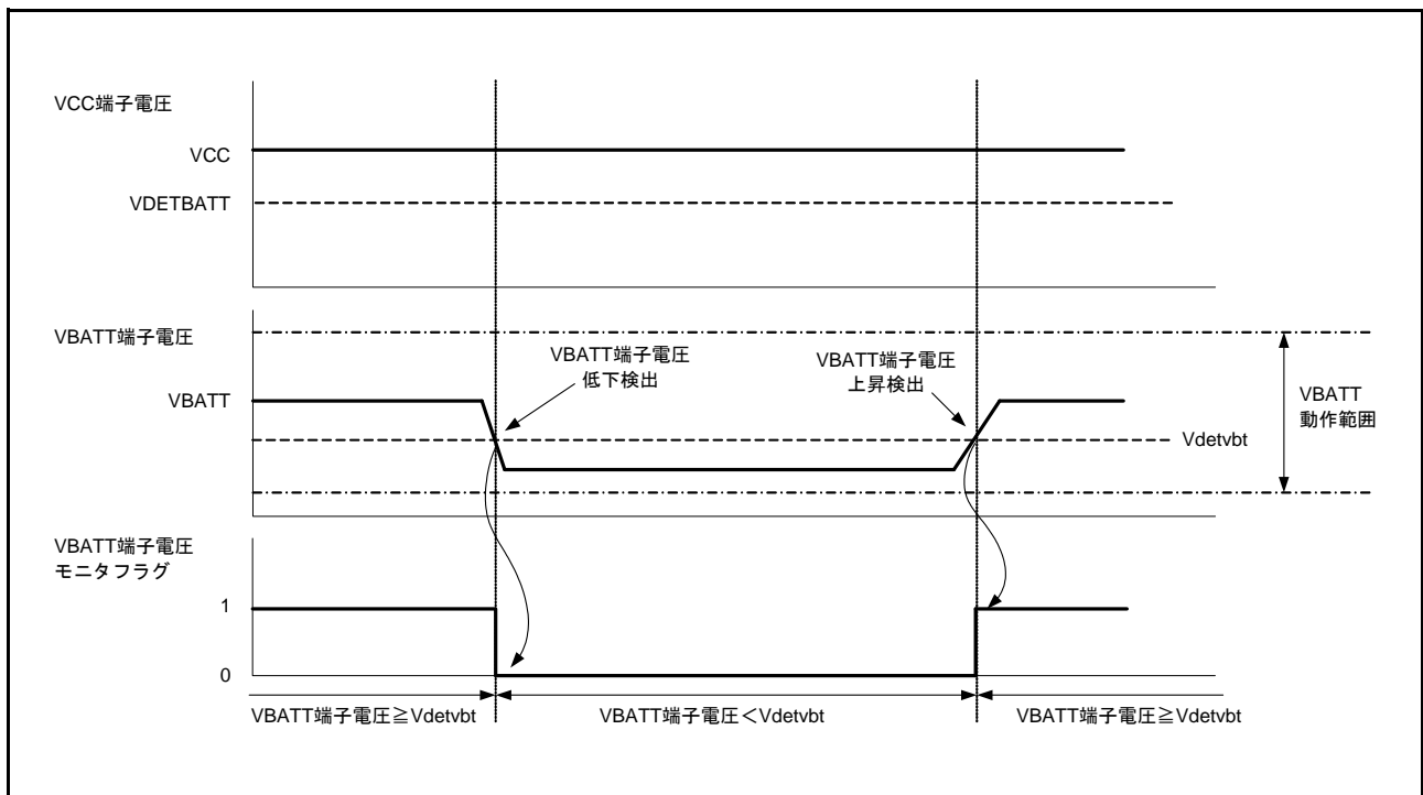
図 12.3 VBATT 端子電源電圧モニタフラグの動作例
