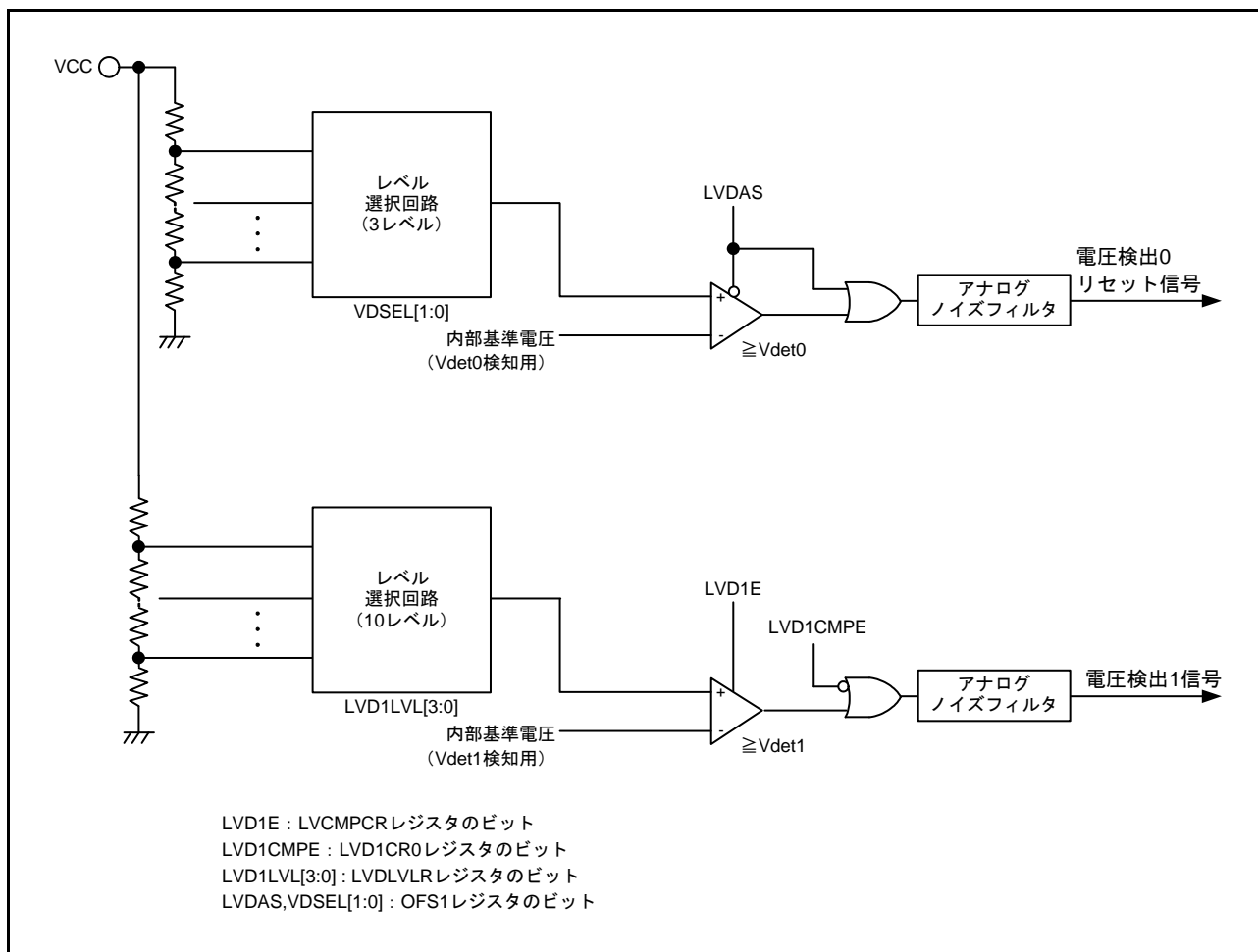
図 8.1 電圧検出回路ブロック図
