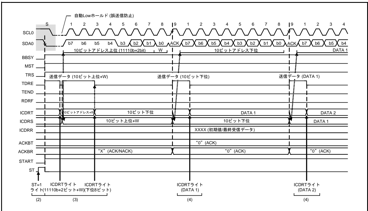
図 35.8 マスタ送信の動作タイミング (2) (10ビットアドレスフォーマットの時)
