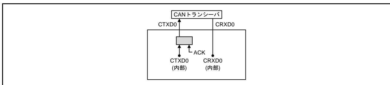
図 36.11 セルフテストモード0選択時の接続
