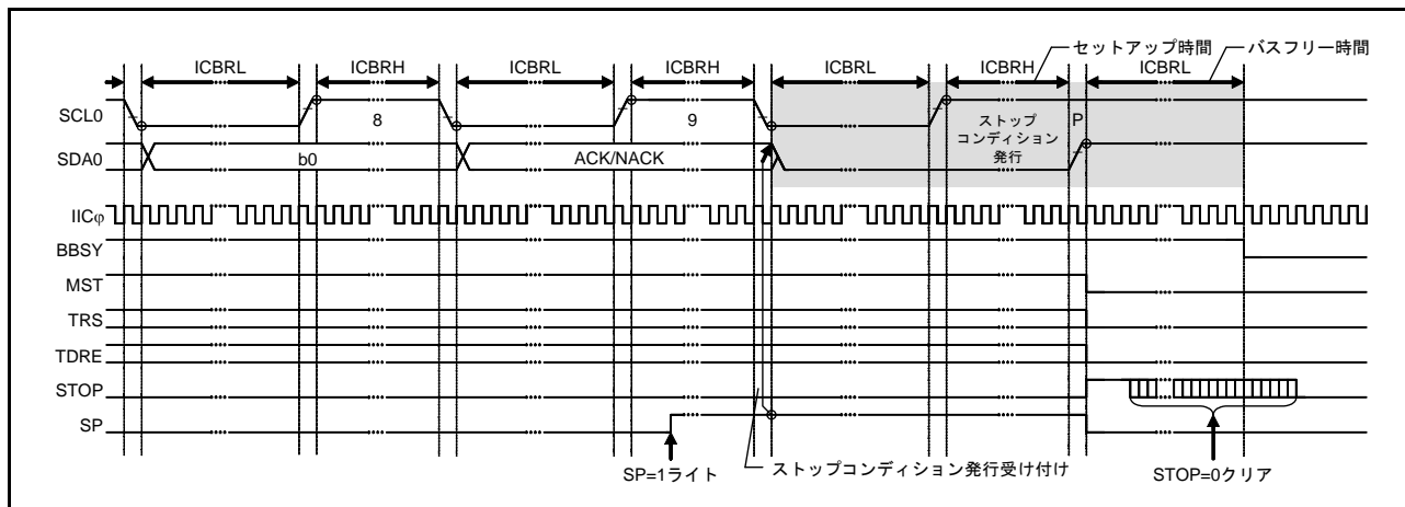
図 35.38 ストップコンディション発行動作タイミング (SP ビット)
