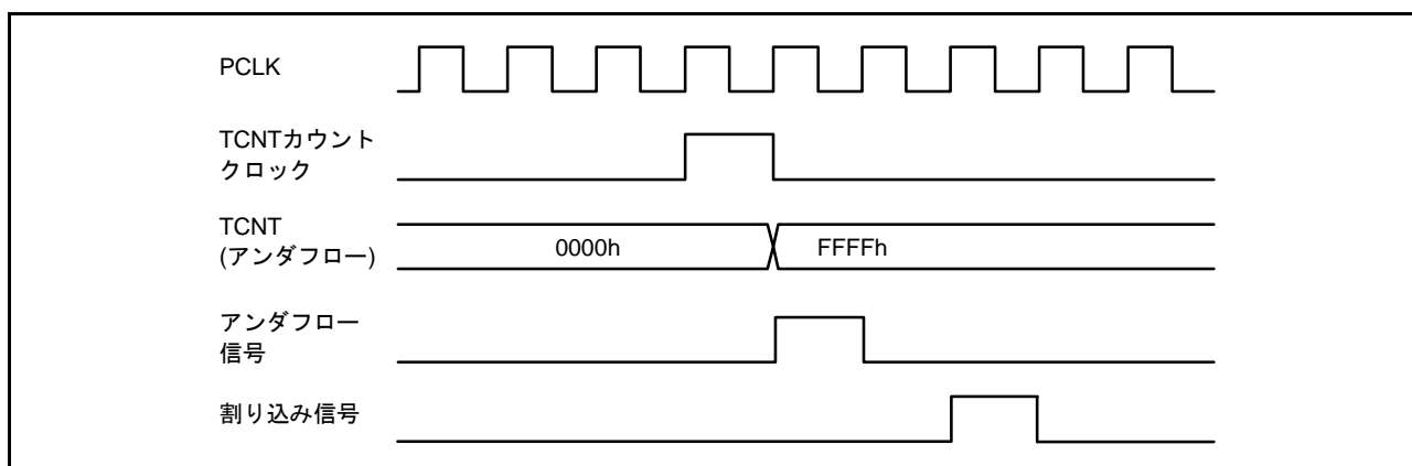
図 23.95 TCIU 割り込みタイミング
