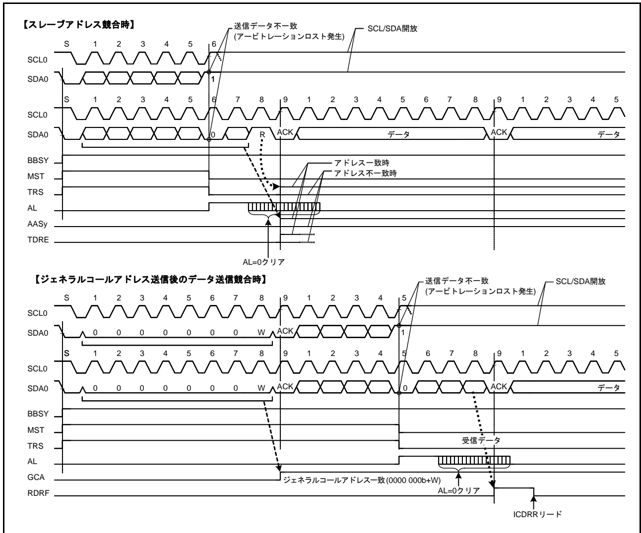
図 35.33 マスターアービトレーションロスト検出動作例 (MALE ビット = 1 のとき)
