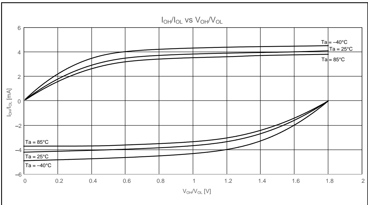
図 51.9 通常出力を選択したときの V OH /V OL 、I OH /I OL 温度特性 VCC = 1.8V (参考データ)
