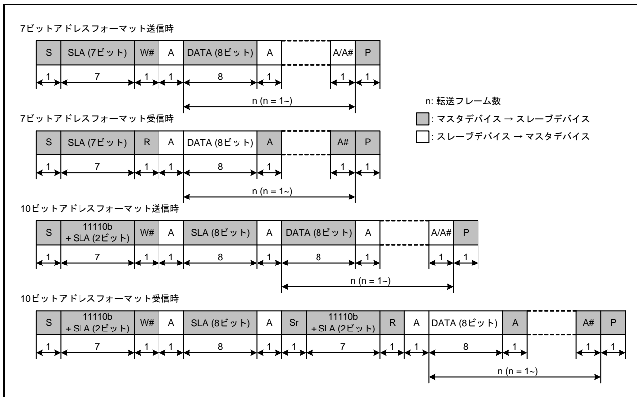
図 33.46 I 2 C バスフォーマット
