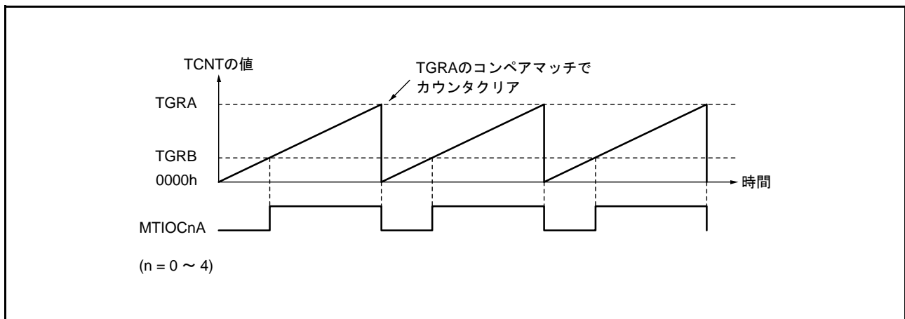
図 23.26 PWM モードの動作例
