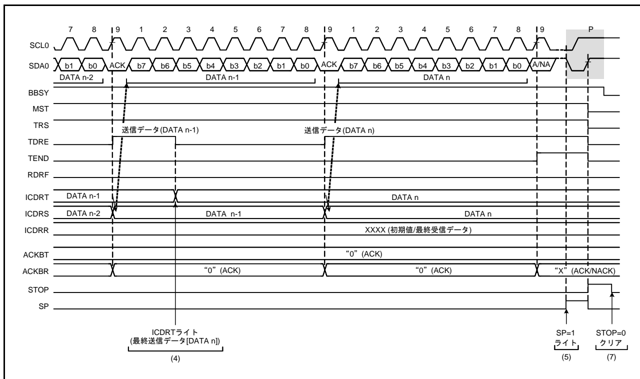
図 35.9 マスタ送信の動作タイミング (3)
