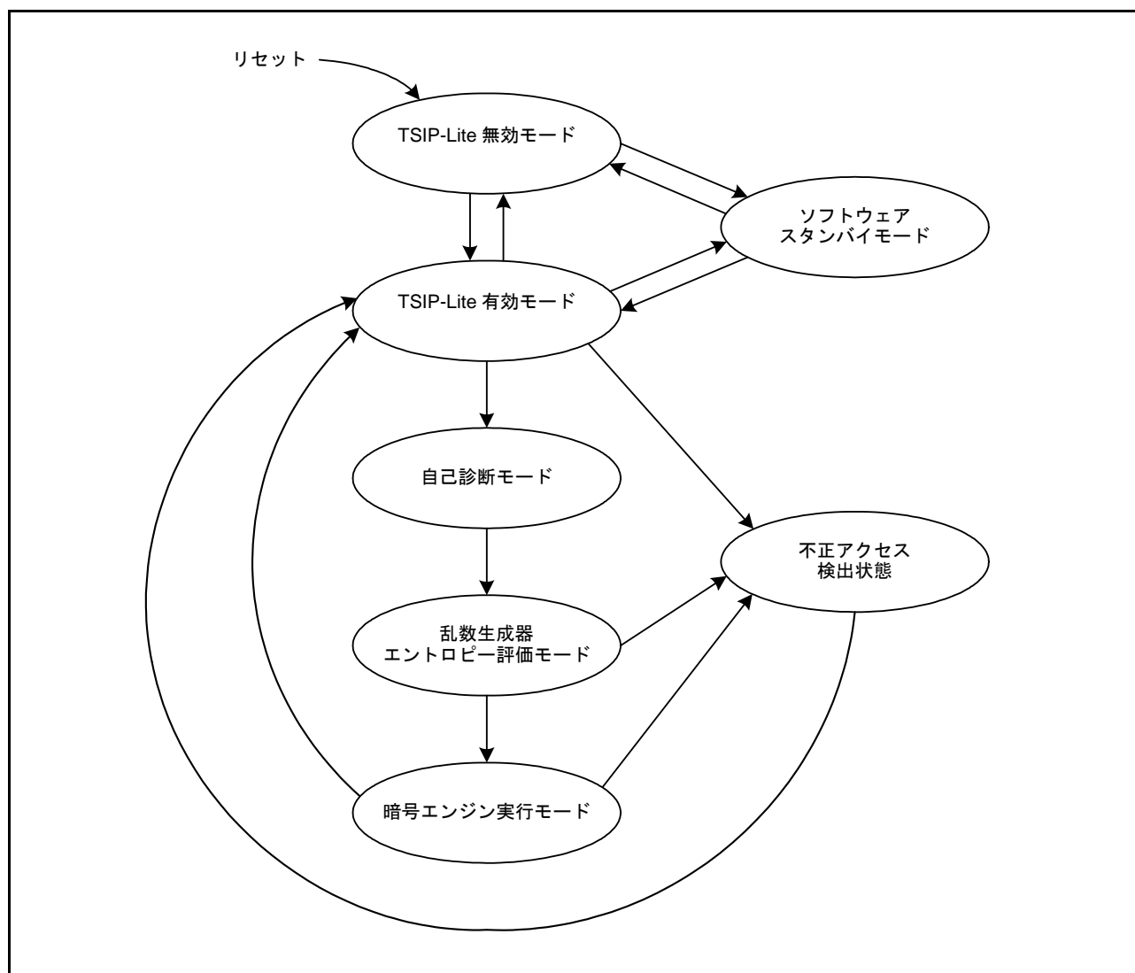
図 42.2 TSIP-Lite の動作モード状態遷移図
