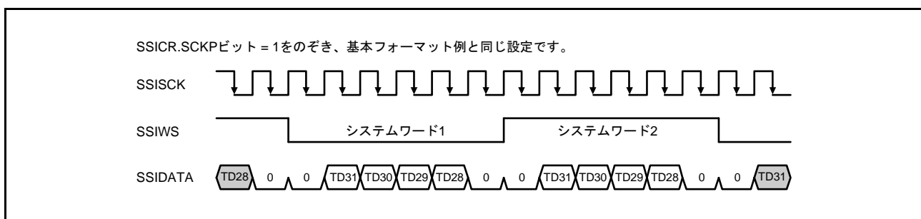
図 37.7 反転クロック
