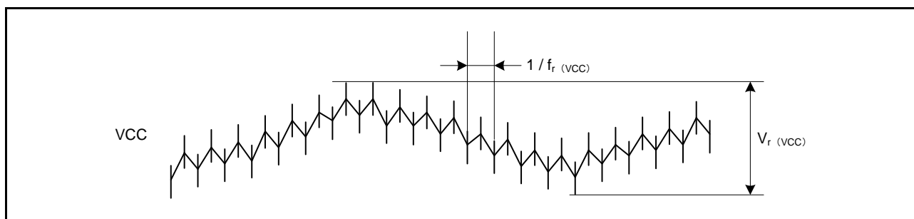
図 51.7 電源リップル波形
