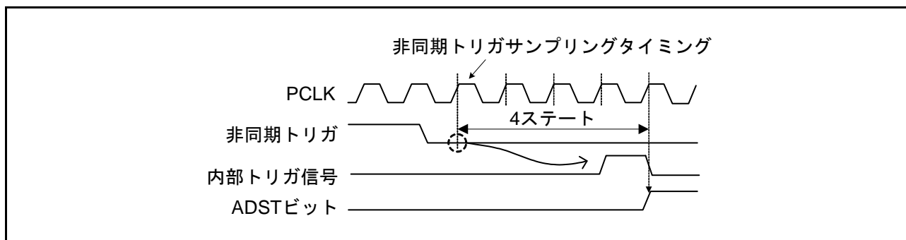
図 44.27 非同期トリガ入力タイミング
