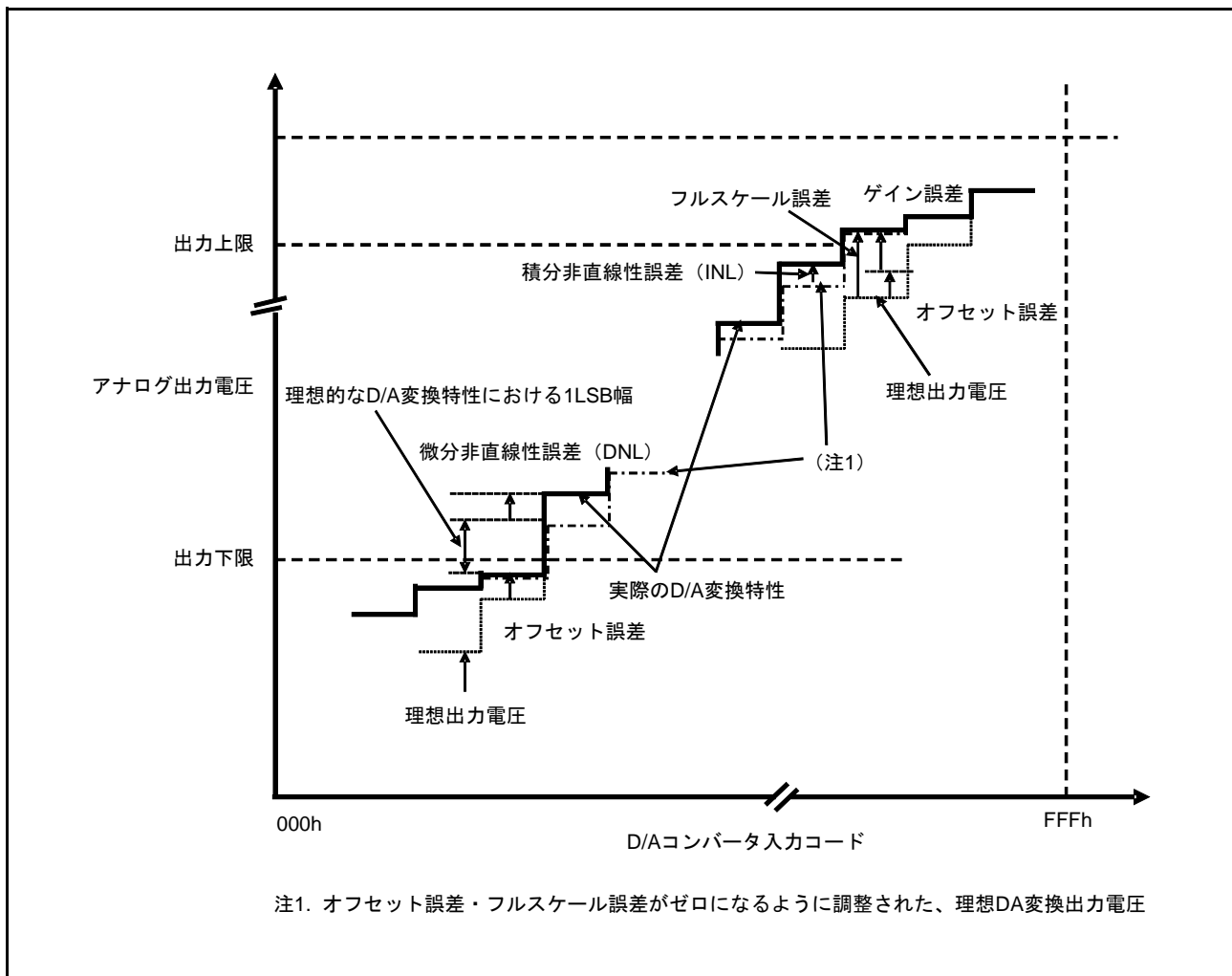
図 51.66 D/A コンバータ特性用語説明図
