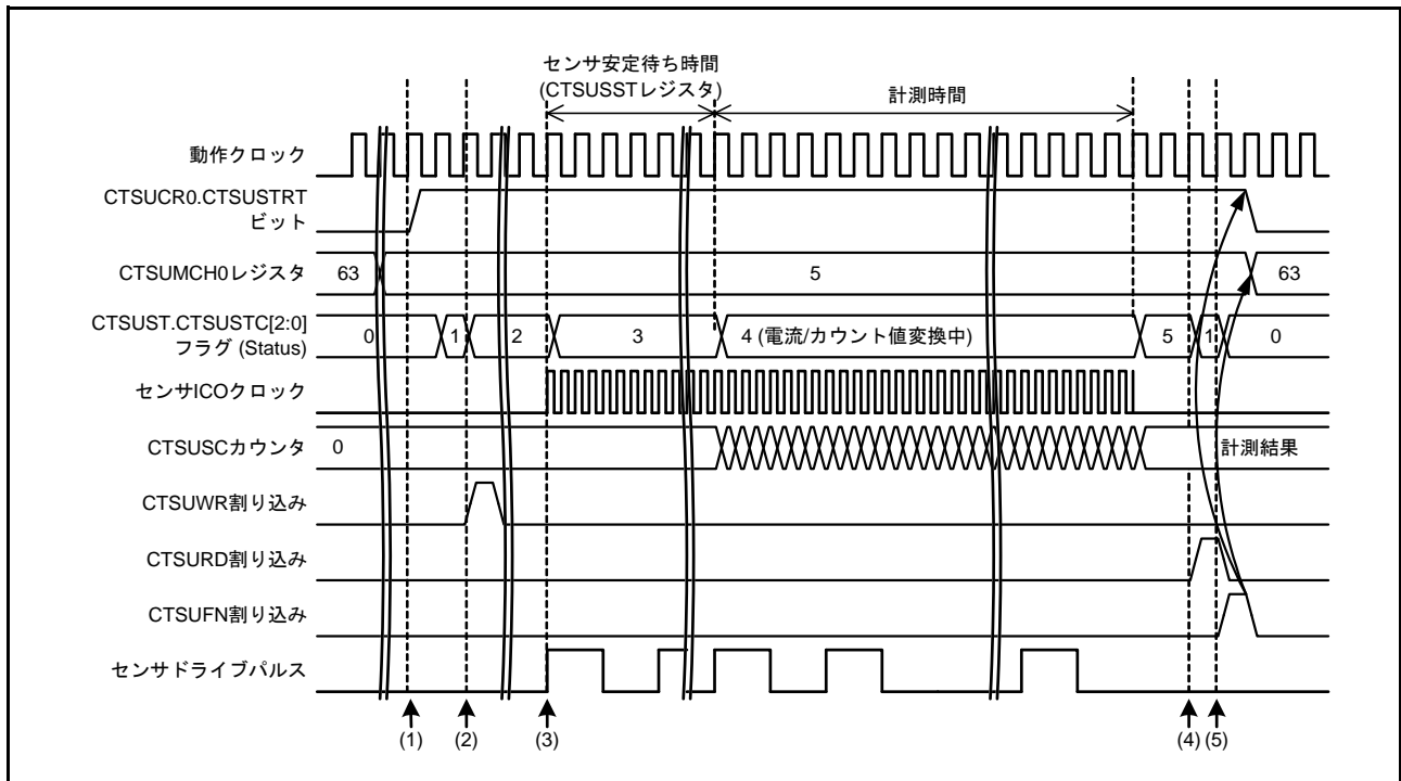
図 43.13 自己容量シングルスキャンモードのタイミングチャート (計測開始条件がソフトウェアトリガの場合)
