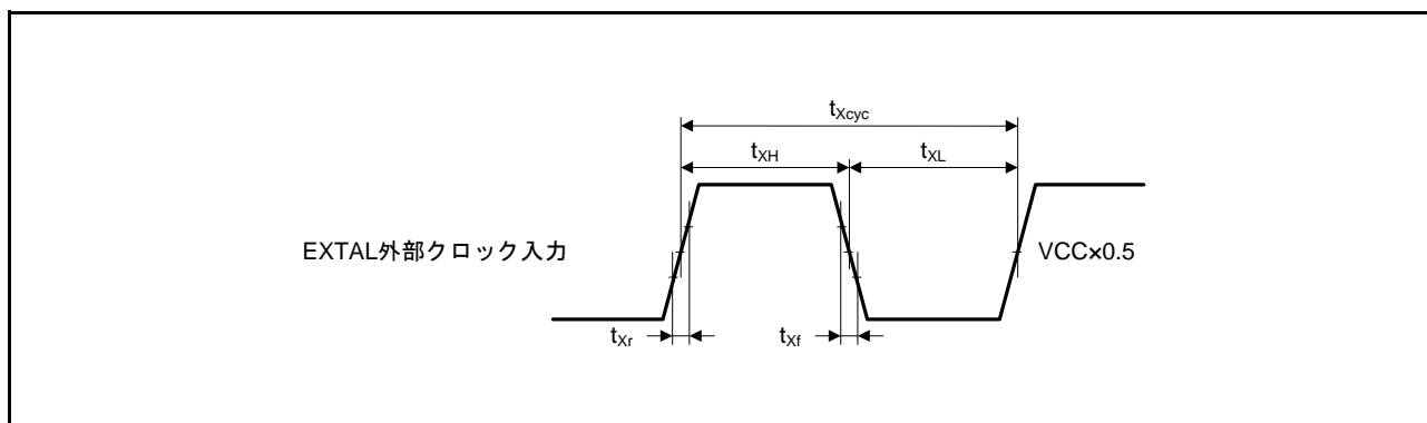
図 51.19 EXTAL 外部クロック入力タイミング
