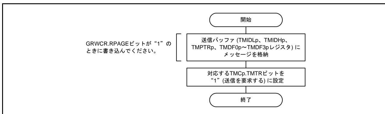
図 36.26 送信バッファからの送信手順
