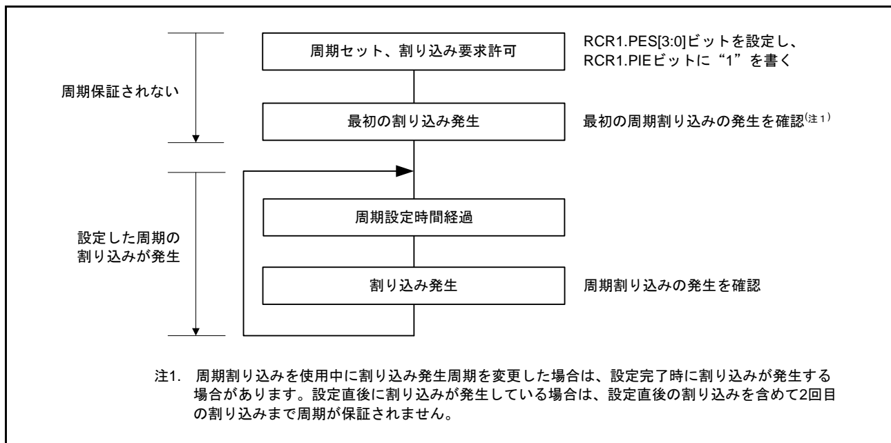
図 28.13 周期割り込み機能の使用法
