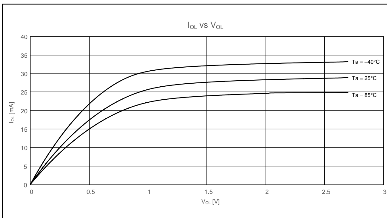
図 51.17 RIIC 出力端子の V_{OL} 、 I_{OL} 温度特性 V_{CC} = 2.7\text{V} (参考データ)
