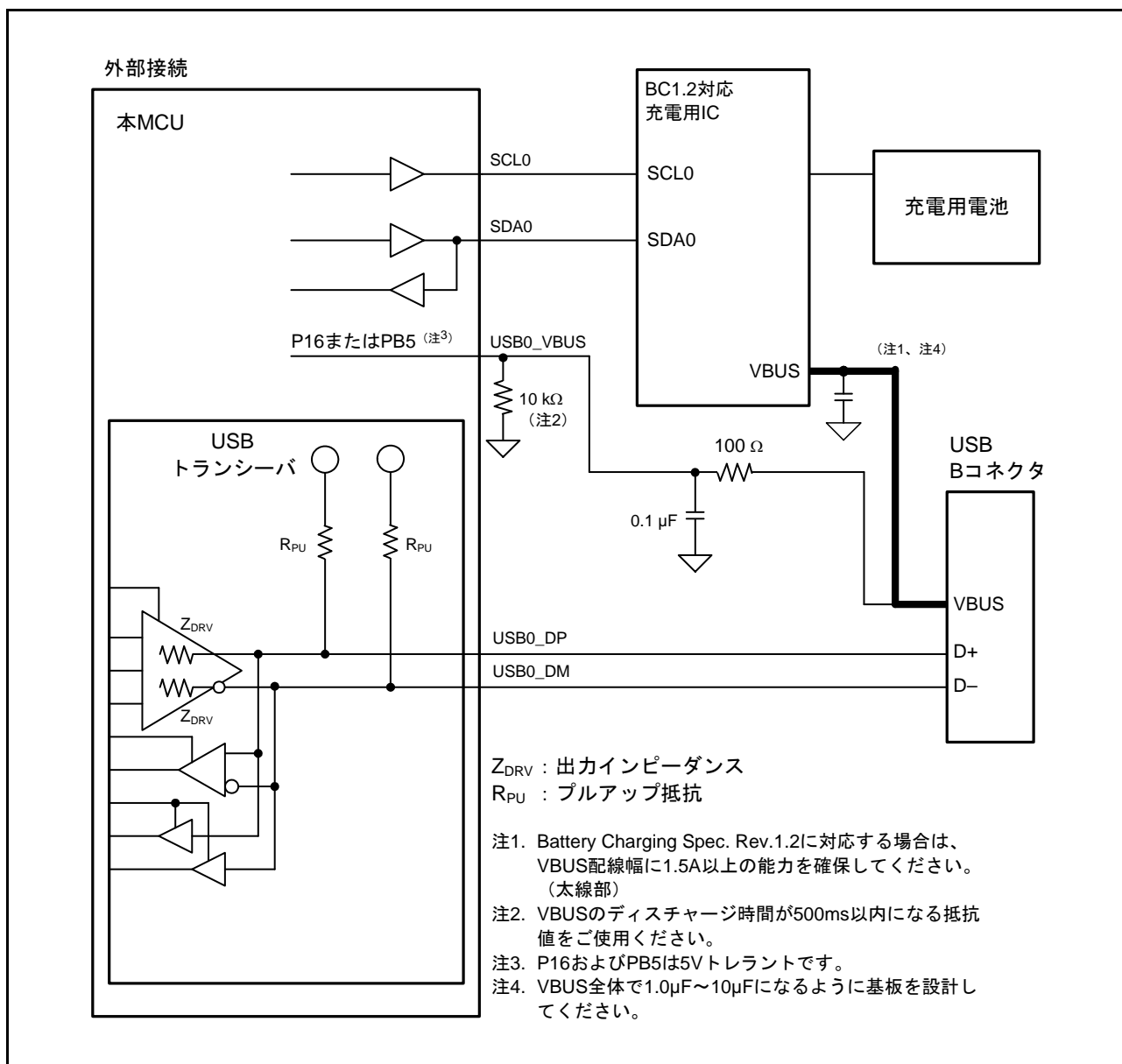
図 32.4 Battery Charging Specification Rev.1.2 対応時の USB コネクタのファンクション接続例
