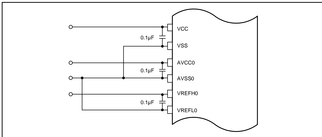
図 44.31 各電源端子の接続例
