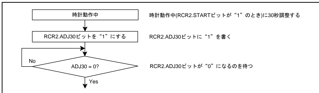
図 28.5 30秒調整手順
