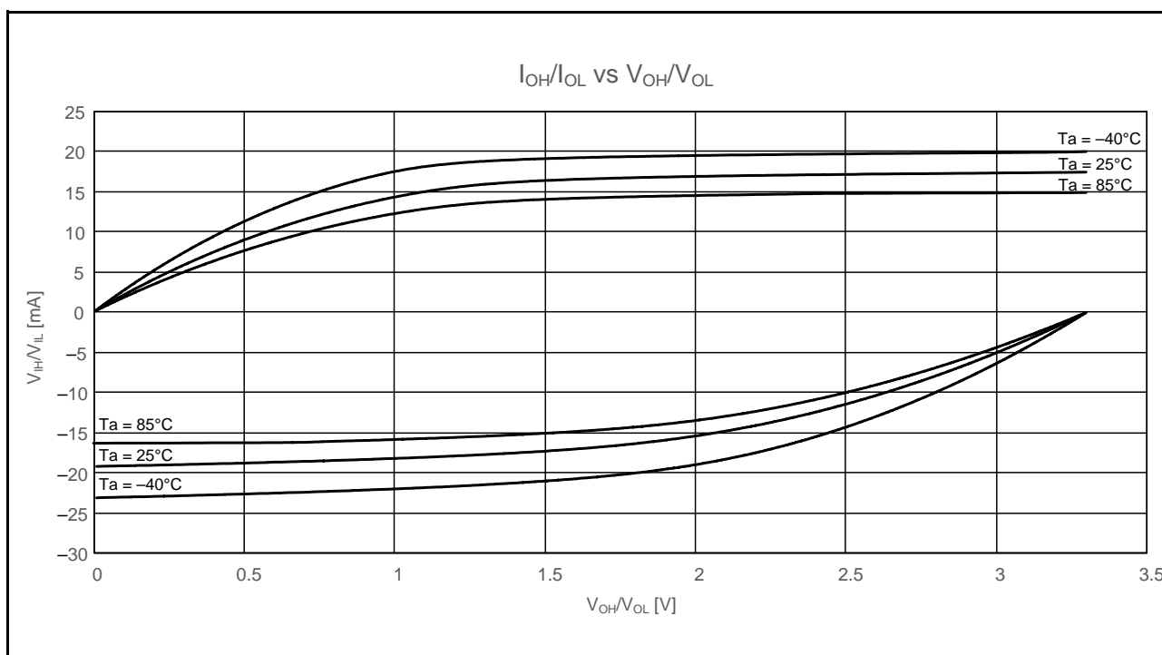
図 51.11 通常出力を選択したときの V_{OH}/V_{OL} 、 I_{OH}/I_{OL} 温度特性 V_{CC} = 3.3V (参考データ)
