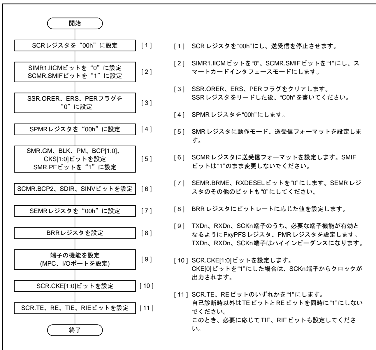
図 33.38 SCIの初期化フローチャートの例 (スマートカードインタフェースモード)
