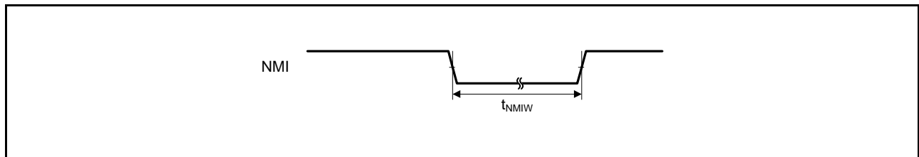
図 51.32 NMI 割り込み入力タイミング
