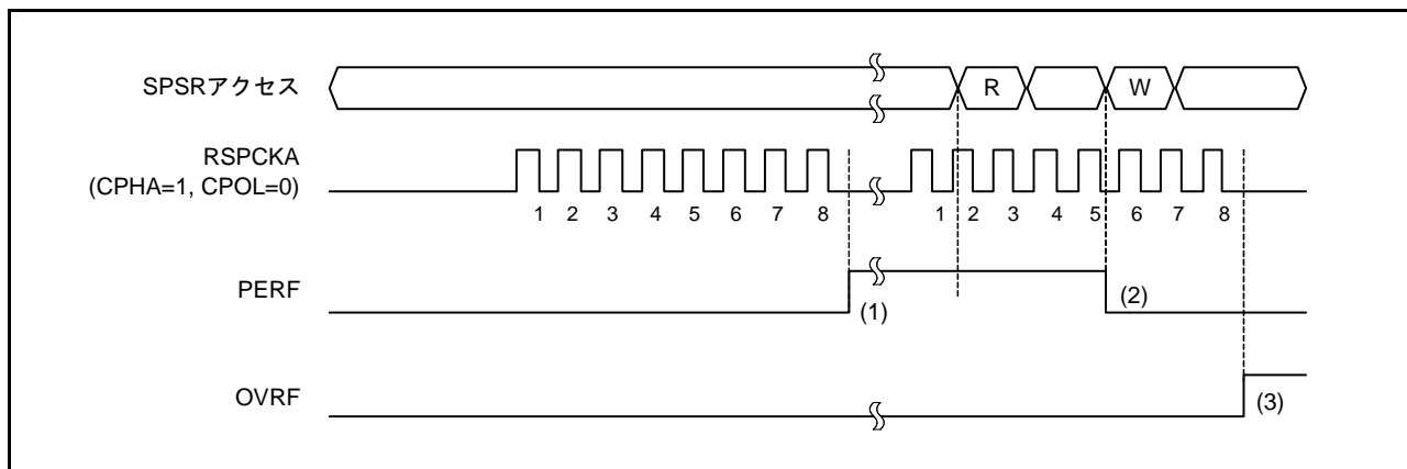
図 38.30 PERF フラグの動作例
