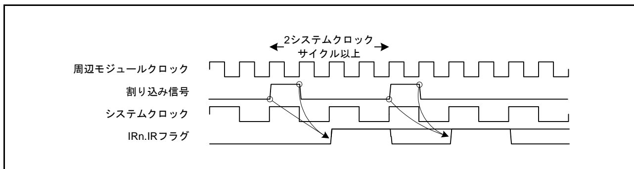
図 15.3 連続する割り込み要求発行の間隔 (システムクロック周波数 < 周辺モジュールクロック周波数の場合)
