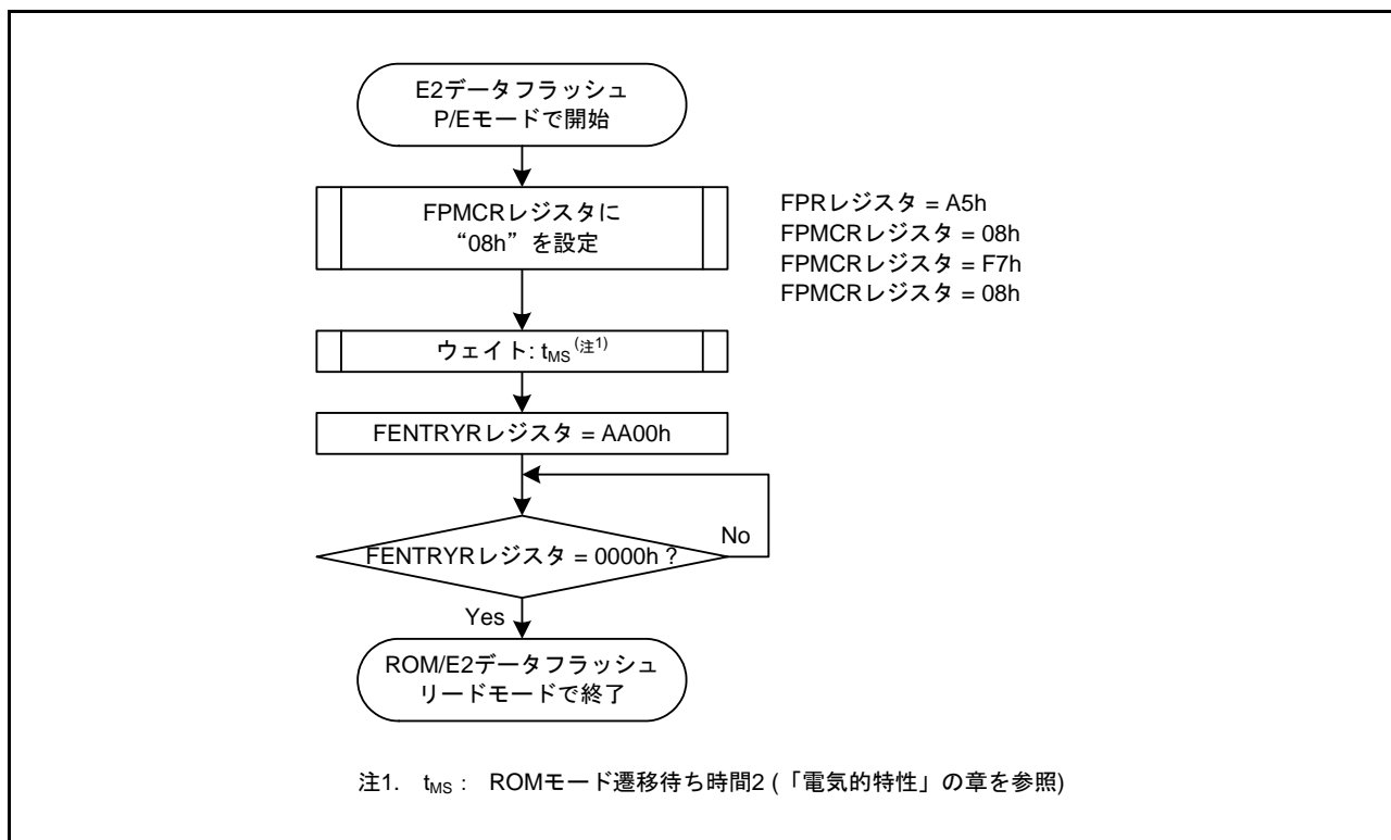
図 50.11 E2 データフラッシュ P/E モードから ROM/E2 データフラッシュリードモードへの遷移フロー
