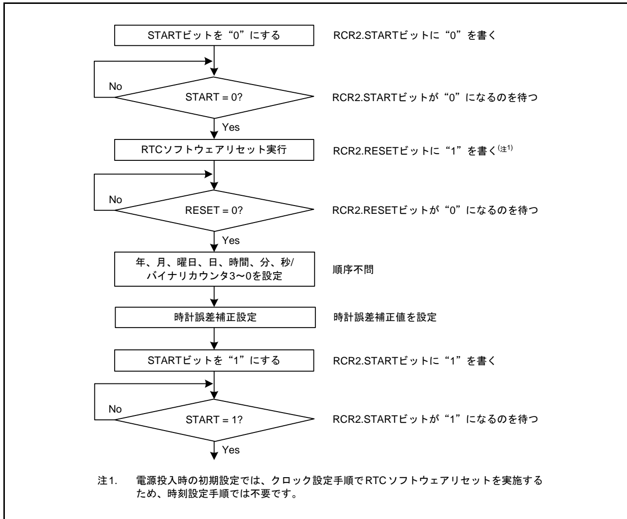
図 28.4 時刻設定手順
