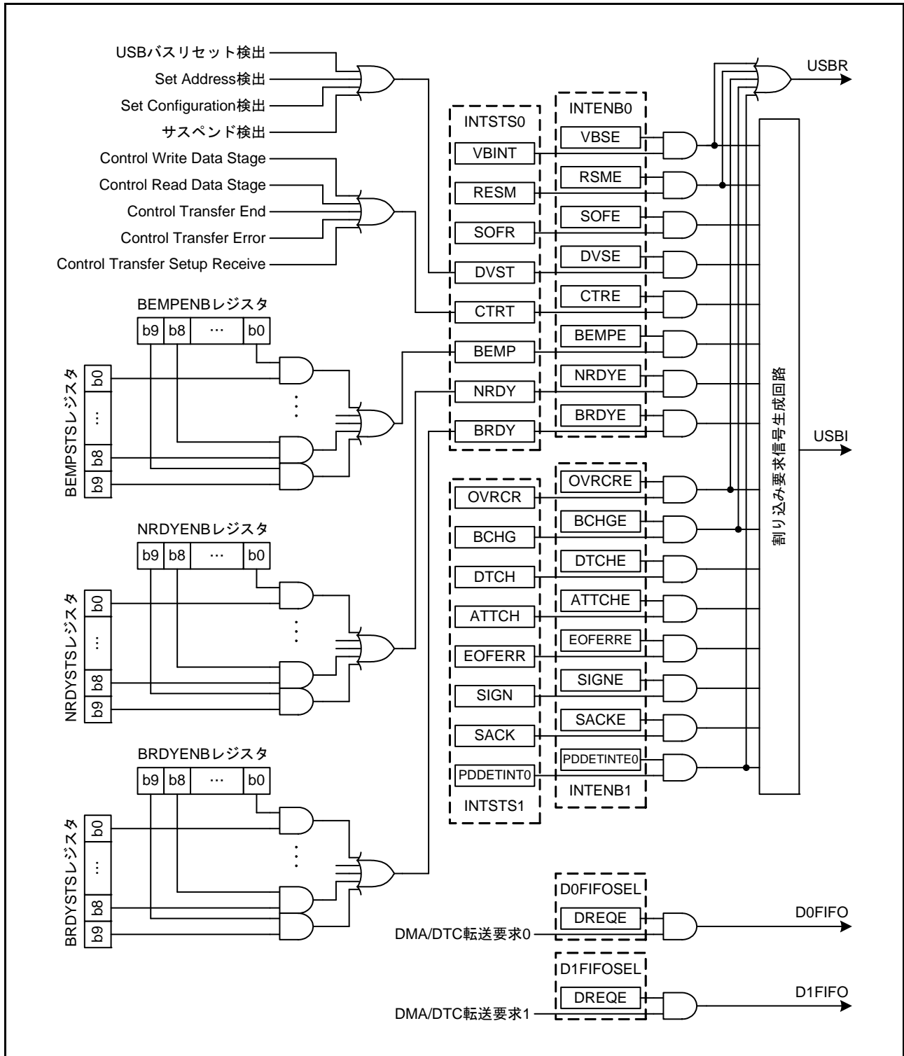
図 32.7 USB 割り込みの関連図
