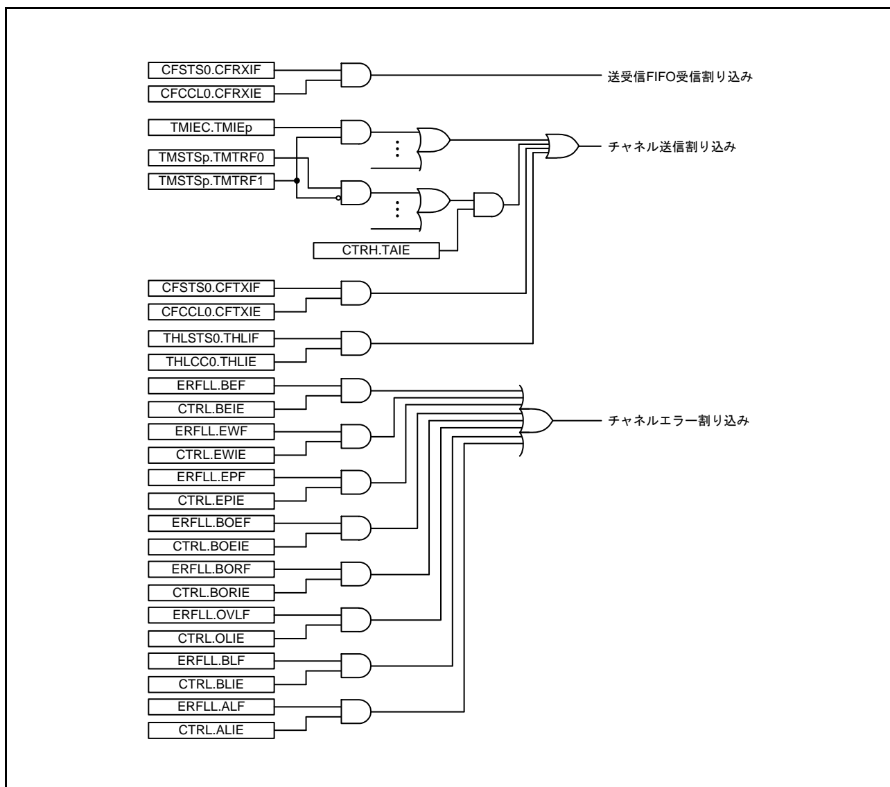
図 36.14 CAN チャンネル割り込みブロック図
