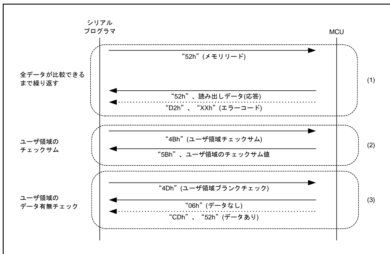
図 50.39 ユーザ領域のデータ確認手順
