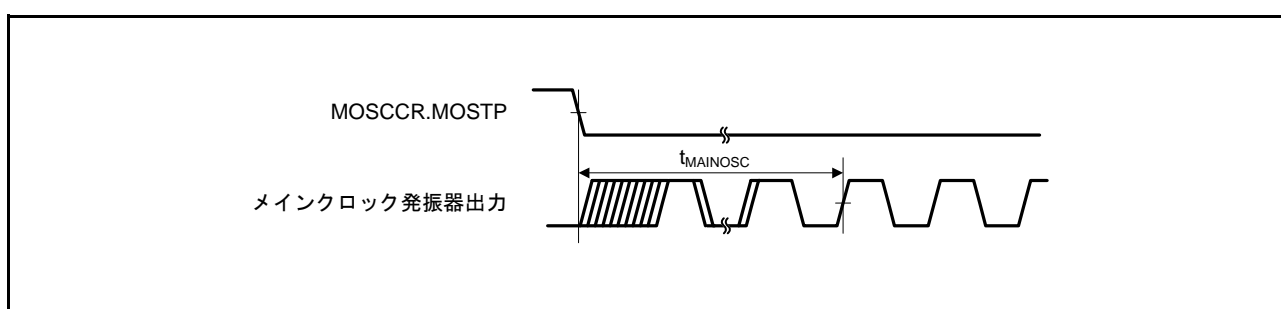
図 51.20 メインクロック発振開始タイミング
