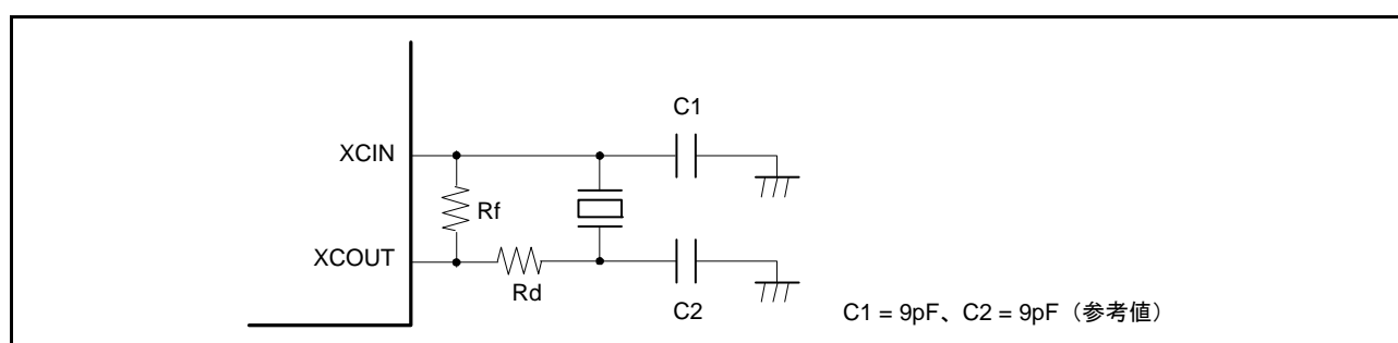
図 9.8 32.768kHz 水晶振動子の接続例
