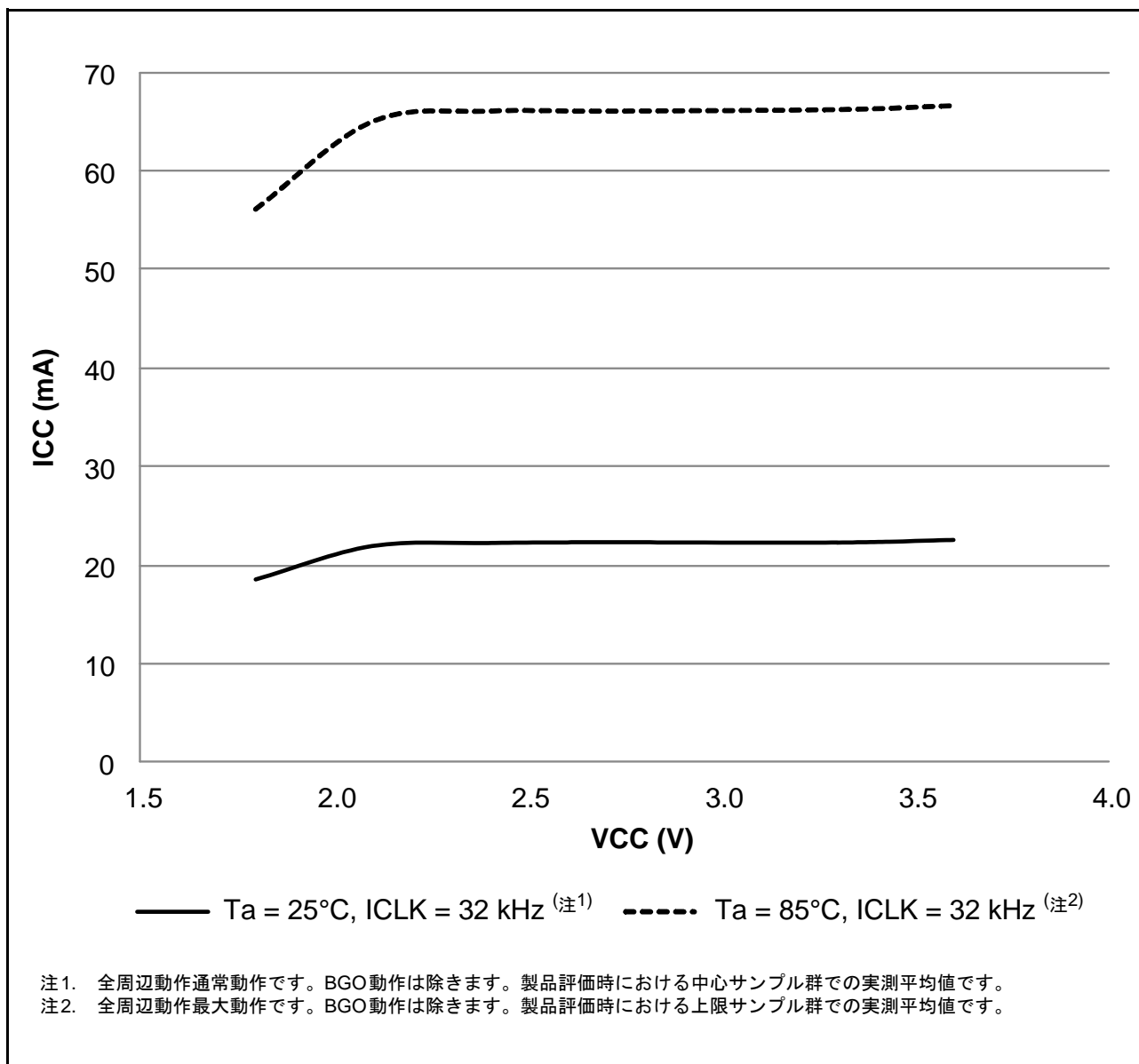
図 51.3 低速動作モードの電圧依存性 (参考データ)
