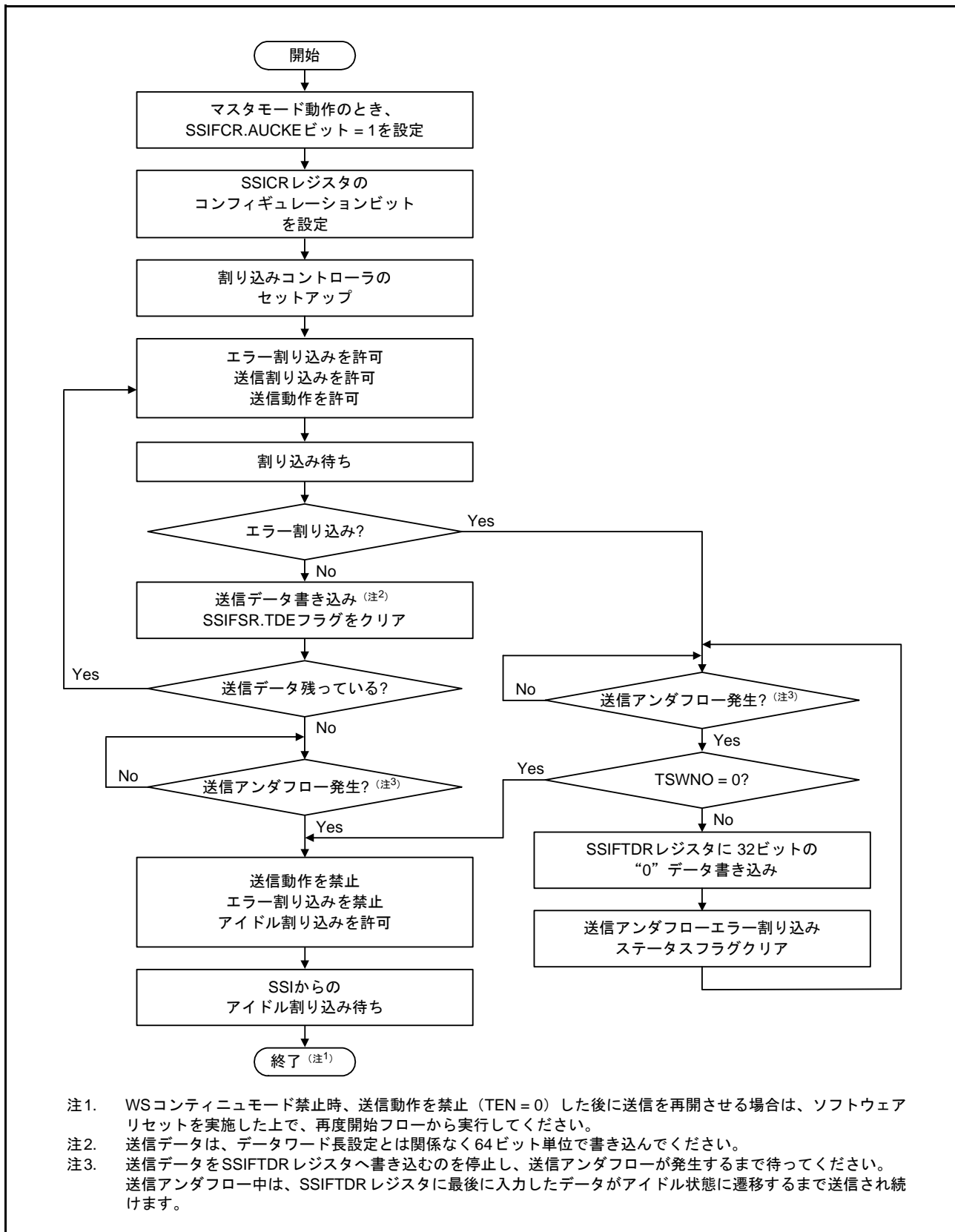
図 37.19 割り込みを使用した送信
