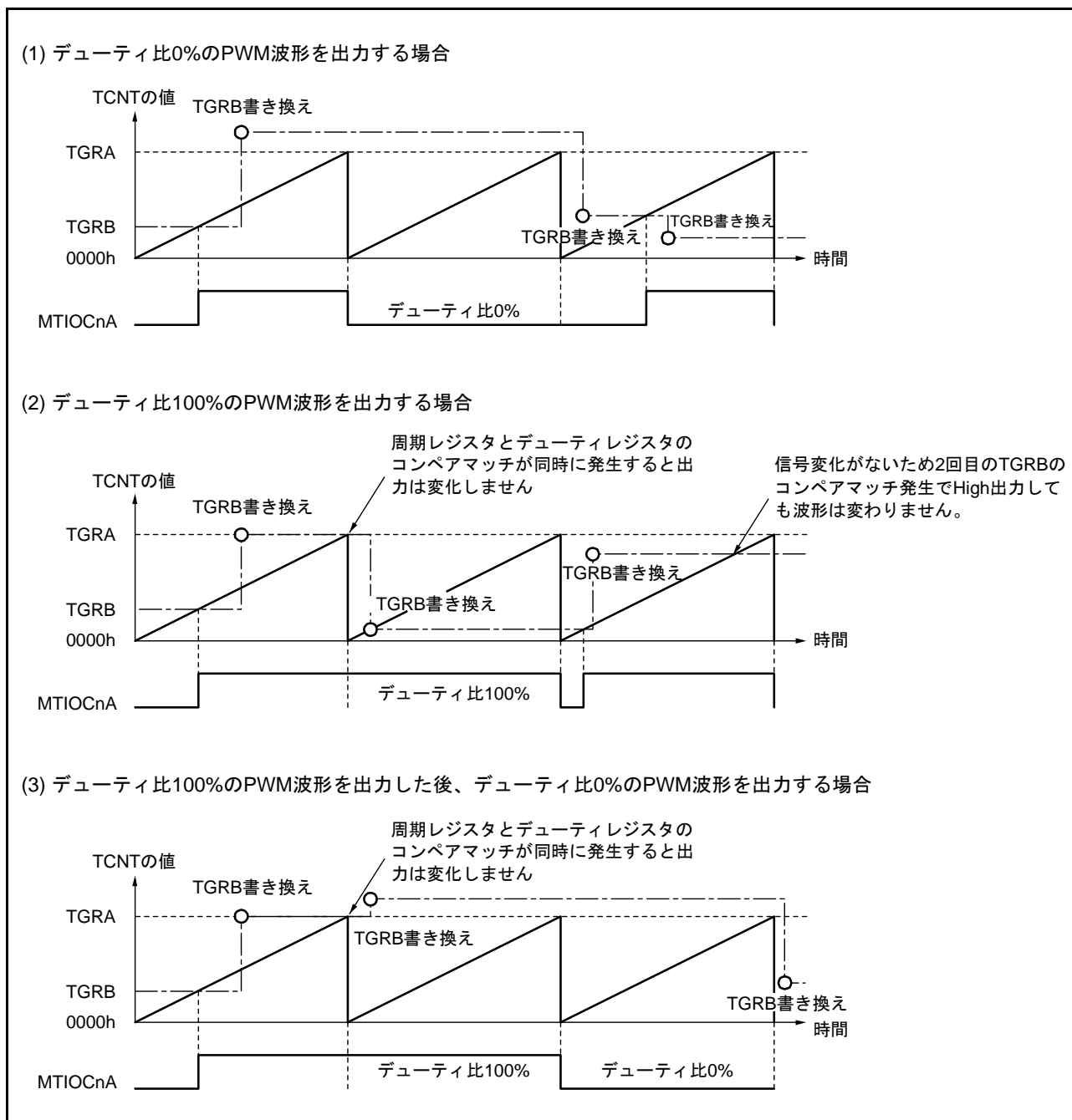
図 23.28 PWMモード動作例 (デューティ0%、デューティ100%のPWM波形を出力する例) (n = 0 ~ 4)
