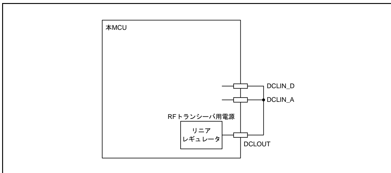
図 41.6 BLE 外部接続回路例 (83 ピン LGA)
