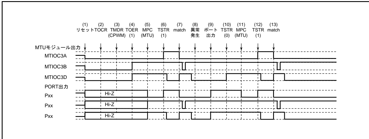
図 23.138 相補 PWM モードで異常が発生し、相補 PWM モードで復帰する場合
