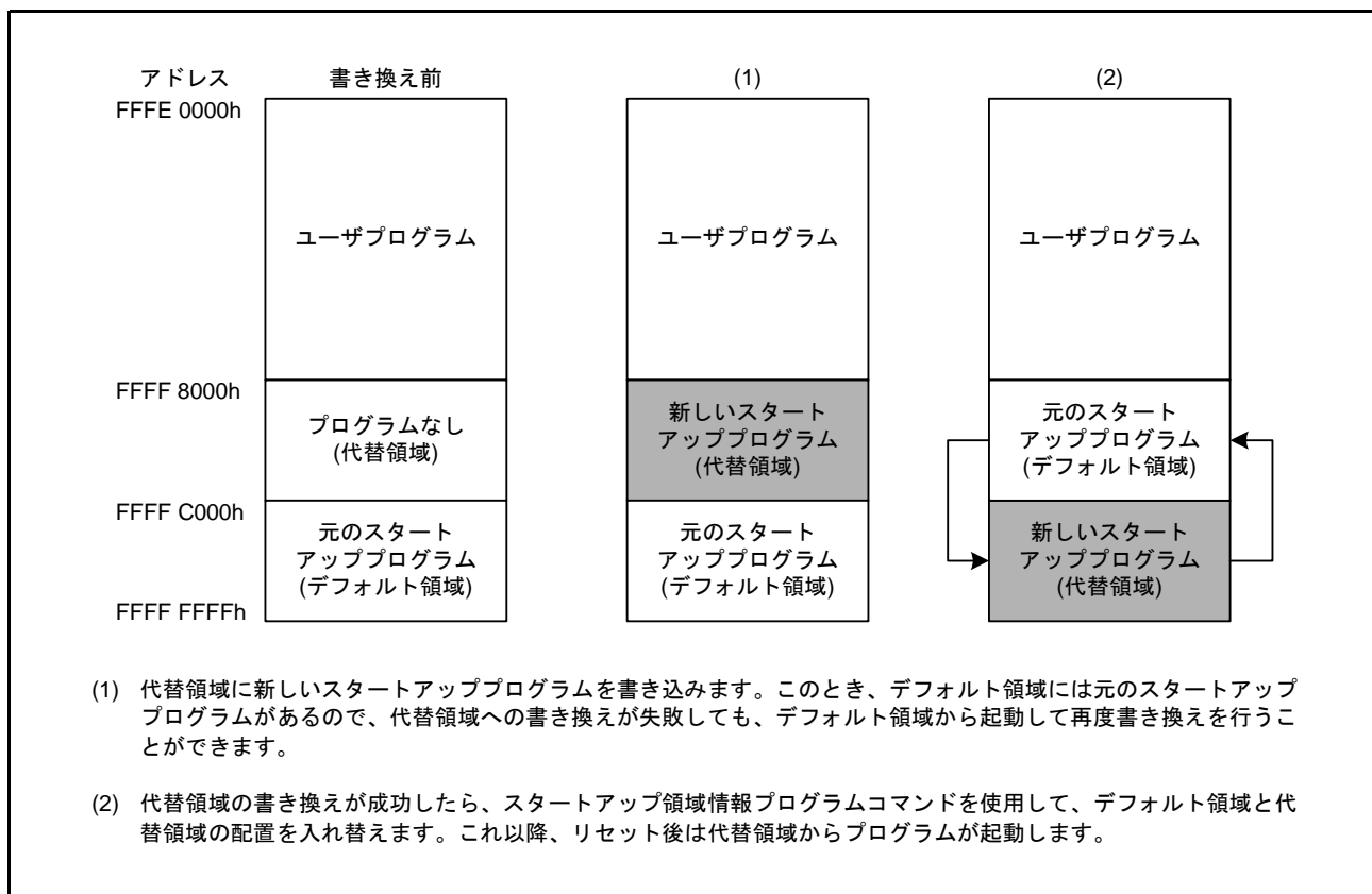
図 50.4 スタートアッププログラム保護機能の概念
