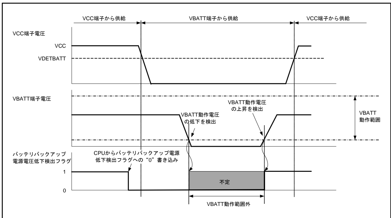
図 12.4 バッテリバックアップ電源低下検出フラグの動作
