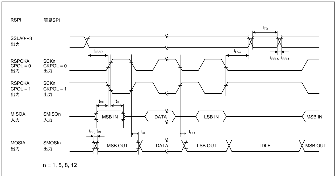
図 51.49 RSPI タイミング (マスタ、CPHA = 0) / 簡易 SPI クロックタイミング (マスタ、CKPH = 1)
