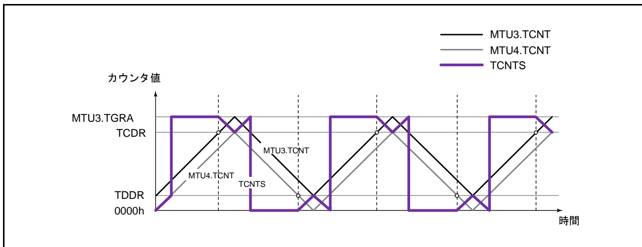
図 23.39 相補 PWM モードのカウンタ動作
