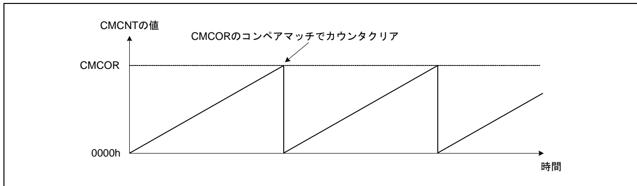
図 27.2 CMCNT カウンタの動作
