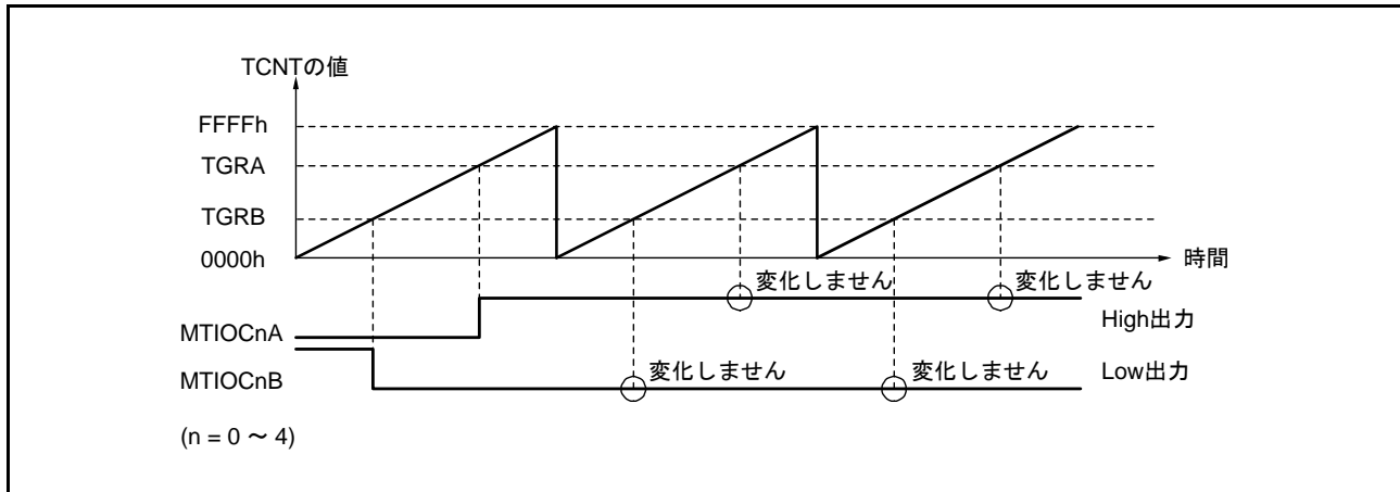
図 23.8 Low 出力 / High 出力の動作例
