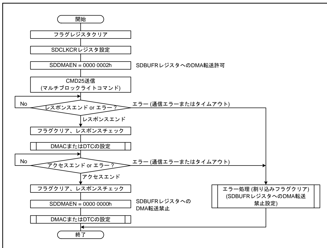
図 40.22 マルチブロックライトコマンド (CMD25) を送信した後、DMA 転送で SDBUFR レジスタへ転送する例
