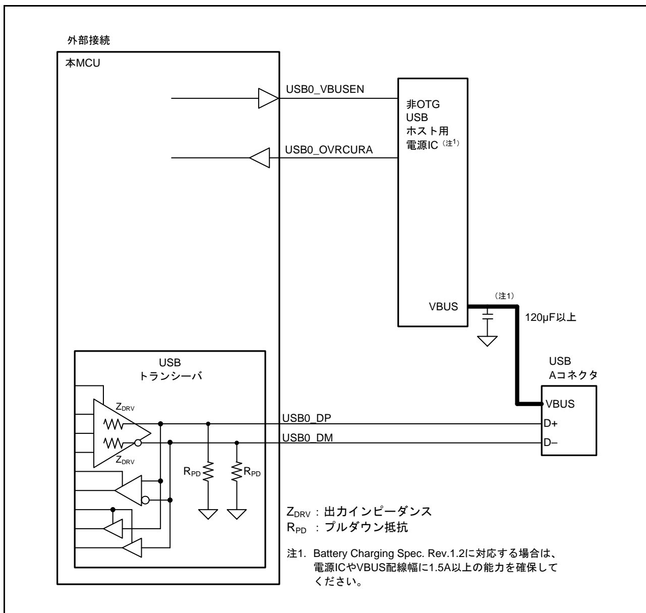
図 32.5 USB コネクタのホスト接続例
