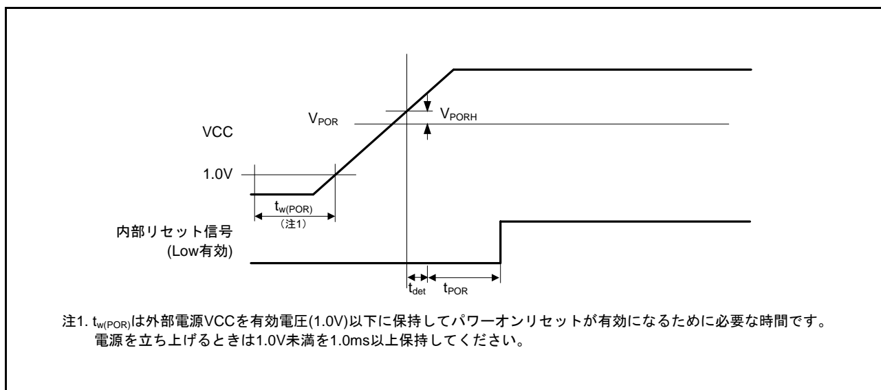
図 51.70 パワーオンリセットタイミング
