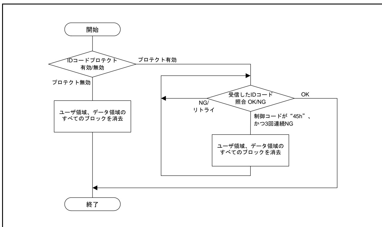
図 50.29 ブートモード ID コードプロテクトの認証フロー
