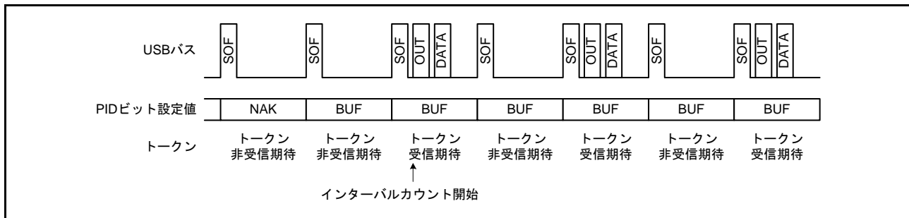
図 32.16 IITV[2:0] = 000b 以外の場合のフレームとトークン受信期待有無の関係
