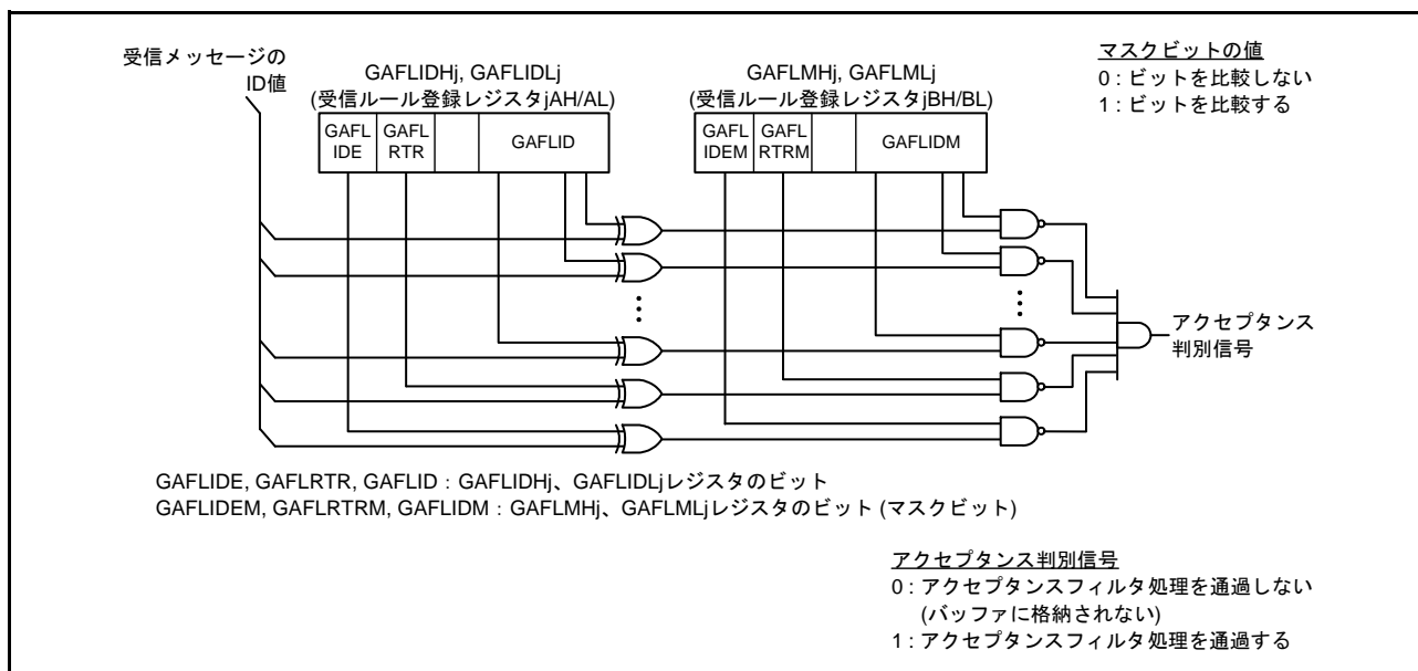
図 36.5 アクセプタンスフィルタ機能
