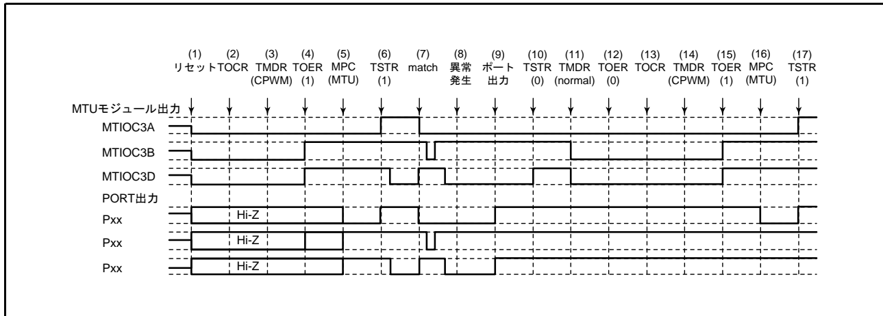
図 23.139 相補 PWM モードで異常が発生し、相補 PWM モードで復帰する場合
