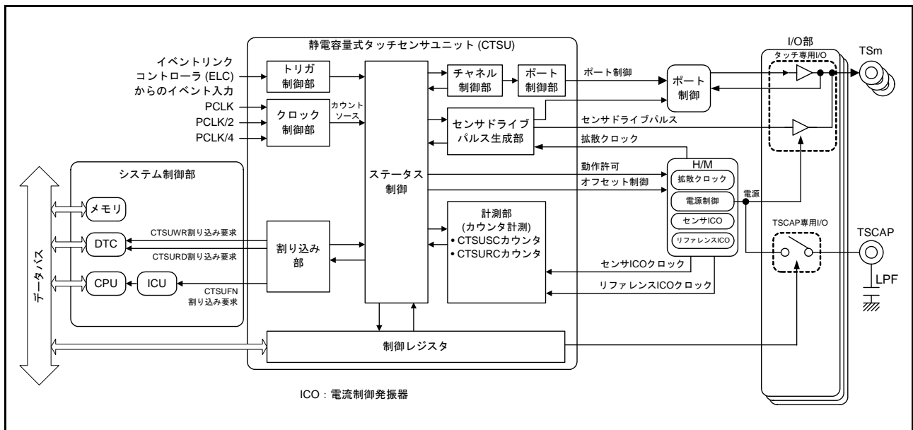
図 43.3 CTSU のブロック図 (m = 2, 3, 4, 7, 8, 12, 13, 22, 23, 27, 30, 35)
