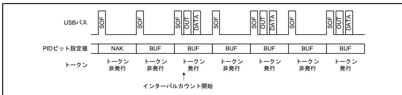
図 32.14 IITV[2:0] = 001b の場合のトークン発行有無
