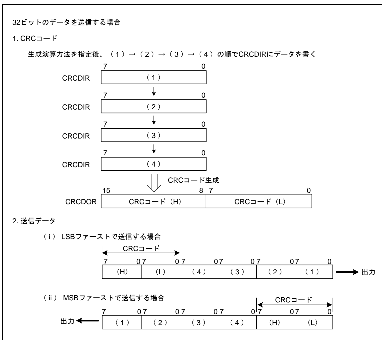
図 39.6 LSB ファーストと MSB ファーストの送信データ
