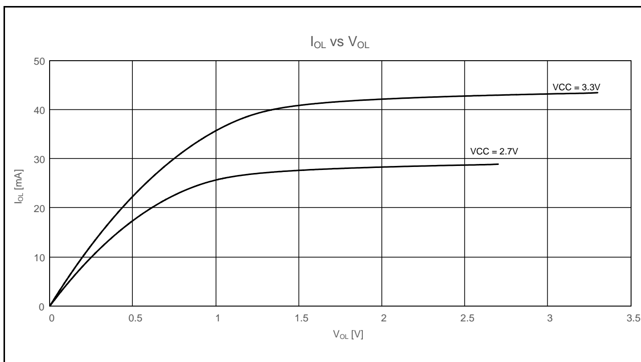
図 51.16 RIIC 出力端子の V_{OL} 、 I_{OL} 電圧特性 T_a = 25^\circ\text{C} (参考データ)
