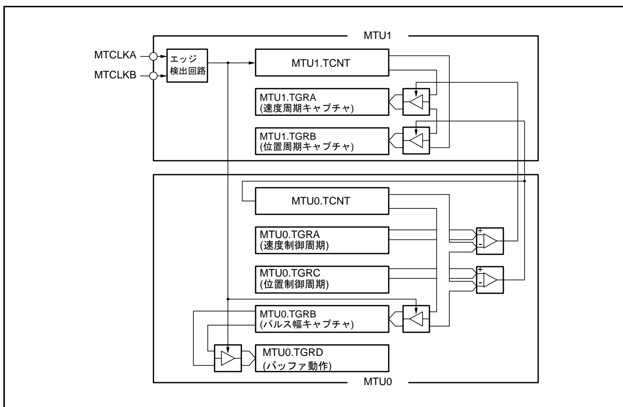
図 23.34 位相計数モードの応用例
