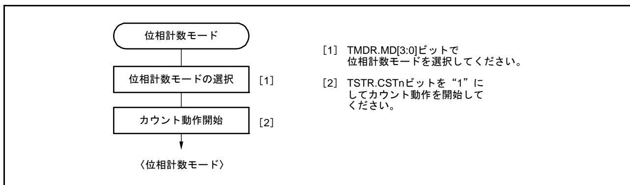
図 23.29 位相計数モードの設定手順例
