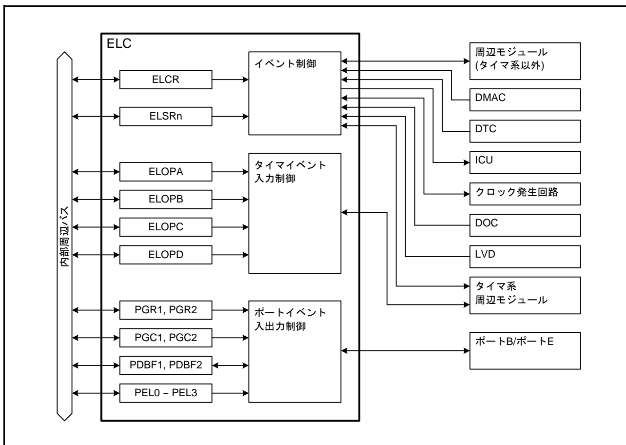
図 20.1 ELC のブロック図 (n = 1 ~ 4, 7, 8, 10, 12, 14 ~ 16, 18 ~ 29)
