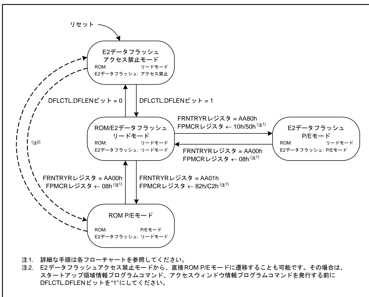
図 50.6 フラッシュメモリのモード遷移図
