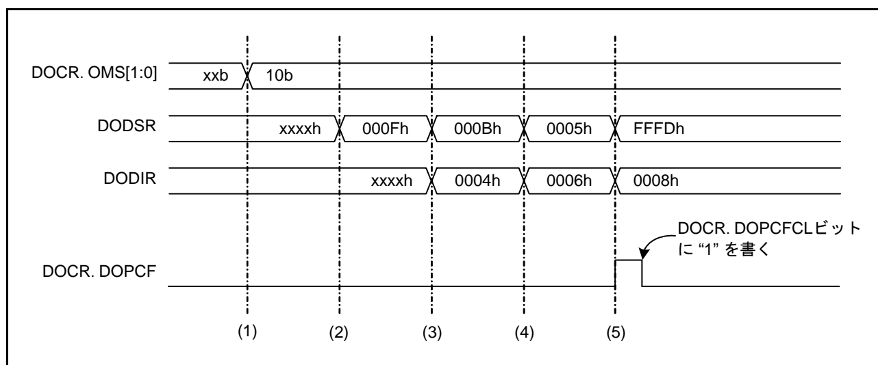
図 48.4 データ減算モードの動作例
