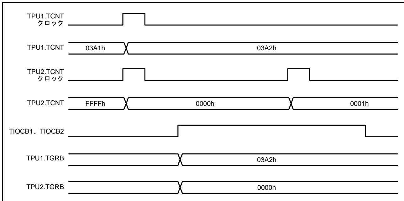
図 25.18 カスケード接続動作例 (1)
