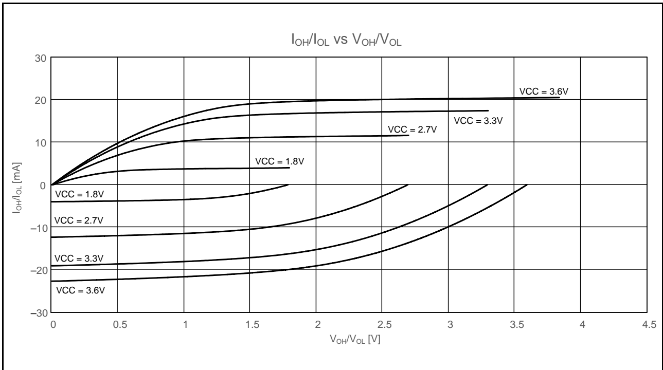
図 51.8 通常出力を選択したときの V OH /V OL 、I OH /I OL 電圧特性 T a = 25°C (参考データ)
