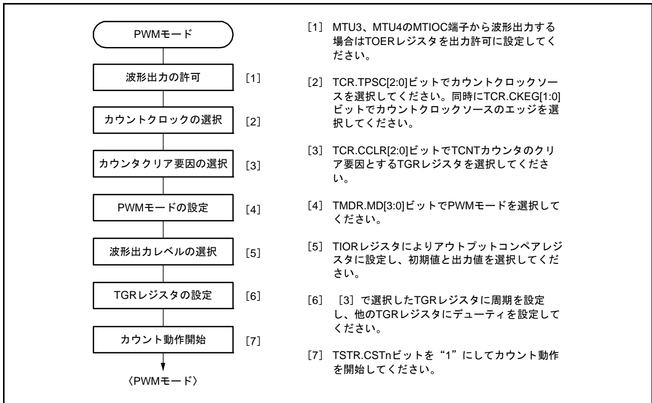
図 23.25 PWM モードの設定手順例
