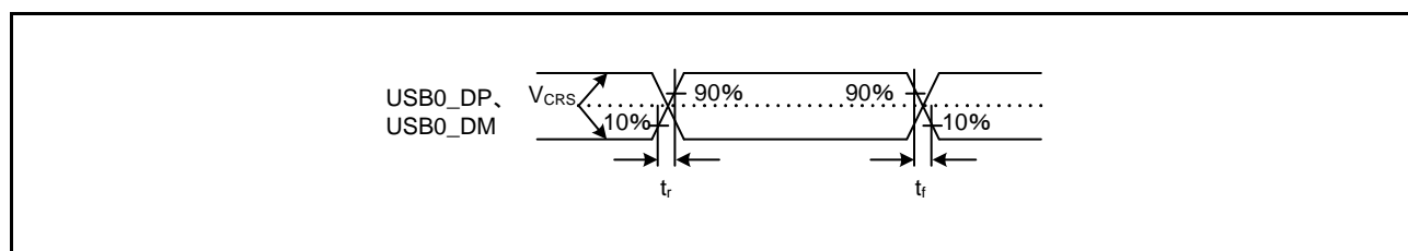
図51.61 USB0_DP、USB0_DM 出力タイミング
