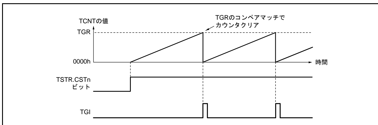
図 23.6 周期カウンタの動作
