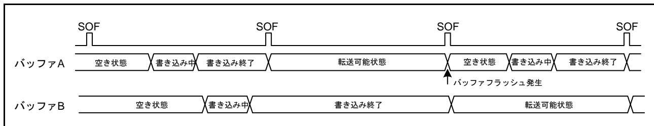
図 32.18 バッファフラッシュ機能動作例
