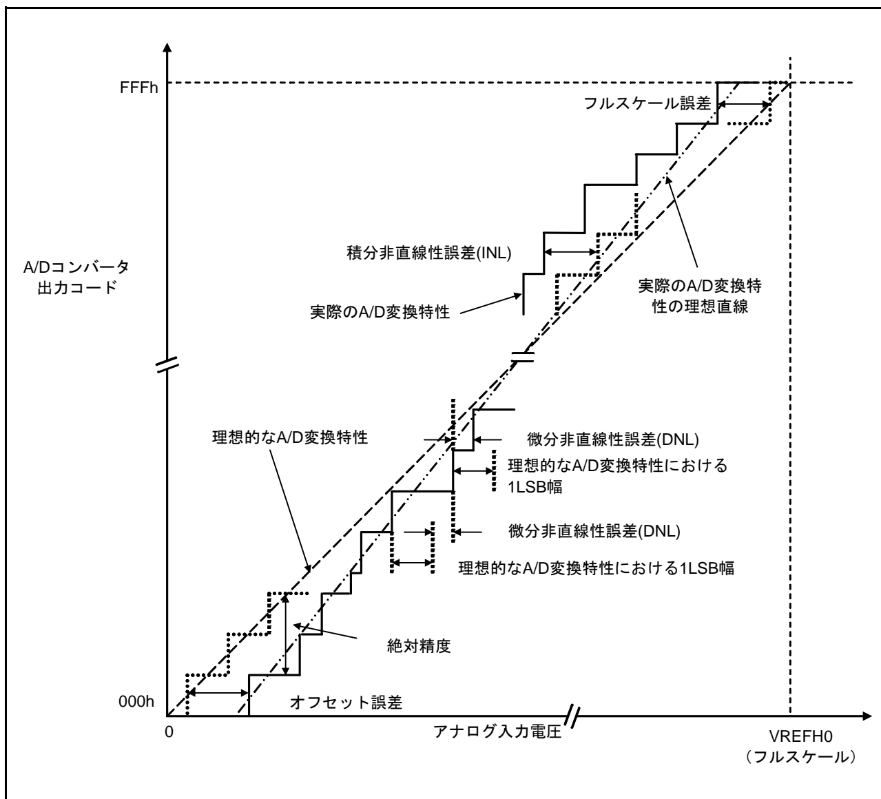
図 51.65 A/D コンバータ特性用語説明図
