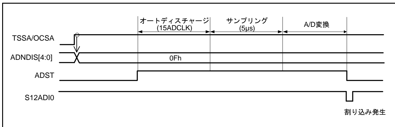
図 44.7 シングルスキャンモードの動作例 (温度センサ出力、内部基準電圧選択)
