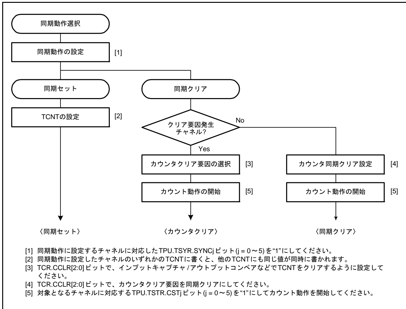
図 25.10 同期動作の設定手順例
