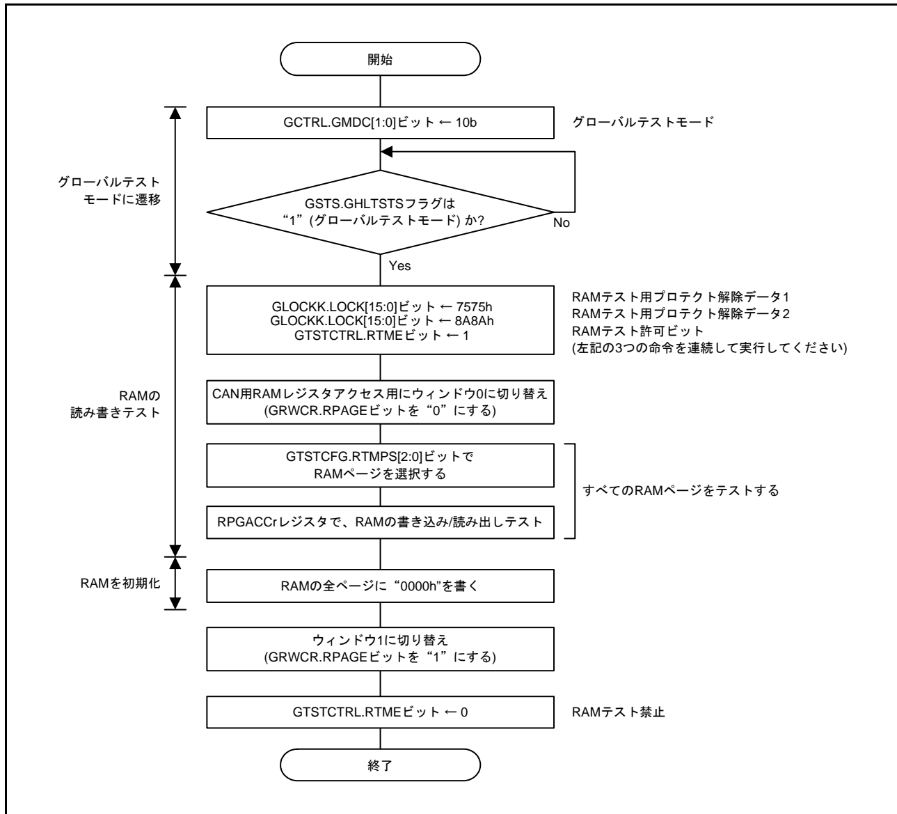
図 36.35 RAMテストの設定手順
