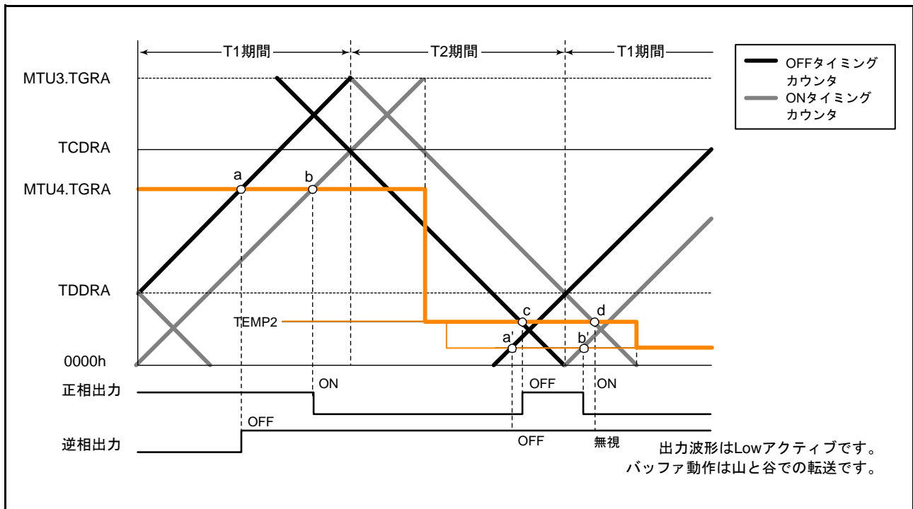
図 23.48 相補 PWM モード波形出力例 (3)
