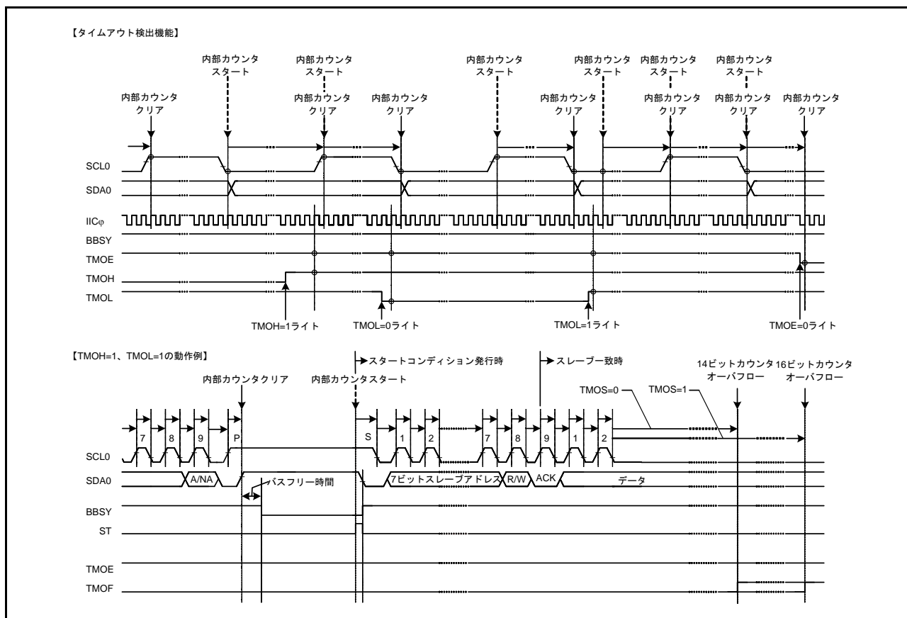
図 35.39 タイムアウト検出機能
