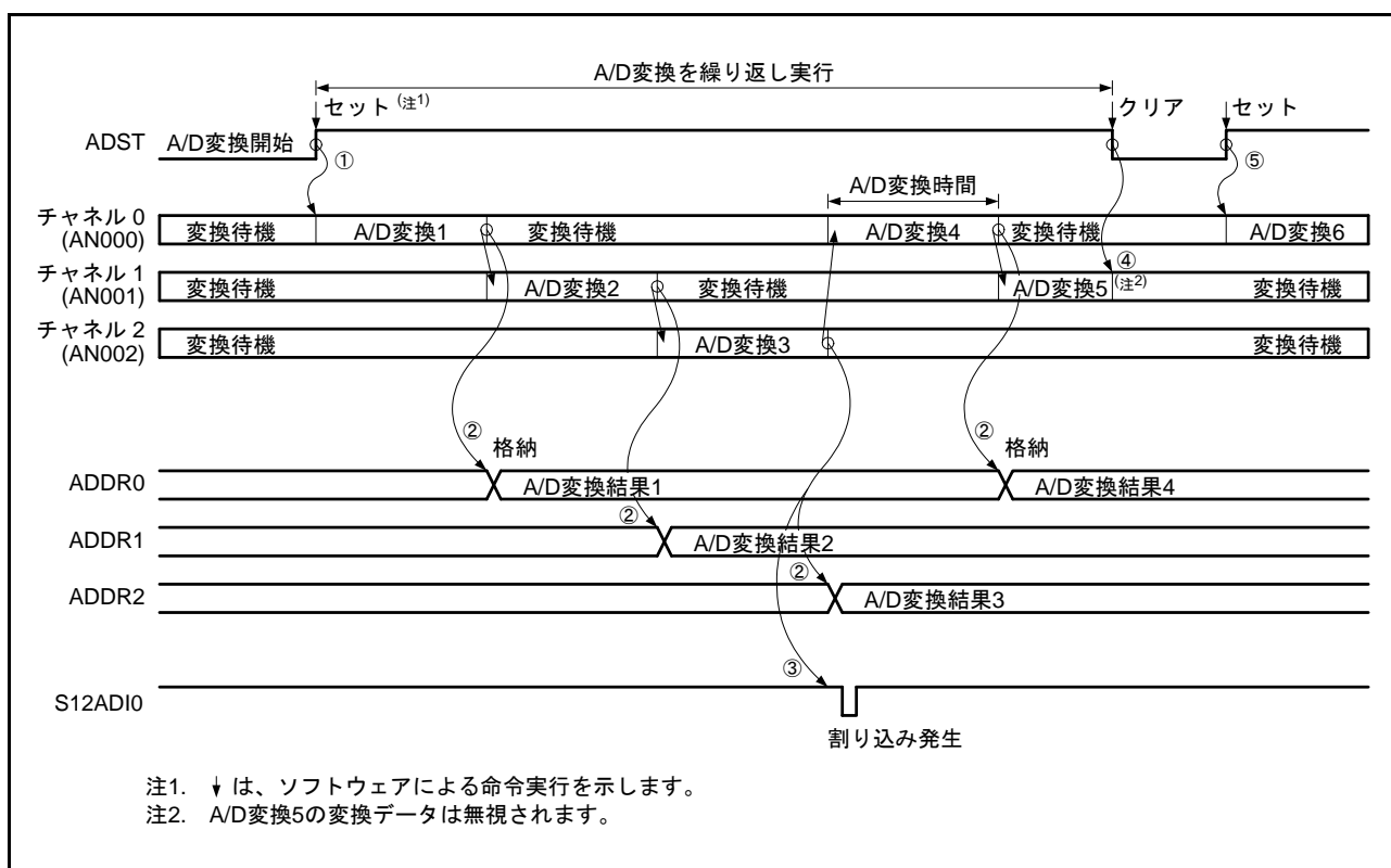
図 44.9 連続スキャンモードの動作例 (基本動作 : AN000、AN001、AN002 選択)
