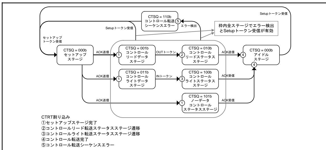
図 32.12 コントロール転送ステージ遷移図
