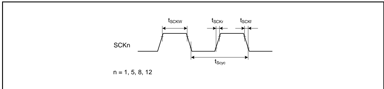
図 51.39 SCKクロック入カタイミング
