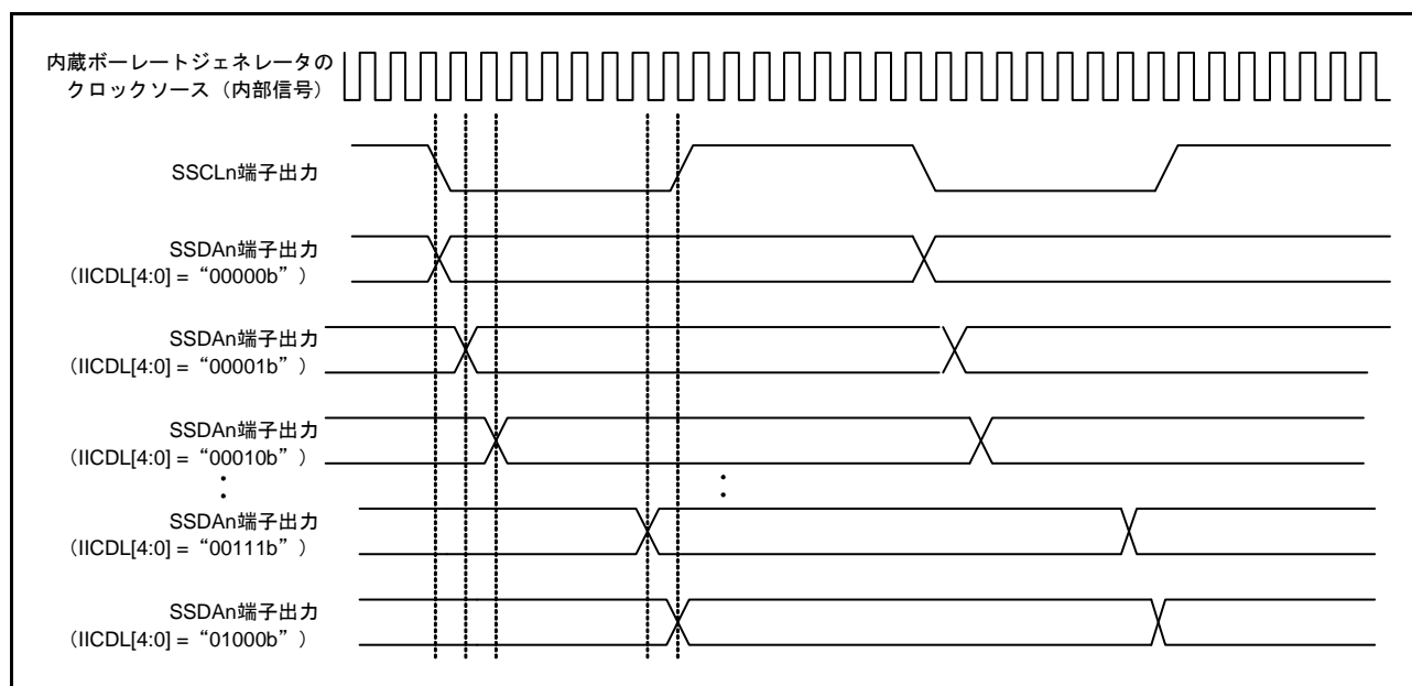
図 33.50 SSDA 出力遅延のタイミング
