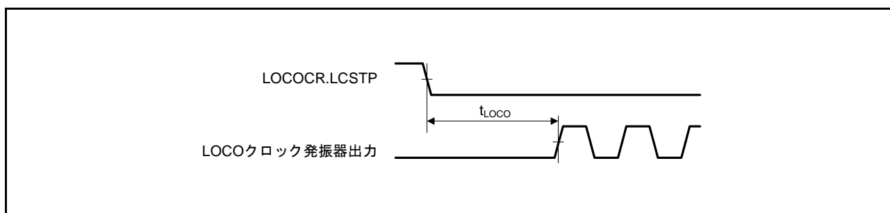
図 51.21 LOCO クロック発振開始タイミング
