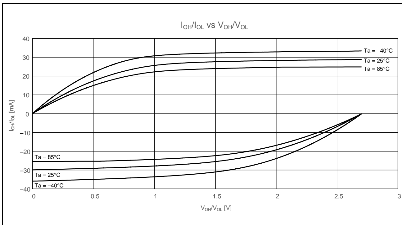
図 51.14 高駆動出力を選択したときの V_{OH}/V_{OL} 、 I_{OH}/I_{OL} 温度特性 VCC = 2.7V (参考データ)
