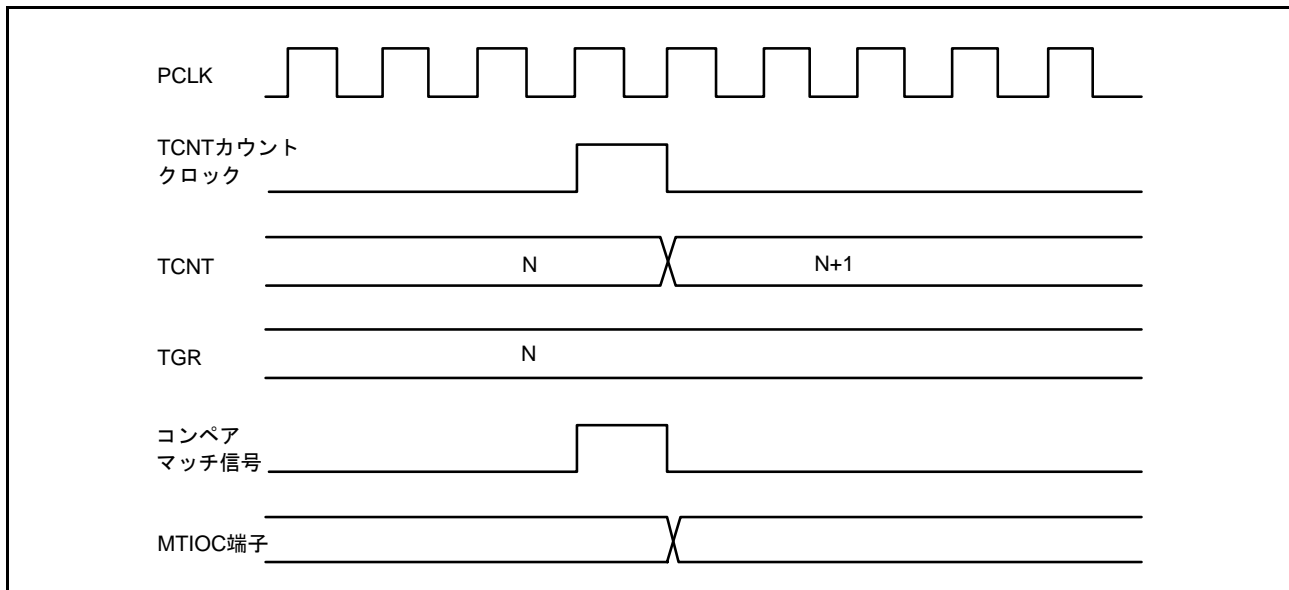
図 23.81 アウトプットコンペア出力タイミング（ノーマルモード、PWM モード）
