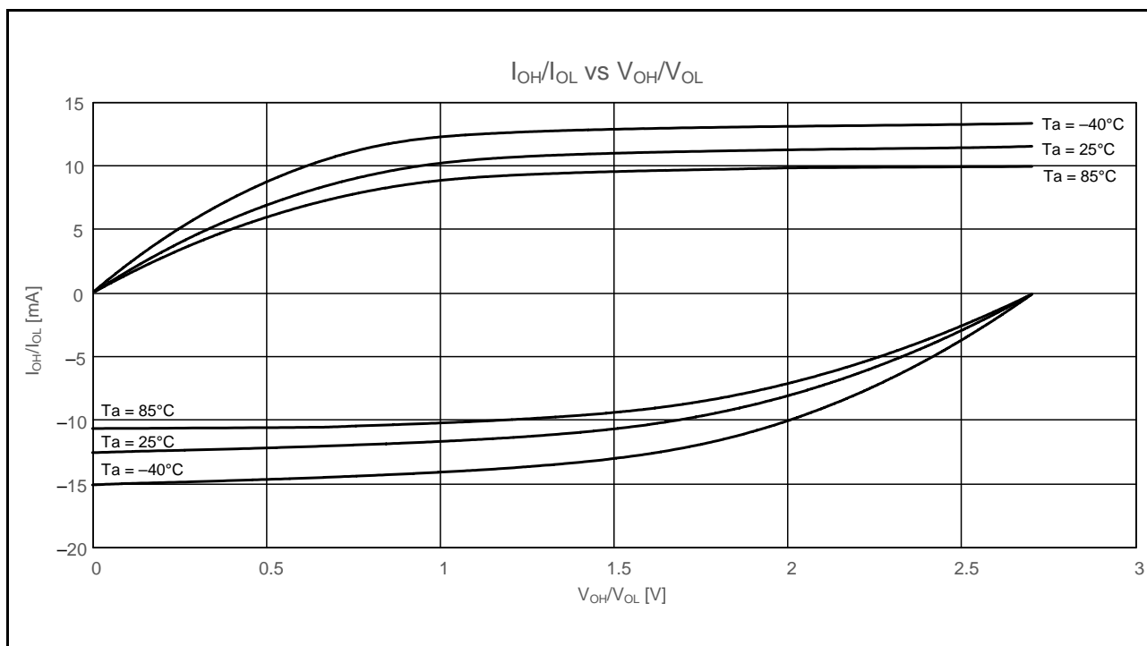
図 51.10 通常出力を選択したときの V_{OH}/V_{OL} 、 I_{OH}/I_{OL} 温度特性 V_{CC} = 2.7V (参考データ)
