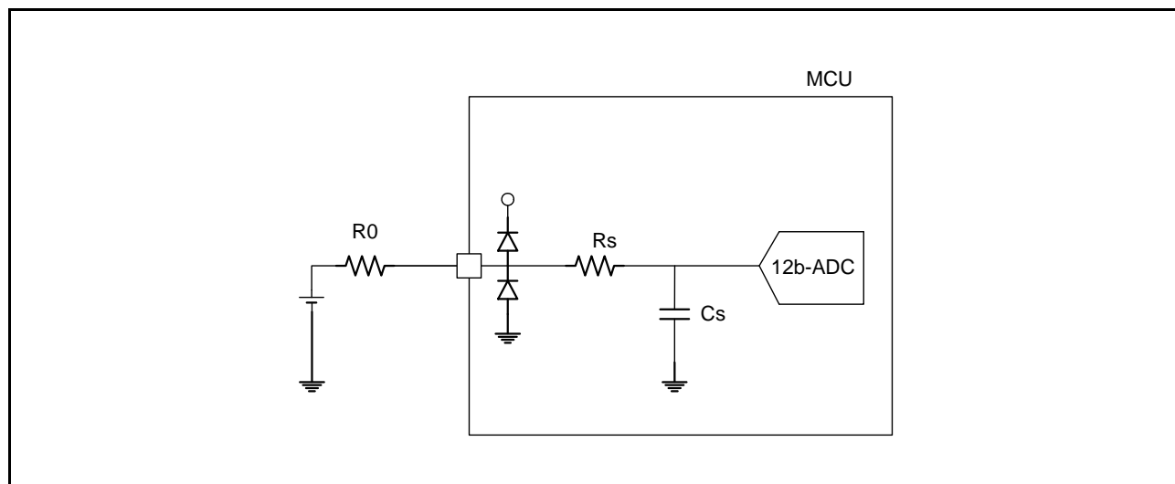
図 51.64 等価回路
