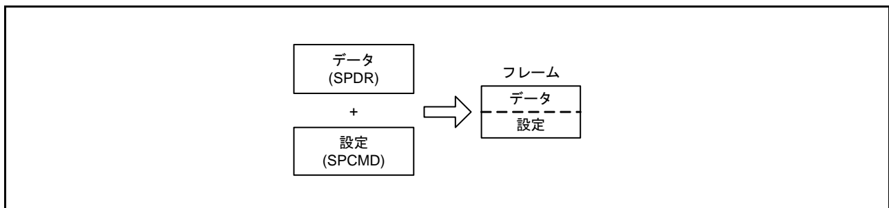
図 38.44 フレーム概念図
