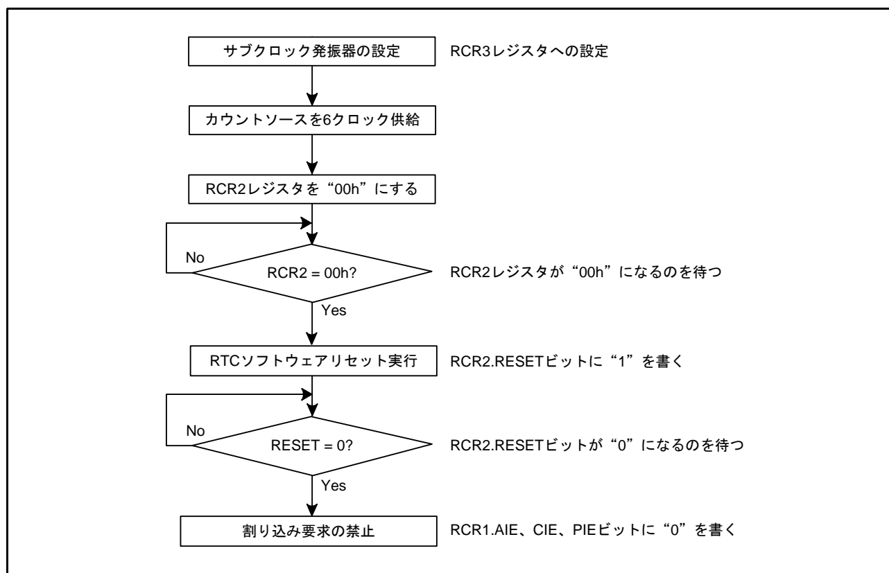
図 28.14 初期化手順
