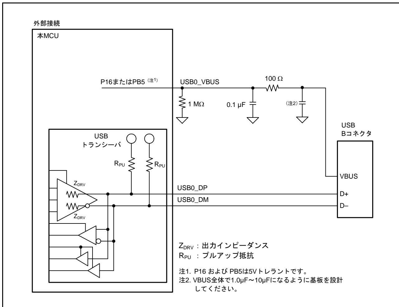
図 32.3 セルフパワー時の USB コネクタのファンクション接続例
