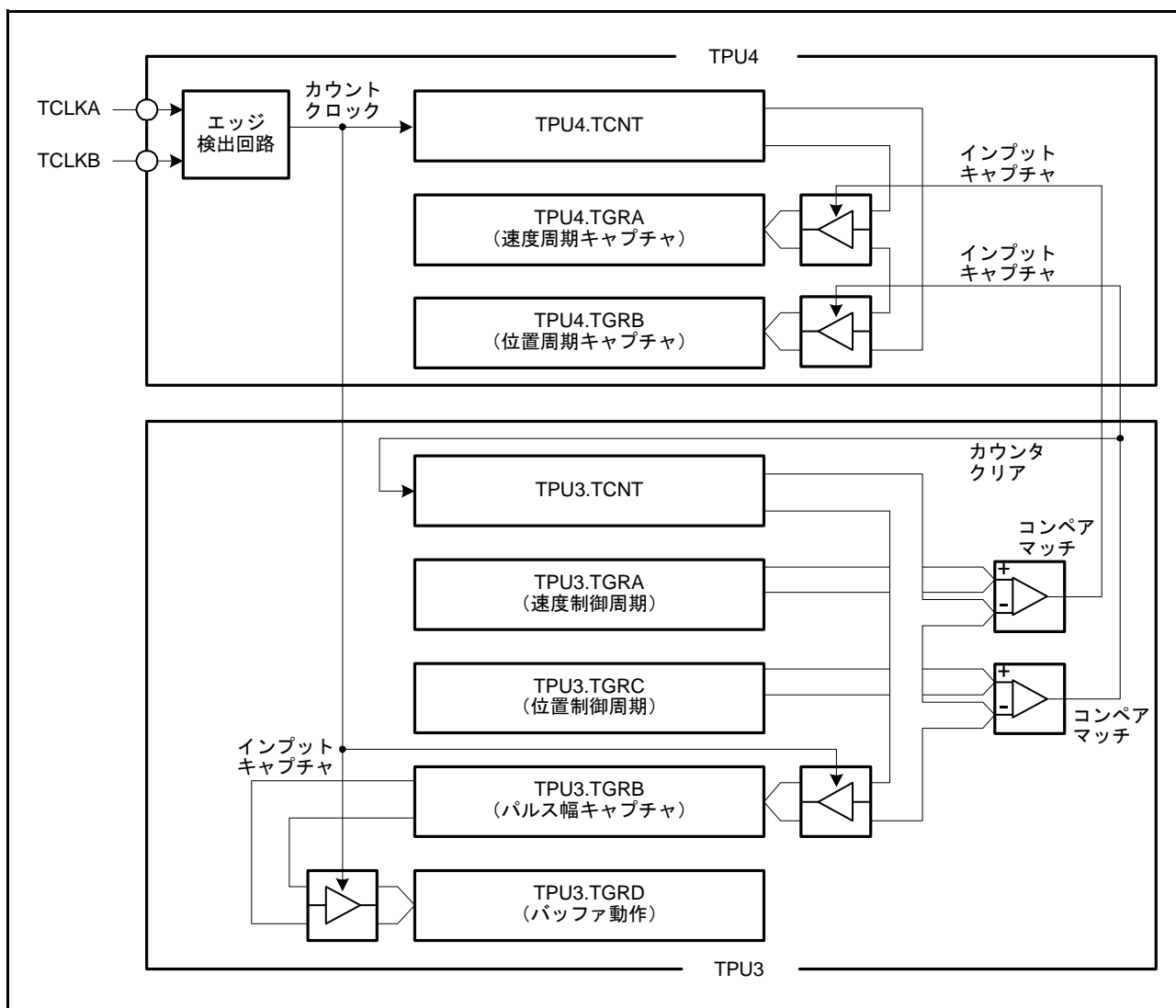
図 25.29 位相計数モードの応用例
