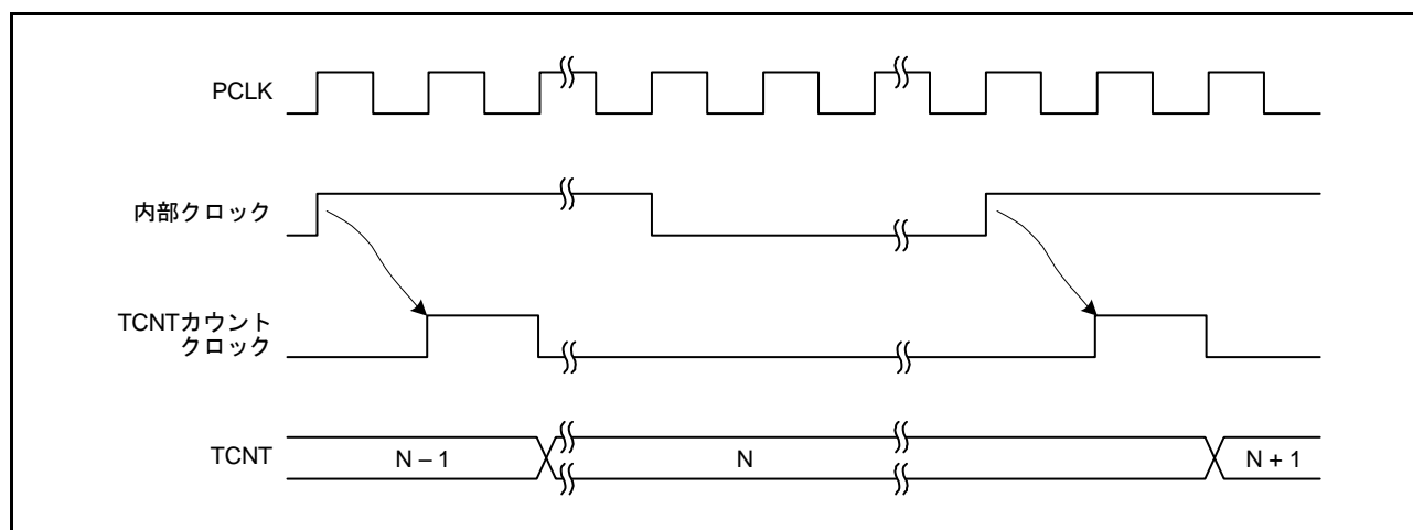
図 26.5 内部クロック動作時のカウントタイミング
