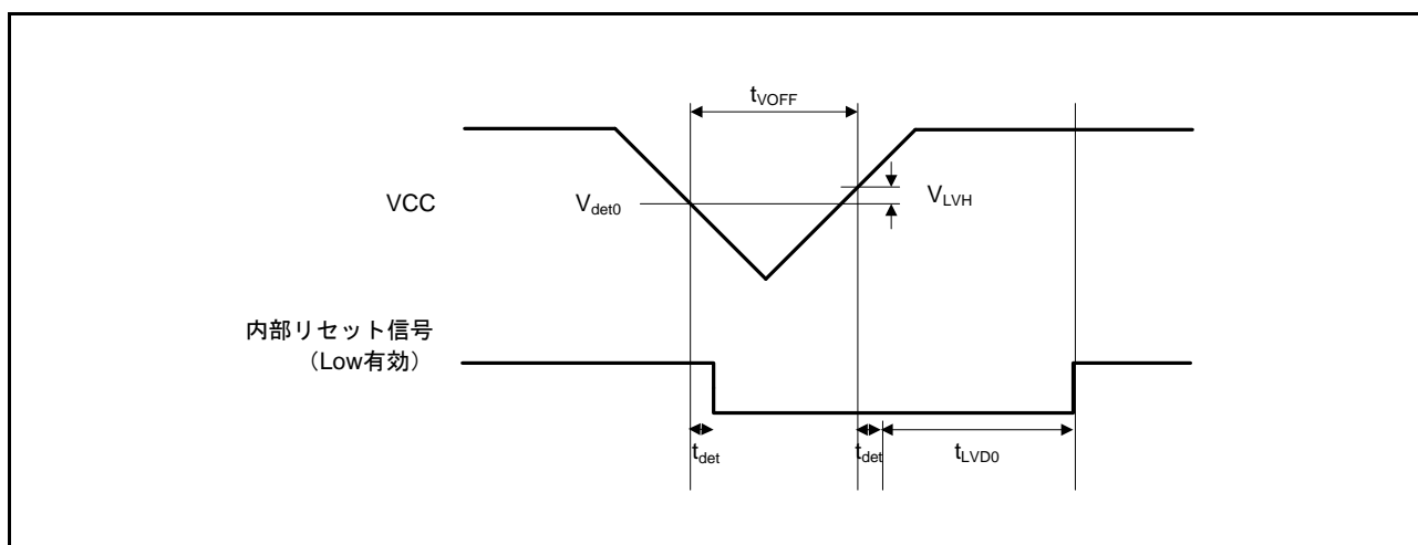
図 51.71 電圧検出回路タイミング (Vdet0)
