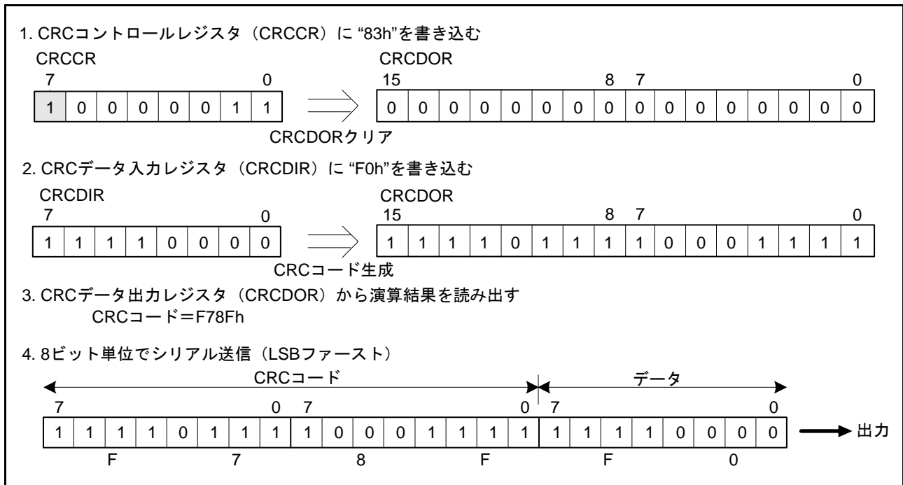
図 39.2 LSBファーストでのデータ送信
