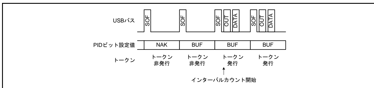
図 32.13 IITV[2:0] = 000b の場合のトークン発行有無
