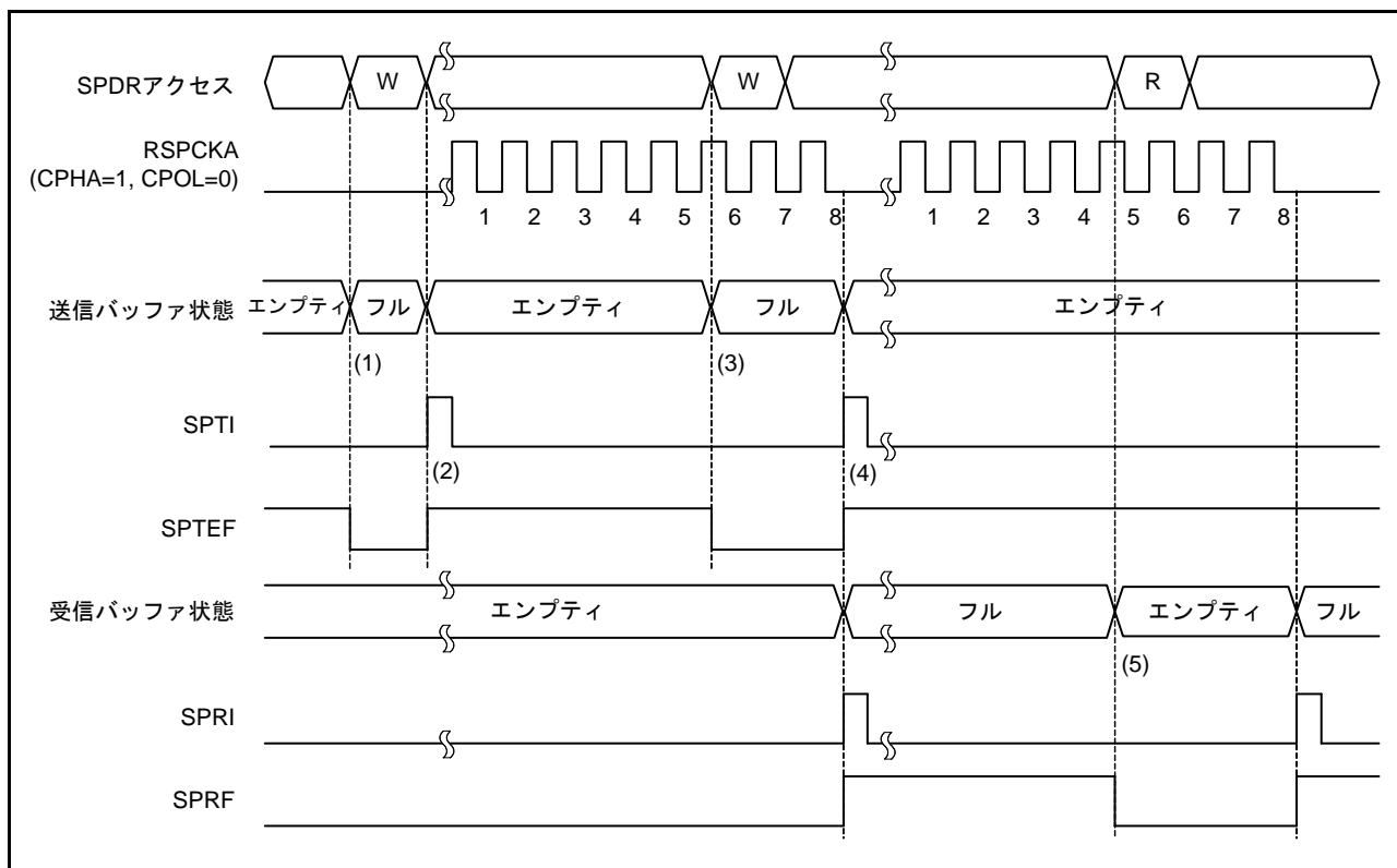
図 38.26 SPTI、SPRI 割り込みの動作例
