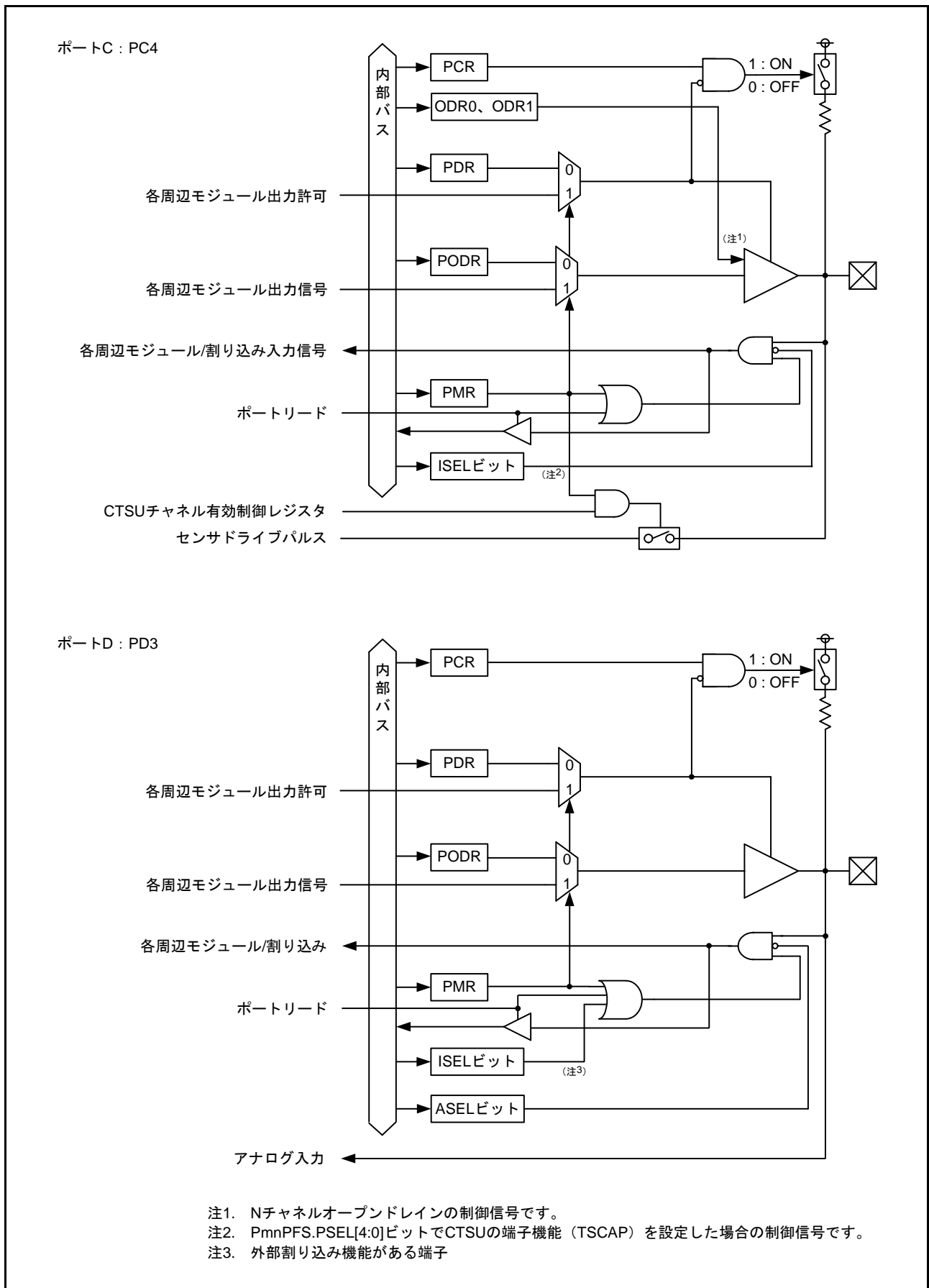
図 21.8 入出力ポートの構成 (8)
