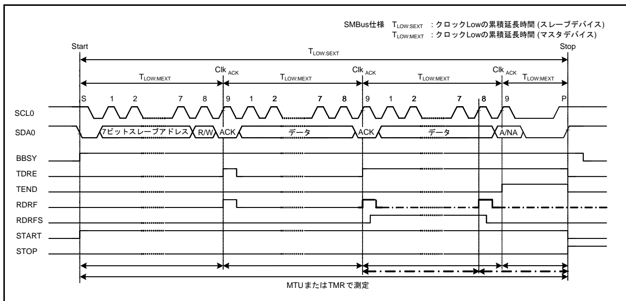
図 35.41 SMBus タイムアウト測定
