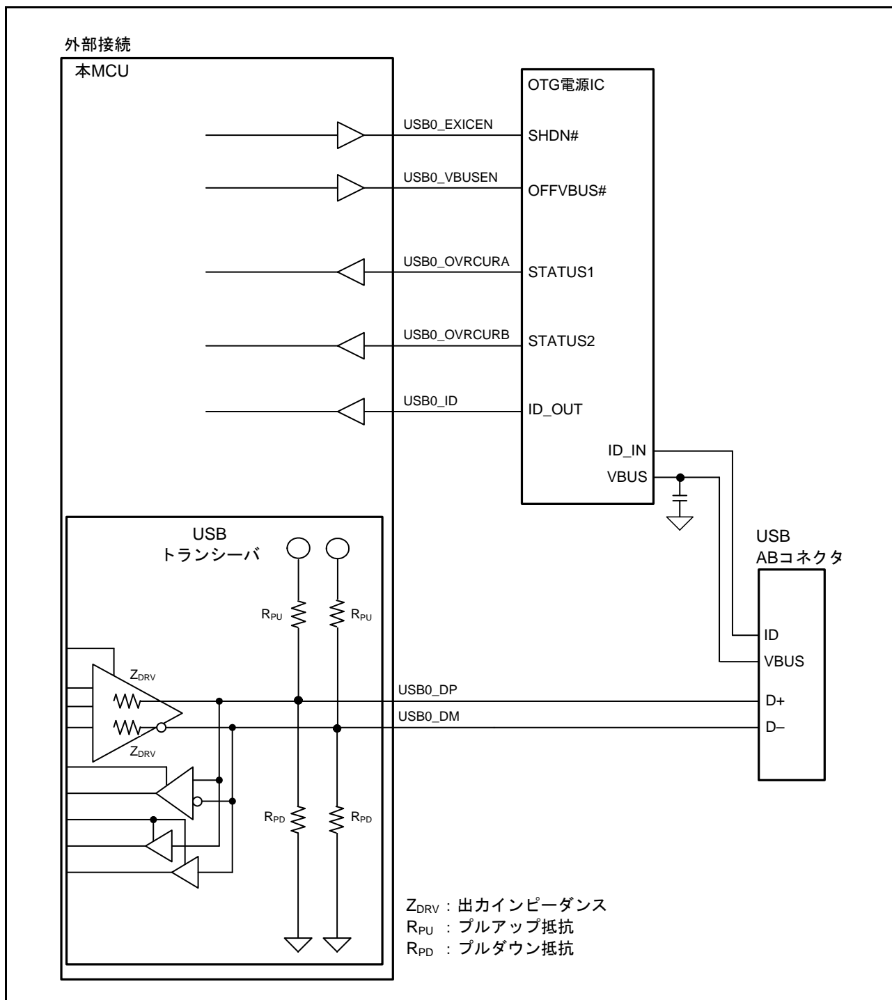
図 32.2 セルフパワー時の USB コネクタの OTG 接続例
