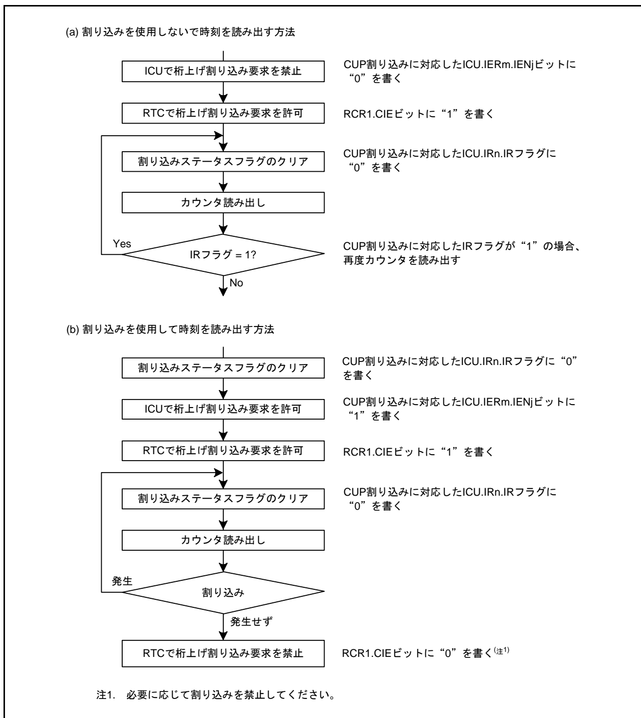
図 28.6 時刻読み出し手順
