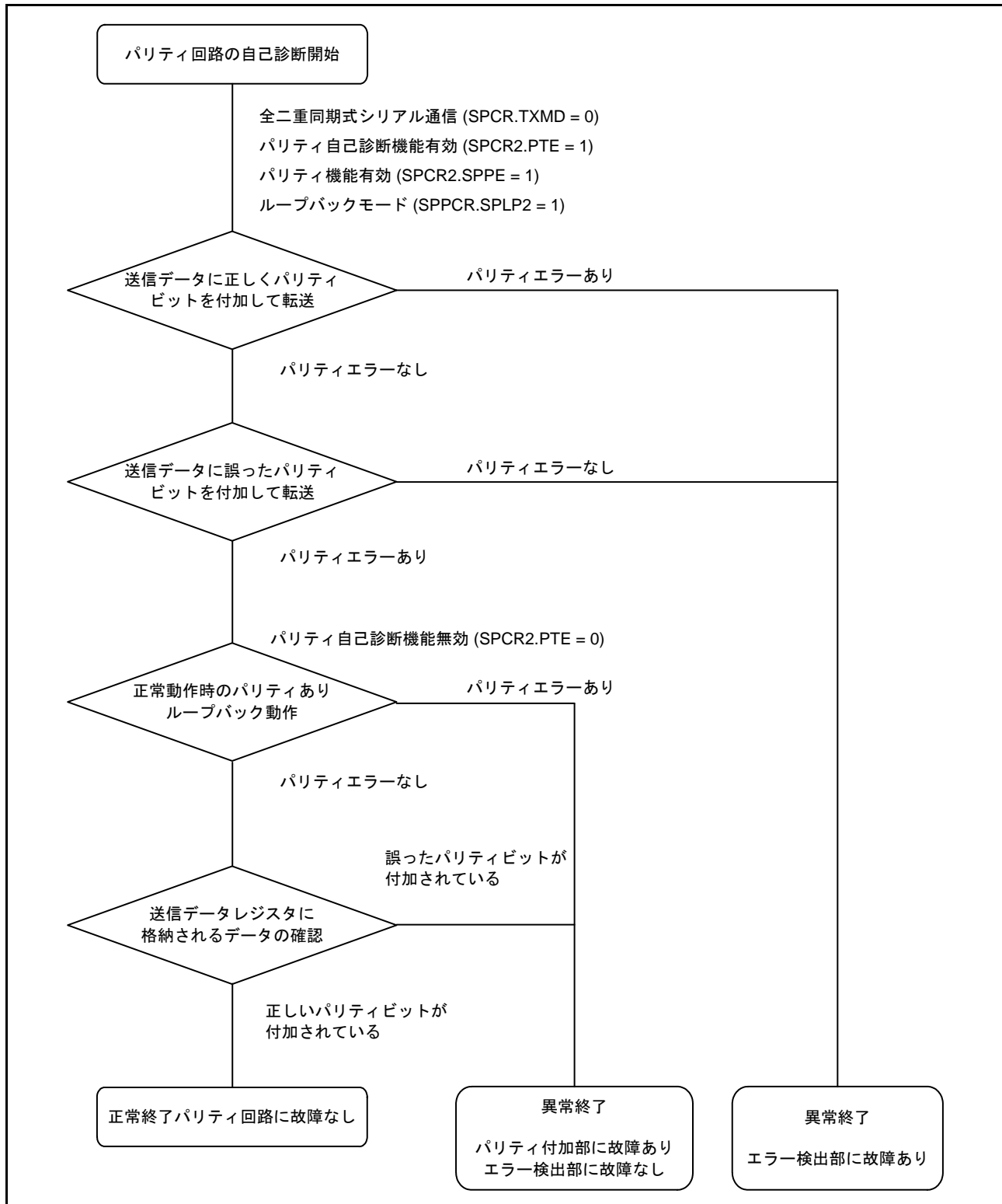
図 38.49 パリティ回路の自己判断フロー
