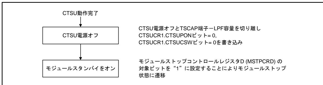
図 43.10 CTSUS 停止フロー
