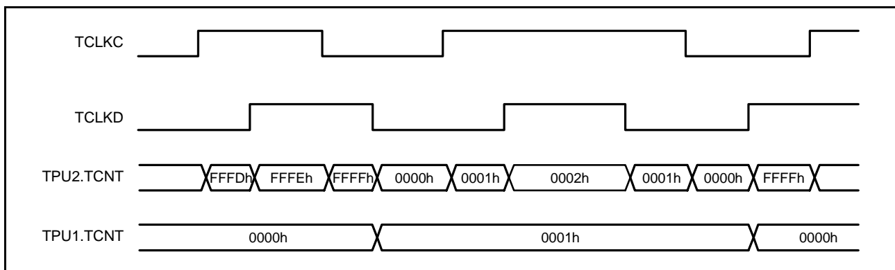
図 25.19 カスケード接続動作例 (2)
