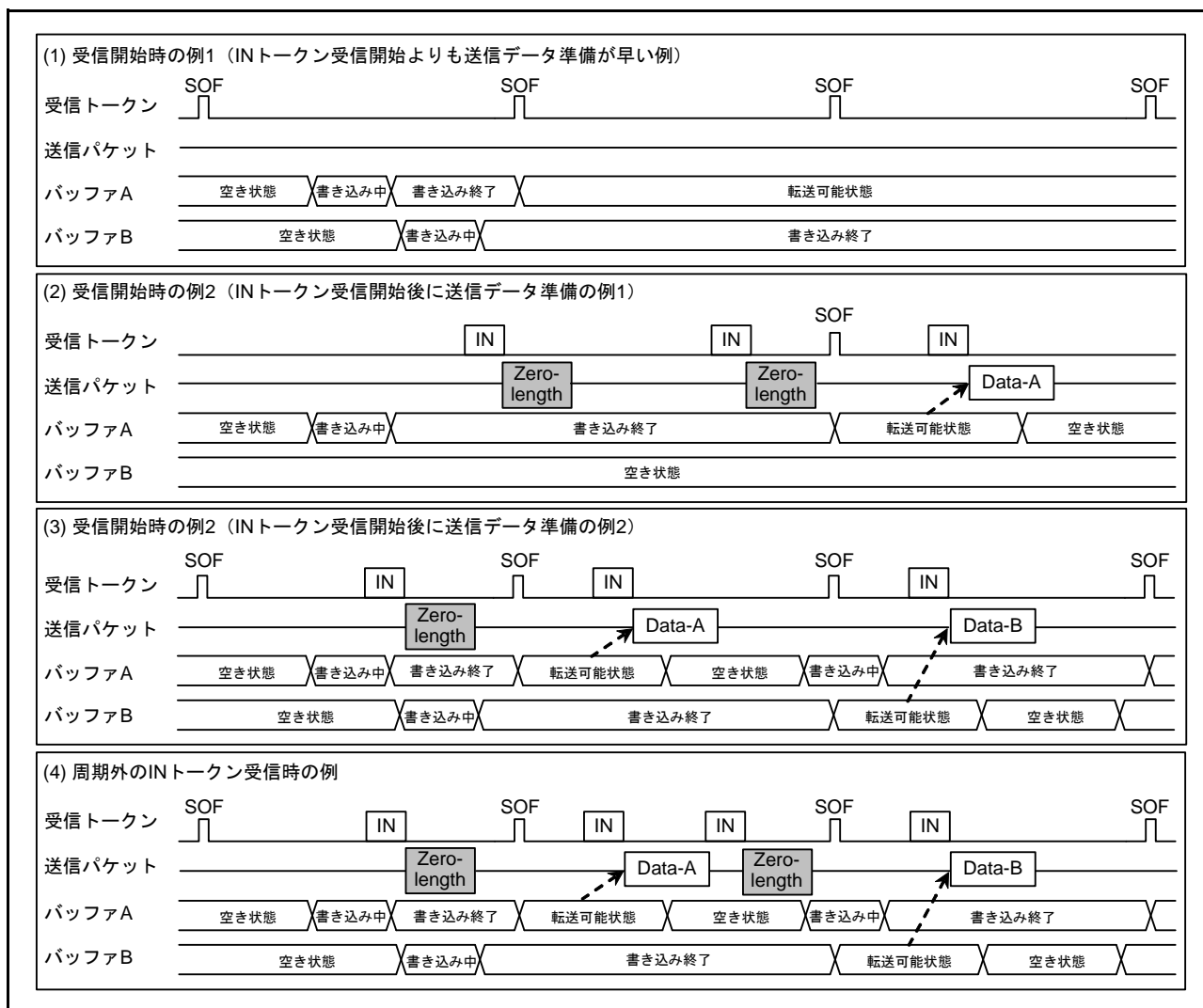
図 32.17 データセットアップ機能動作例
