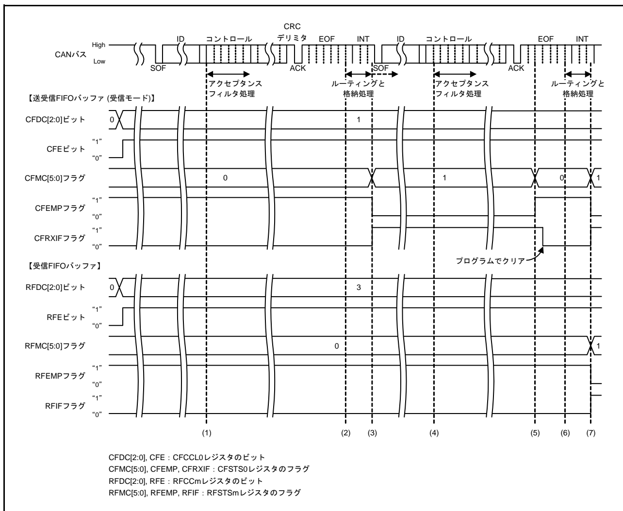
図 36.25 FIFO バッファの受信タイミング図
