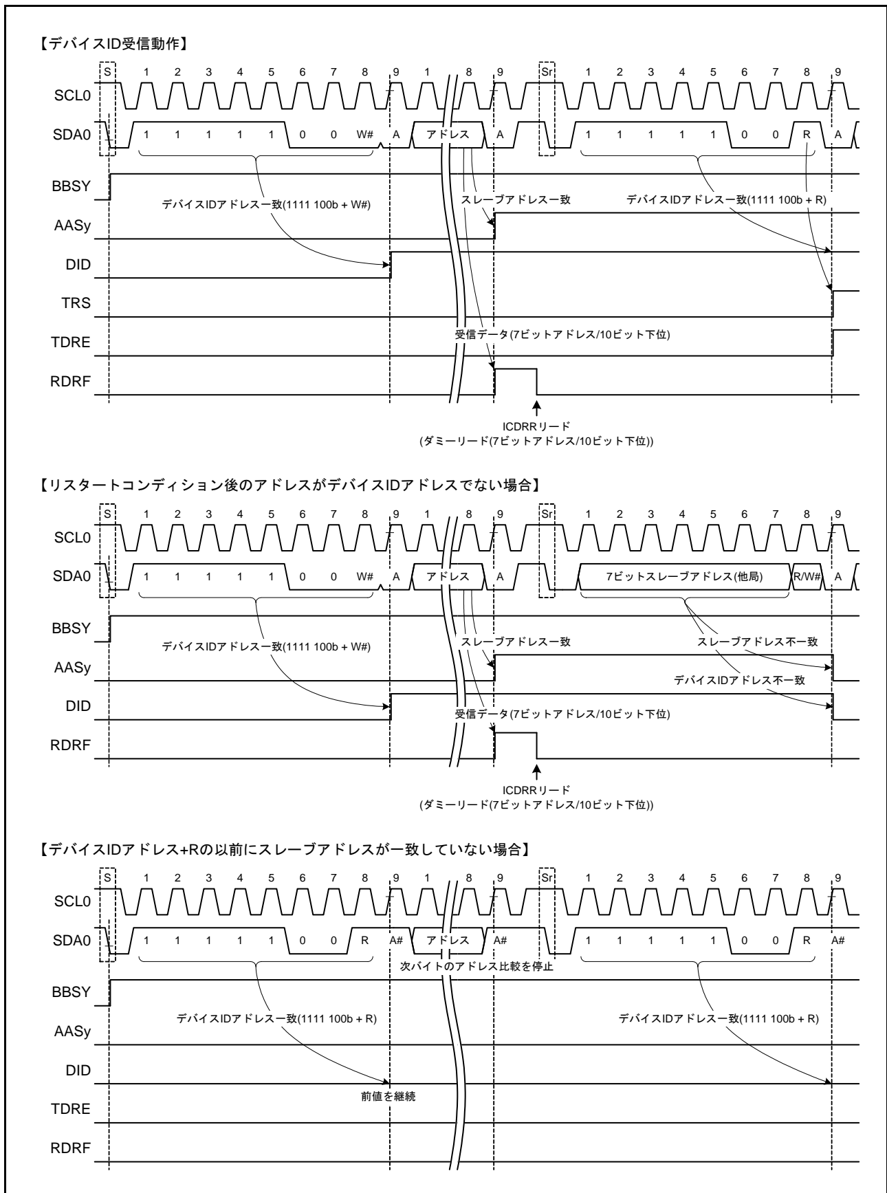
図 35.28 デバイス ID アドレス受信時の AASy、DID フラグセット/クリアタイミング
