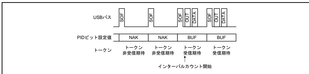
図 32.15 IITV[2:0] = 000b の場合のフレームとトークン受信期待有無の関係
