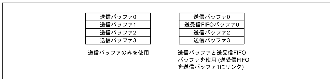
図 36.7 送受信 FIFO バッファのリンク
