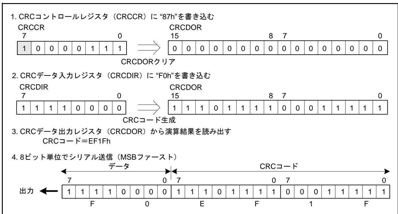
図 39.3 MSBファーストでのデータ送信
