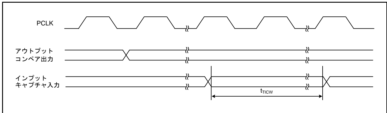
図 51.35 MTU入出力タイミング
