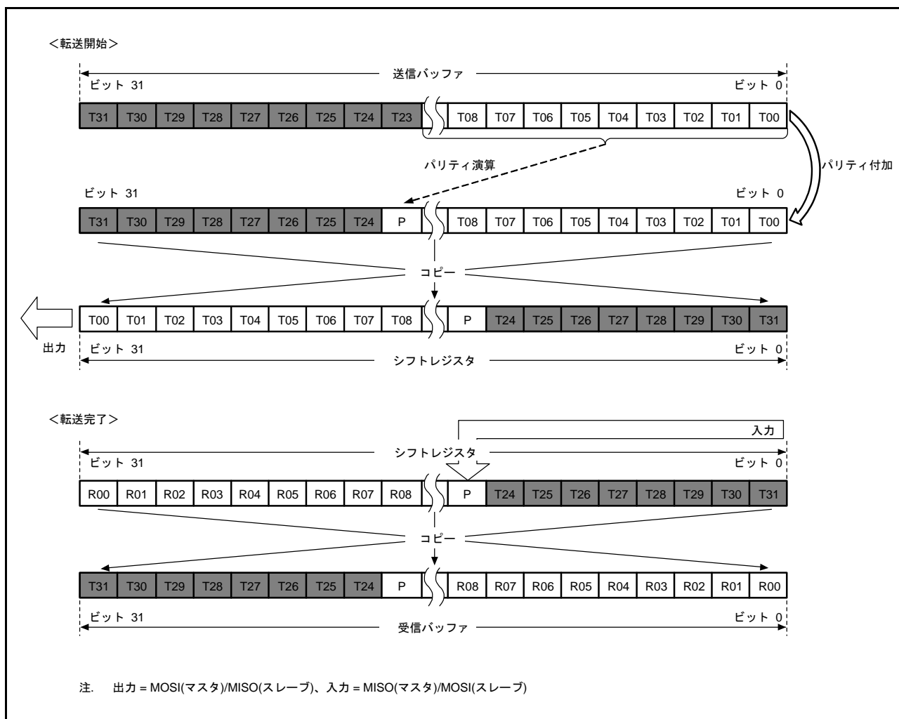
図 38.21 LSB ファースト (24 ビットデータ / パリティ機能有効)
