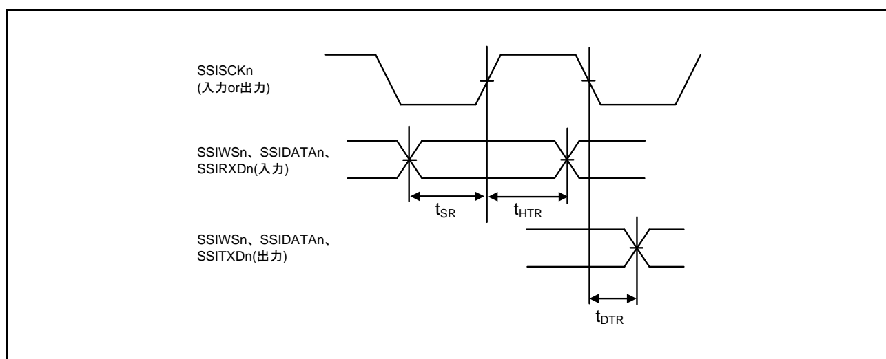
図 51.54 SSI 送受信タイミング (SSICR.SCKP=0)
