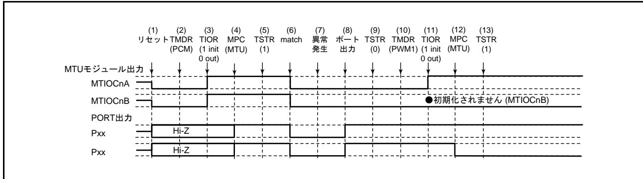
図 23.133 位相計数モードで異常が発生し、PWM モード1で復帰する場合
