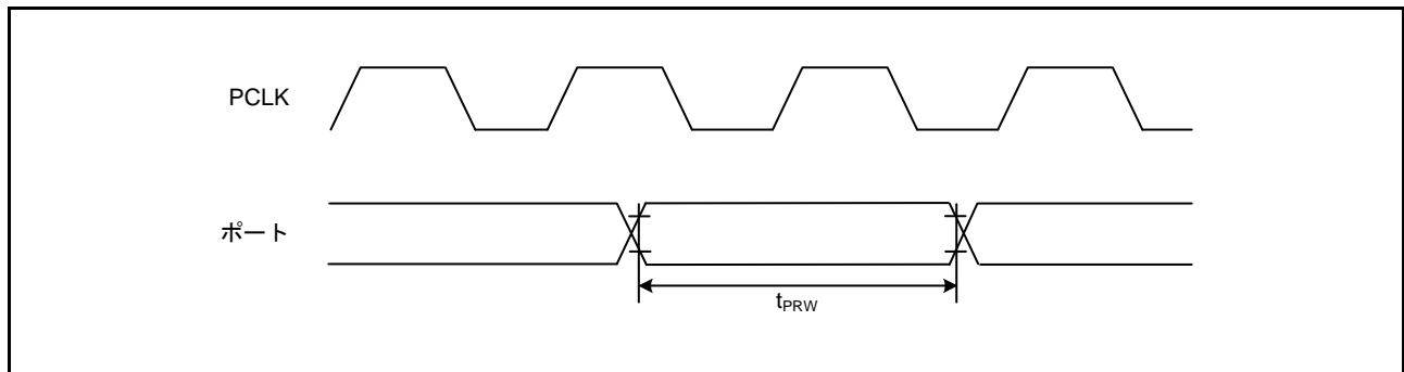
図 51.34 I/Oポート入力タイミング
