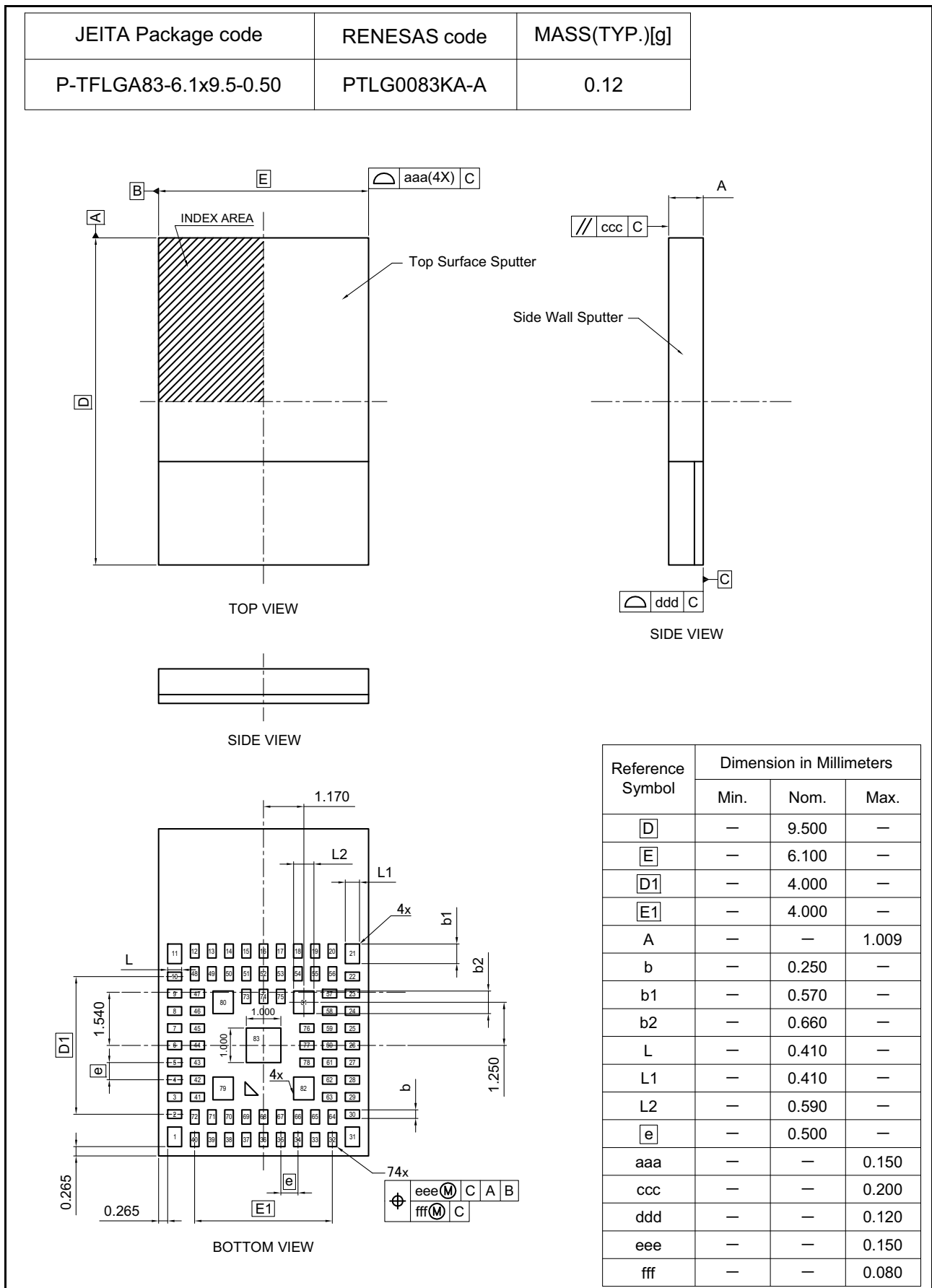
図 B. 83 ピン LGA (PTLG0083KA-A)
