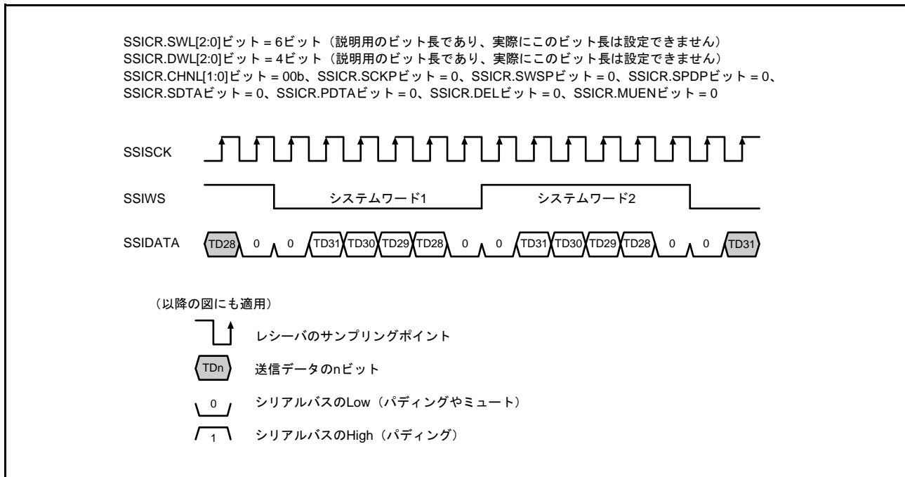
図 37.6 基本フォーマット例 (送信モード)
