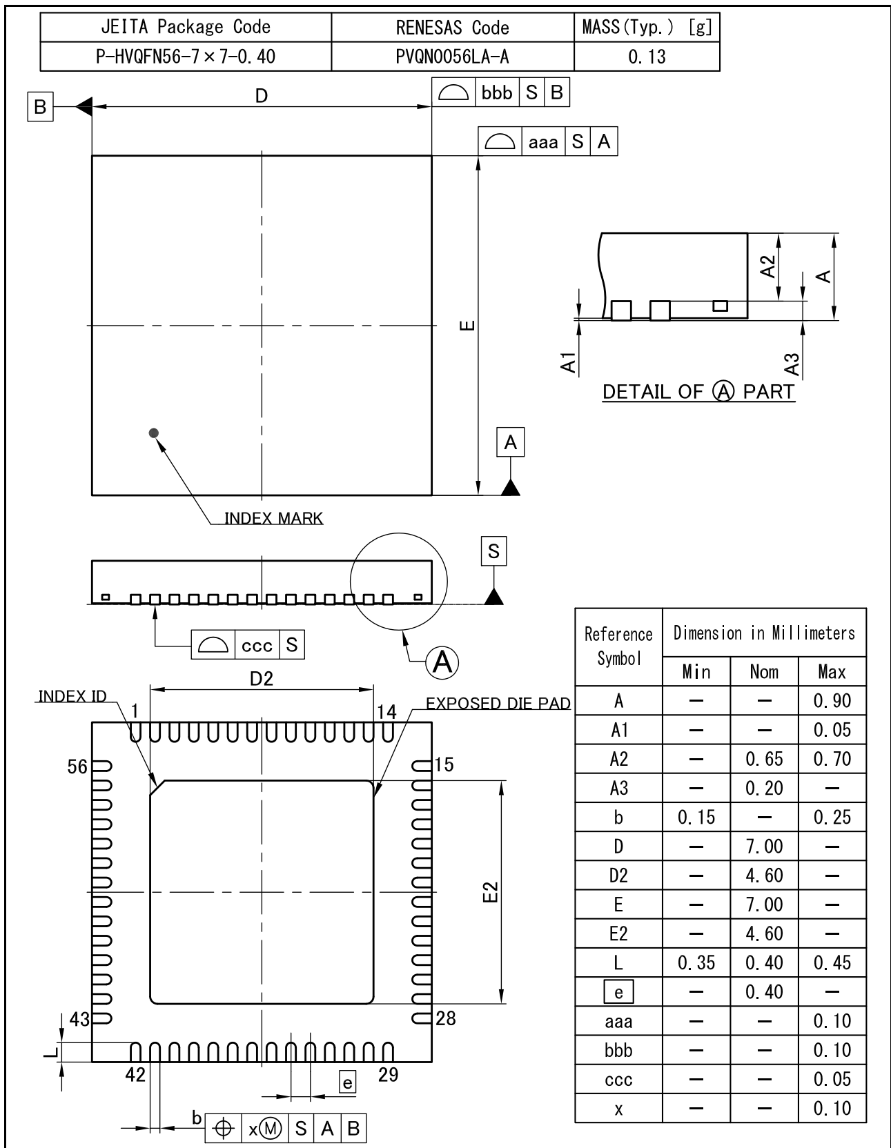
図 C. 56ピンQFN (PVQN0056LA-A)
