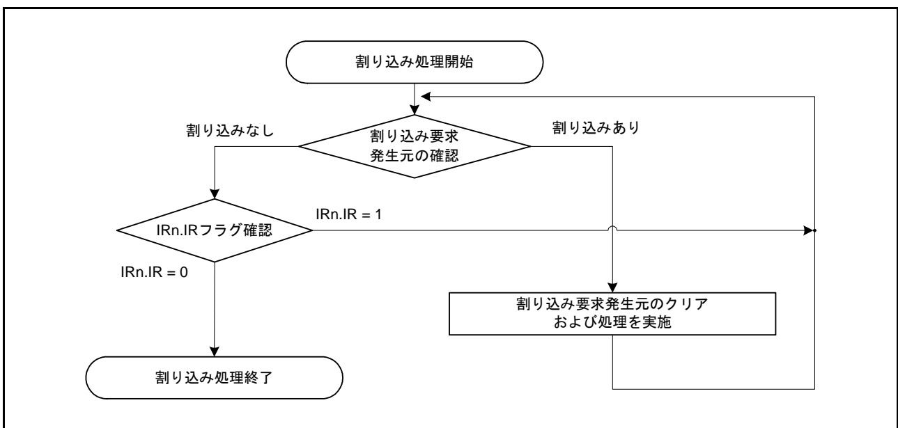
図 15.7 レベル検出割り込み処理手順
