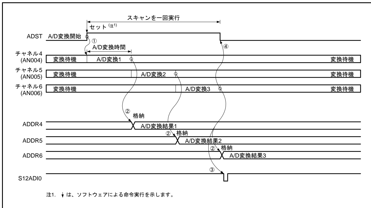
図 44.5 シングルスキャンモードの動作例 (基本動作 : AN004、AN005、AN006 選択)
