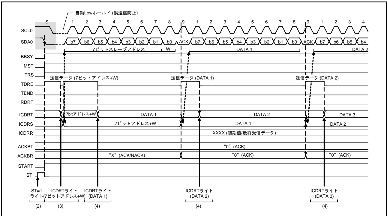
図 35.7 マスタ送信の動作タイミング (1) (7ビットアドレスフォーマットの時)
