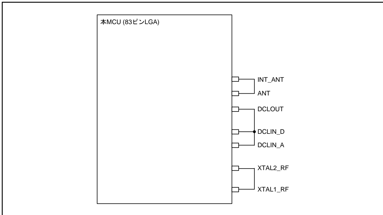
図 41.2 外部接続回路例 (83 ピン LGA)
