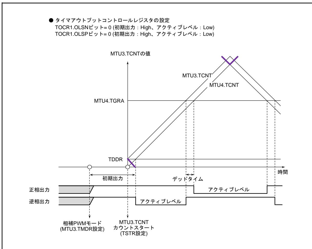
図 23.44 相補 PWM モードの初期出力例 (1)
