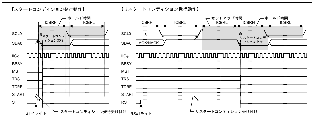
図 35.37 スタートコンディション/リスタートコンディション発行動作タイミング (ST、RS ビット)
