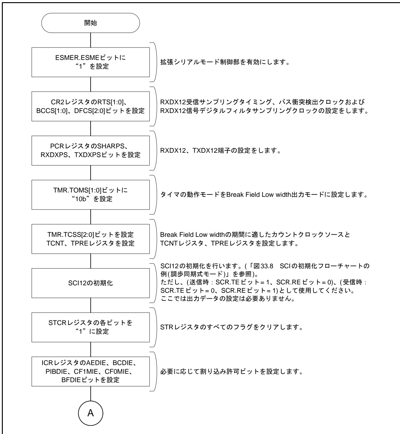
図 33.62 Start Frame 送信フローチャート例 (1)
