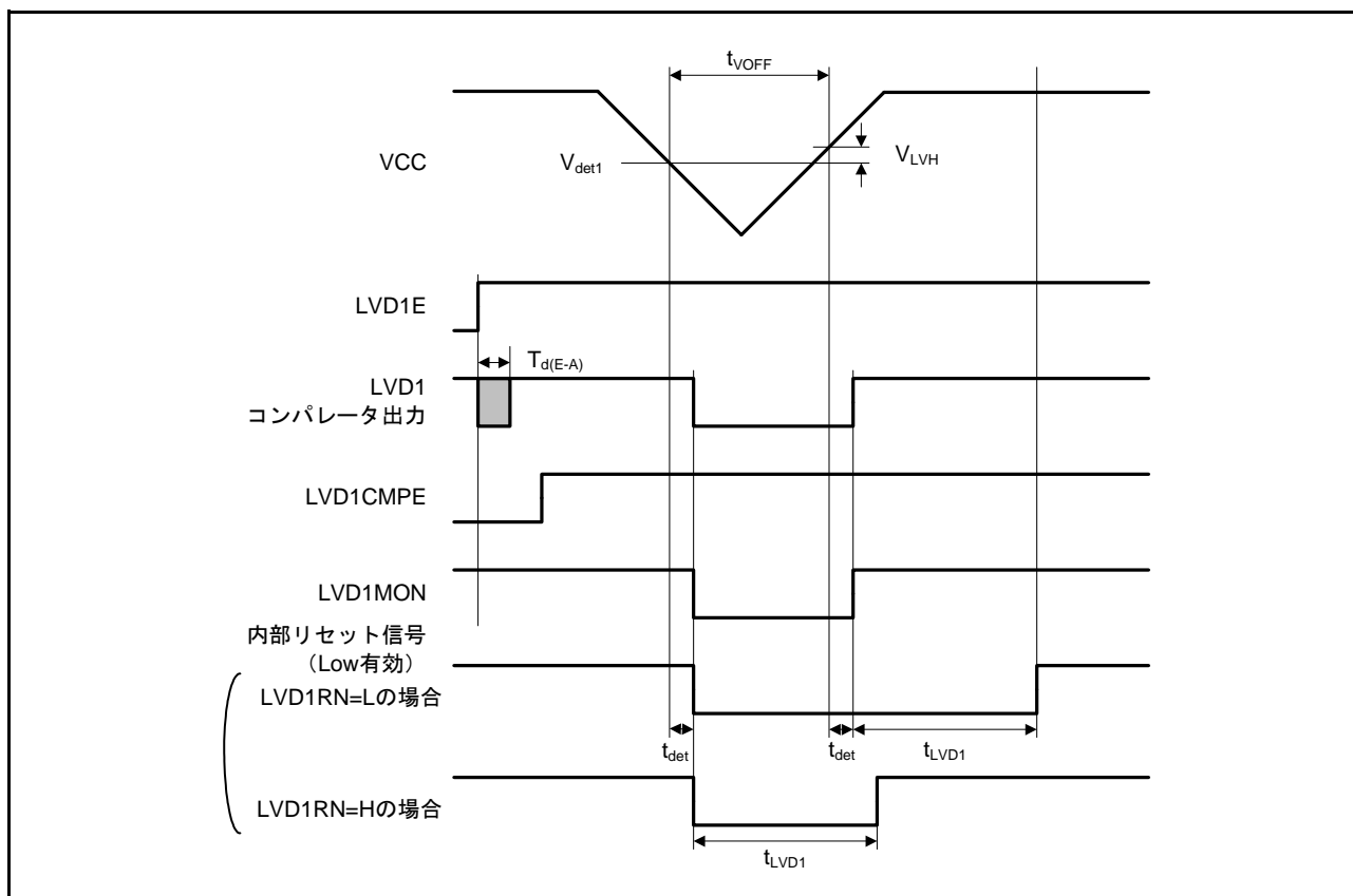
図 51.72 電圧検出回路タイミング ( V_{det1} )
