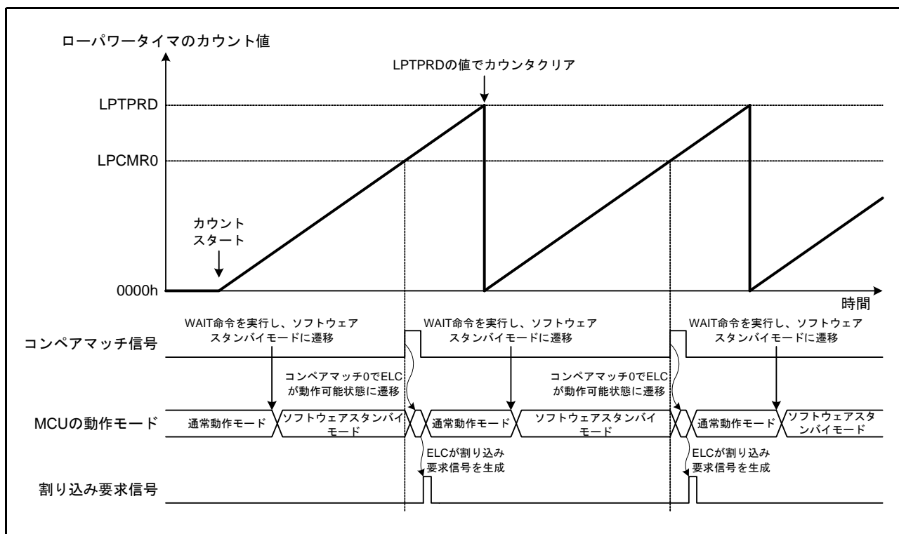
図 29.2 ローパワータイマの動作
