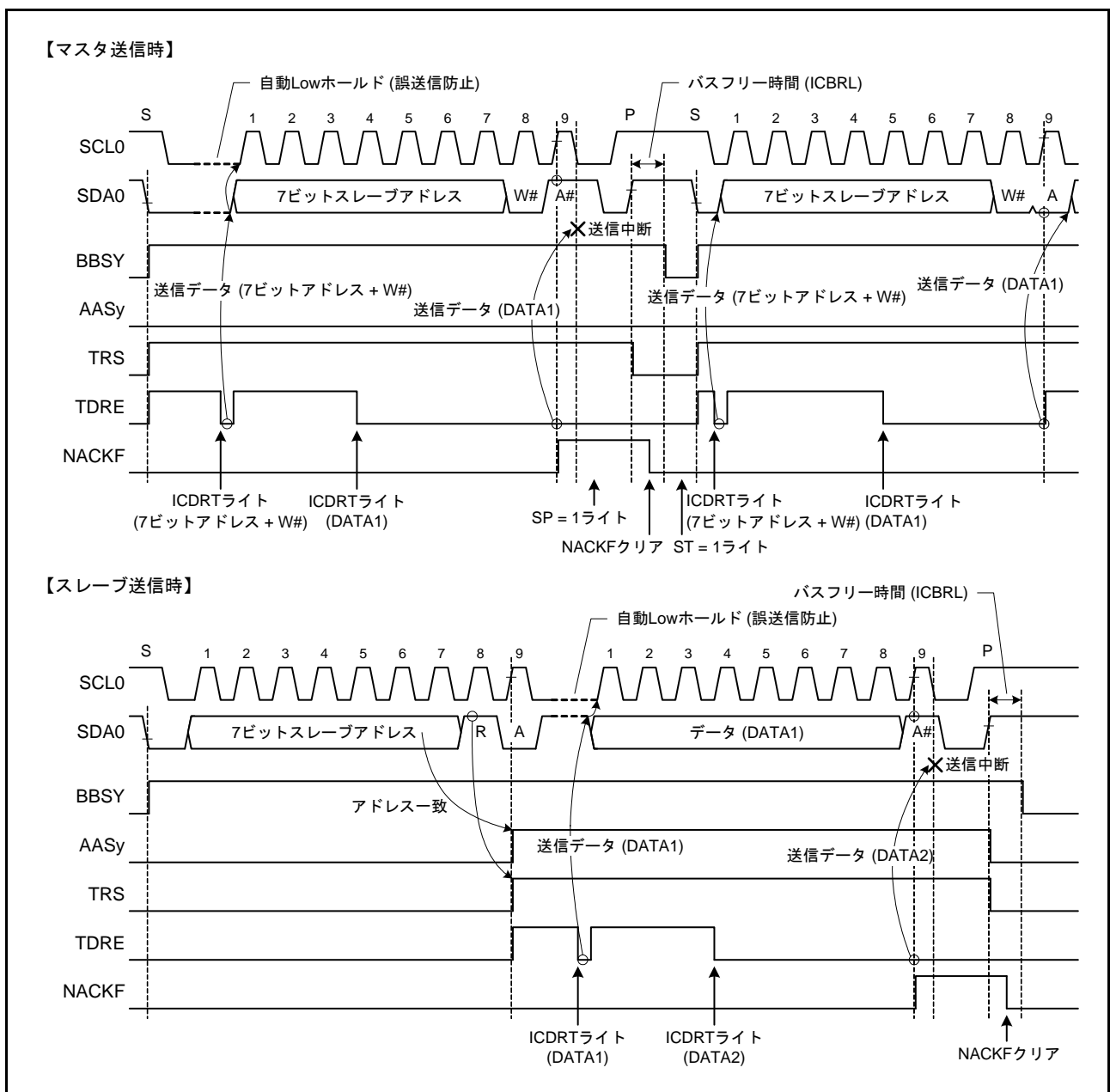
図 35.31 NACK 受信時の転送中断動作 (NACKF ビット = 1 のとき)
