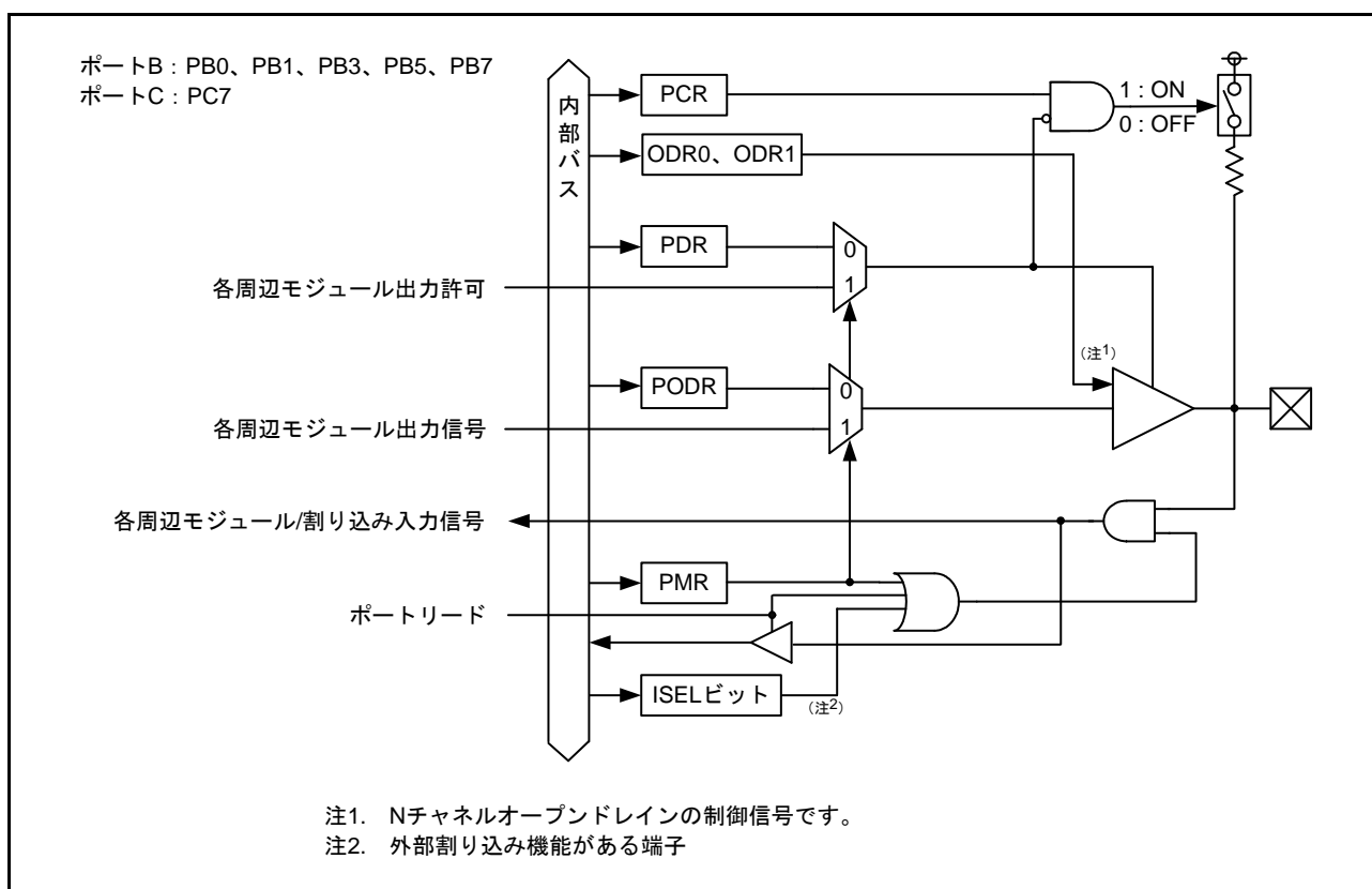
図 21.7 入出力ポートの構成 (7)
