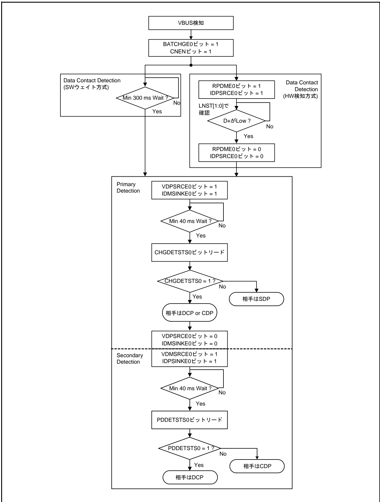
図 32.20 Portable Device としての処理フロー
