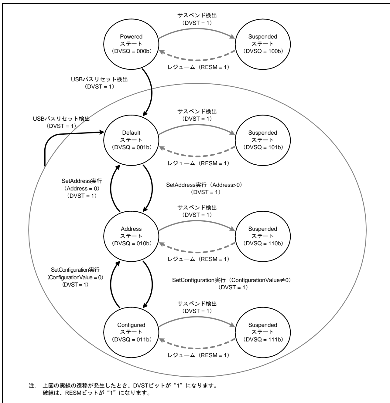
図 32.11 デバイスステート遷移図
