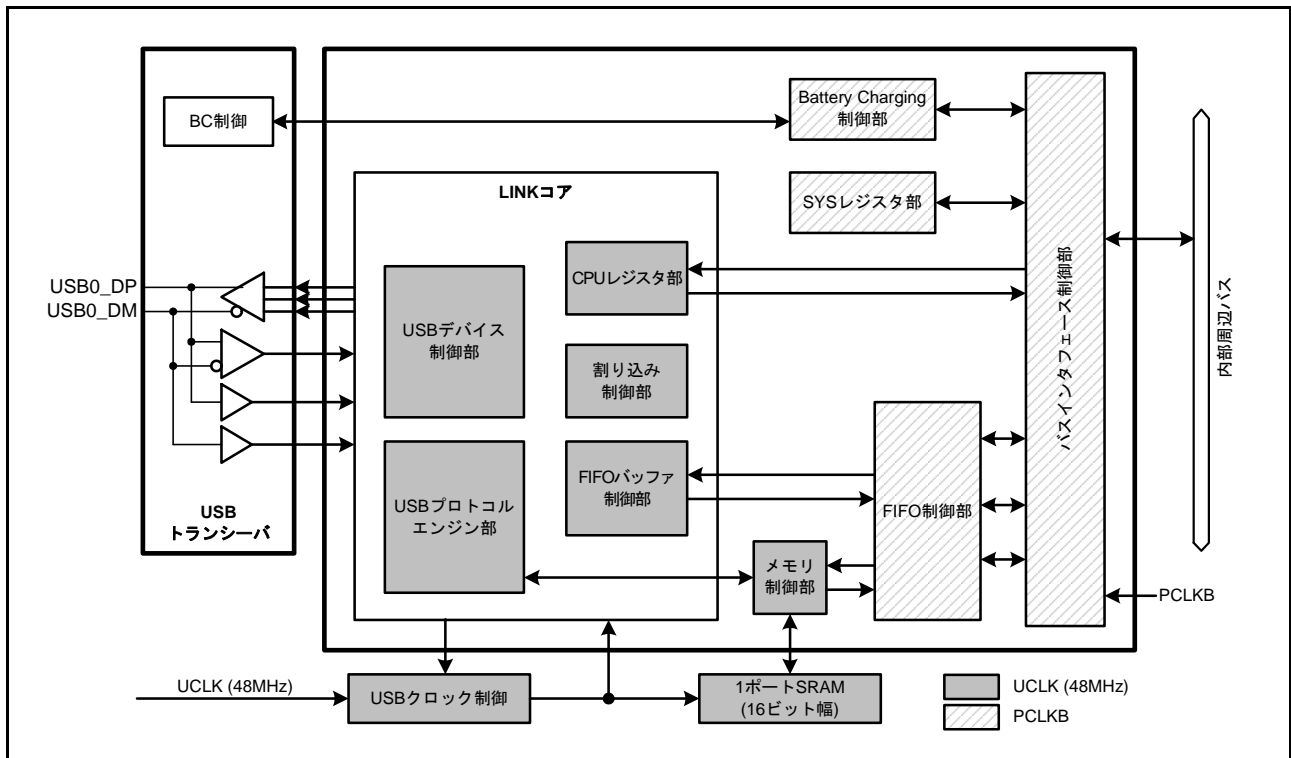
図 32.1 USB のブロック図
