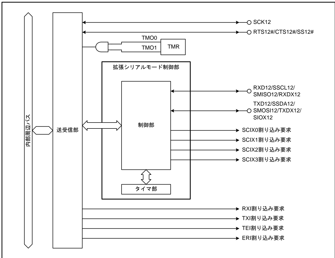
図 33.3 SCIH (SCI12) のブロック図
