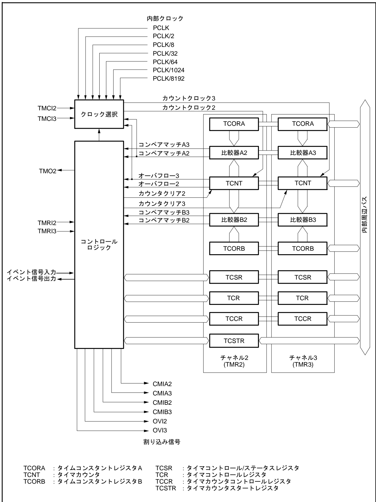
図 26.2 TMR (ユニット1) のブロック図
