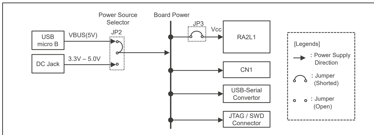
図 4 電源系統図
