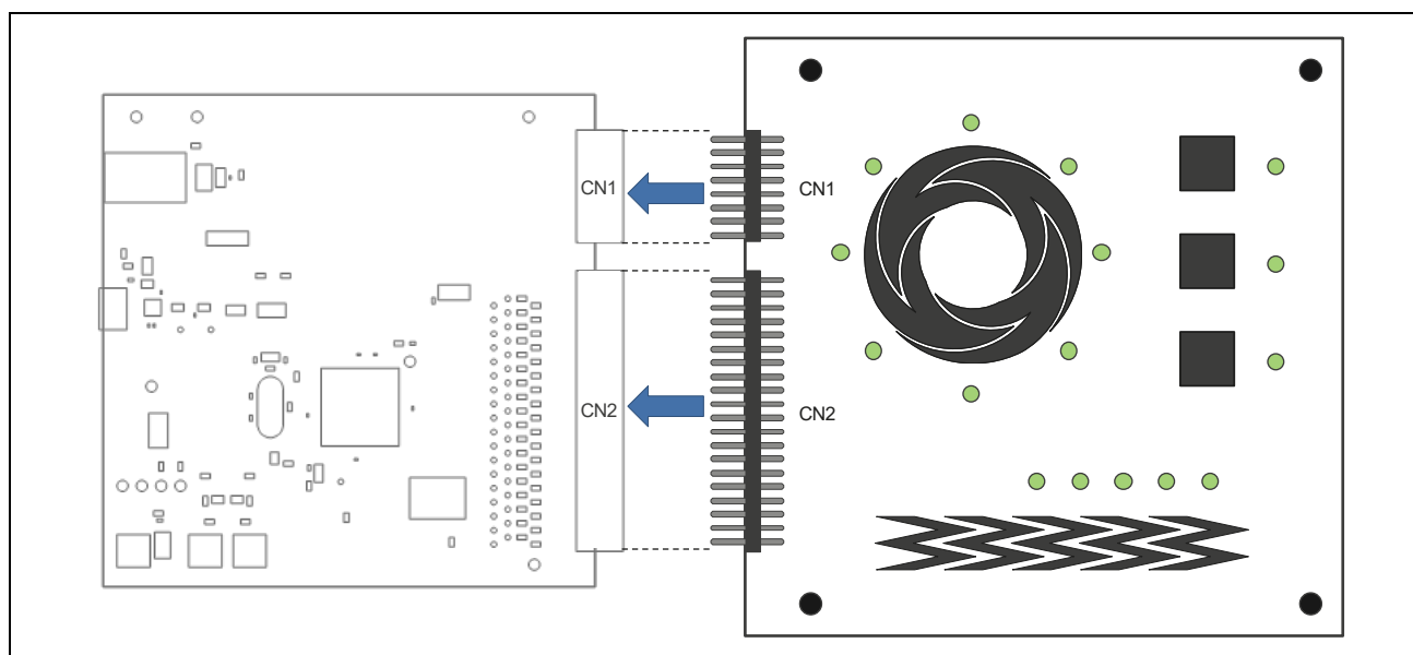
図 7 RA2L1 Cap Touch CPU ボードと静電容量タッチアプリケーションボードの接続方法
