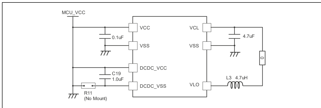
図 6 内部電圧レギュレータ回路
