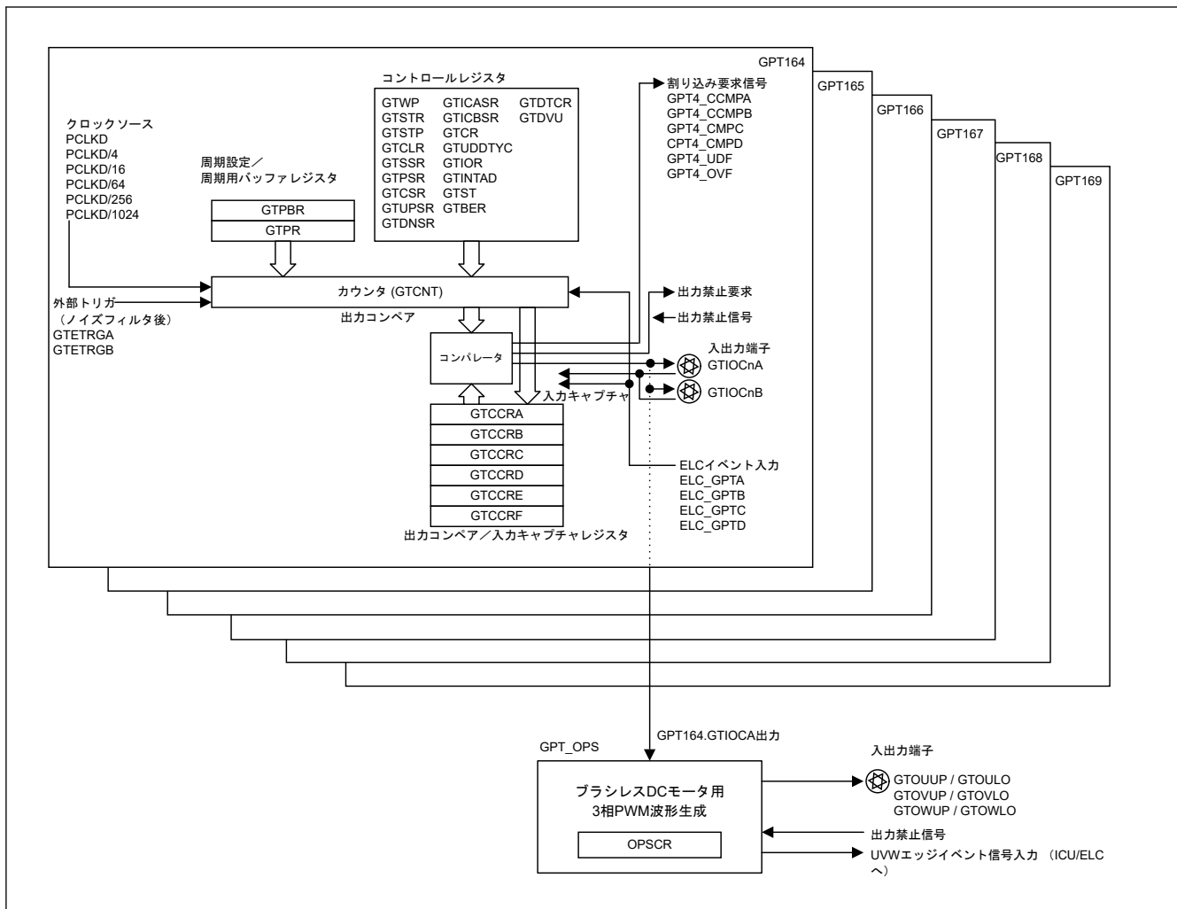
図 20.1 GPT のブロック図
