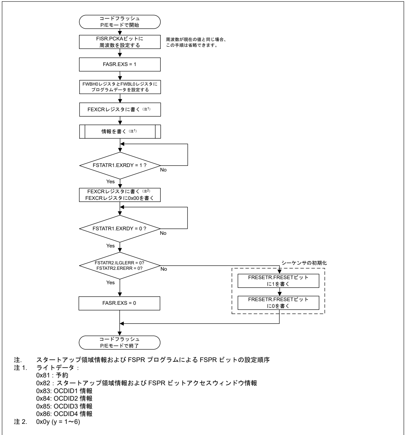
図 32.29 スタートアップ領域情報および FSPR プログラム/アクセスウィンドウ情報プログラム/OCDID 情報プログラムの手順を示す簡易フローチャート
