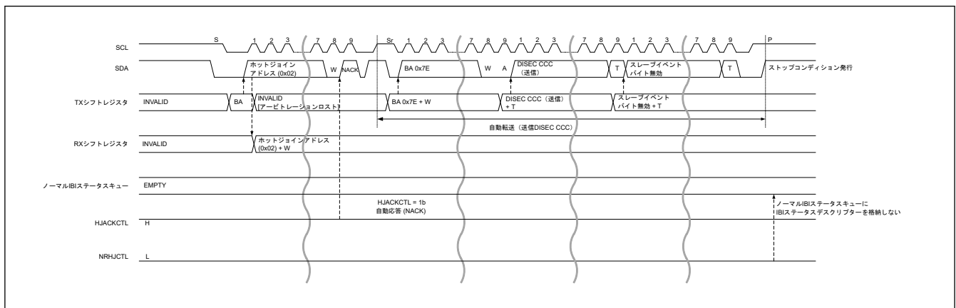
図 25.89 ホットジョインイベント : NACK (HJACKCTL が 1) かつ NRHJCTL が 0 の場合
