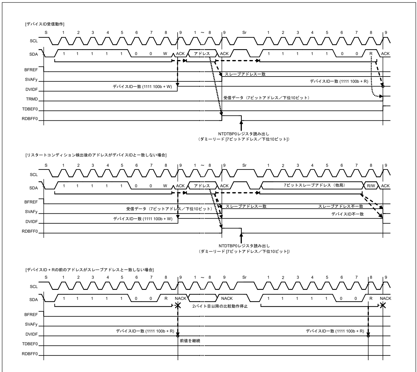
図 25.62 デバイス ID 受信時の SVAFy、DVIDF フラグのセット/クリアタイミング
