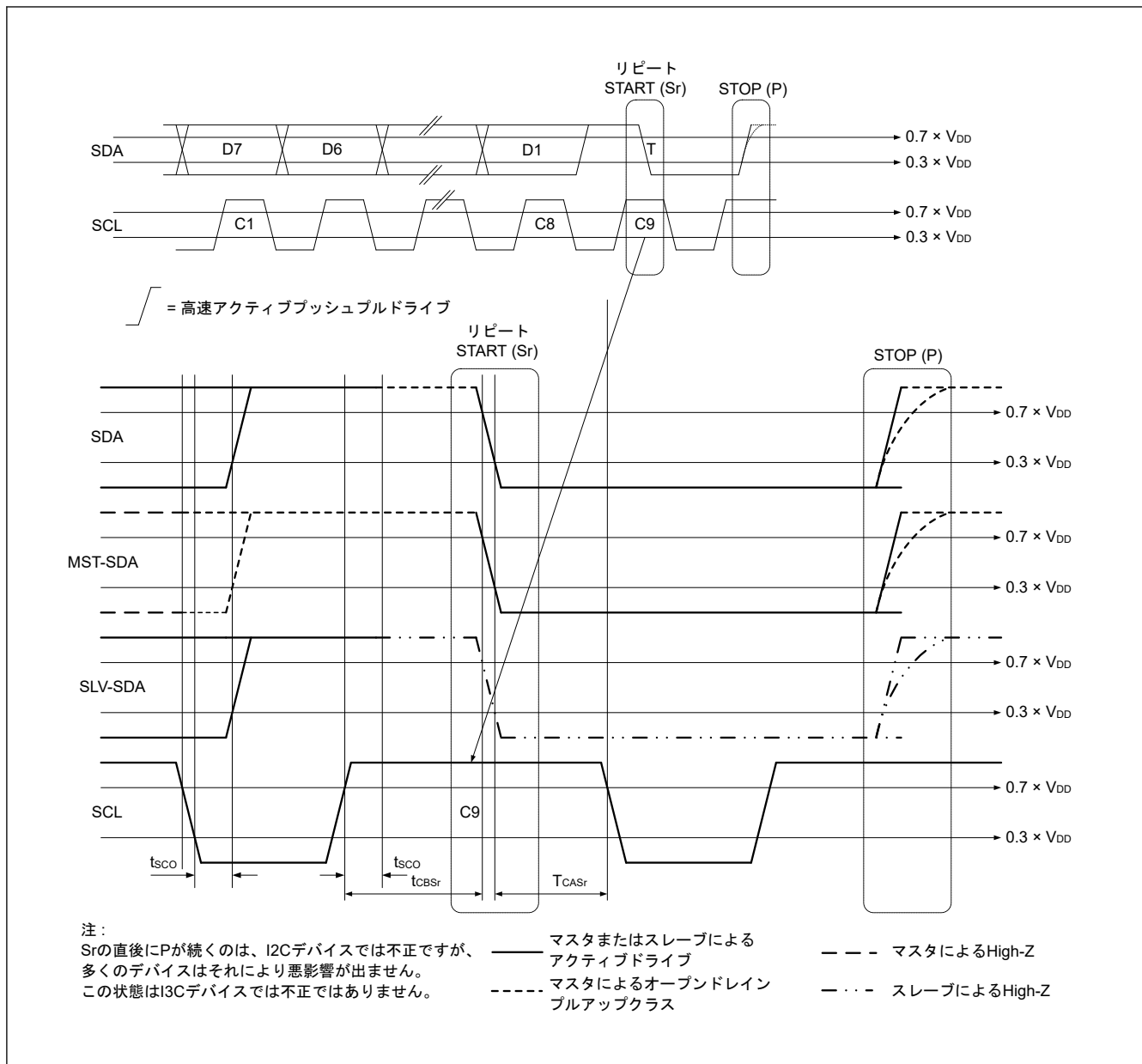
図 36.41 繰り返しのスタートコンディションおよびストップコンディションでのマスタ終了時のTビット読み出し
