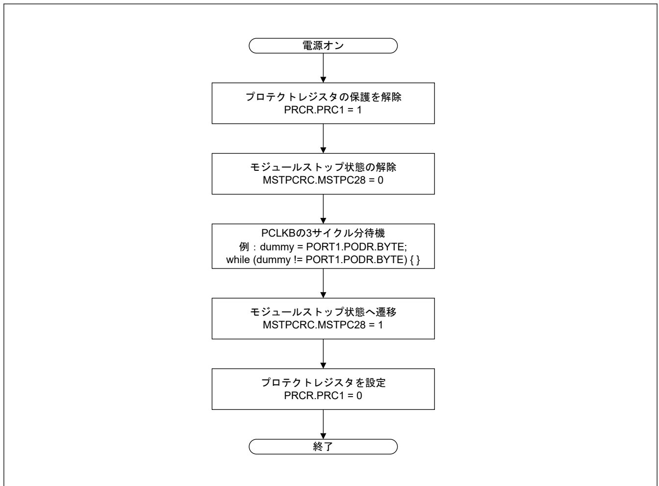
図 10.11 未使用回路の初期設定フロー例
