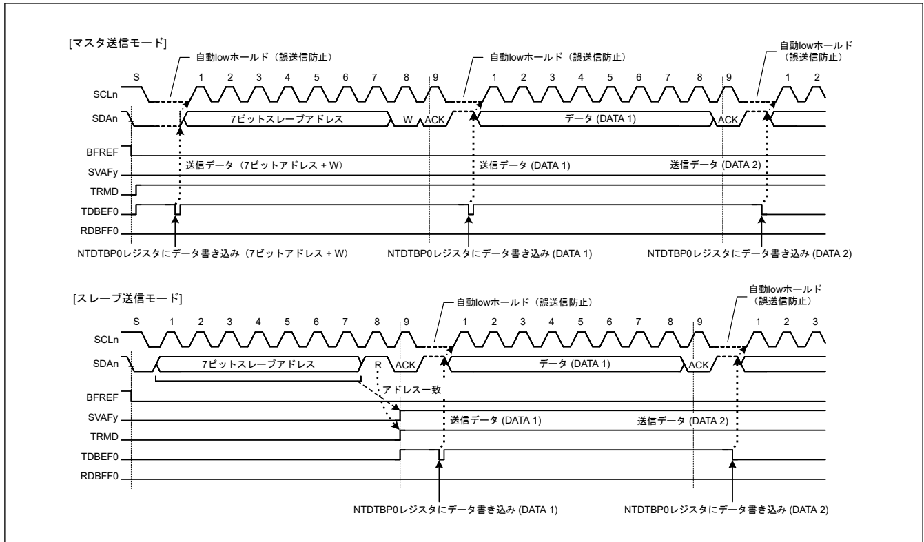
図 25.69 送信モード時の自動 Low ホールド動作
