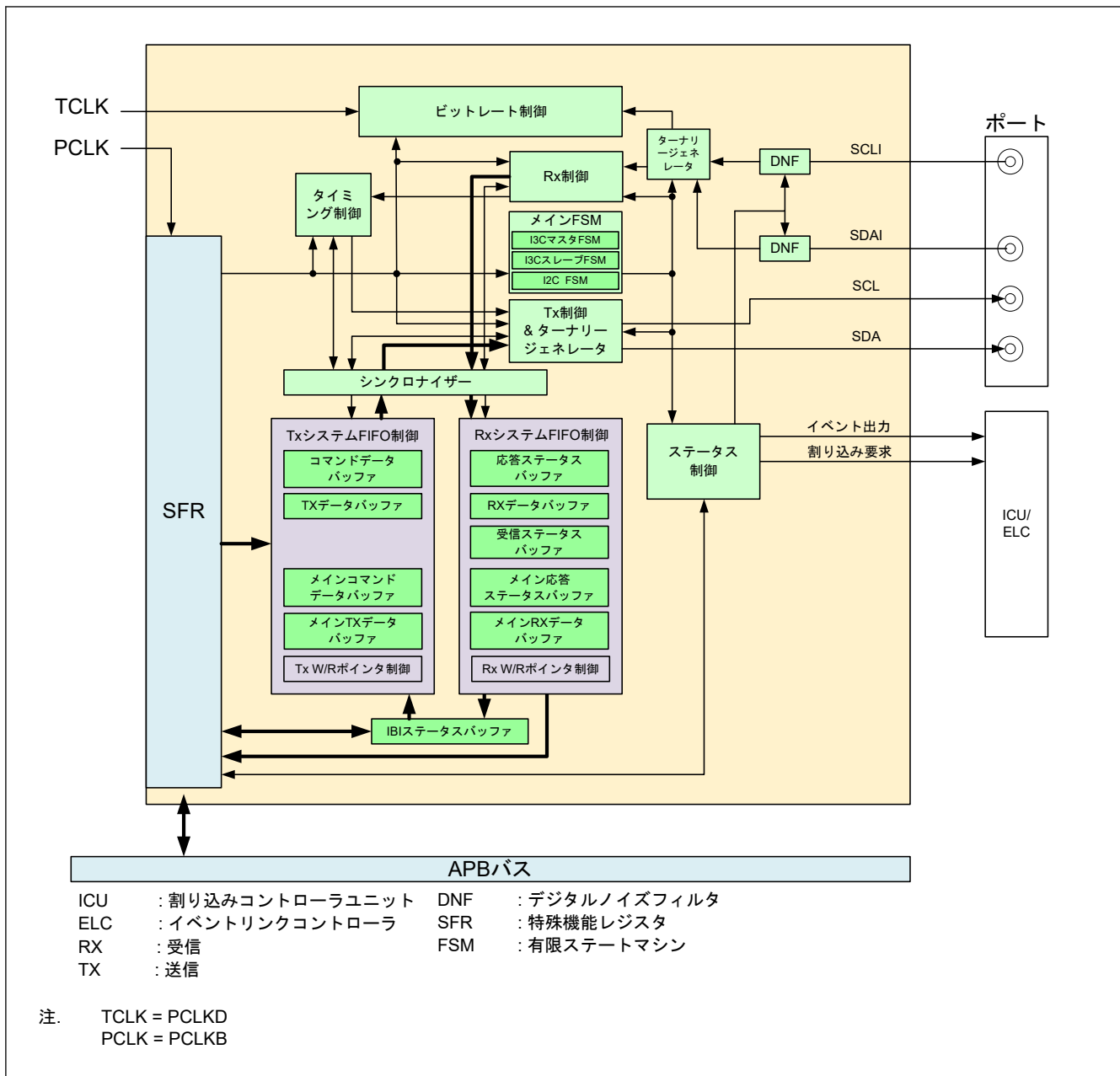
図 25.1 I3C ブロック図
