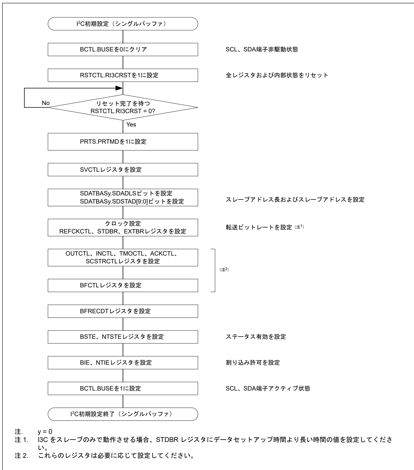
図 25.103 I²C 初期化のフローチャート例 (シングルバッファ転送)
