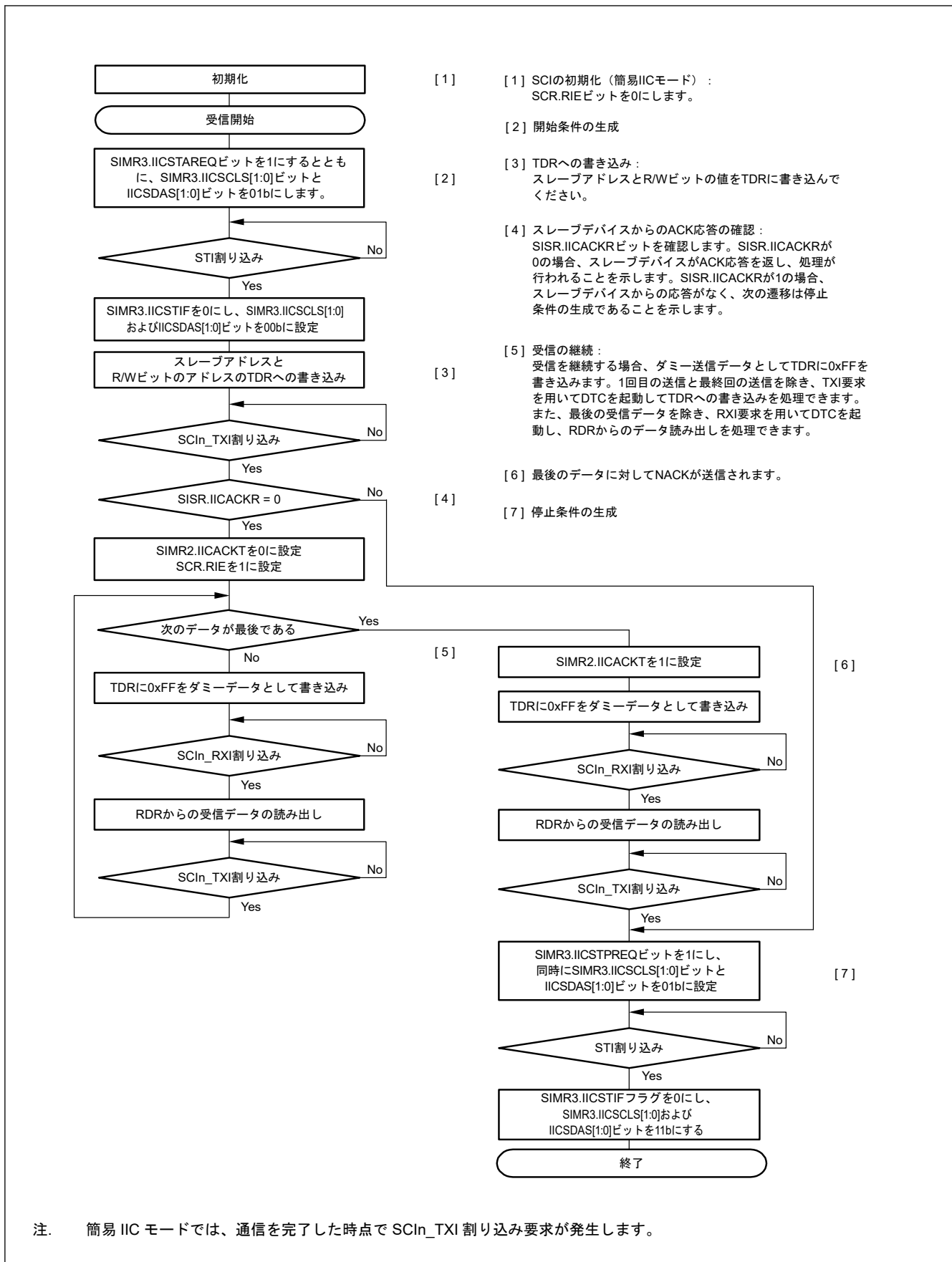
図 24.52 簡易 IIC モードにおけるマスタ受信のフローチャート例（送信割り込み、受信割り込み使用時）
