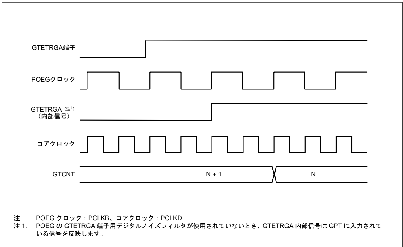
図 20.6 ハードウェア要因によるダウンカウント時のイベントカウンタ動作例
