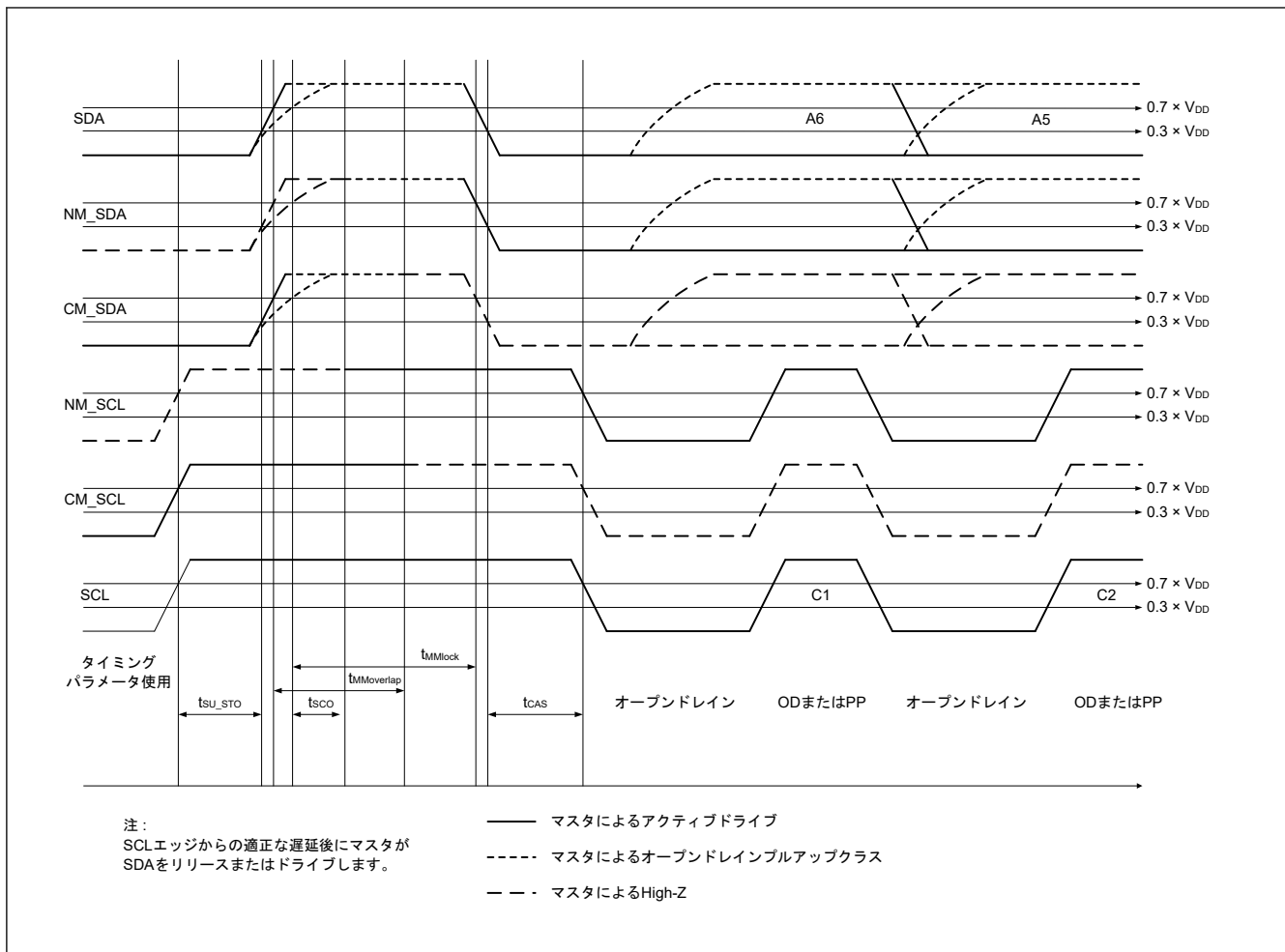
図 36.42 I3C タイミング
