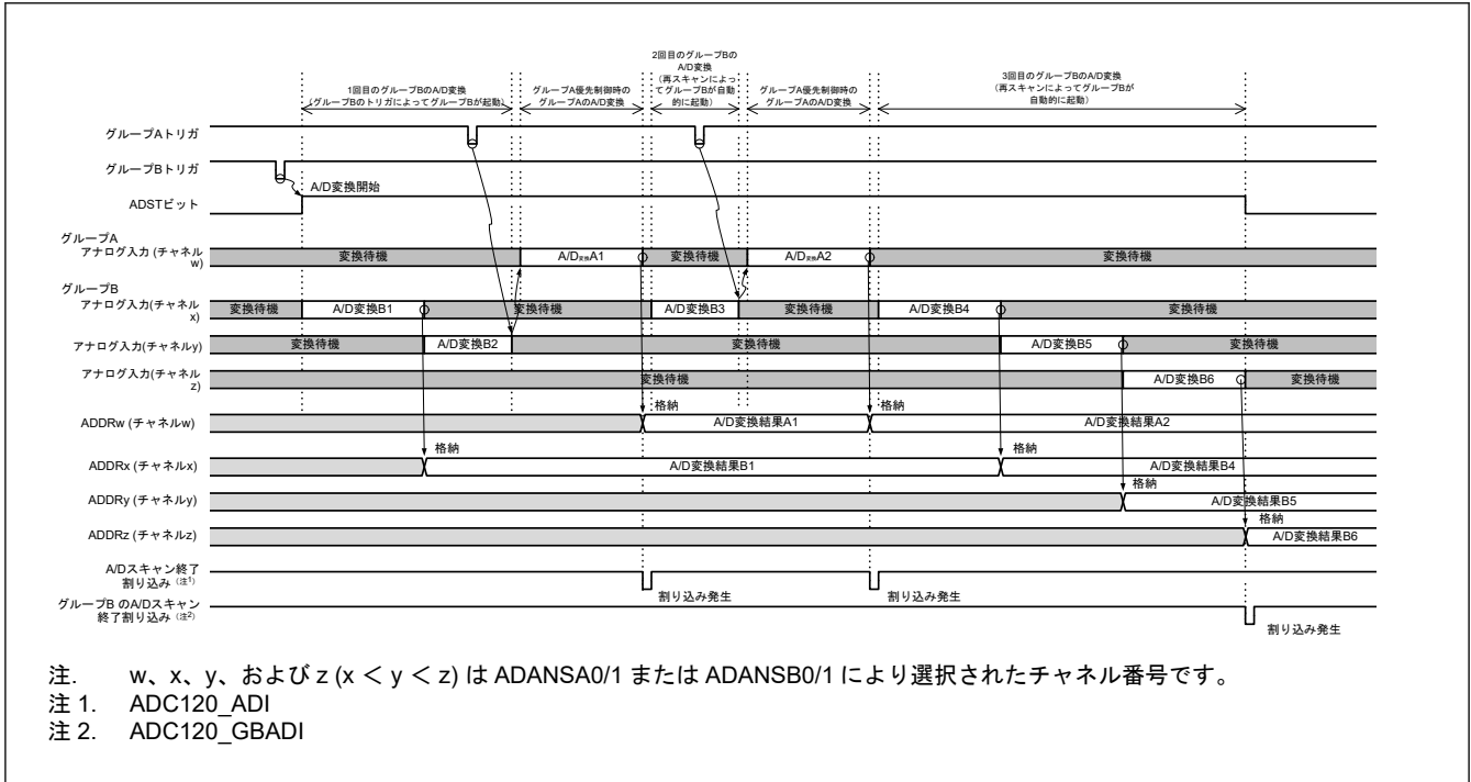
図 28.18 グループ優先動作の例 1-2 : グループ B 再スキャン中のグループ A トリガ入力、再スキャンあり (ADGSPCR.GBRSCN = 1、ADGSPCR.GBRP = 0 の場合)
