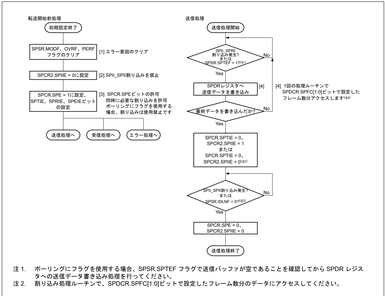
図 26.35 スレーブモードでの送信フロー
