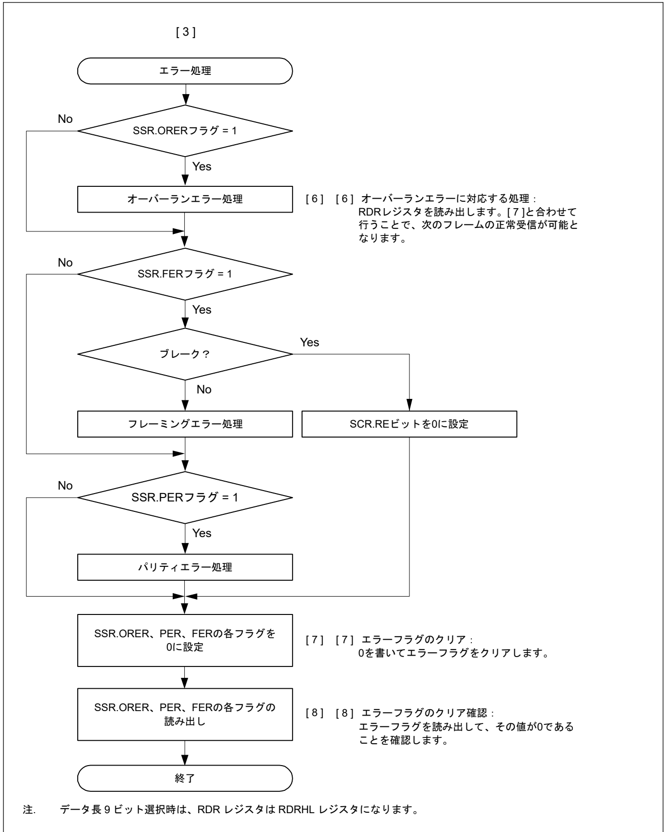
図 24.14 調歩同期式モードにおけるシリアル受信のフローチャート例（アドレス一致検出無効時）(2)
