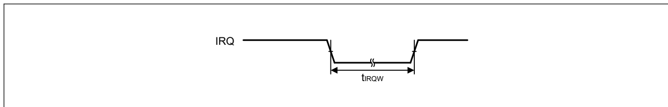
図 36.11 IRQ 割り込み入力タイミング
