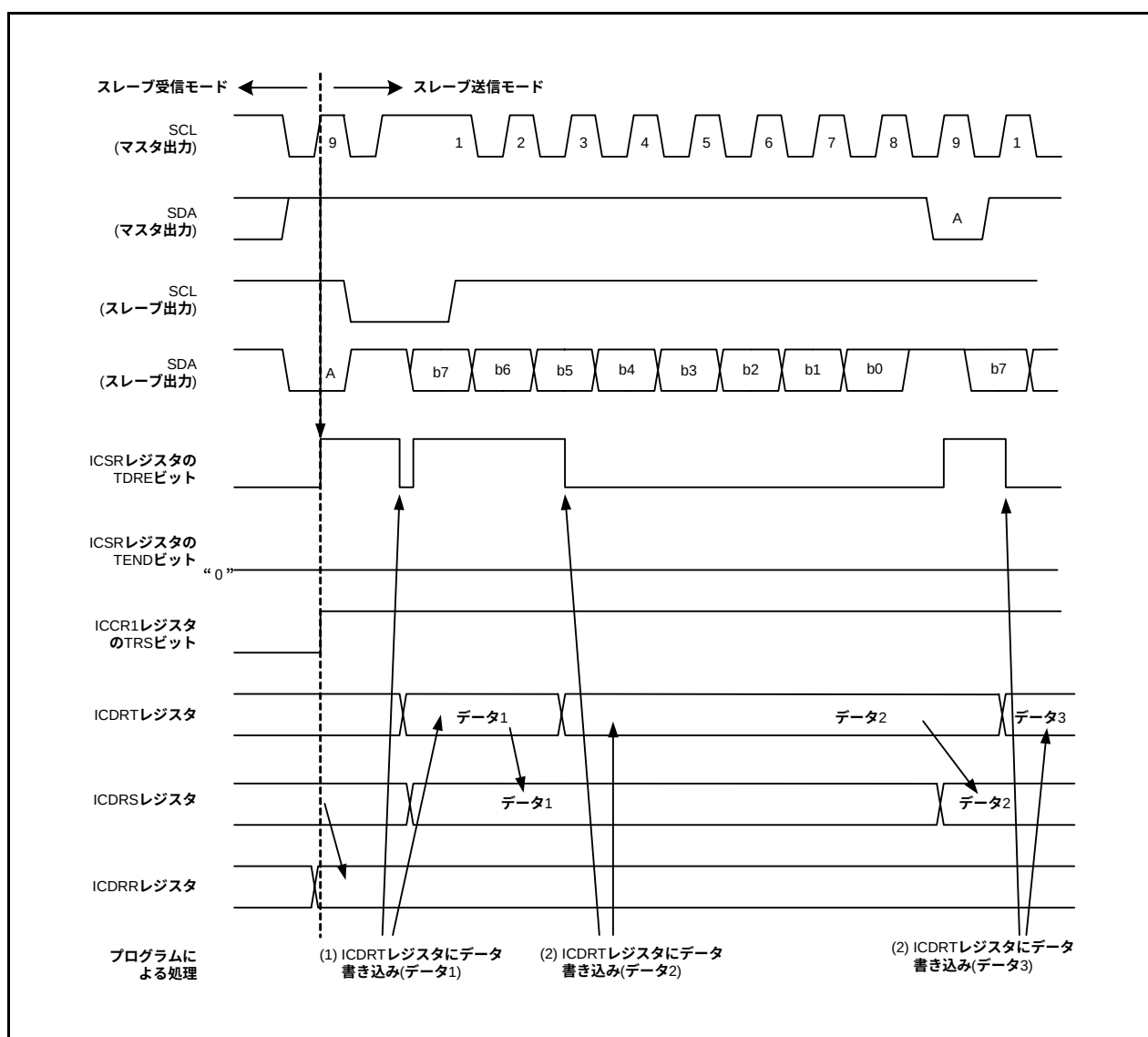
図 24.9 スレーブ送信モードの動作タイミング (I 2 Cバスイタフェースモード)(1)
