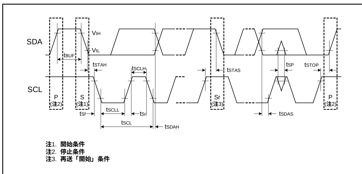
図31.30 I 2 Cバスインタフェースの入出力タイミング
