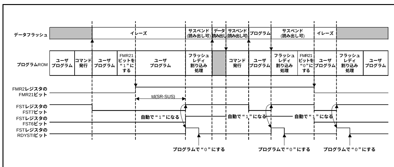
図 29.4 サスペンド動作に関するタイミング
