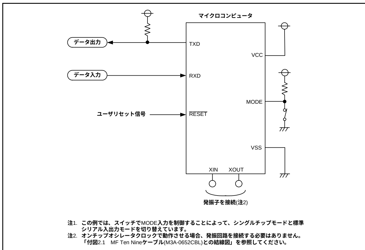
図 29.18 標準シリアル入出力モード2を使用する場合の端子処理例
