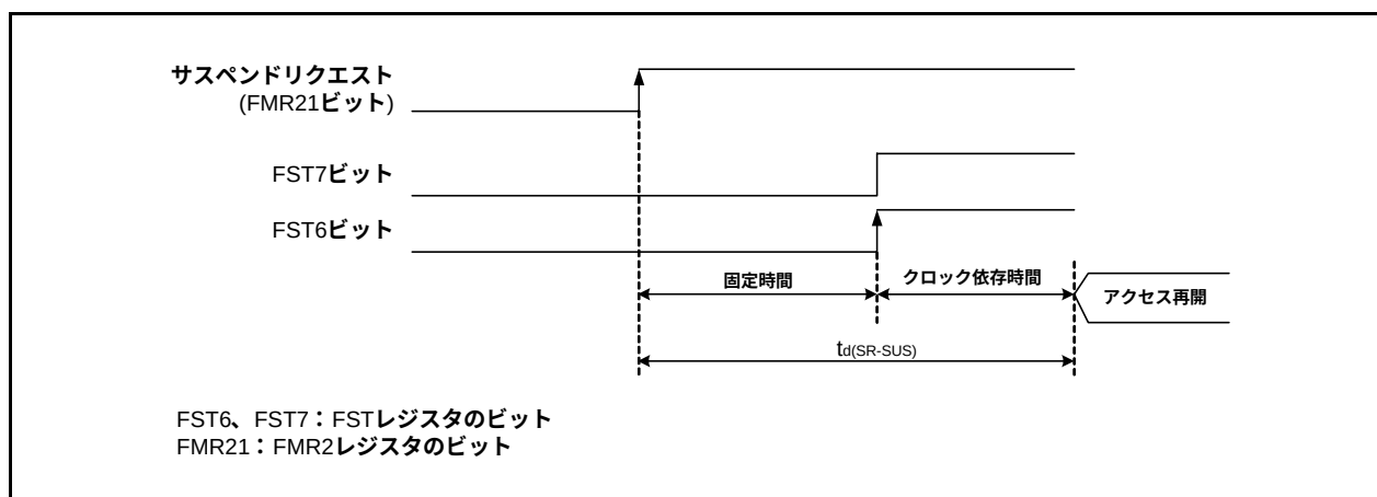
図31.4 サスペンドへの遷移時間
