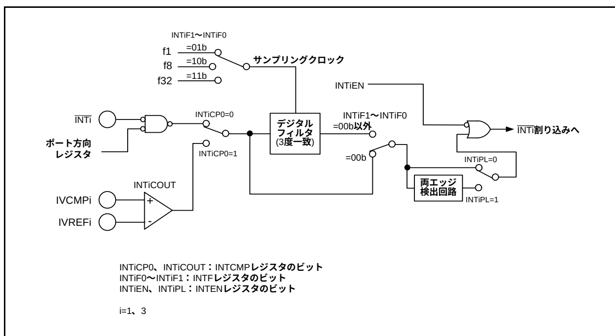
図 28.3 コンパレータ Bi デジタルフィルタの構成
