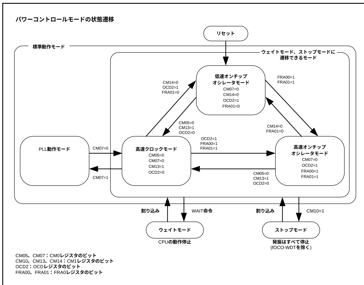
図9.9 パワーコントロールモードの状態遷移
