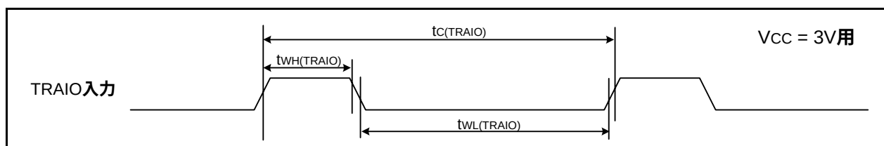
図31.15 V_{CC} = 3V 時のTRAIO入力タイミング
