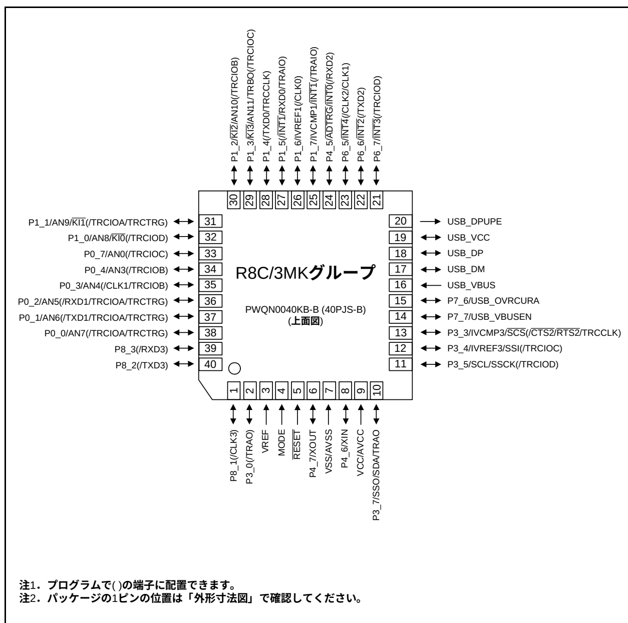
図1.6 R8C/3MKグループのピン配置図(上面図)
