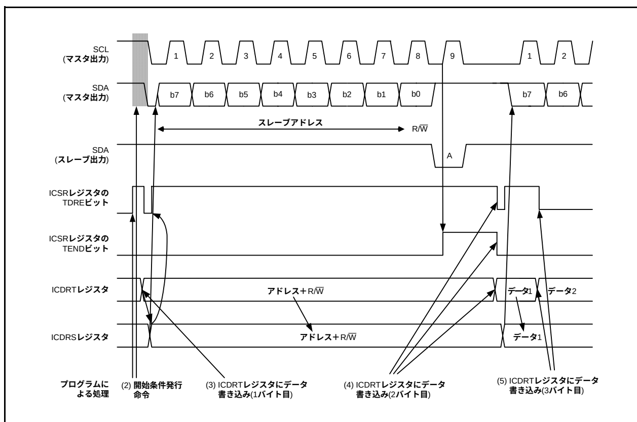
図 24.5 マスタ送信モードの動作タイミング(I 2 Cバスイインタフェースモード)(1)
