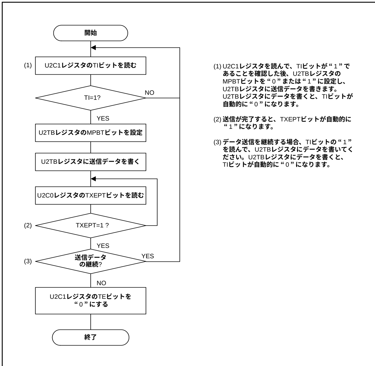
図 21.15 マルチプロセッサデータ送信のフローチャートの例
