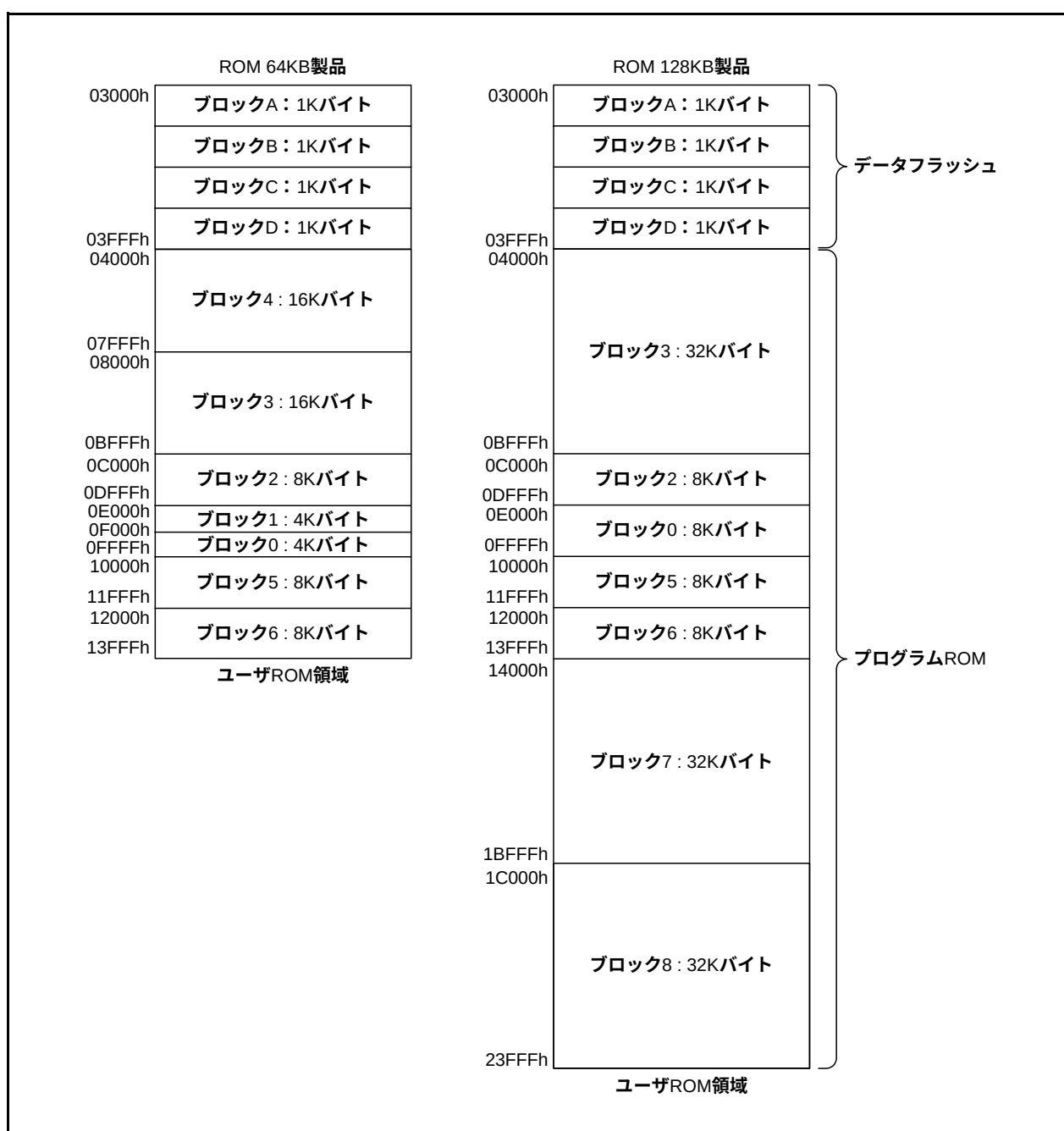
図 29.2 R8C/3MKグループのフラッシュメモリのブロック図
