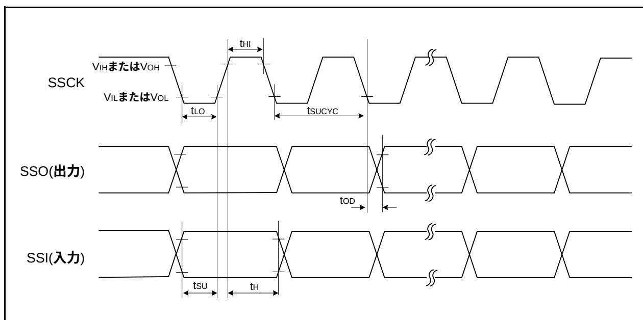
図 31.8 シンクロナスシリアルコミュニケーションユニット (SSU) の入出力タイミング (クロック同期式通信モード)
