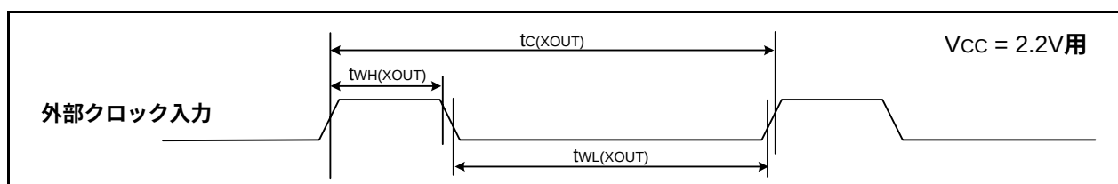
図 31.18 V_{CC} = 2.2V 時の外部クロック入力タイミング
