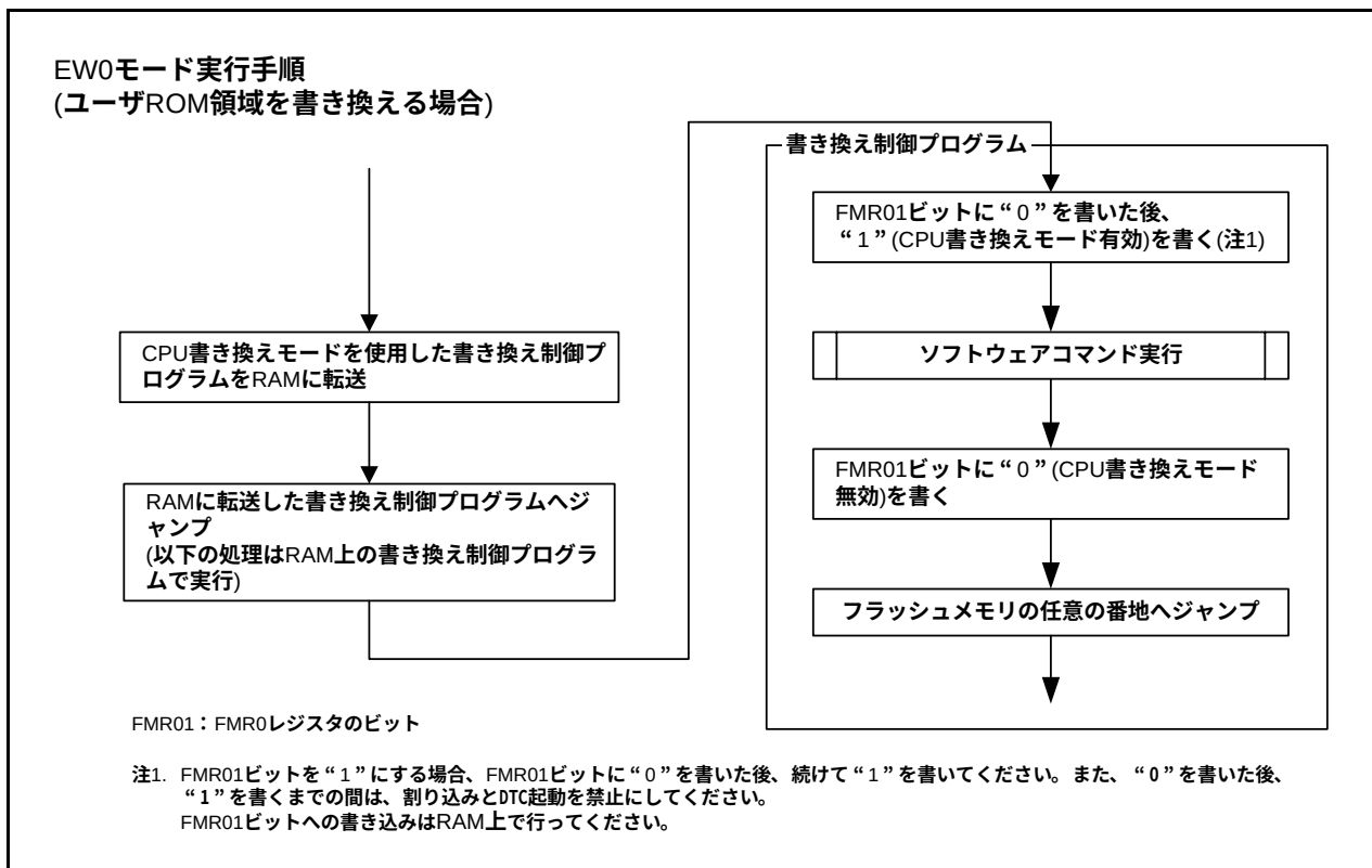
図29.5 EW0モードの設定と解除方法
