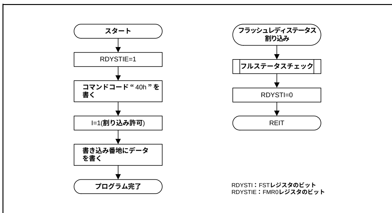
図 29.10 プログラムフローチャート(フラッシュレディステータス割り込み許可)
