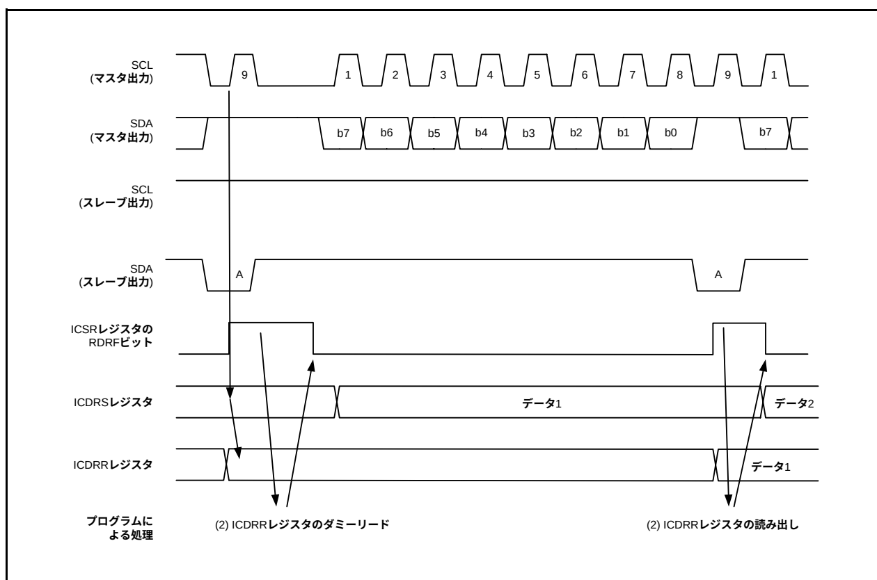
図 24.11 スレーブ受信モードの動作タイミング (I 2 C バスインタフェースモード) (1)
