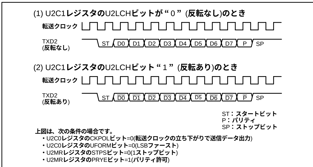
図21.10 シリアルデータ論理
