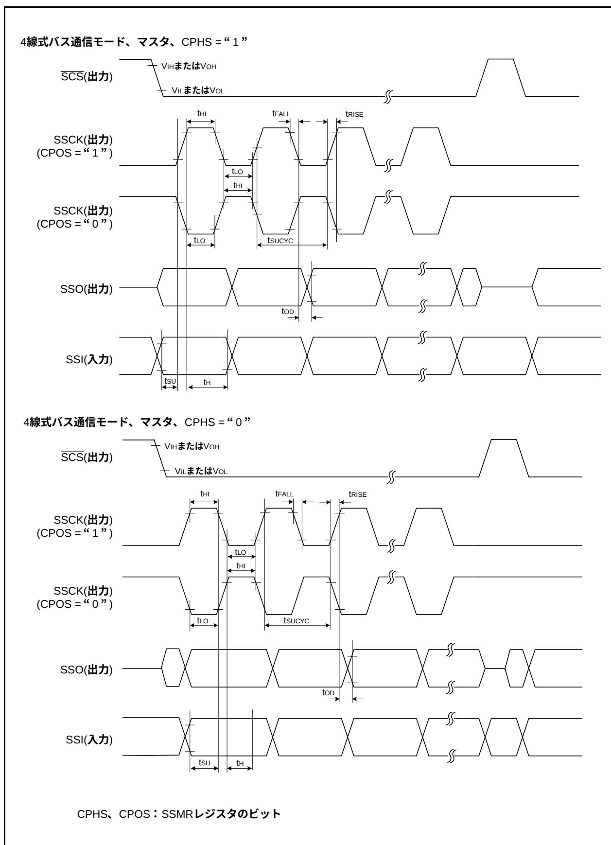
図31.6 シンクロナスシリアルコミュニケーションユニット (SSU) の入出力タイミング (マスタ)
