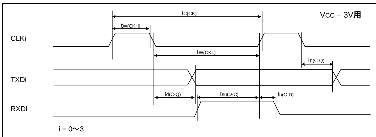
図31.37 VCC = 3V時のシリアルインタフェースのタイミング
