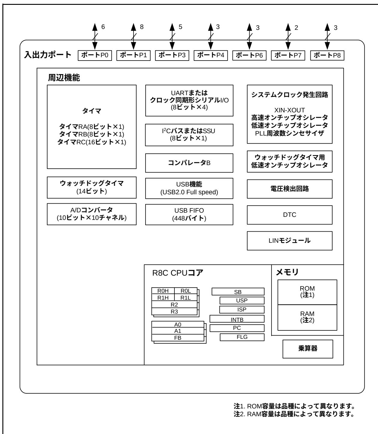
図1.4 R8C/3MKグループのブロック図
