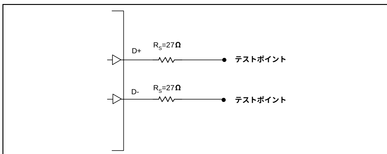
図31.3 負荷条件
