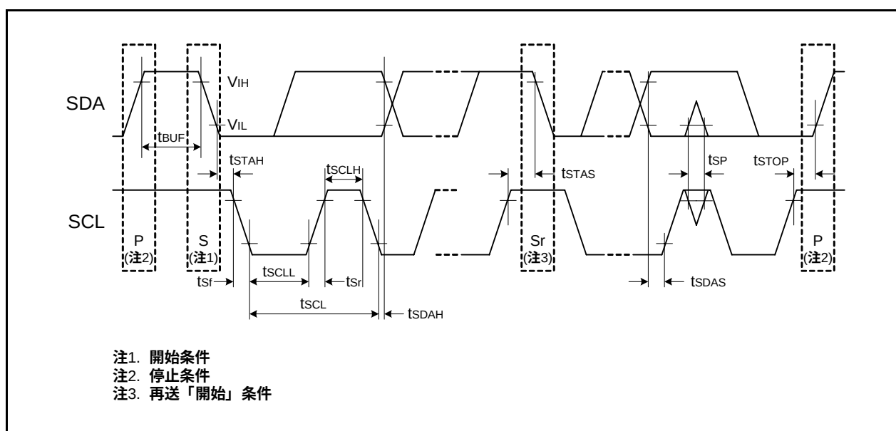
図31.9 I 2 Cバスインタフェースの入出力タイミング
