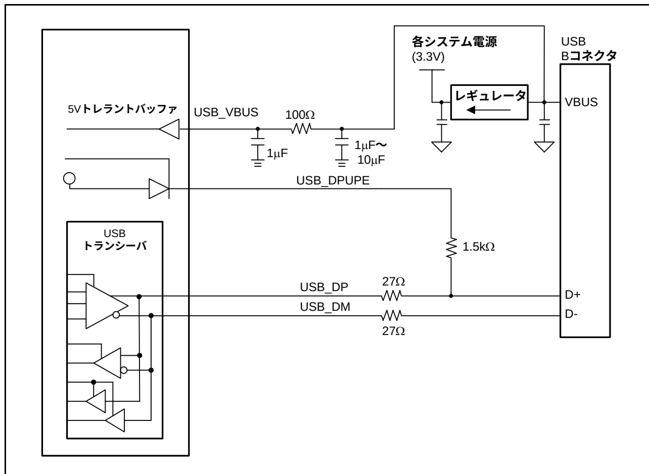
図26.4 バスパワード時のUSBコネクタのファンクション接続例
