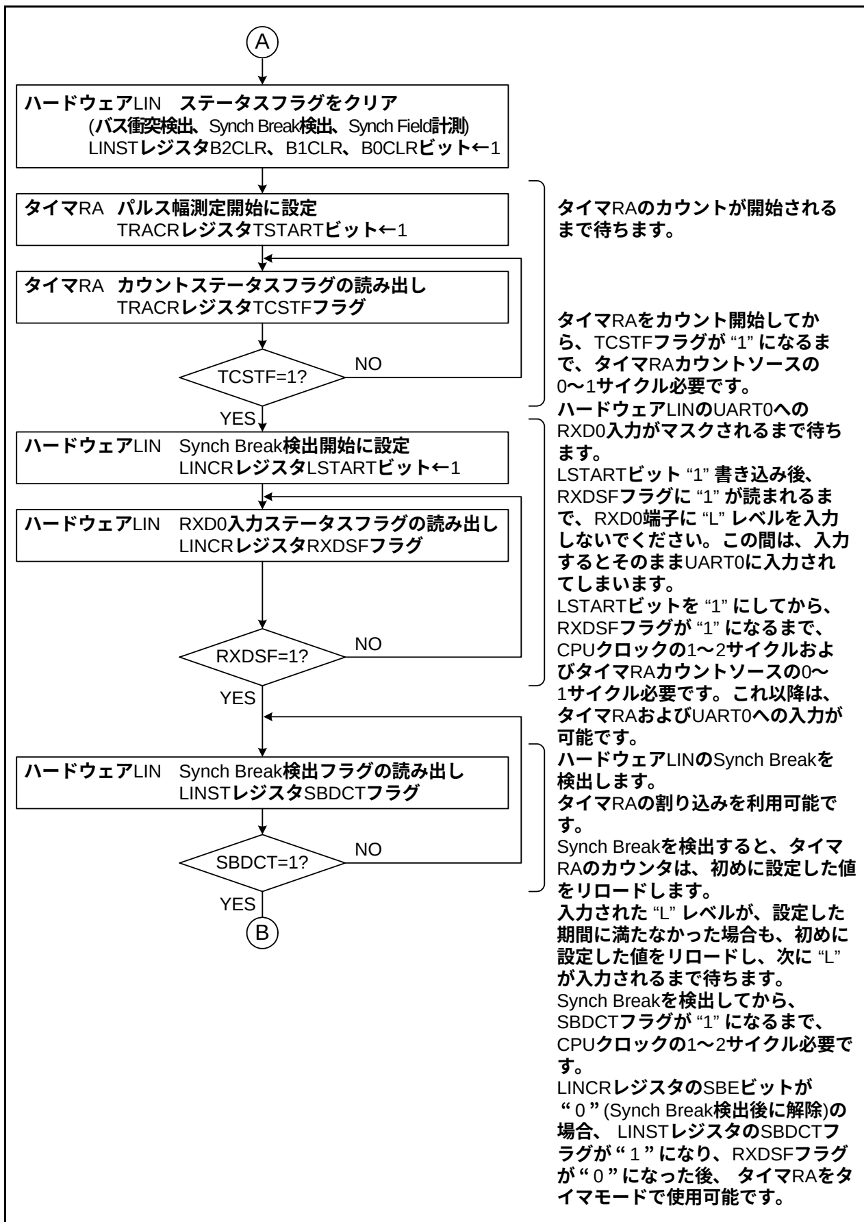
図 25.7 ヘッダフィールド受信フローチャート例(2)
