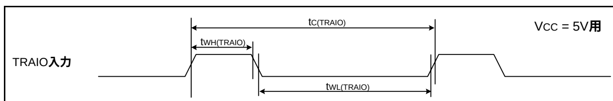
図31.11 V_{CC} = 5V 時のTRAIO入力タイミング
