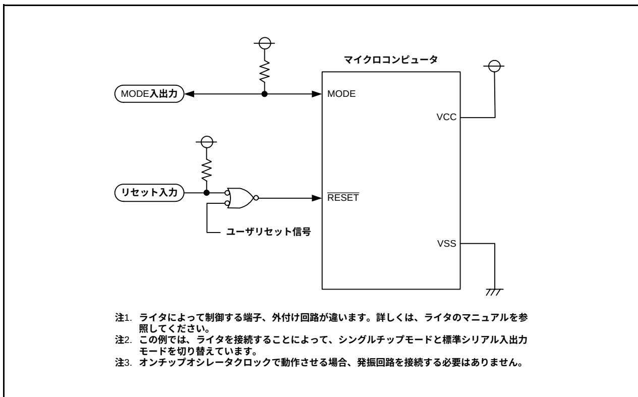
図 29.19 標準シリアル入出力モード3を使用する場合の端子処理例
