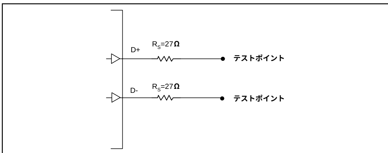
図31.24 負荷条件
