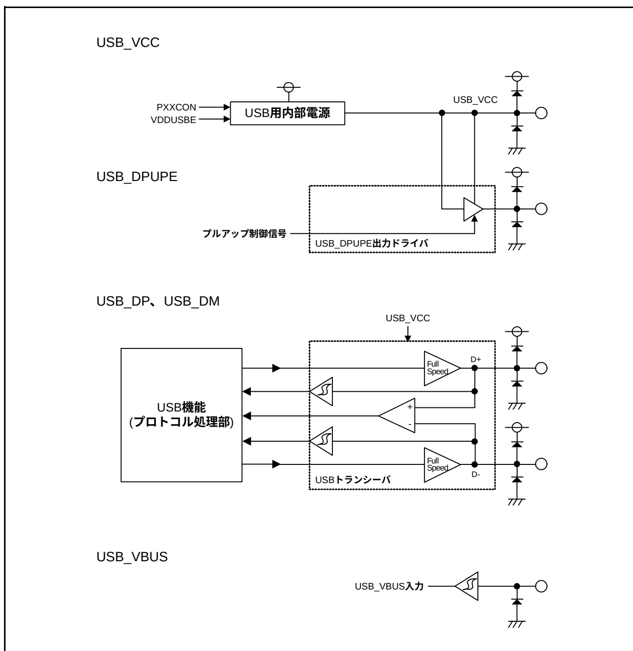
図 7.14 I/Oポートの構成(14)
