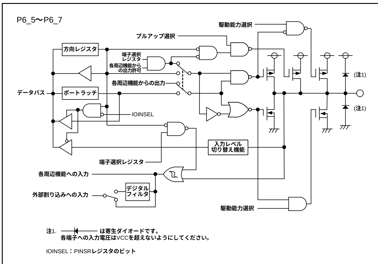
図7.11 I/Oポートの構成(11)
