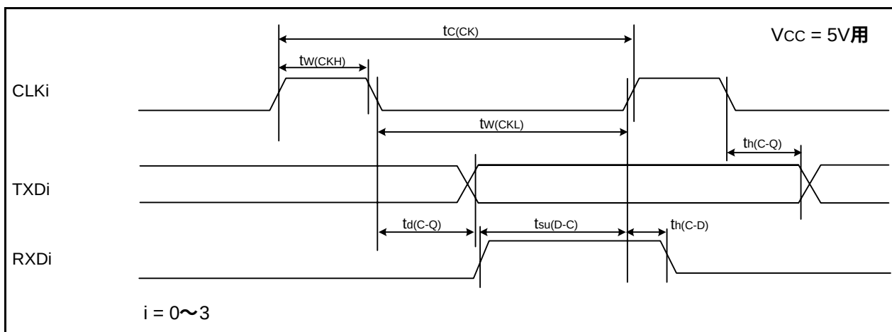
図31.12 VCC = 5V時のシリアルインタフェースのタイミング
