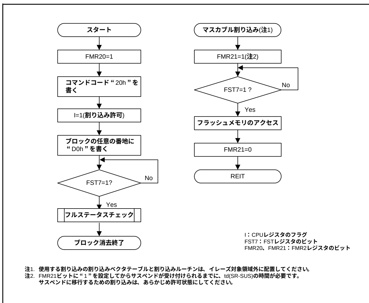
図 29.12 ブロックイレーズフローチャート(フラッシュレディステータス割り込み禁止かつサスペンド許可)
