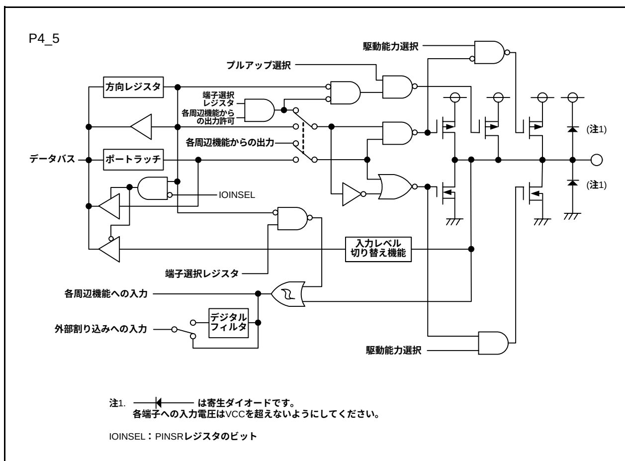
図 7.9 I/Oポートの構成(9)
