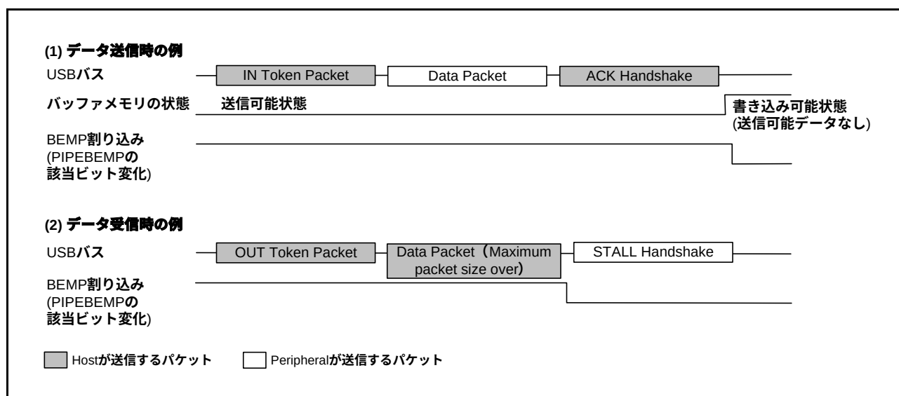
図26.8 ファンクションコントローラ機能選択時のBEMP割り込み発生タイミング図
