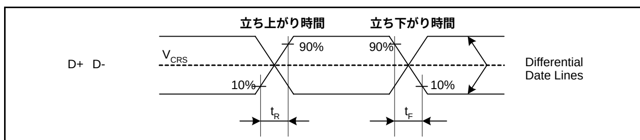
図31.2 データ信号タイミング
