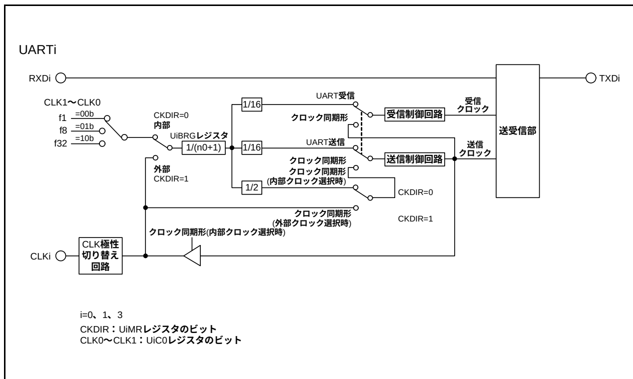
図20.1 UARTi (i=0、1、3)のブロック図
