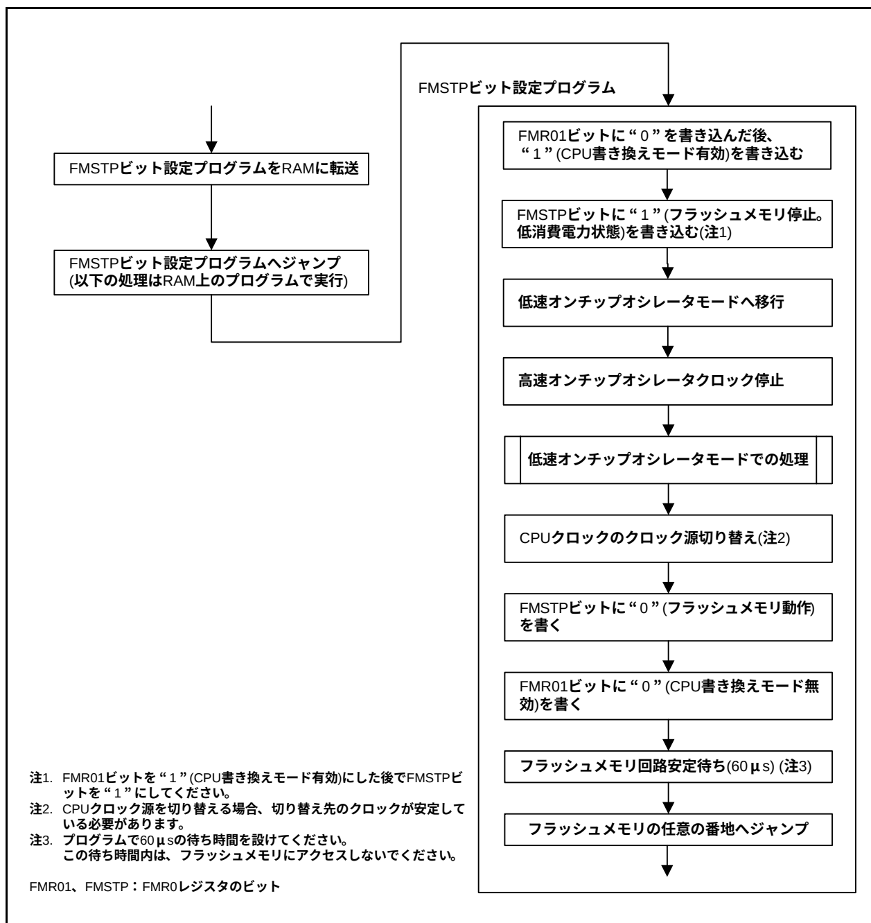
図30.2 FMSTPビットによる低消費電力操作手順例
