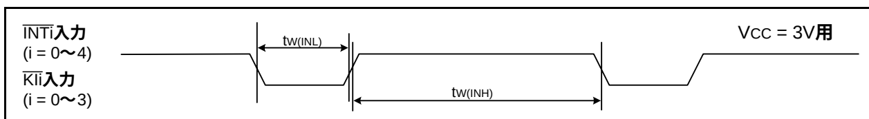
図31.38 VCC = 3V時の外部割り込み \overline{INTi} およびキー入力割り込み \overline{Kli} 入力タイミング
