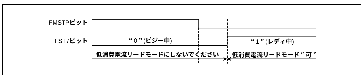
図 29.3 低消費電流リードモードへの移行
