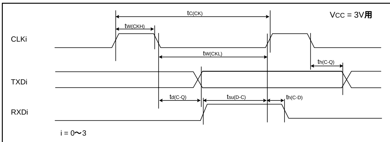
図31.16 VCC = 3V時のシリアルインタフェースのタイミング
