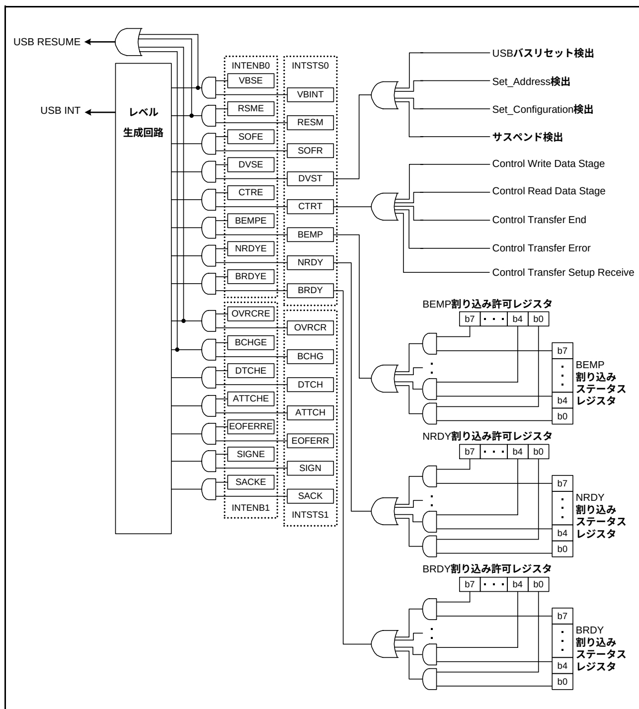
図26.5 割り込みの関連図
