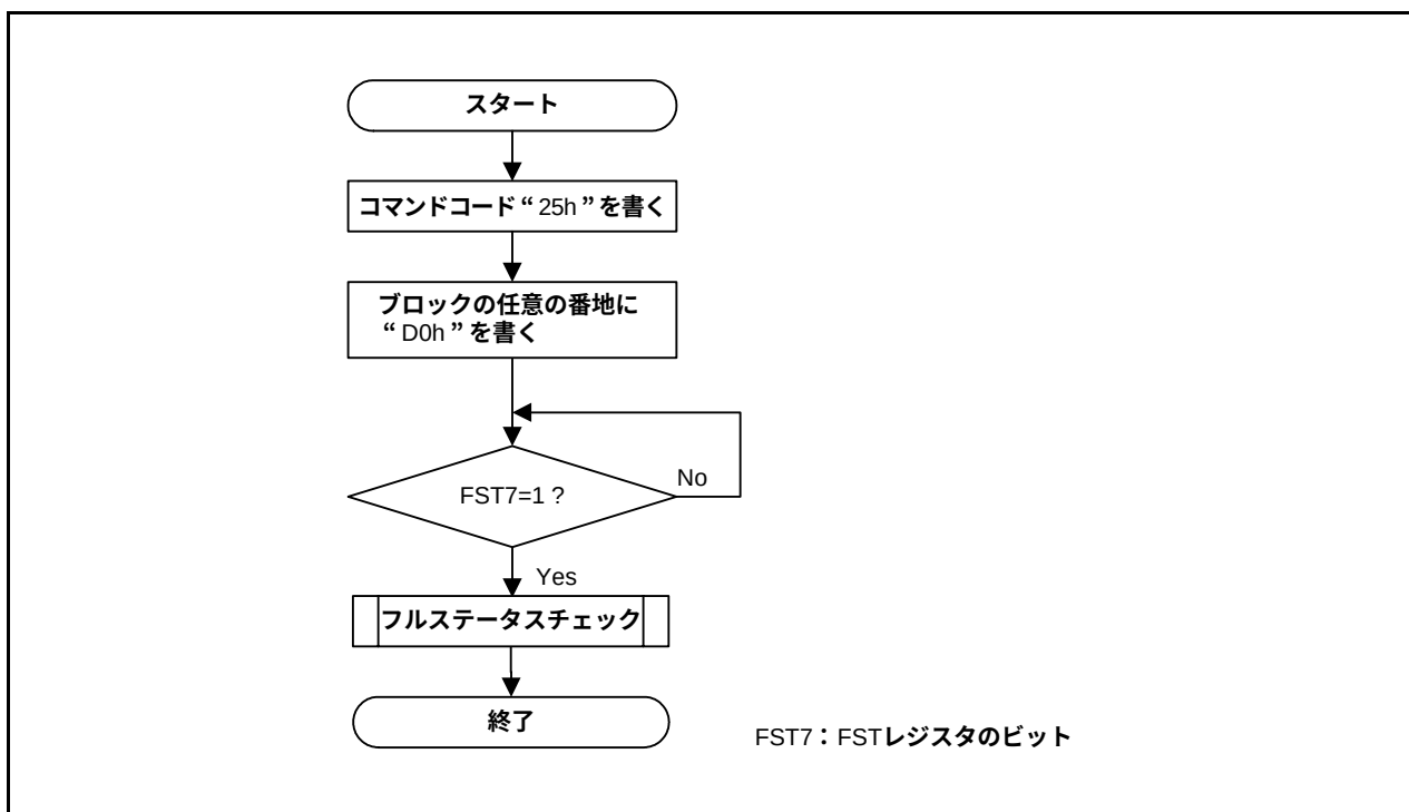
図29.16 ブロックブランクチェックフローチャート
