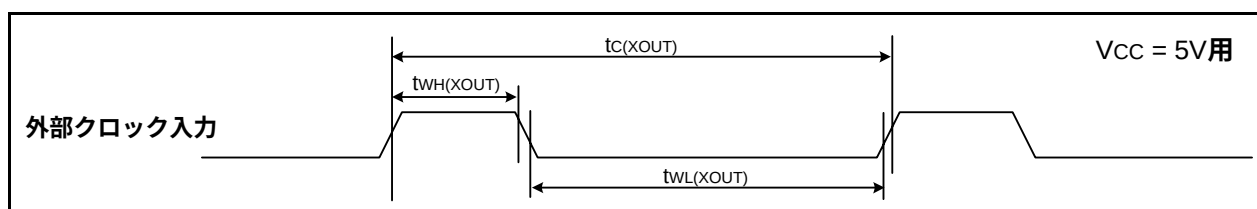
図31.10 V_{CC} = 5V 時の外部クロック入力タイミング
