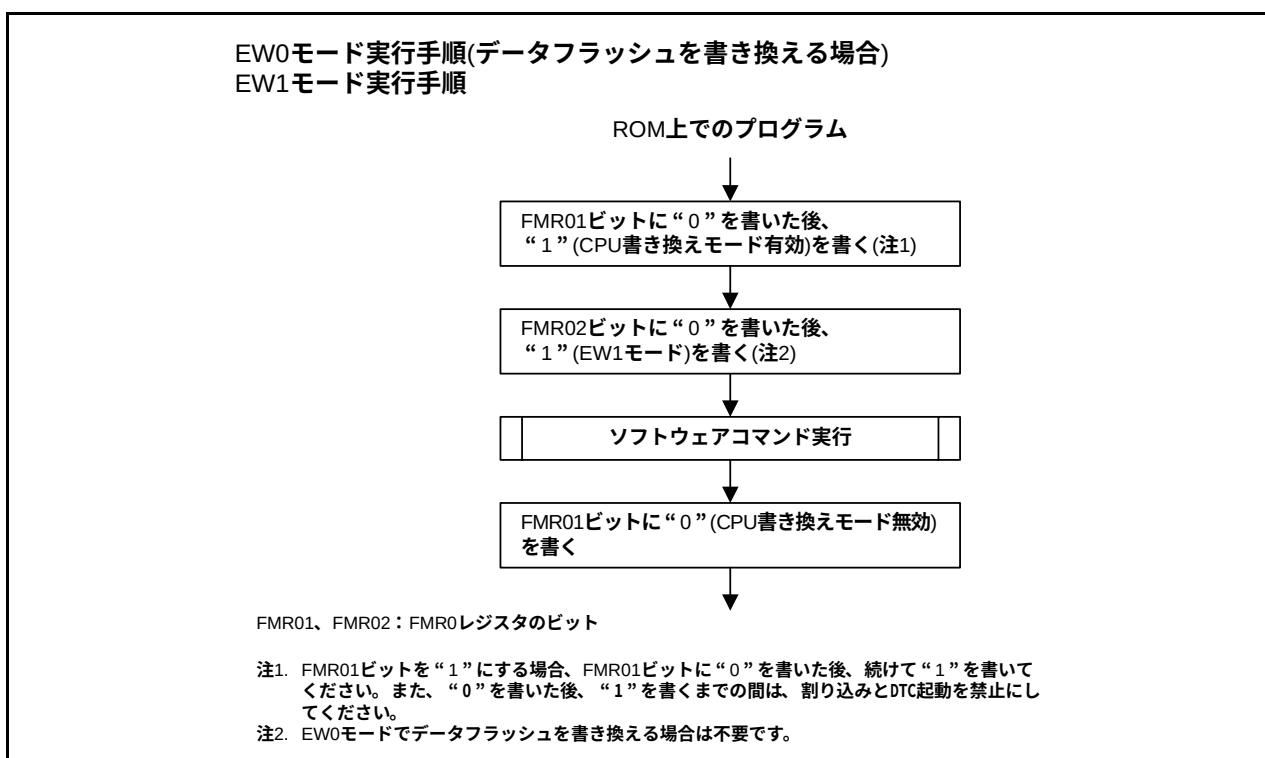
図29.6 EW0モード(データフラッシュを書き換える場合)、EW1モードの設定と解除方法
