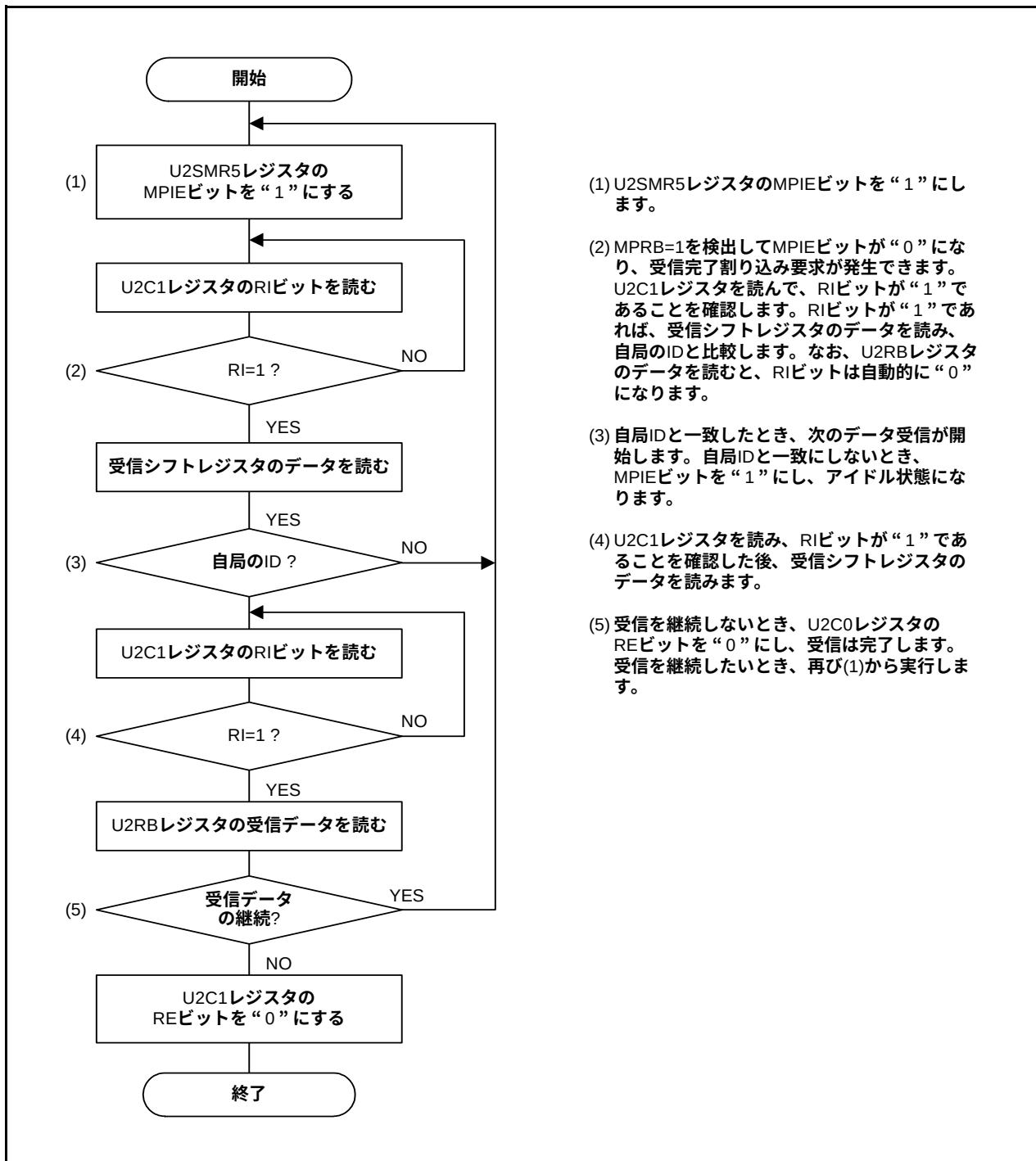
図 21.16 マルチプロセッサデータ受信のフローチャートの例
