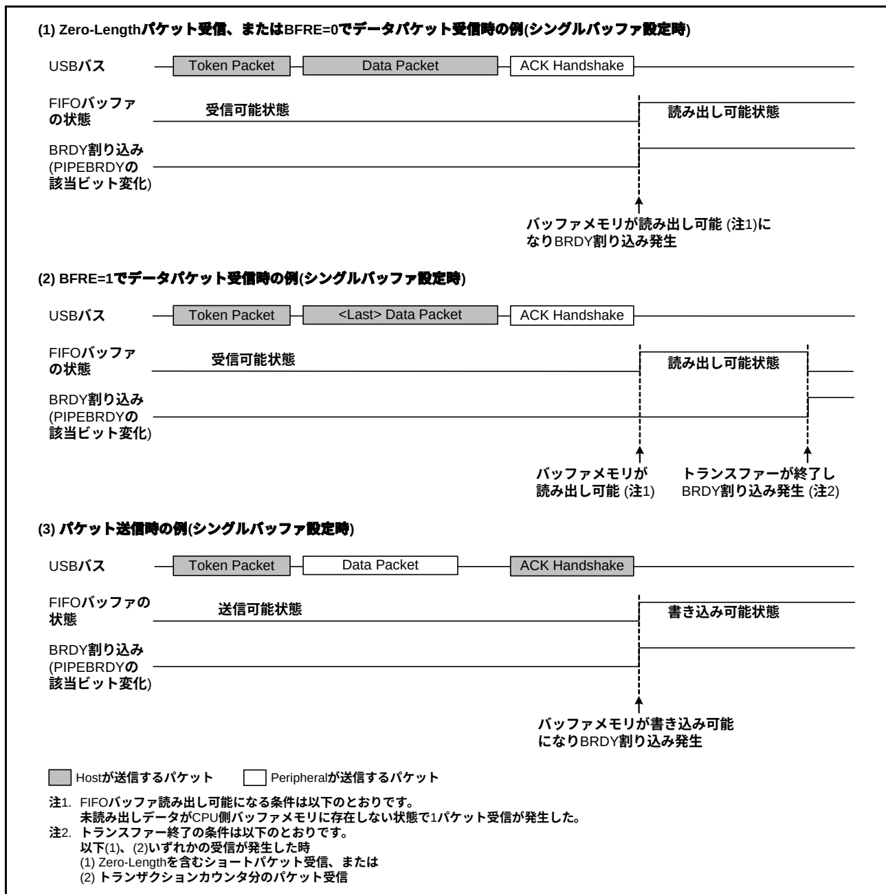
図26.6 BRDY割り込み発生タイミング図
