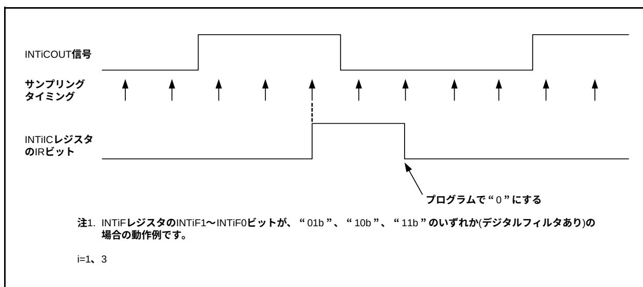
図 28.4 コンパレータ Bi デジタルフィルタ動作例
