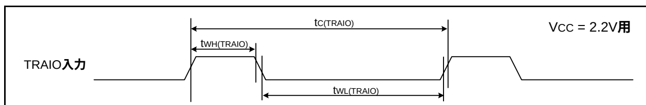
図 31.40 V_{CC} = 2.2V 時のTRAIO入力タイミング
