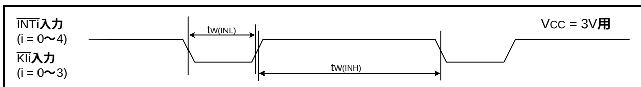
図31.17 VCC = 3V時の外部割り込み \overline{\text{INTi}} およびキー入力割り込み \overline{\text{Kli}} 入力タイミング
