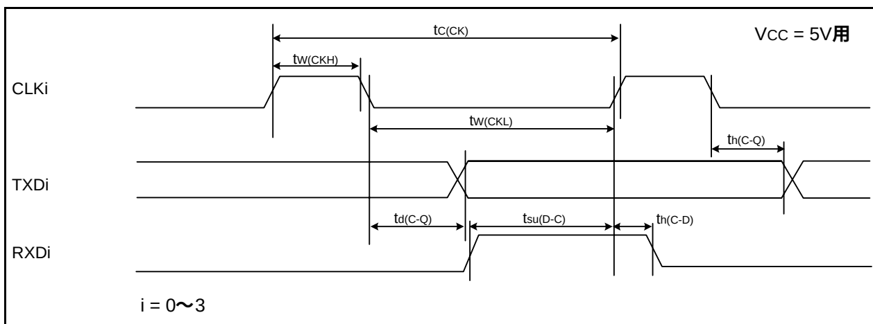
図31.33 VCC = 5V時のシリアルインタフェースのタイミング
