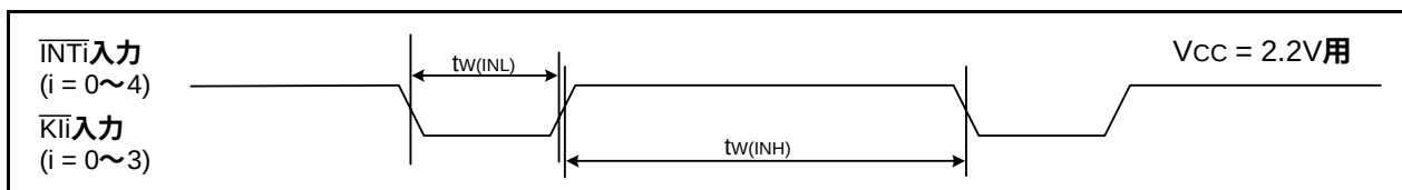
図31.42 VCC = 2.2V時の外部割り込み \overline{INTi} およびキー入力割り込み \overline{Kli} 入力タイミング
