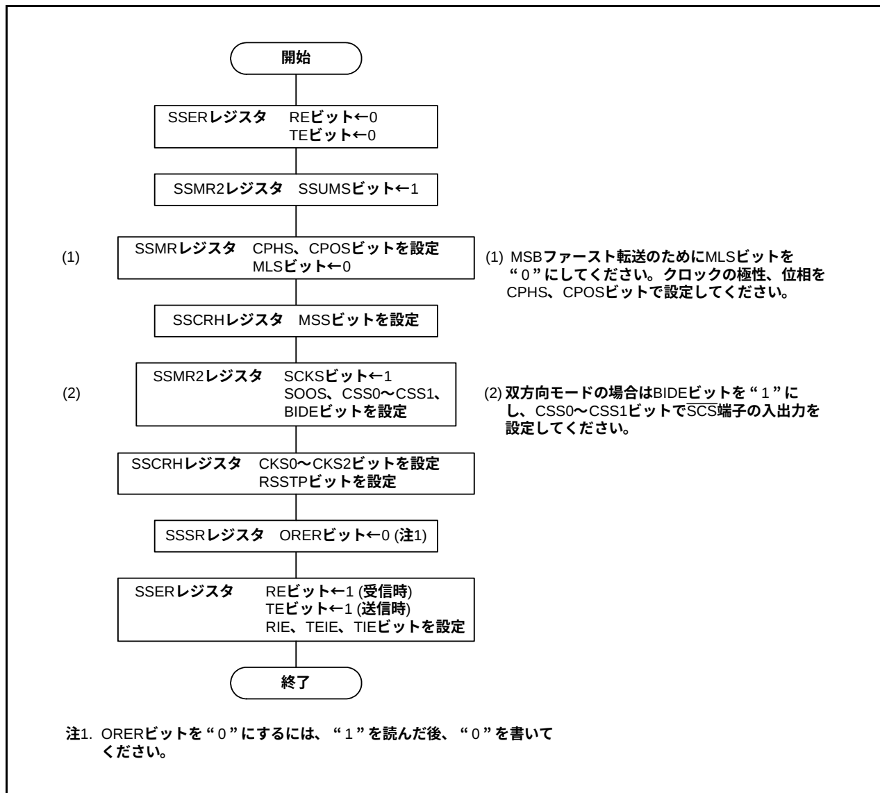
図23.10 4線式バス通信モードの初期化
