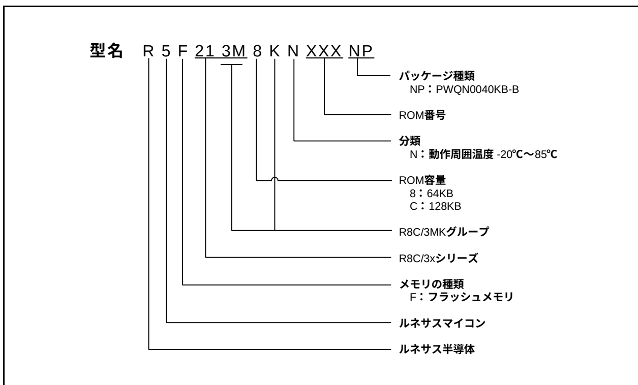
図1.2 R8C/3MKグループの型名とメモリサイズ・パッケージ
