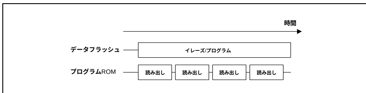
図29.7 BGO機能
