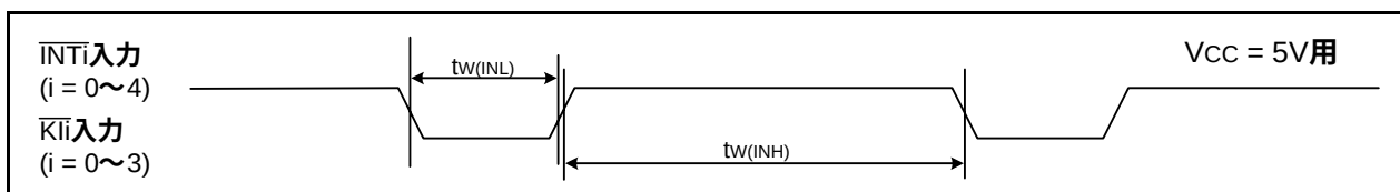
図31.13 VCC = 5V時の外部割り込み \overline{\text{INT}}i およびキー入力割り込み \overline{\text{K}}li 入力タイミング
