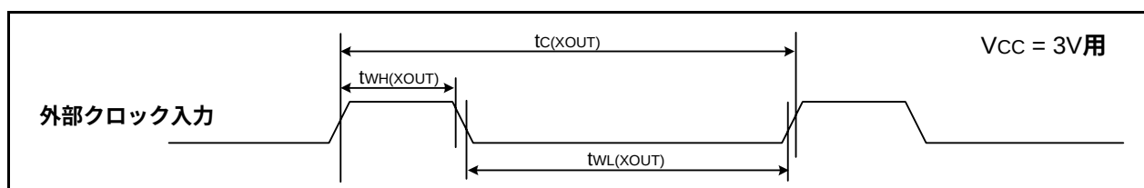
図31.14 V_{CC} = 3V 時の外部クロック入力タイミング
