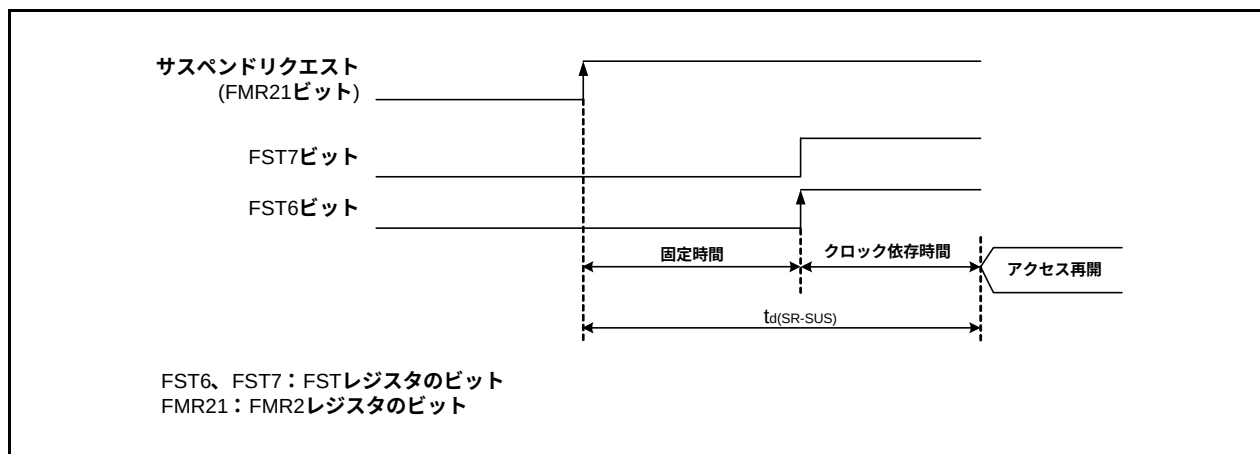
図31.25 サスペンドへの遷移時間
