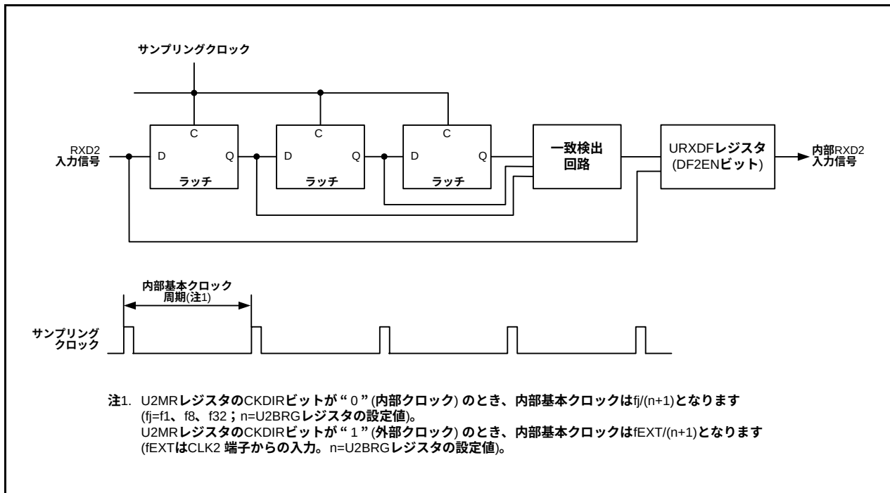
図21.18 RXD2デジタルフィルタ回路のブロック図
