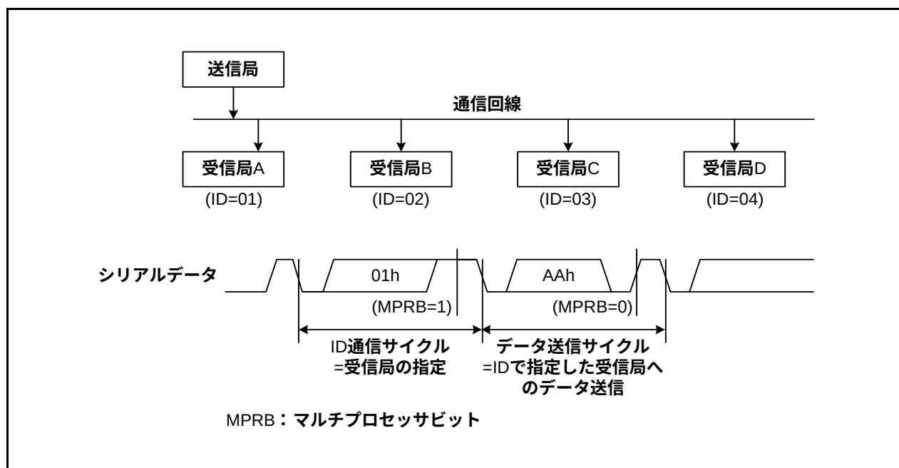
図21.13 マルチプロセッサフォーマットを使用したプロセッサ間通信の例(受信局AへのデータAAhの送信の例)
