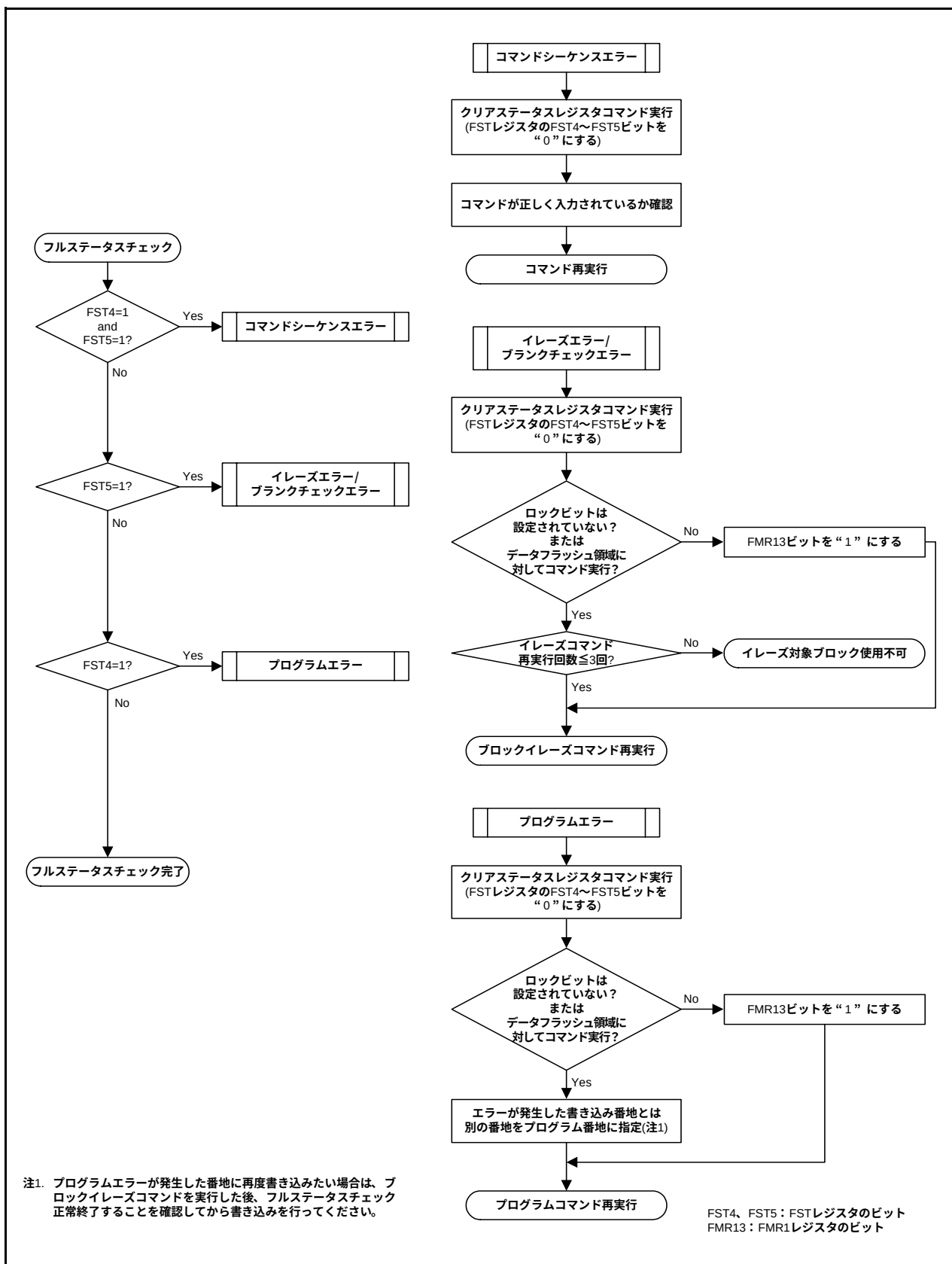
図 29.17 フルステータスチェックフローチャート、各エラー発生時の対処方法
