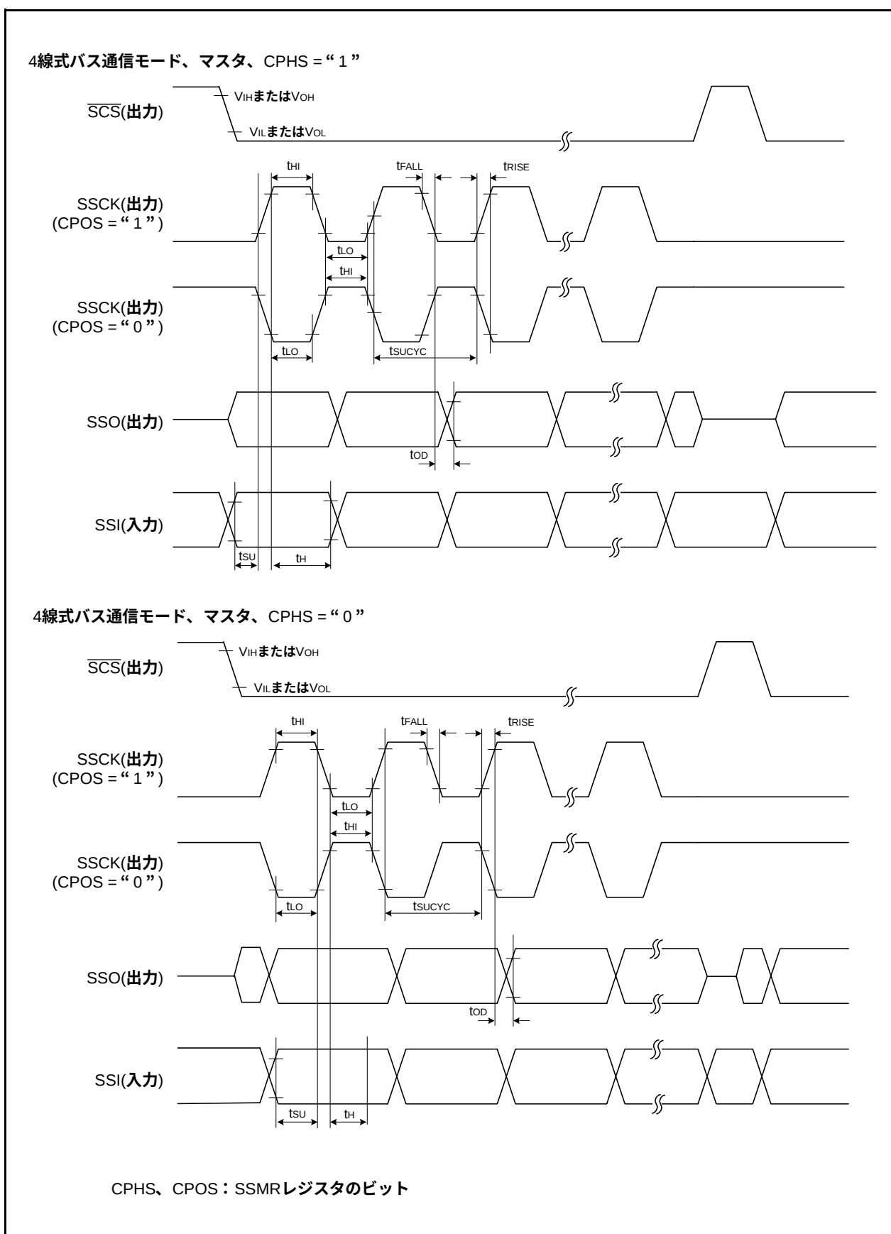
図31.27 シンクロナスシリアルコミュニケーションユニット (SSU) の入出力タイミング (マスタ)
