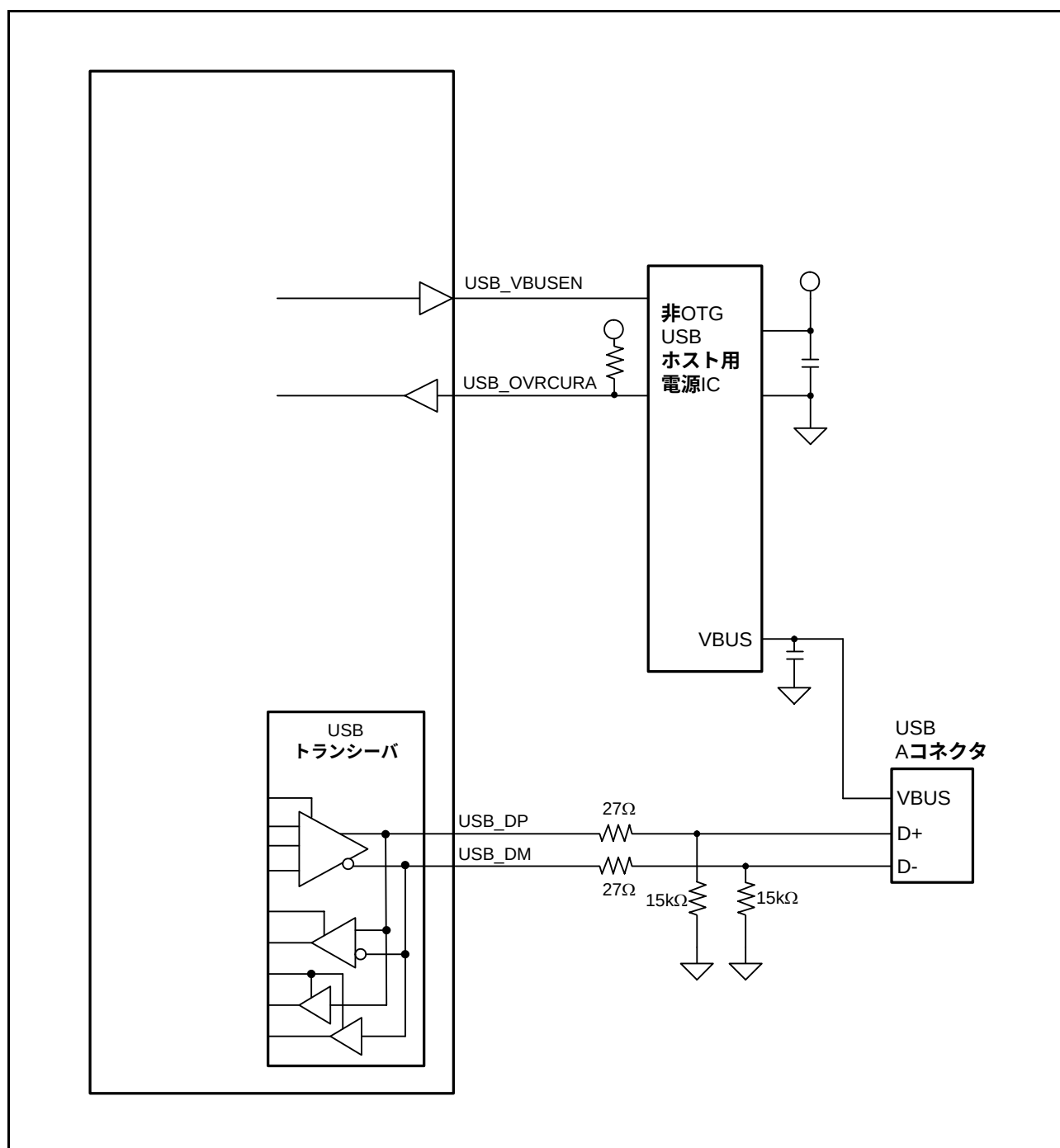
図 26.3 USBコネクタのホスト接続例
