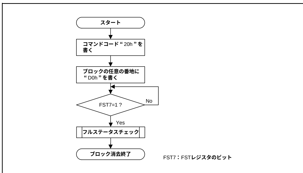
図 29.11 ブロックイレーズフローチャート(フラッシュレディステータス割り込み禁止)
