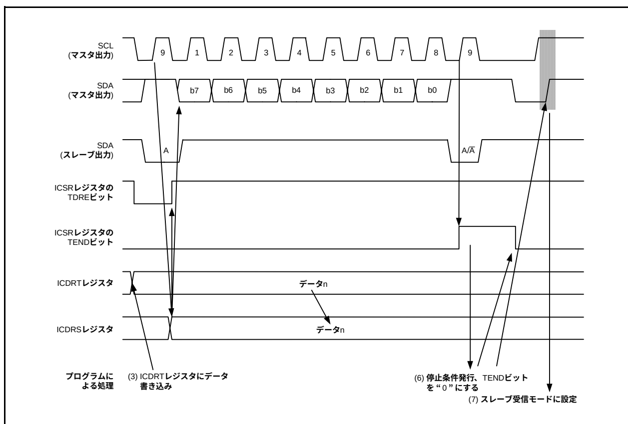
図 24.6 マスタ送信モードの動作タイミング(I 2 Cバスイインタフェースモード)(2)
