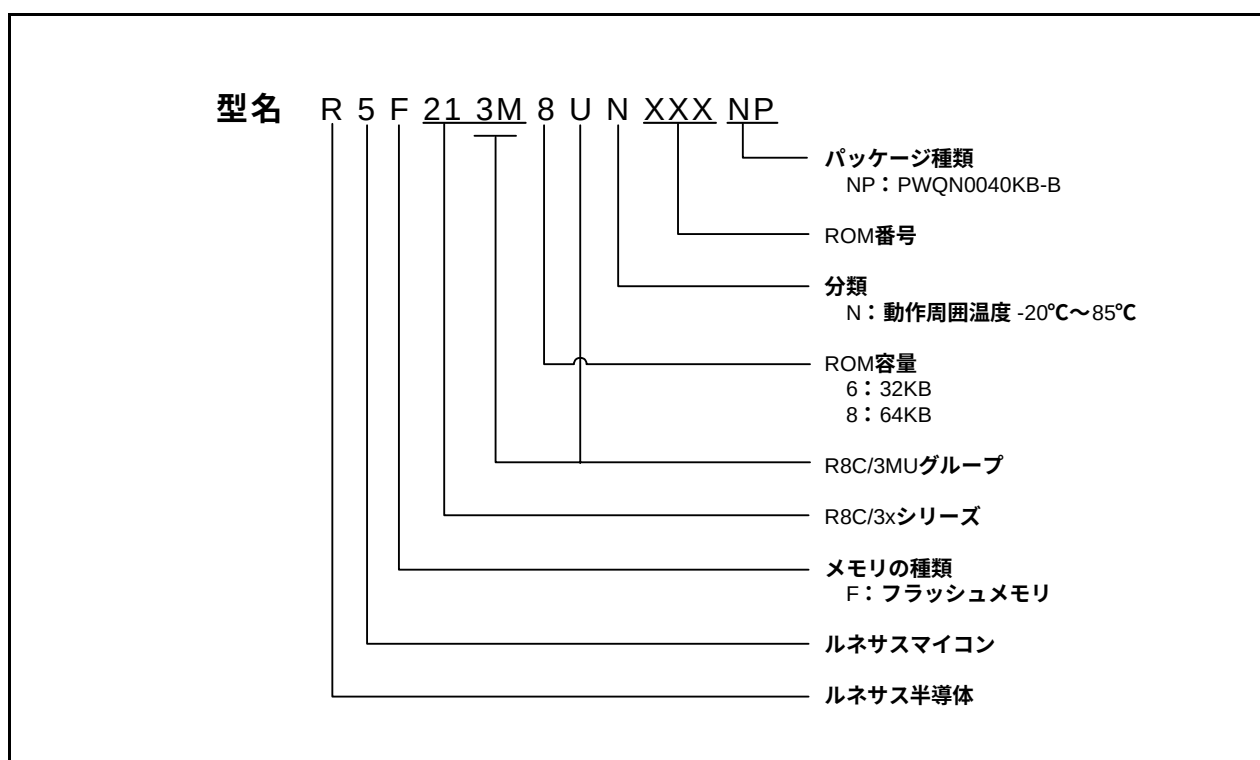
図1.1 R8C/3MUグループの型名とメモリサイズ・パッケージ
