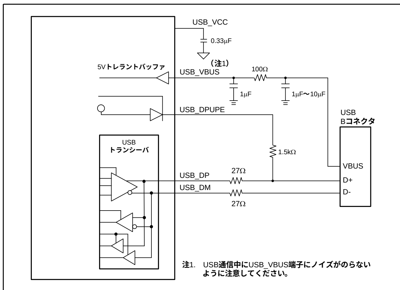
図26.2 セルフパワード時のUSBコネクタのファンクション接続例
