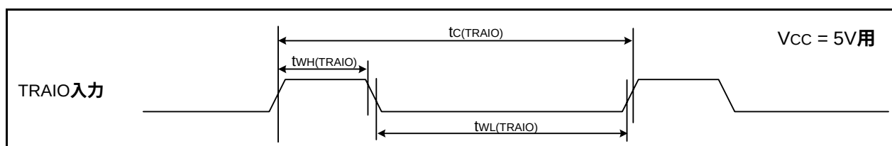
図31.32 VCC = 5V時のTRAIO入力タイミング
