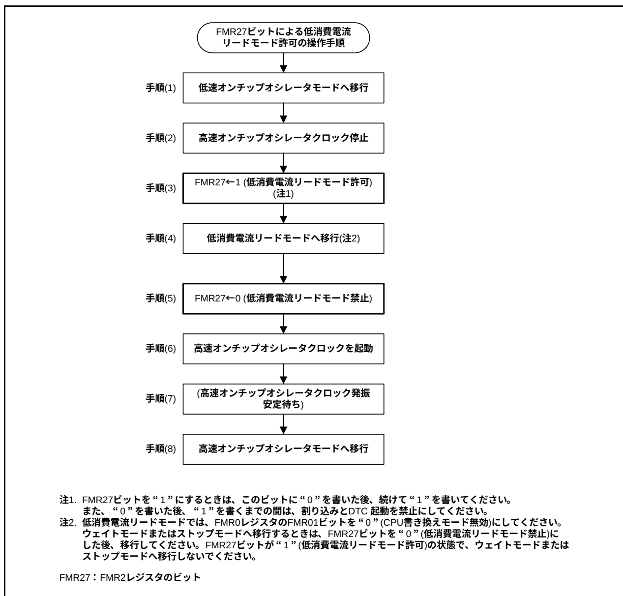
図30.3 低消費電流リードモードの操作手順例
