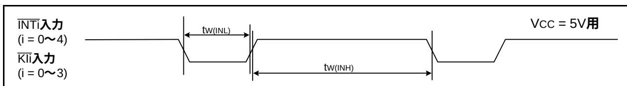
図31.34 VCC = 5V時の外部割り込み \overline{\text{INTi}} およびキー入力割り込み \overline{\text{Kli}} 入力タイミング
