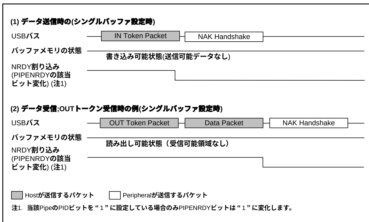
図26.7 NRDY割り込み発生タイミング図 (ファンクションコントローラ機能選択時)
