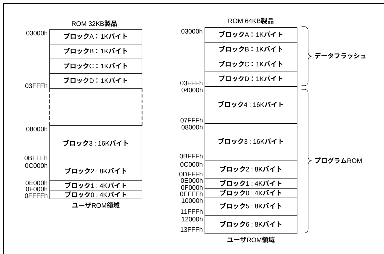
図29.1 R8C/3MUグループのフラッシュメモリのブロック図
