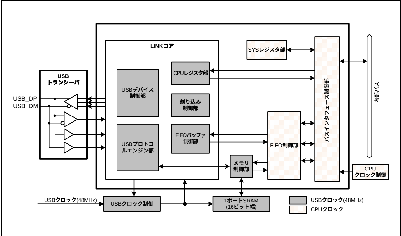
図 26.1 USBのブロック図
