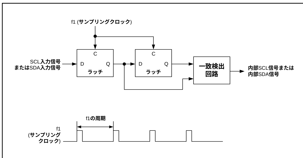
図 24.20 ノイズ除去回路のブロック図
