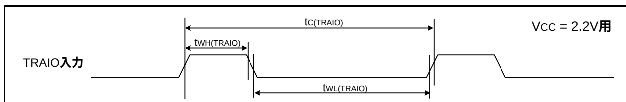
図 31.19 V_{CC} = 2.2V 時のTRAIO入力タイミング
