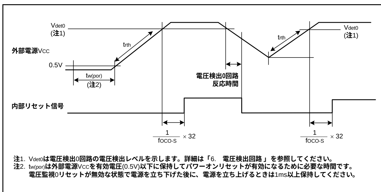
図31.26 パワーオンリセット回路の電気的特性
