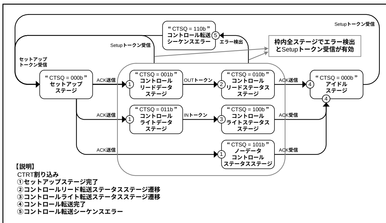
図26.10 コントロール転送ステージ遷移図
