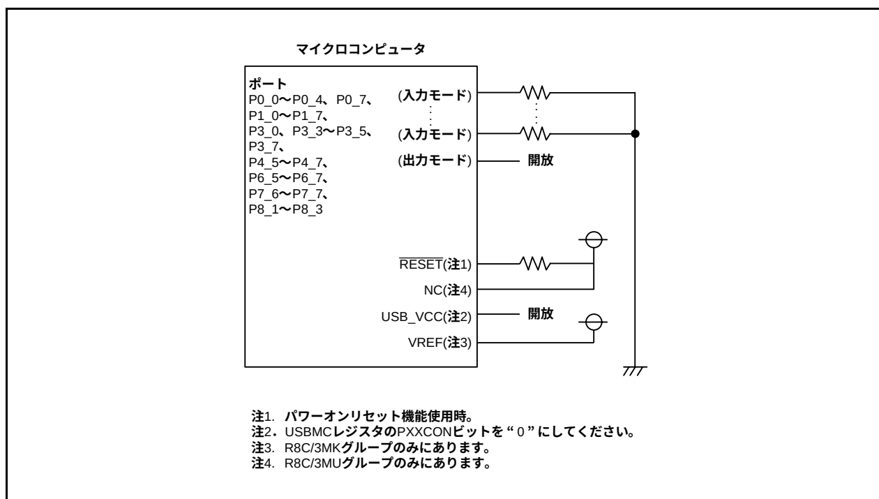
図7.16 未使用端子の処理例
