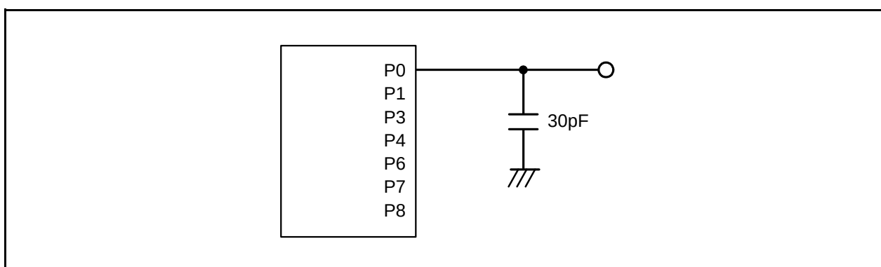
図31.1 ポートP0、P1、P3、P4、P6、P7、P8のタイミング測定回路
