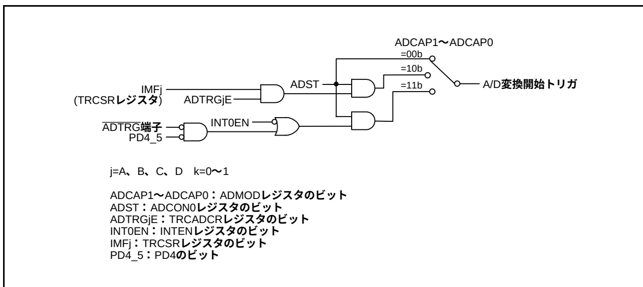
図27.4 A/D変換開始制御部のブロック図
