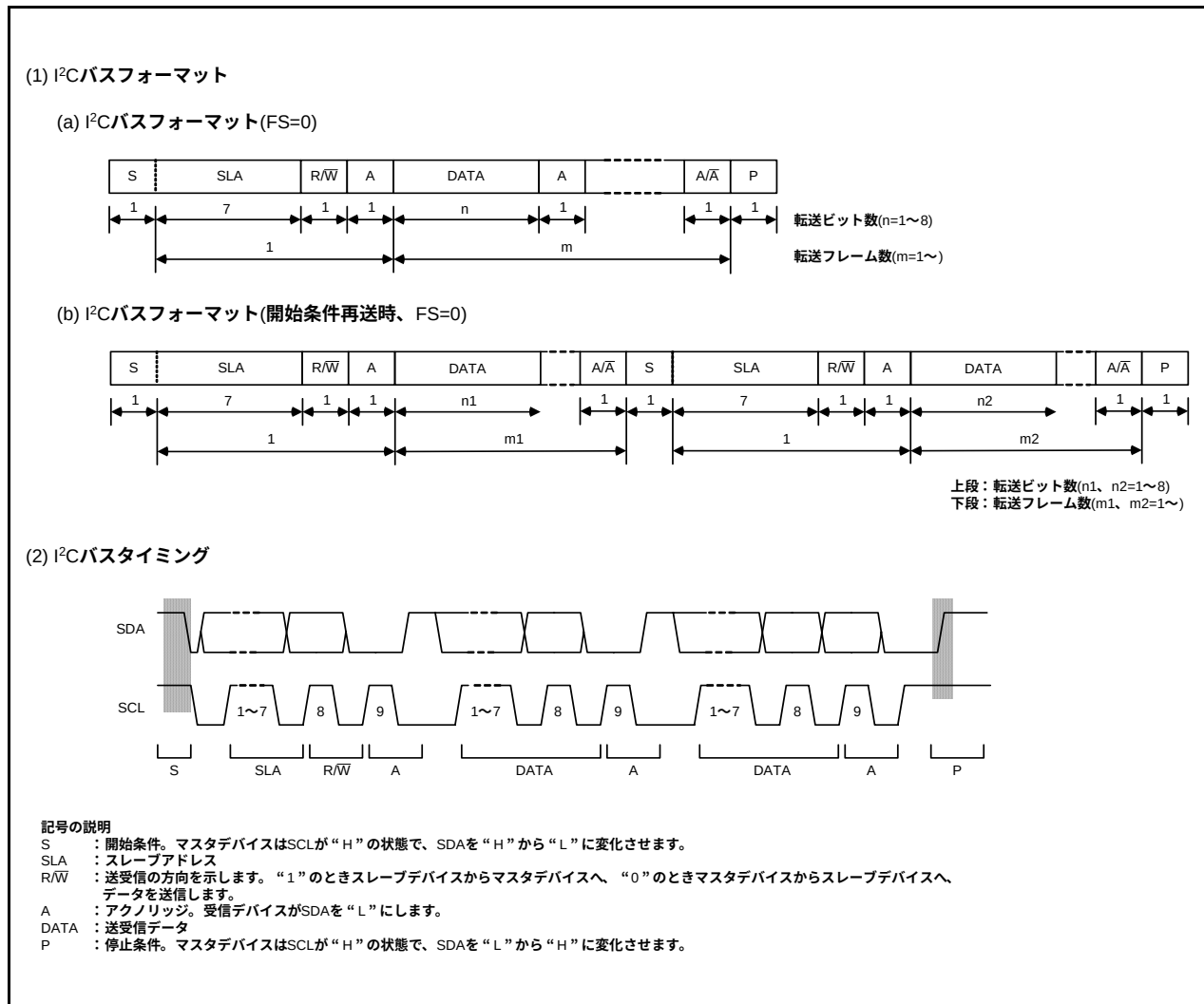
図24.4 I 2 Cバスフォーマットとバスタイミング
