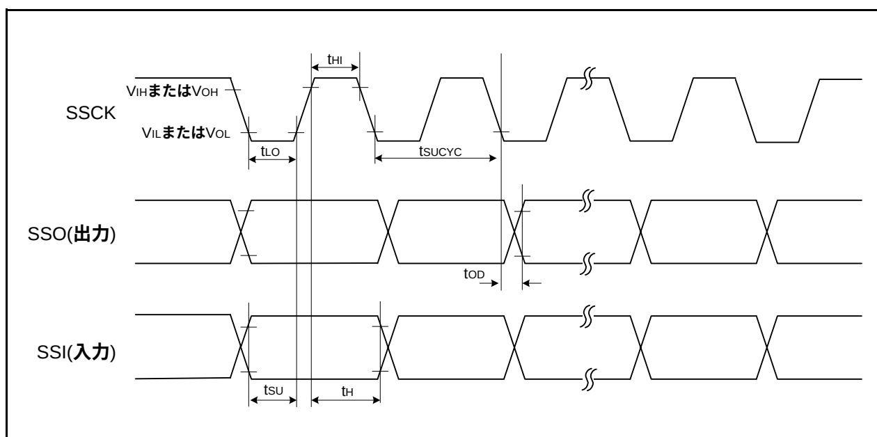
図 31.29 シンクロナスシリアルコミュニケーションユニット (SSU) の入出力タイミング (クロック同期式通信モード)
