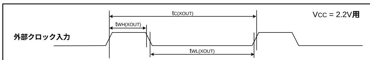
図 31.39 V_{CC} = 2.2V 時の外部クロック入力タイミング
