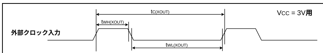
図31.35 V_{CC} = 3V 時の外部クロック入力タイミング
