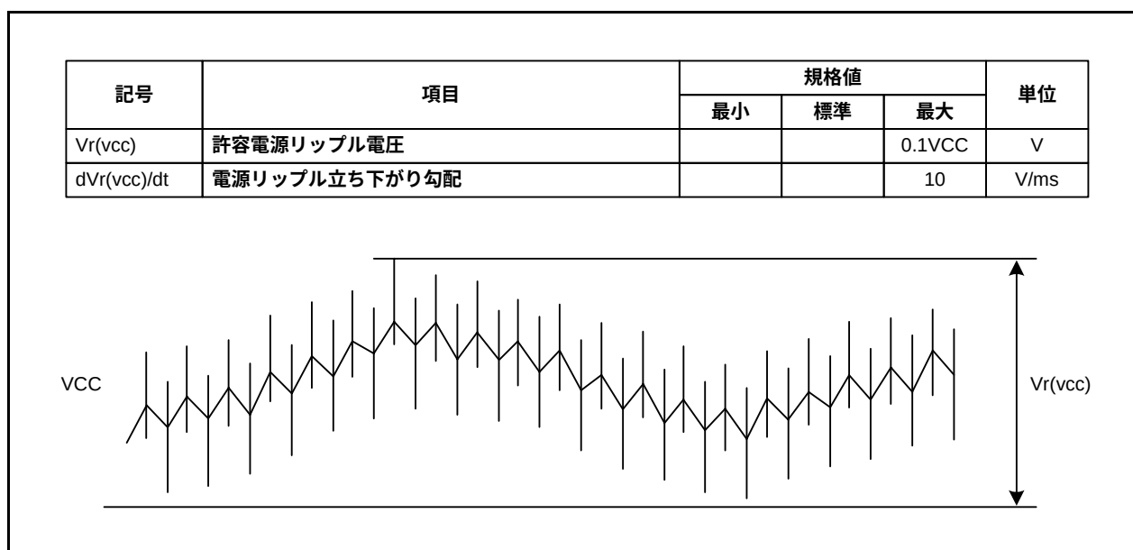
図32.2 電源リップルの定義
