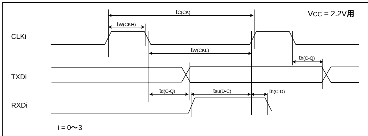
図31.20 V_{CC} = 2.2V 時のシリアルインタフェースのタイミング
