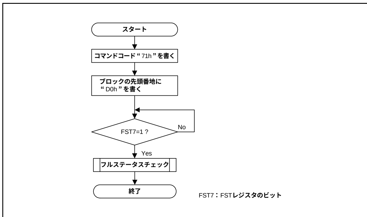
図29.15 リードロックビットステータスフローチャート
