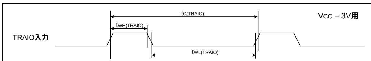
図31.36 V_{CC} = 3V 時のTRAIO入力タイミング
