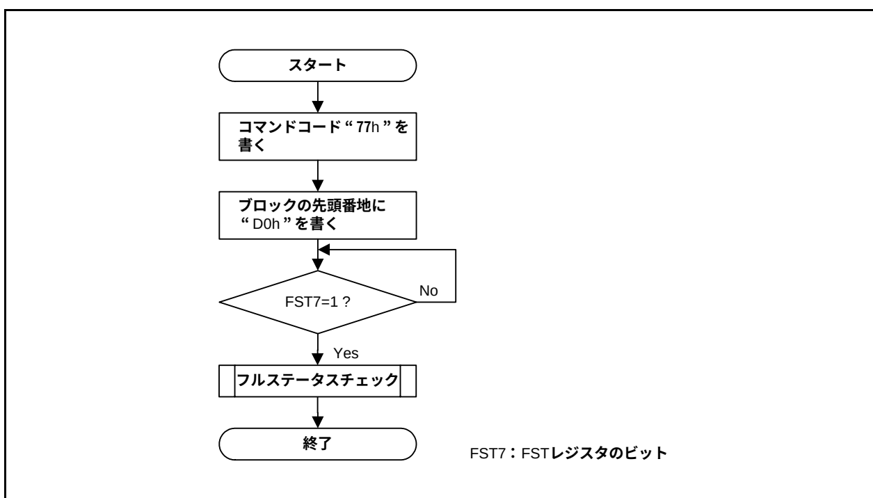
図29.14 ロックビットプログラムフローチャート
