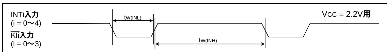
図31.21 V_{CC} = 2.2V 時の外部割り込み \overline{INTi} およびキー入力割り込み \overline{Kli} 入力タイミング
