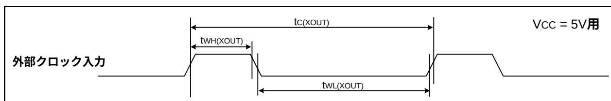
図31.31 VCC = 5V時の外部クロック入力タイミング
