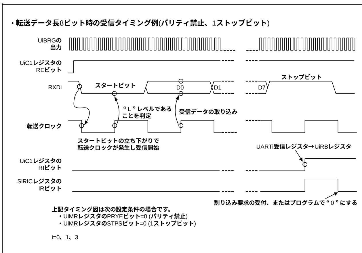
図 20.7 UART モード時の受信タイミング例
