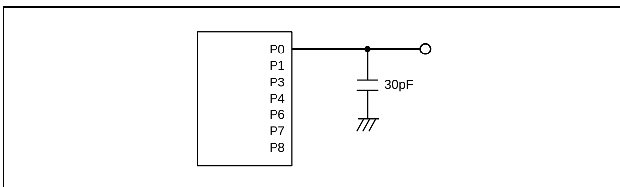
図31.22 ポートP0、P1、P3、P4、P6、P7、P8のタイミング測定回路
