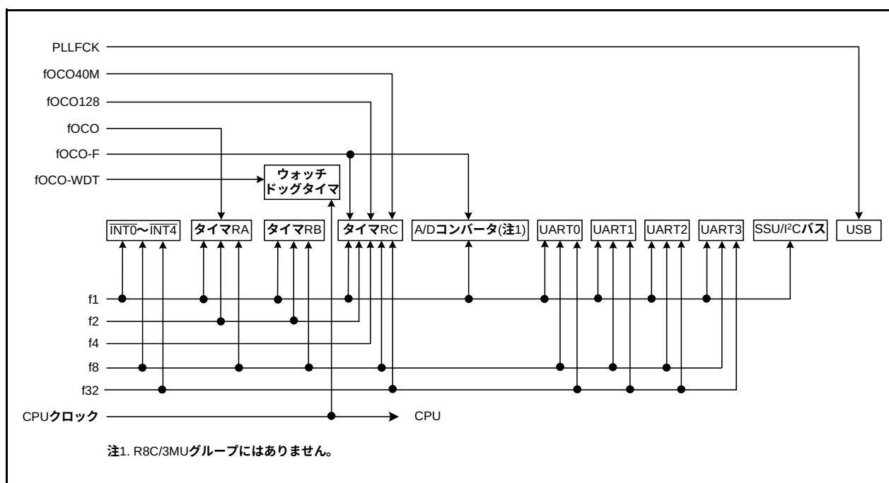
図9.2 周辺機能のクロック
