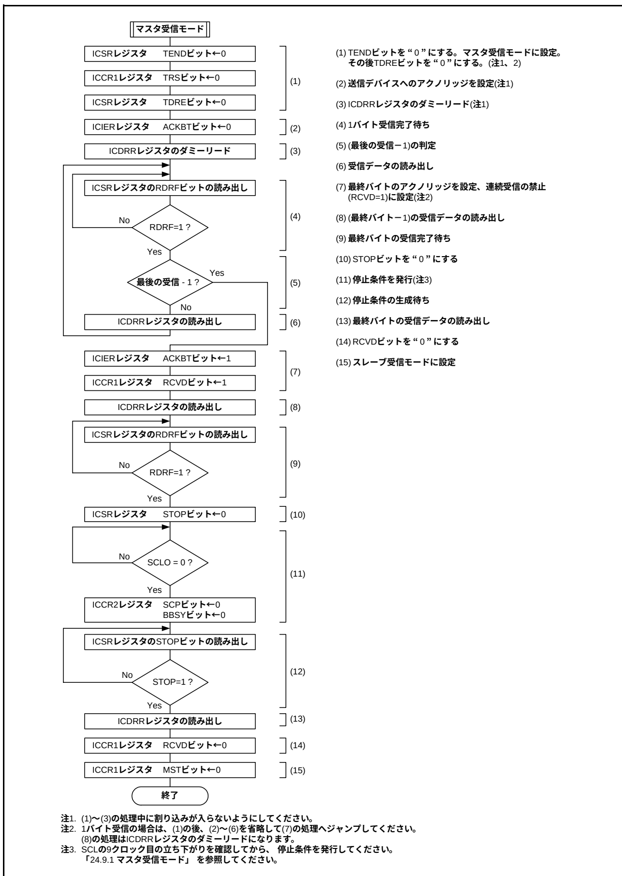
図 24.17 マスタ受信モードのレジスタ設定例(I 2 Cバスイインタフェースモード)
