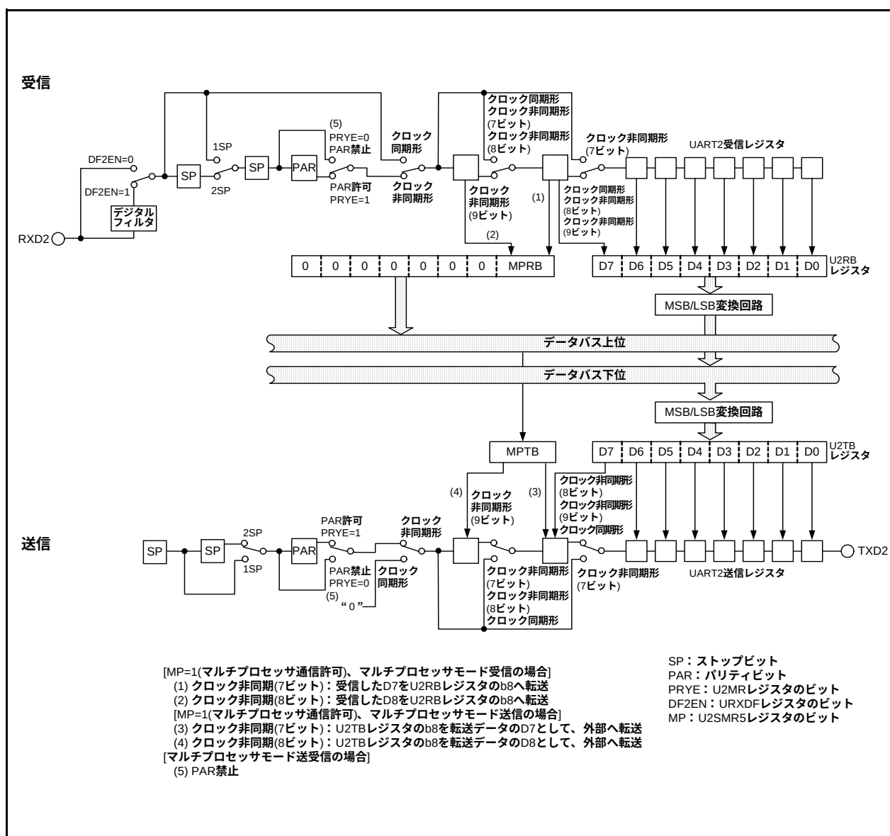
図 21.14 マルチプロセッサ通信機能のブロック図
