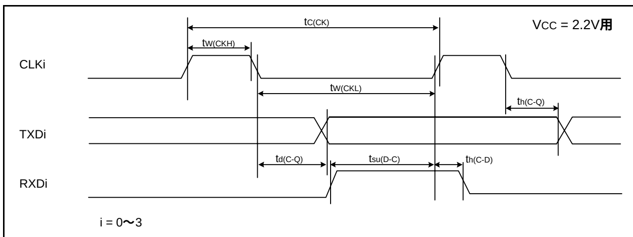
図31.41 VCC = 2.2V時のシリアルインタフェースのタイミング
