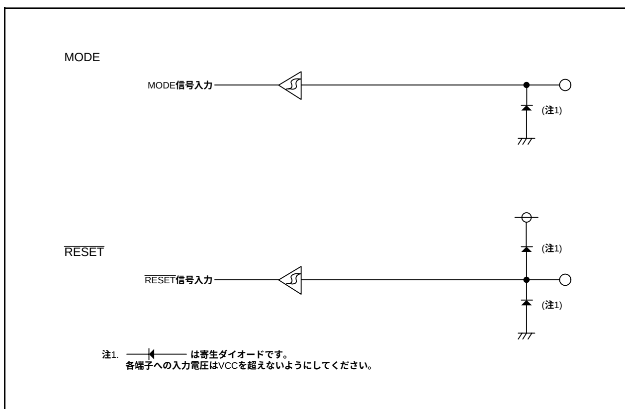
図 7.15 端子の構成
