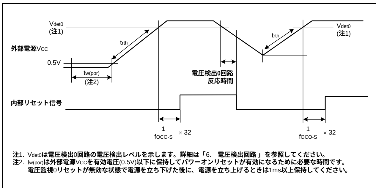
図31.5 パワーオンリセット回路の電気的特性
