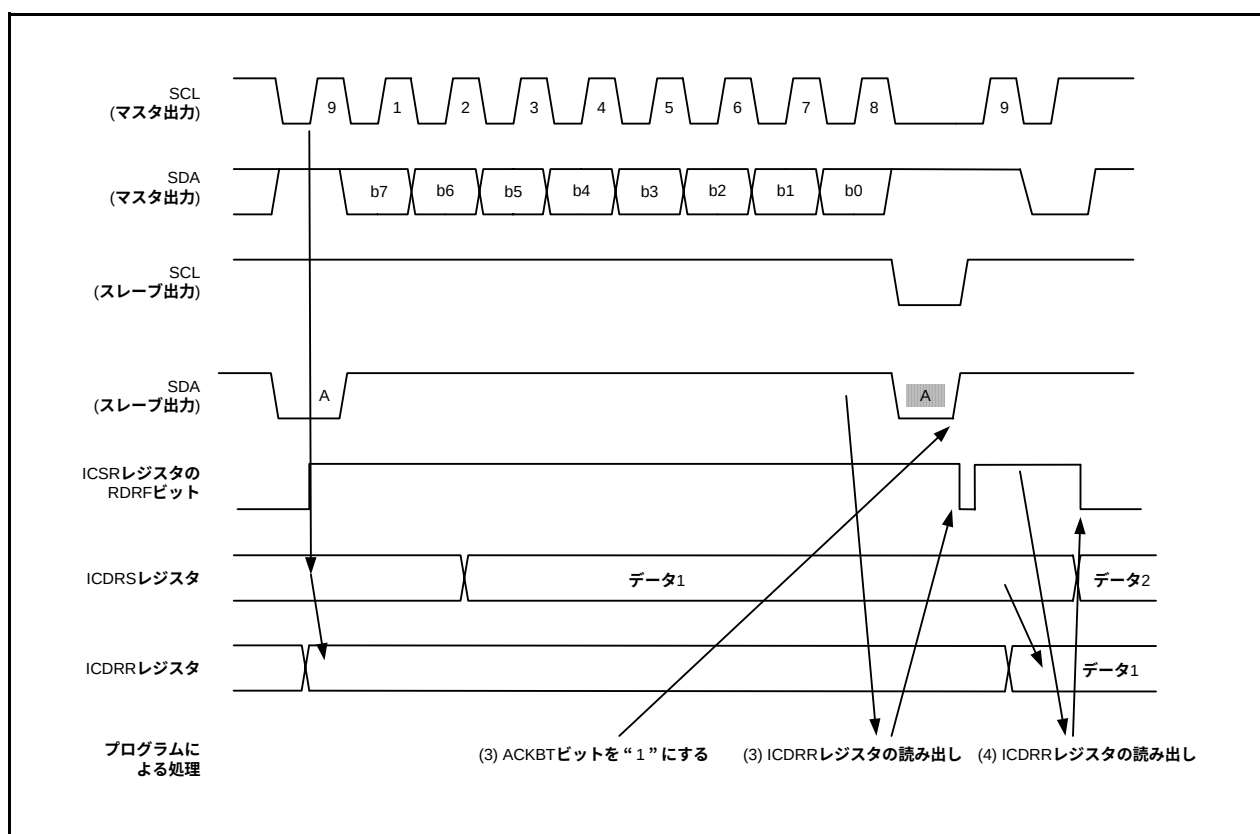
図 24.12 スレーブ受信モードの動作タイミング (I 2 C バスインタフェースモード) (2)
