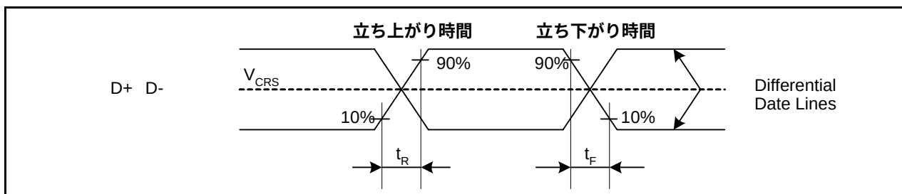
図31.23 データ信号タイミング
