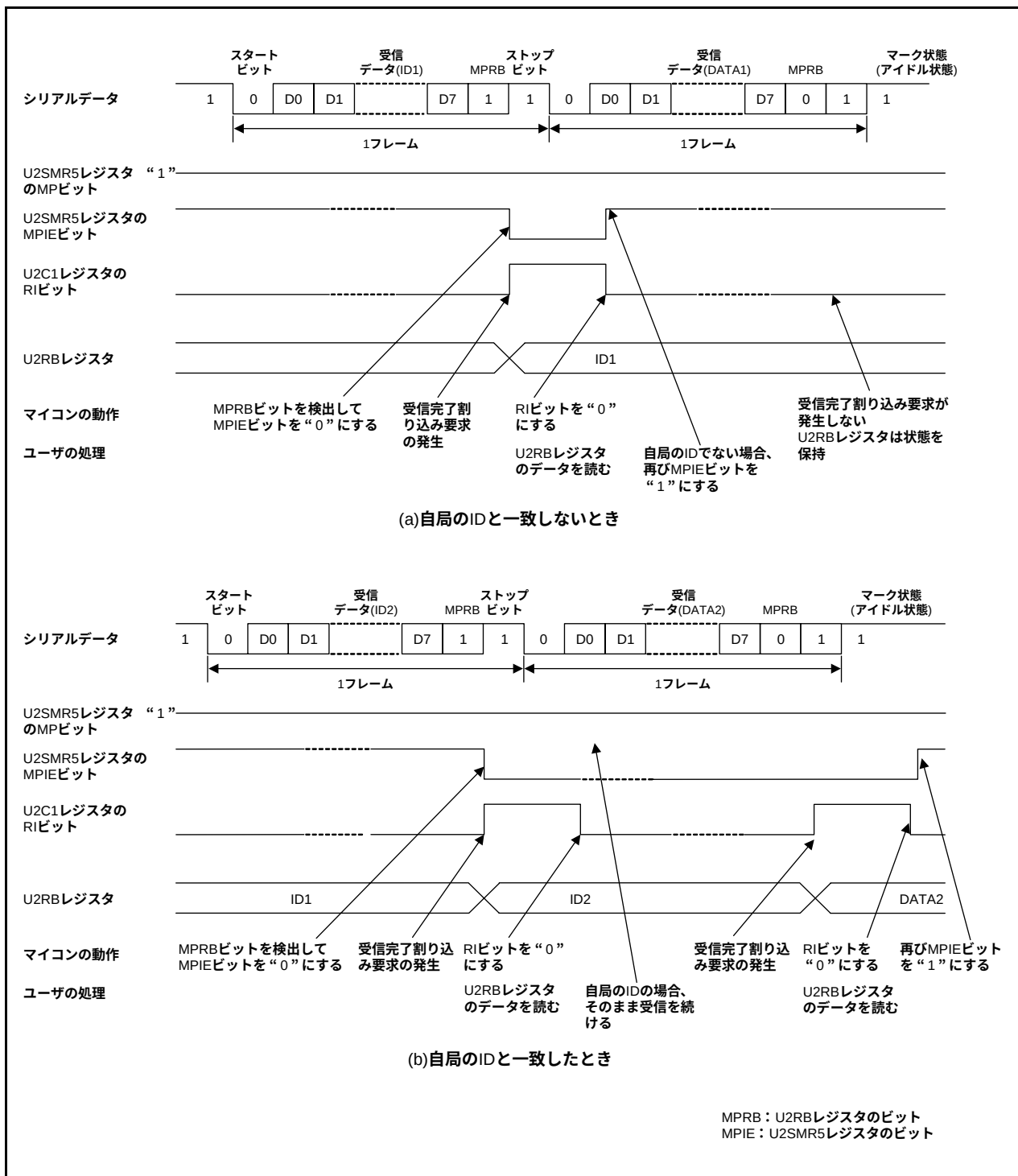
図 21.17 マルチプロセッサ通信の受信時の動作例(8ビットデータ/マルチプロセッサビットあり/1ビットストップビットの例)
