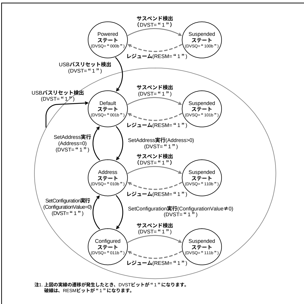
図 26.9 デバイスステート遷移図
