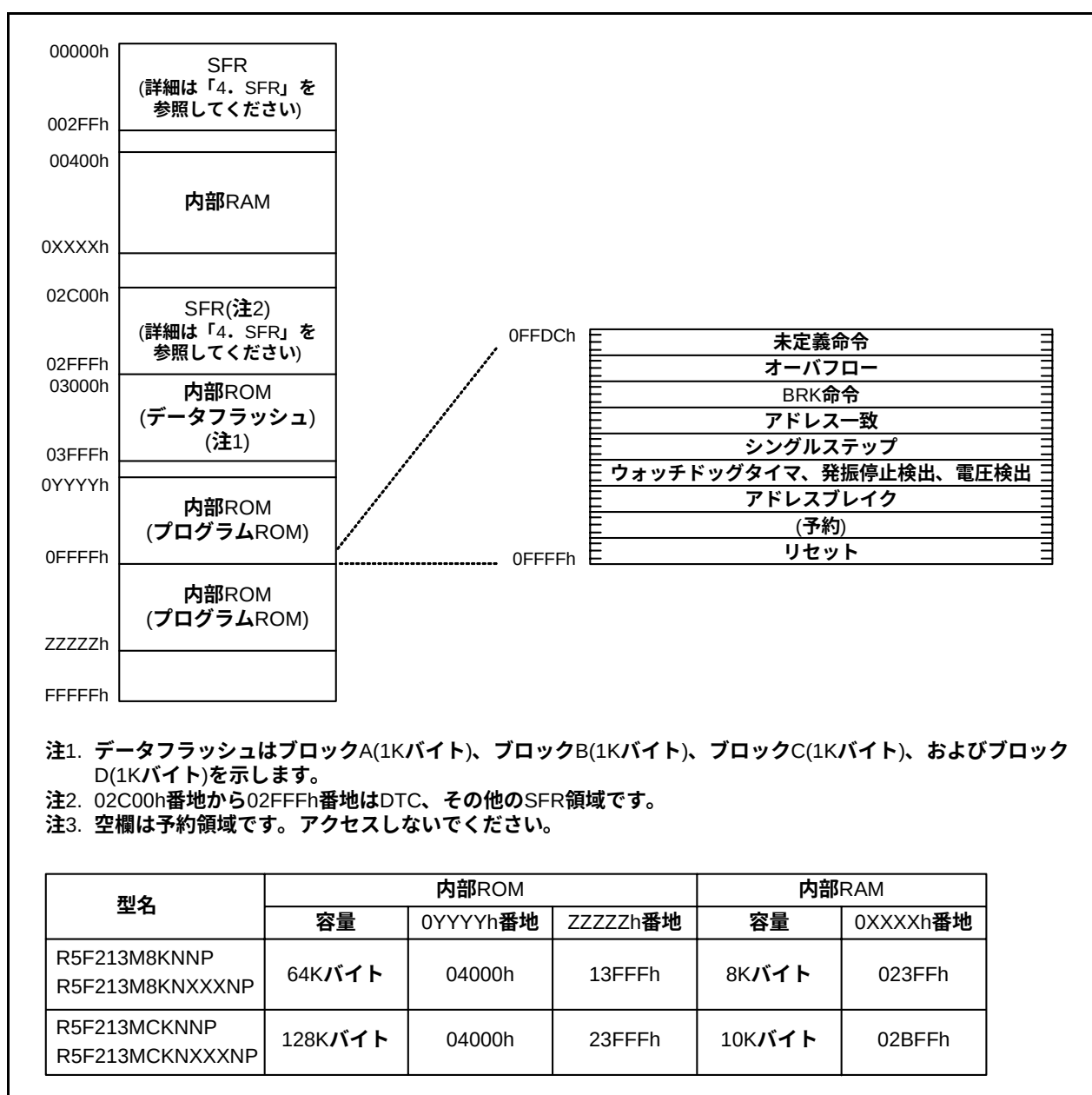
図3.2 R8C/3MKグループのメモリ配置図
