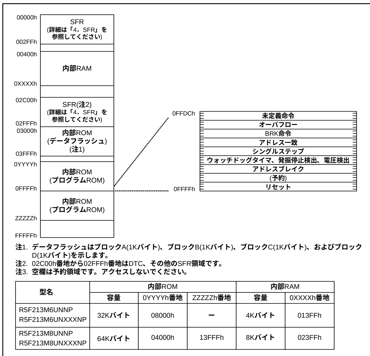
図3.1 R8C/3MUグループのメモリ配置図
