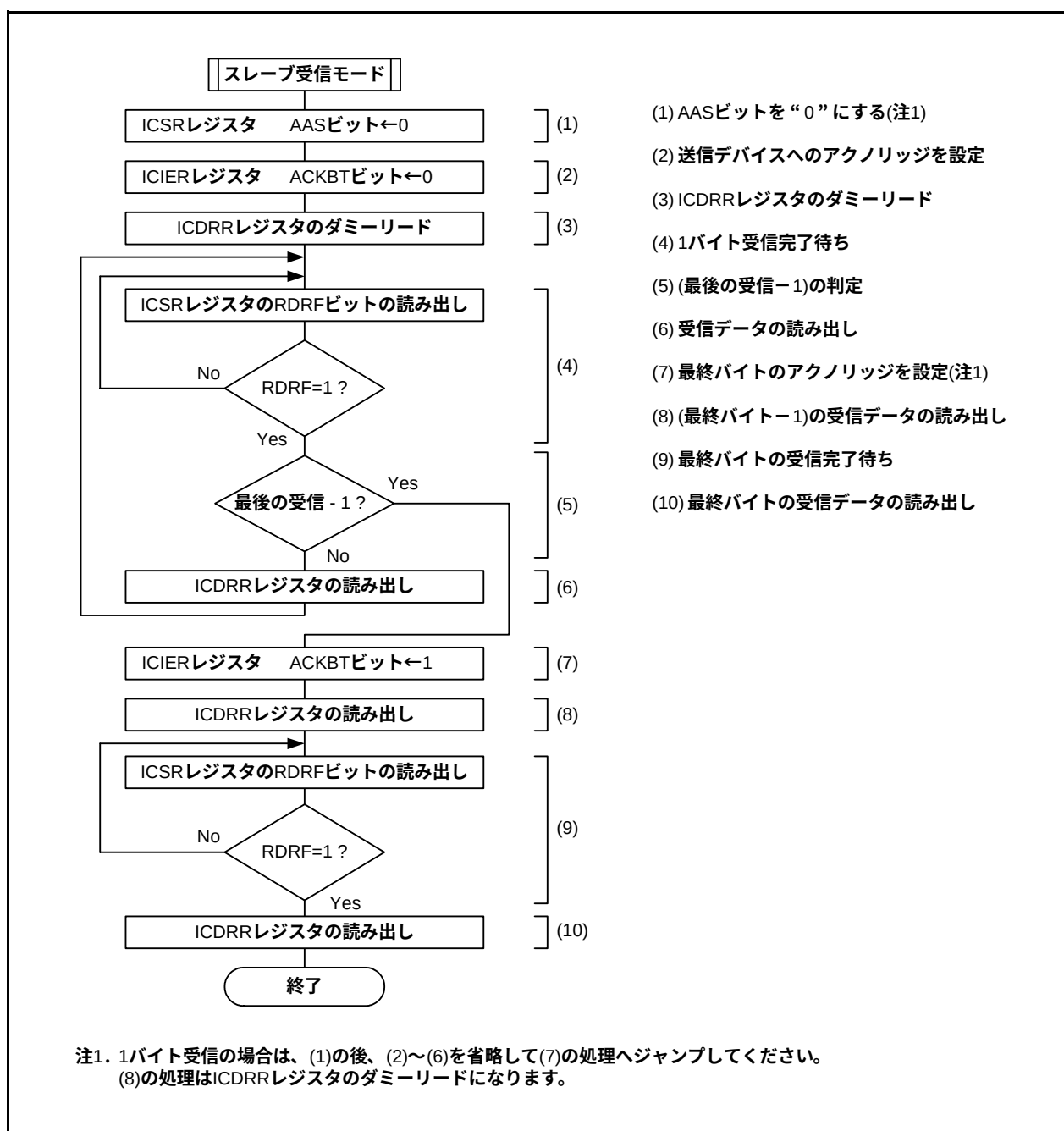
図 24.19 スレープ受信モードのレジスタ設定例(I 2 Cバスインタフェースモード)
