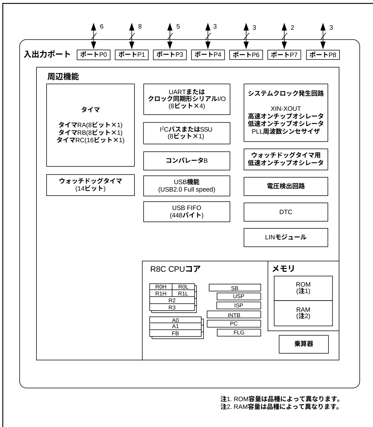
図1.3 R8C/3MUグループのブロック図
